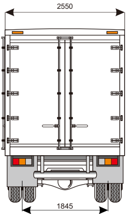
TAMPAK DEPAN
