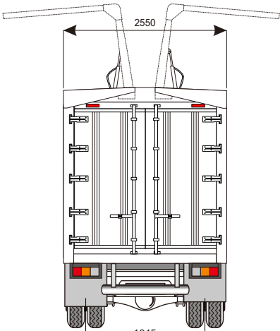
TAMPAK DEPAN
