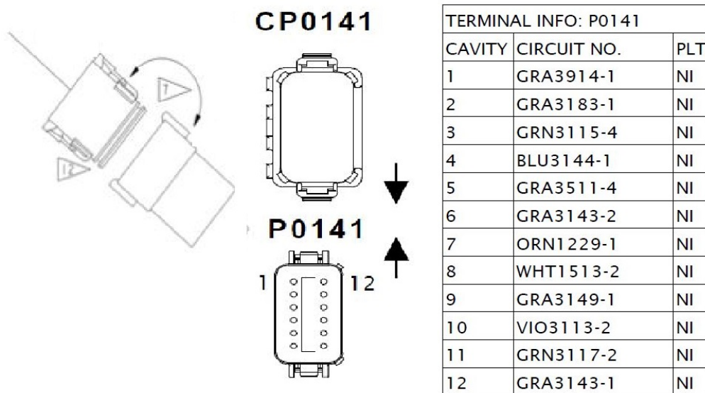
FIGURE 6-26. PACCAR PX-7 &amp; PX-9.
