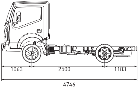
2500 mm EINZELKABINE
