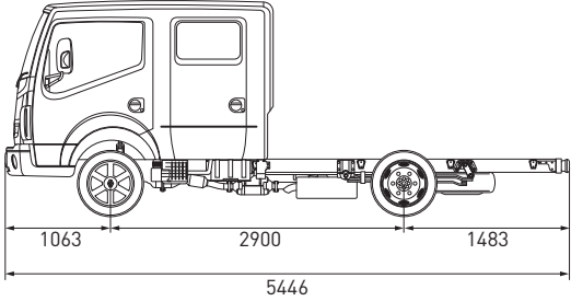
2900 mm DOPPELKABINE
