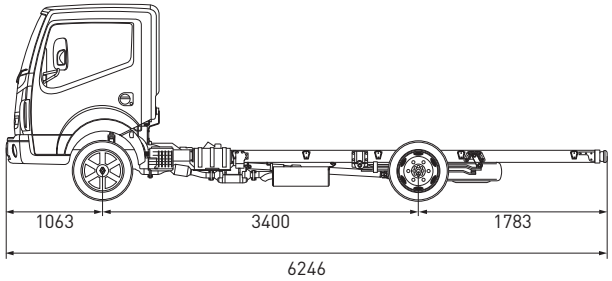
3400 mm EINZELKABINE
