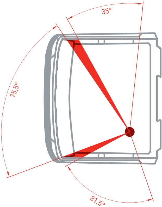
DER 192°-SICHTWINKEL bietet hervorragende Sicht in Stadtgebieten mit starkem Verkehr.
