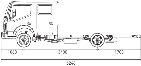
3400 mm DOPPELKABINE
