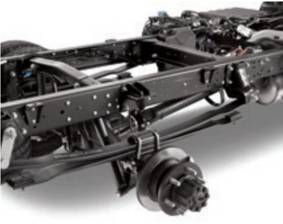
VERSTÄRKTE HINTERACHSFEDERUNG der 3,5 t- bis 4,5 t-Versionen für hohe Anforderungen (Bau- und Müllfahrzeuge).
