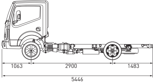
2900 mm EINZELKABINE
