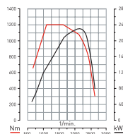
DTI 8 - 320 PS
