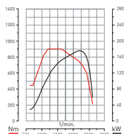
DTI 5 - 240 PS
