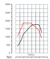
DTI 11 - 380 PS
