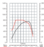
DTI 5 - 210 PS
