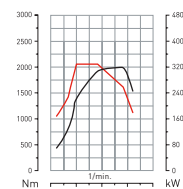
DTI 11 - 430 PS
