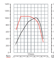
DTI 8 - 280 PS
