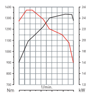
NGT 9 - 320 PS
