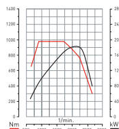
DTI 8 - 250 PS
