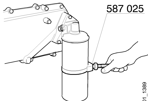
Remoção do filtro de óleo
