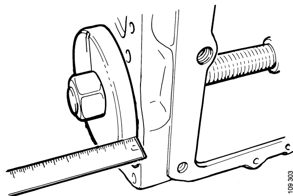
Medição de controle do mancal 1.
