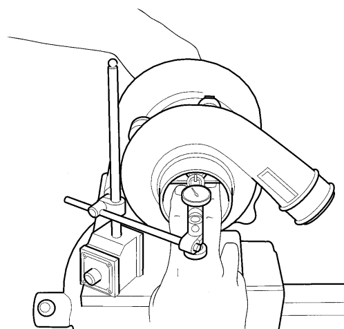
Medição da folga radial do rotor do compressor
