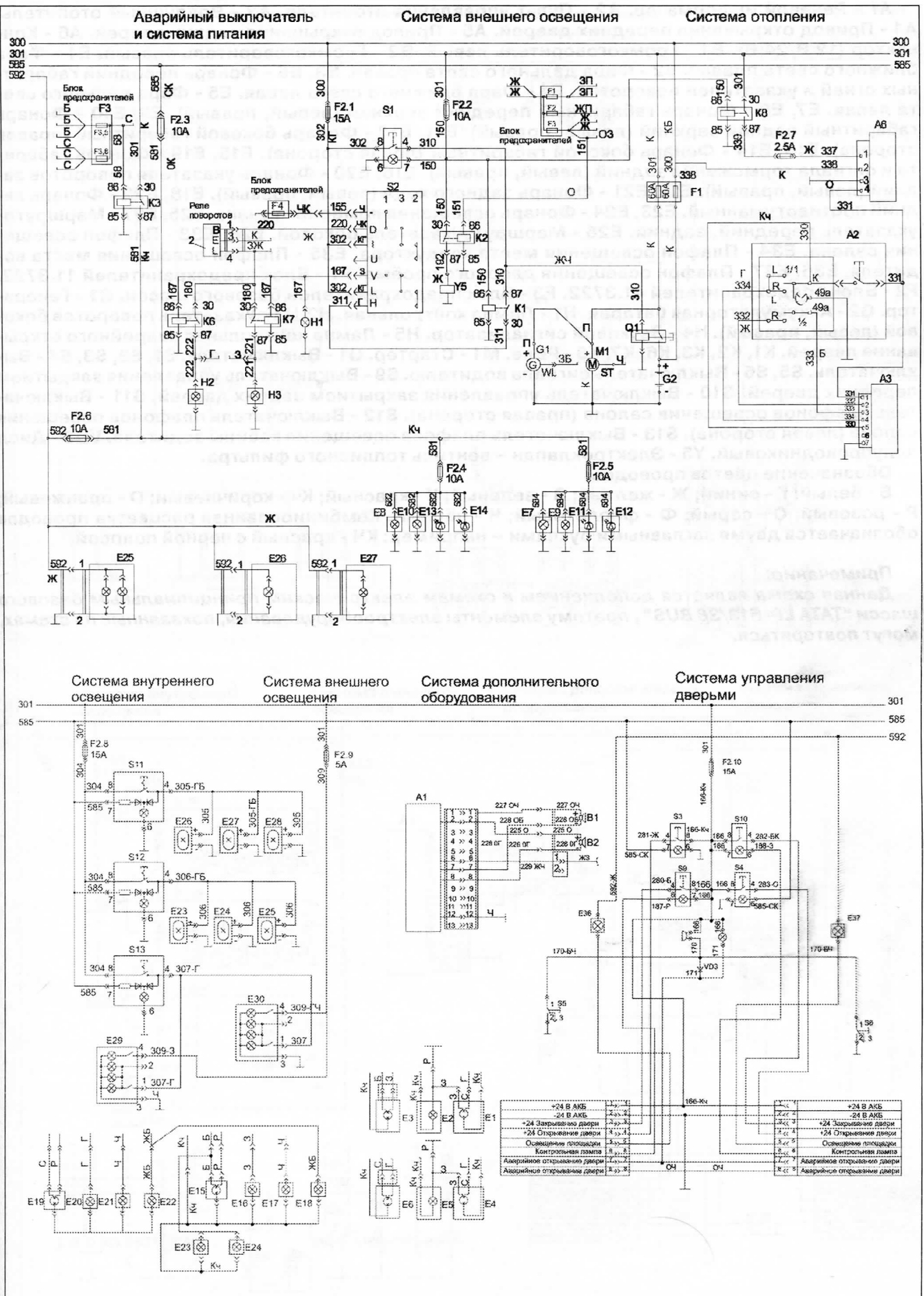
Принципиальная схема электрооборудования автобуса А07А1 с напряжением бортовой сети 12 В
