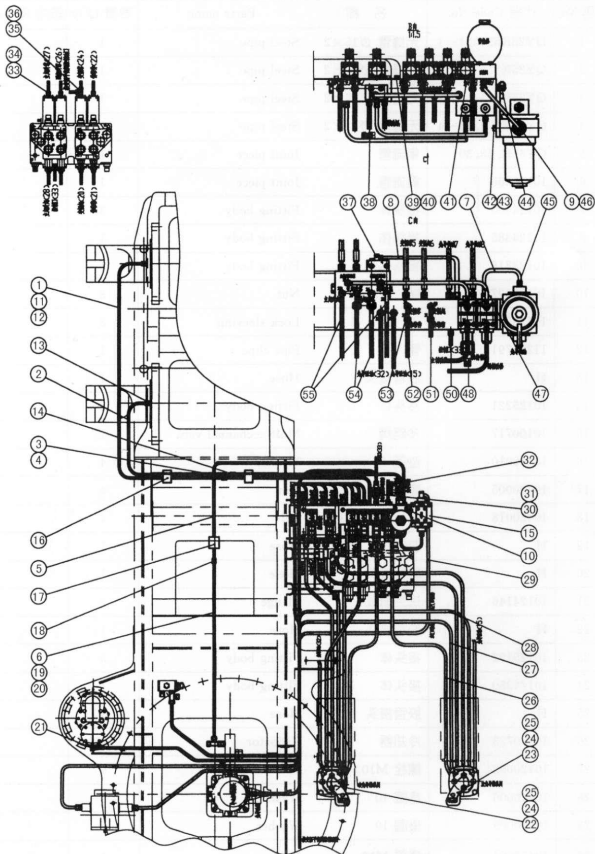
QY25K5. 13.2 先导控制管路配管 Guide Control's Piping Plan
