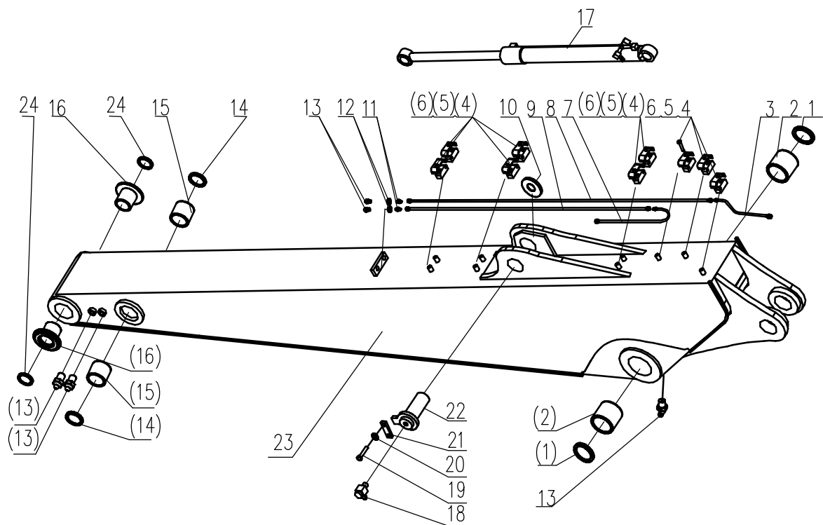
斗杆总成 ARM ASS'Y
