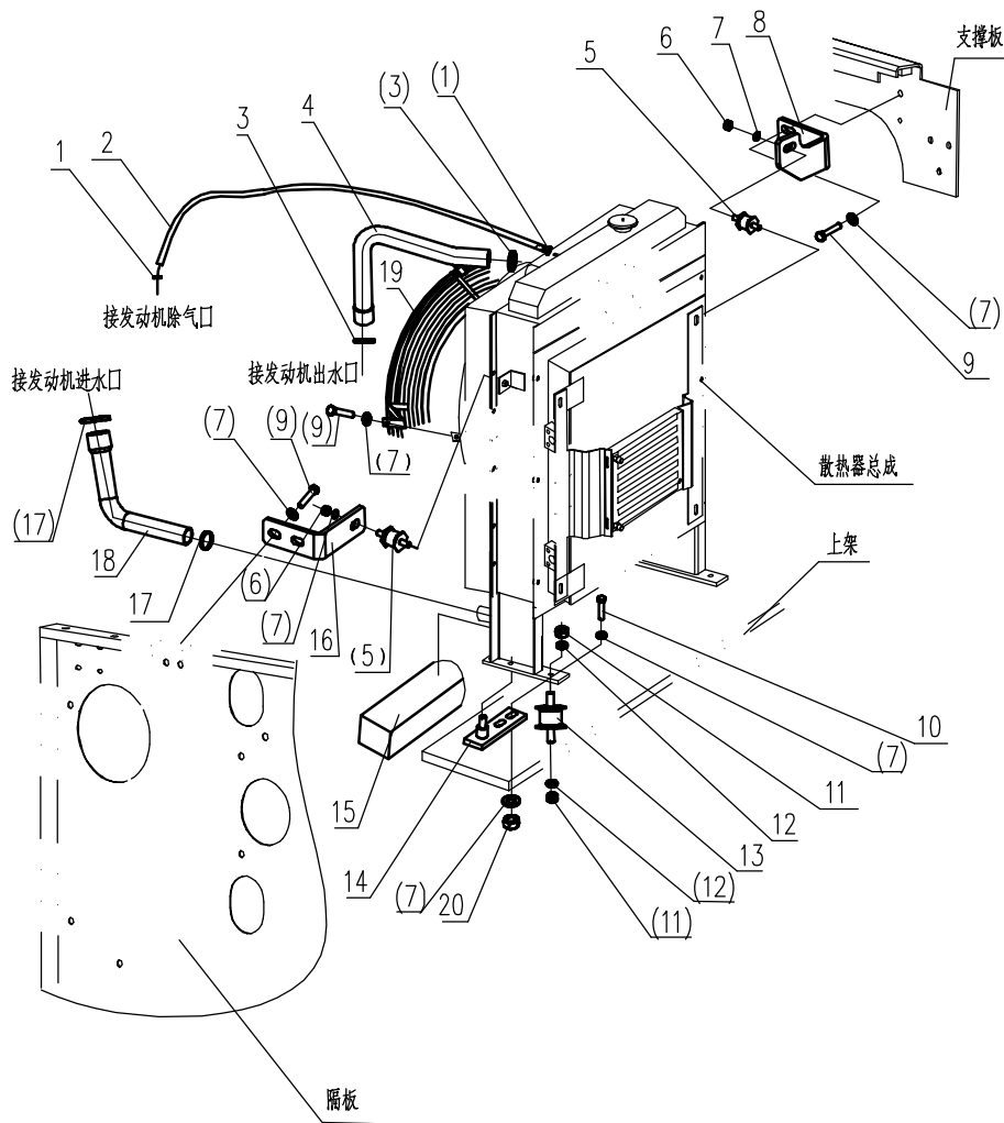
水箱 左侧门安装 2
