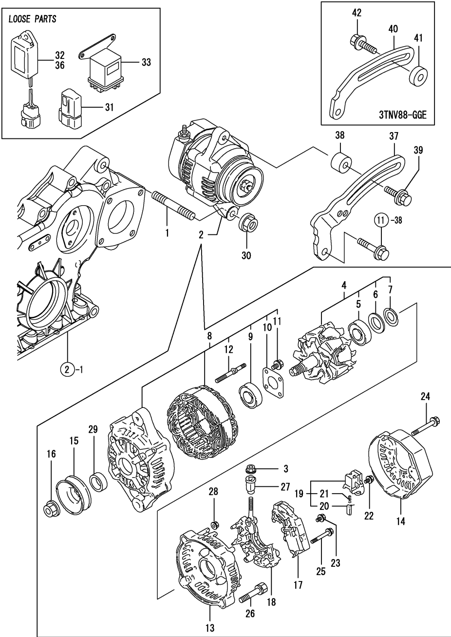
Fig.17. GENERATOR
