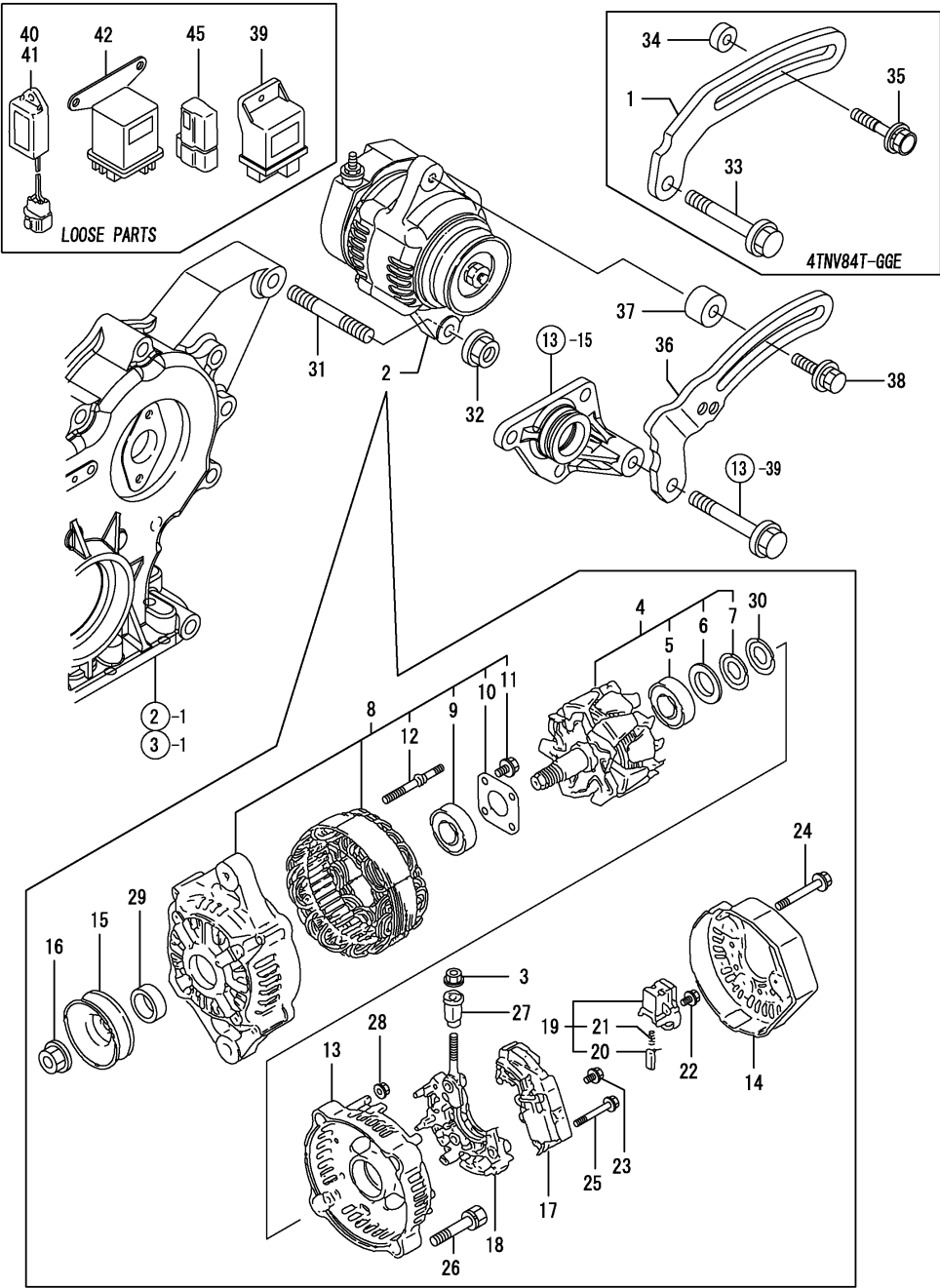
Fig.21. GENERATOR
