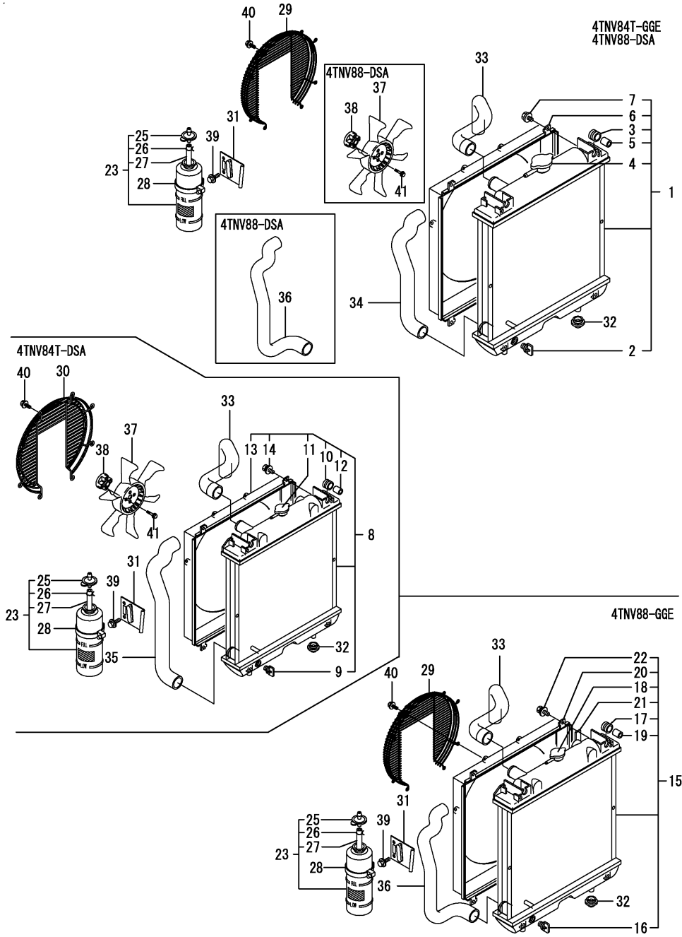
Fig.7. RADIATOR
