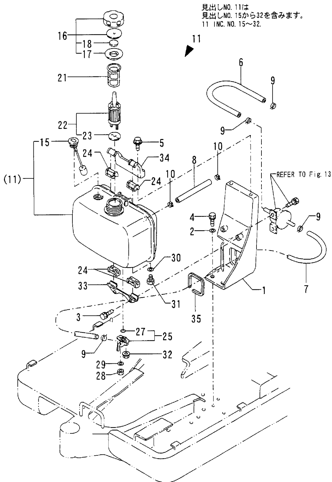
Fig. 11 燃料タンク & 燃料パイプ FUEL TANK & FUEL LINE
