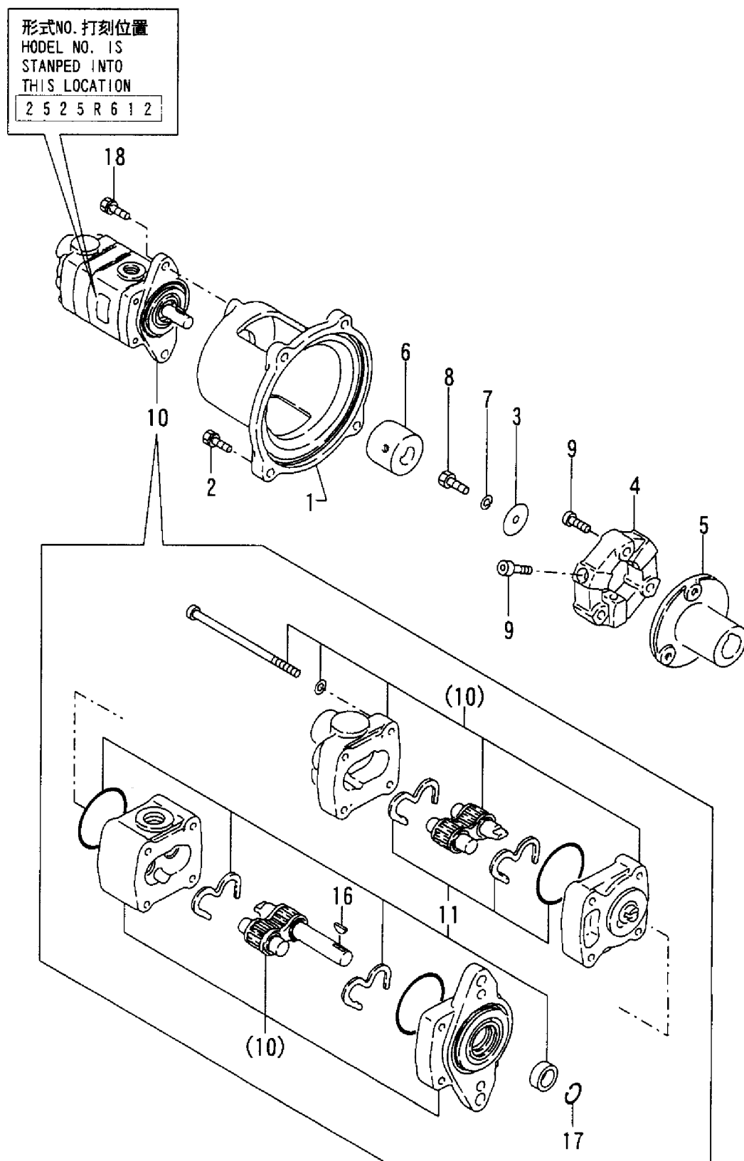
Fig. 25 油圧ポンプ & 軸継手 HYD. OIL PUMP & JOINT
