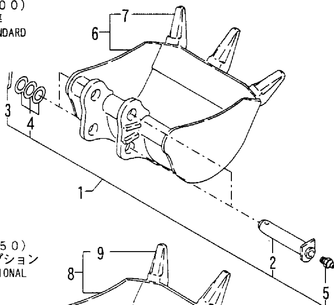
Fig. 49 バケット BUCKET
