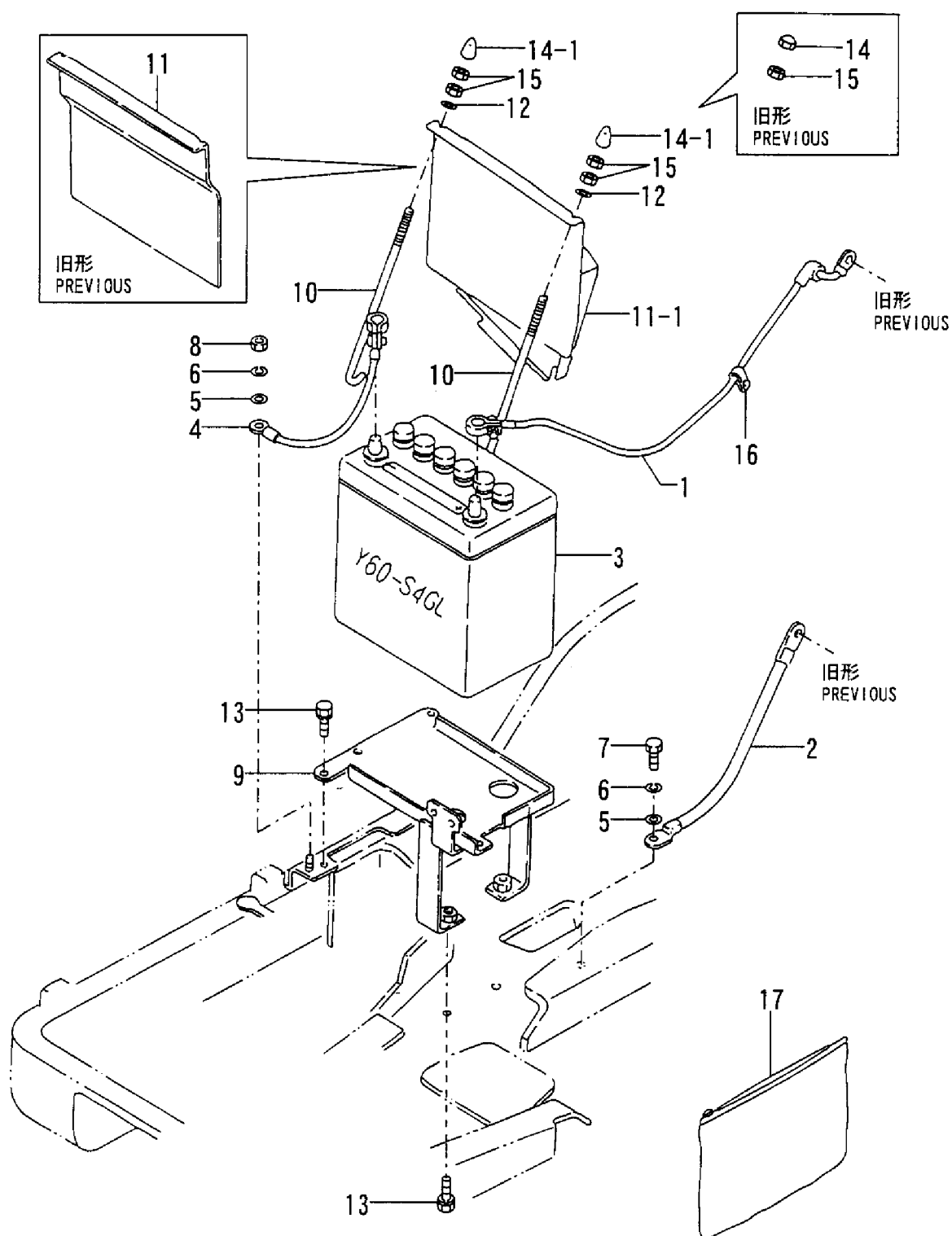
Fig. 12 バッテリー BATTERY
