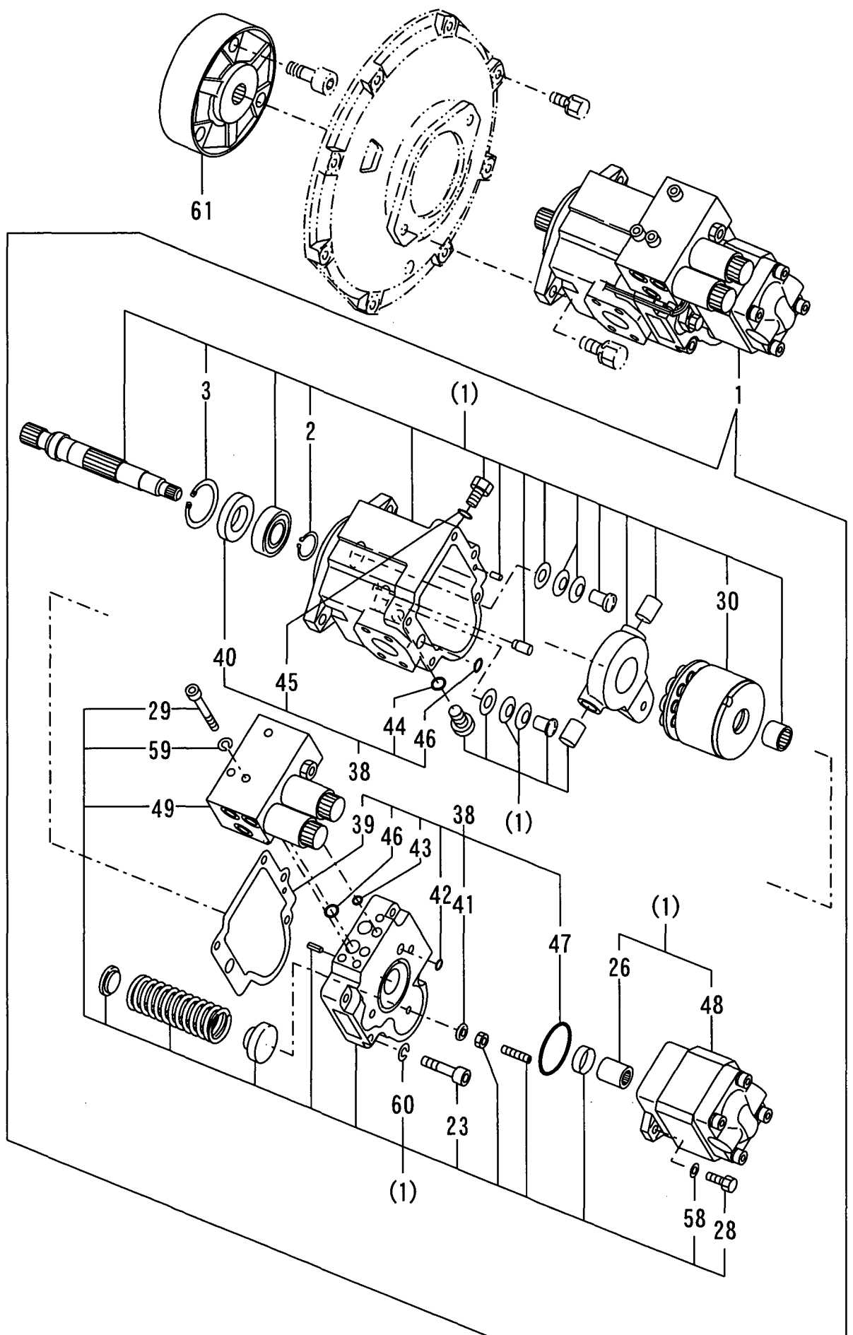
Fig. 3 HYD. OIL PUMP & JOINT https://truckmanuals.ru/sub.com/
