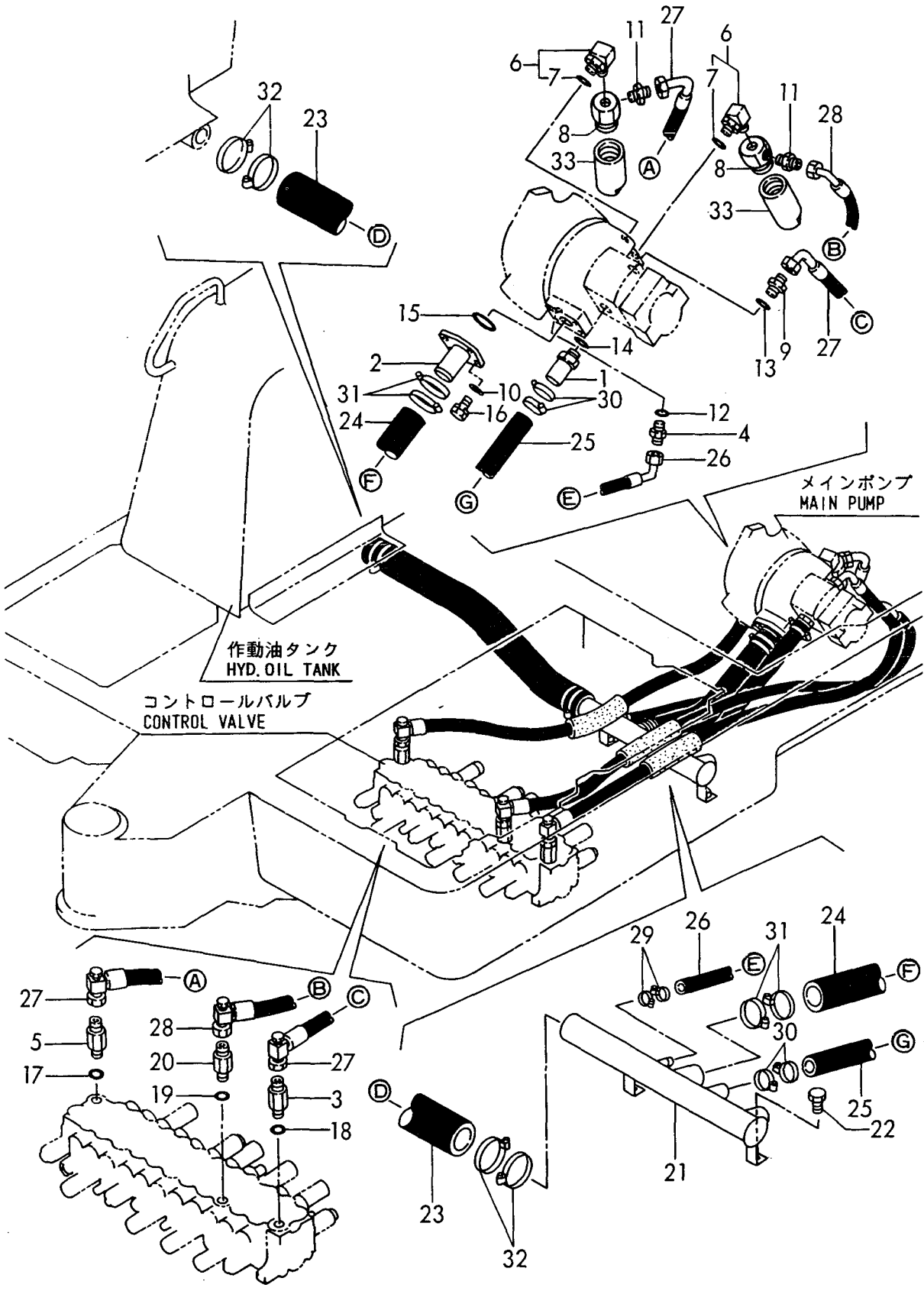
https://truckmanualshub.com/ Fig. 50 油圧配管(タンク〜ポンプ〜バルブ) HYD. OIL PIPING(TANK~PUMP~VALVE)
