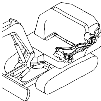
Fig. 51 油圧配管 (バルブ〜モータ、ブーム) HYD. OIL PIPING (VALVE~MOTOR, BOOM)
