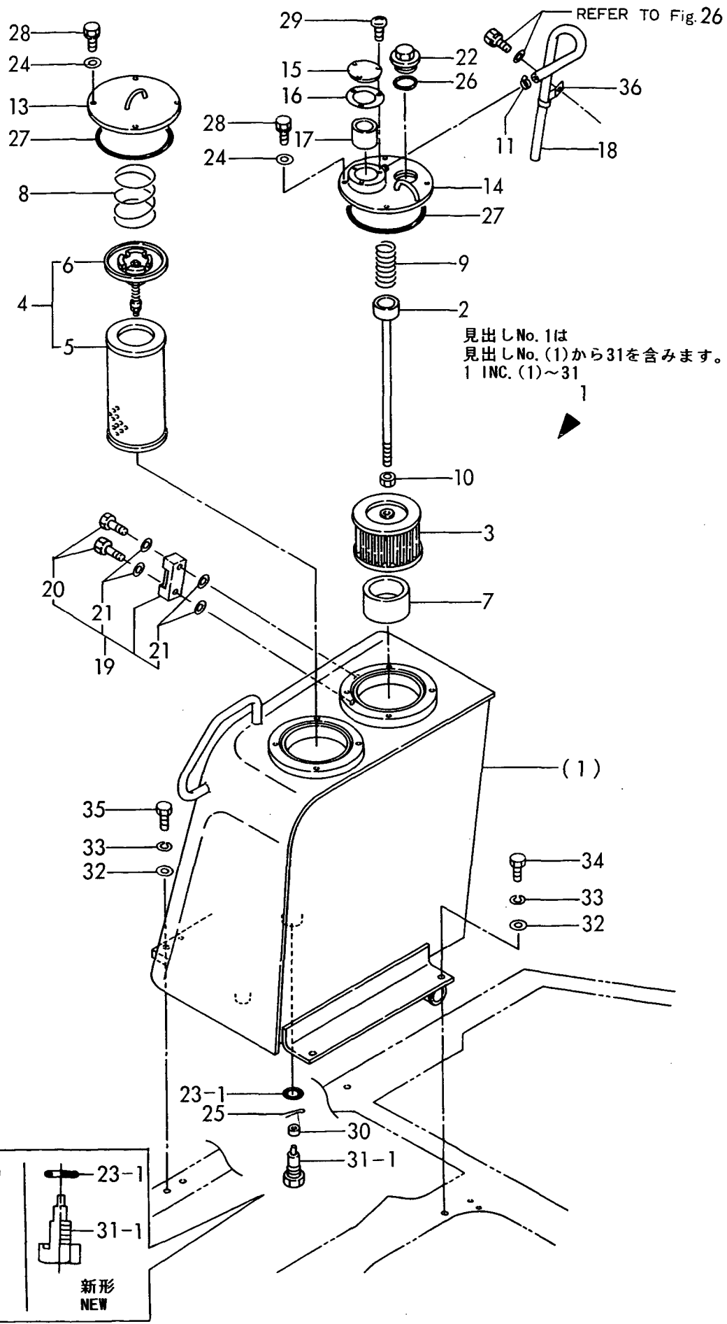
Fig. 49 作動油タンク HYD. OIL TANK
