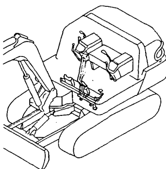
Fig.18 操縦装置(スイング) CONTROL EQUIPMENT(SWING)
