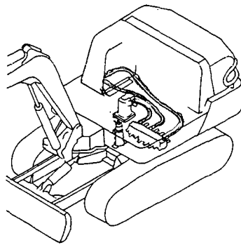
Fig. 54 P. T. O. 油圧配管(フレーム) P. T. O. HYD. OIL PIPING (FRAME)
