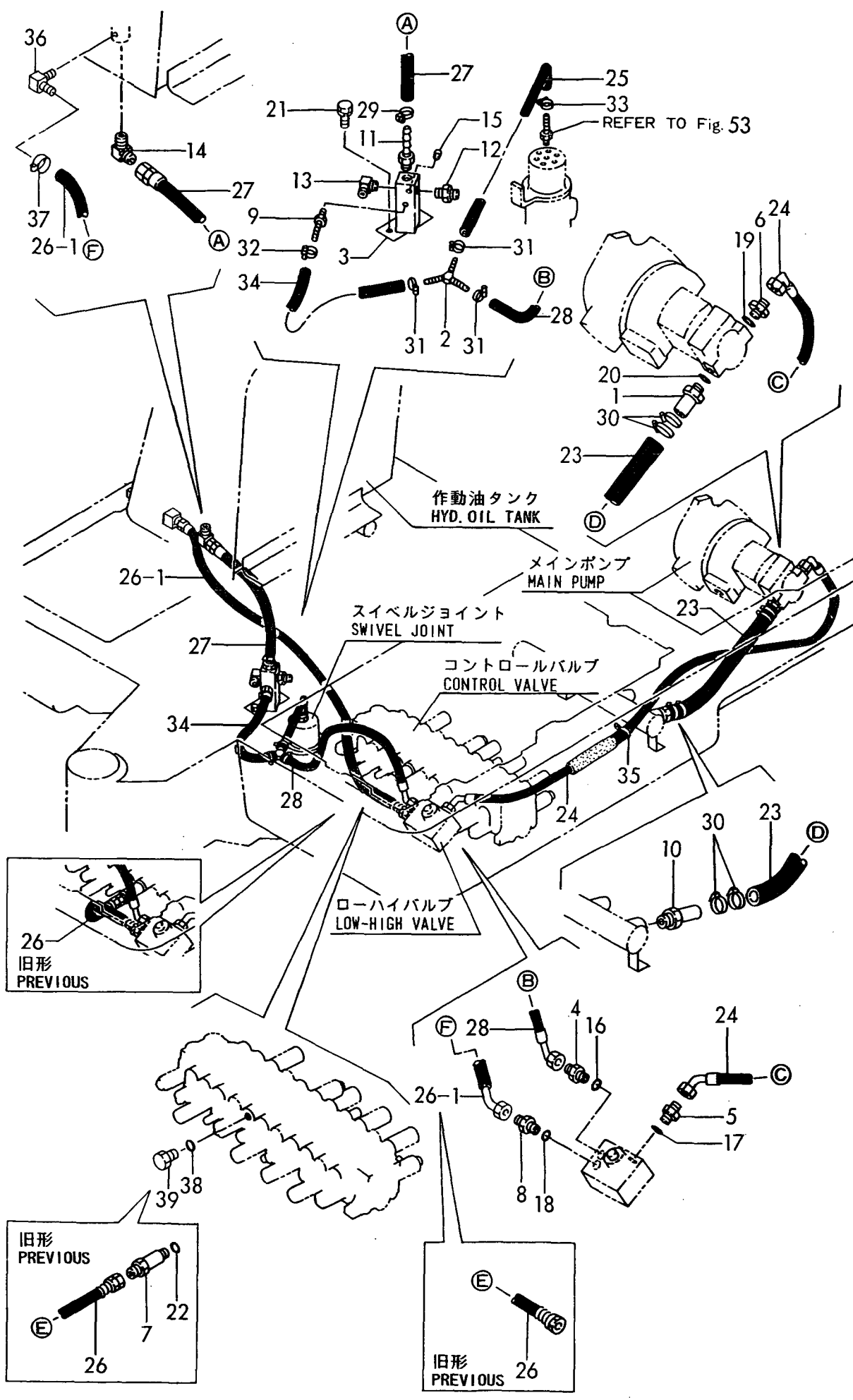
58 コントロール配管(ポンプ～ローハイルブ～リターン) Fig. 58 CONTROL PIPING(PUMP～LOW-HIGH VALVE～RETURN)
