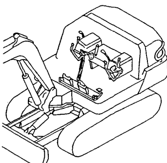
Fig.20 操縦装置 (カットオフレバー & ペダル) CONTROL EQUIP. (CUT-OFF LEVER & LOW-HIGH PEDAL)
