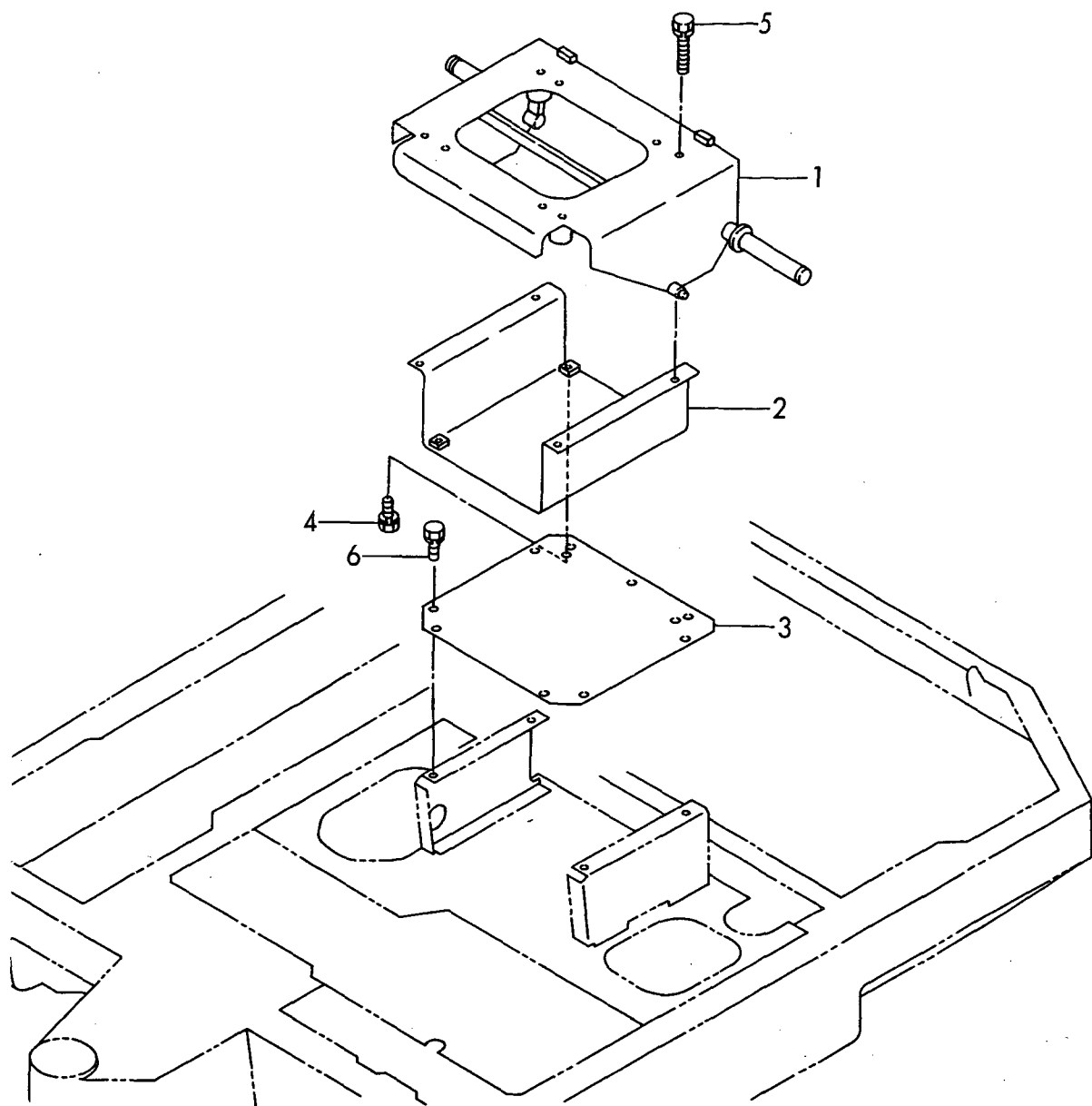
Fig. 25 シートマウント SEAT MOUNT https://truckmanualshub.com/
