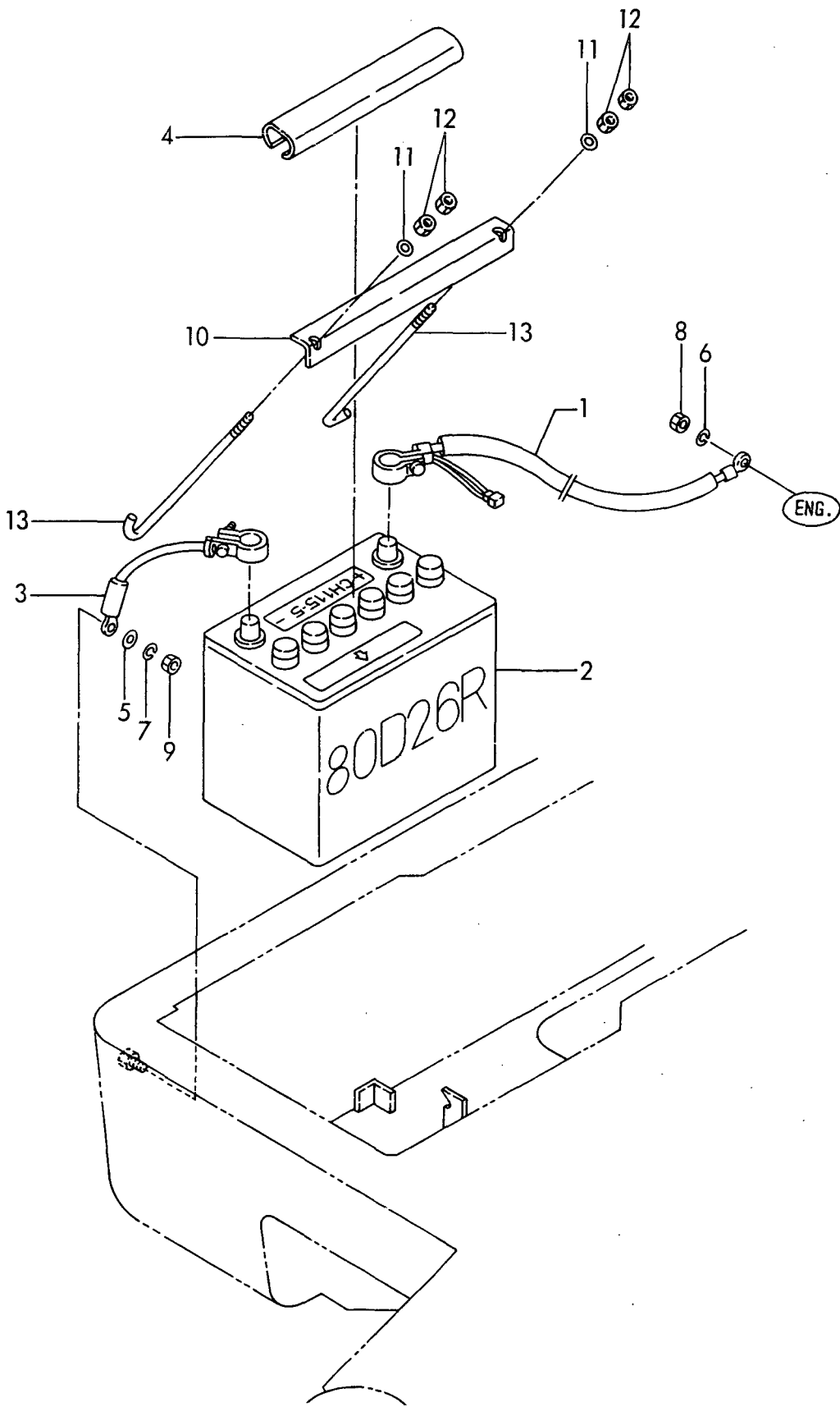
Fig. 9 バッテリー BATTERY
