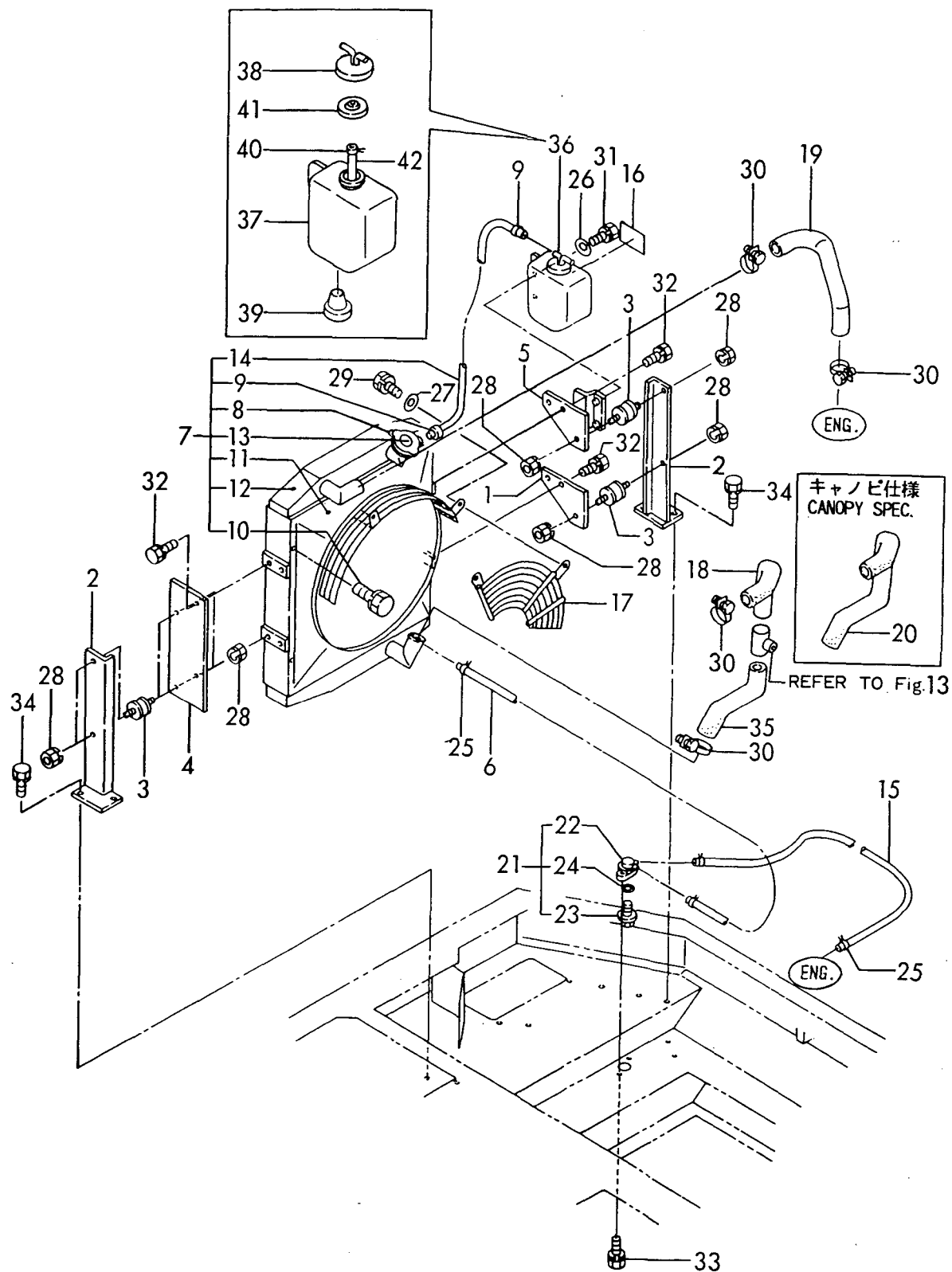
Fig. 7 ラジエータ & マウント https://truckmanualshub.com/ RADIATOR & MOUNT
