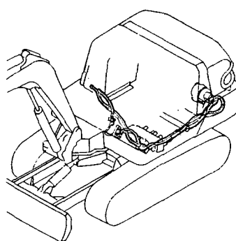
Fig. 59 コントロール配管 (ダイレクト仕様) CONTROL PIPING (DIRECT SPEC.)
