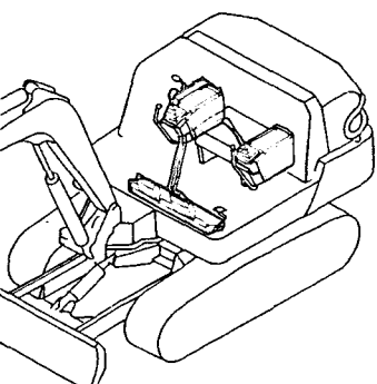
Fig.16 操縦装置(レバー・スタンド) CONTROL EQUIPMENT (LEVER STAND)
