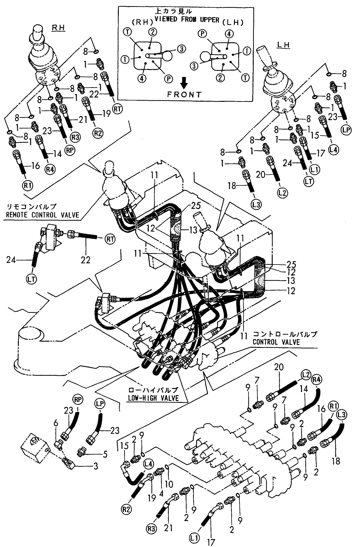
Fig. 59 コントロール配管(ダレ外仕様) CONTROL PIPING(DIRECT SPEC.)
