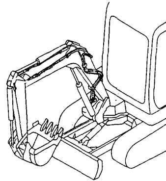
Fig. 58 コントロール配管 (ポンプ〜ローハイパワ〜リターン) CONTROL PIPING(PUMP ~LOW-HIGH V. ~RETURN)
