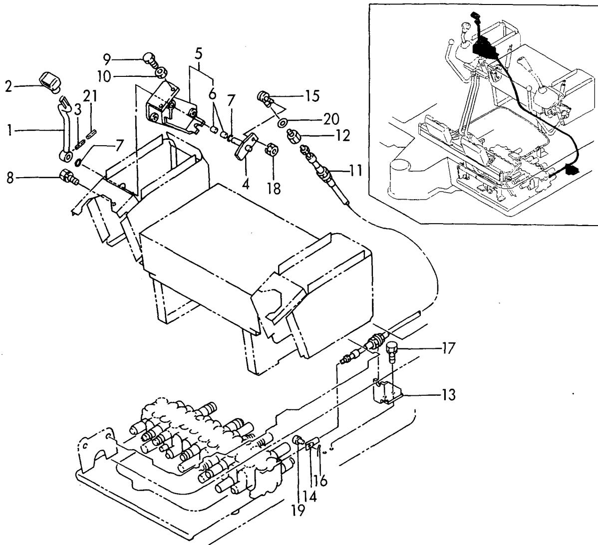
Fig. 19 操縦装置(ブレード) https://truckmanualshub.com/ CONTROL EQUIPMENT (BLADE)
