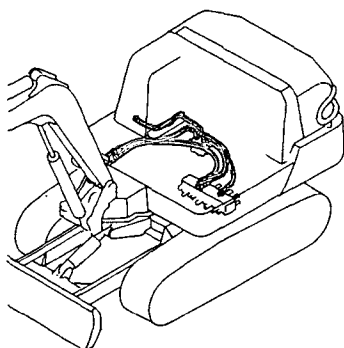
Fig. 55 油圧配管(トラックフレーム) HYD. OIL PIPING (TRACK FRAME)
