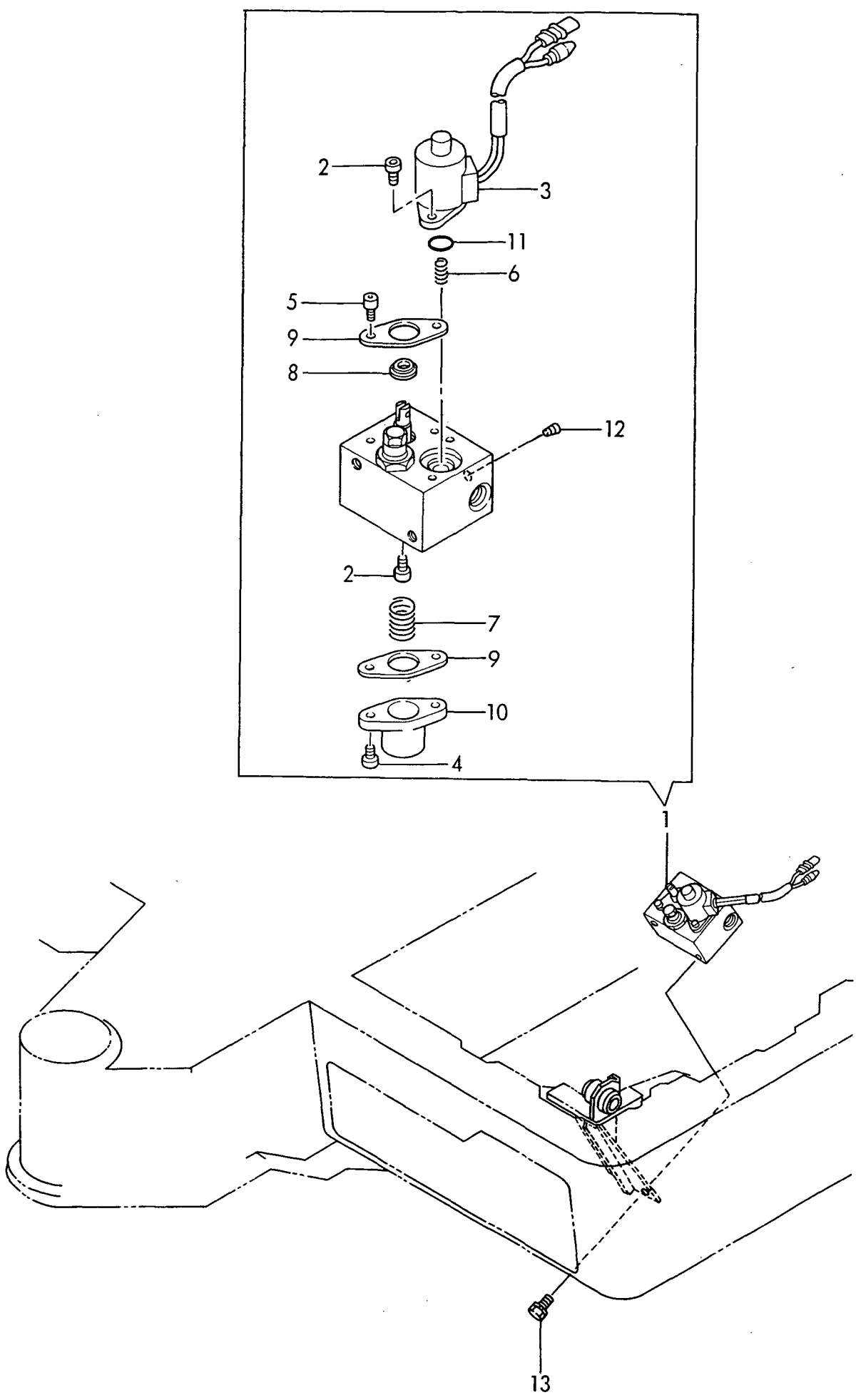
Fig. 47 ローハイバルブ LOW-HIGH VALVE https://truckmanualshub.com/
