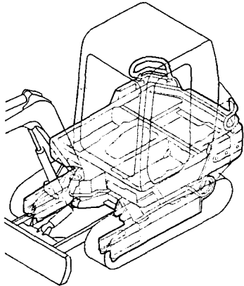
Fig.23 フレームカバー FRAME COVER
