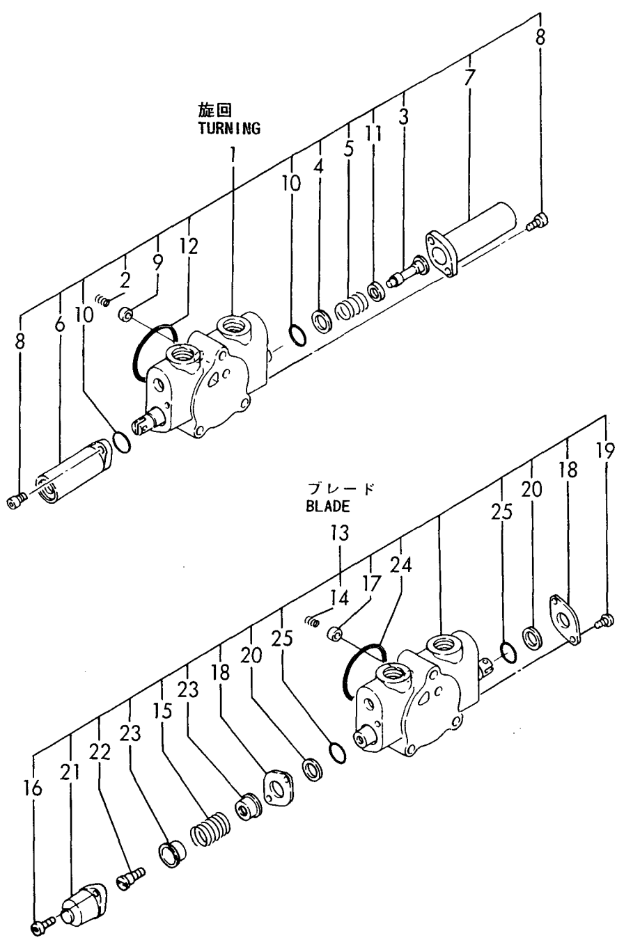
Fig. 44 44 コントロールバルブ(旋回 & ブレード) CONTROL VALVE(TURNING & BLADE)
