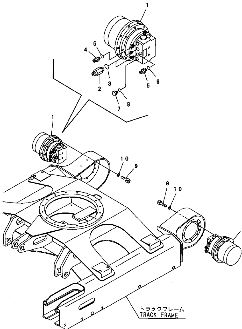
Fig. 71 走行モータ TRAVEL MOTOR
