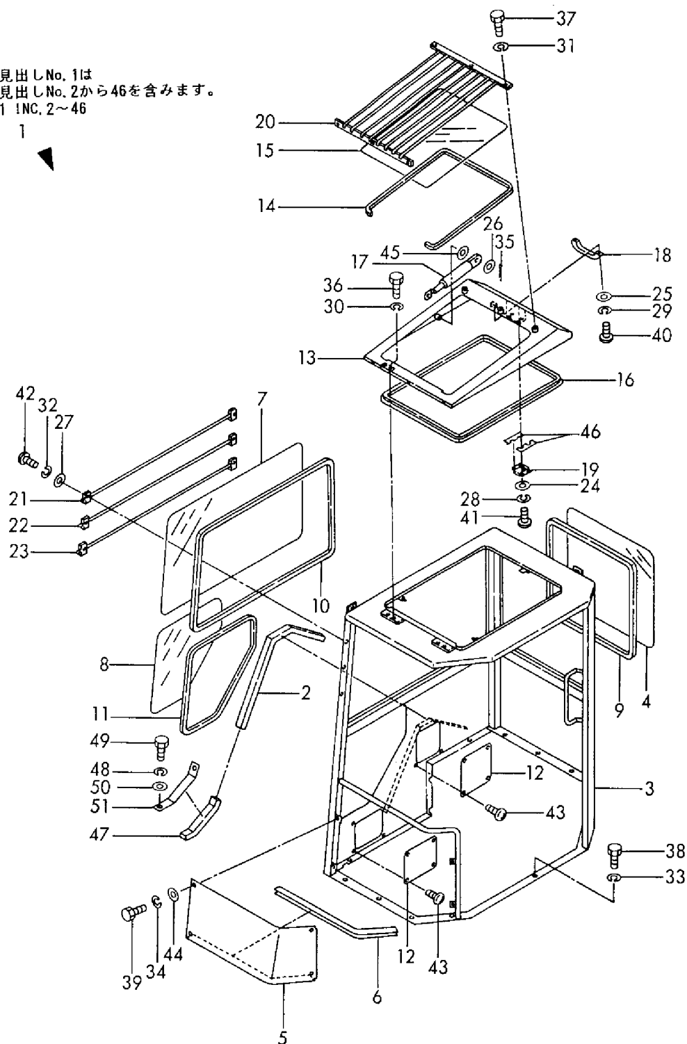
Fig. 42 キャンピ CANOPY
