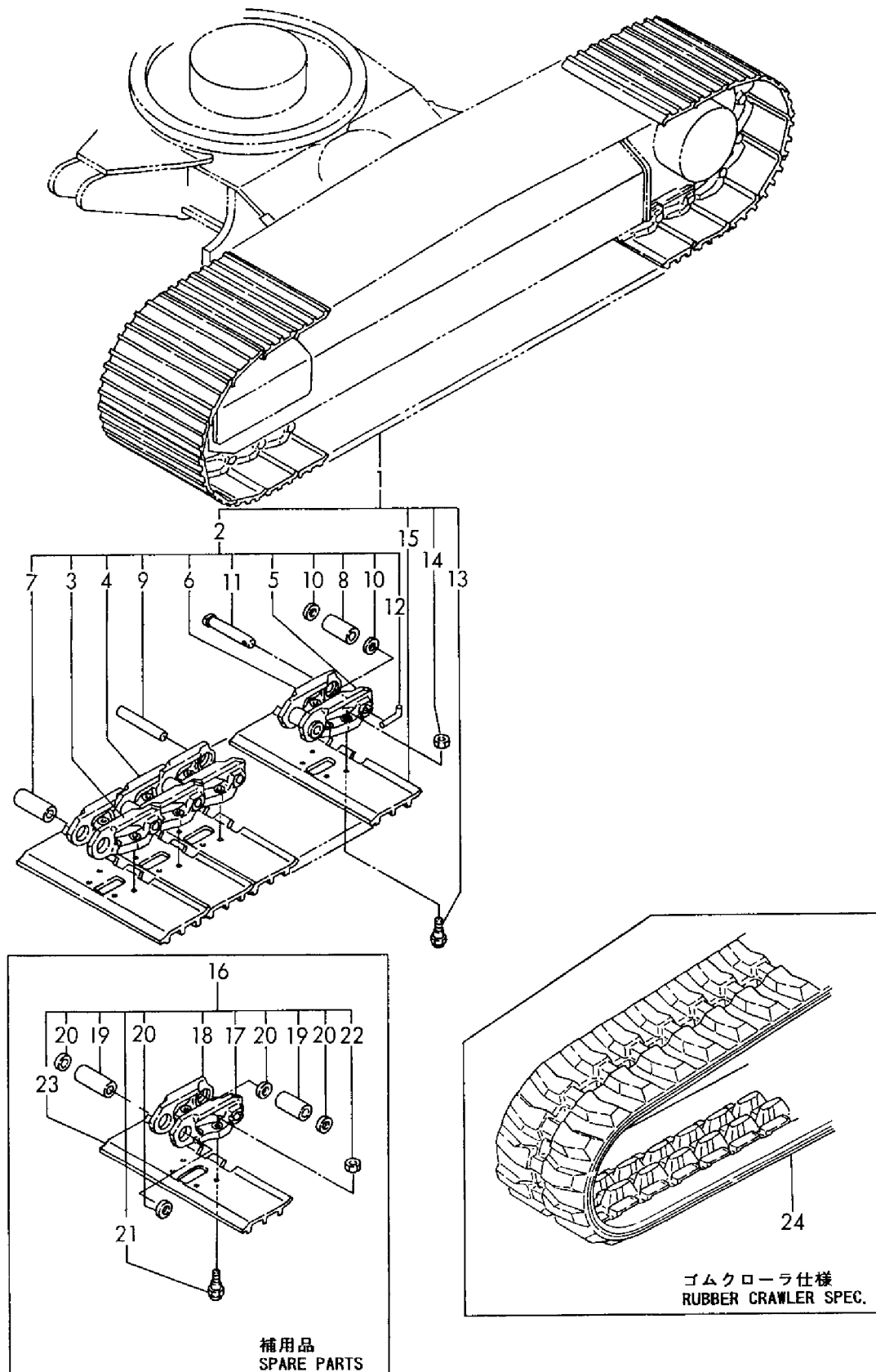
Fig. 29 クローラ(450) CRAWLER(450)
