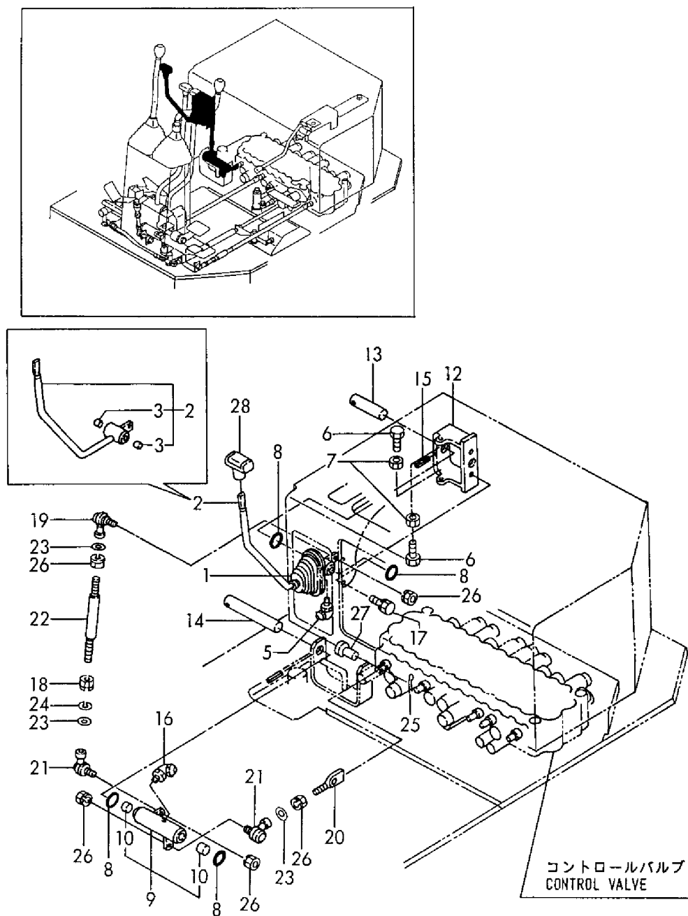
Fig. 32 操縦装置(ブレード) CONTROL EQUIPMENT (BLADE)
