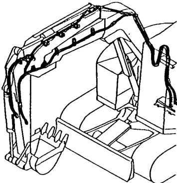
Fig. 74 コントロール配管 (パイロットバ ヴェ-隔壁) CONTROL PIPING (PILOT VALVE-PLATE)
