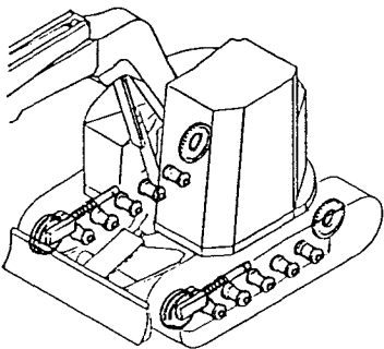
Fig. 28 ローラ & アジャスト (ゴムローラ仕様) ROLLER & ADJUST (RUBBER CRAWLER SPEC.)
