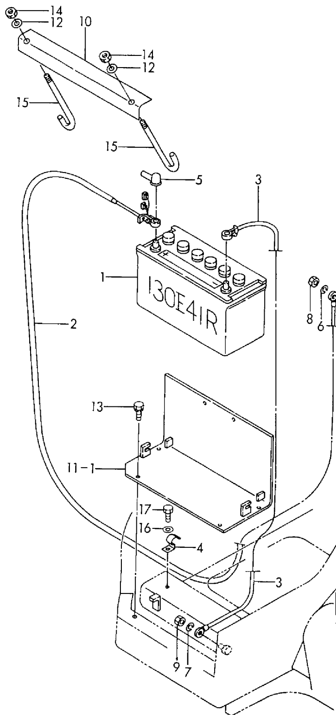
Fig. 14 バッテリー BATTERY
