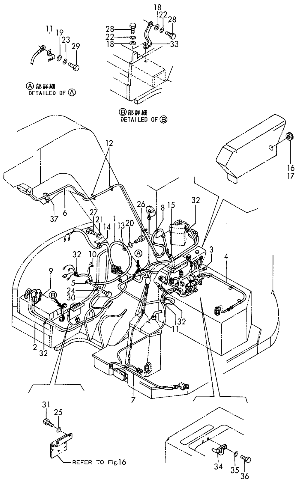
Fig. 15 電装品(ワイリング:キャビン, キャノピー 共通) ELECTRIC PART(WIRING: CABIN, CANOPY)
