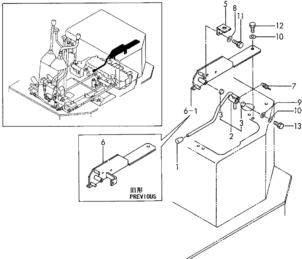
Fig. 35 操縦装置(カットワ) CONTROL EQUIPMENT(CUT-OFF)
