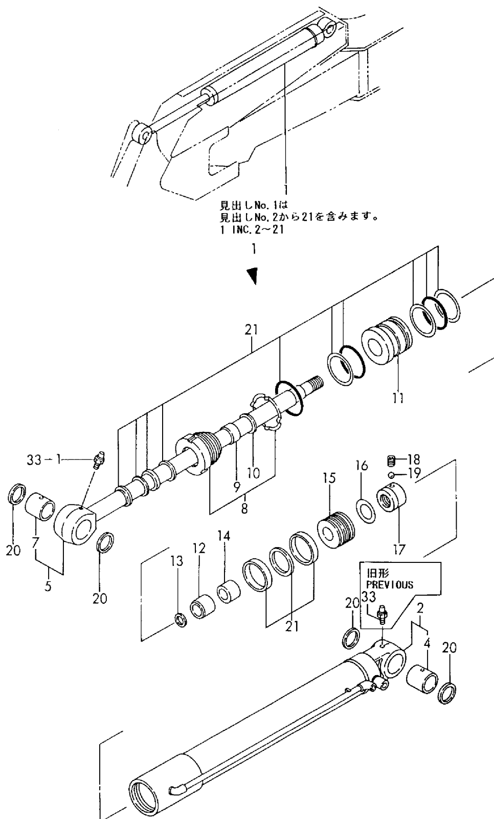
Fig. 52 アームシリンダ ARM CYLINDER
