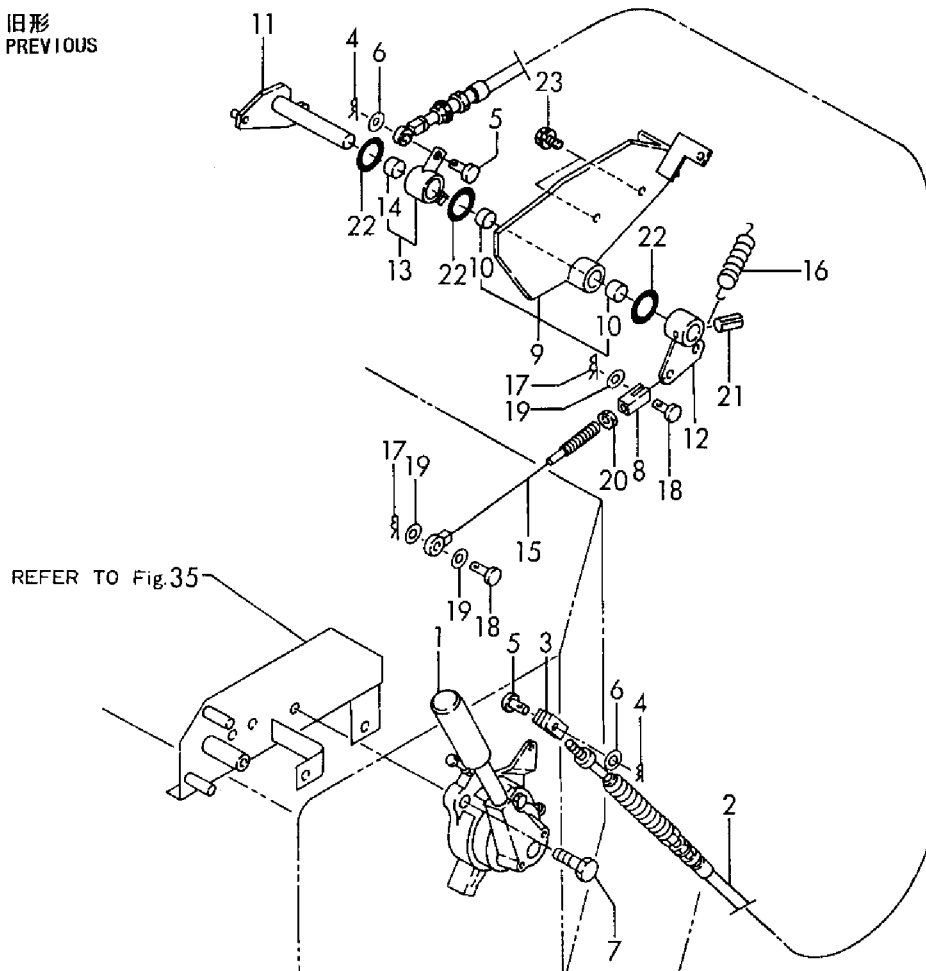
Fig. 9 アクセル ACCELERATOR
