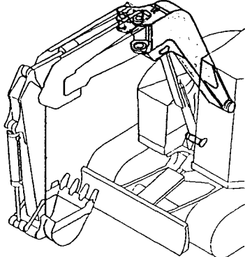
Fig. 80 ブーム(B) BOOM(B)
