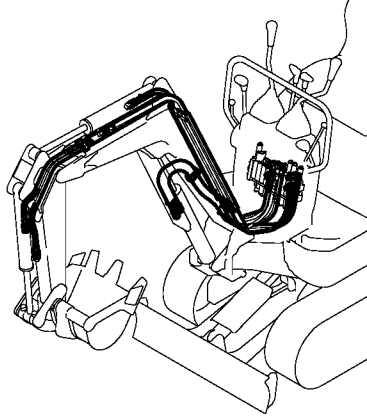
Fig. 54 HYD.OIL PIPING (P. T. O. : BOOM END)
