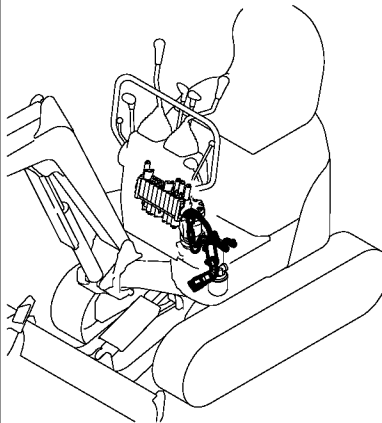
Fig. 51 HYD.OIL PIPING (P. T. O. : FRAME END)
