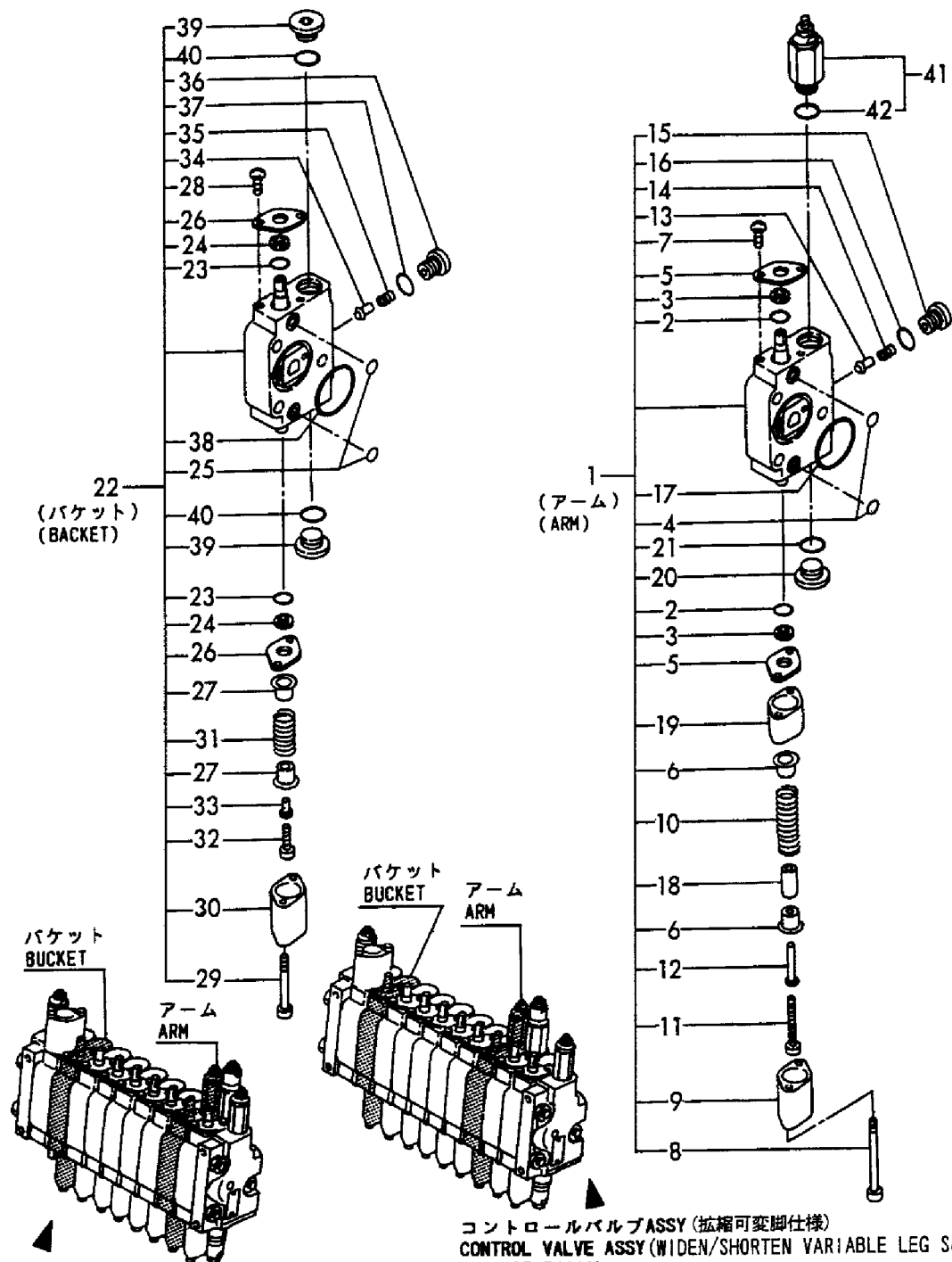
コントロールバルブASSY (固定脚仕様) CONTROL VALVE ASSY (FIX LEG SPEC.) (172157-74100)
