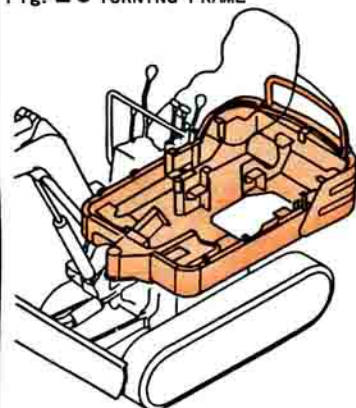
Fig. 27 フレームカバー & インパネ FRAME COVER & INSTRUMENT PANEL
