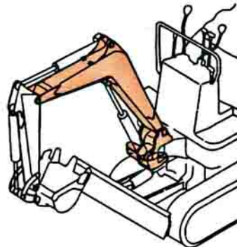
Fig. 59 アーム & バケットリンク ARM & BUCKET LINK
