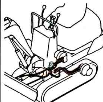
Fig. 51 油圧配管(走行フレーム: リンク仕様) HYD. OIL PIPING (DRIVING FRAME: LOTUS ROOT SPEC.)
