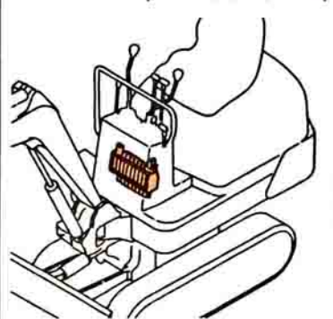
Fig. 42 コントロールバルブ (スイング & ブーム) CONTROL VALVE (SWING & BOOM)
