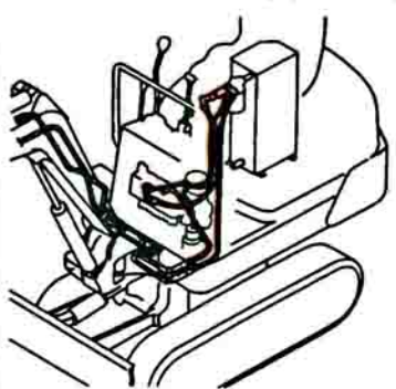
Fig. 55 油圧配管(PTO, ブームエンド) (オプション) (旧形) HYD. OIL PIPING (P.T.O., BOOM END) (OPTIONAL) (PREVIOUS)
