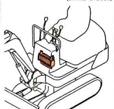
Fig. 43 コントロールバルブ (アーム & バケット) CONTROL VALVE (ARM & BUCKET)
