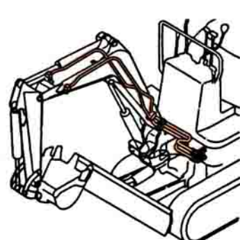
Fig. 56 油圧配管(PTO, ブームエンド) (オプション) (新形) HYD. OIL PIPING (P.T.O., BOOM END) (OPTIONAL) (NEW)
