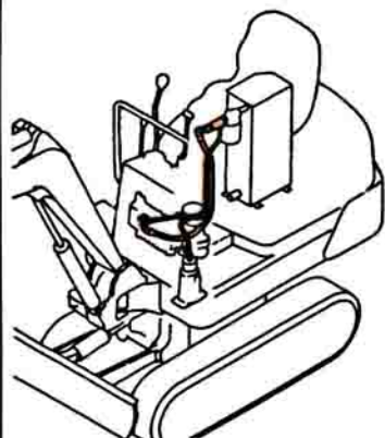
Fig. 50 油圧配管(走行フレーム: 固定脚仕様) HYD. OIL PIPING (DRIVING FRAME: FIX LEG SPEC.)
