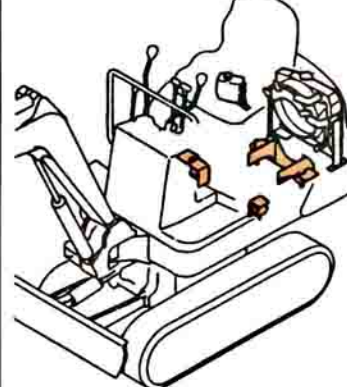
Fig. 11 ラジエータ & マウント RADIATOR & MOUNT
