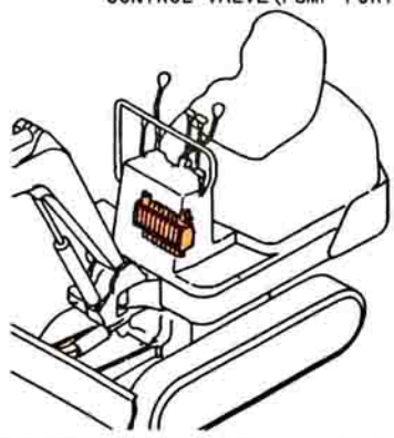
Fig. 40 コントロールバルブ (ポンプポート) CONTROL VALVE (PUMP PORT)
