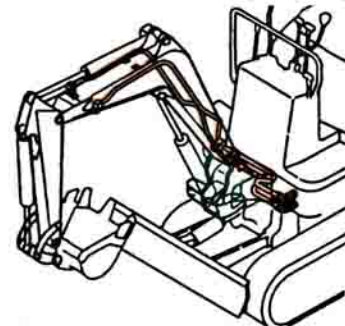
Fig. 56 油圧配管(PTO, ブームエンド) (オプション) (新形) HYD. OIL PIPING (P.T.O., BOOM END) (OPTIONAL) (NEW)
