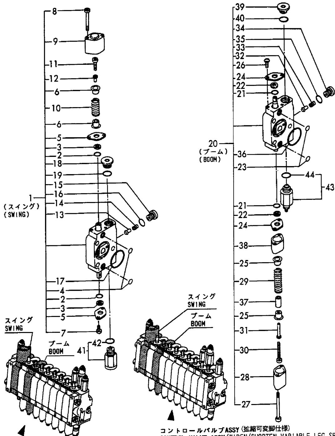
コントロールバルブASSY (固定脚仕様) CONTROL VALVE ASSY (FIX LEG SPEC.) (172157-74100)
