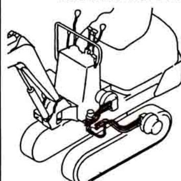
Fig. 52 油圧配管(走行フレーム: 拡張可変脚仕様) HYD. OIL PIPING (DRIVING FRAME: WIDEN/SHORTEN VARIABLE LEG SPEC.)
