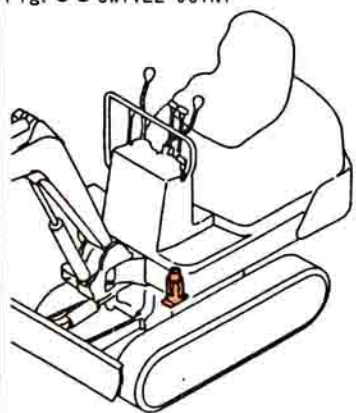
Fig. 40 コントロールバルブ (ポンプポート) CONTROL VALVE (PUMP PORT)
