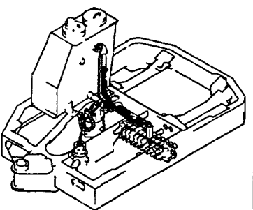
Fig. 51 油圧配管 (リターン) HYD. OIL PIPING (RETURN)
