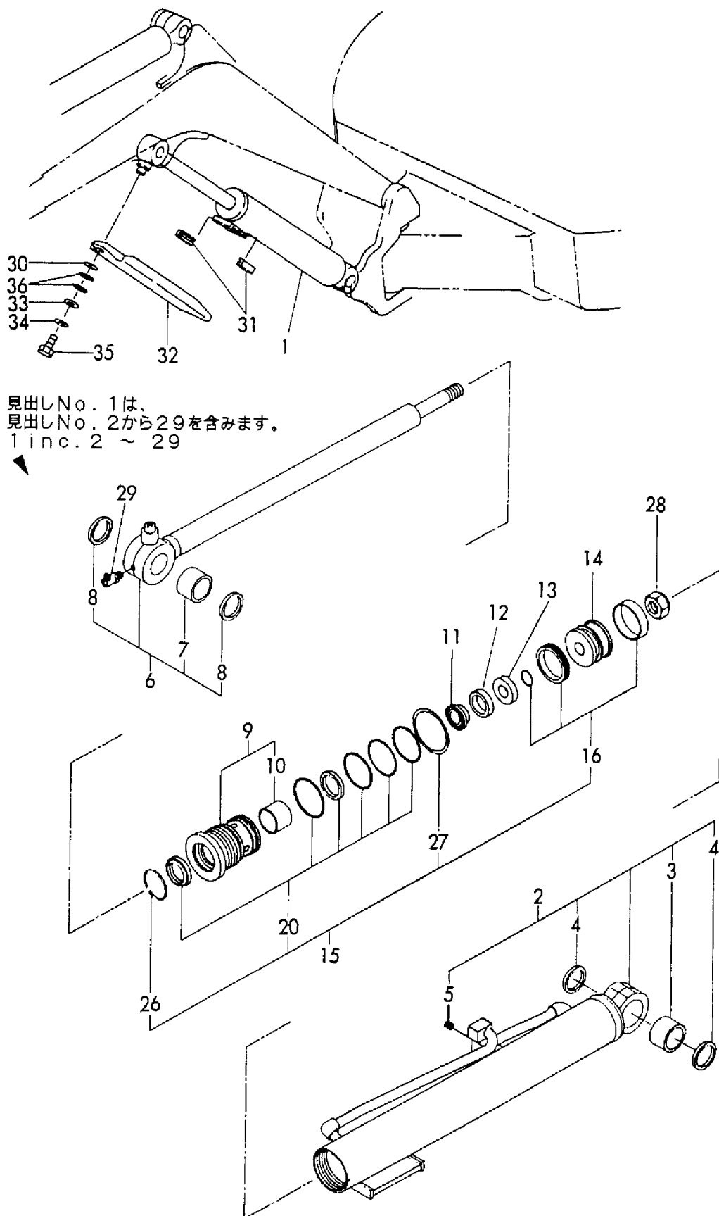
Fig. 28 ブームシリンダ BOOM CYLINDER
