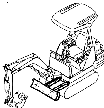
Fig. 64 ブレード BLADE
