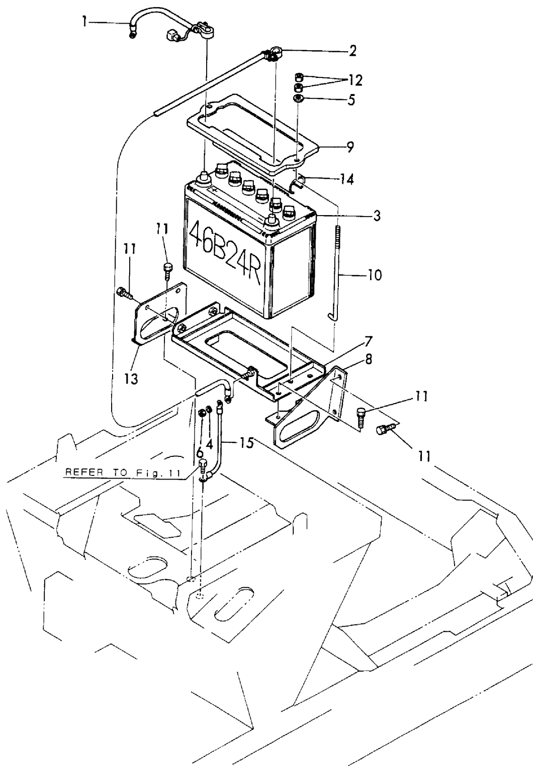
Fig. 10 バッテリー BATTERY
