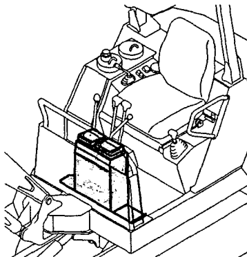
Fig. 18 操縦装置 (ブーム&バケット) CONTROL EQUIPMENT (BOOM & BUCKET)
