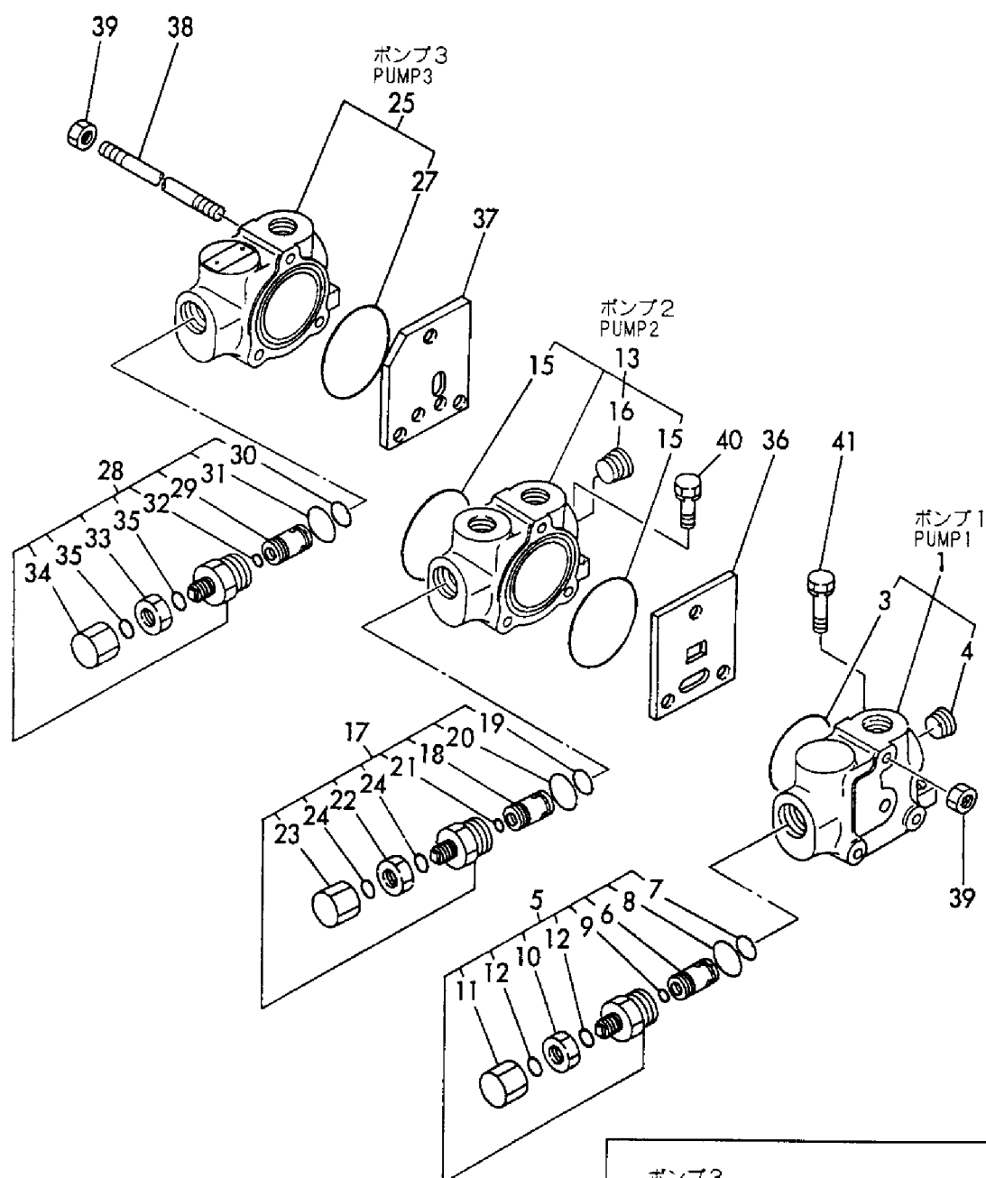
Fig. 43 コントロールバルブ (P1, P2, P3) CONTROL VALVE (P1, P2, P3)
