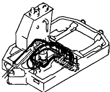
Fig. 50 油圧配管 (バルブ~スイベル ~モータ) (レンコン仕様) HYD. OIL PIPING (VALVE~SWIVEL~MOTOR) (LOTUS ROOT SPEC.)
