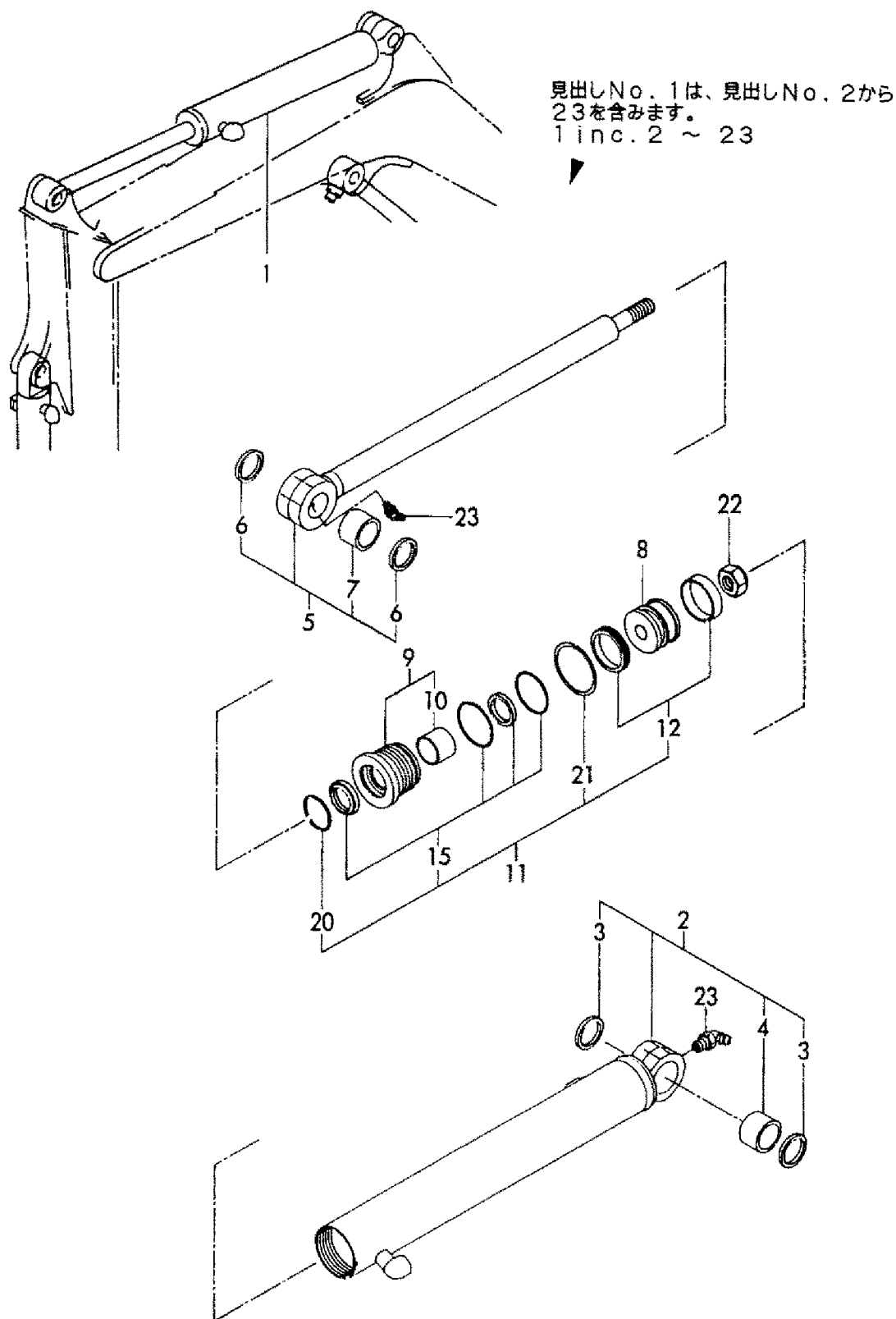
Fig. 29 アームシリンダ ARM CYLINDER
