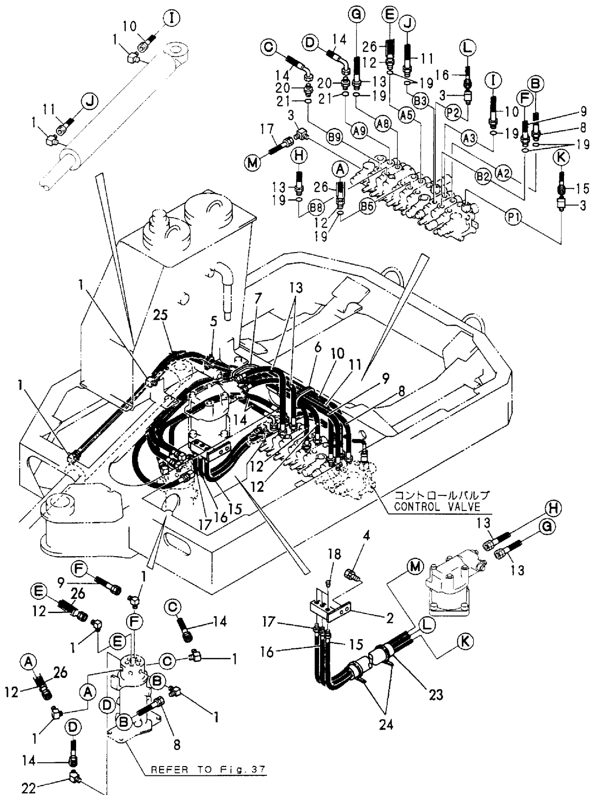
Fig. 49 油圧配管 (バルブ~スィベル~モータ) HYD. OIL PIPING (VALVE~SWIVEL~MOTOR)
