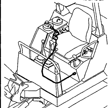
Fig. 21 操縦装置 (ブレード) CONTROL EQUIPMENT (BLADE)
