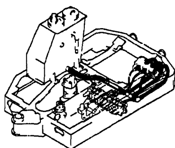
Fig. 48 油圧配管 (タンク～バルブ) (レンコン仕様) HYD. OIL PIPING (TANK~VALVE) (LOTUS ROOT SPEC.)
