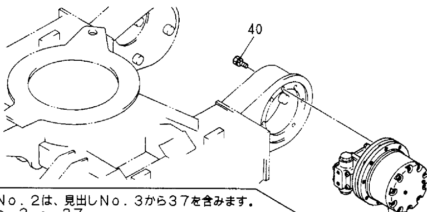
Fig. 35 走行モータ TRAVEL MOTOR
