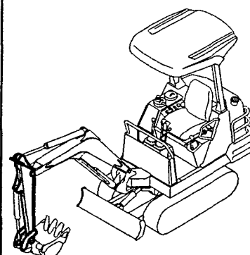
Fig. 60 アーム&バケットリンク (レンコン仕様) ARM & BUCKET LINK (LOTUS ROOT SPEC.)
