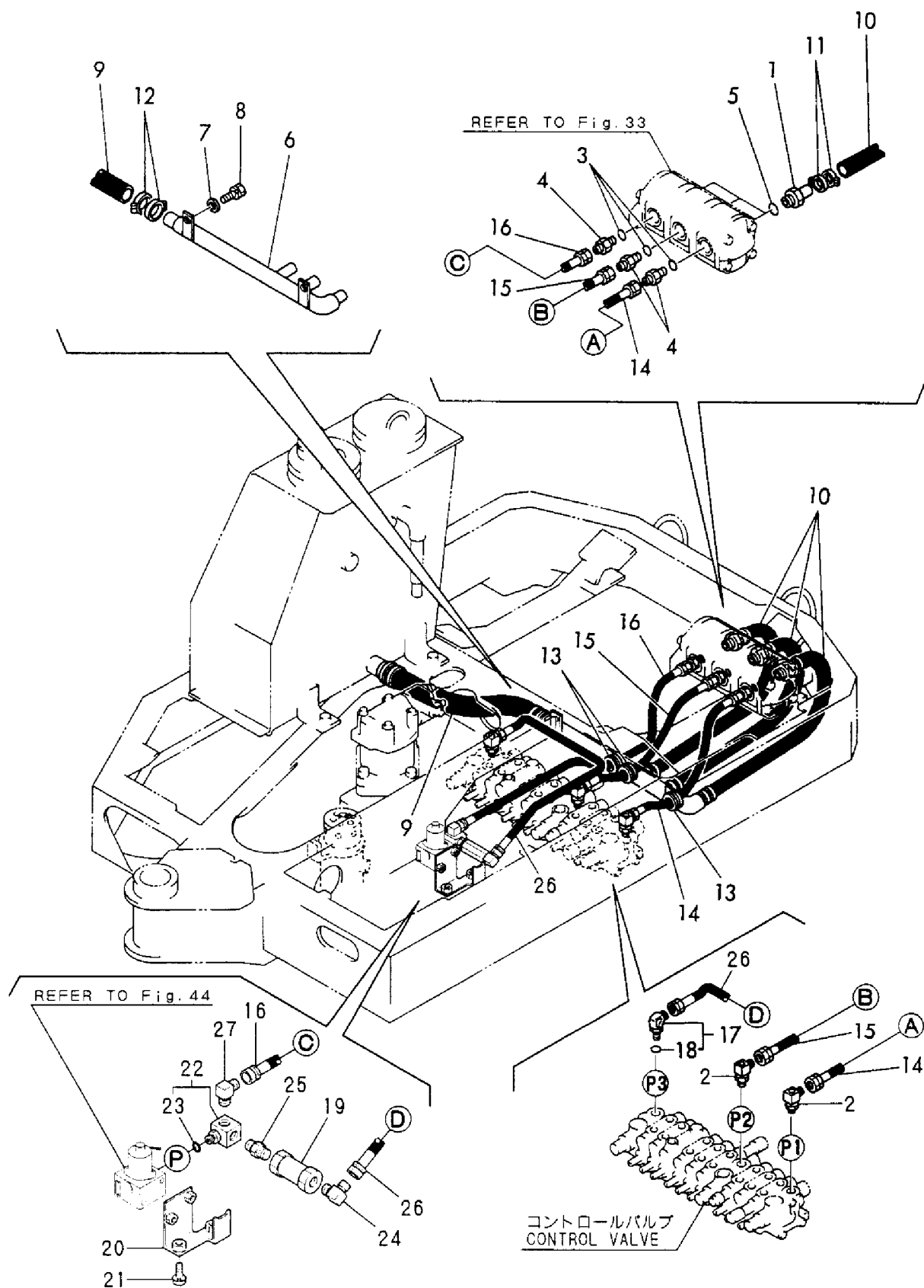
Fig. 48 油圧配管 (タンク~バルブ) (レンコン仕様) HYD. OIL PIPING (TANK~VALVE) (LOTUS ROOT SPEC.)
