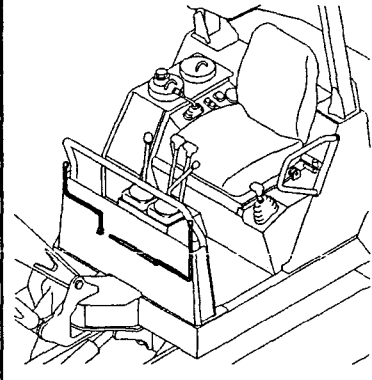
Fig. 23 旋回フレーム TURNING FRAME
