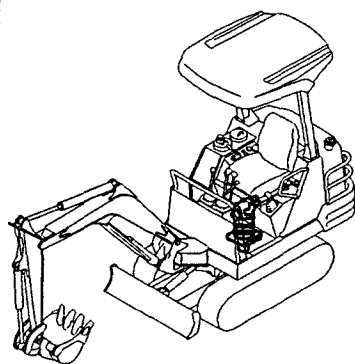
Fig. 35 走行モータ TRAVEL MOTOR
