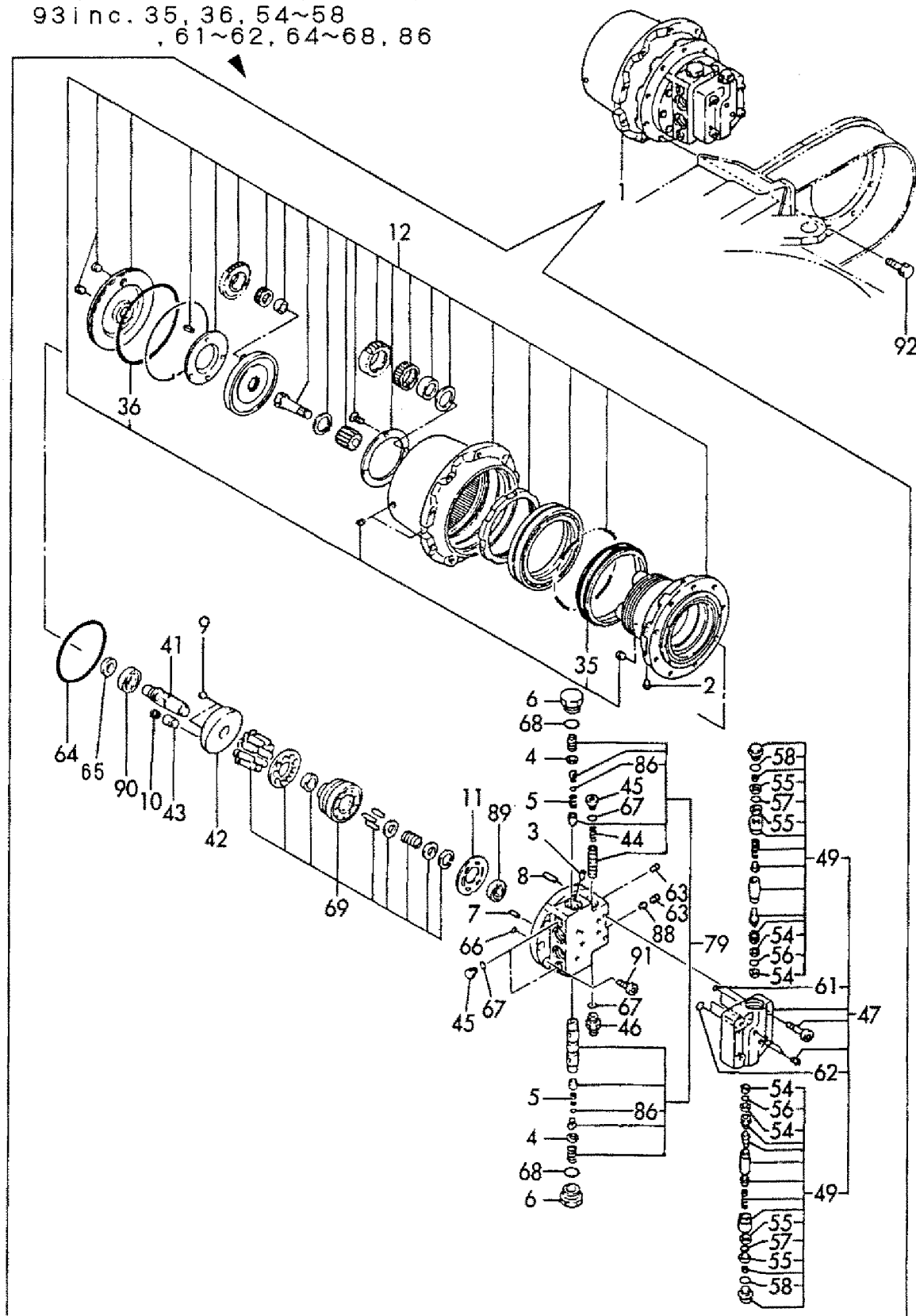
Fig. 36 走行モータ (レンコン仕様) TRAVEL MOTOR (LOTUS ROOT SPEC.)
