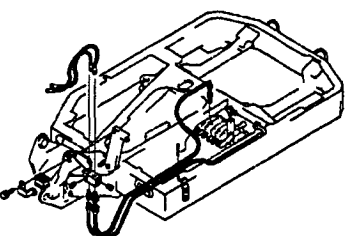
Fig. 56 油圧配管 (PTOバルブ ~ブームブラケット) HYD. OIL PIPING (P. T. O. VALVE ~BOOM BRACKET)
