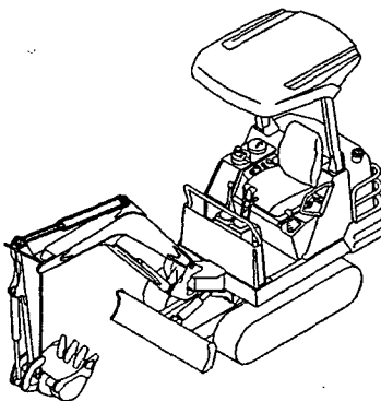
Fig. 30 バケットシリンダ BUCKET CYLINDER
