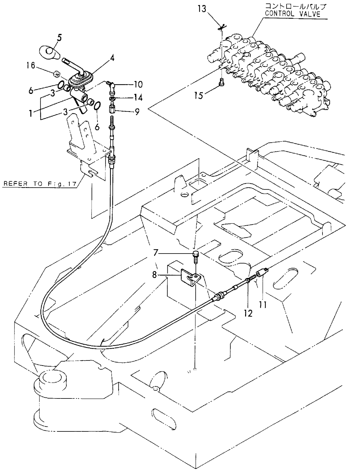
Fig. 21 操縦装置 (ブレード) CONTROL EQUIPMENT (BLADE)
