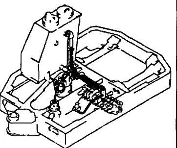
Fig. 52 油圧配管 (リターン) (レンコン仕様) HYD. OIL PIPING (RETURN) (LOTUS ROOT SPEC.)
