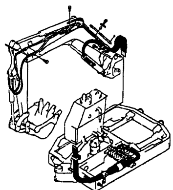
Fig. 56 油圧配管 (PTOバルブ ~ブームブラケット) HYD. OIL PIPING (P. T. O. VALVE ~BOOM BRACKET)
