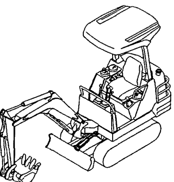
Fig. 32 ブレードシリンダ BLADE CYLINDER
