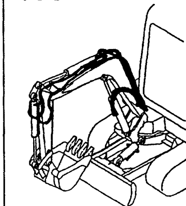
Fig. 96 油圧配管 (ブーム) HYD. OIL PIPING (BOOM)
