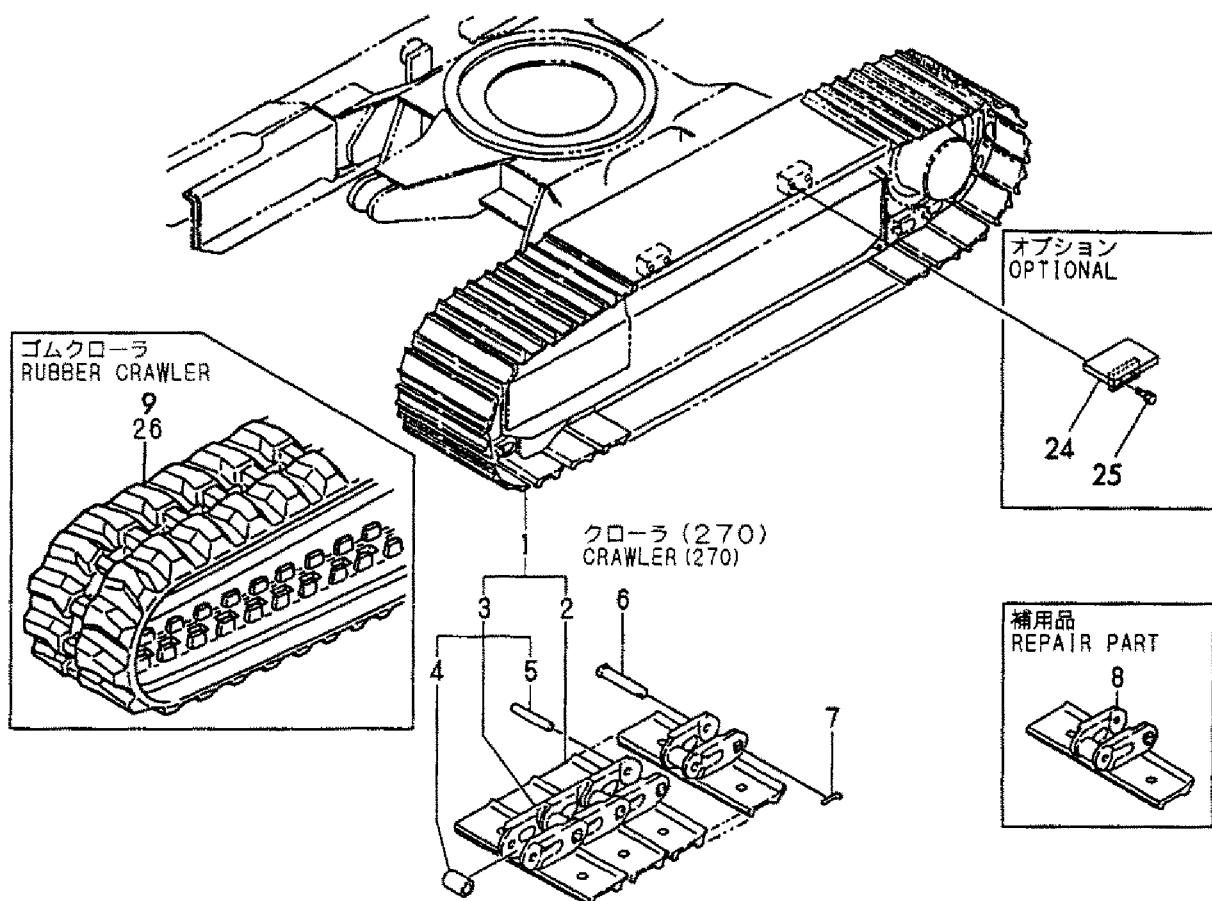
Fig. 23 クローラ CRAWLER
