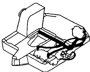
Fig. 85 油圧配管 (タンク〜ポンプ〜バルブ) (レンコン仕様) HYD. OIL PIPING (TANK~PUMP~VALVE) (LOTUS ROOT SPEC.)
