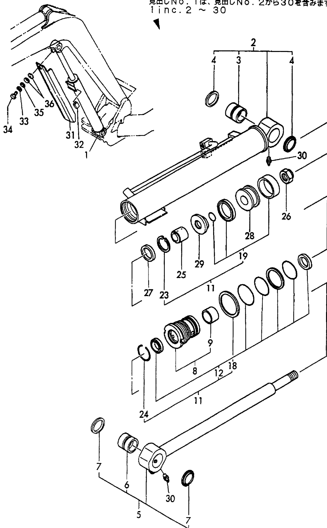
Fig. 50 ブームシリンダ (キャビン) BOOM CYLINDER (CABIN)
