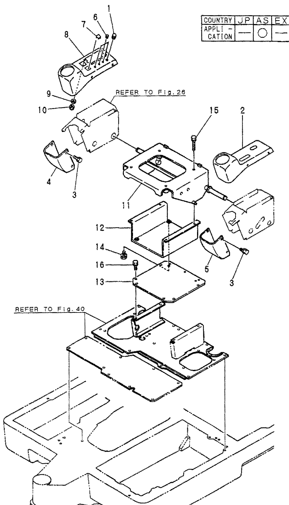
Fig. 42 シートマウント (AS) SEAT MOUNT (AS)
