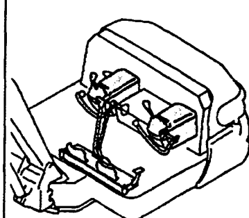
Fig. 34 操縦装置 (PTOコントロール) CONTROL EQUIPMENT (P. T. O. CONTROL)
