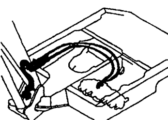
Fig. 92 油圧配管 (PTOバルブ〜フレーム) HYD. OIL PIPING (P. T. O. VALVE~FRAME)
