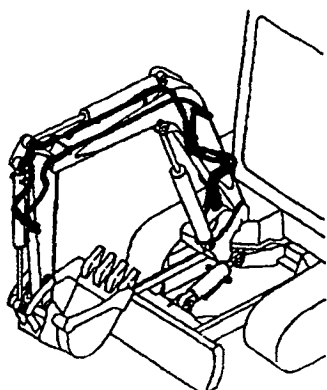
Fig. 98 コントロール配管 (リモコンバルブ~ ~チェンジバルブ) (フロントマルチ) CONTROL PIPING (REMO-CON VALVE~ CHANGE VALVE) (FRONT MULTI)
