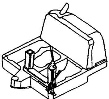
Fig. 28 操縦装置 (アーム&旋回) CONTROL EQUIPMENT (ARM & TURNING)
