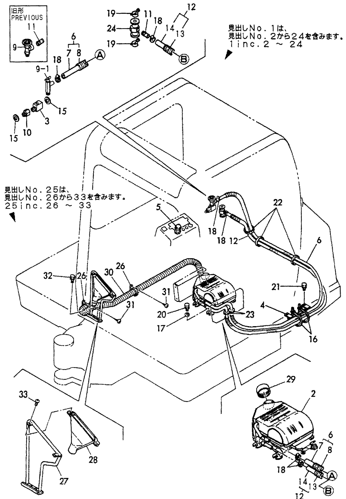
Fig. 19 ヒータ&デフロスタ HEATER & DEFROSTER
