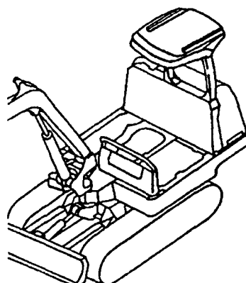
Fig. 48 油圧ポンプ&軸継手 HYD. OIL PUMP & JOINT
