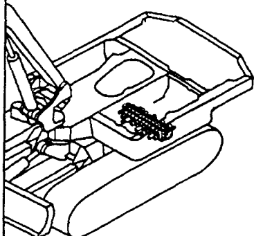
Fig. 76 コントロールバルブ (旋回&ブレード) (AS) CONTROL VALVE (TURNING & BLADE) (AS)
