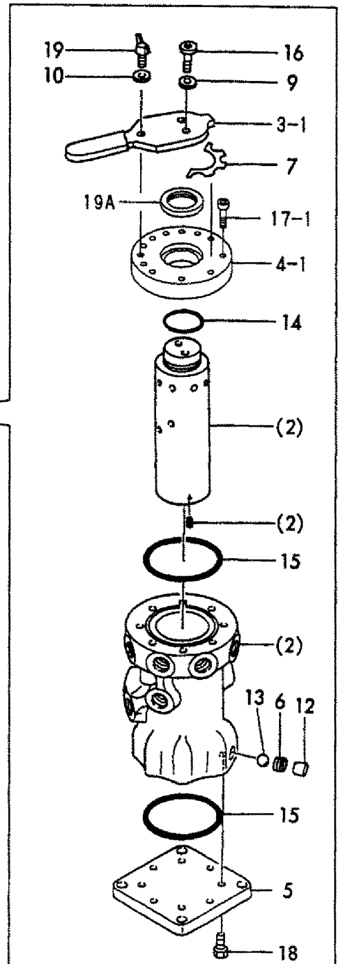
Fig. 82 ロータリバルブ (フロントマルチ) ROTARY VALVE (FRONT MALT)
