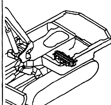
Fig. 71 コントロールバルブ (旋回& ブレード) (フロントマルチ) CONTROL VALVE (TURNING & BLADE) (FRONT MULTI)
