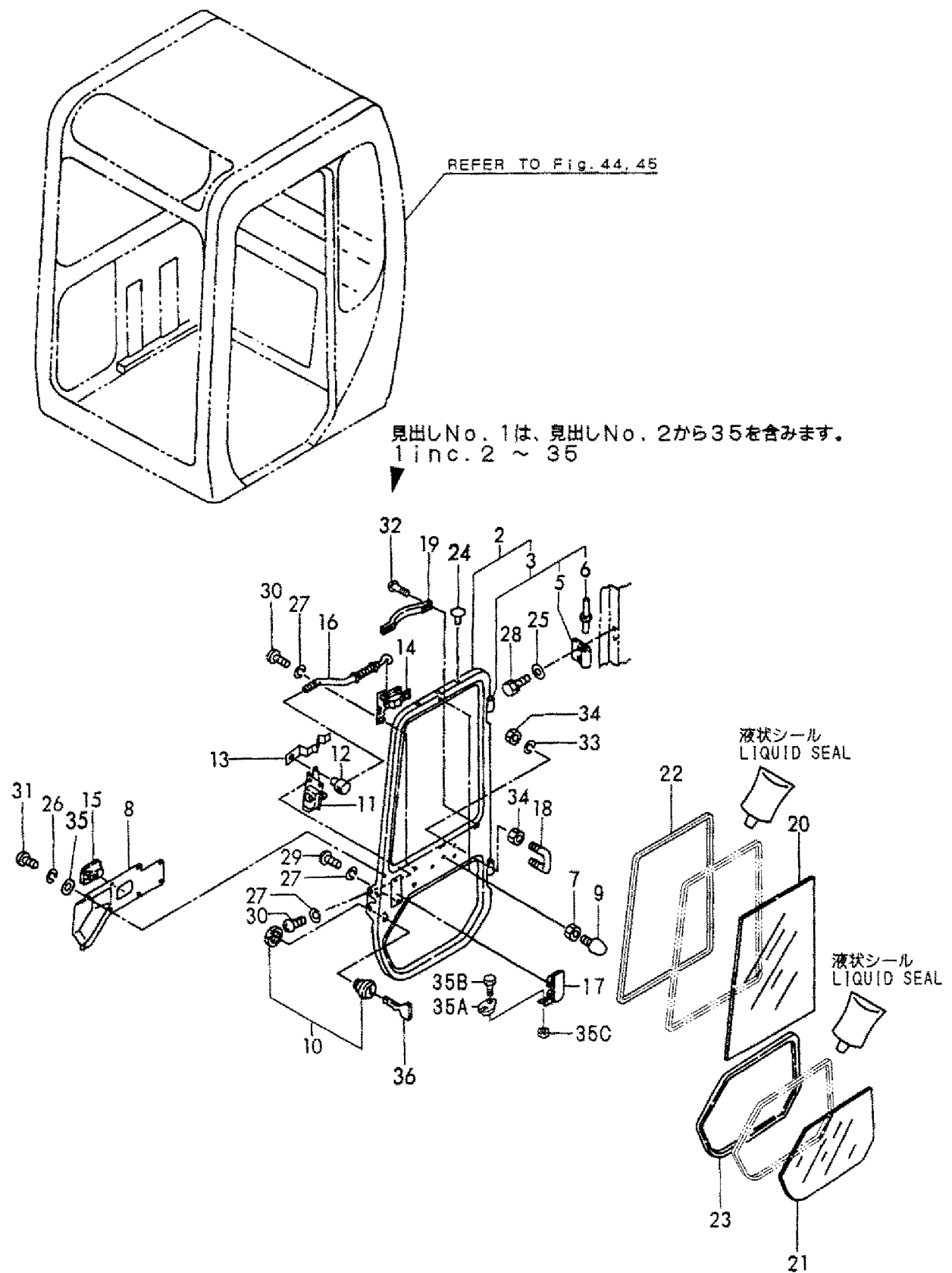
Fig. 46 キャビンドア CABIN DOOR
