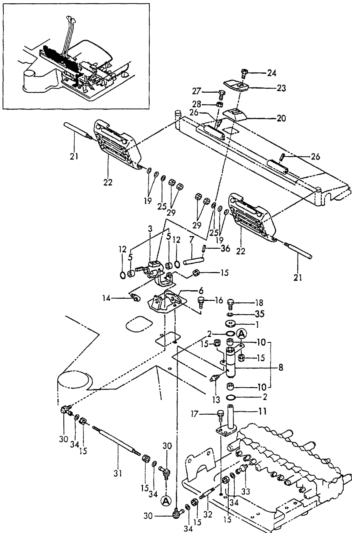
Fig. 30 操縦装置 (スイング) CONTROL EQUIPMENT (SWING)
