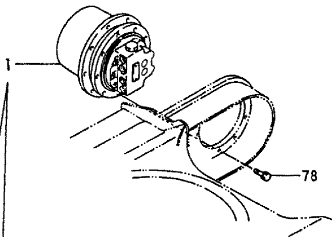
Fig. 58 走行モータ (レンコン仕様) TRAVEL MOTOR (LOTUS ROOT SPEC.)
