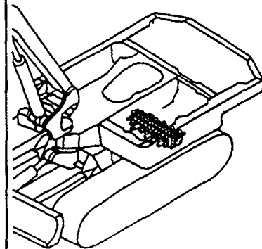
Fig. 72 コントロールバルブ (Pポート) (AS) CONTROL VALVE (P PORT) (AS)
