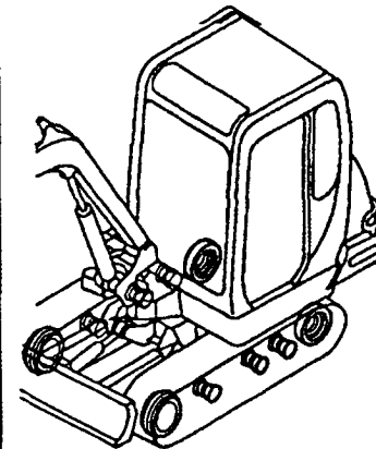
Fig. 22 ローラ&アジャスト (レンコン仕様) ROLLER & ADJUST (LOTUS ROOT SPEC.)
