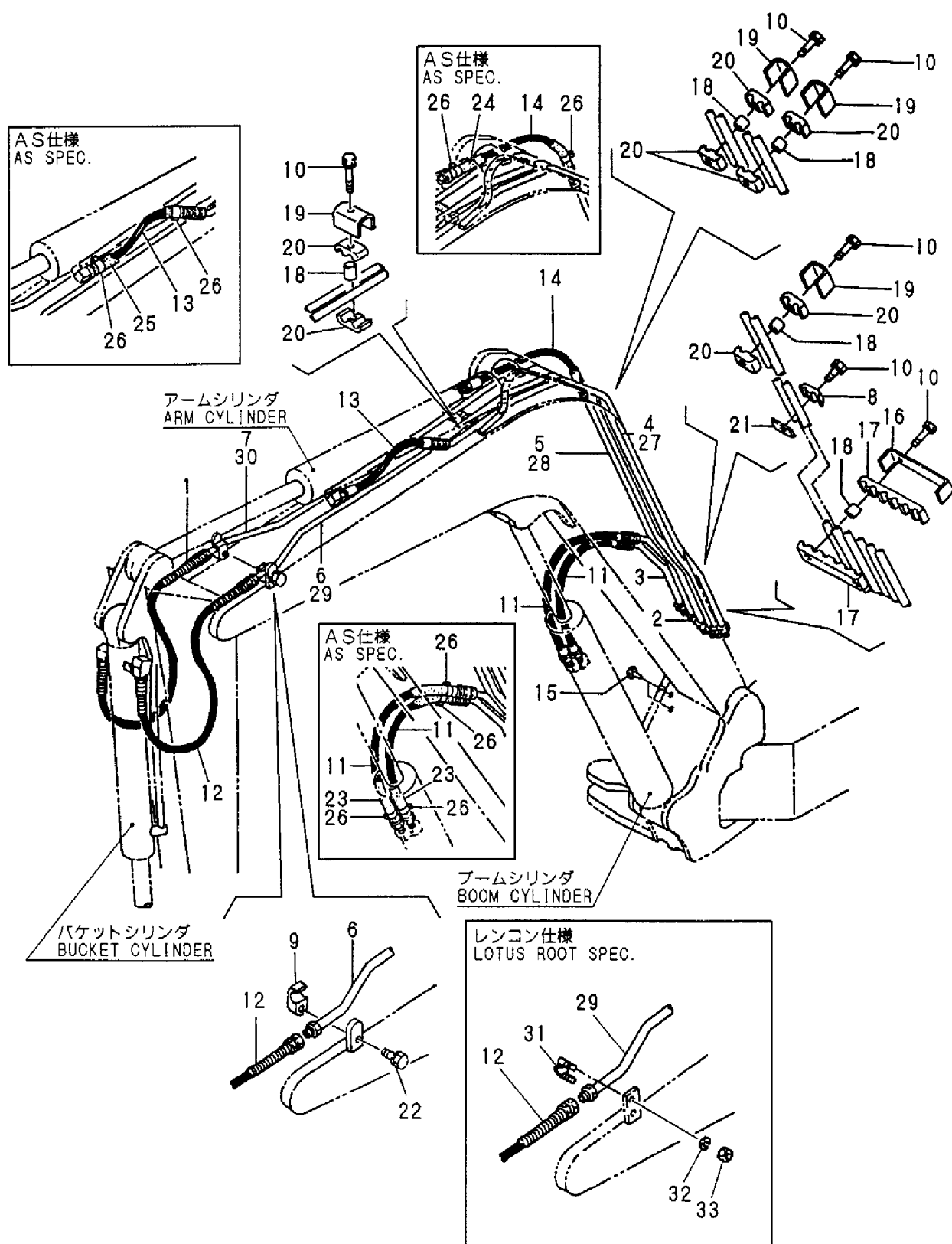
Fig. 96 油圧配管 (ブーム) HYD. OIL PIPING (BOOM)
