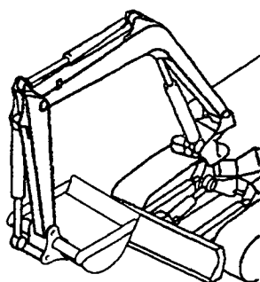
Fig. 104 ブーム&アーム (レンコン仕様) BOOM & ARM (LOTUS ROOT SPEC.)
