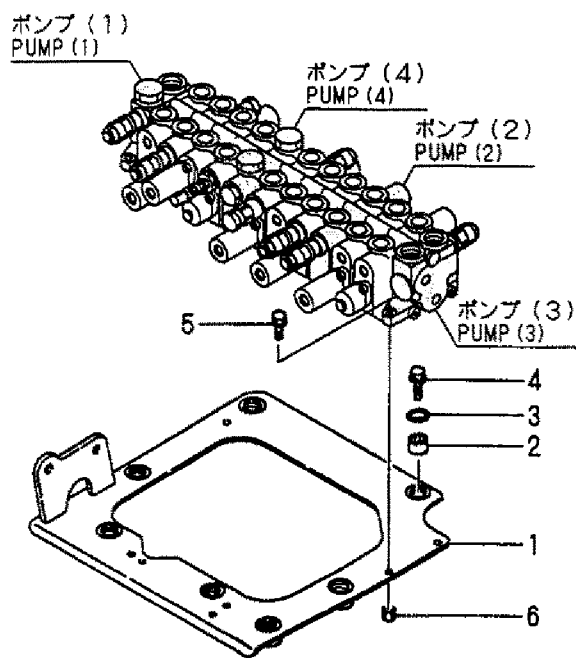
Fig. 72 コントロールバルブ (Pポート) (AS) CONTROL VALVE (P PORT) (AS)
