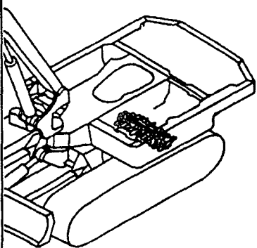
Fig. 64 コントロールバルブ (アーム&スイング) CONTROL VALVE (ARM & SWING)
