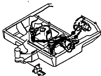
Fig. 100 コントロール配管 (ダイレクト) (AS) CONTROL PIPING (DIRECT) (AS)
