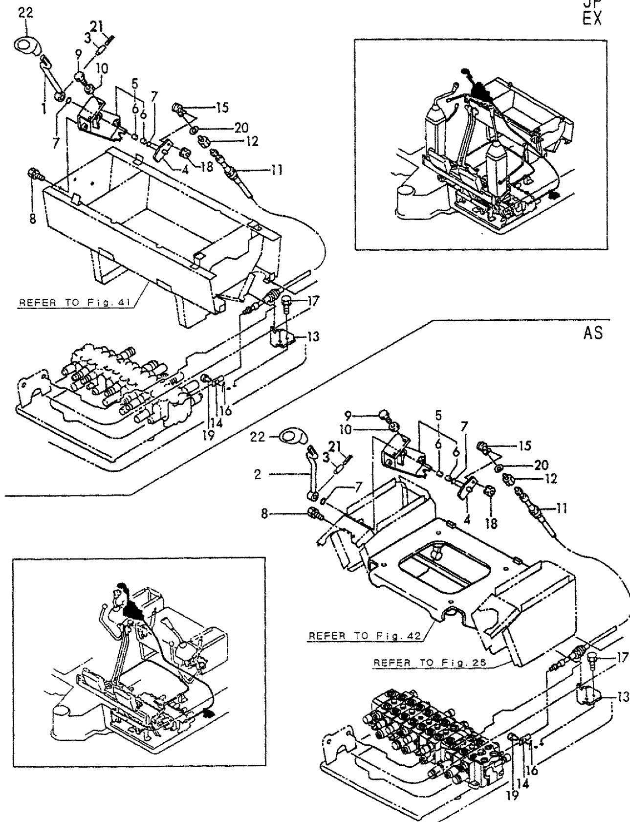
Fig. 31 操縦装置 (ブレード) CONTROL EQUIPMENT (BLADE)
