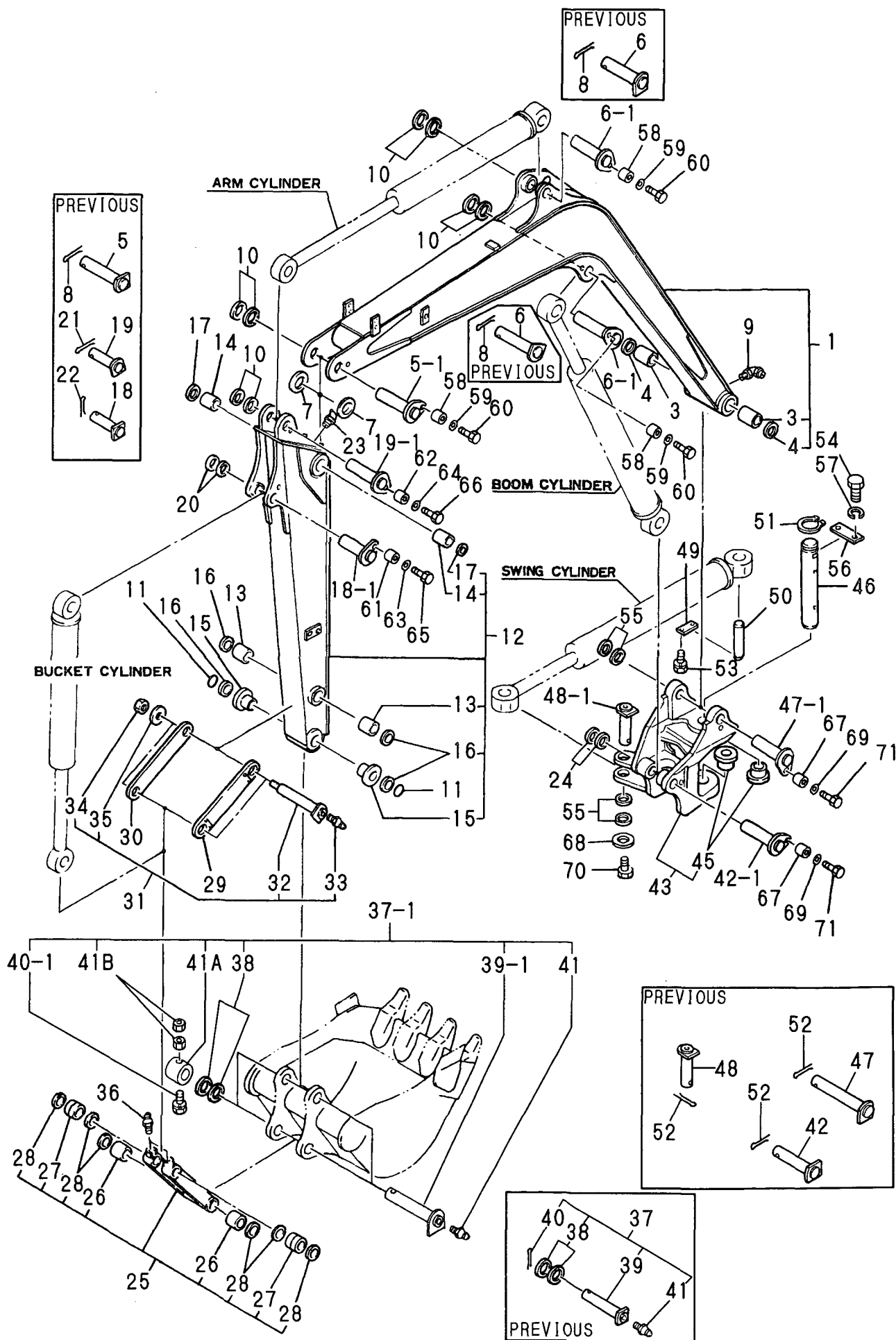
Fig. 62 BOOM & ARM
