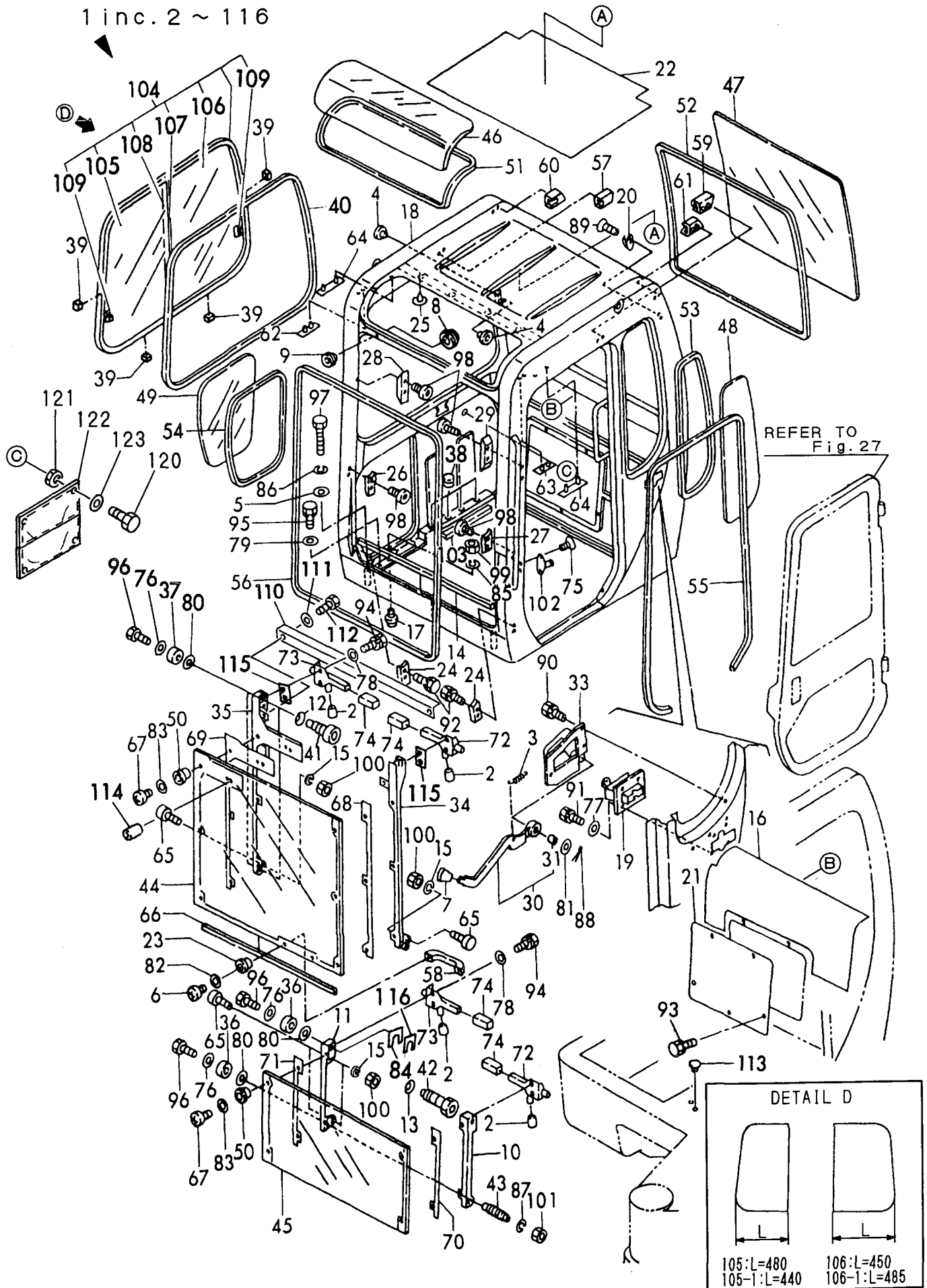
Fig. 26 CABIN
