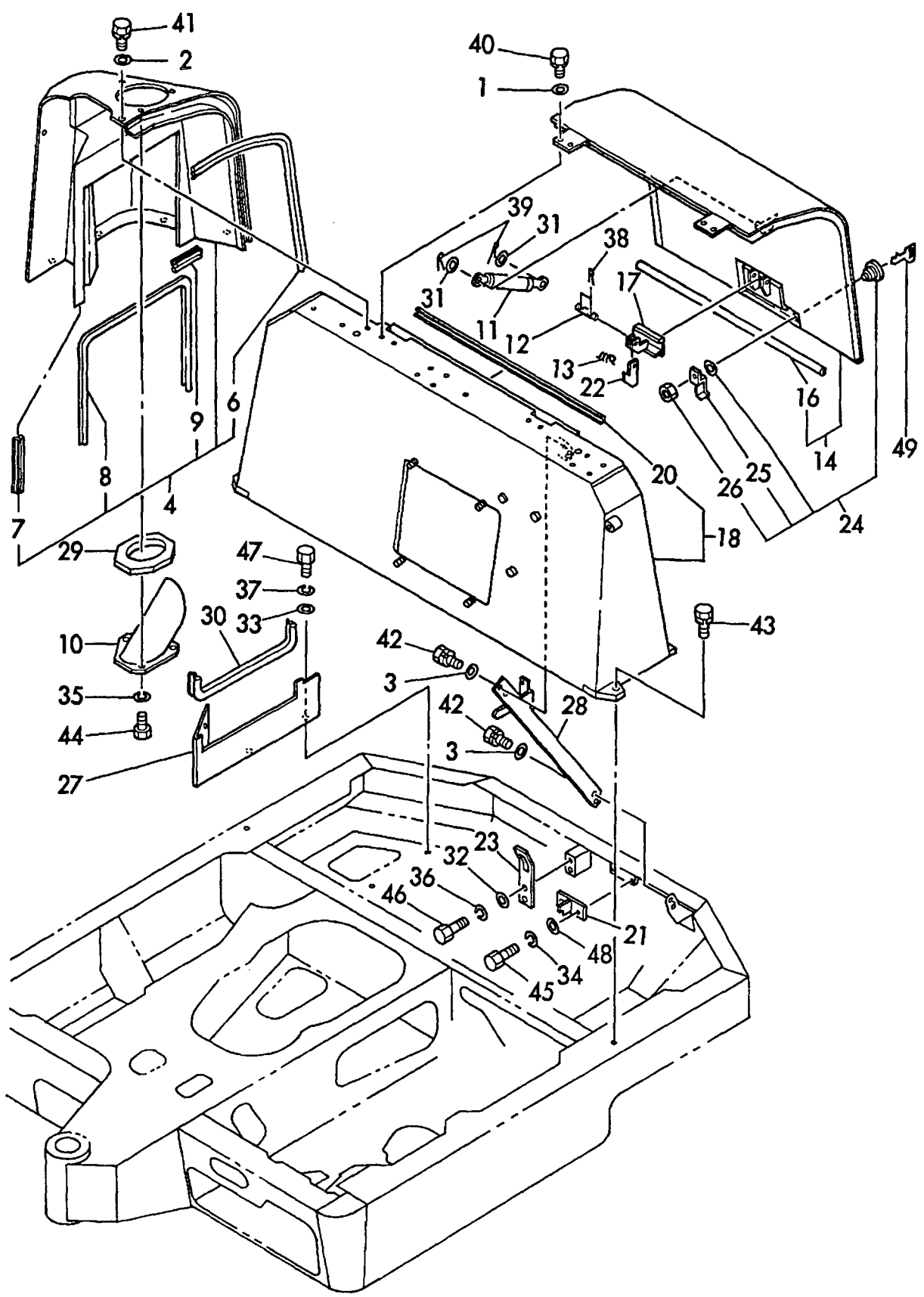
Fig. 22 BONNET
