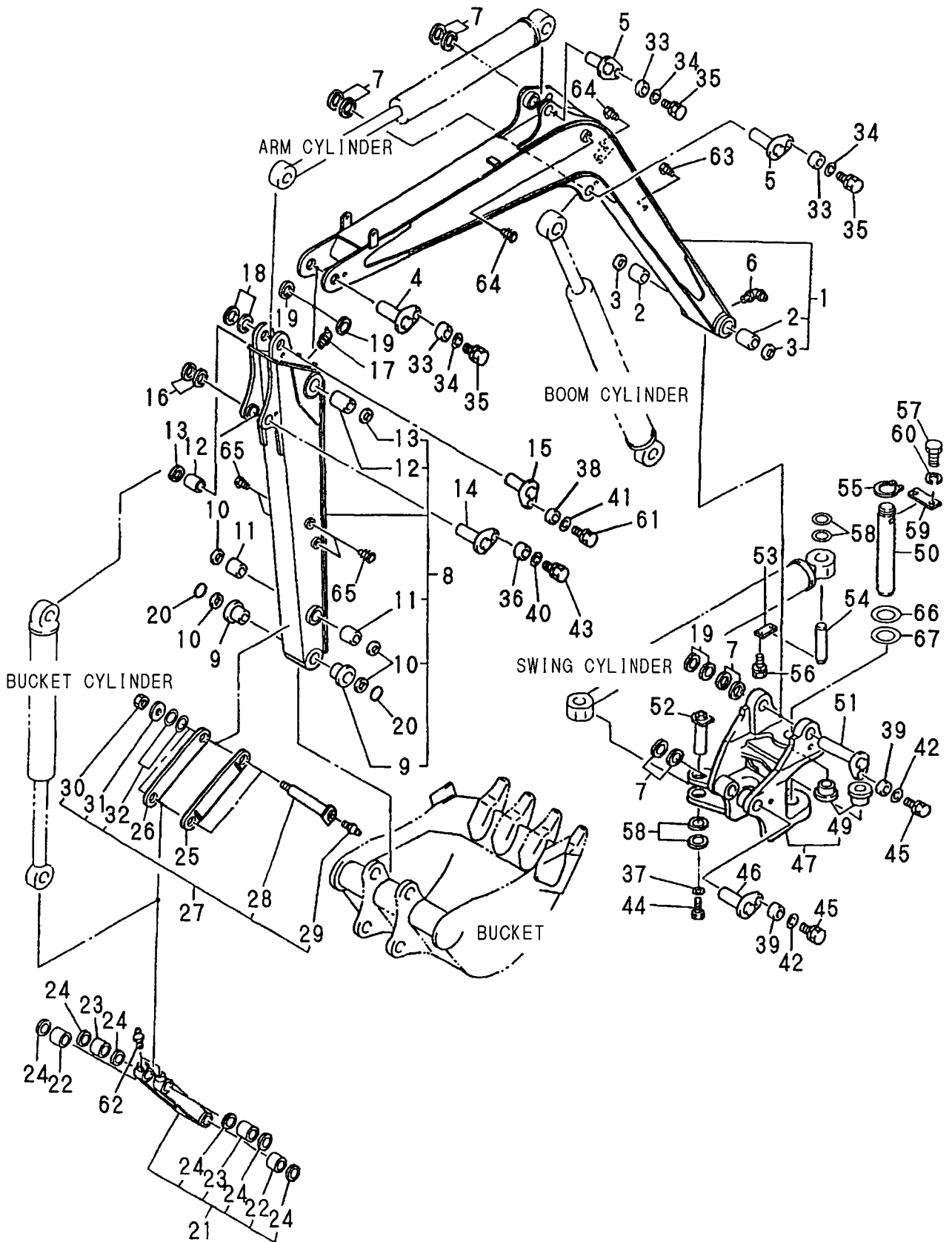
Fig. 49 BOOM & ARM
