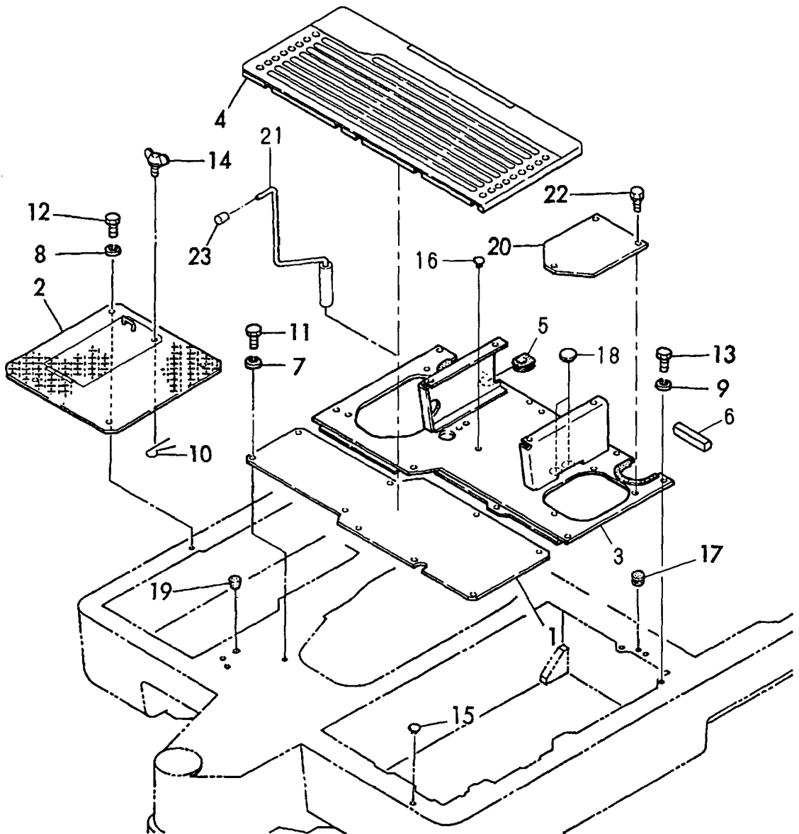
Fig. 20 STEP
