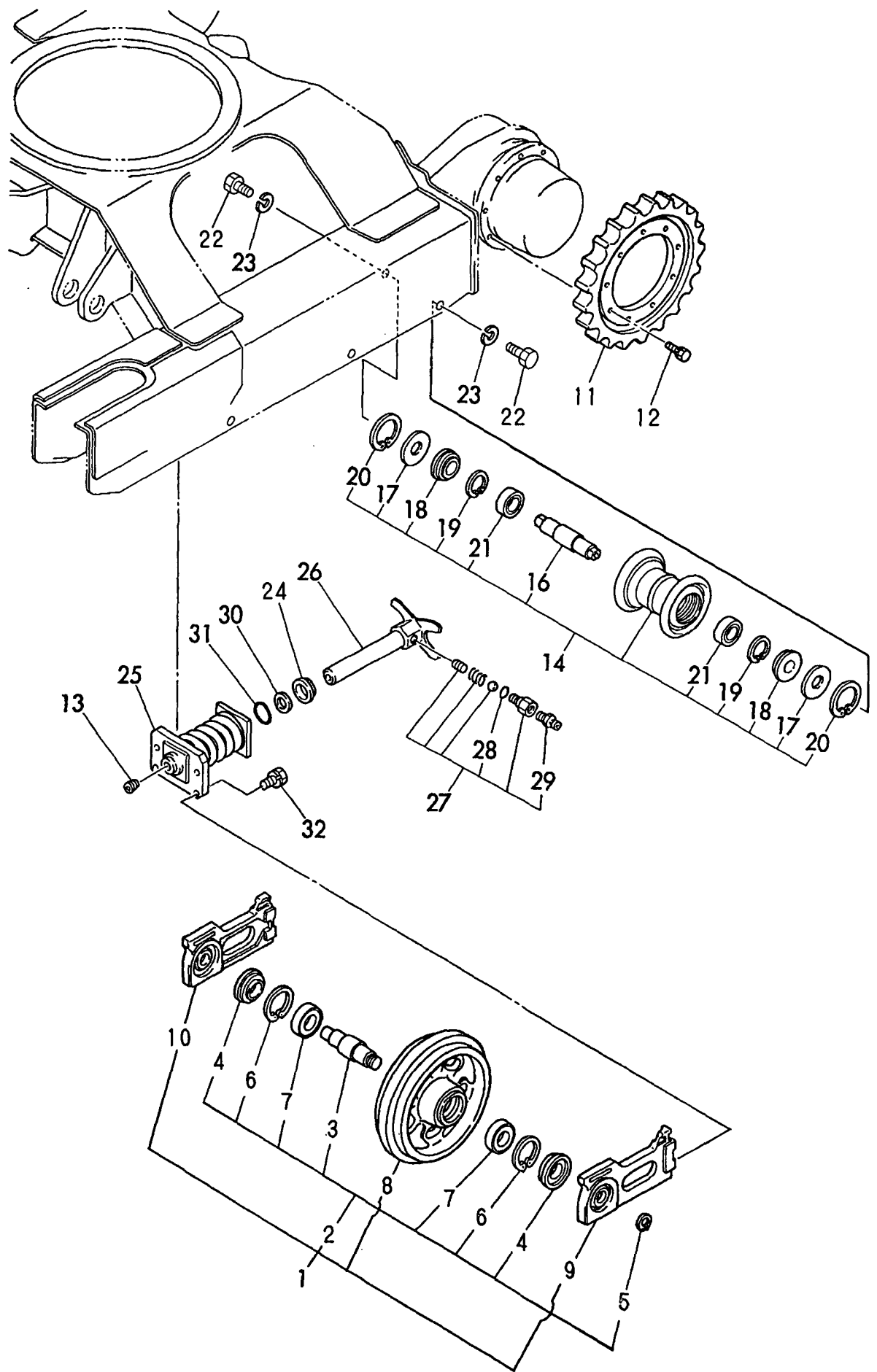
Fig. 11 ROLLER & ADJUST
