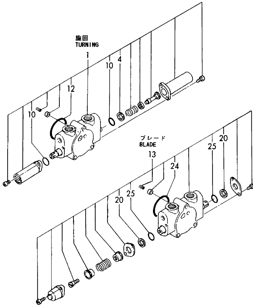
Fig. 68 68 コントロールバルブ(旋回 & ブレード :PTO仕様) CONTROL VALVE(TURNING & BLADE:P.T.O. SPEC.)
