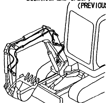
Fig. 84 油圧配管(P.T.O. フレーム :7-メント仕様)(旧形) HYD. OIL PIPING(P.T.O. BOOM:ARM END SPEC.) (PREVIOUS)
