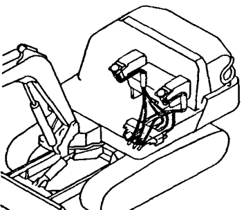
Fig. 92 コントロール配管 (リモコンバルブ～コントロールバルブ :ダイレクト, サイドレバー AS仕様) CONTROL PIPING(REMO.-CON. V.～CON. V.:DIRECT, SIDE LEVER AS SPEC.)
