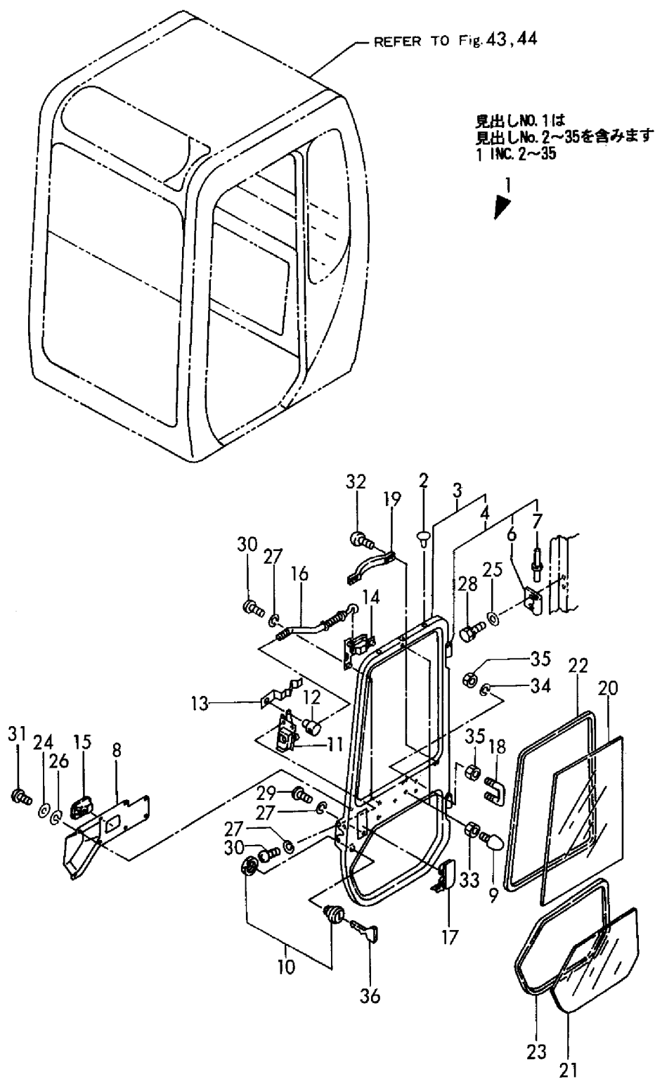
Fig. 45 キャビンドア CABIN DOOR
