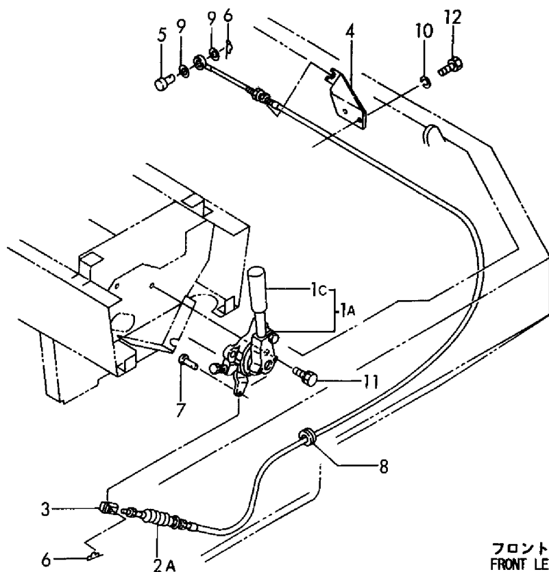
Fig. 11 アクセル(標準仕様) ACCELERATOR(STANDARD SPEC.)
