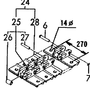
クローラ(370) CRAWLER(370)
