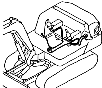
Fig. 90 コントロール配管 (リモコンバルブ～コントロールバルブ :ダイレクト, フロントレバー) CONTROL PIPING (REMO.-CON. V.～CON. V. :DIRECT, FRONT LEVER)
