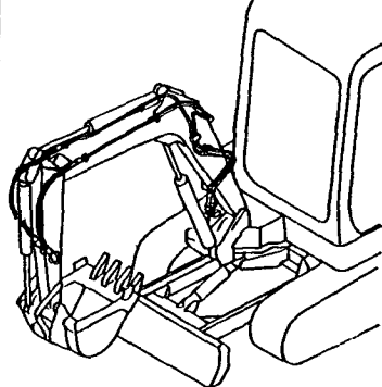
Fig. 86 油圧配管(テレスコピックアーム) HYD. OIL PIPING (TELESCOPIC ARM)
