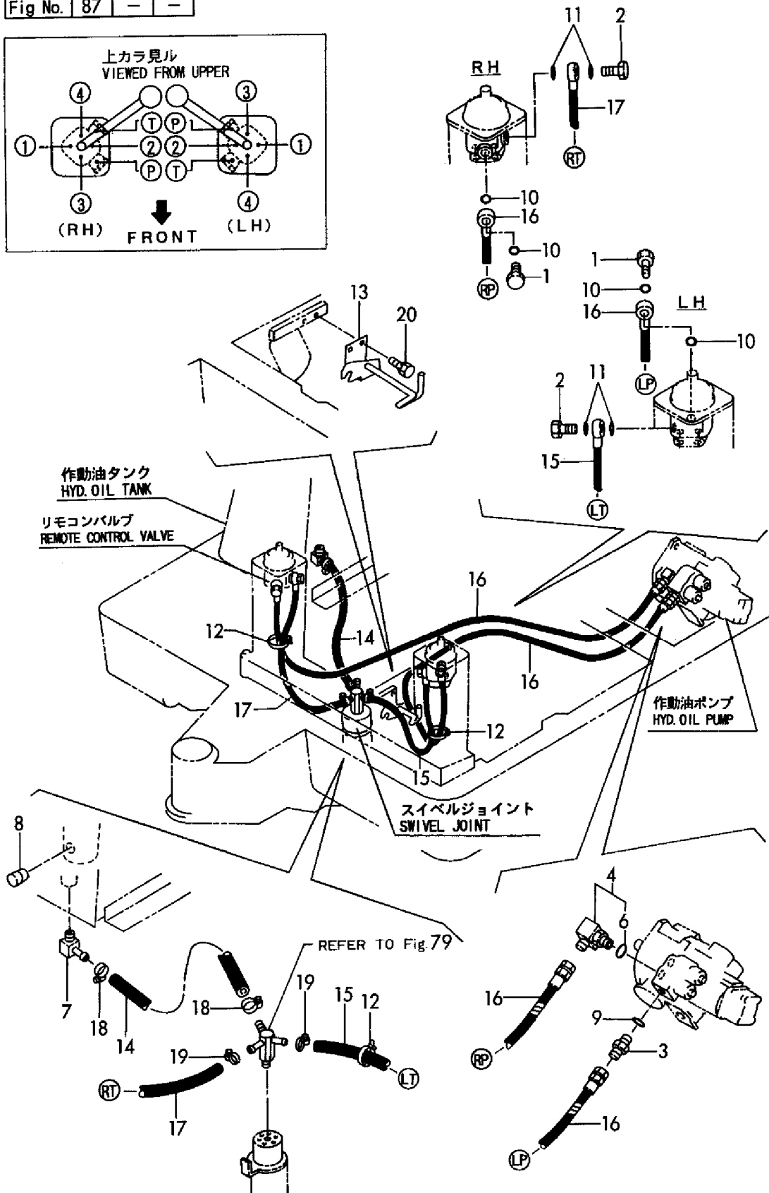
Fig. 87 コントロール配管(ポンプ～リモコンバルブ～リターン :フロントレバー) CONTROL PIPING(PUMP～REMO. -CON. V. ～RETURN :FRONT LEVER)
