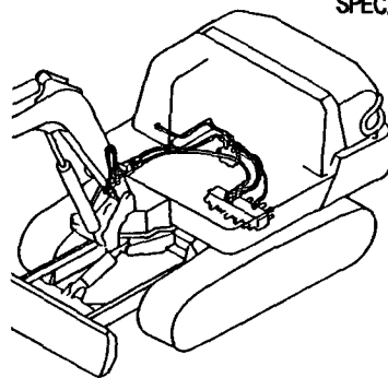
Fig. 82 油圧配管(トラックフレーム) HYD. OIL PIPING (TRACK FRAME)
