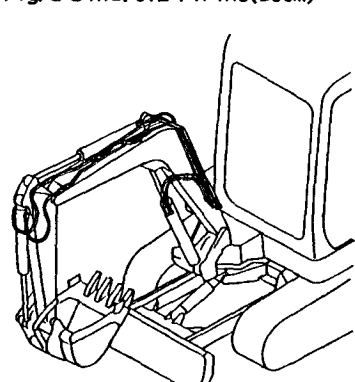
Fig. 83 油圧配管(ブーム) HYD. OIL PIPING(BOOM)
