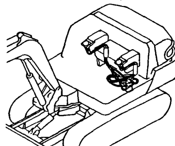
Fig. 94 コントロール配管 (リモコンバルブ～マルチバルブ :4ウェイ, サイドレバー) CONTROL PIPING (REMO.-CON. V.～MULTI V. :4-WAY, SIDE LEVER)
