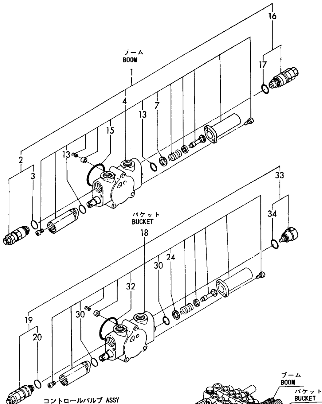
Fig. 67 67 コントロールバルブ(ブーム & バケット:PTO仕様) CONTROL VALVE(BOOM & BUCKET:P.T.O. SPEC.)
