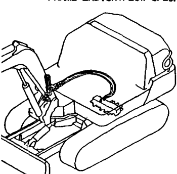
Fig. 80 油圧配管(P.T.O. フレームエンド) (単流仕様) HYD. OIL PIPING(P.T.O., FRAME END:UNIFLOW SPEC.)
