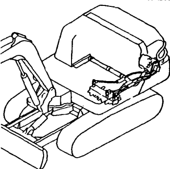
Fig. 76 油圧配管(タンク〜ポンプ) (バルブ) HYD. OIL PIPING(TANK~PUMP ~VALVE)
