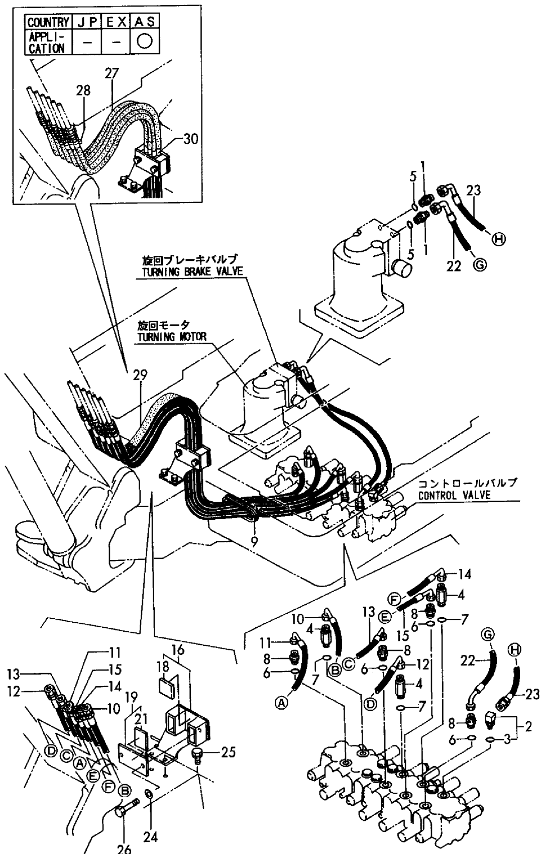
Fig. 77 油圧配管(バルブ～モータ、ブーム) HYD. OIL PIPING (VALVE ~ MOTOR, BOOM)
