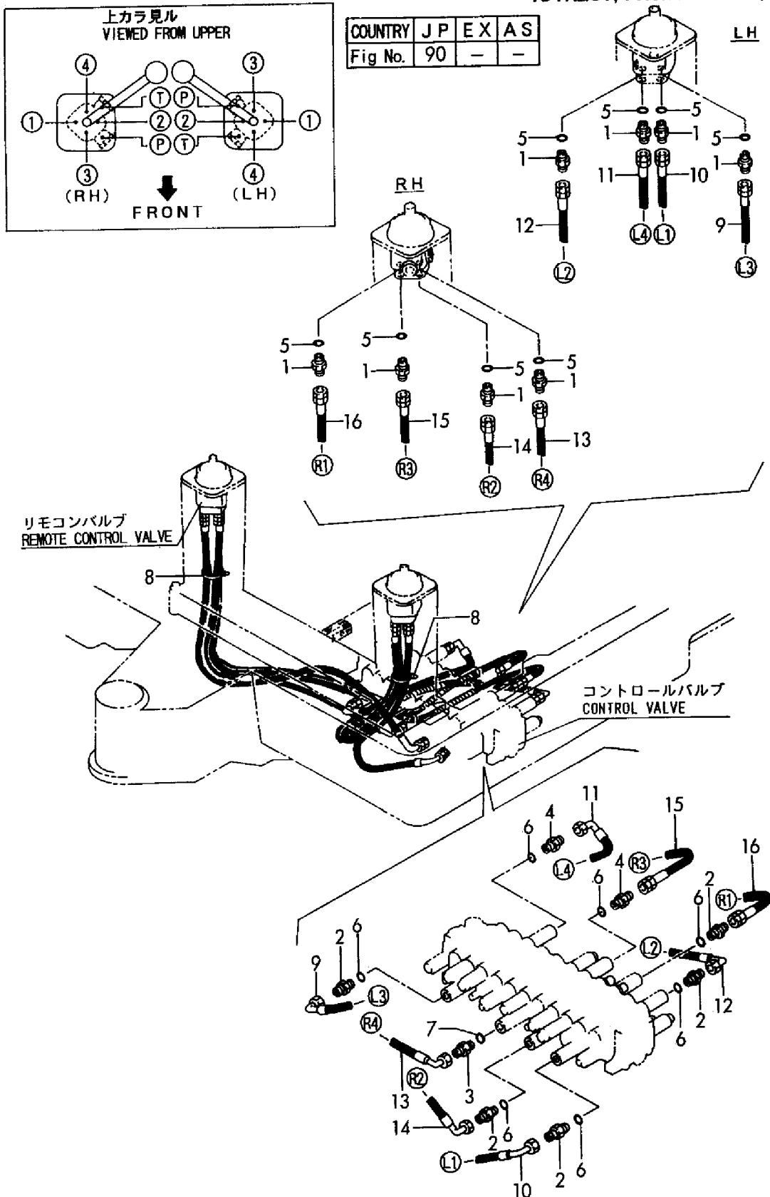
Fig. 90 90 コントロール配管(リモコンバルブ ~コントロールバルブ :ダイレクト, フロントレバー) CONTROL PIPING(REMO. -CON. V. ~CONTROL V. :DIRECT, FRONT LEVER)
