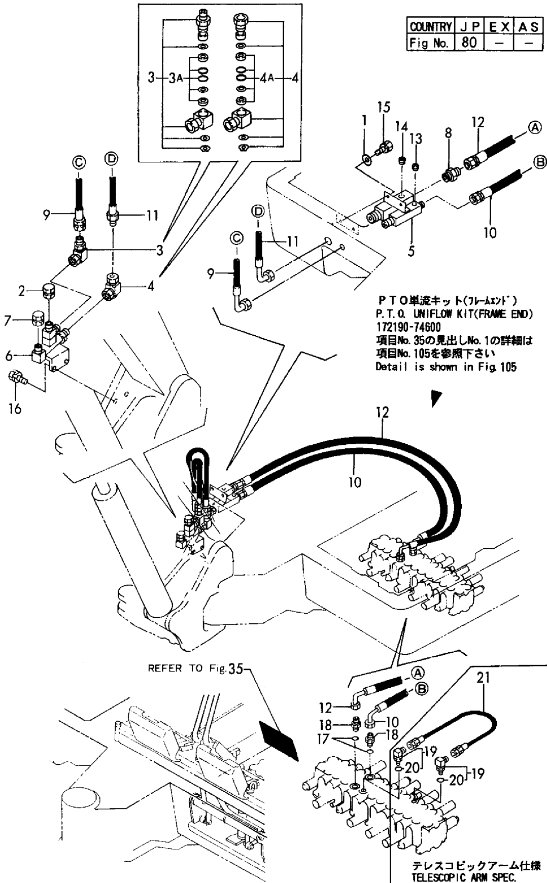
80 油圧配管(PTO, フレーム: 単流仕様) Fig. 80 HYD. OIL PIPING(P. T. O., FRAME END: UNIFLOW SPEC.)
