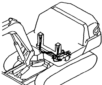
Fig. 90 コントロール配管 (リモコンバルブ～コントロールバルブ :ダイレクト, フロントレバー) CONTROL PIPING (REMO.-CON. V.～CON. V. :DIRECT, FRONT LEVER)
