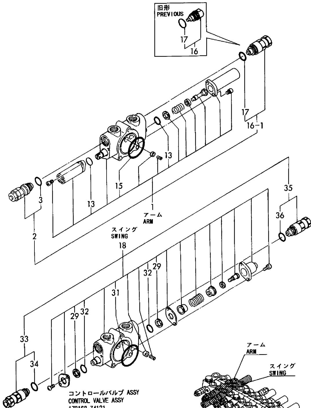
Fig. 66 66 コントロールバルブ(アーム & スイング :PTO仕様) CONTROL VALVE(ARM & SWING:P. T. O. SPEC.)
