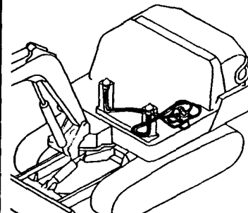
Fig. 94 コントロール配管 (リモコンバルブ～マルチバルブ :4ウェイ, サイドレバー) CONTROL PIPING (REMO.-CON. V.～MULTI V. :4-WAY, SIDE LEVER)
