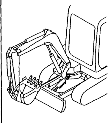
Fig. 55 スライドシリンダ (テレスコピックアーム) SLIDE CYLINDER (TELESCOPIC ARM)
