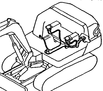
Fig. 88 コントロール配管(ポンプ～ リモコンバルブ～リターン :サイドレバー JP, EX仕様) CONTROL PIPING(PUMP～ REMO.-CON. VALVE～RETURN :SIDE LEVER JP, EX仕様)
