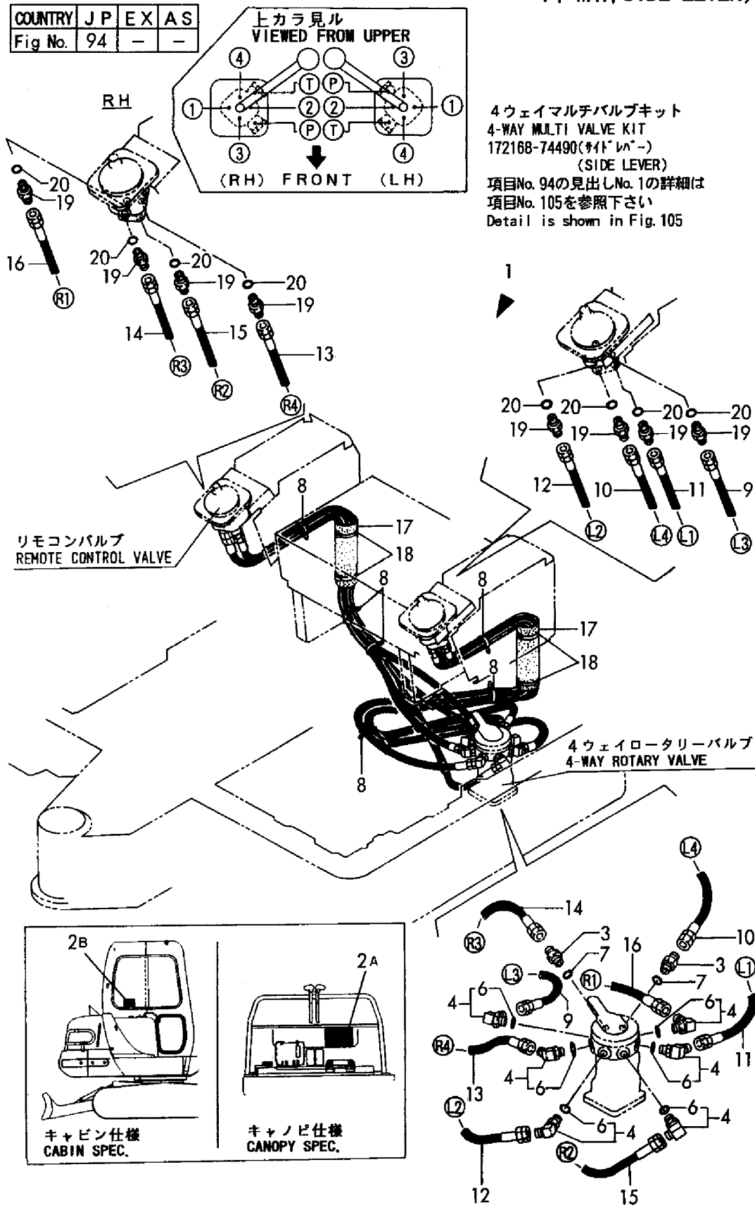
Fig. 94 94 コントロール配管(リモコンバルブ ~マルチバルブ) :4ウェイ, サイドレバー-) CONTROL PIPING(REMO. -CON. V. ~MULTI V. :4-WAY, SIDE LEVER)
