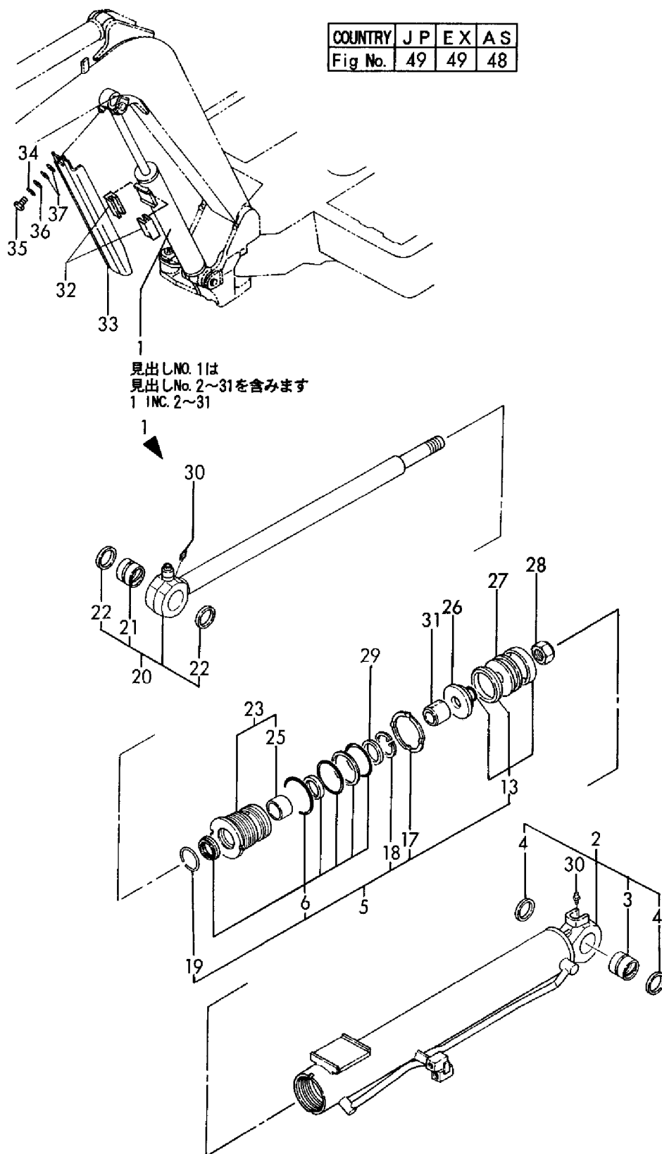
Fig. 49 ブームシリンダ UZ(キャピ°) BOOM CYLINDER UZ(CANOPY)
