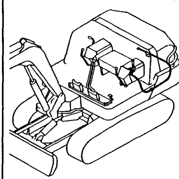
Fig.11 アクセル(標準仕様) ACCELERATOR(STANDARD SPEC.)
