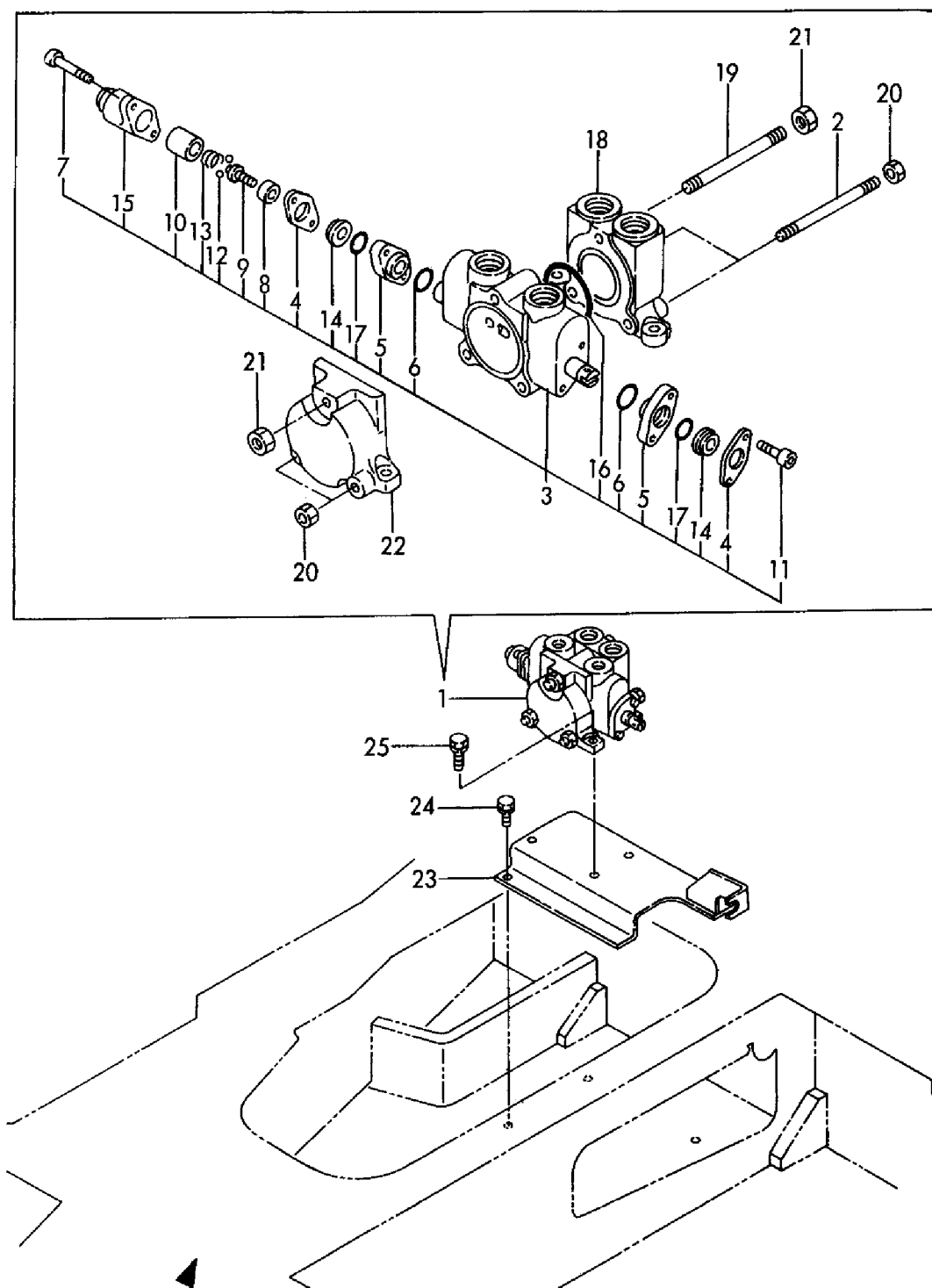
Fig. 74 P.T.O.バルブ(合流) P.T.O. VALVE(CONFLUENCE)
