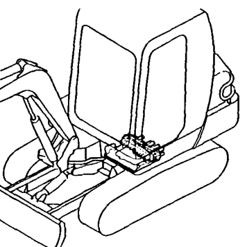
Fig.64 コントロールバルブ (Pポート & バック台:PTO仕様) CONTROL VALVE(P PORT & VALVE STAND:P.T.O. SPEC.)
