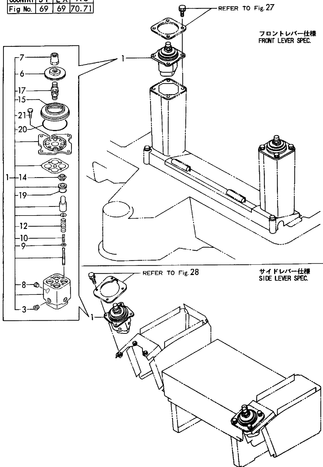
Fig. 69 リモコンバルブ(JP, EX仕様) REMOTE CONTROL VALVE(JP, EX SPEC.)
