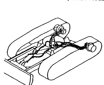
Fig. 82 油圧配管(トラックフレーム) HYD. OIL PIPING (TRACK FRAME)
