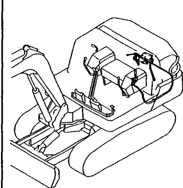
Fig.12 アクセル(ワンタッチ仕様) ACCELERATOR(ONE TOUCH DECEL SPEC.)
