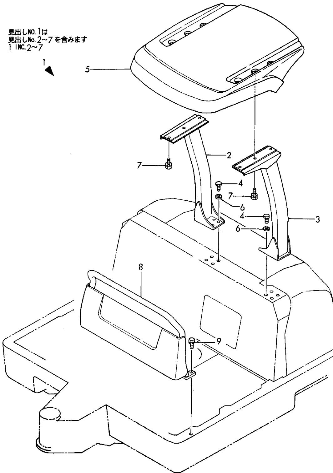
Fig. 46 キャノピ CANOPY
