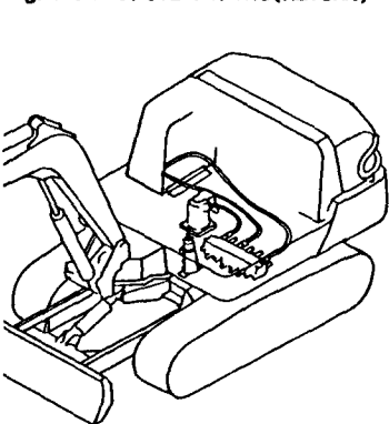
Fig. 79 油圧配管(リターン) HYD. OIL PIPING(RETURN)
