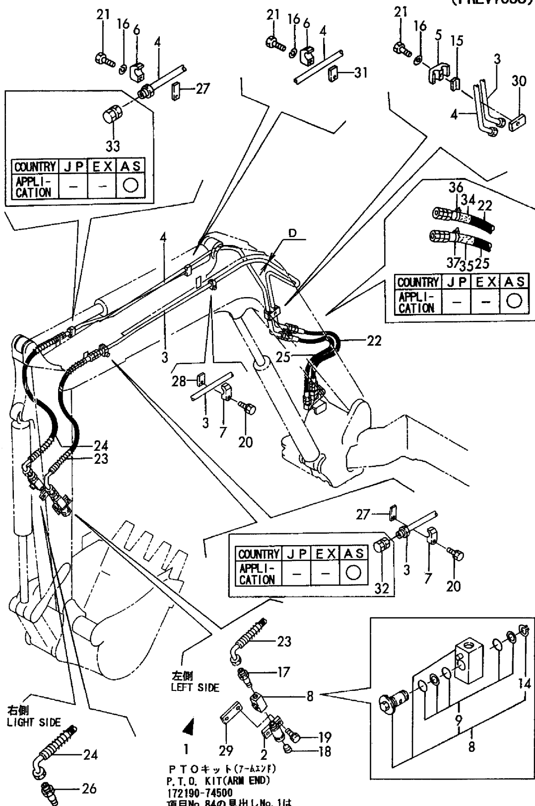
Fig. 84 油圧配管(PTO 7-4 アームエンド仕様)(旧形) HYD. OIL PIPING(P. T. O. BOOM:ARM END SPEC.) (PREVIOUS)
