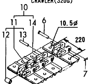
クローラ(320G) CRAWLER(320G)
