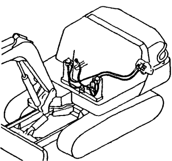
Fig. 88 コントロール配管(ポンプ～ リモコンバルブ～リターン :サイドレバー JP, EX仕様) CONTROL PIPING(PUMP～ REMO.-CON. VALVE～RETURN :SIDE LEVER JP, EX仕様)
