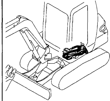
Fig. 96 コントロール配管 (マルチバルブ ~ コントロールバルブ: 4ウェイ) CONTROL PIPING (MULT V. ~ CONTROL V.: 4-WAY)
