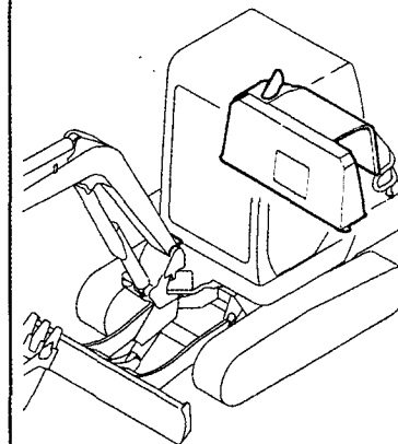
Fig. 48 キャビン (本体 & 付属) CABIN (BODY & FITTING PART)
