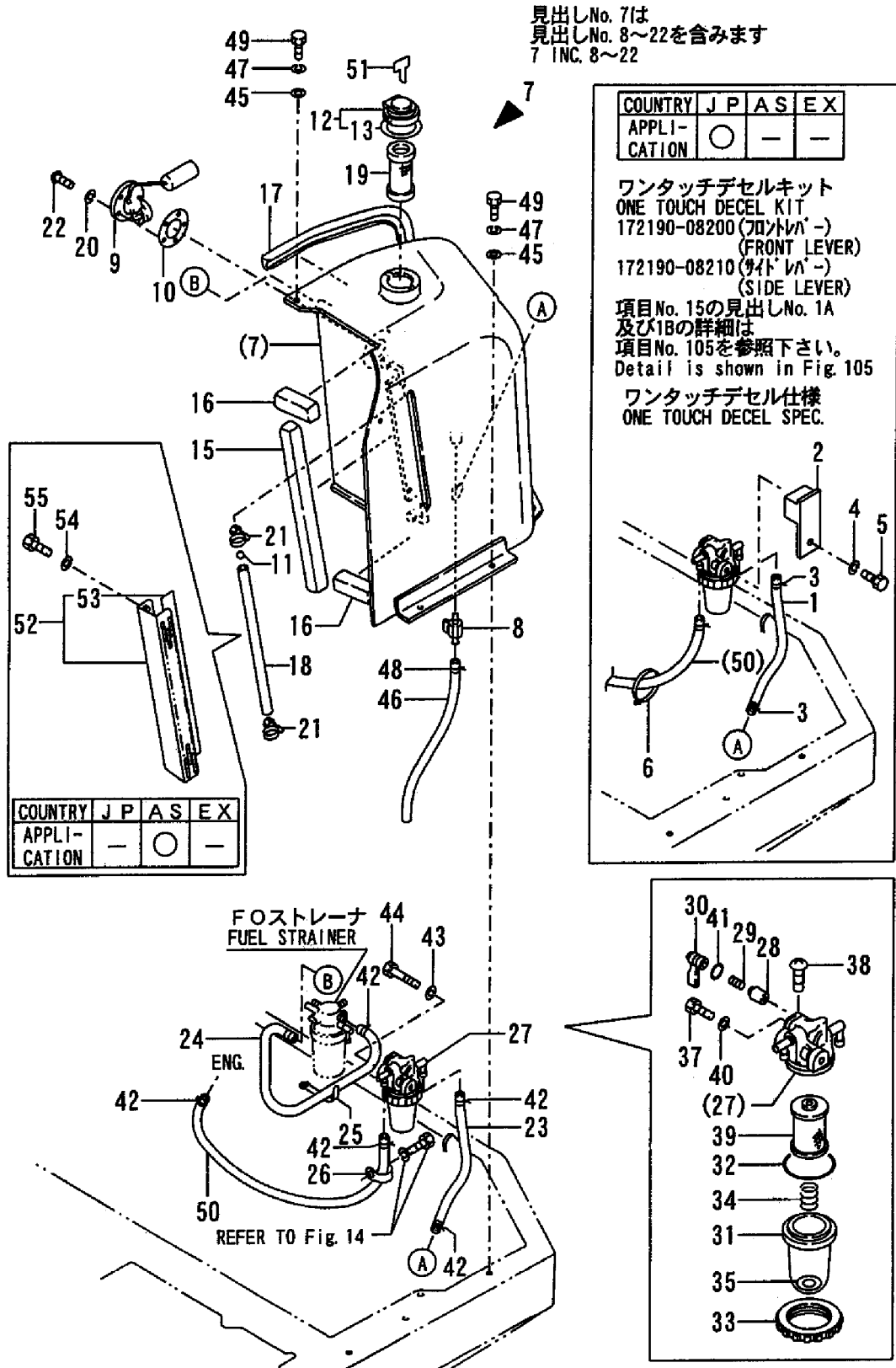
Fig. 18 燃料タンク & 燃料パイプ FUEL TANK & FUEL LINE
