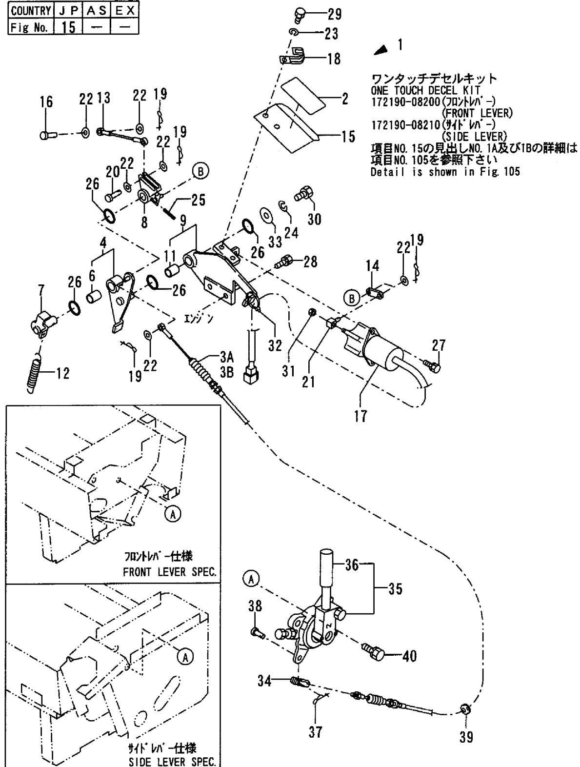
Fig. 15 アクセル(ワンタッチセル仕様) ACCELERATOR LEVER (ONE TOUCH DECEL SPEC.)
