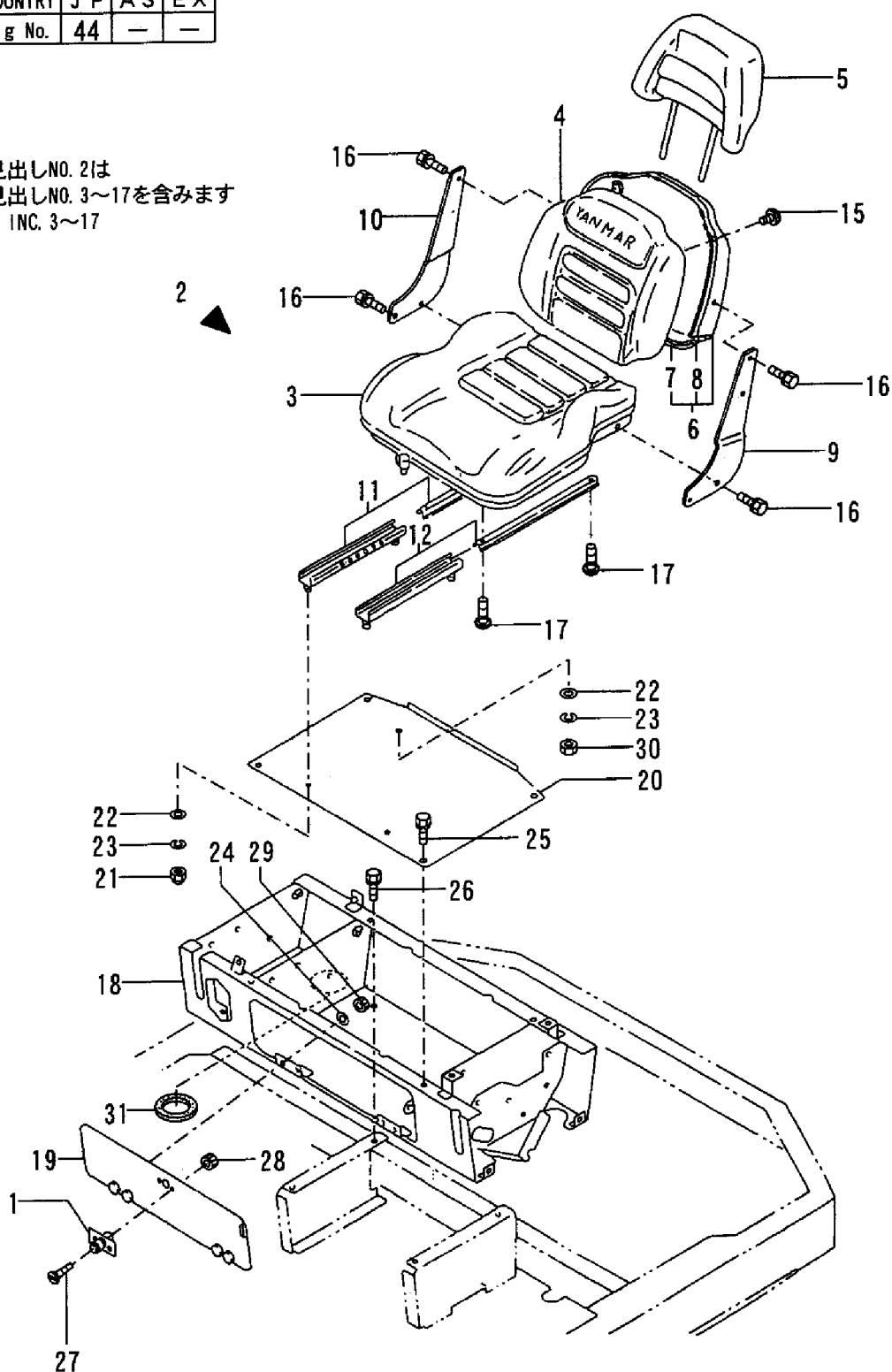
Fig. 44 シート & シートマウント(フロントバ-) SEAT & SEAT MOUNT(FRONT LEVER)
