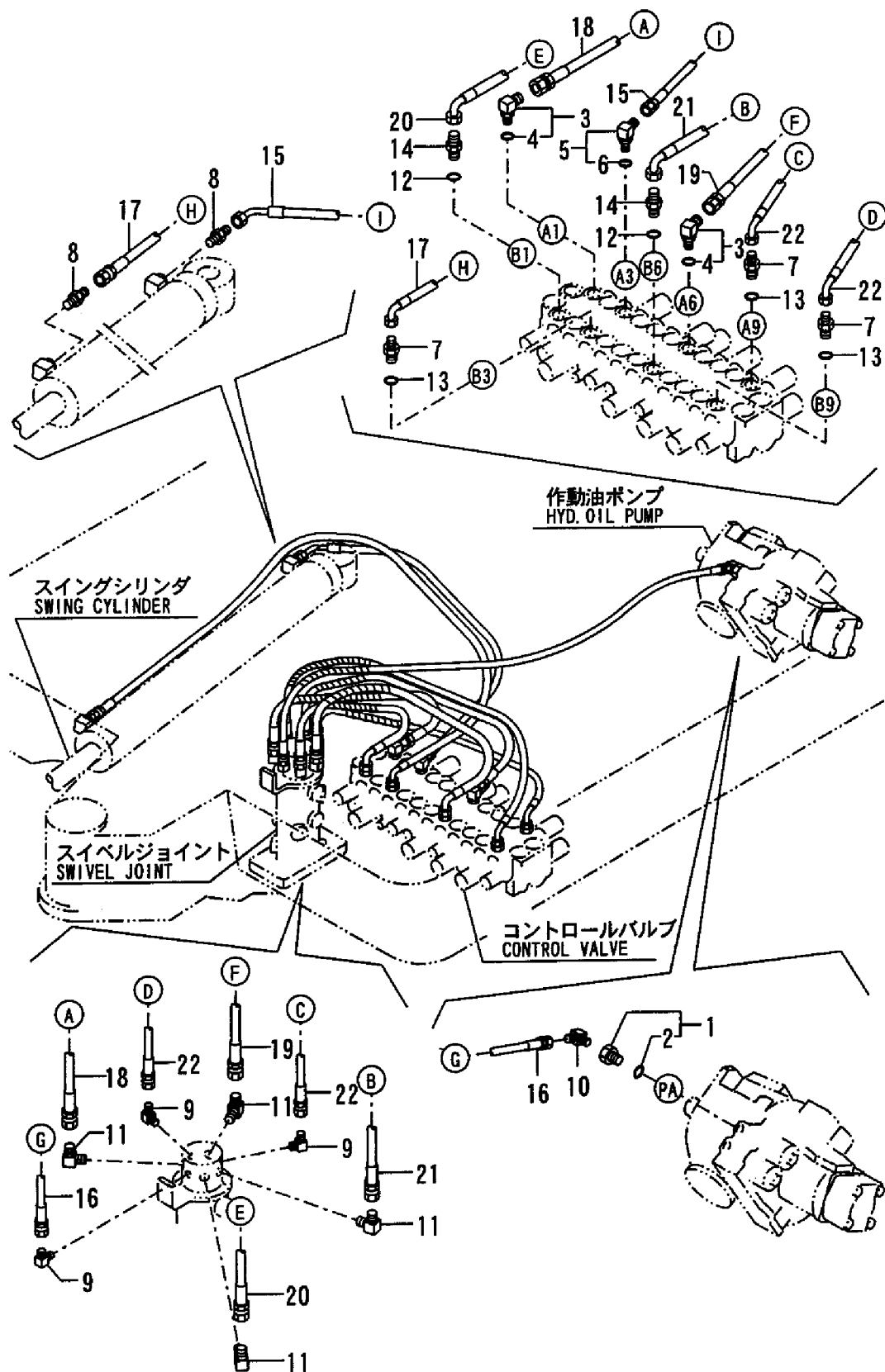
Fig. 81 油圧配管(バルブ ~スイベル, スイング) HYD. OIL PIPING (VALVE ~ SWIVEL, SWING)
