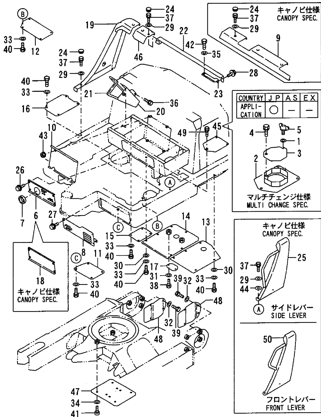
Fig. 40 フレームカバー FRAME COVER
