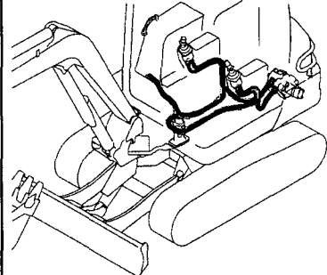
Fig. 91 コントロール配管 (リモコンバルブ ~ コントロールバルブ: ダイレクト, フロントレバー) CONTROL PIPING (REMOTE-CONTROL V. ~ CONTROL V.: DIRECT, FRONT LEVER)
