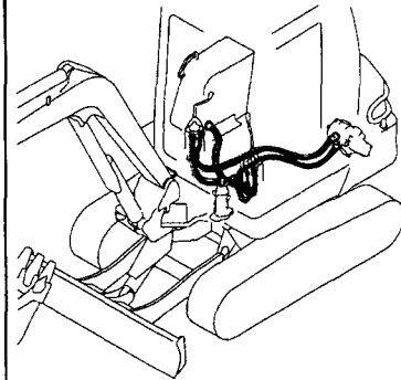
Fig. 88 コントロール配管 (ポンプ ~ リモコンV. ~ リターン: フロントレバー) CONTROL PIPING (PUMP ~ REMOTE CONTROL V. ~ RETURN: FRONT LEVER)
