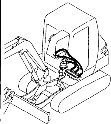
Fig. 83 油圧配管 (PTO, フレームエンド : 単流仕様) HYD. OIL PIPING (P. T. O., FRAME END: UNIFLOW SPEC.)
