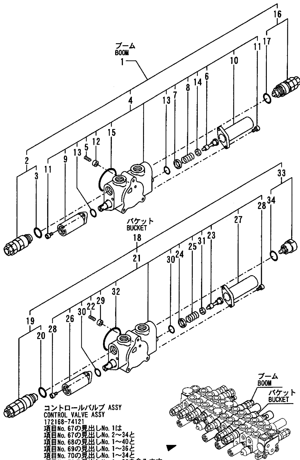
Fig. 70 70 コントロールバルブ(ブーム & バケット:PTO仕様) CONTROL VALVE (BOOM & BUCKET: P. T. O. SPEC.)
