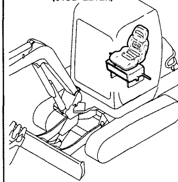
Fig. 46 シートマウント (サイドレバー) (AS) SEAT MOUNT (SIDE LEVER) (AS)
