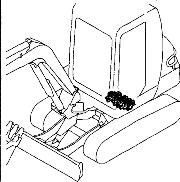
Fig. 71 コントロールバルブ (旋回 & ブレード: PTO仕様) CONTROL VALVE (TURNING & BLADE: P. T. O. SPEC.)
