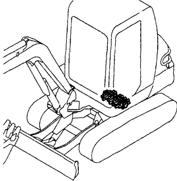
Fig. 66 コントロールバルブ (旋回 & ブレード: 標準仕様) CONTROL VALVE (TURNING & BLADE : STANDARD SPEC.)
