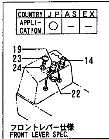
Fig. 24 電装品(キャビン専用) ELECTRIC PART (CABIN)
