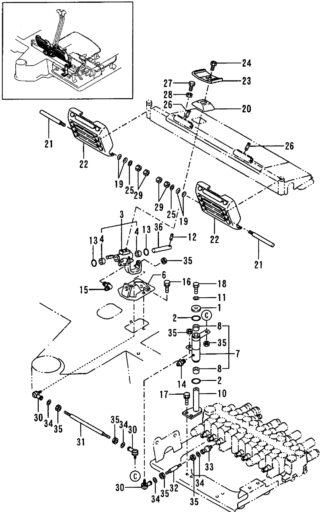
Fig. 34 操縦装置(スイング) CONTROL EQUIPMENT (SWING)
