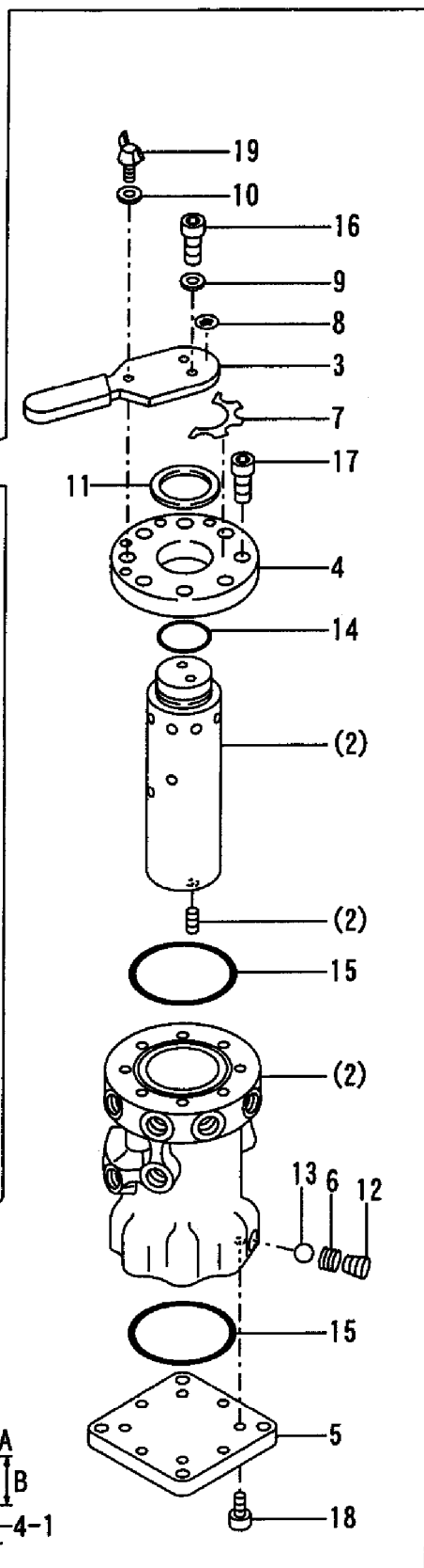
Fig. 75 4ウェイロータリーバルブ(マルチチェンジ仕様) 4-WAY ROTARY VALVE (MULTI CHANGE SPEC.)
