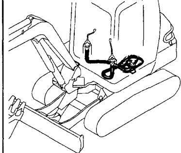
Fig. 95 コントロール配管 (リモコンバルブ ~ マルチバルブ: 4ウェイ, サイドレバー) CONTROL PIPING (REMOTE-CONTROL V. ~ MULTI V.: 4-WAY SIDE LEVER)
