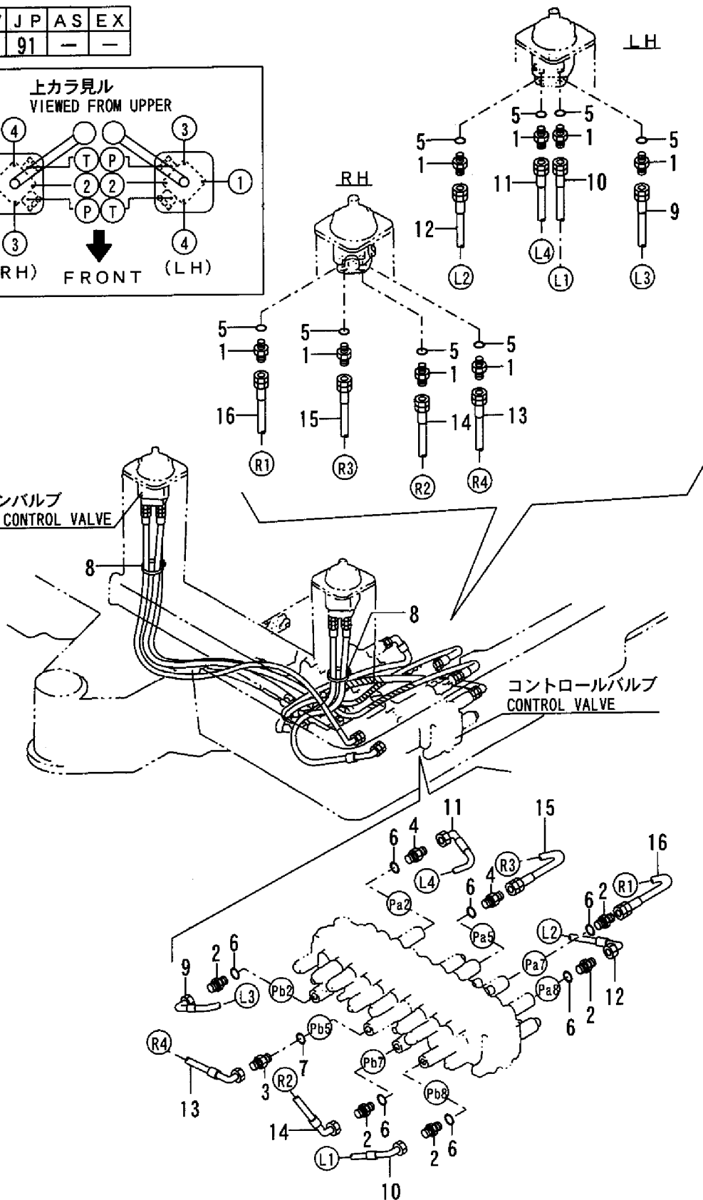
Fig. 91 コントロール配管 (リモコンバルブ ~ コントロールバルブ : ダイレクト, フロントレバー) CONTROL PIPING (REMOTE CONTROL V. ~ CONTROL V. : DIRECT, FRONT LEVER)
