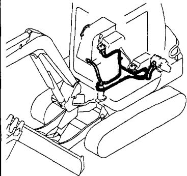
Fig. 90 コントロール配管 (ポンプ ~ リモコンV. ~ リターン: サイドレバー) (AS) CONTROL PIPING (PUMP ~ REMOTE CONTROL V. ~ RETURN: SIDE LEVER) (AS)
