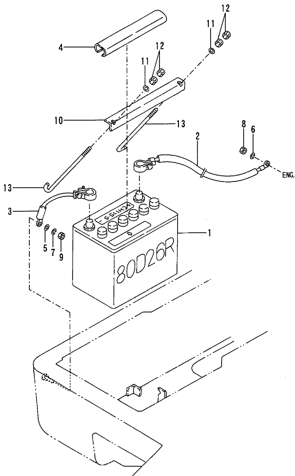
Fig. 19 バッテリー BATTERY
