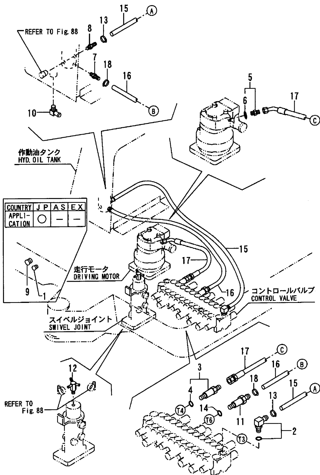
Fig. 82 油圧配管(リターン) HYD. OIL PIPING(RETURN)
