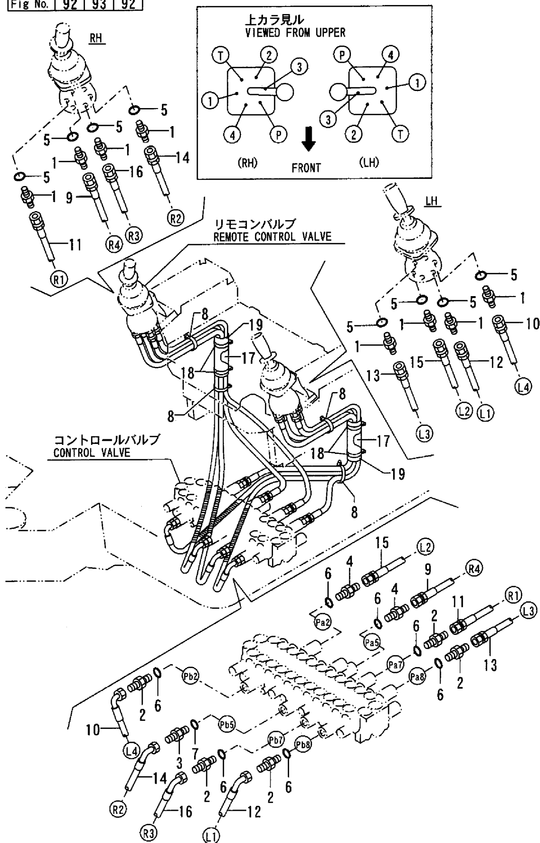
Fig. 93 コントロール配管 (リモコンバルブ ~ コントロールバルブ : ダイレクト, サイドレバー) (AS) CONTROL PIPING (REMOTE CONTROL V. ~ CONTROL V. : DIRECT, SIDE LEVER) (AS)
