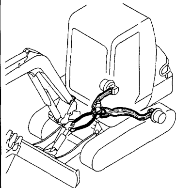
Fig. 86 油圧配管 (ブーム) HYD. OIL PIPING (BOOM)
