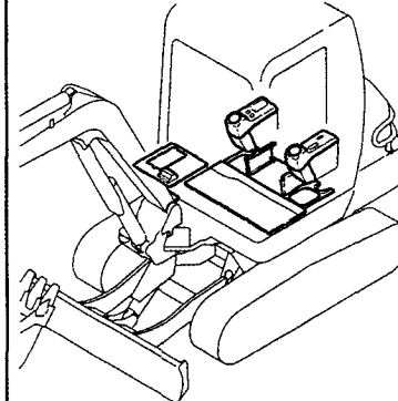
Fig. 44 シート & シートマウント (フロントレバー) SEAT & SEAT-MOUNT (FRONT LEVER)
