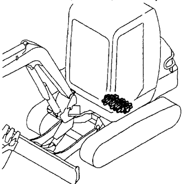
Fig. 68 コントロールバルブ (走行 & PTO: PTO仕様) CONTROL VALVE (DRIVE & P. T. O. : P. T. O. SPEC.)
