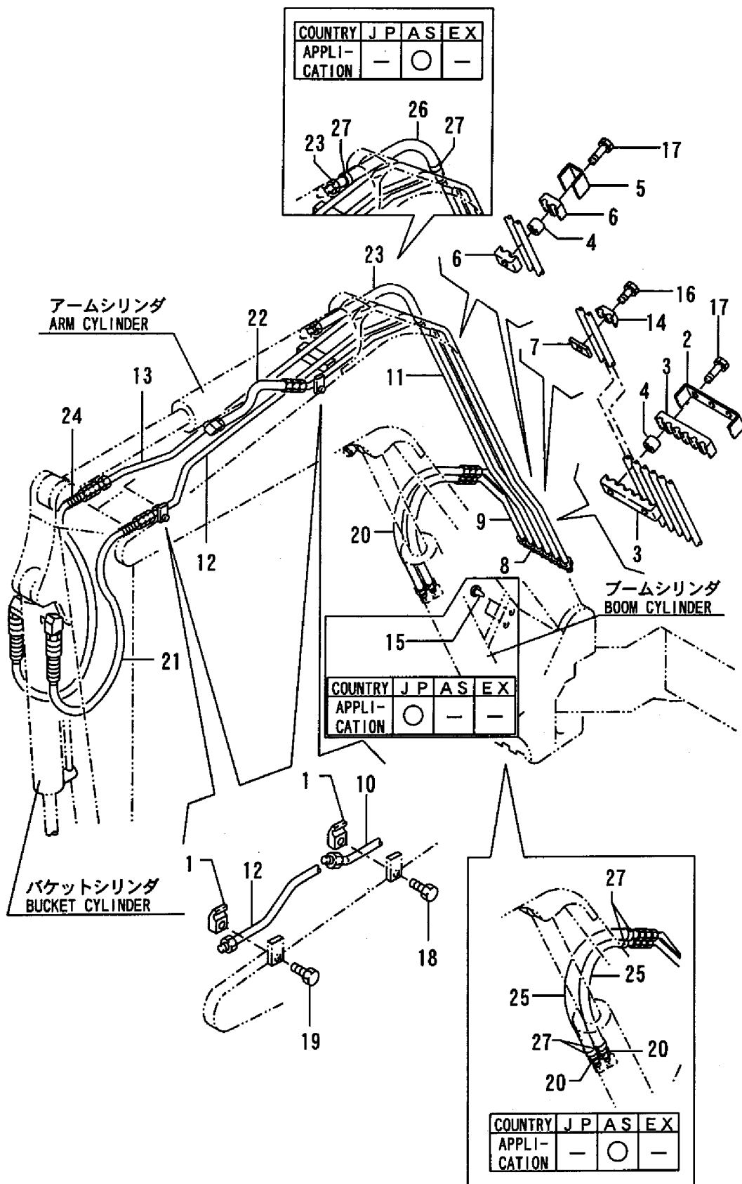
Fig. 86 油圧配管(ブーム) HYD. OIL PIPING (BOOM)
