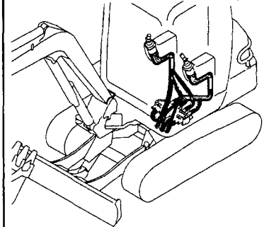
Fig. 94 コントロール配管 (リモコンバルブ ~ マルチバルブ: 4ウェイ, フロントレバー) CONTROL PIPING (REMOTE-CONTROL V. ~ MULTI V.: 4-WAY FRONT LEVER)
