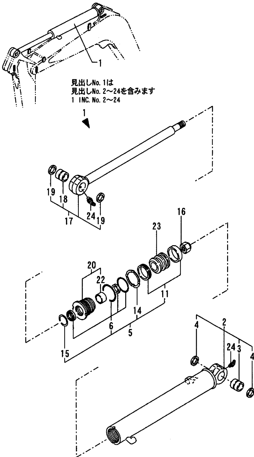
Fig. 55 アームシリンダ ARM CYLINDER
