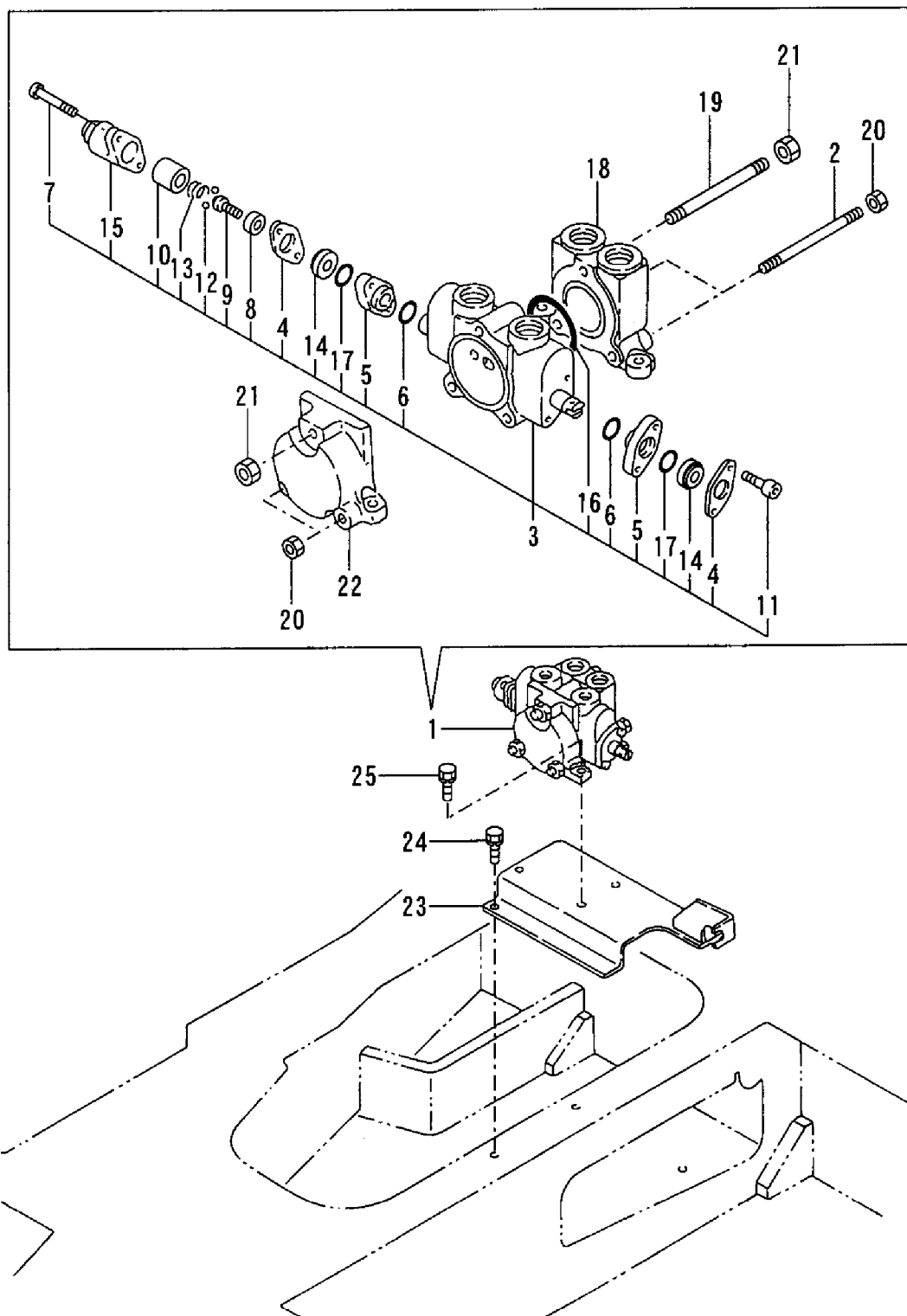
Fig. 77 P.T.O. VALVE (CONFLUENCE)
