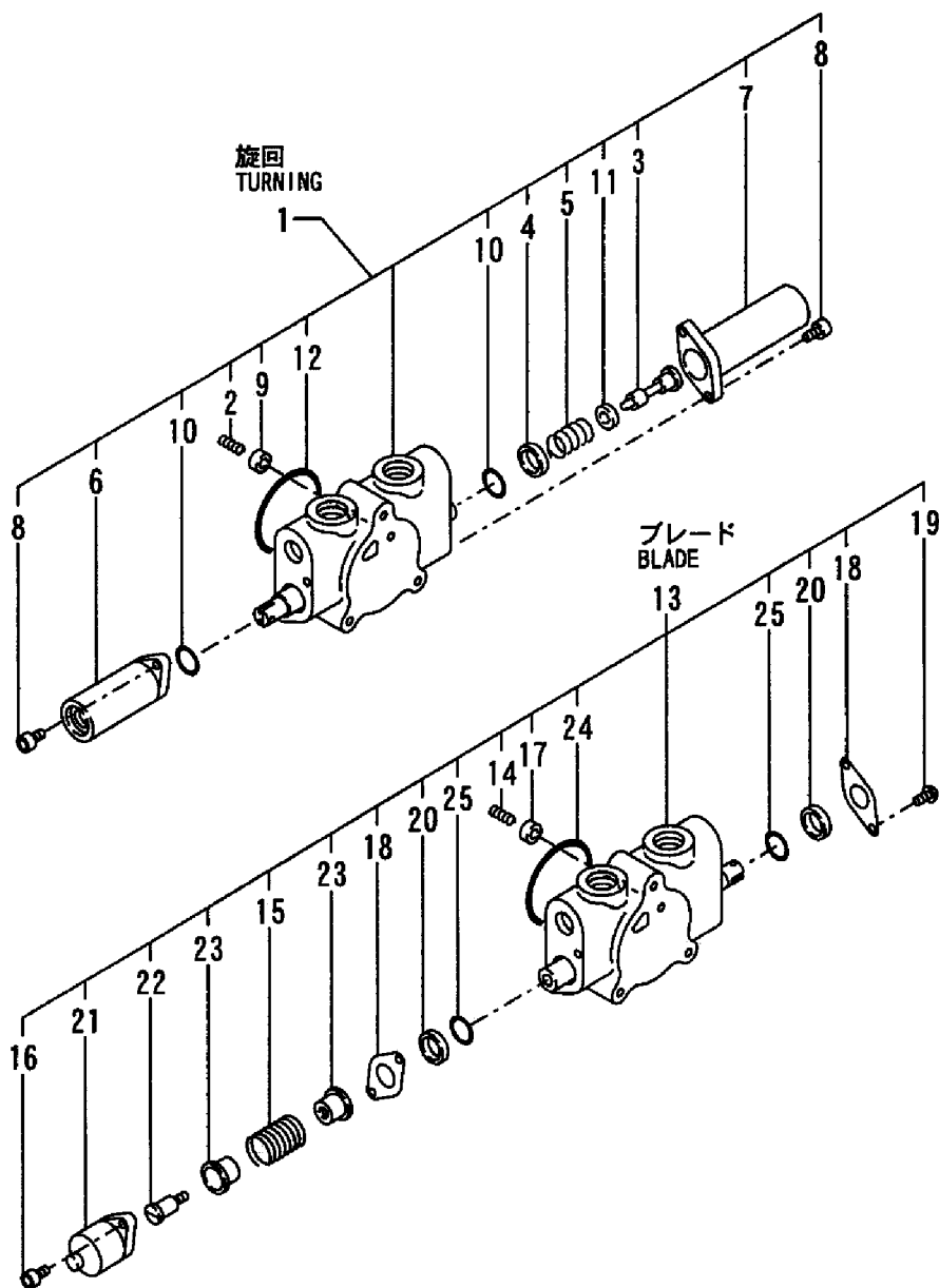
Fig. 71 71 コントロールバルブ(旋回 & ブレード :PTO仕様) CONTROL VALVE(TURNING & BLADE:P. T. O. SPEC.)
