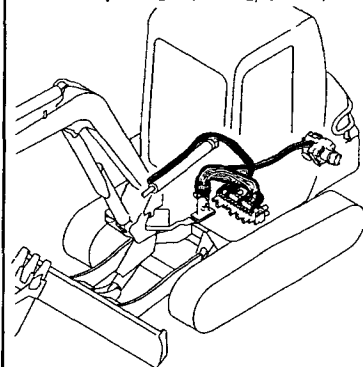
Fig. 82 油圧配管 (リターン) HYD. OIL PIPING (RETURN)
