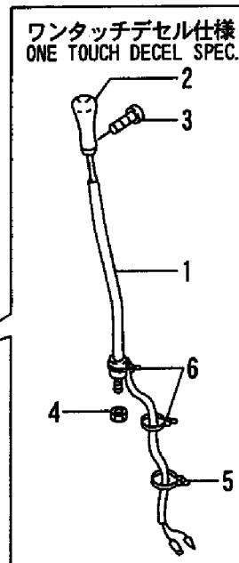
Fig. 30 操縦装置 (レバー & スタンド : フロントレバー) CONTROL EQUIPMENT (LEVER & STAND : FRONT LEVER)
