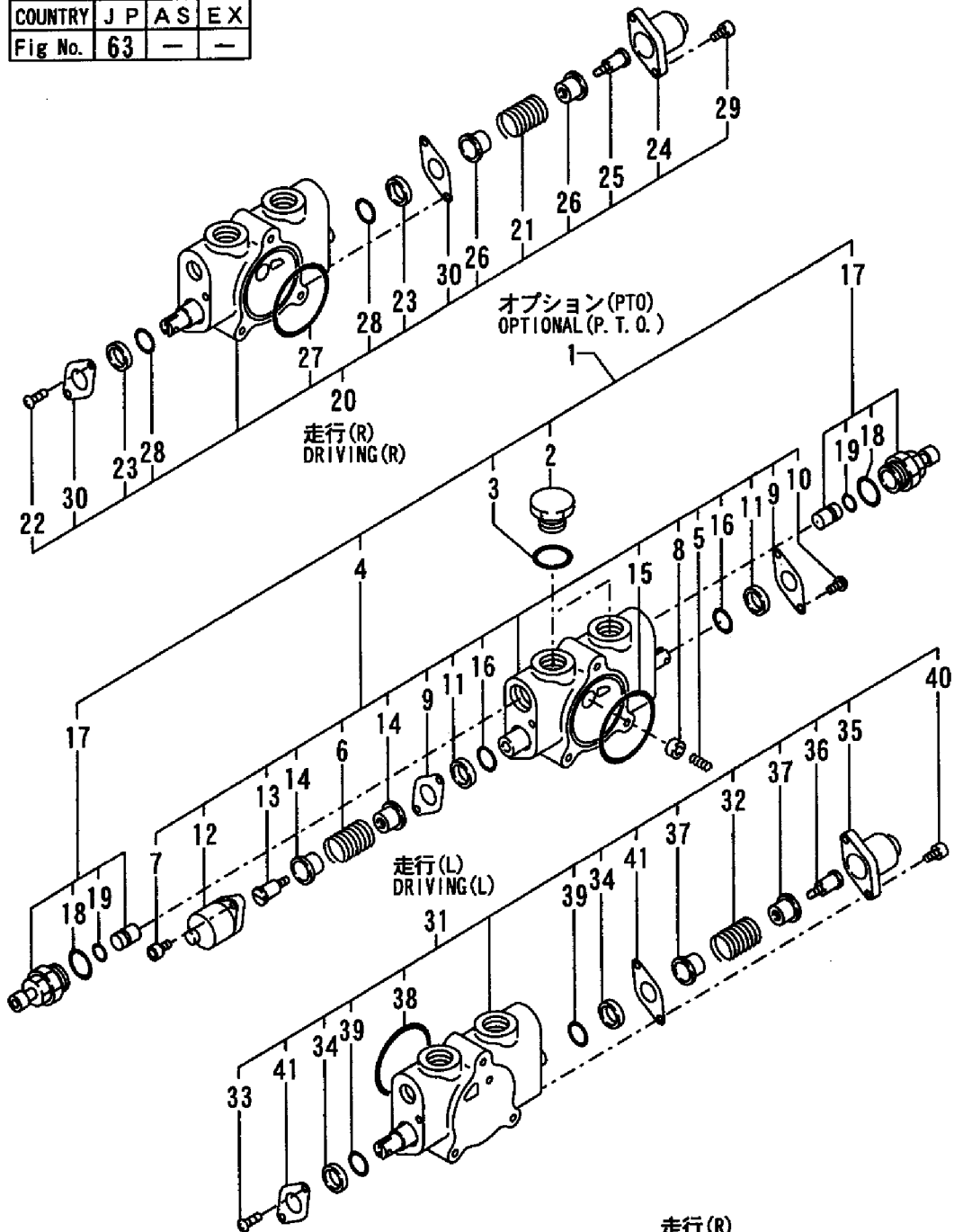
Fig. 63 63 コントロールバルブ(走行 & PTO:標準仕様) CONTROL VALVE (DRIVE & P. T. O. : STANDARD SPEC.)
