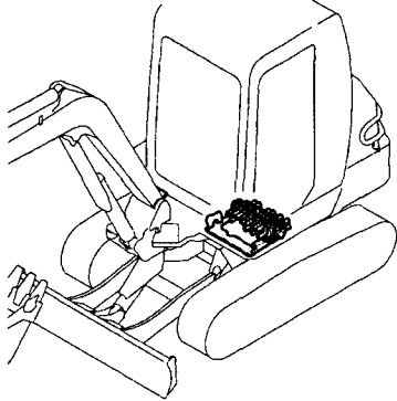
Fig. 63 コントロールバルブ (走行 & PTO:標準仕様) CONTROL VALVE (DRIVE & P. T. O : STANDARD SPEC.)
