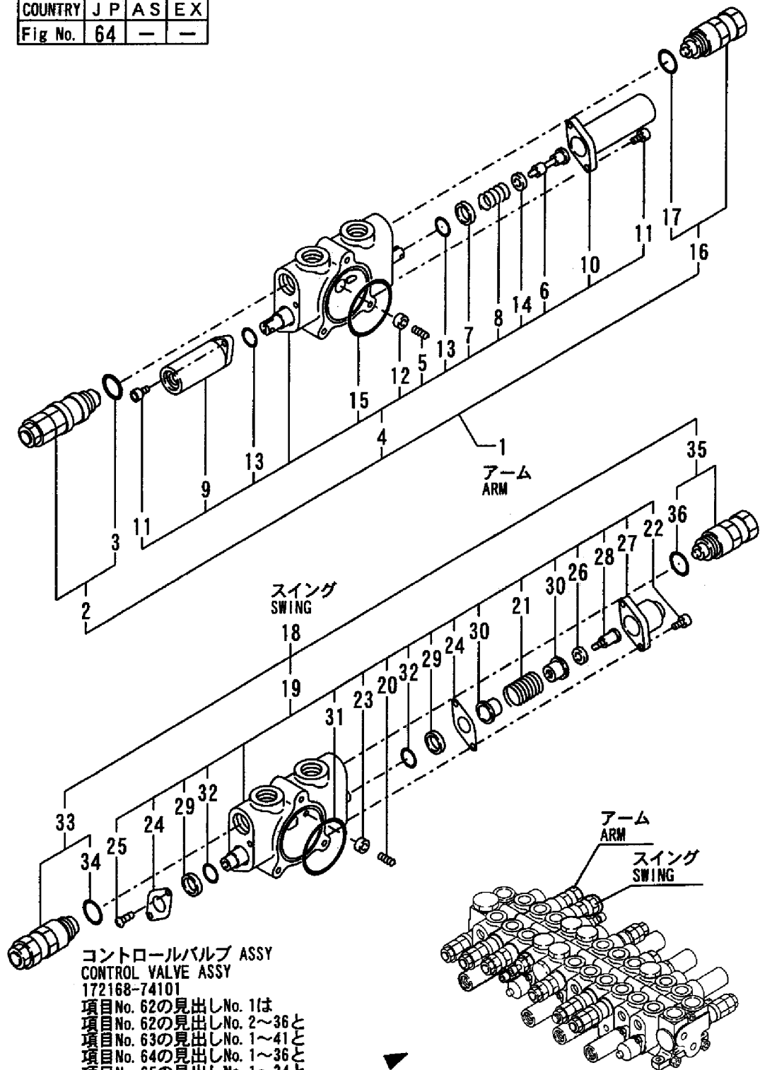
Fig. 64 64 コントロールバルブ(アーム & スイング:標準仕様) CONTROL VALVE (ARM & SWING: STANDARD SPEC.)
