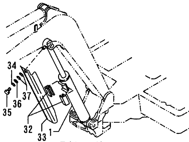
Fig. 54 ブームシリンダ(キャピ°) BOOM CYLINDER (CANOPY)
