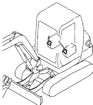
Fig. 72 リモコンバルブ REMOTE CONTROL VALVE
