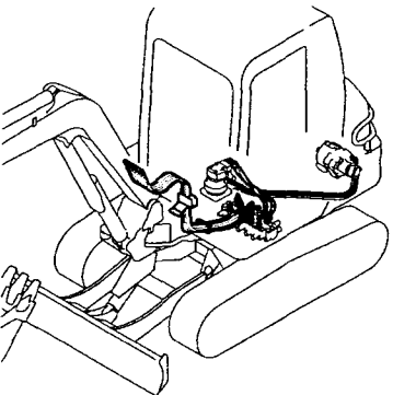
Fig. 80 油圧配管 (ポンプ、バルブ～モータ、ブーム) HYD. OIL PIPING (PUMP, VALVE～MOTOR, BOOM)
