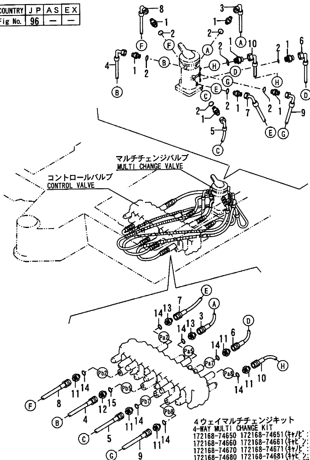
Fig. 96 96 コントロール配管(マルチバルブ ~コントロールバルブ :4ウェイ) CONTROL PIPING(MULTI V. ~CONTROL V. :4-WAY)
