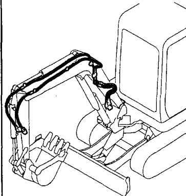
Fig. 88 コントロール配管 (ポンプ ~ リモコンV. ~ リターン: フロントレバー) CONTROL PIPING (PUMP ~ REMOTE CONTROL V. ~ RETURN: FRONT LEVER)
