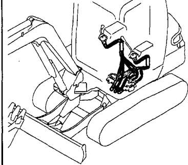
Fig. 92 コントロール配管 (リモコンバルブ ~ コントロールバルブ: ダイレクト, サイドレバー) CONTROL PIPING (REMOTE-CONTROL V. ~ CONTROL V.: DIRECT, SIDE LEVER)
