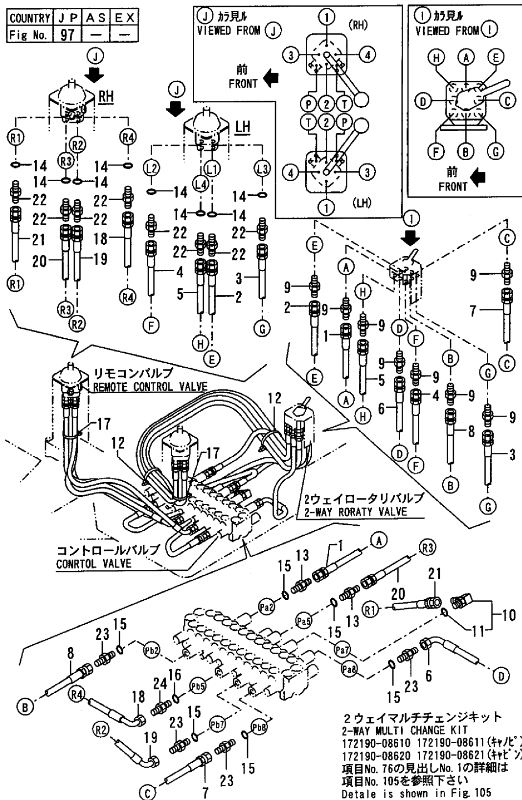
Fig. 97 97 コントロール配管 (マルチチェンジ : 2ウェイ, フロントレバー) CONTROL PIPING (MULTI CHANGE: 2-WAY, FRONT LEVER)
