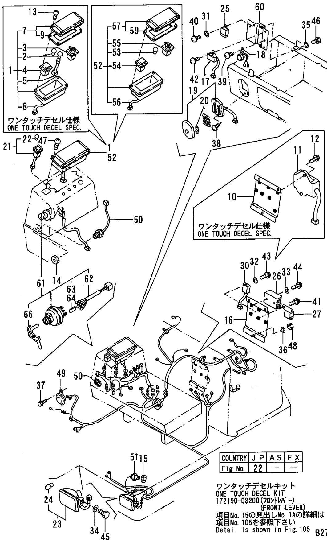
Fig. 22 電装品(機器:フロントレバ-) ELECTRIC PART (EQUIPMENT: FRONT LEVER)
