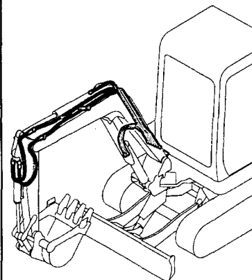
Fig. 87 油圧配管 (PTO アーム) HYD. OIL PIPING (P. T. O. ARM END)
