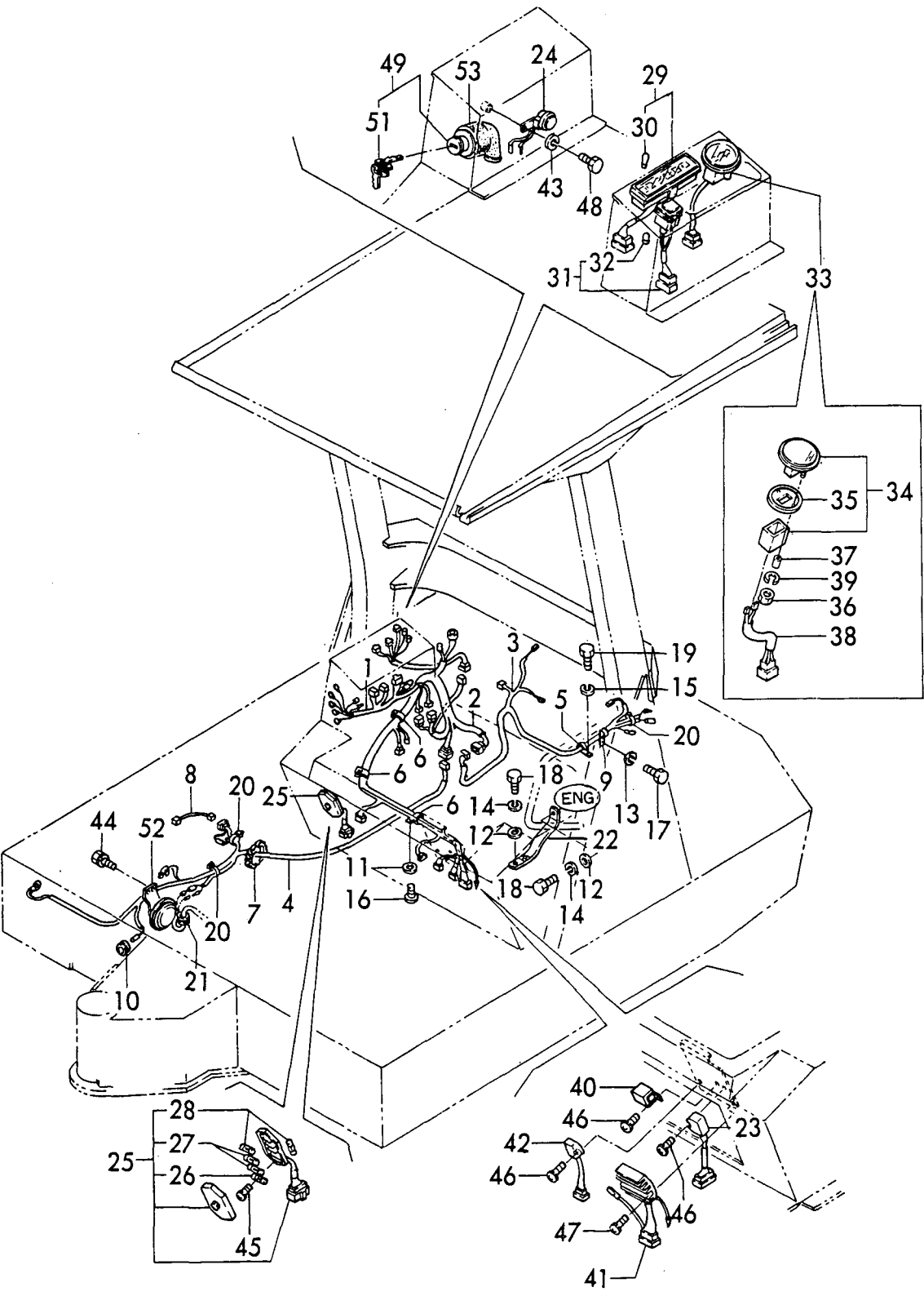
Fig. 15 デンソウヒン(キャノピ) https://truckmanualshub.com/ ELECTRIC PART (CANOPY SPEC.)
