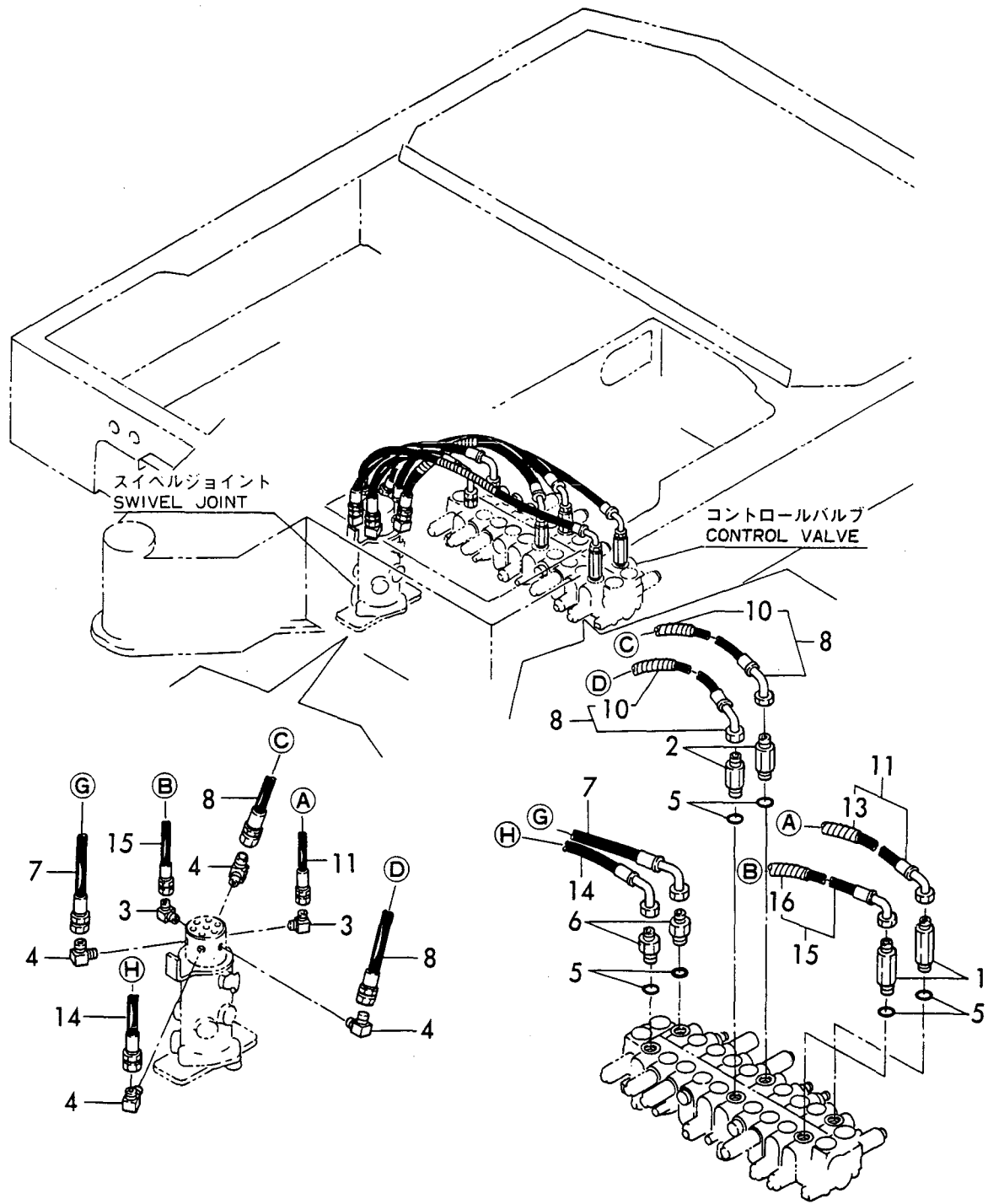
Fig. 55 ユアツハイカン(バルブスィベル) https://truckmanualshub.com/ HYD. OIL PIPING (VALVE-SWIVEL)
