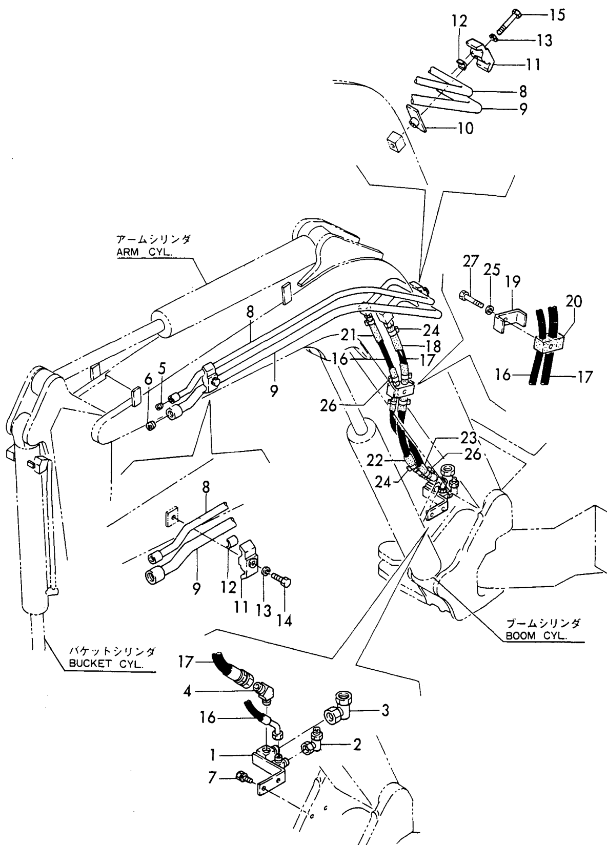
Fig. 60 ユアツハイカン(サードバルブ, ブーム) https://truckmanualshub.com/ HYD. OIL PIPING (3RD VALVE, BOOM)
