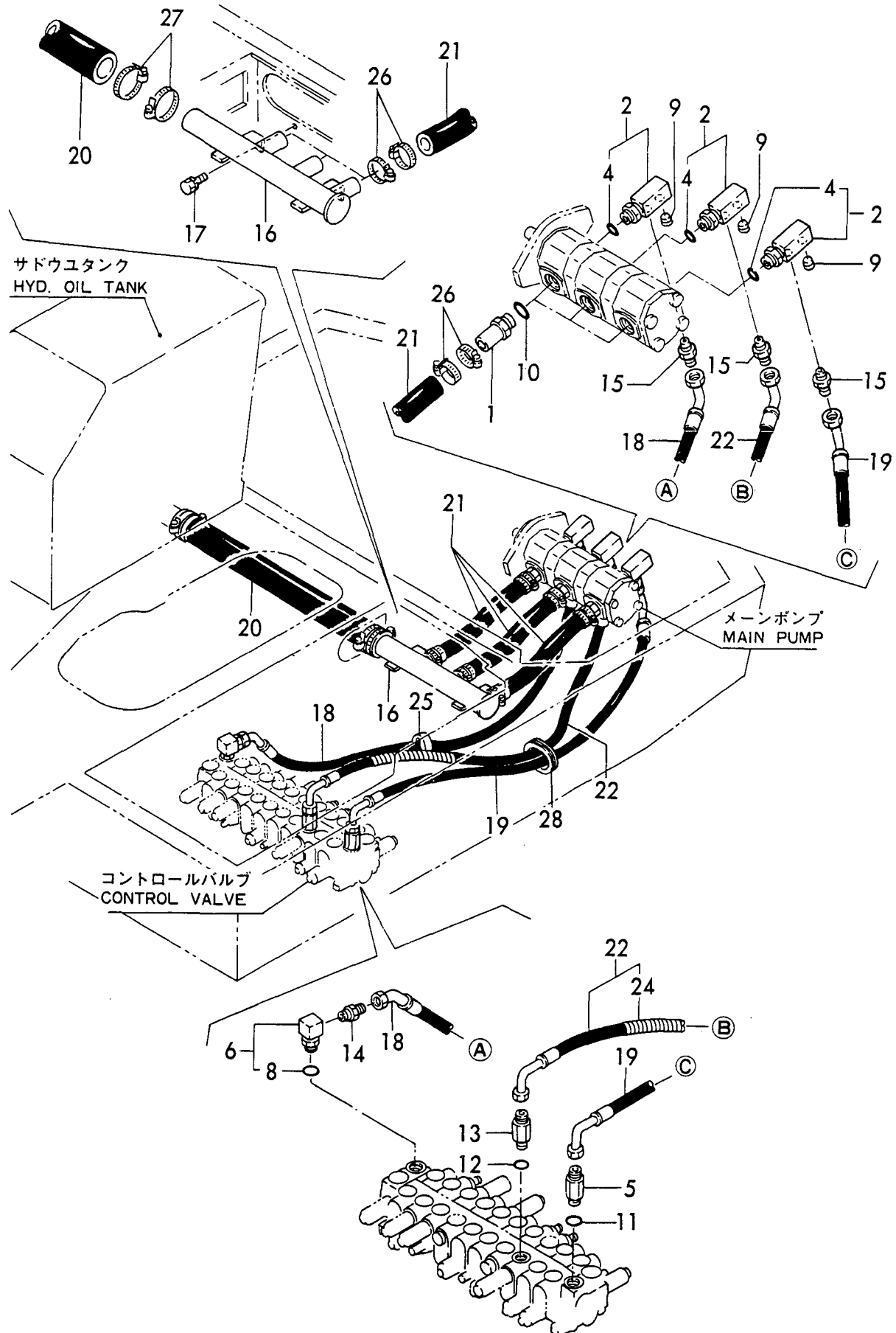
Fig. 53 ユアツハイカン(タンク-ポンプ-バルブ) HYD. OIL PIPING (TANK-PUMP-VALVE)
