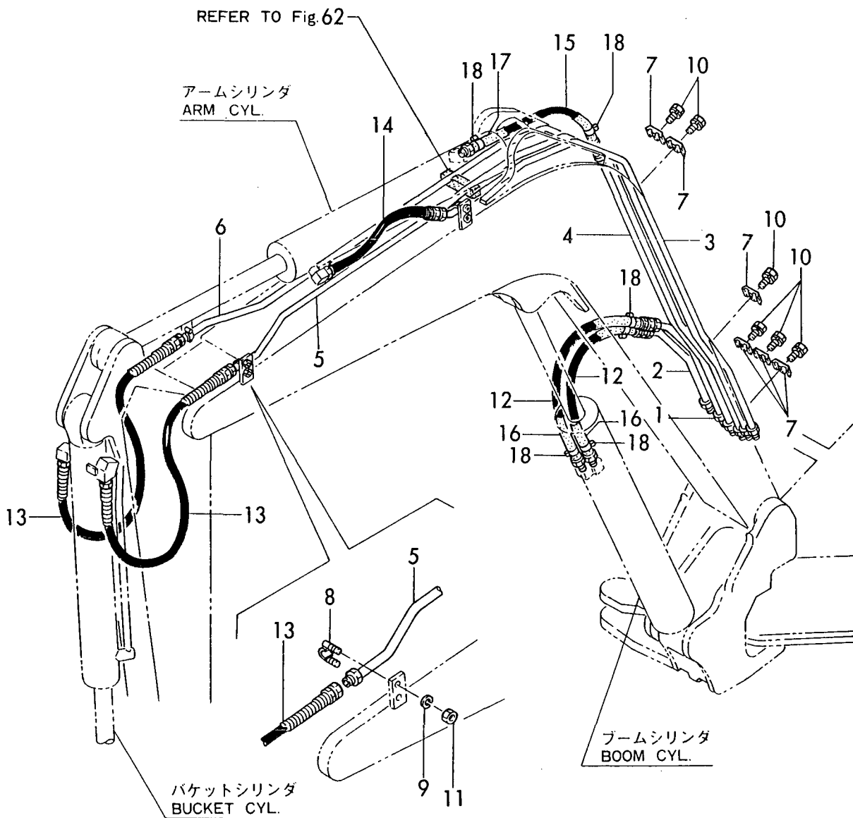
Fig. 58 ユアツハイカン(ブーム) HYD. OIL PIPING (BOOM) https://truckmanualshub.com/
