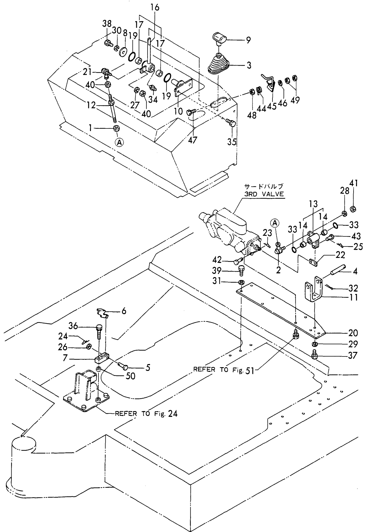
Fig. 26 ソウジュウソウチ(サードバルブ) CONTROL EQUIPMENT (3RD VALVE)
