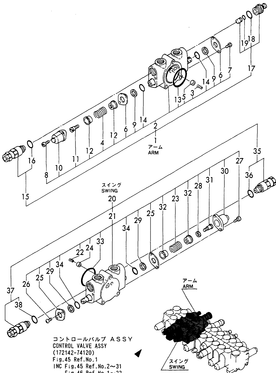
Fig. 47 コントロールバルブ (アーム & スイング) CONTROL VALVE (ARM & SWING)
