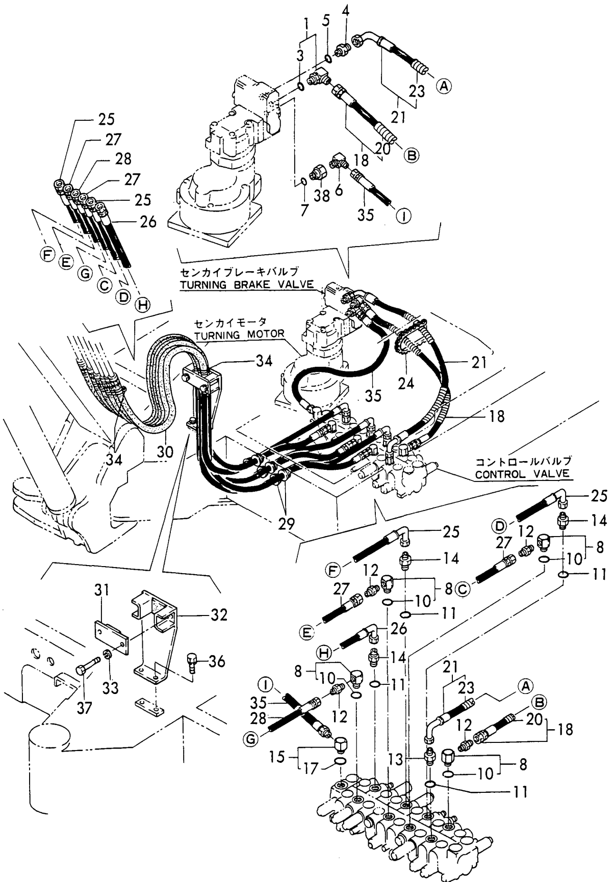
Fig. 54 ユアツハイカン (バルブモータ, ブーム) HYD. OIL PIPING (VALVE-MOTOR, BOOM)
