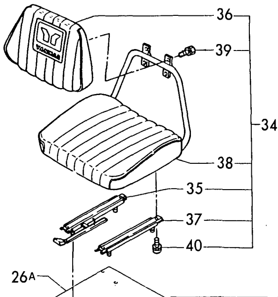
Fig. 31 ステップ、インパネ & シート STEP, INSTRUMENT PANEL & SEAT
