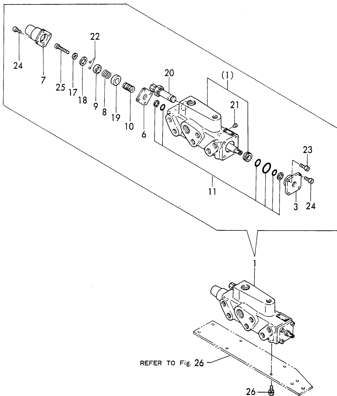
Fig. 51 サードバルブ (バルブ) https://truckmanualshub.com/ 3RD VALVE (VALVE)
