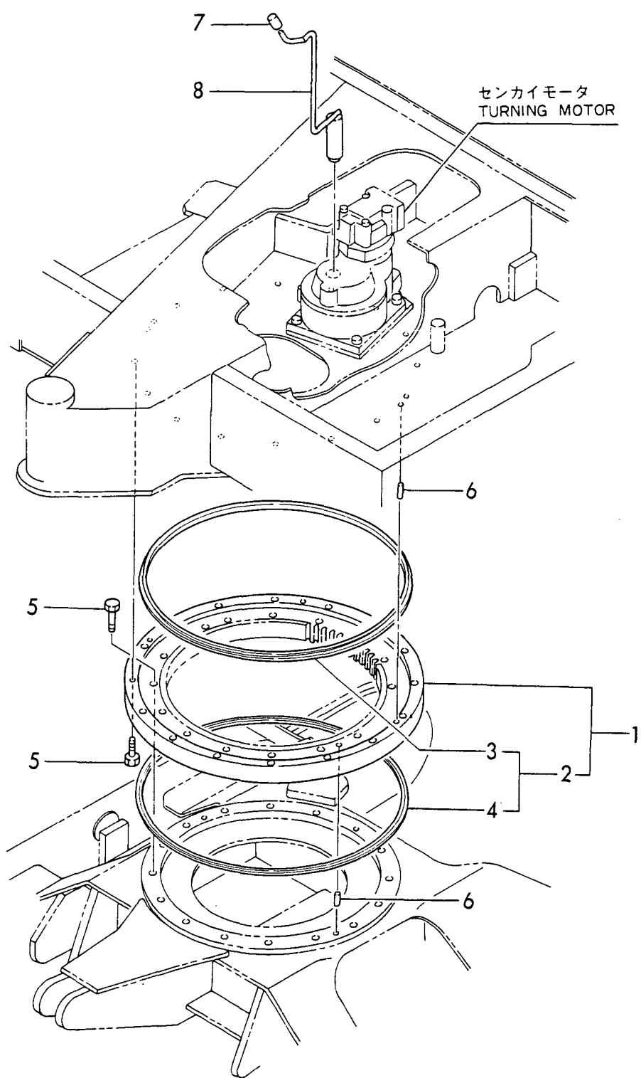
Fig. 29 センカイベアリング & センカイロック https://truckmanualshub.com/ TURNING BEARING & TURNING LOCK
