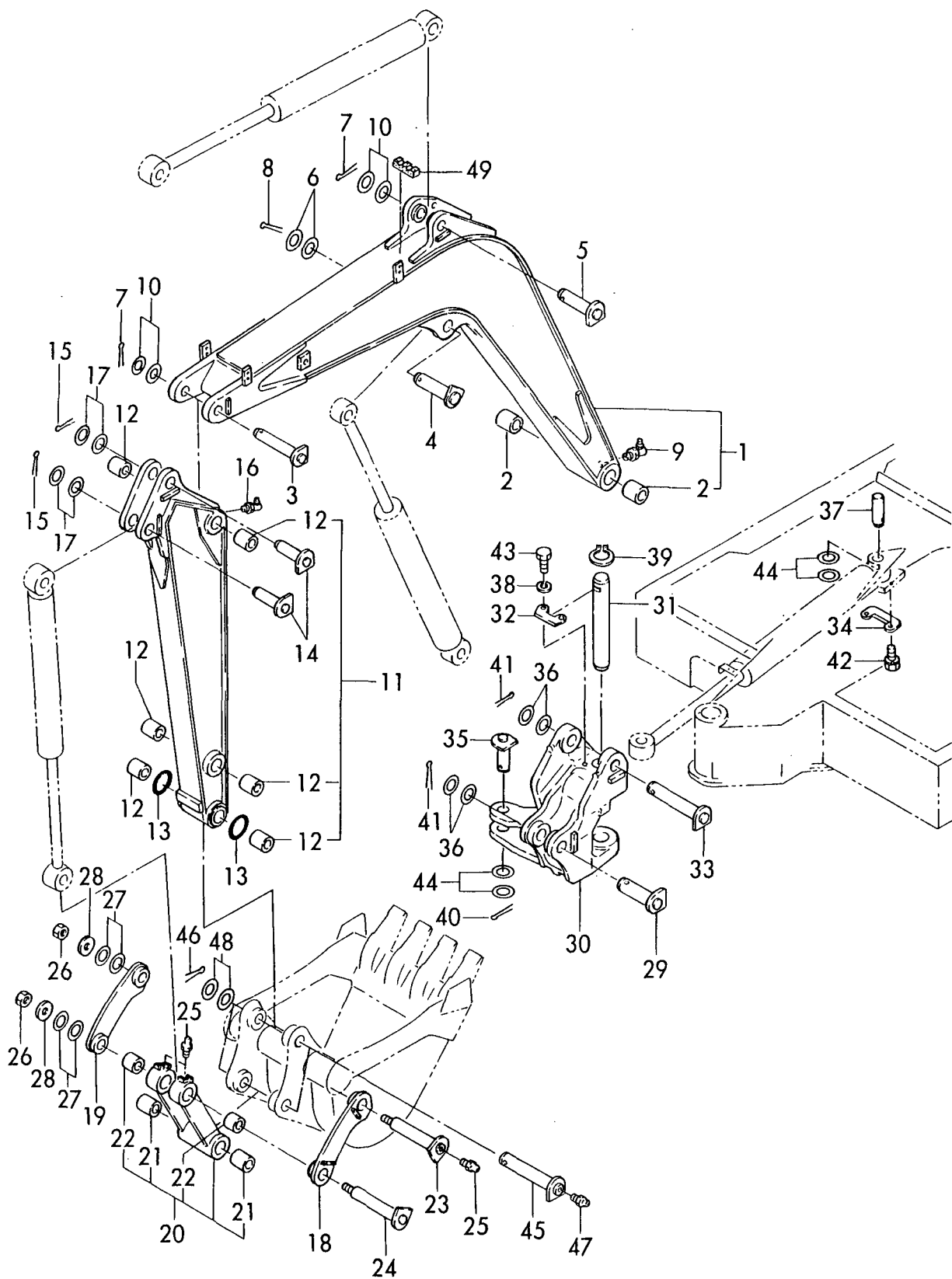
Fig. 62 ブーム & アーム BOOM & ARM https://truckmanualshub.com/
