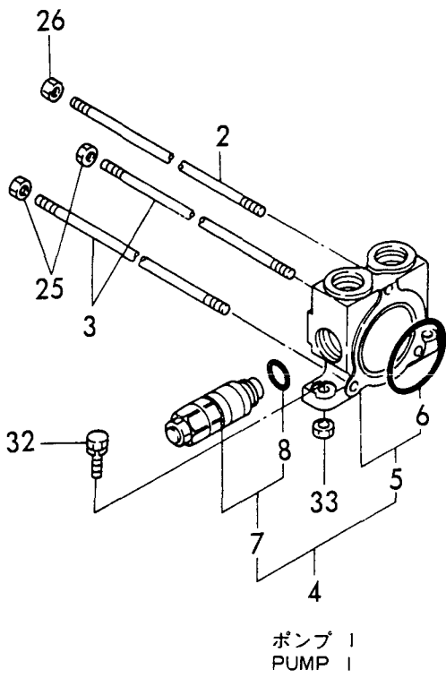
Fig. 45 45 コントロールバルブ(Pポート) CONTROL VALVE (P PORT)
