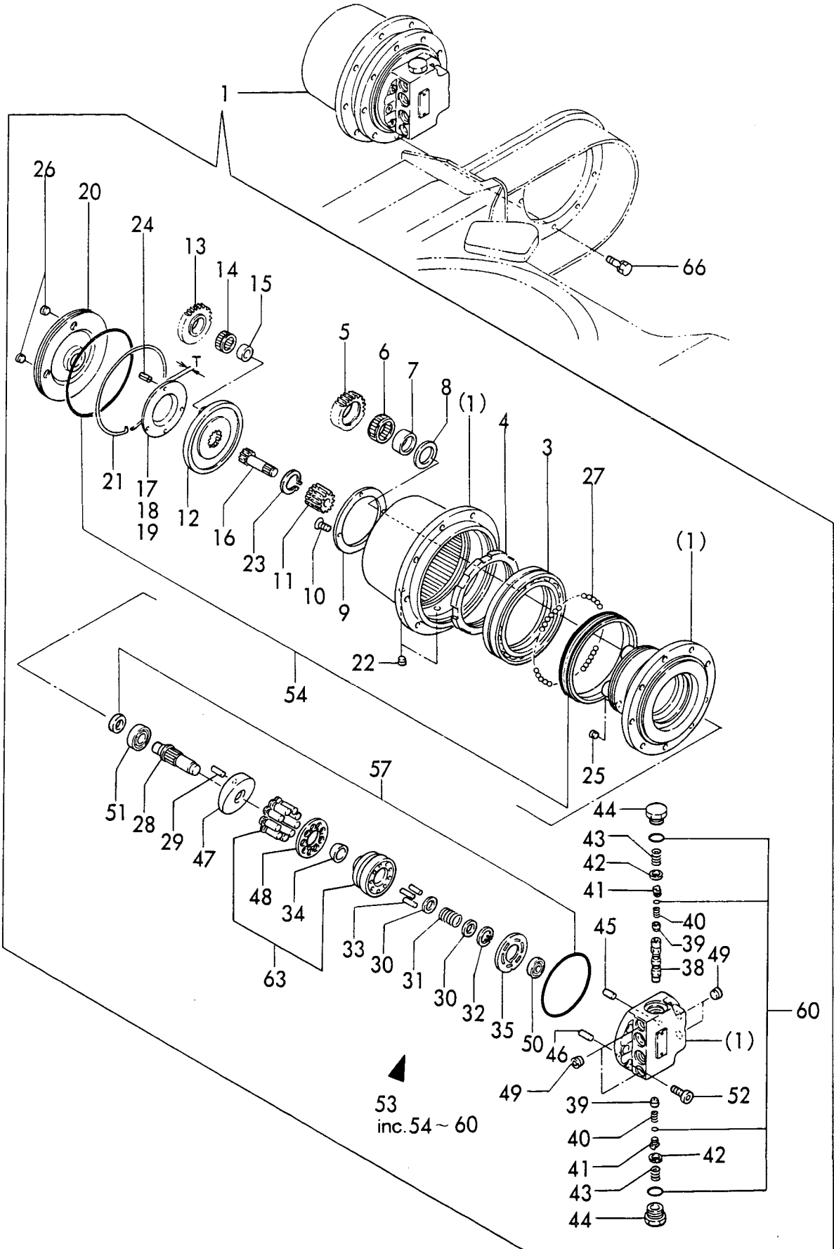
Fig. 42 ソウコウモータ https://truckmanualshub.com/ DRIVING MOTOR
