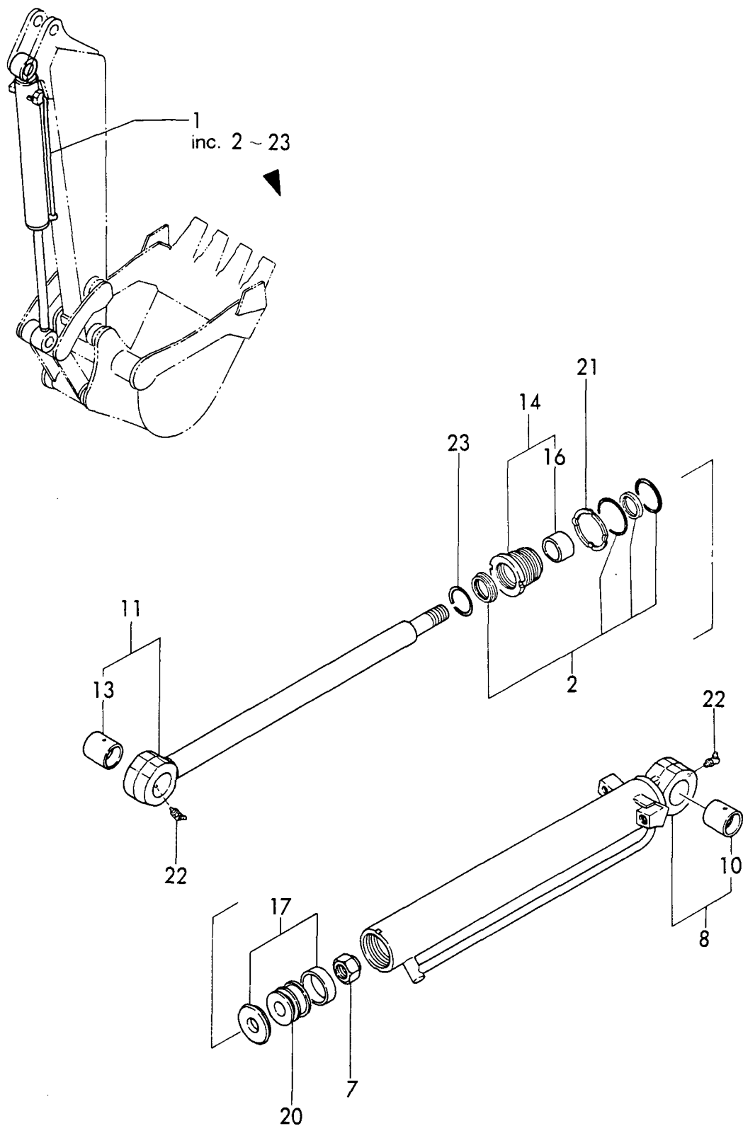
Fig. 38 バケットシリンダ https://truckmanualshub.com/ BUCKET CYLINDER
