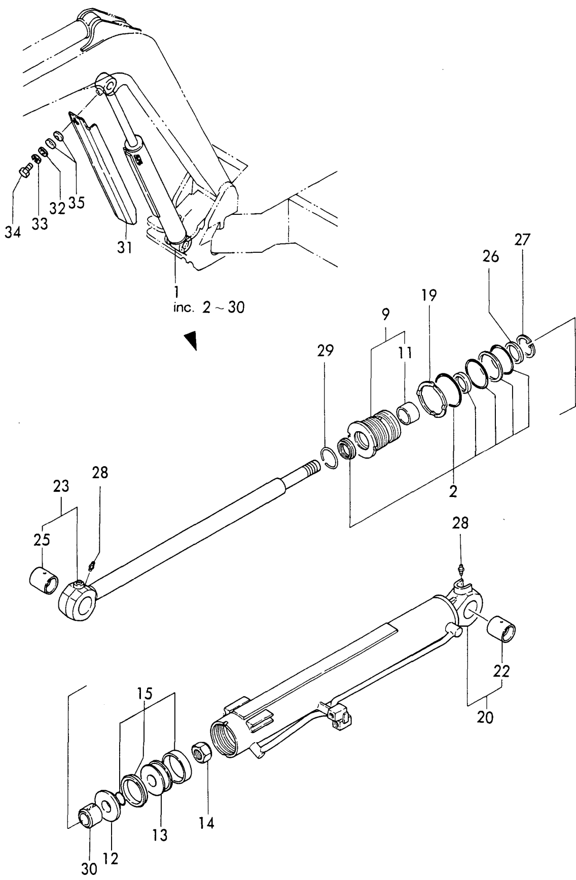
Fig. 36 ブームシリンダ(UZ)(キャノピ) https://truckmanualshub.com/ BOOM CYLINDER (UZ) (CANOPY SPEC.)
