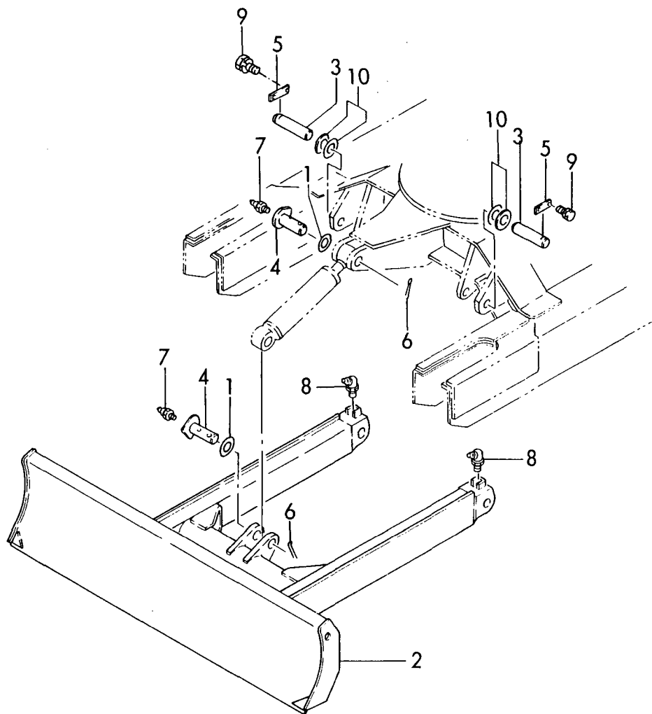
Fig. 64 ブレード BLADE https://truckmanualshub.com/
