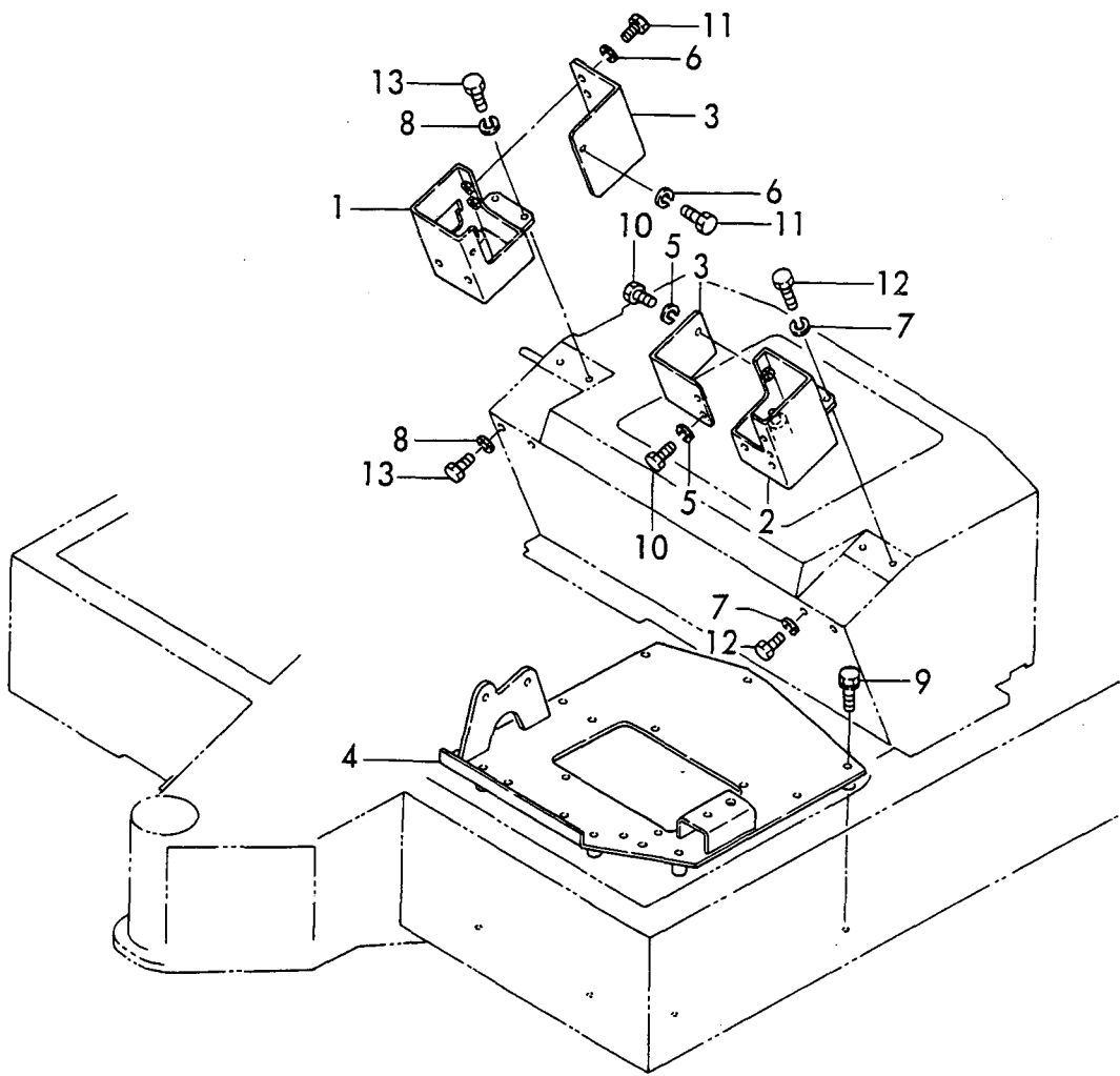
Fig. 21 リンクダイ LINK STAND https://truckmanualshub.com/
