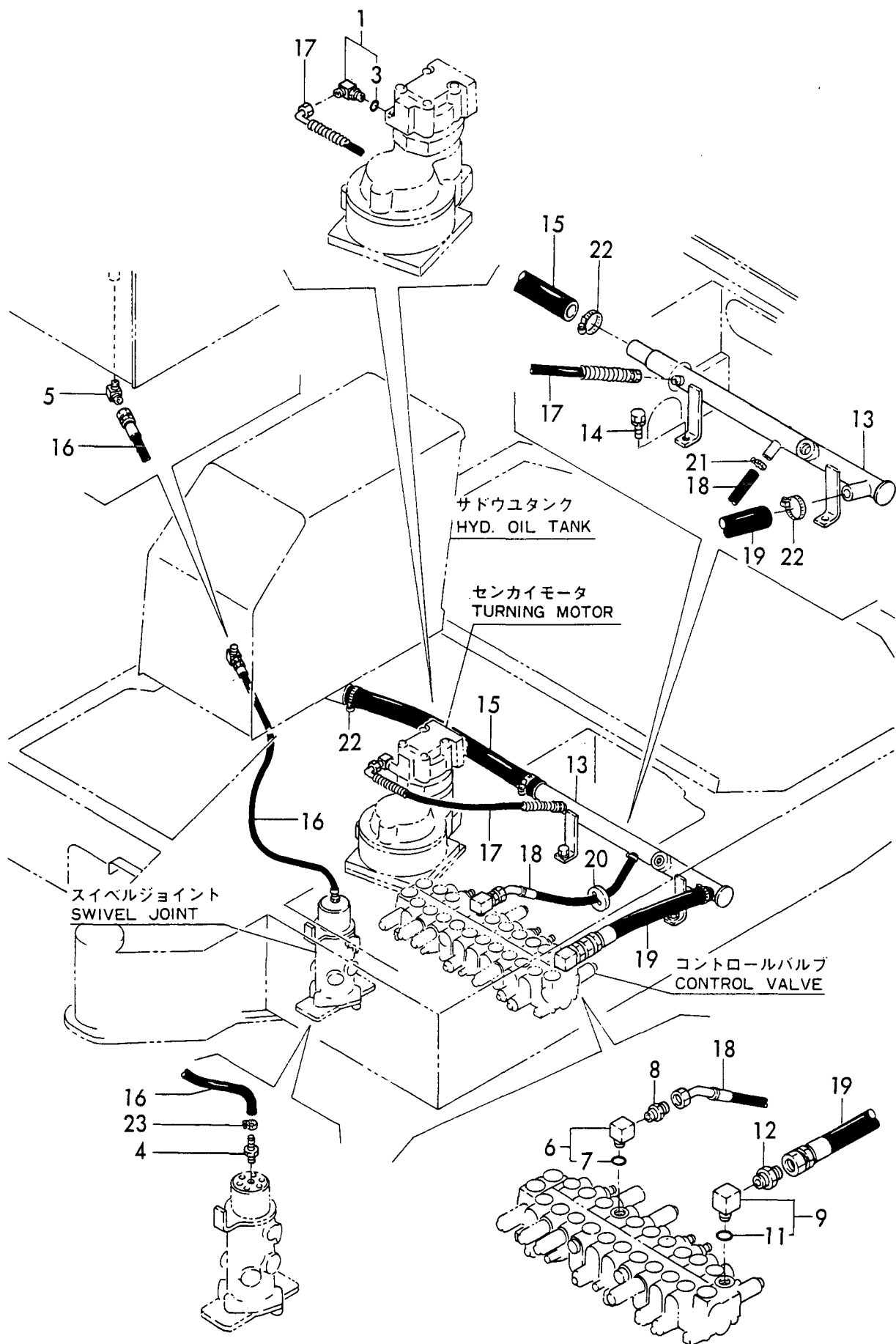
Fig. 56 ユアツハイカン(リターン) HYD. OIL PIPING (RETURN) https://truckmanualshub.com/
