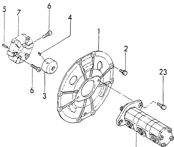
Fig. 41 ポンプ & ジクツギテ https://truckmanualshub.com/ HYD. OIL PUMP & JOINT
