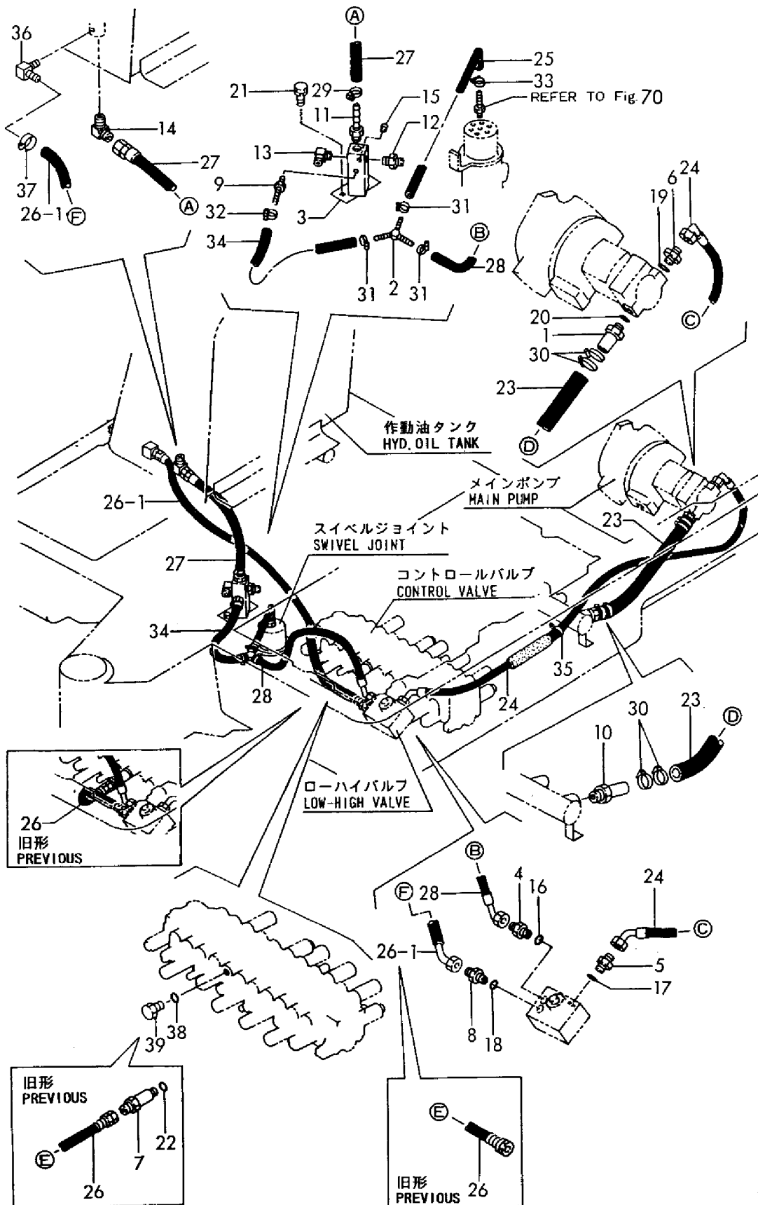
Fig. 76 コントロール配管(ポンプ～ローハイバルブ～リターン) CONTROL PIPING(PUMP～LOW-HIGH VALVE～RETURN)
