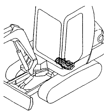
Fig. 59 コントロールバルブ (アーム & シング:P.T.O. 仕様) CONTROL VALVE (ARM & SWING:P.T.O. SPEC.)
