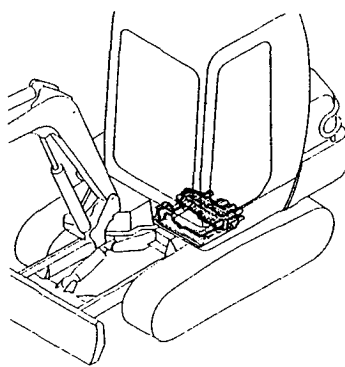
Fig. 58 コントロールバルブ (走行 & P.T.O. :P.T.O. 仕様) CONTROL VALVE(DRIVING & P.T.O. :P.T.O. SPEC.)
