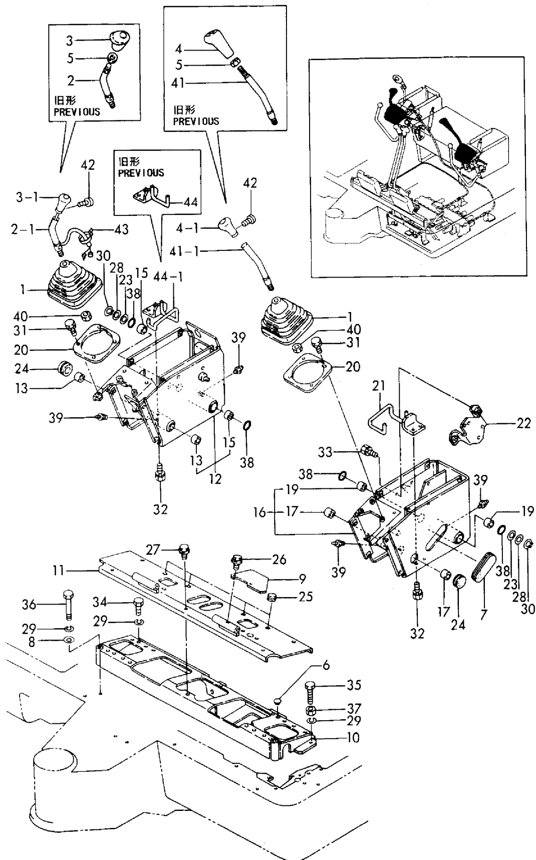
Fig. 24 操縦装置(レバー & スタンド:サイド仕様) CONTROL EQUIPMENT(LEVER & STAND:SIDE SPEC.)
