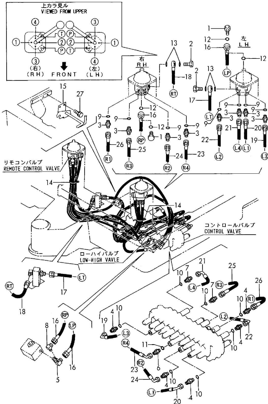
Fig. 77 77 コントロール配管(フロントレバー, ダイレクト仕様) CONTROL PIPING(FRONT LEVER, DIRECT SPEC.)
