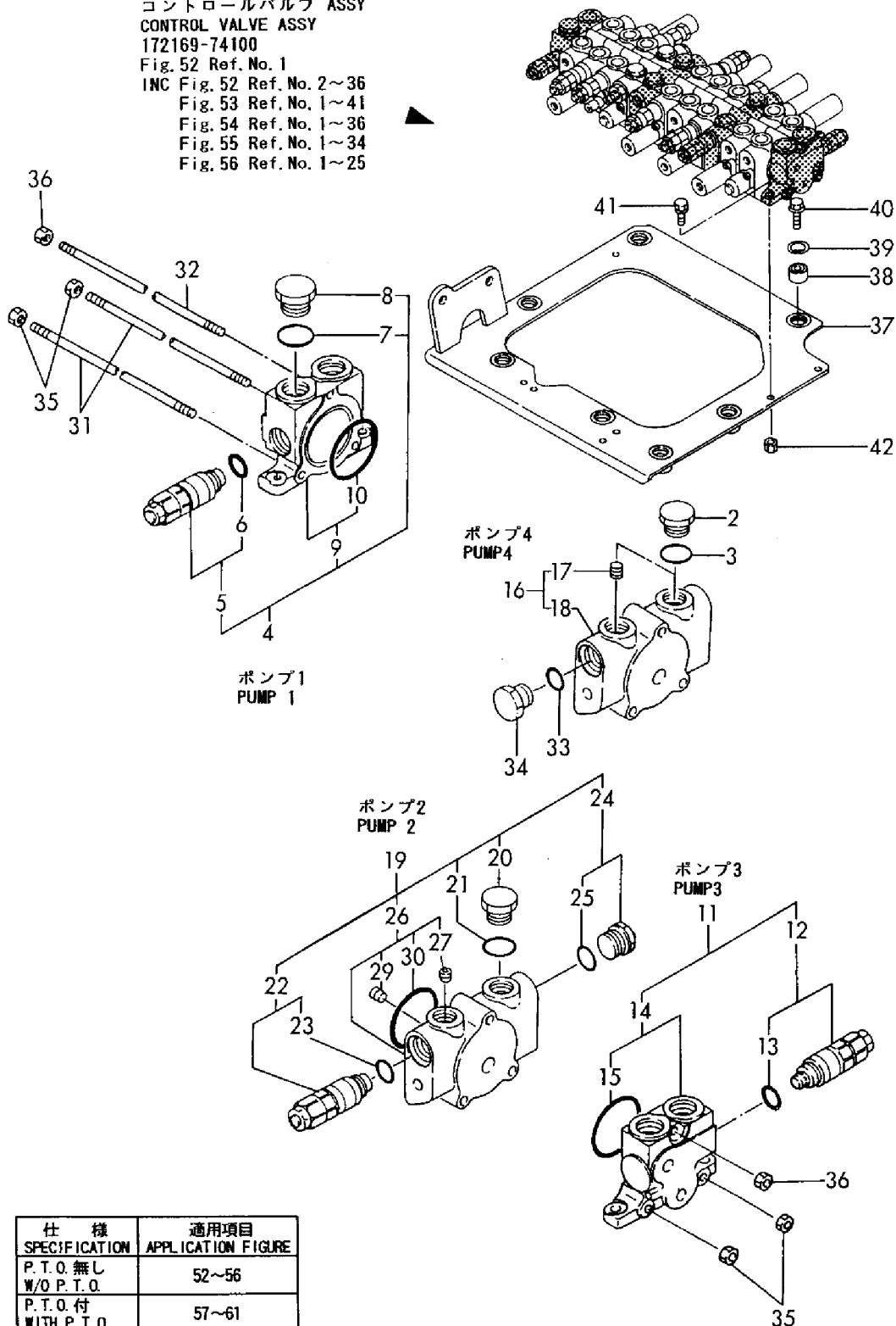
Fig. 52 52 コントロールバルブ(油圧P.T.O. 無:Pポート & バルブ台) CONTROL VALVE(W/O HYD. OIL P. T. O. :P PORT & VALVE STAND)
