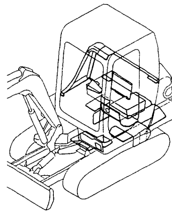
Fig.32 フレームカバー FRAME COVER
