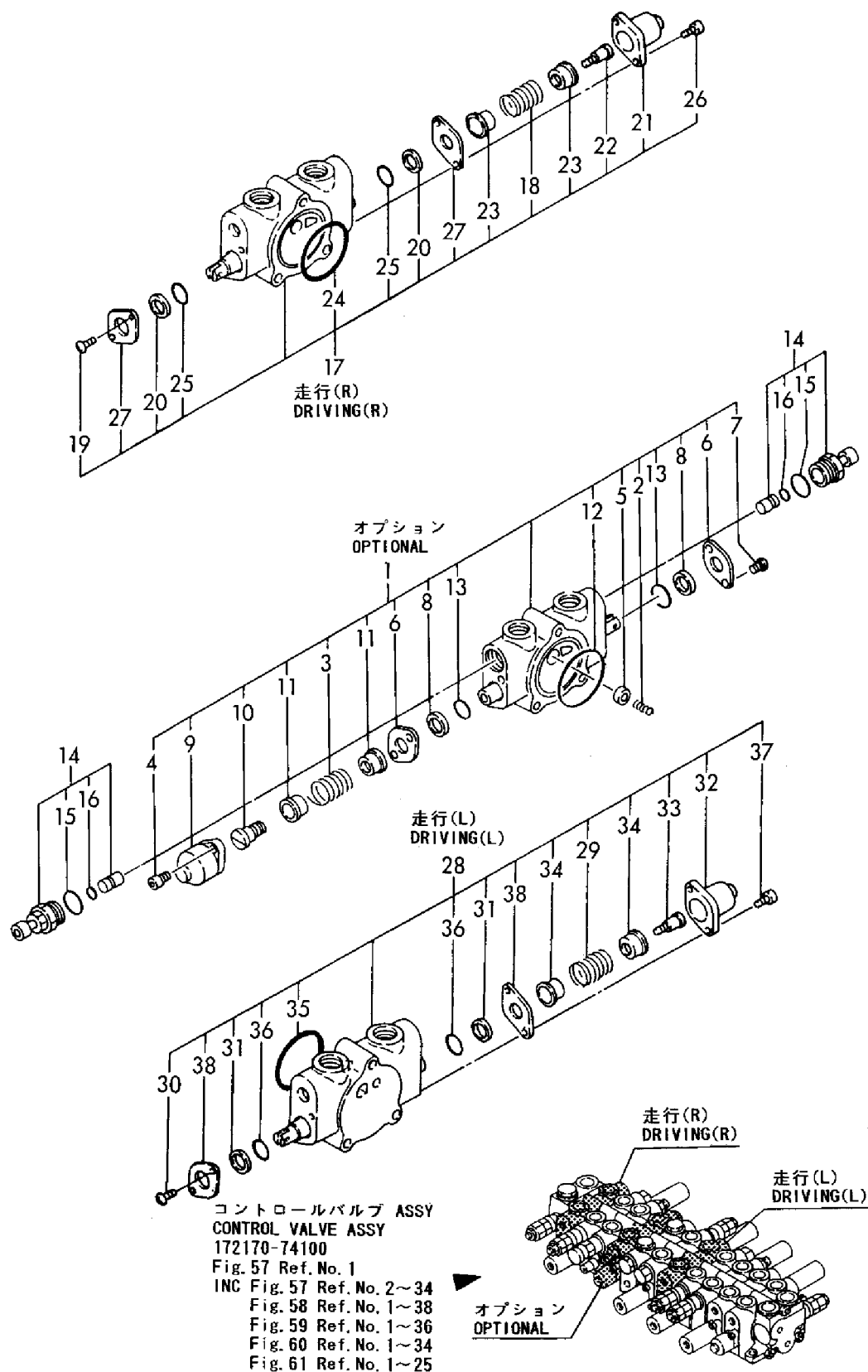
Fig. 58 58 コントロールバルブ(走行 & P.T.O. :P.T.O.仕様) CONTROL VALVE(DRIVING & P.T.O. :P.T.O. SPEC.)
