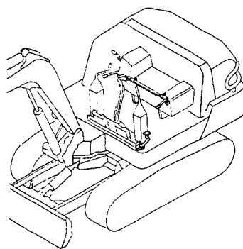
Fig.28 操縦装置(カットオフレバー & ペダル:フロント仕様) CONTROL EQUIPMENT(CUT-OFF LEVER & LOW-HIGH PEDAL :FRONT SPEC.)
