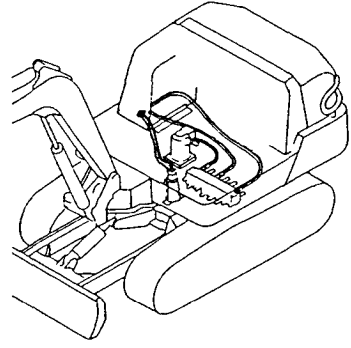
Fig.71 P.T.O. 油圧配管 (フレーム:単流仕様) P.T.O. HYD. OIL PIPING (FRAME:UNI-FLOW SPEC.)
