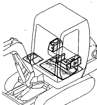
Fig.34 ステップ & インパネ (サイドレバー仕様) STEP & INSTRUMENT PANEL (SIDE LEVER SPEC.)
