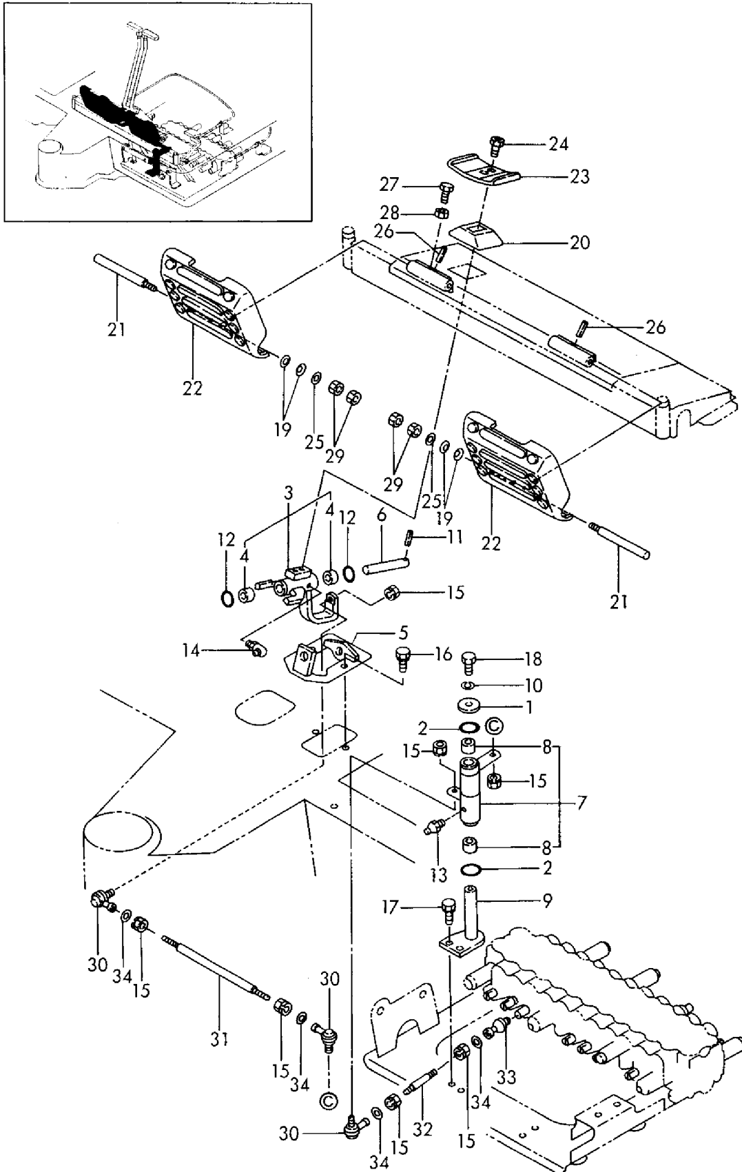
Fig. 26 操縦装置(スイング) CONTROL EQUIPMENT(SWING)
