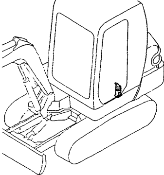
Fig.64 ローハイバルブ LOW-HIGH VALVE
