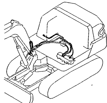
Fig.72 P.T.O. 油圧配管 (フレーム:合流仕様) P.T.O. HYD. OIL PIPING (FRAME:CONFLUENCE SPEC.)
