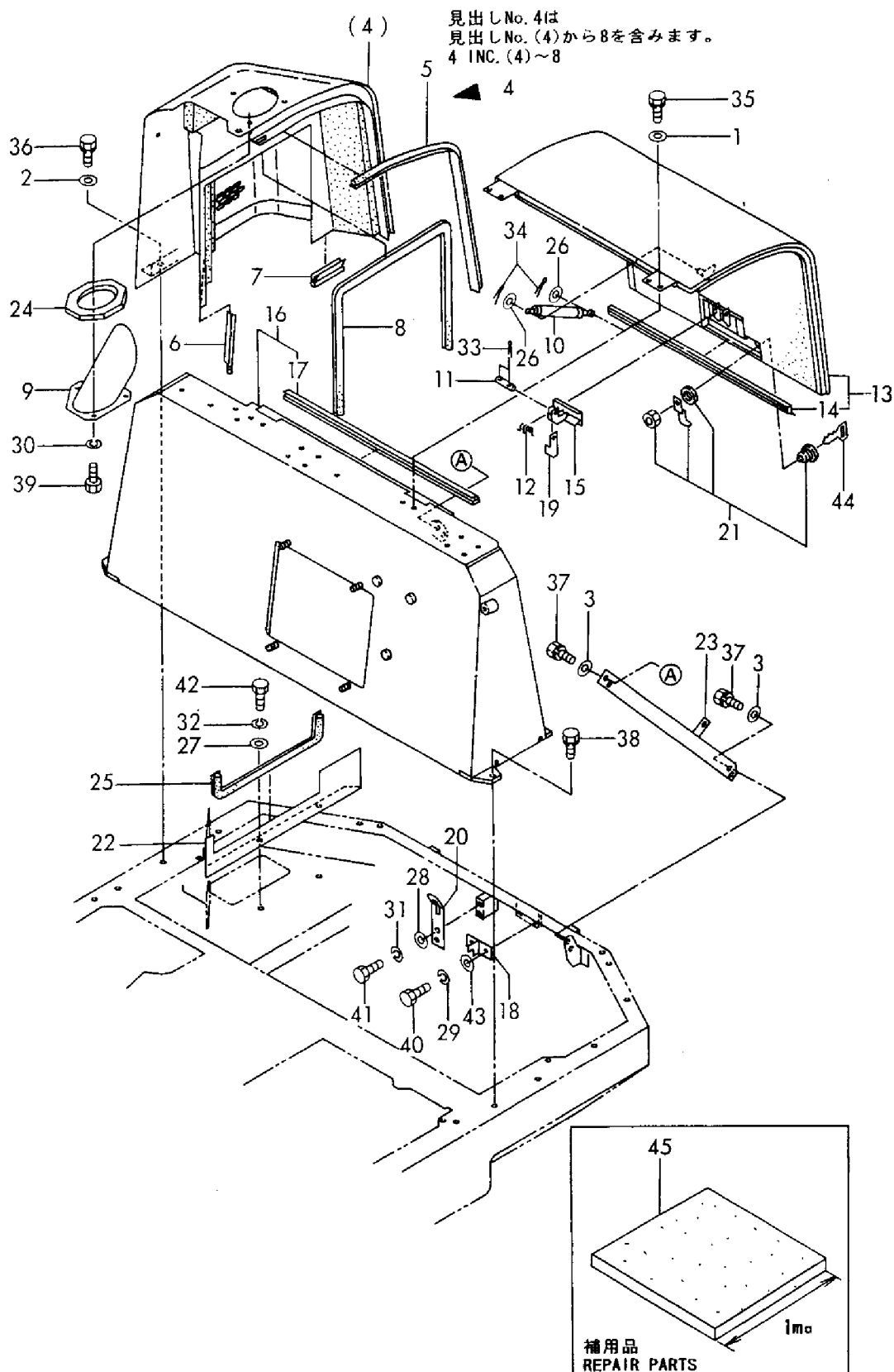
Fig. 37 ボンネット BONNET
