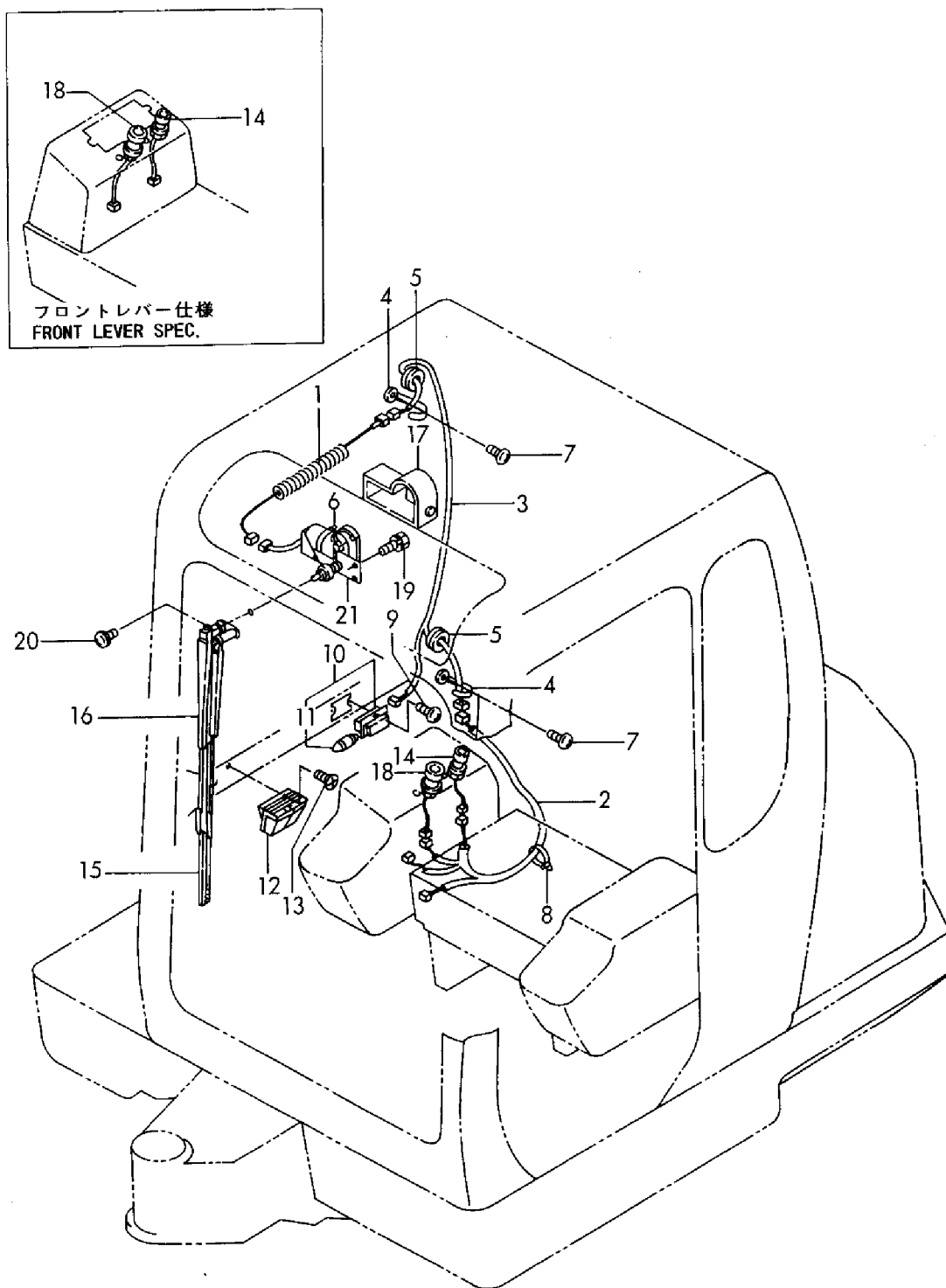
Fig. 17 電装品(キャビン専用) ELECTRIC PART(CABIN)
