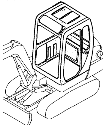
Fig.39 キャビン(ガラス & サッシ) CABIN(GLASS & SASH)
