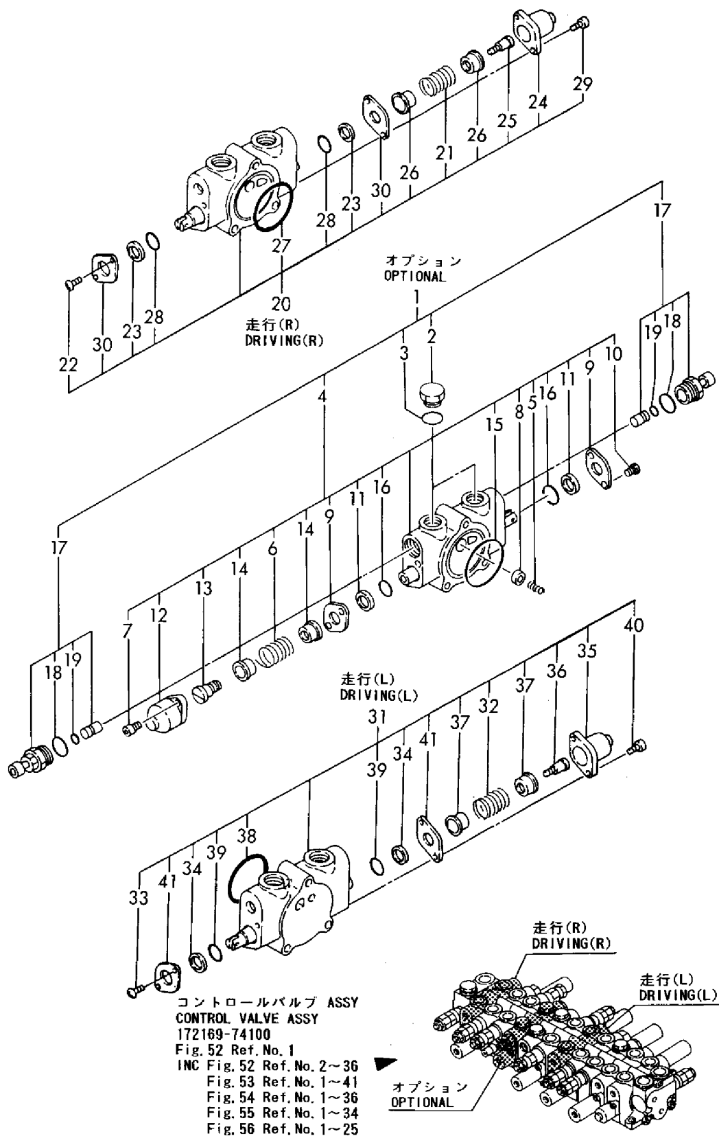
Fig. 53 53 コントロールバルブ(油圧P.T.O. 無:走行 & P.T.O.) CONTROL VALVE(W/O HYD. OIL P.T.O. :DRIVING & P.T.O.)
