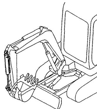
Fig.47 スイングシリンダ SWING CYLINDER
