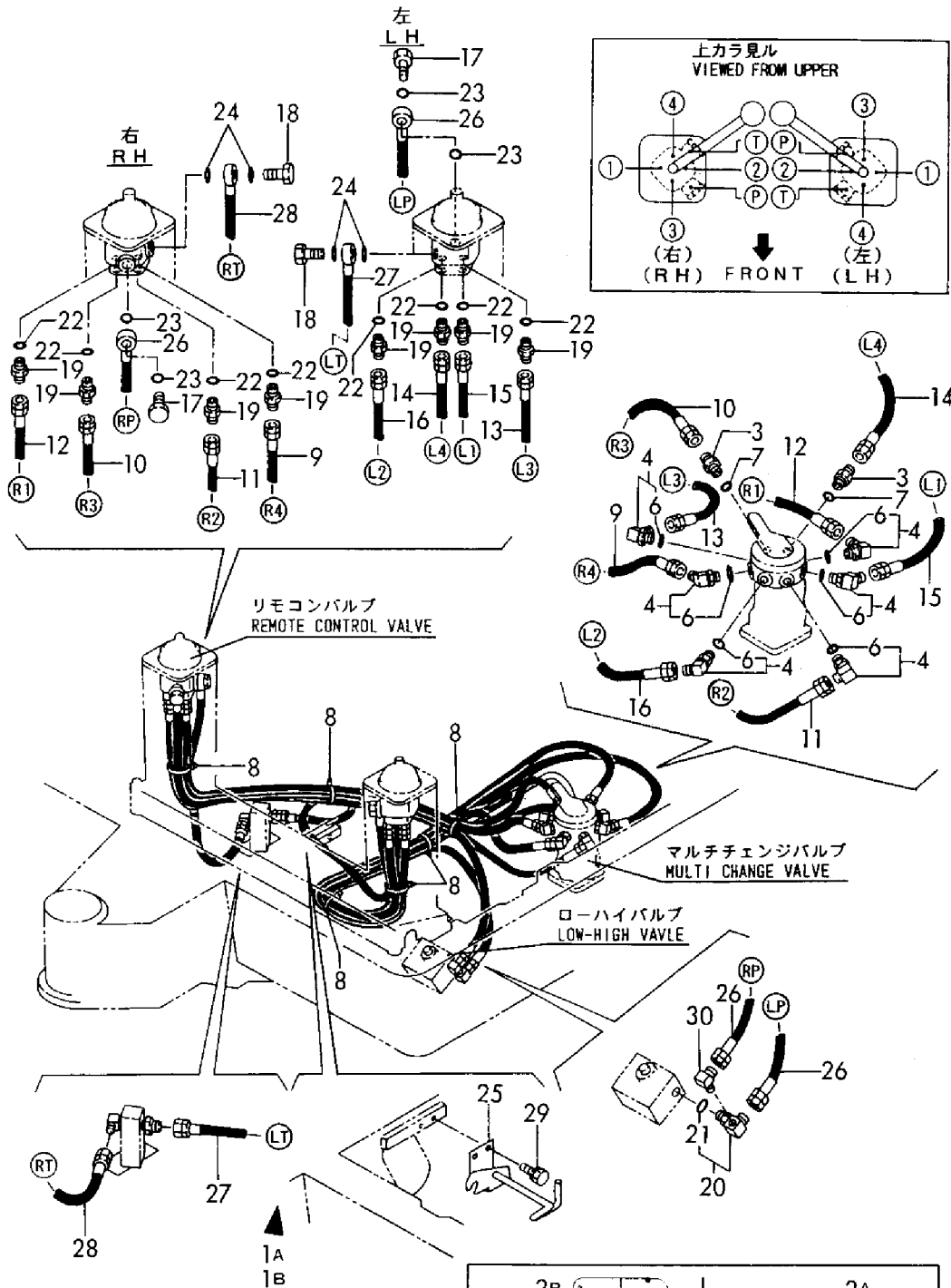
Fig. 79 79 コントロール配管(フロントマルチチェンジ仕様) CONTROL PIPING(FRONT MULTI CHANGE SPEC.)
