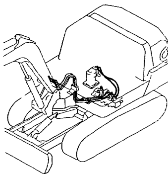
Fig.68 油圧配管(バルブ〜モータ、ブーム) HYD. OIL PIPING (VALVE~MOTOR, BOOM)
