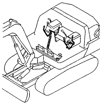
Fig.30 操縦装置(P.T.O.コントロール) CONTROL EQUIPMENT (P.T.O. CONTROL)
