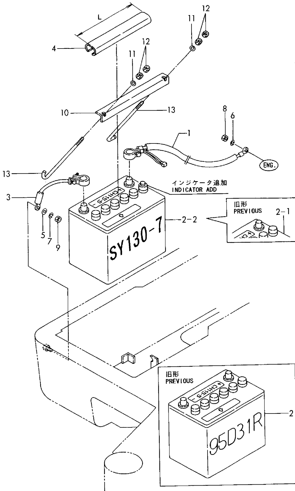
Fig. 14 バッテリー BATTERY
