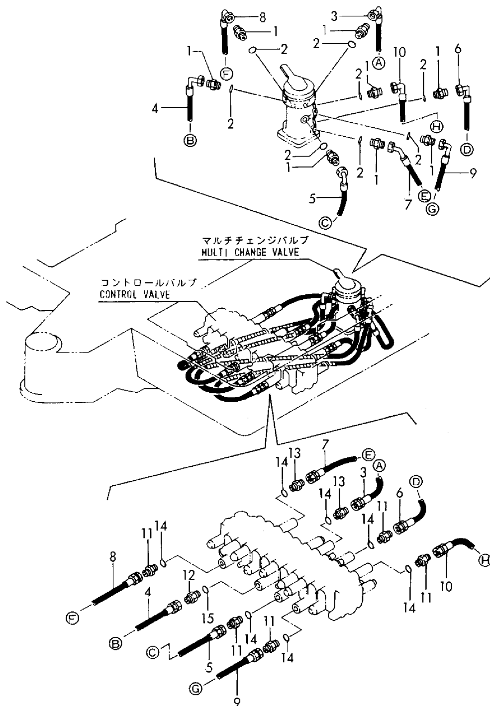
Fig. 81 81 コントロール配管(マルチチェンジ仕様共通) CONTROL PIPING(MULTI CHANGE SPEC. COMMON)
