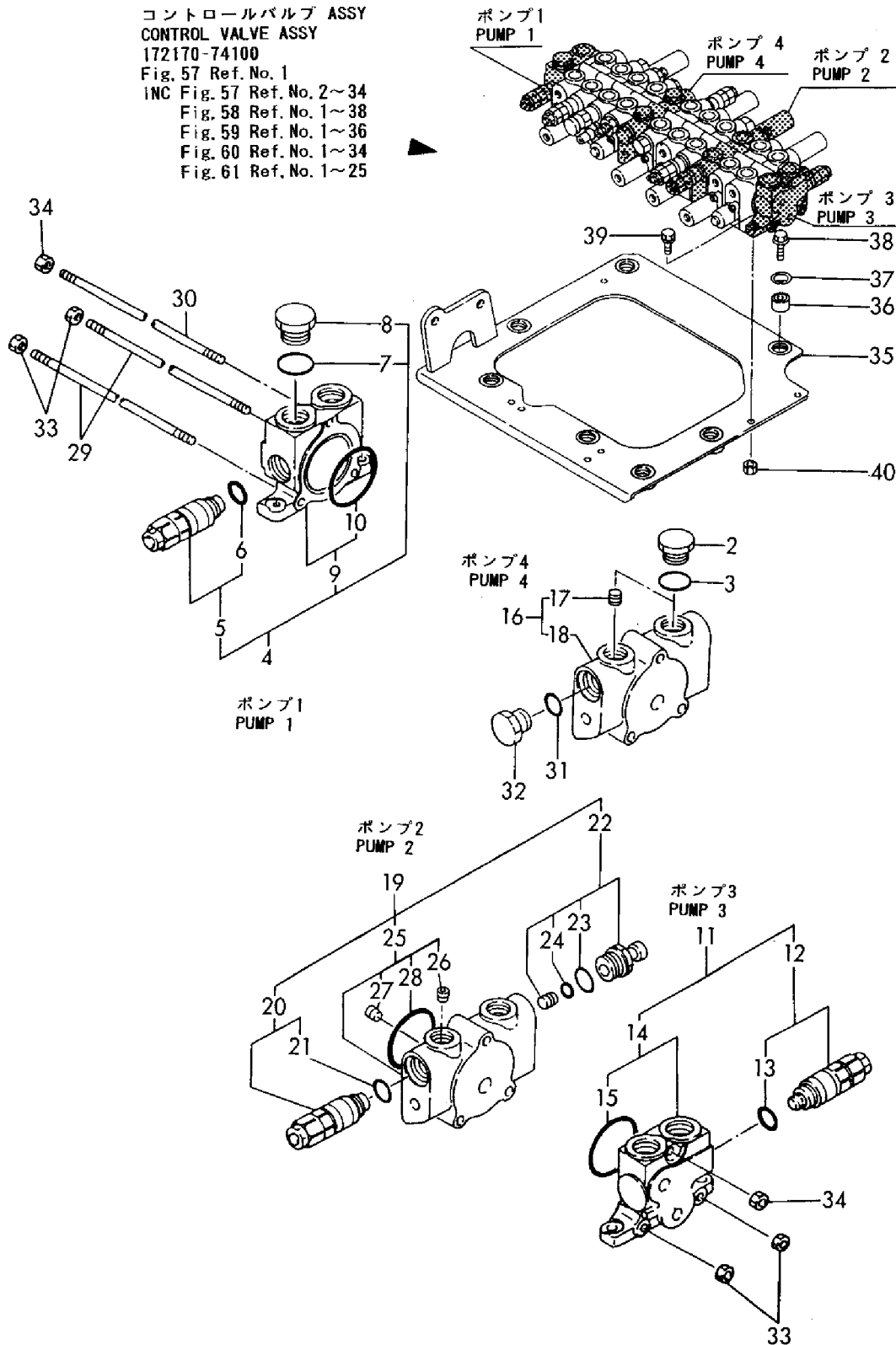
Fig. 57 57 コントロールバルブ(Pポート & バルブ台:P. T. O.仕様) CONTROL VALVE(P PORT & VALVE STAND:P. T. O. SPEC.)
