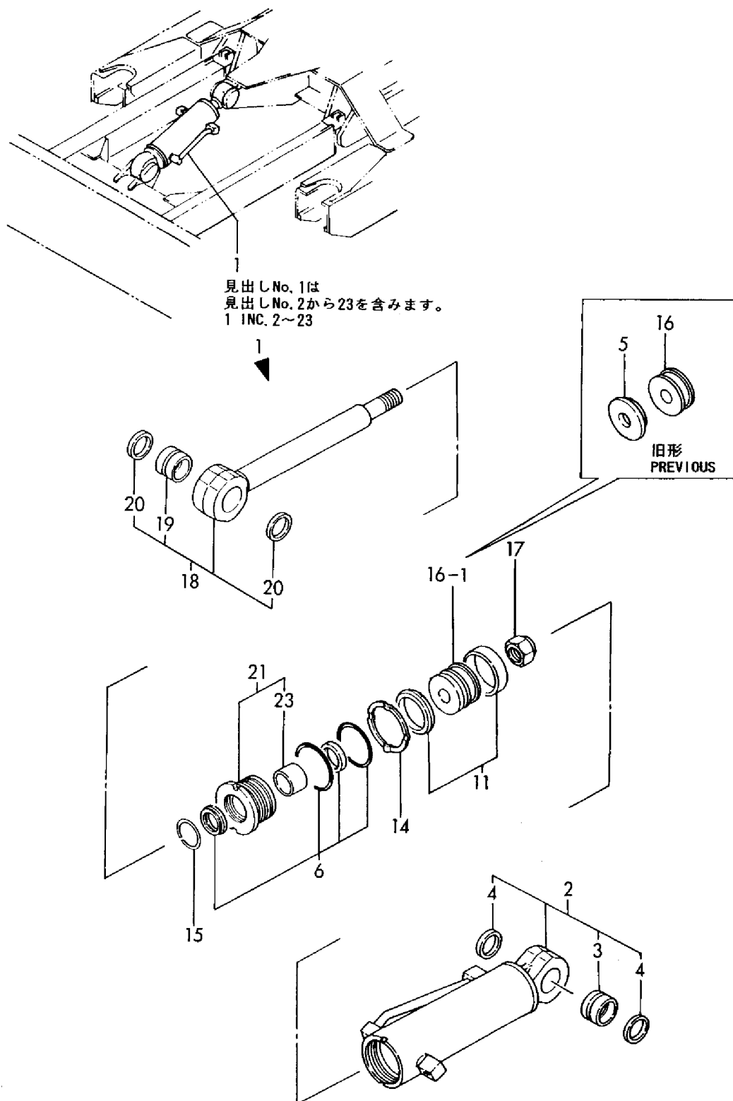
Fig. 48 ブレードシリンダ BLADE CYLINDER
