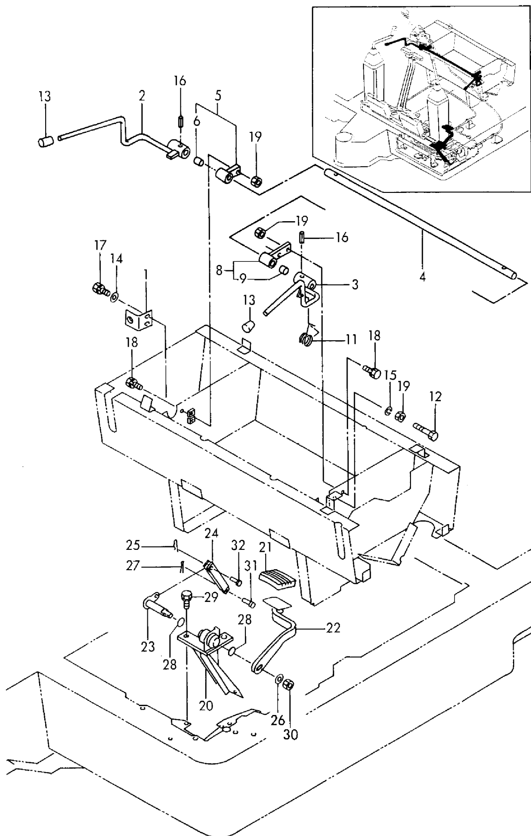
Fig. 28 操縦装置(カットオーバー & ペダル:フロント仕様) CONTROL EQUIPMENT(CUT OFF LEVER & LOW-HIGH PEDAL:FRONT SPEC.)
