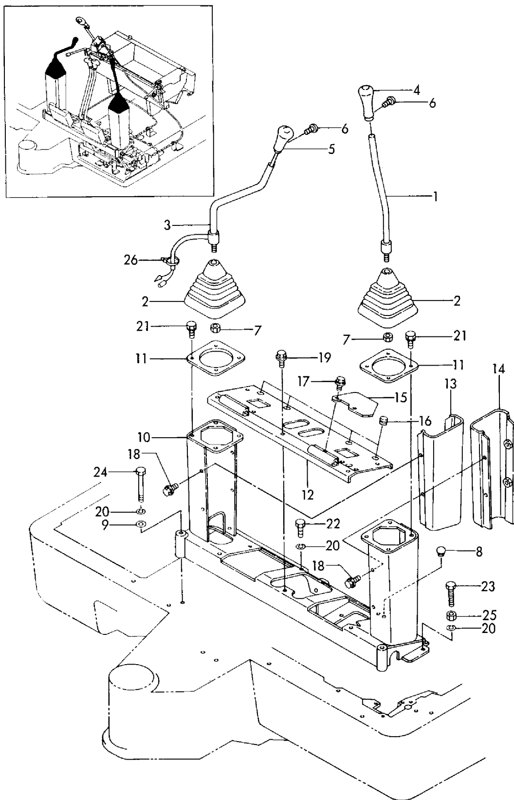
https://truckmanualshub.com/ Fig. 23 操縦装置(レバー & スタンド:フロント仕様) CONTROL EQUIPMENT(LEVER & STAND:FRONT SPEC.)
