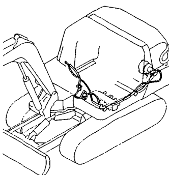
Fig. 76 コントロール配管 (ポンプ～ローハイバルブ～リターン) CONTROL PIPING(PUMP ~LOW-HIGH VALVE~RETURN)
