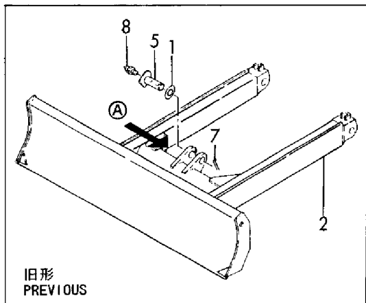
Fig. 87 ブレード BLADE
