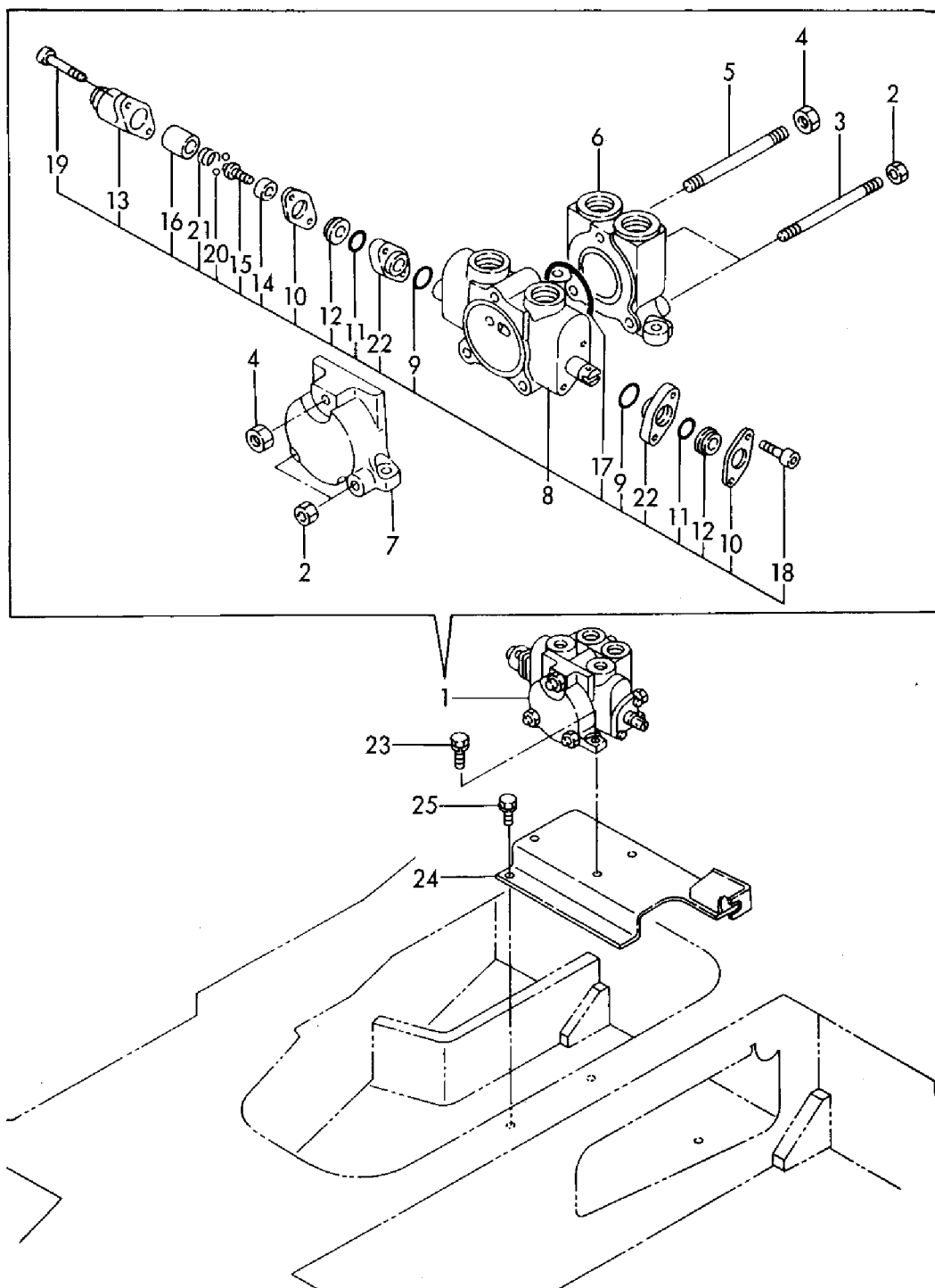
Fig. 65 P. T. O. バルブ(合流仕様) P. T. O. VALVE (CONFLUENCE SPEC.)
