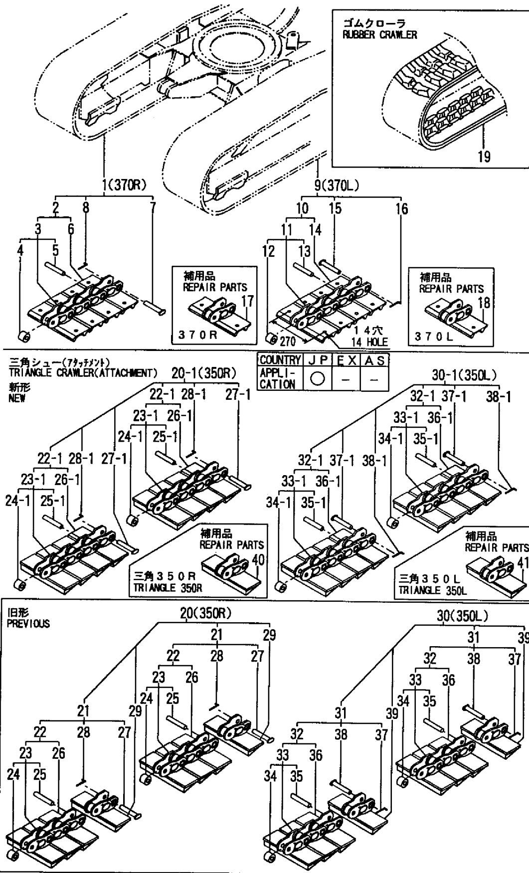
Fig. 26 クローラ CRAWLER
