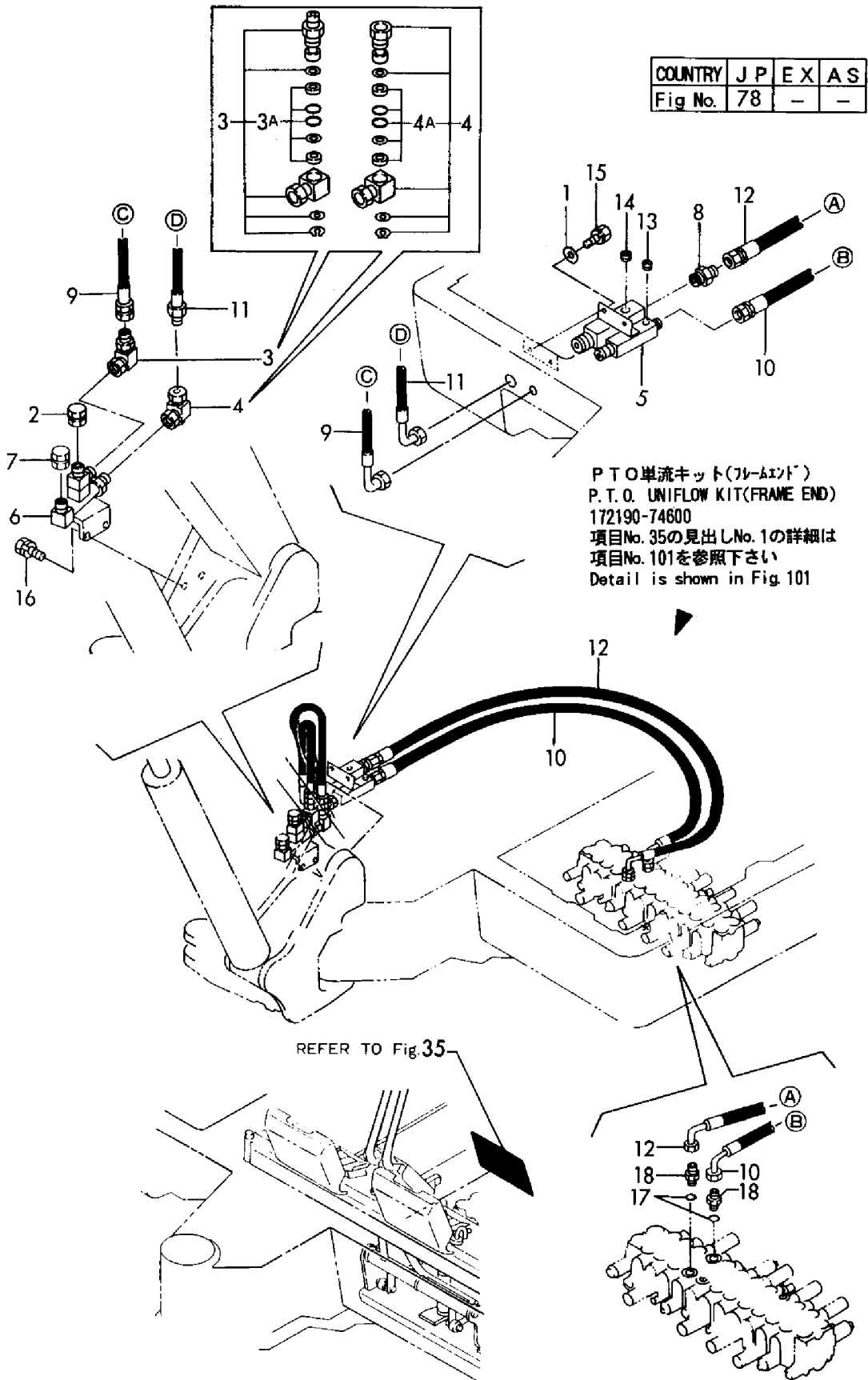
Fig. 78 油圧配管(PTO, フレームエンド: 単流仕様) HYD. OIL PIPING(P. T. O., FRAME END: UNIFLOW SPEC.)
