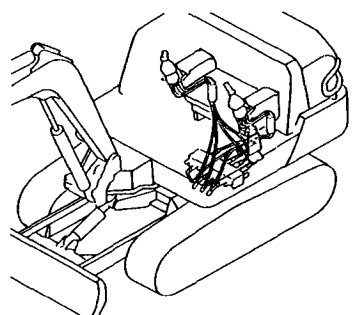
Fig. 94 コントロール配管 (2ウェイ:サイドレバー) CONTROL PIPING (2-WAY:SIDE LEVER)
