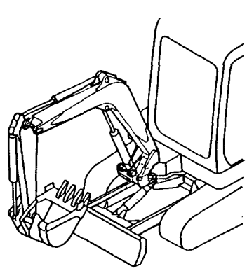
Fig. 96 ブーム & ブームブラケット BOOM & BOOM BRACKET
