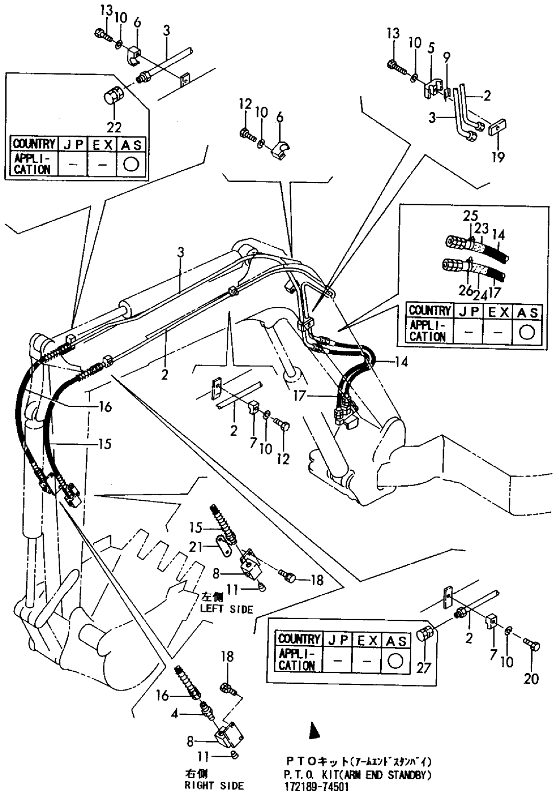
Fig. 83 油圧配管(PTO 7 -M:アームエンド仕様)(新形) HYD. OIL PIPING(P. T. O. BOOM: ARM END SPEC. )(NEW)
