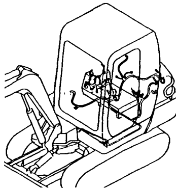
Fig.18 電装品(ワイヤリング:サイドレバー) ELECTRIC PART(WIRING :SIDE LEVER)
