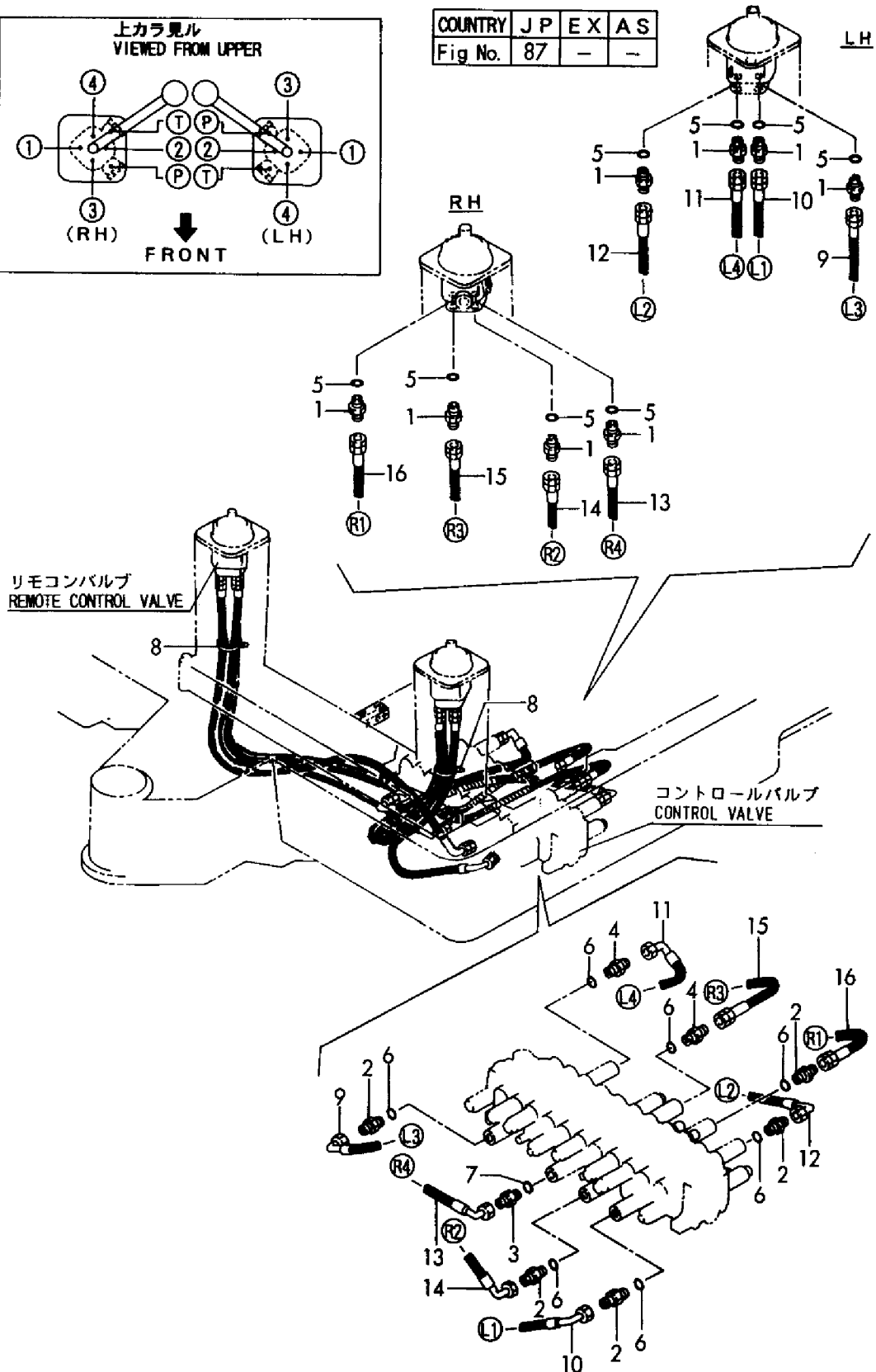
Fig. 87 コントロール配管(リモコンバルブ～コントロールバルブ) :ダイレクト, フロントレバー) CONTROL PIPING(REMO. -CON. V. ~CONTROL V. :DIRECT, FRONT LEVER)
