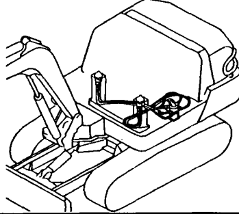
Fig. 91 コントロール配管 (リモコン) 47～マルチ) 47 :4ウェイ, サイドレバー) CONTROL PIPING (REMO. -CON. V.～MULTI V. :4-WAY, SIDE LEVER)
