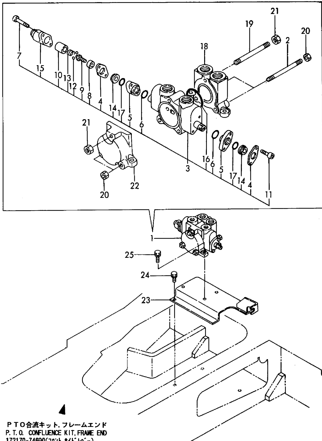
Fig. 72 P.T.O. VALVE(CONFLUENCE)
