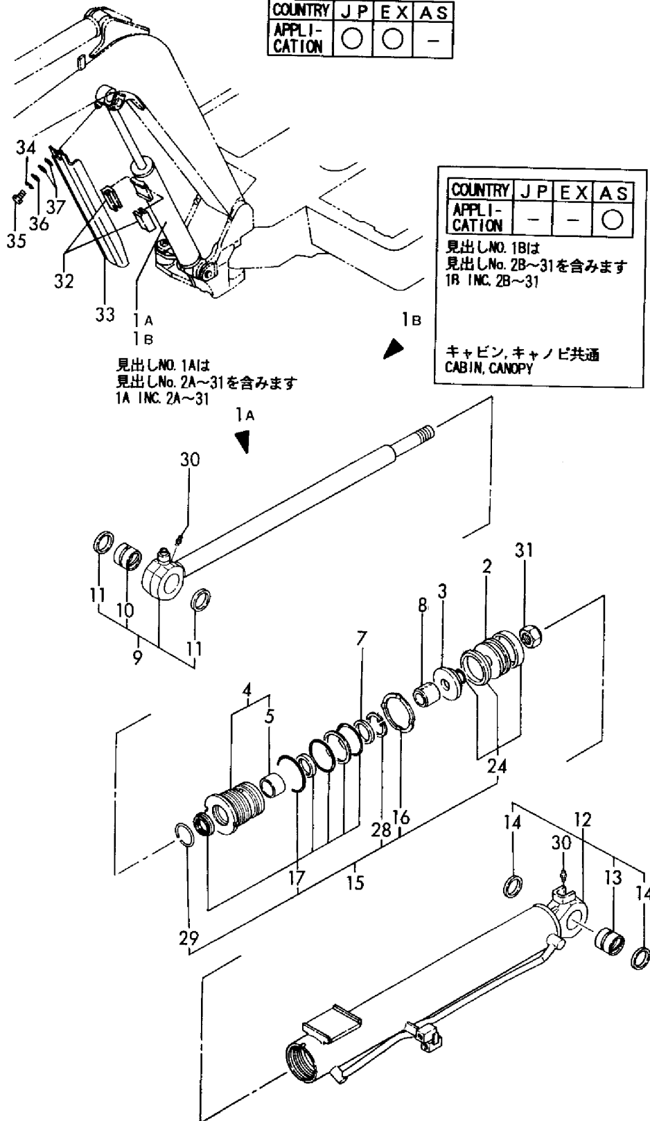
Fig. 48 ブームシリンダ UT(キャビン) BOOM CYLINDER UT(CABIN)
