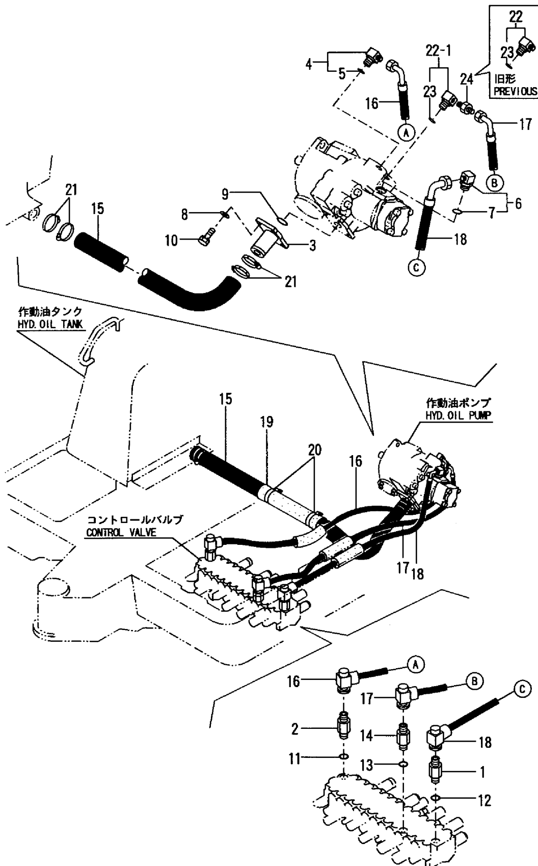
Fig. 74 油圧配管(タンク〜ポンプ〜バルブ) HYD. OIL PIPING(TANK~PUMP~VALVE)
