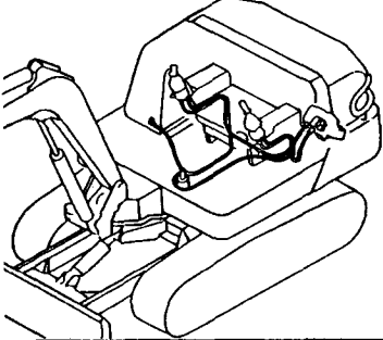
Fig. 87 コントロール配管 (リモコン) 47～コントロール) 47 :ダイレクト, フロントレバー) CONTROL PIPING (REMO. -CON. V.～CON. V. :DIRECT, FRONT LEVER)
