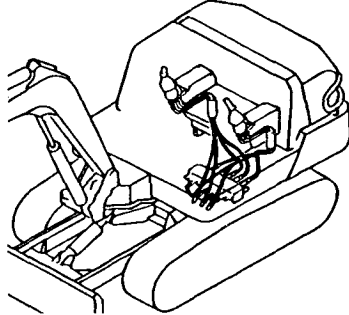
Fig. 90 コントロール配管 (リモコン) 47～マルチ) 47 :4ウェイ, フロントレバー) CONTROL PIPING (REMO. -CON. V.～MULTI V. :4-WAY, FRONT LEVER)
