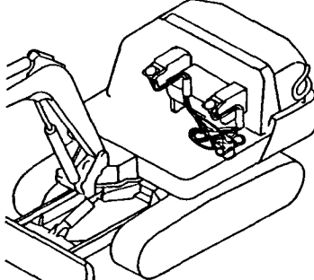
Fig. 92 コントロール配管 (マルチ) 47～コントロール) 47 :4ウェイ) CONTROL PIPING (MULTI V.～CON. V. :4-WAY)
