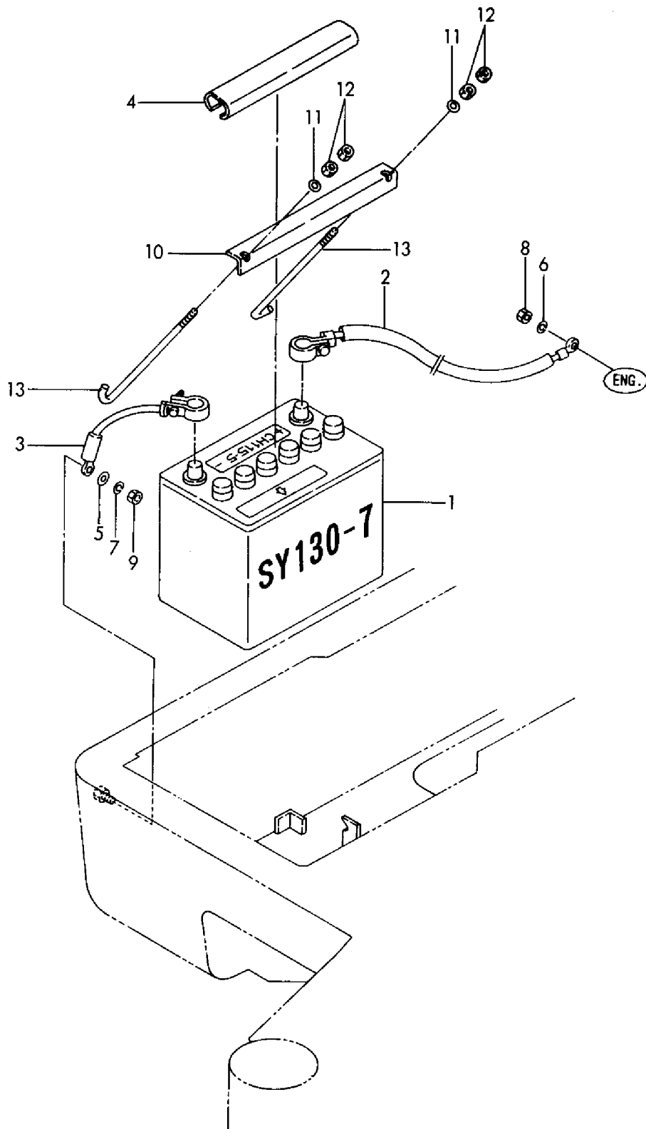
Fig. 16 バッテリー BATTERY
