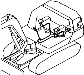
Fig. 86 コントロール配管(ポンプ～リモコン) 47～リターン :サイドレバー AS仕様) CONTROL PIPING(PUMP～REMO. -CON. VALVE～RETURN :SIDE LEVER AS SPEC.)
