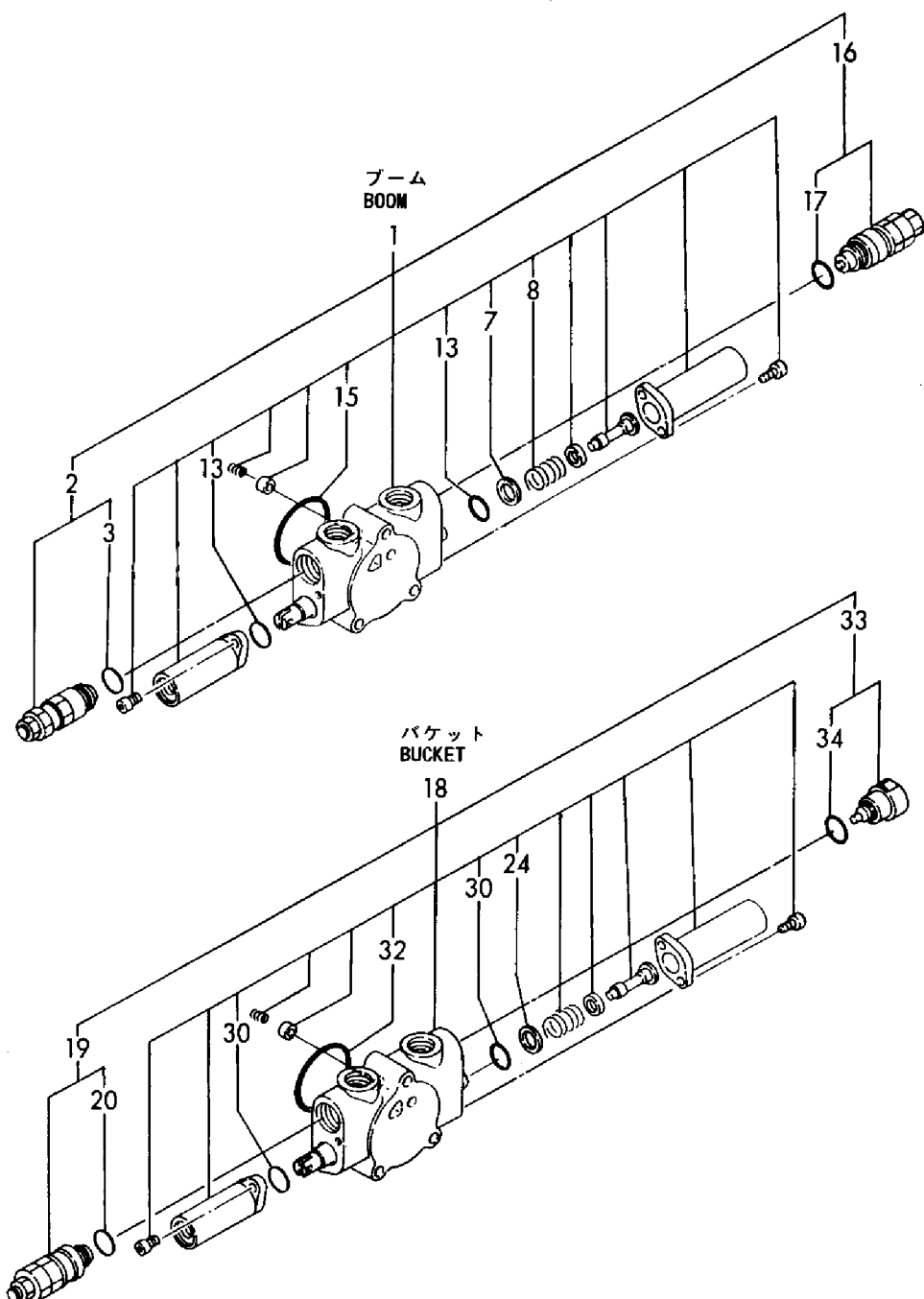
コントロールバルブ ASSY CONTROL VALVE ASSY 172170-74121
