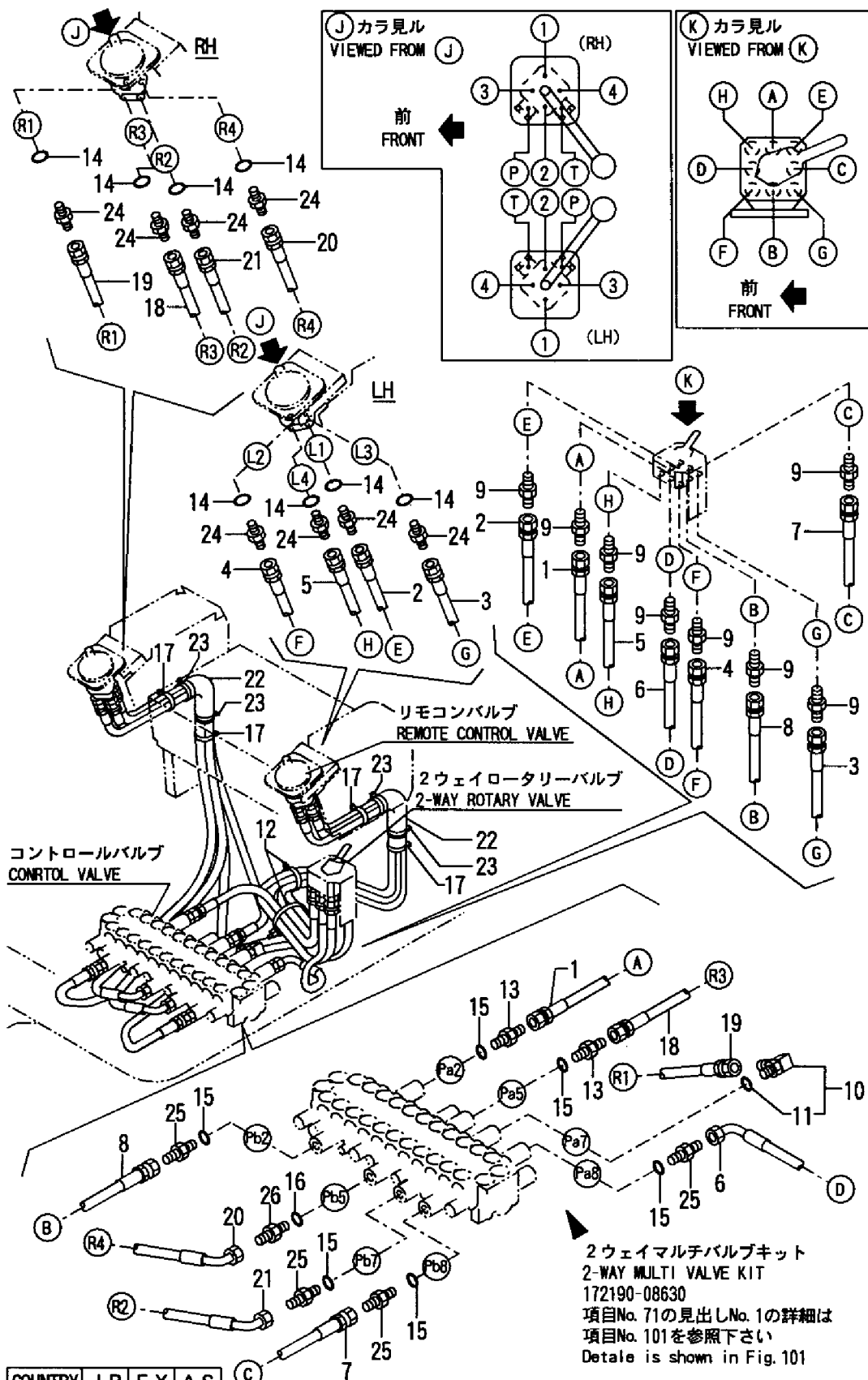
Fig. 94 94 コントロール配管(2ウェイ:サイドレバー) CONTROL PIPING(2-WAY:SIDE LEVER)
