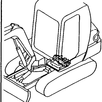
Fig.58 コントロールバルブ (走行 & PTO) CONTROL VALVE(DRIVE & P.T.O.)
