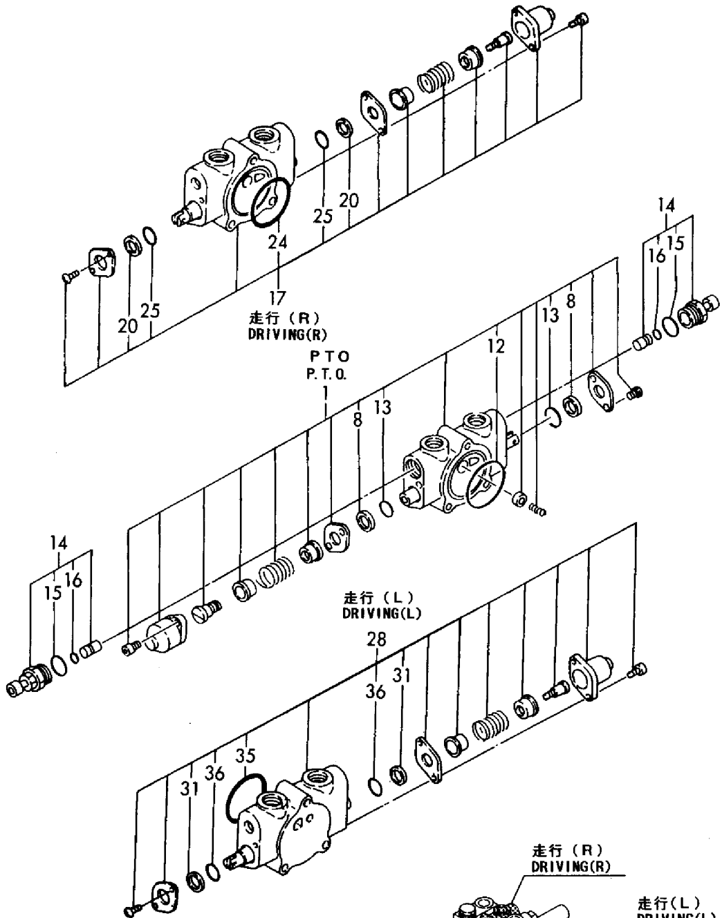
Fig. 63 63 コントロールバルブ(走行 & PTO:PTO仕様) CONTROL VALVE(DRIVE & P. T. O. :P. T. O. SPEC.)
