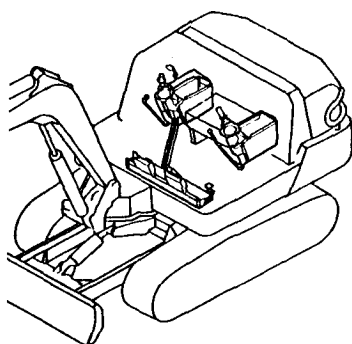
Fig.29 操縦装置(レバー-スタンド) :サイドレバー- AS仕様) CON. EQUIP. (LEVER STAND :SIDE LEVER AS SPEC.)
