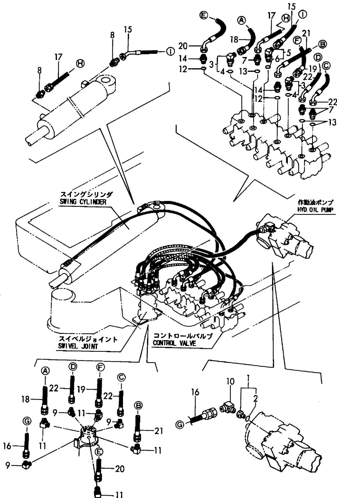
Fig. 76 油圧配管(バルブ～スイベル, スイング) HYD. OIL PIPING (VALVE ~ SWIVEL, SWING)
