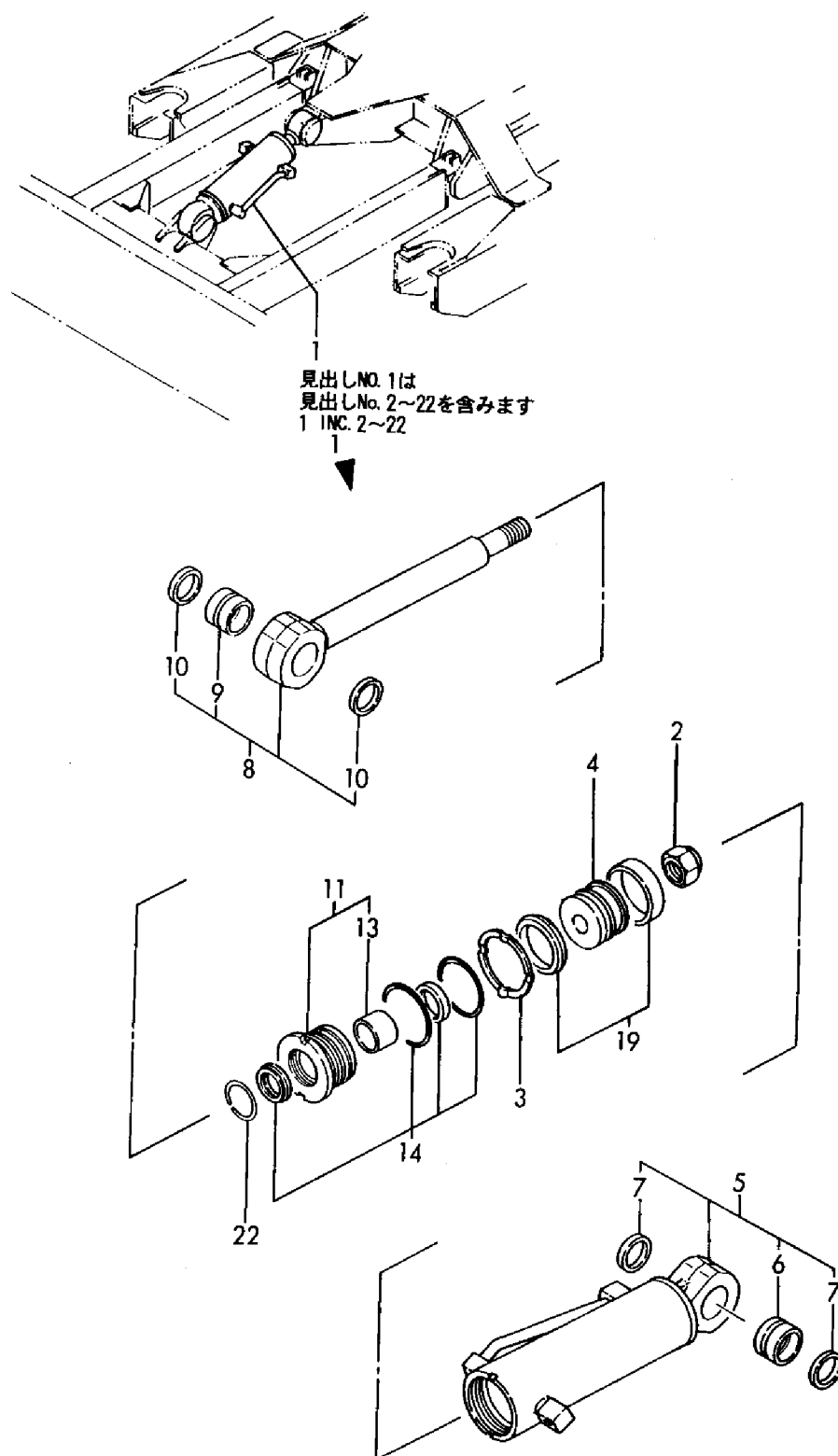
Fig. 53 ブレードシリンダ BLADE CYLINDER
