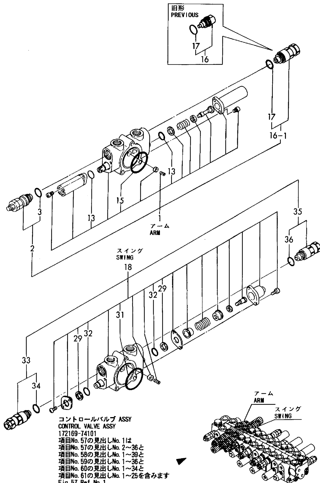
Fig. 59 コントロールバルブ(アーム & スイング) CONTROL VALVE(ARM & SWING)
