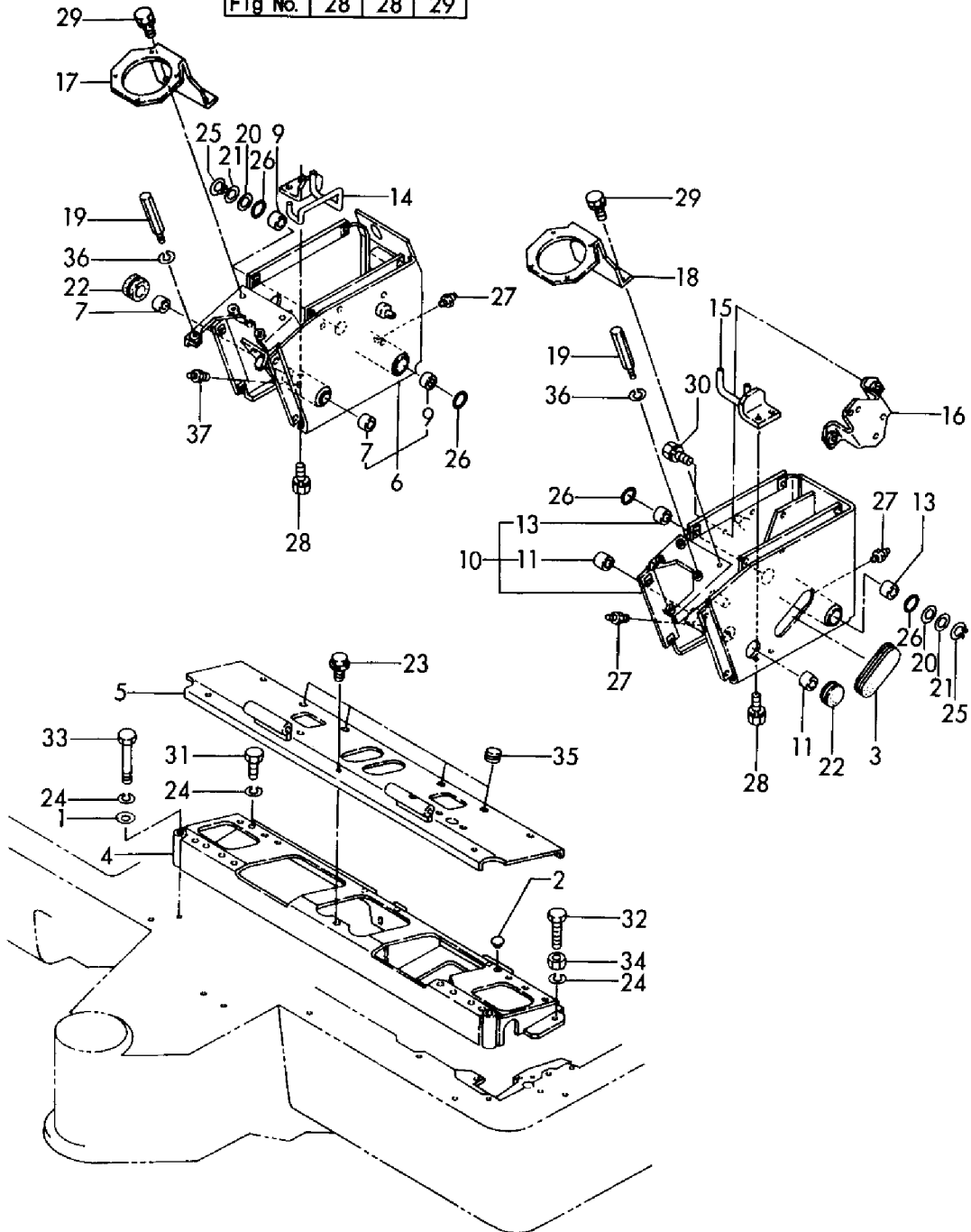
Fig. 29 操縦装置(レバー・スタンド:サイドレバー AS仕様) CONTROL EQUIP. (LEVER STAND:SIDE LEVER AS SPEC. )
