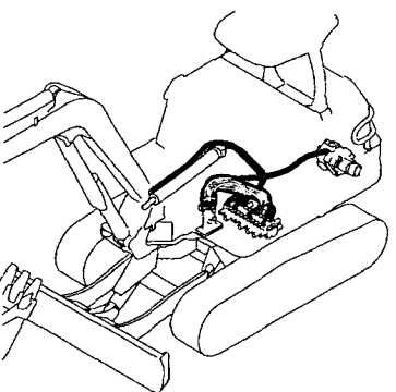
Fig. 92 油圧配管 (リターン) HYD. OIL PIPING (RETURN)
