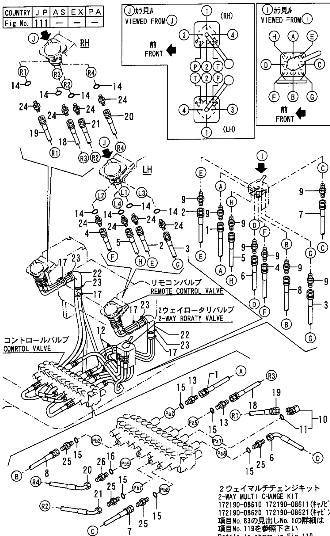
Fig. 111 カントロル配管(マルチチェンジ:2ウェイ、サイドレバー) CONTROL PIPING (MULTI CHANGE: 2-WAY, SIDE LEVER)
