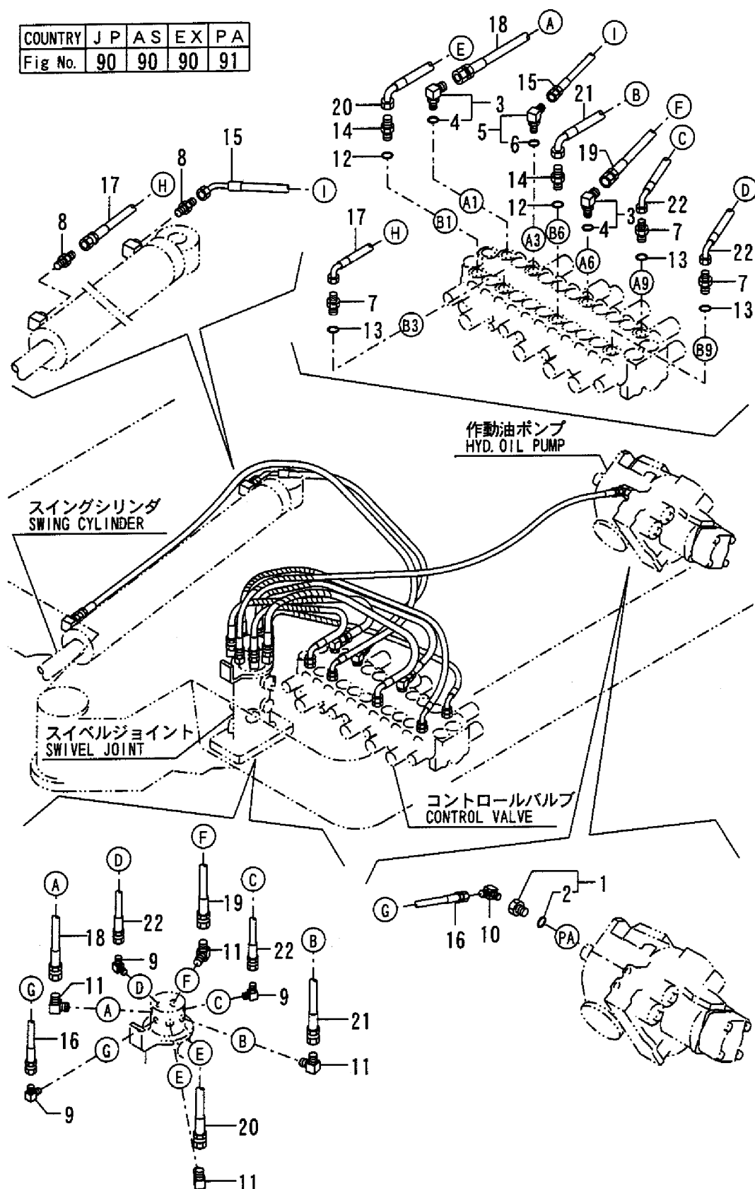
Fig. 91 油圧配管(バルブ〜スイング、スイング) (PA) HYD. OIL PIPING (VALVE~SWIVEL, SWING) (PA)
