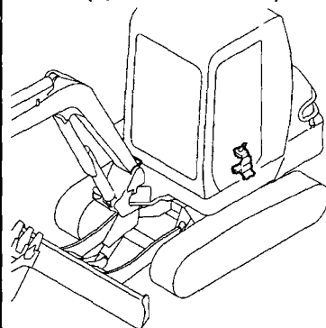
Fig. 84 P.T.O.バルブ (合流) P. T. O. VALVE (CONFLUENCE)
