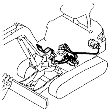
Fig. 90 油圧配管 (バルブ ~ スイベル、スイング) HYD. OIL PIPING (VALVE ~ SWIVEL, SWING)
