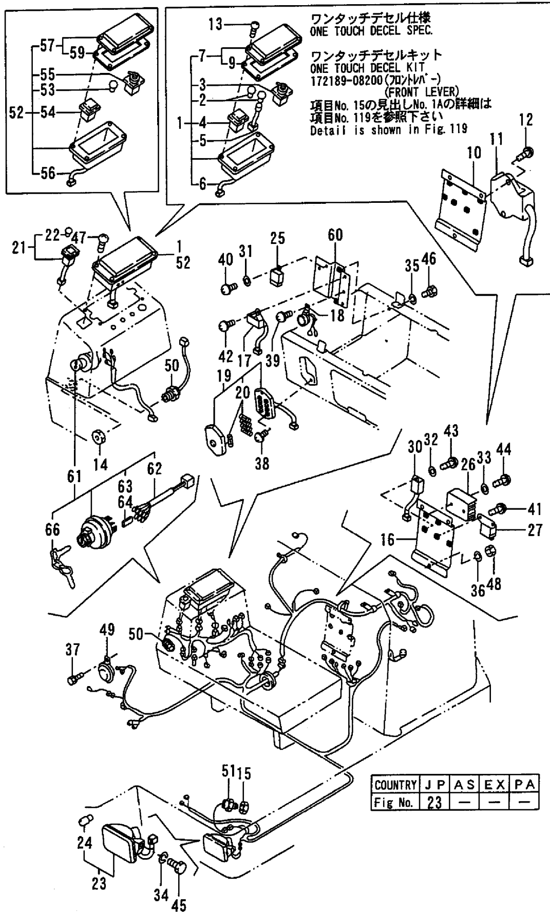
Fig. 23 電装品(機器:フロントレバー) ELECTRIC PART (EQUIPMENT: FRONT LEVER)
