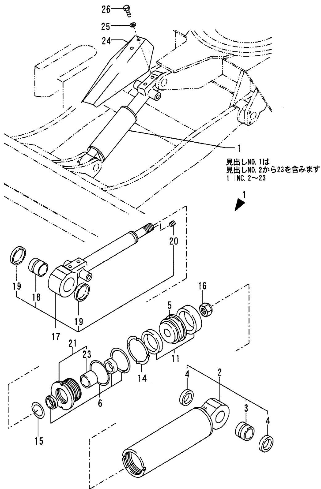
Fig. 63 ブレードシリンダ BLADE CYLINDER
