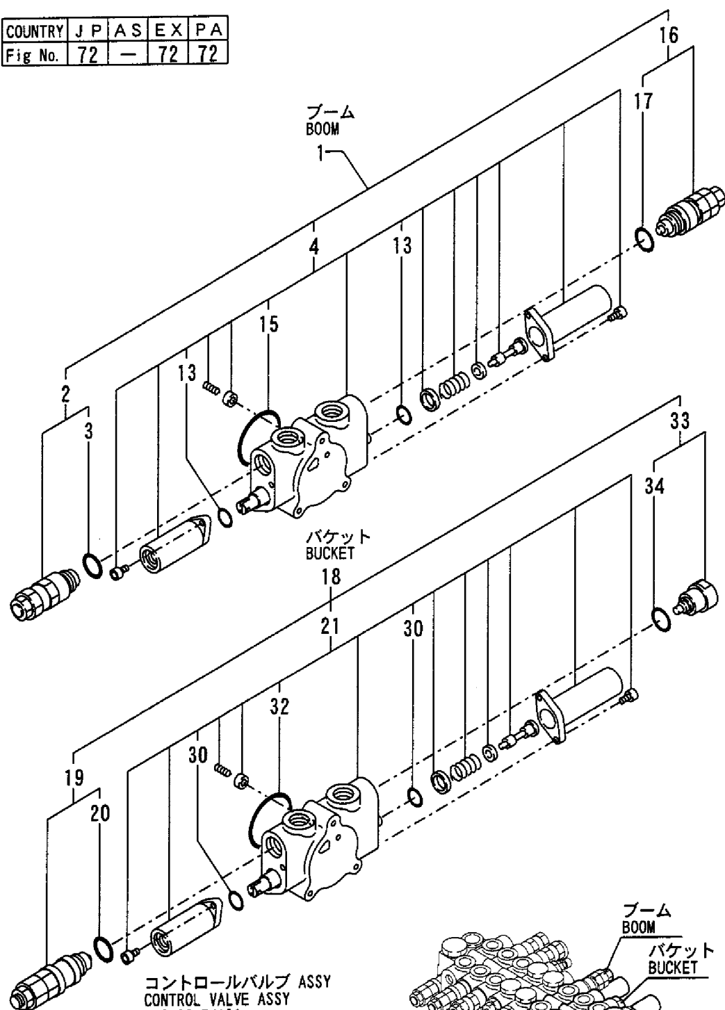
Fig. 72 コントロールバルブ(ブーム & バケット:標準仕様) CONTROL VALVE (BOOM & BUCKET:STANDARD SPEC.)
