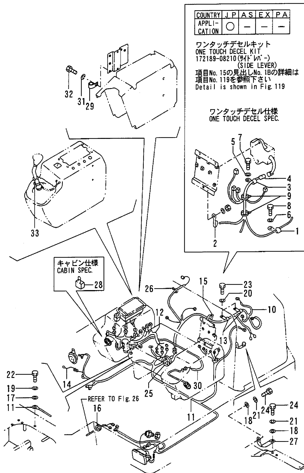
Fig. 22 電装品 (ワयर) (Wiring) (サイドレバー) ELECTRIC PART (WIRING: SIDE LEVER)
