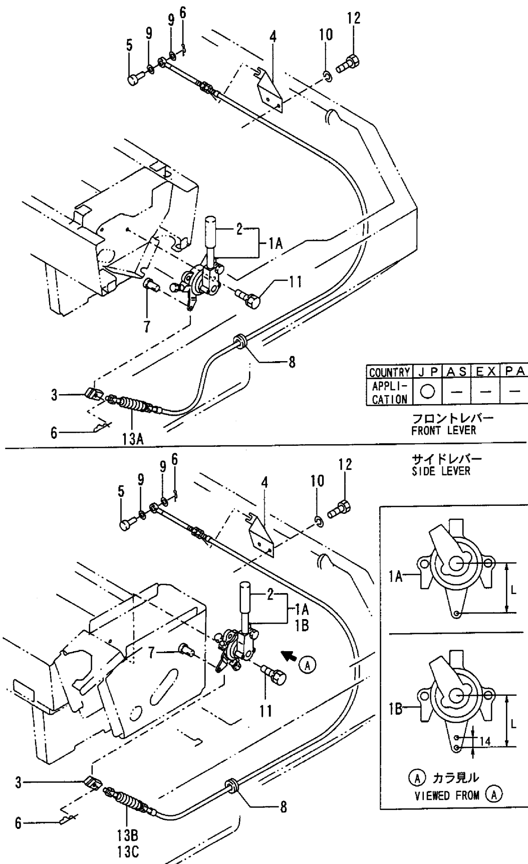
Fig. 14 アクセル(標準仕様) ACCELERATOR LEVER (STANDARD SPEC.)
