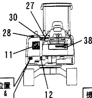
2ウェイバルブ部 2-WAY VALVE PART
