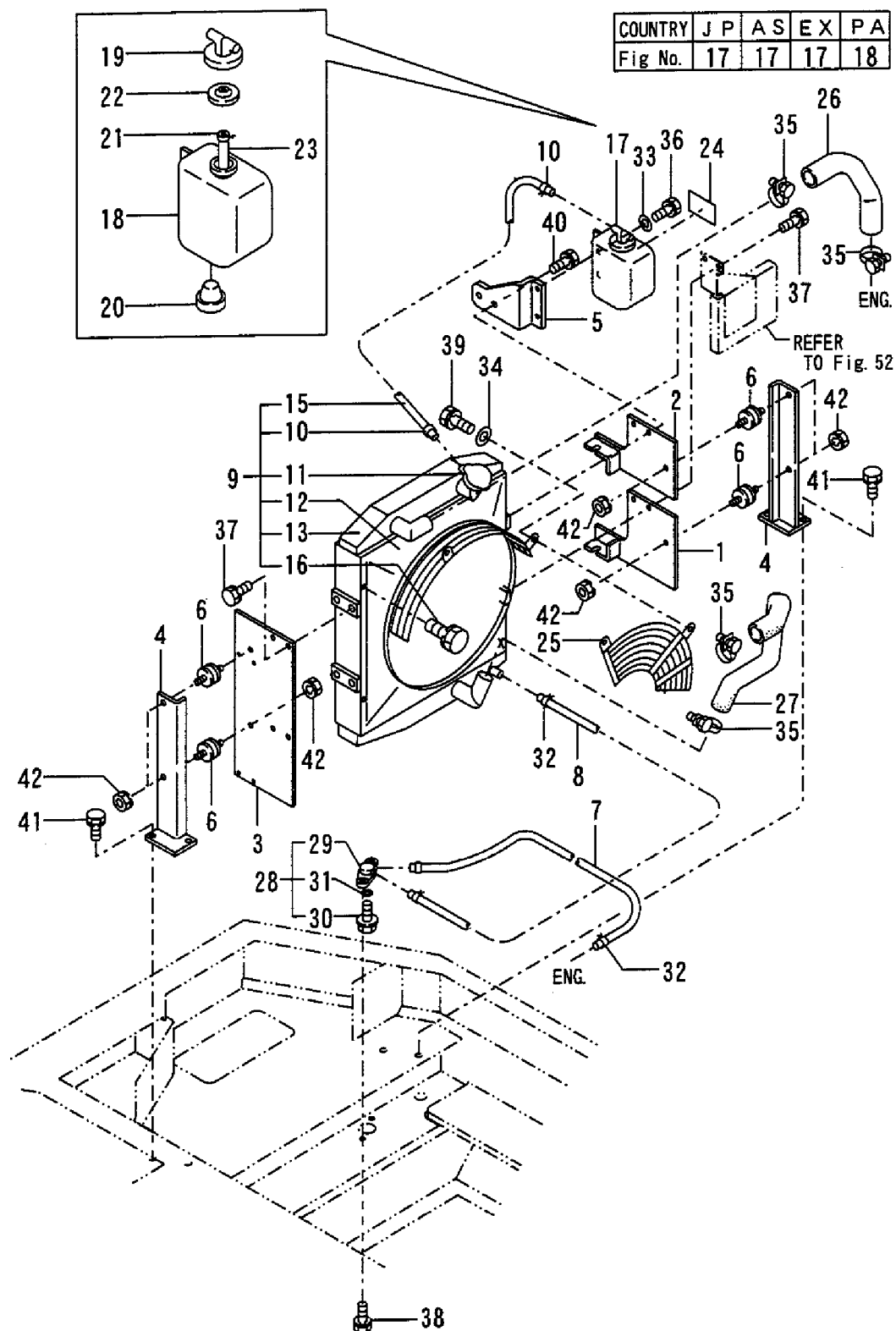
Fig. 18 ラジエータ & マウント (PA) RADIATOR & MOUNT (PA)
