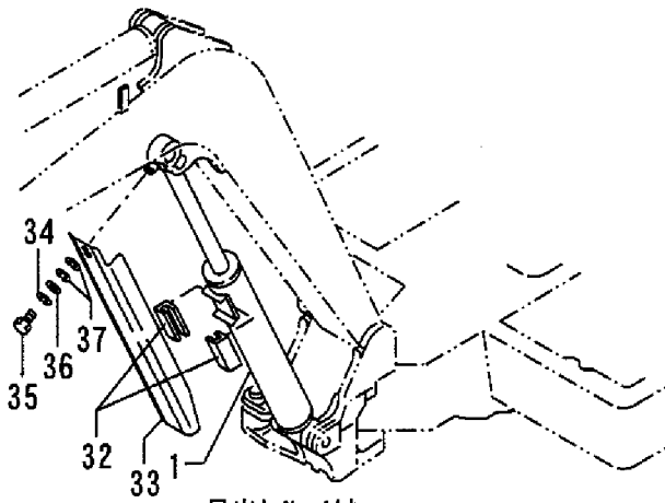
Fig. 59 ブームシリンダ(キャブ) BOOM CYLINDER (CANOPY)
