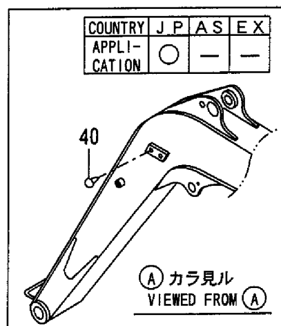
Fig. 113 ブーム & アームブレース BOOM & BOOM BRACKET
