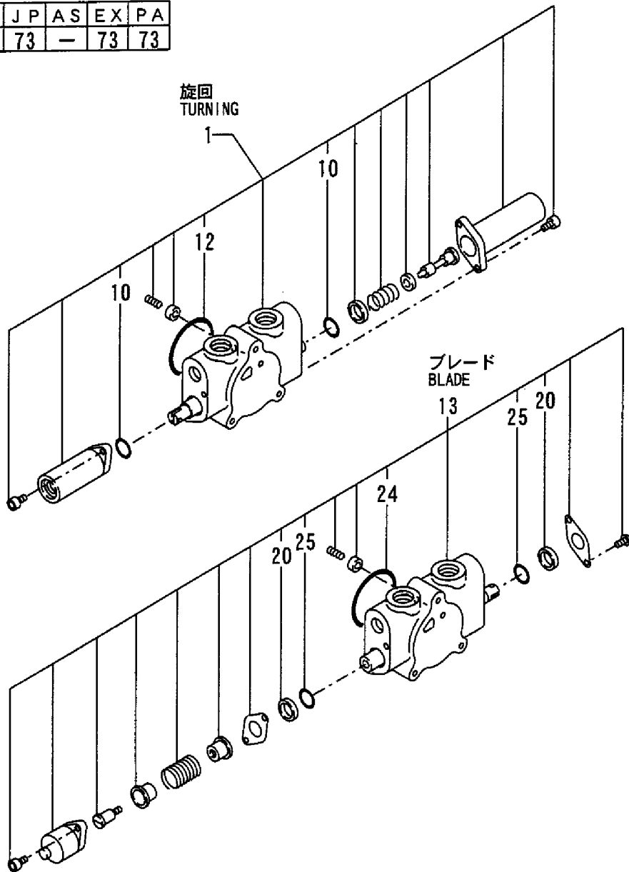
Fig. 73 73 コントロールバルブ(旋回 & ブレード:標準仕様) CONTROL VALVE (TURNING & BLADE: STANDARD SPEC.)
