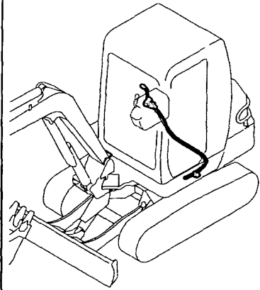
Fig. 38 操縦装置(カットオフレバー & ペダル:フロントレバー) CONTROL EQUIPMENT (CUT OFF LEVER & PEDAL: FRONT LEVER)
