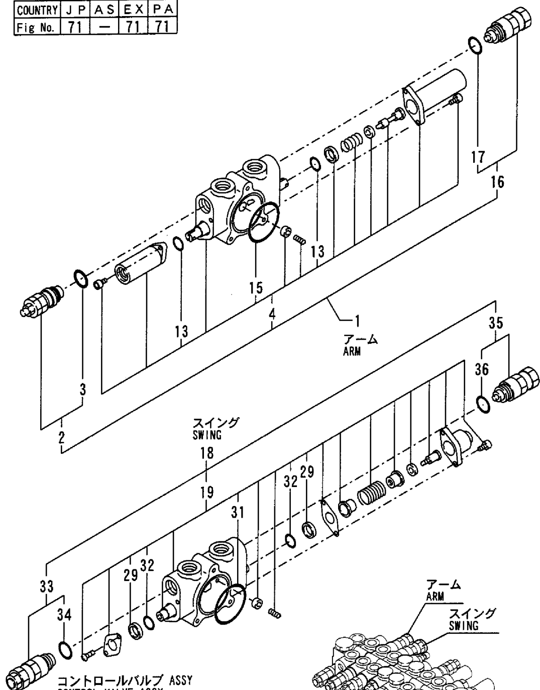
Fig. 71 コントロールバルブ(アーム & スイング : 標準仕様) CONTROL VALVE (ARM & SWING: STANDARD SPEC.)
