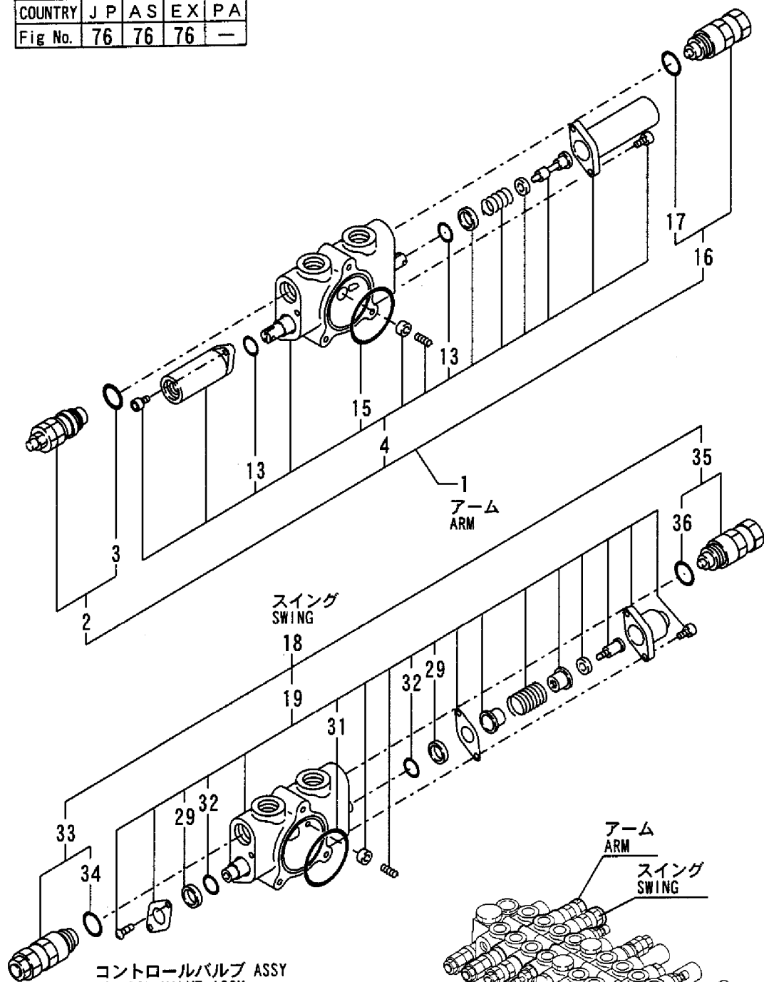
Fig. 76 コントロールバルブ(アーム & スイング : P.T.O仕様) CONTROL VALVE (ARM & SWING: P. T. O. SPEC.)
