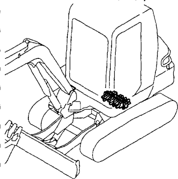
Fig. 79 リモコンバルブ REMOTE CONTROL VALVE
