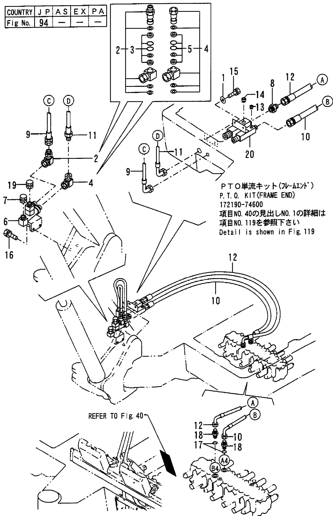
Fig. 94 油圧配管 (P.T.O., フレームエンド: 単流仕様) HYD. OIL PIPING (P. T. O., FRAME END: UNIFLOW SPEC.)
