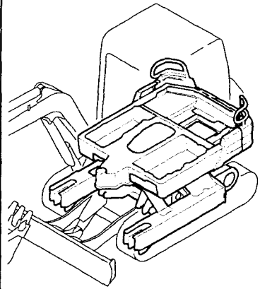
Fig. 42 フレーム & 旋回ベアリング (PA) FRAME & TURNING BEARING (PA)
