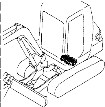
Fig. 74 コントロールバルブ (ポート & バルブ台: P.T.O.仕様) CONTROL VALVE (P. PORT & V. STAND: P. T. O.)
