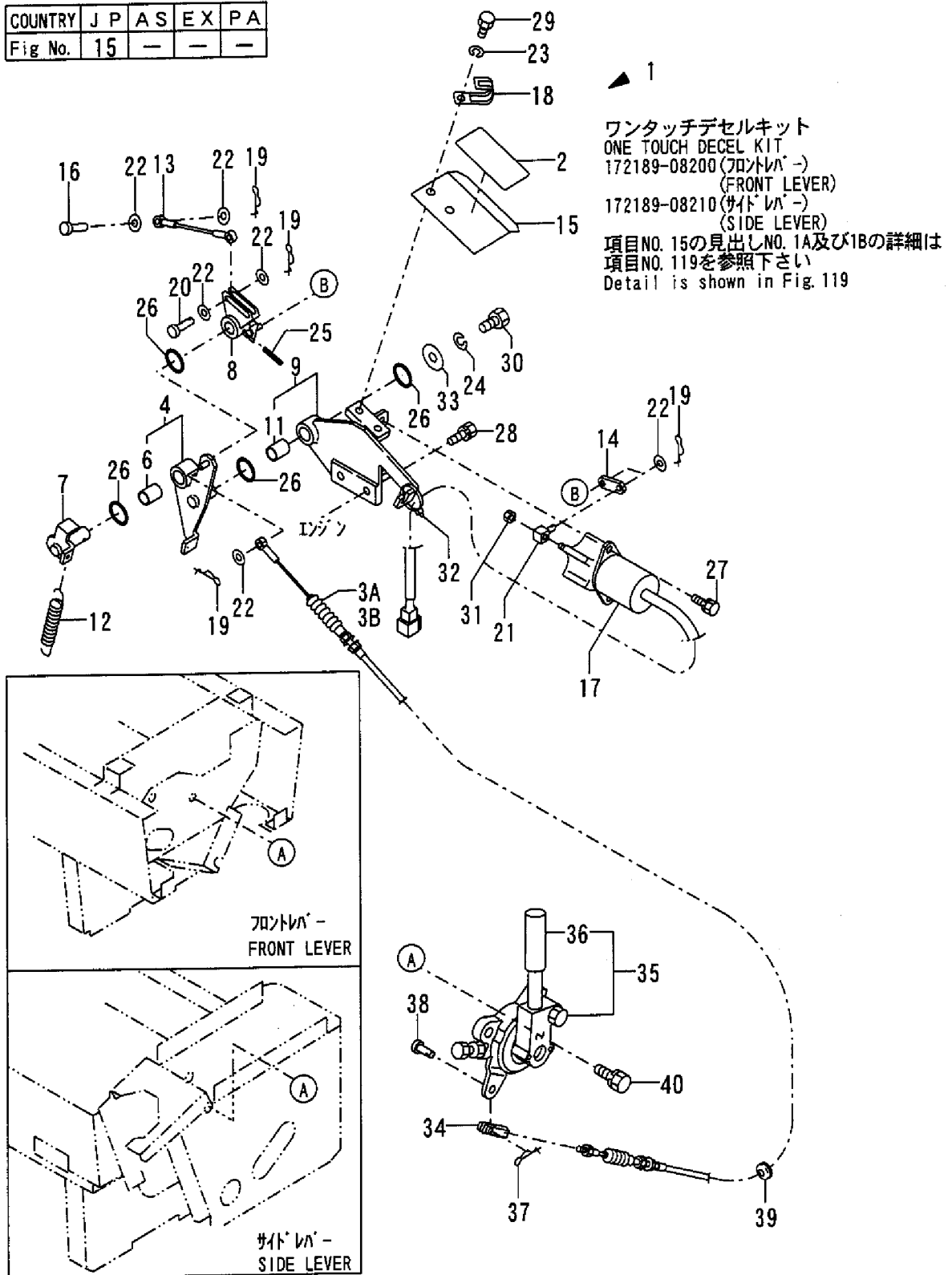
Fig. 15 アクセル(ワンタッチデセル仕様) ACCELERATOR LEVER(ONE TOUCH DECEL SPEC.)
