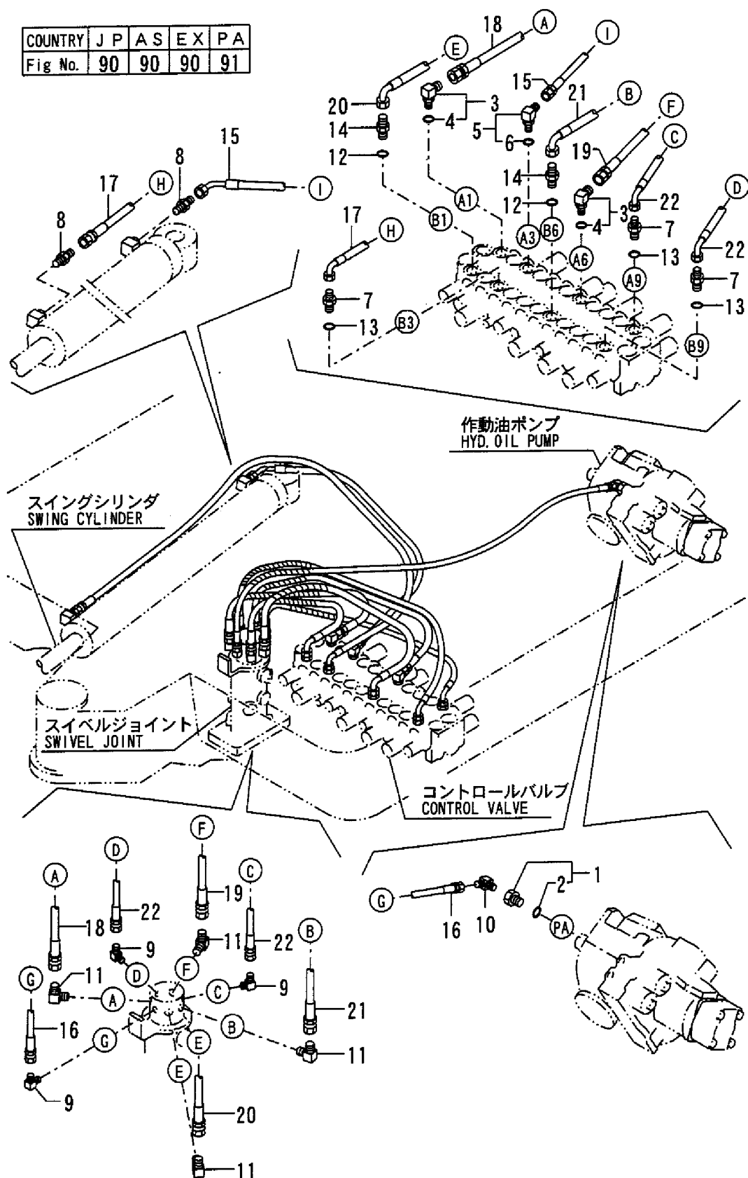
Fig. 90 油圧配管(バルブ～スイング、スウィング) HYD. OIL PIPING (VALVE~SWIVEL, SWING)
