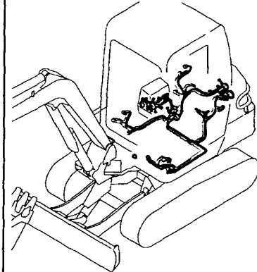
Fig. 22 電装品 (ワイリグ : サイドバー) ELECTRIC PART (WIRING: SIDE LEVER)
