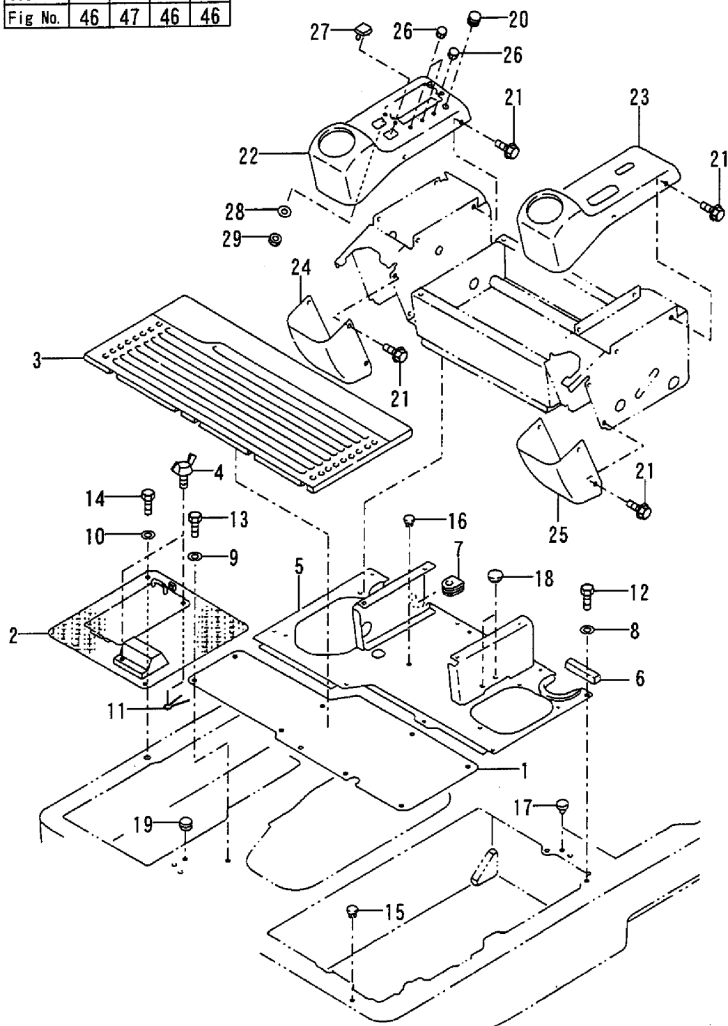
Fig. 47 ステップ & インstrument パネル (サイドバー) (AS) STEP & INSTRUMENT PANEL (SIDE LEVER) (AS)
