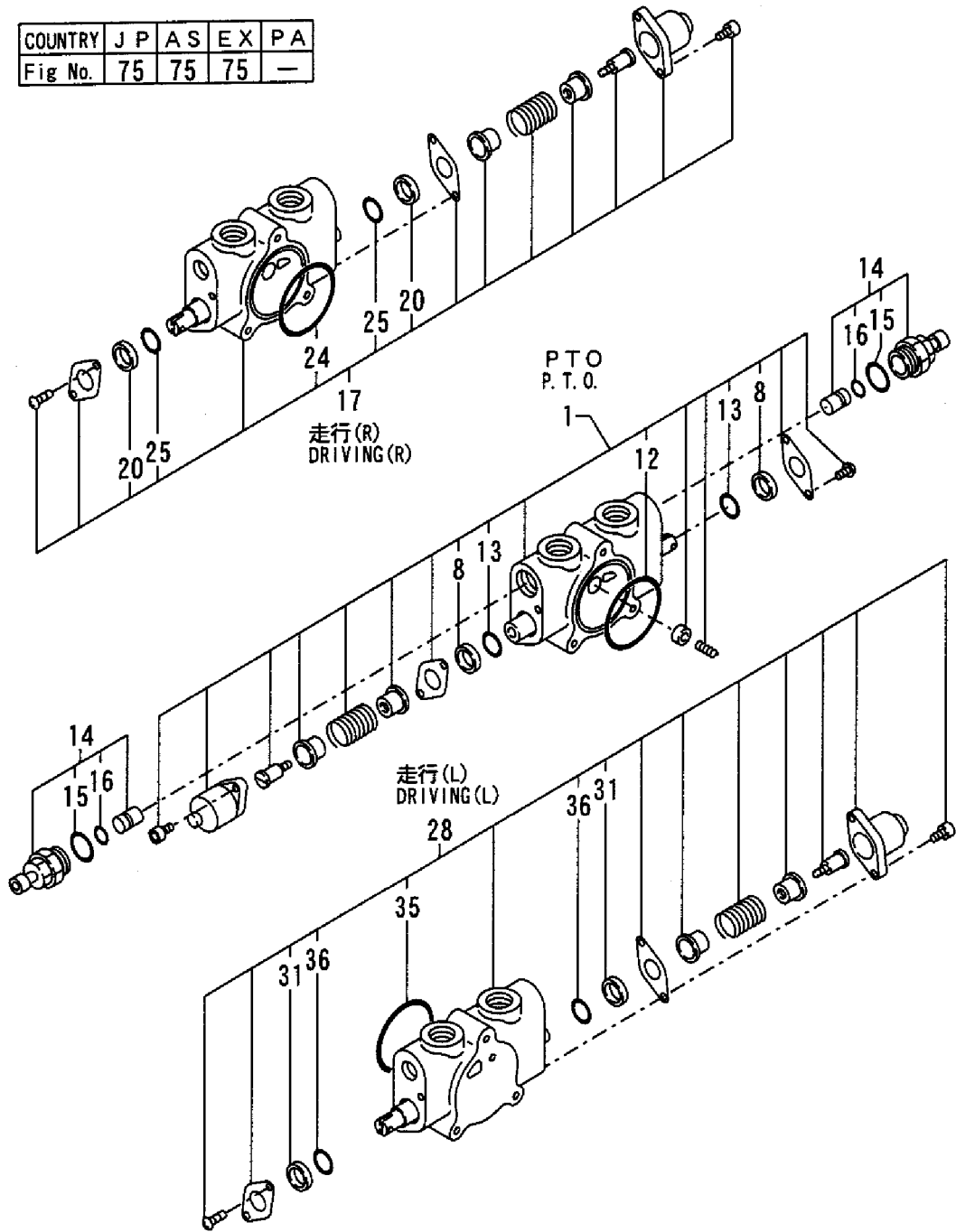
Fig. 75 75 コントロールバルブ(走行 & PTO:PTO仕様) CONTROL VALVE (DRIVE & P. T. O. : P. T. O. SPEC.)
