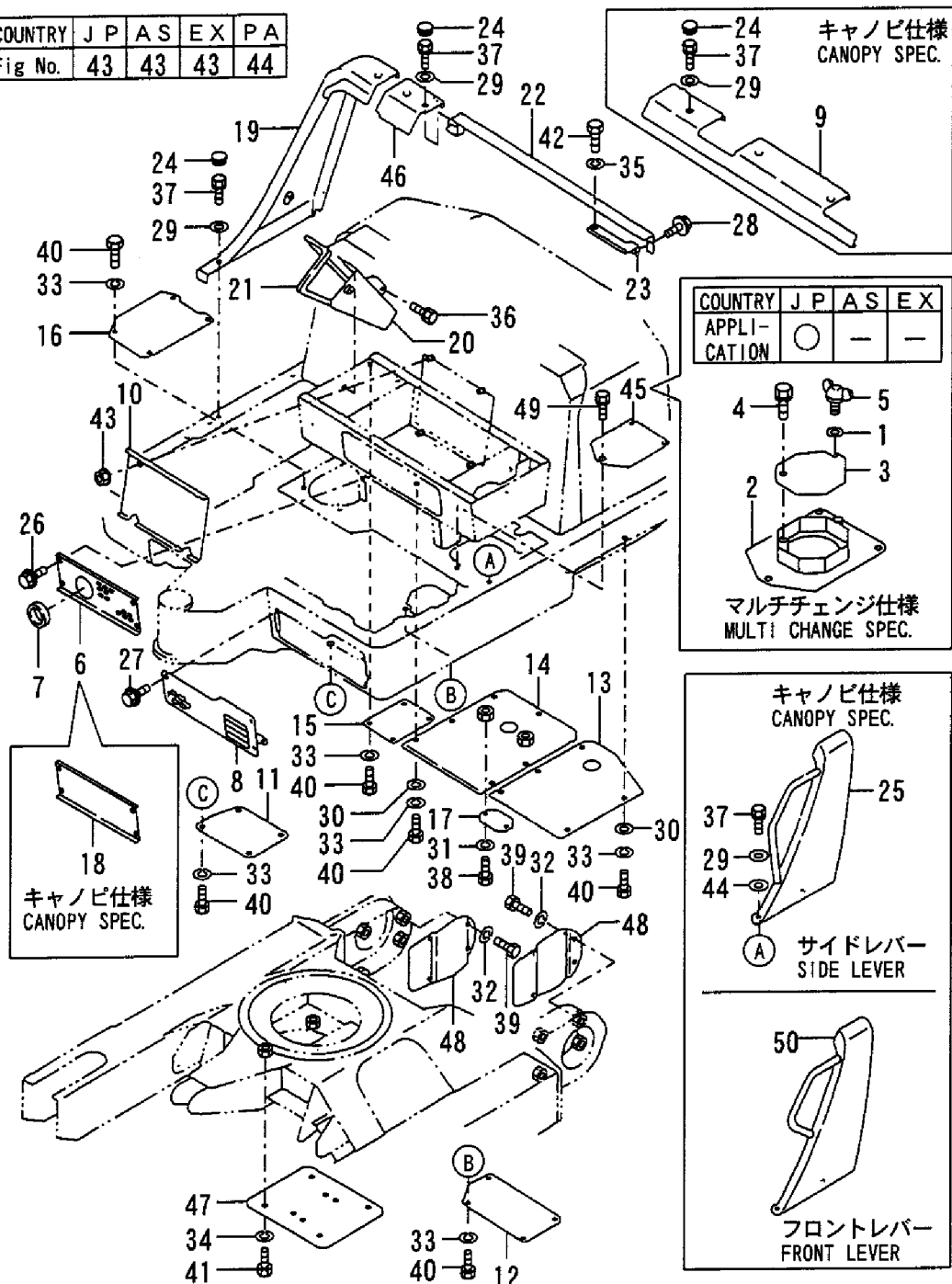
Fig. 43 フレームカバー FRAME COVER
