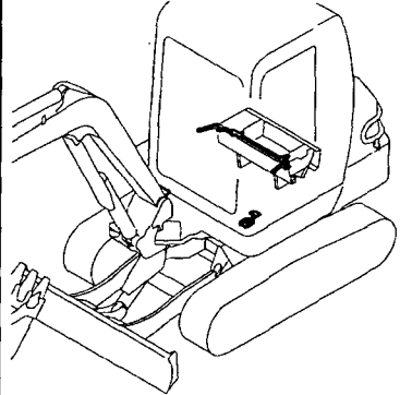
Fig. 39 操縦装置(カットオフレバー & ペダル:サイドレバー) CONTROL EQUIPMENT (CUT OFF LEVER & PEDAL: SIDE LEVER)
