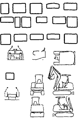
Fig. 8 安全銘板(キャビン) (JP) SAFETY LABEL (CANOPY) (JP)
