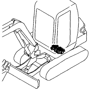
Fig. 72 コントロールバルブ (ブーム & バケット: 標準仕様) CONTROL VALVE (BOOM & BUCKET : STANDARD SPEC.)
