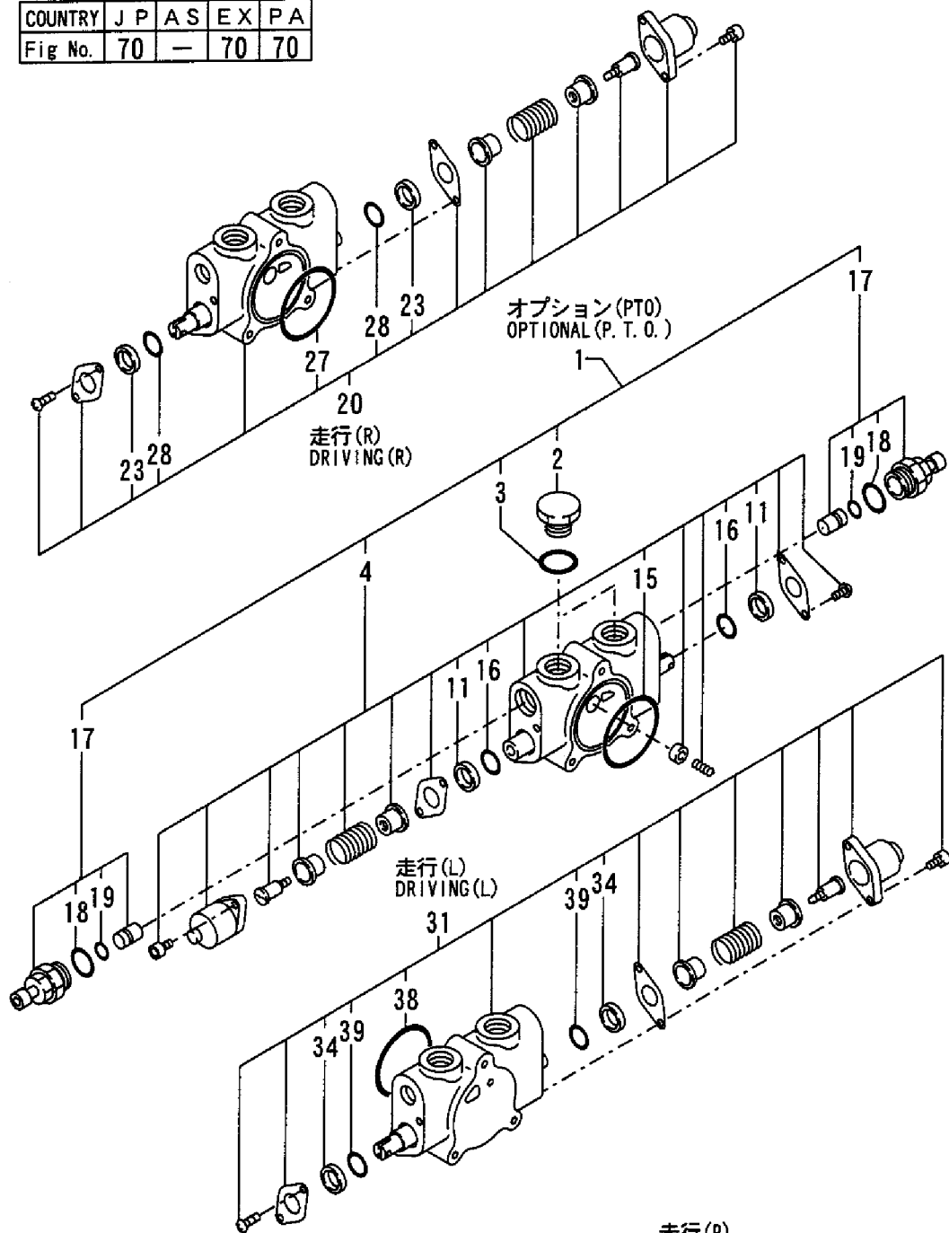
Fig. 70 70 コントロールバルブ(走行 & PTO:標準仕様) CONTROL VALVE (DRIVE & P. T. O. : STANDARD SPEC.)
