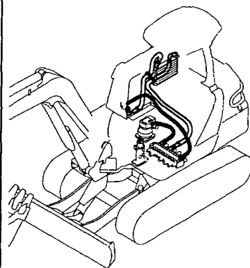
Fig. 94 油圧配管 (PTO、フレームエンド : 単流仕様) HYD. OIL PIPING (P. T. O., FRAME END: UNIFLOW SPEC.)
