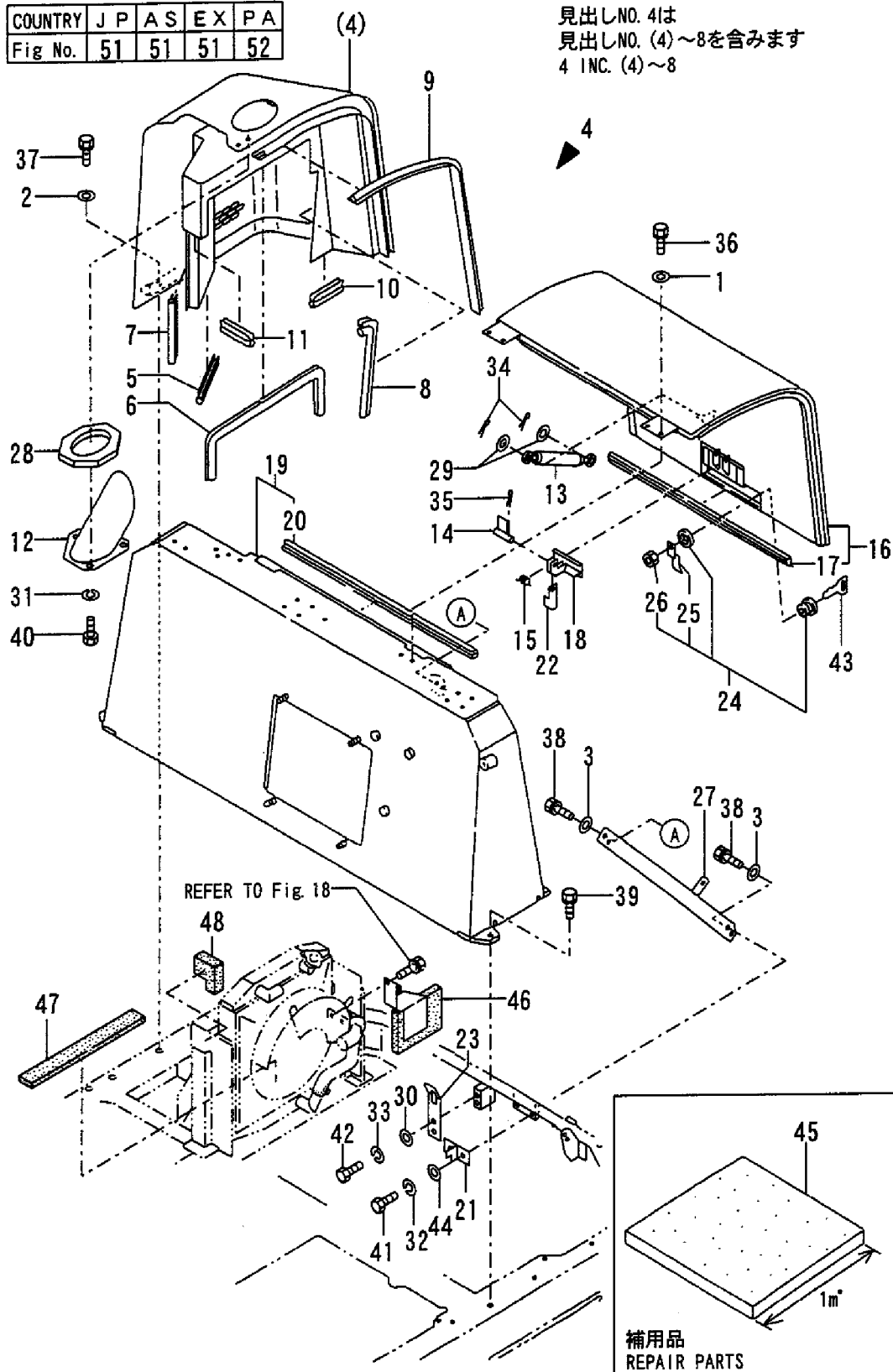
Fig. 52 ボンネット(PA) BONNET (PA)
