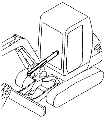
Fig. 63 ブレードシリンダ BLADE CYLINDER
