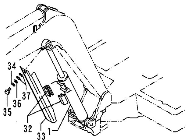
Fig. 58 ブームシリンダ(キャビン) BOOM CYLINDER (CABIN)
