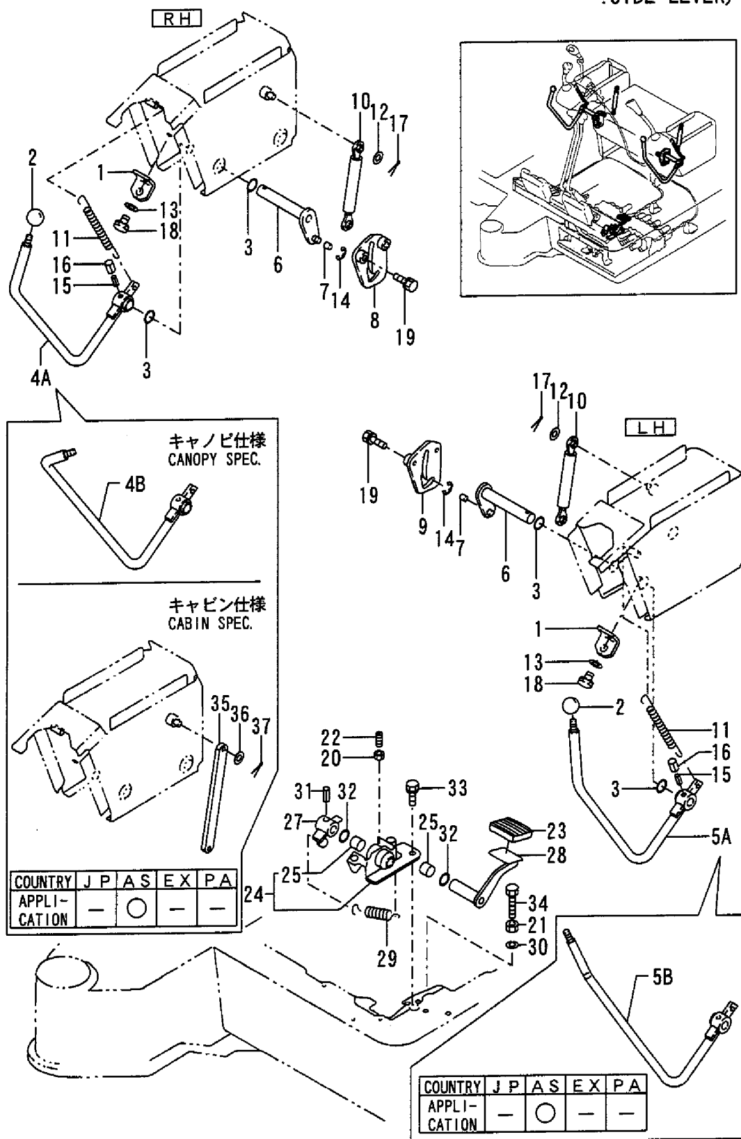
39 操縦装置(カトリバ & ハンダル:サイドレバー) Fig. 39 CONTROL EQUIPMENT (CUT OFF LEVER & PEDAL :SIDE LEVER)
