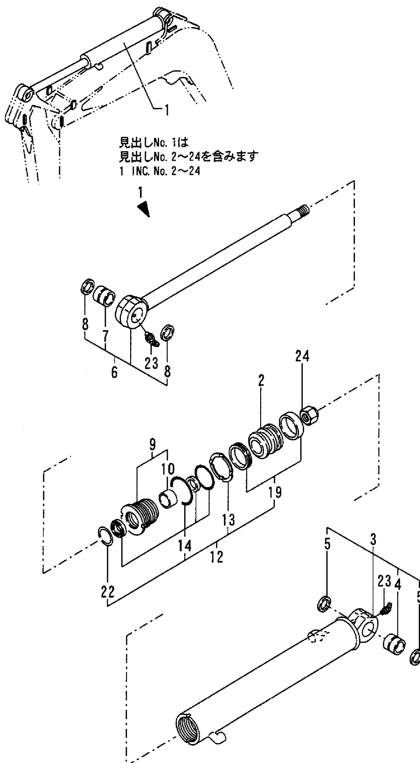
Fig. 60 アーミングシリンダ ARM CYLINDER https://truckingmanualshub.com/
