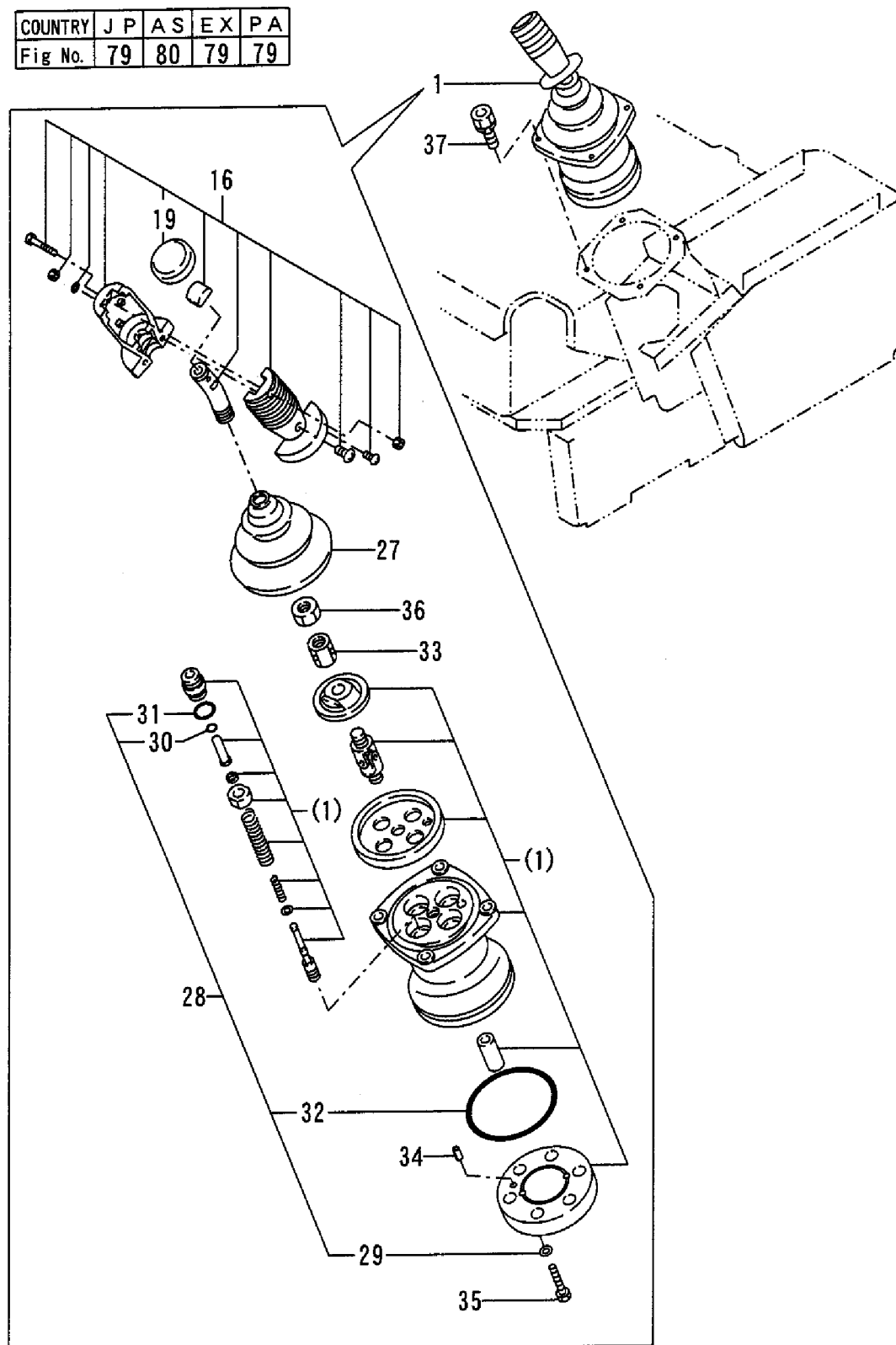
リモコンバルブ(L)(AS) REMOTE CONTROL VALVE(L)(AS)
