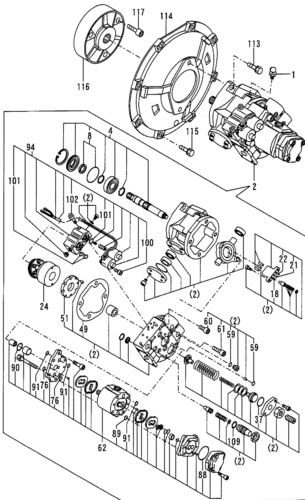
57 油圧ポンプ & 軸継手 Fig. 57 HYD. OIL PUMP & JOINT
