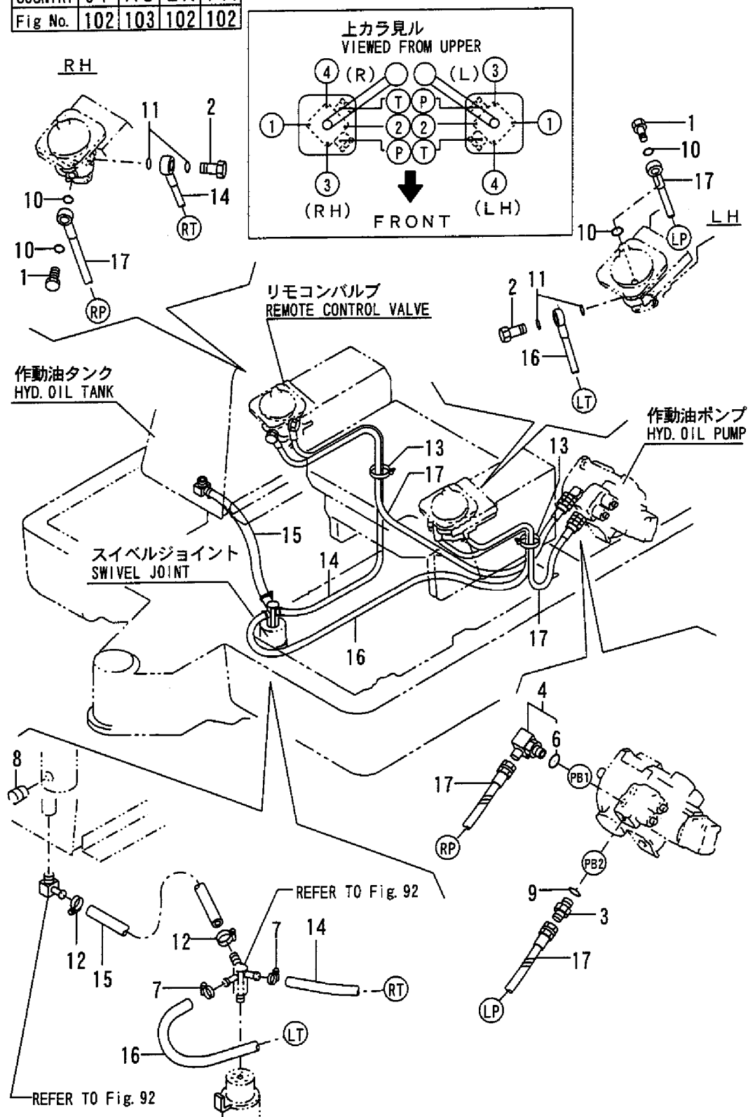
Fig. 102 http://www.mh.co.jp/ (ポンプ～リモコンバルブ～リターン:サイドレバー) CONTROL PIPING (PUMP~REMOTE CONTROL V.~RETURN:SIDE LEVER)
