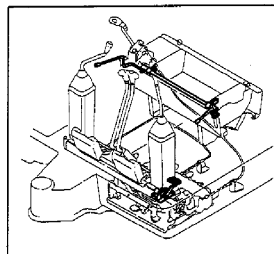
Fig. 38 38 操縦装置(カットオフレバー & ペダル:フロントレバー) CONTROL EQUIPMENT (CUT OFF LEVER & PEDAL :FRONT LEVER)
