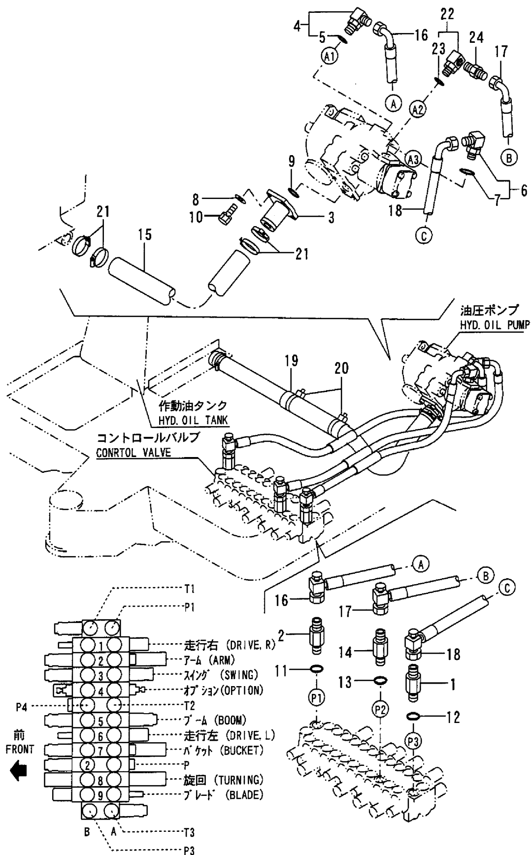
Fig. 87 油圧配管(タンク～ポンプ～バルブ) HYD. OIL PIPING (TANK ~ PUMP ~ VALVE)
