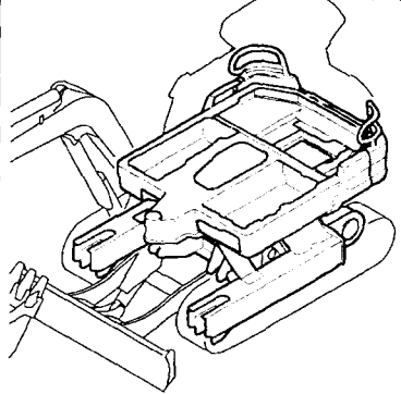
Fig. 43 フレームカバー FRAME COVER
