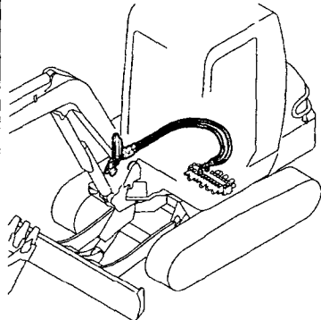
Fig. 95 油圧配管 (PTO、フレームエンド : 合流仕様) HYD. OIL PIPING (P. T. O., FRAME END: CONFLUENCE SPEC.)
