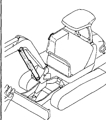
Fig. 60 アームシリンダ ARM CYLINDER
