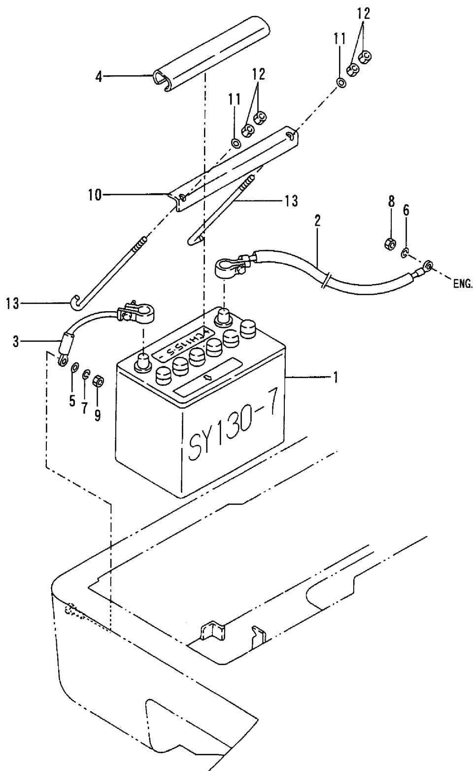
Fig. 20 バッテリー BATTERY http://truckmanualshub.com/
