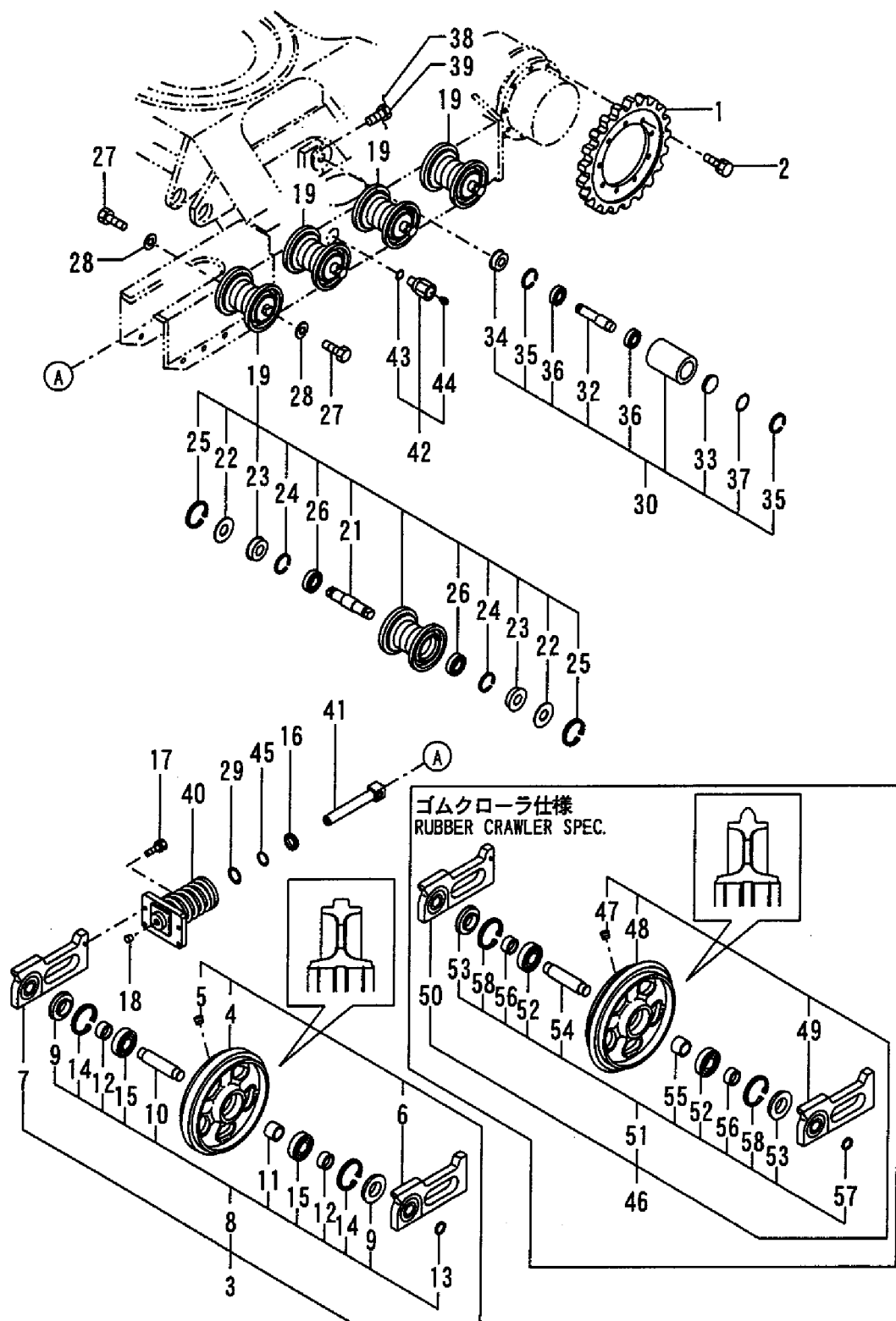
Fig. 29 ローラー & アジャスト ROLLER & ADJUST
