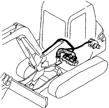
Fig. 91 油圧配管 (バルブ ~ スイベル、スイング) (PA) HYD. OIL PIPING (VALVE ~ SWIVEL, SWING) (PA)
