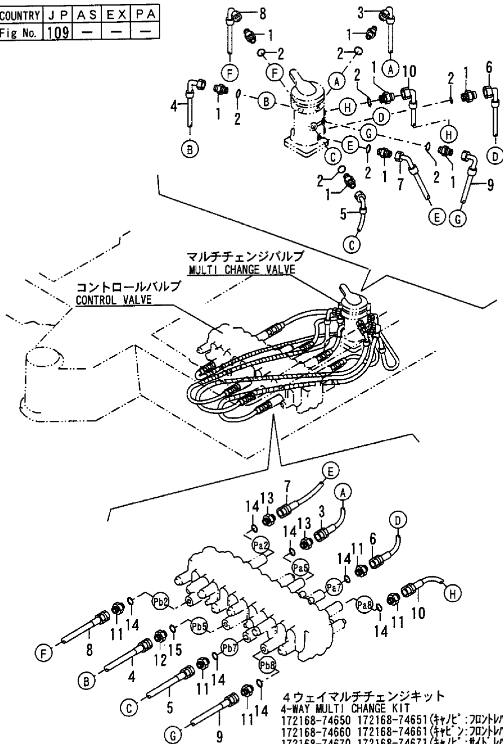
Fig. 109 コントロール配管(マルチバルブ ~コントロールバルブ :4ウェイ) CONTROL PIPING (MULTI V. ~CONTROL V. :4-WAY)
