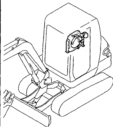
Fig. 18 ラジエータ & マウント (PA) RADIATOR & MOUNT (PA)
