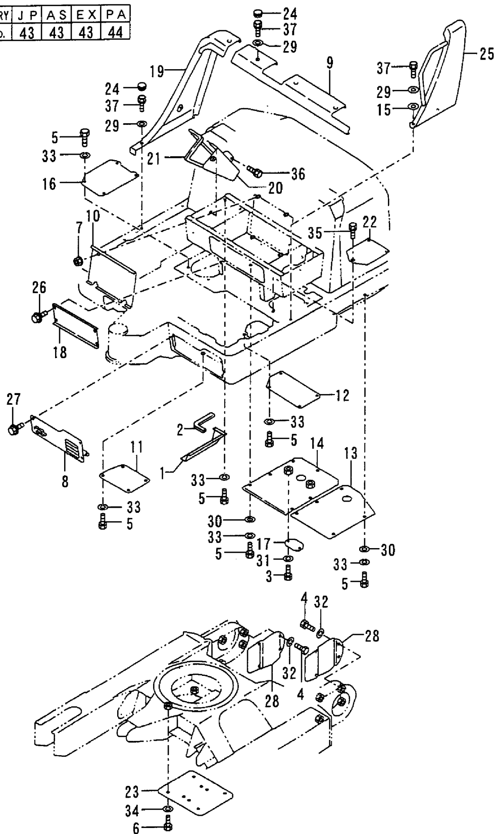
Fig. 44 フレームカバー (PA) FRAME COVER (PA)
