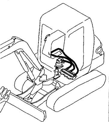
Fig. 92 油圧配管 (リターン) HYD. OIL PIPING (RETURN)
