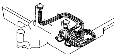
Fig. 91 コントロール配管 (リモコンバルブ ～コントロールバルブ /ダイレクト, サイドレバー) CONTROL PIPING (REMO. -CON. V. ~ CONTROL V. / DIRECT, SIDE LEVER)
