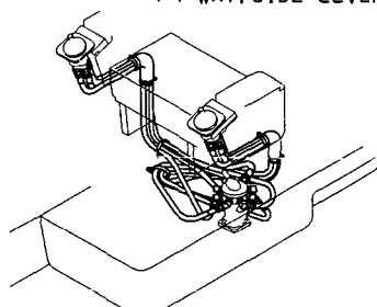
Fig. 95 コントロール配管 (マルチバルブ ～コントロールバルブ /4ウェイマルチ) CONTROL PIPING (MULTI V. ~ CONTROL V. / 4-WAY MULTI)
