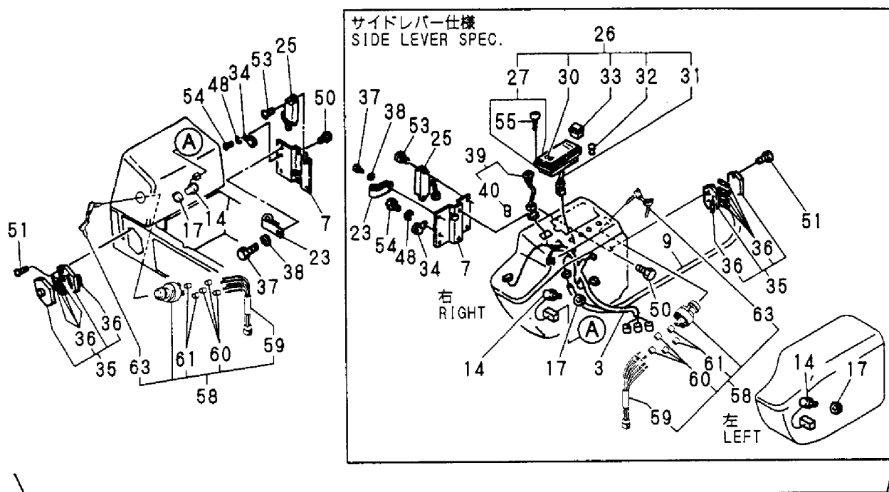
Fig. 17 電装品 (キャビン、キャノピ) ELECTRIC PART (CABIN, CANOPY)
