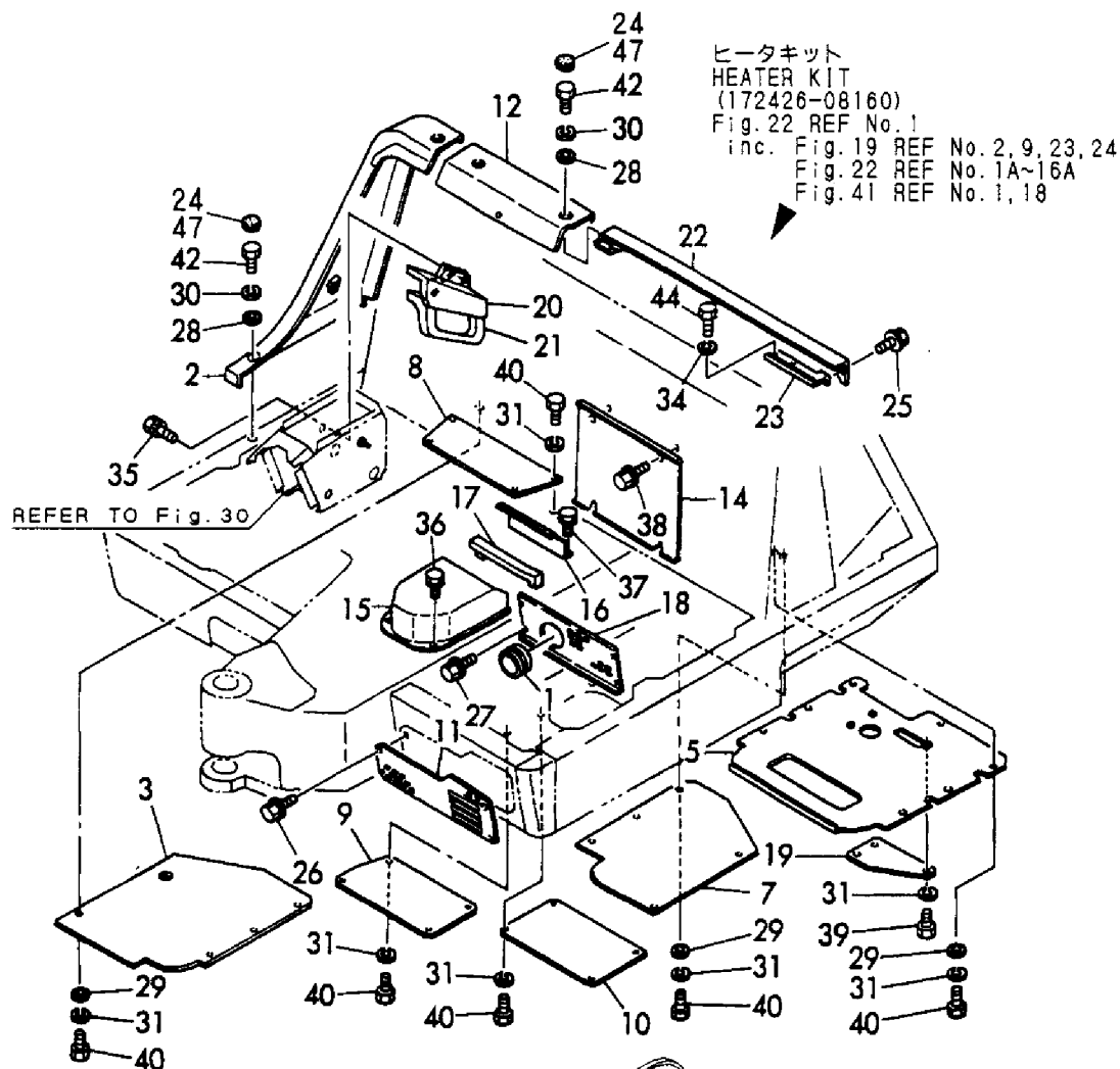
Fig. 41 フレームカバー (キャビン) FRAME COVER (CABIN)
