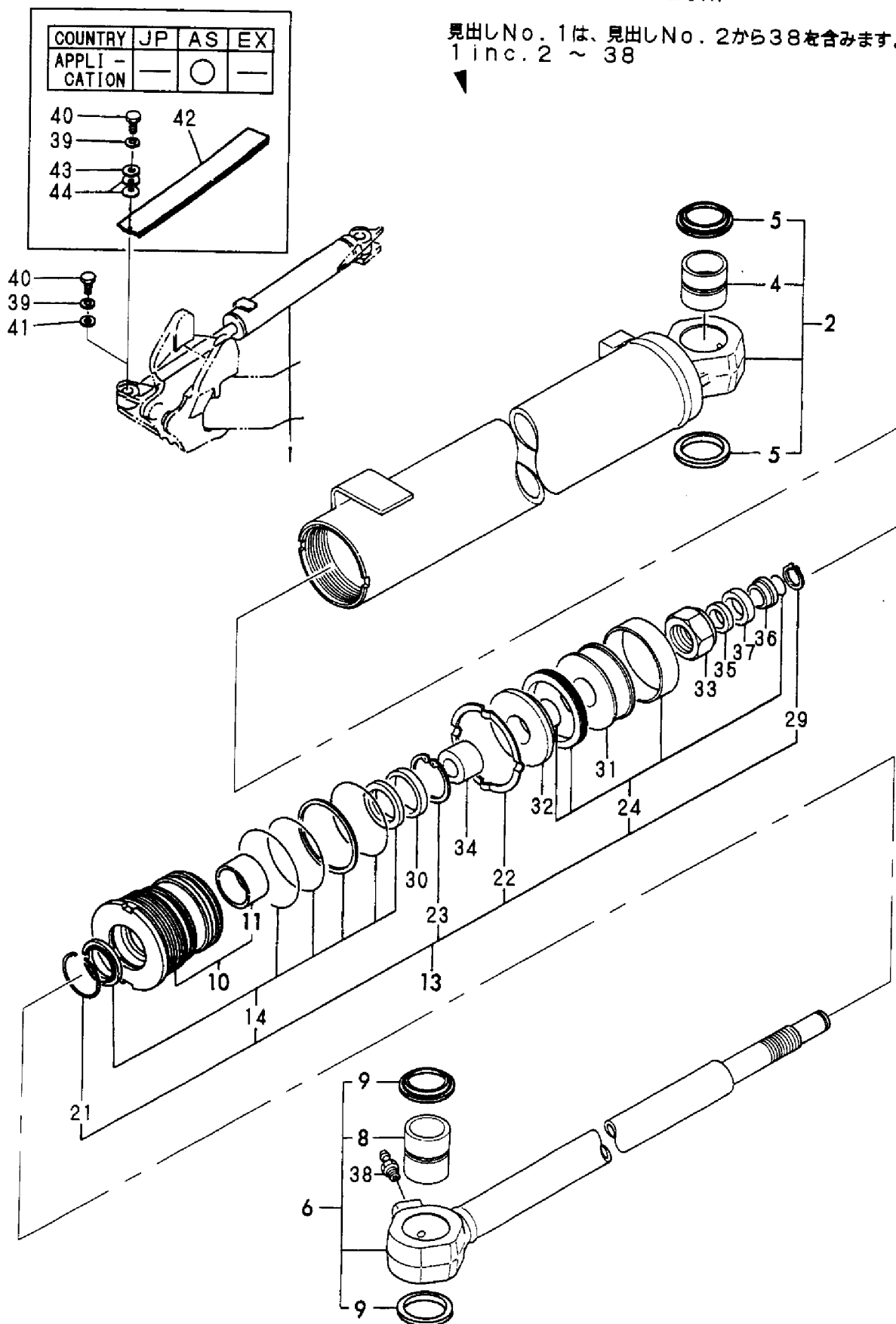
Fig. 60 スイングシリンダ (キャビン) SWING CYLINDER (CABIN)
