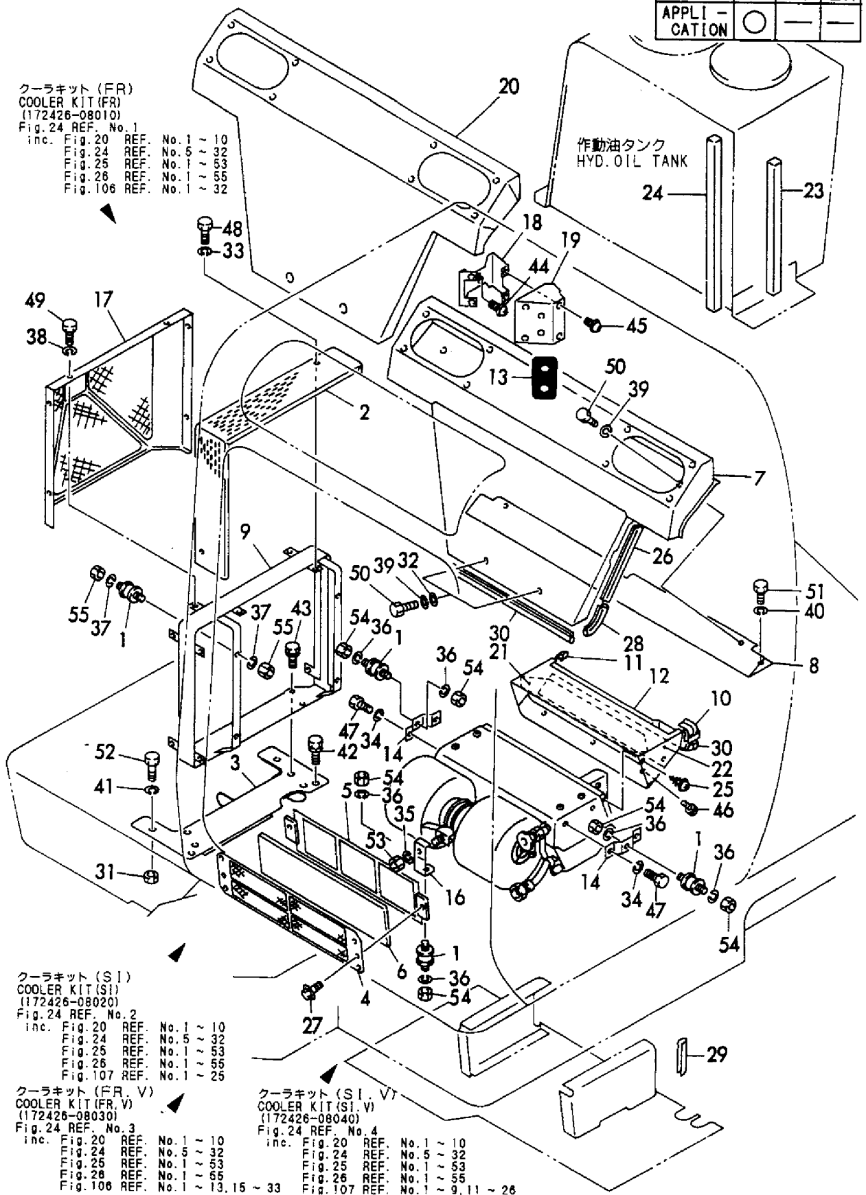
Fig. 26 カバー (クーラ仕様) COVER (COOLER SPEC.)
