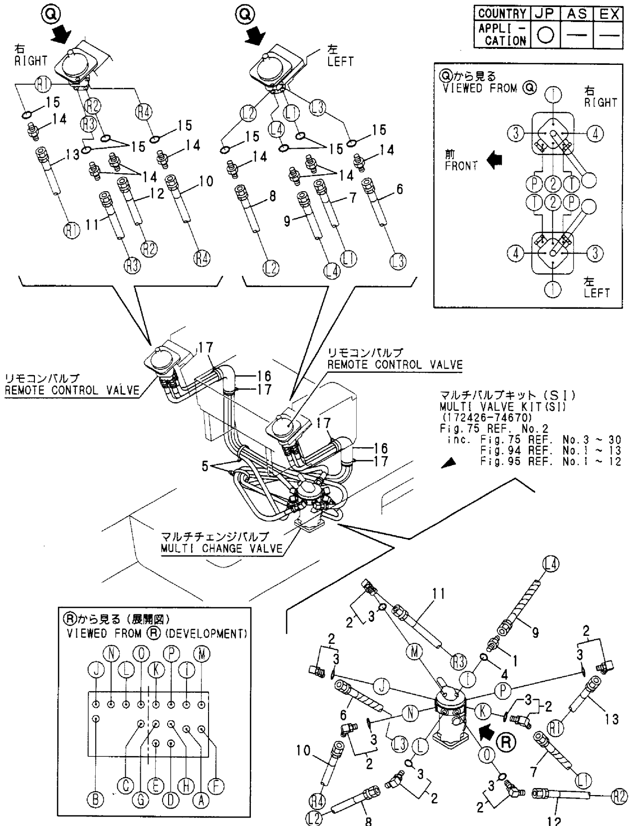
Fig. 94 コントロール配管 (リモコンバルブ~マルチバルブ/4ウェイ, サイドレバー) CONTROL PIPING (REMO.-CON. V. ~ MULTI V./4-WAY, SIDE LEVER)
