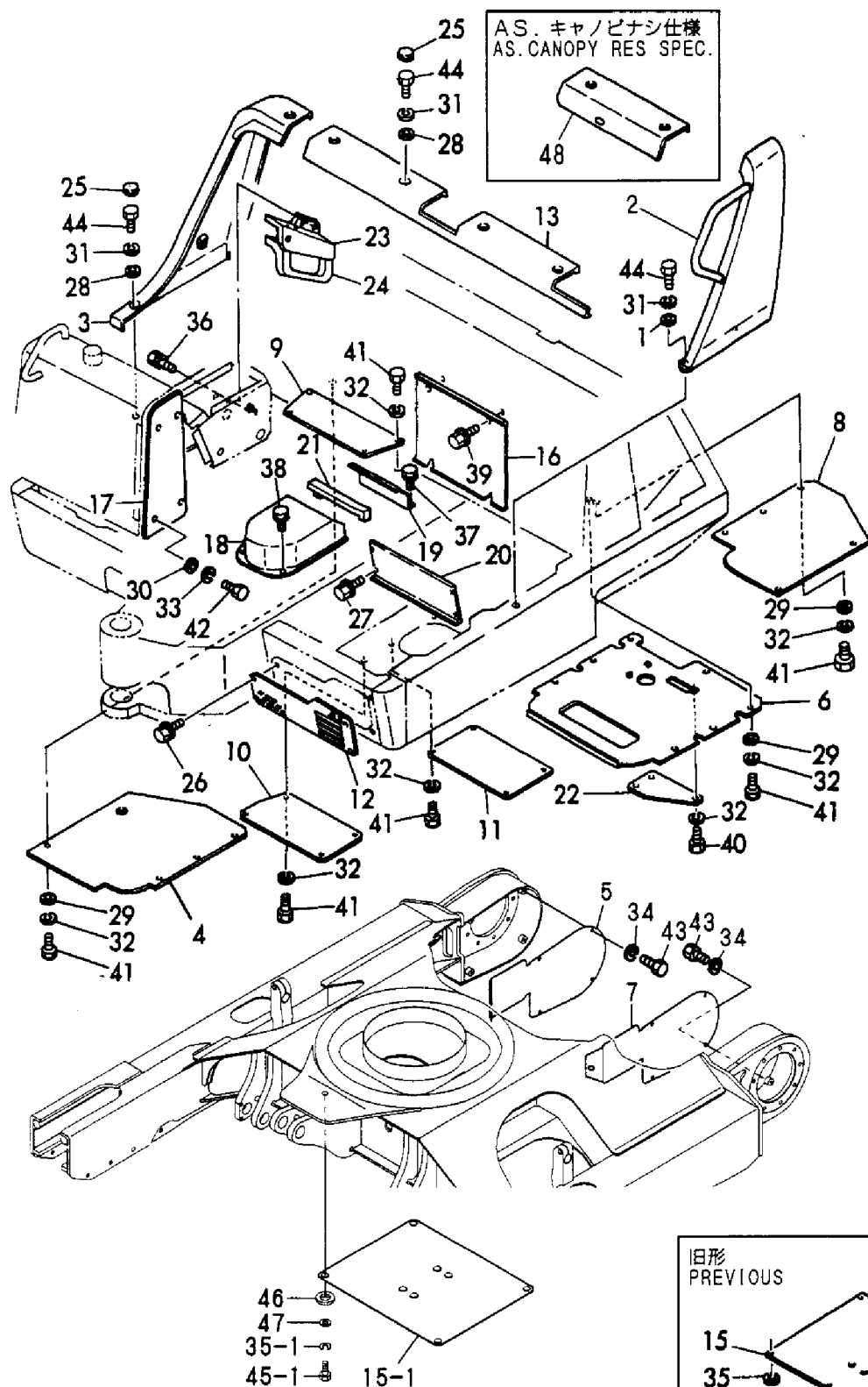
Fig. 42 フレームカバー (キャノピ) FRAME COVER (CANOPY)
