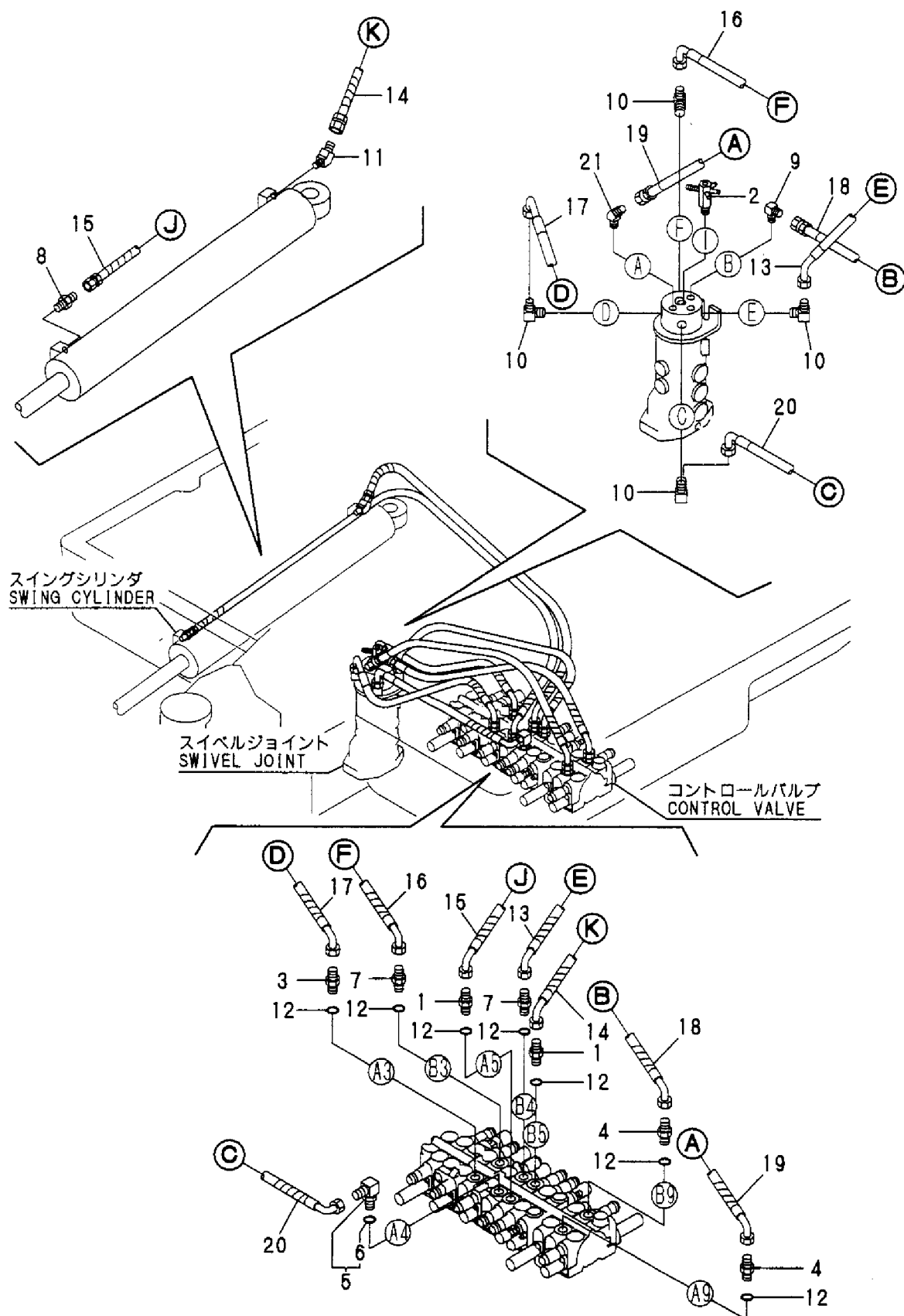
Fig. 79 油圧配管 (バルブ~スィベル、スイング) HYD. OIL PIPING (VALVE~SWIVEL, SWING)
