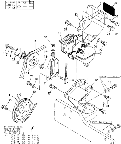
Fig. 24 コンプレッサ&Vプーリ (クーラ仕様) COMPRESSOR & V PULLEY (COOLER SPEC.) https://truckmanualshub.com/
