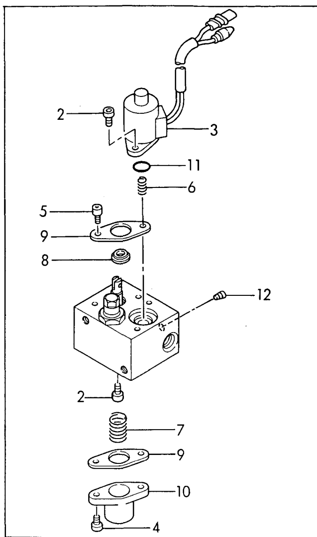
Fig. 47 ローハイバルブ ROW-HIGH VALVE https://truckmanualshub.com/
