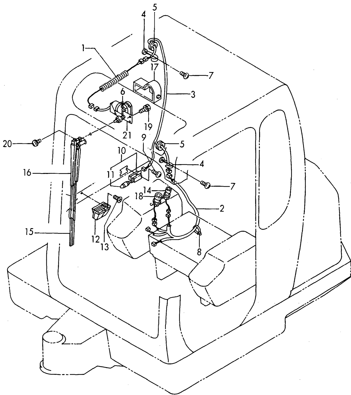
Fig. 11 電装品(キャビン専用) ELECTRIC PART(CABIN) https://truckmanualshub.com/
