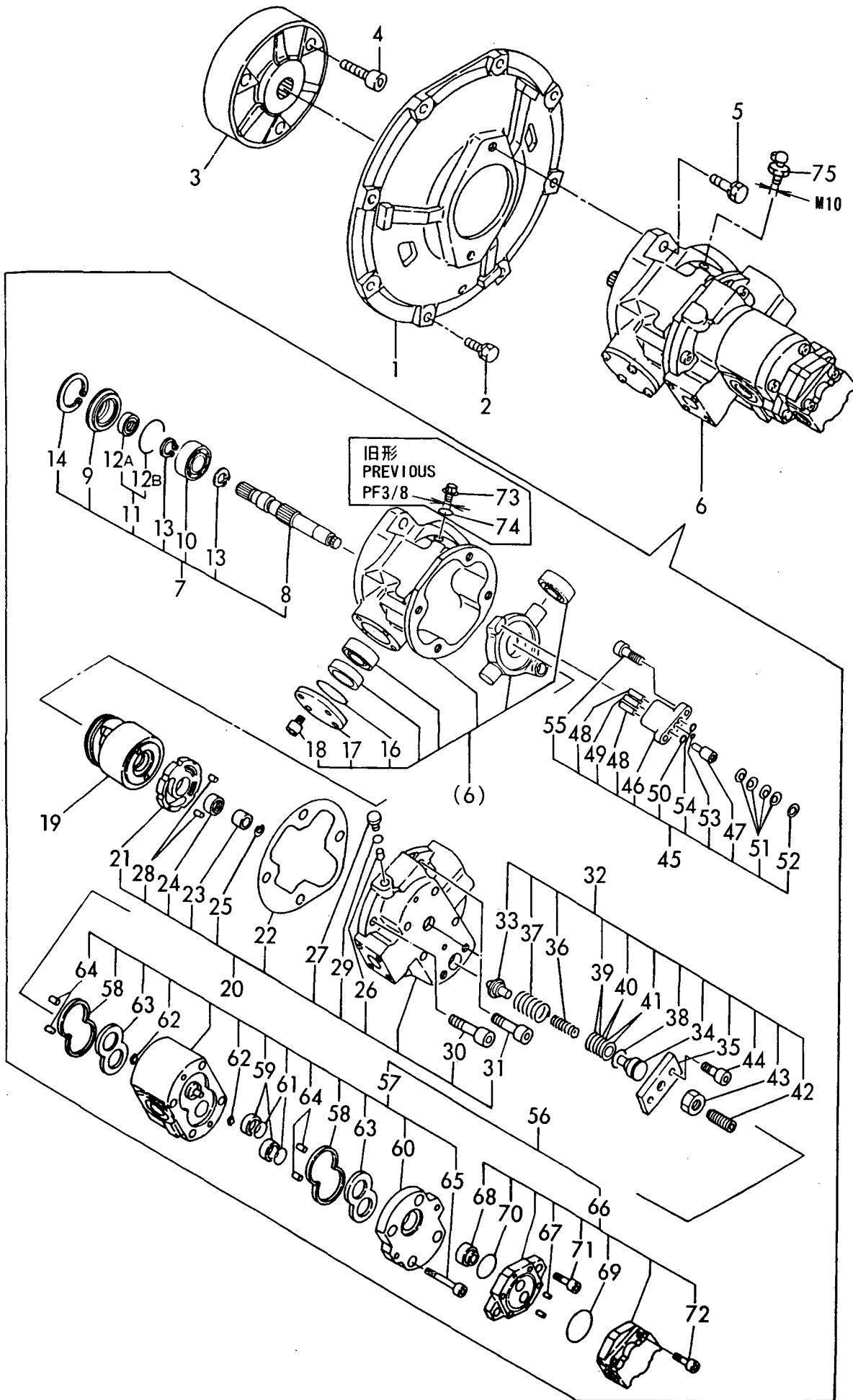
Fig. 31 ポンプ & 軸継手 HYD. OIL PUMP & JOINT http://trkmanualshub.com/
