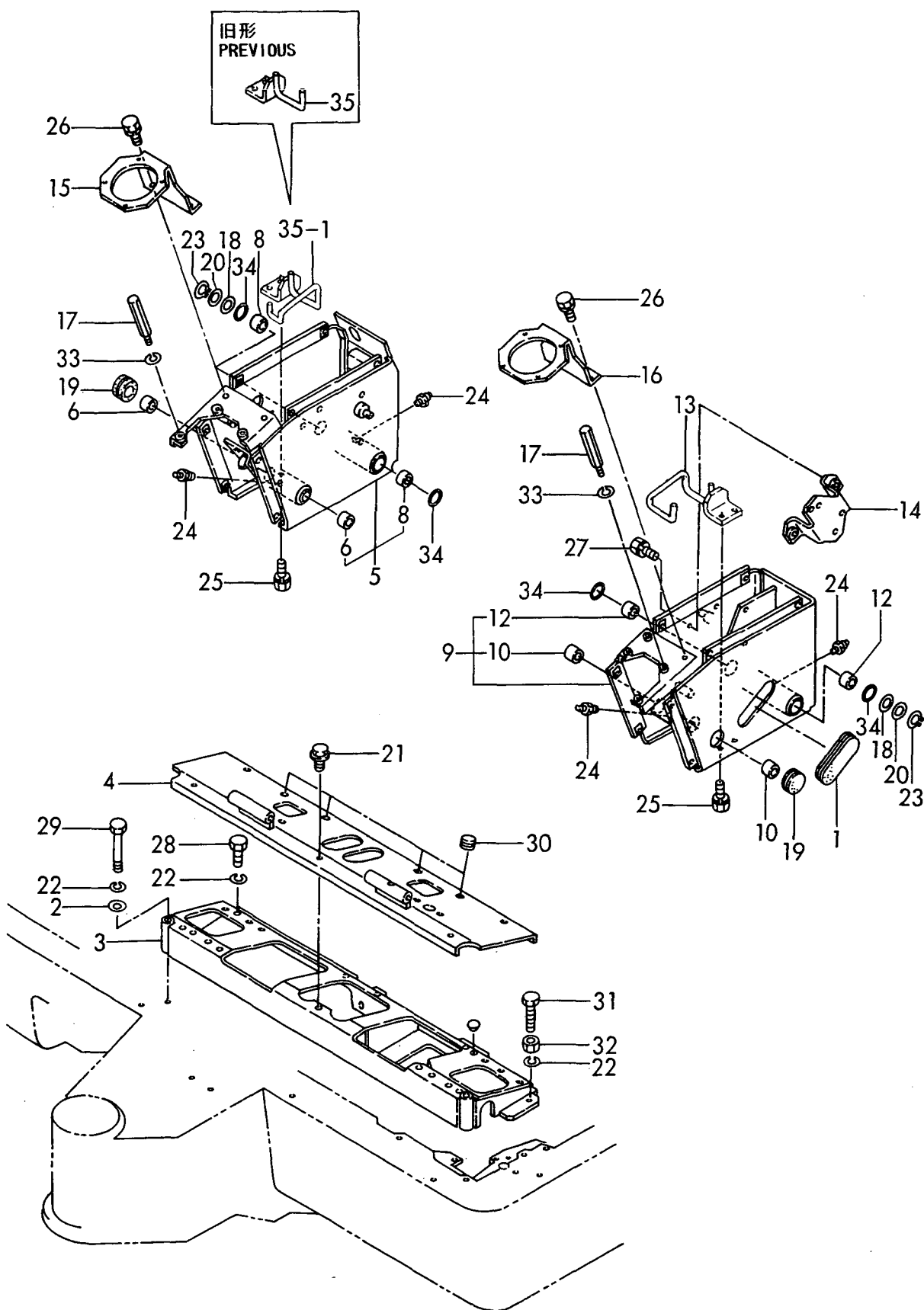
Fig. 16 操縦装置(バー & スタンド) https://truckmanualshub.com/ CONTROL EQUIPMENT (LEVER & STAND)
