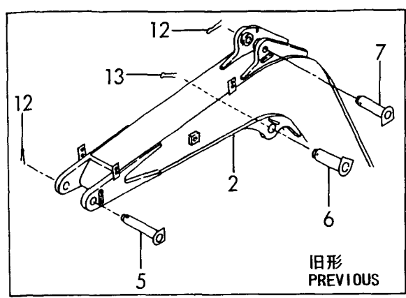
Fig. 61 ブーム & ブームブラケット BOOM & BOOM BRACKET https://truckmanualshub.com/
