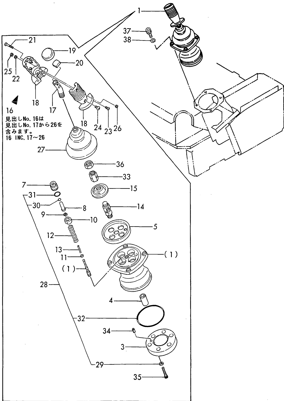
Fig. 45 リモコンバルブ(L) REMOTE CONTROL VALVE(L) https://truckmanualshub.com/
