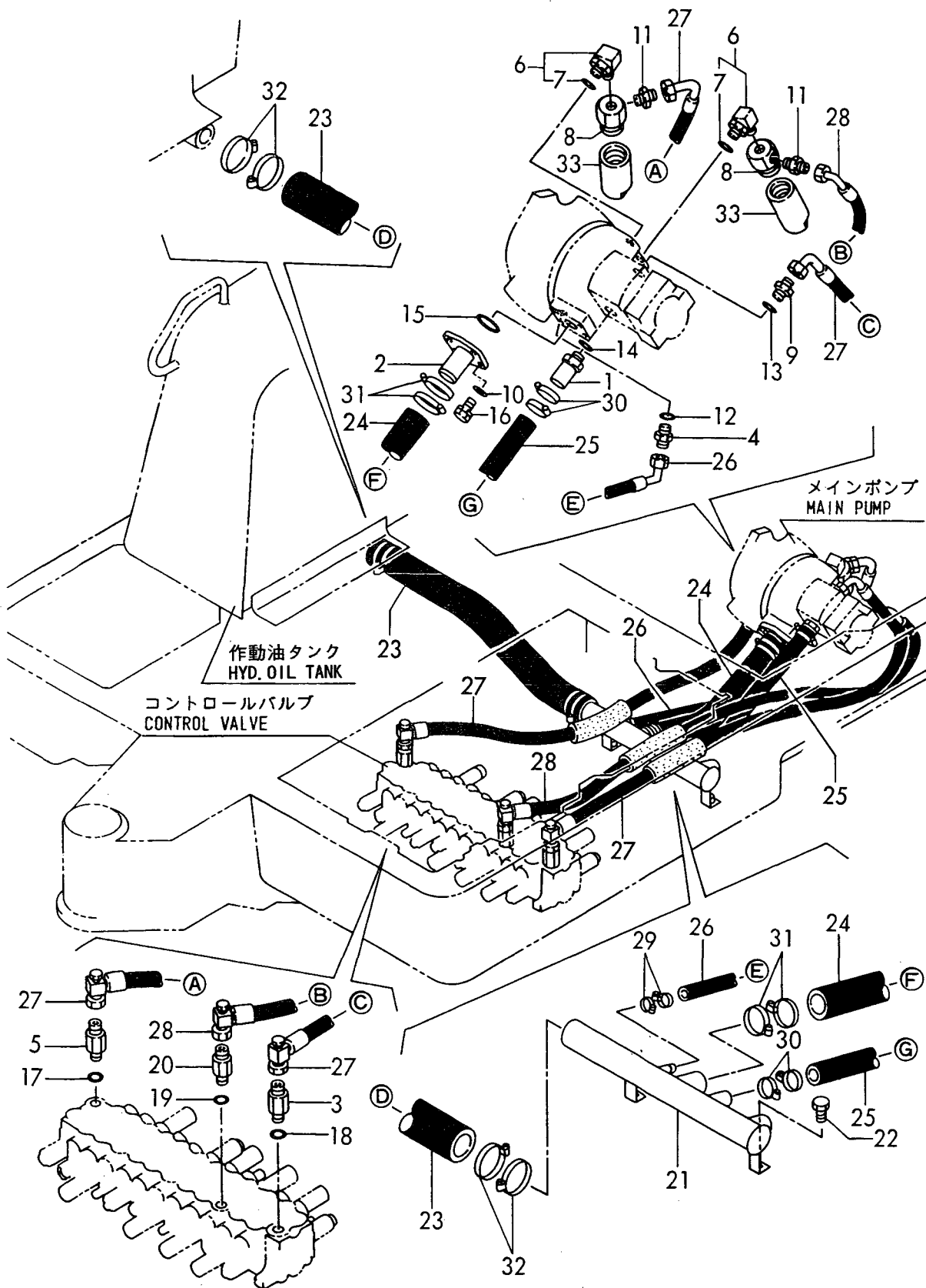
50 油圧配管(タンク〜ポンプ〜バルブ) Fig. 50 HYD. OIL PIPING(TANK~PUMP~VALVE)
