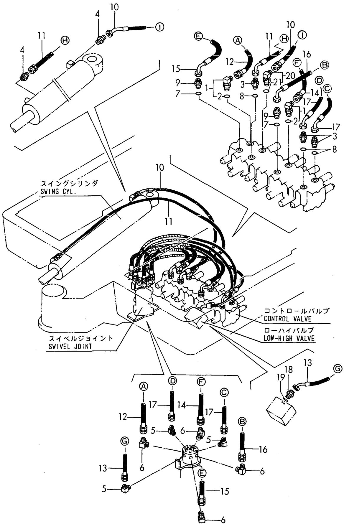
Fig. 52 油圧配管(バルブ～スィベル, スイグ) HYD. OIL PIPING (VALVE ~ SWIVEL, SWING)
