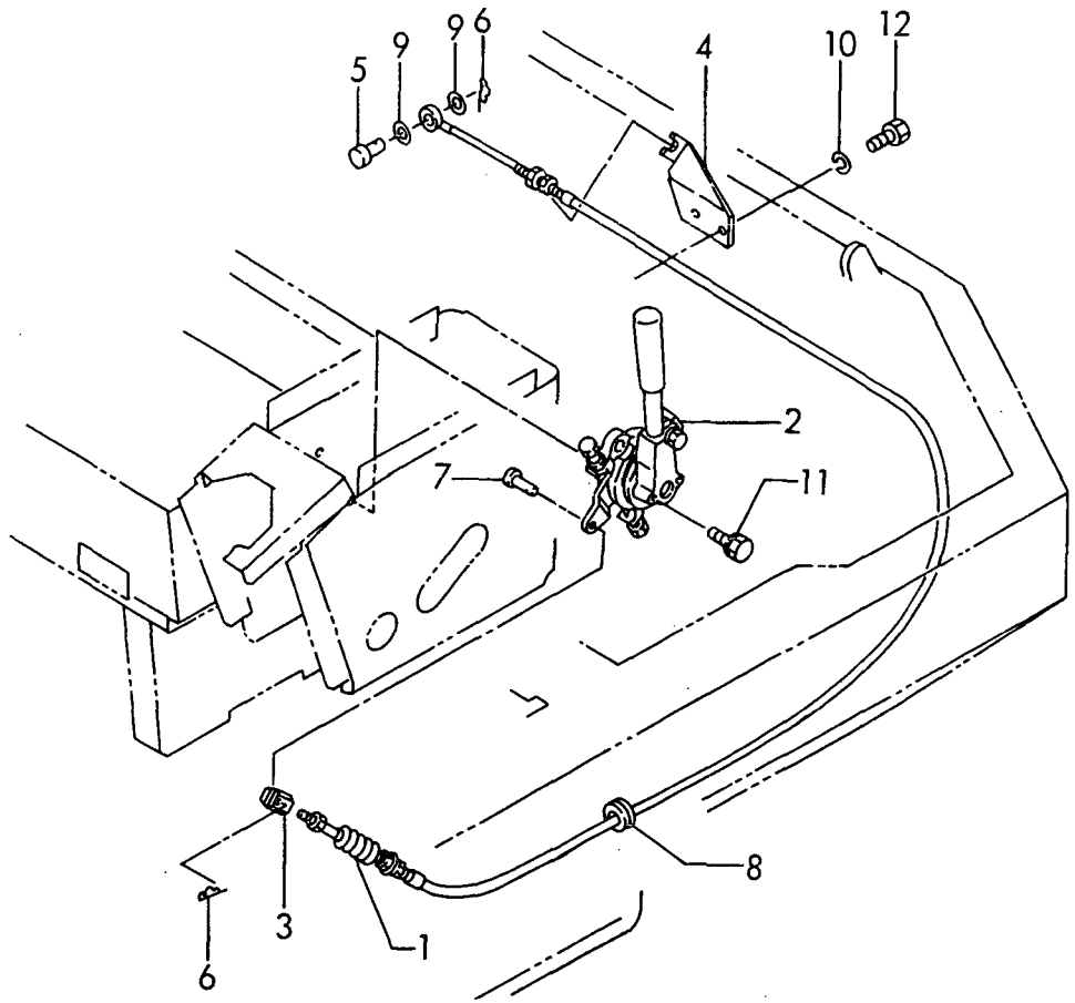
Fig. 5 アクセル ACCELERATOR https://truckmanualshub.com/
