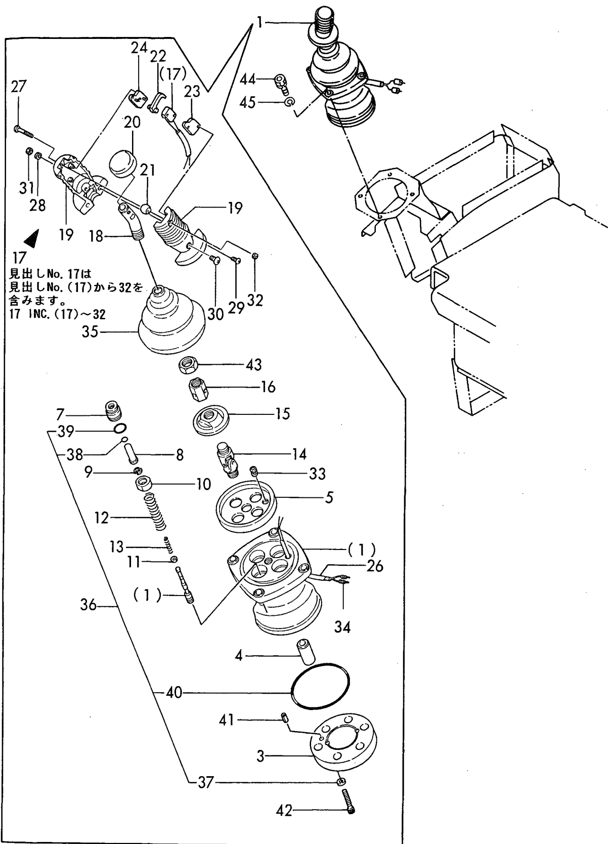
Fig. 46 リモコンバルブ(R) REMOTE CONTROL VALVE(R) https://truckmanualshub.com/
