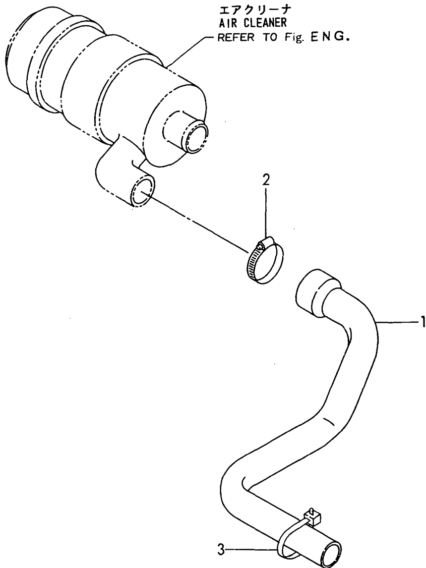
Fig. 4 エアクリーナ AIR CLEANER https://truckmanualshub.com/
