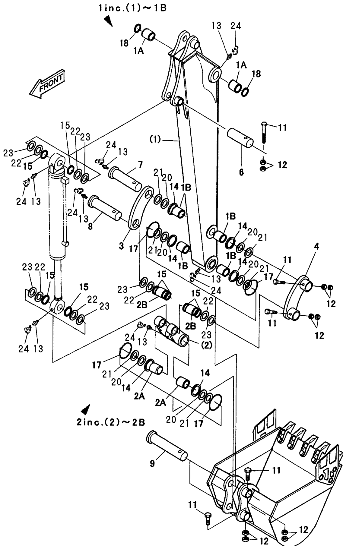
Fig. 133 ARM-1. 6M (NEW)
