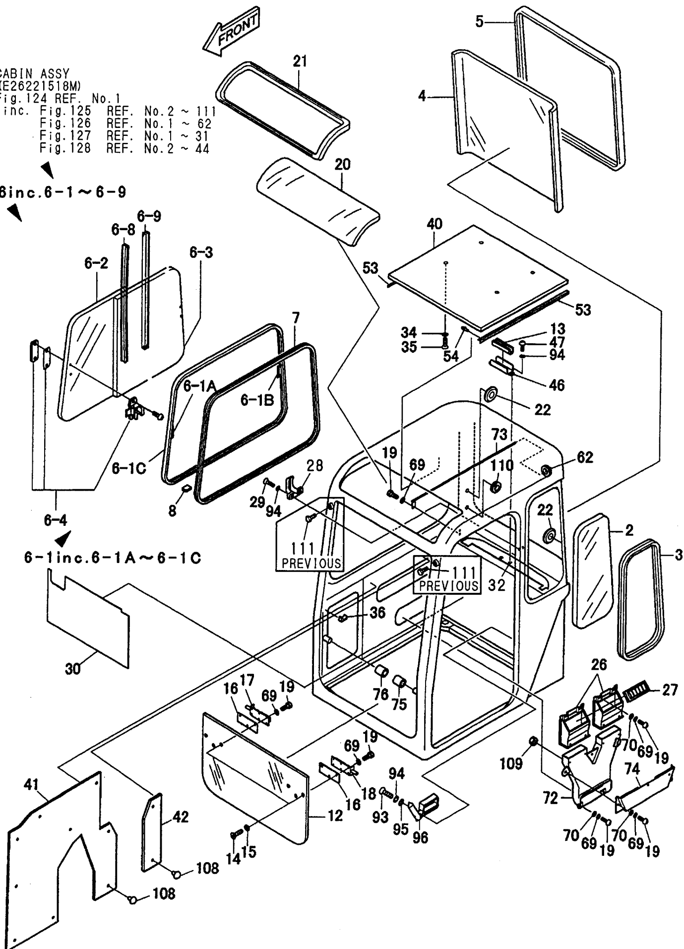
Fig. 125 CABIN (2)
