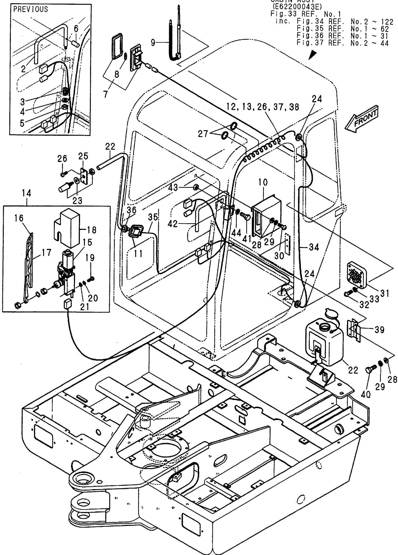
Fig. 37 CABIN (5)
