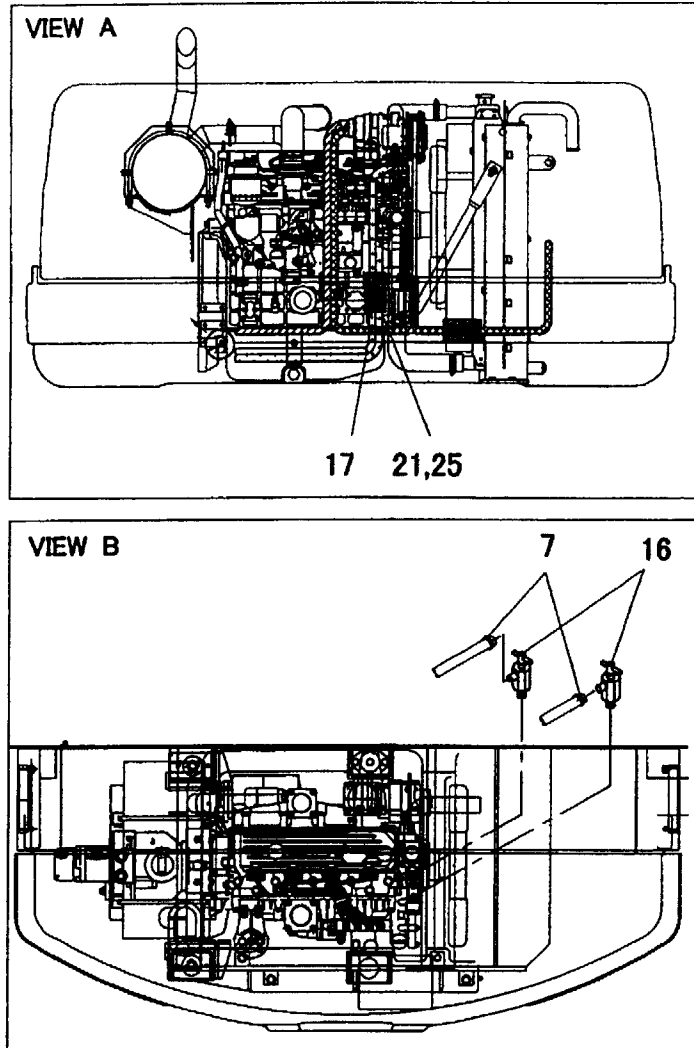
Fig. 50 HEATER
