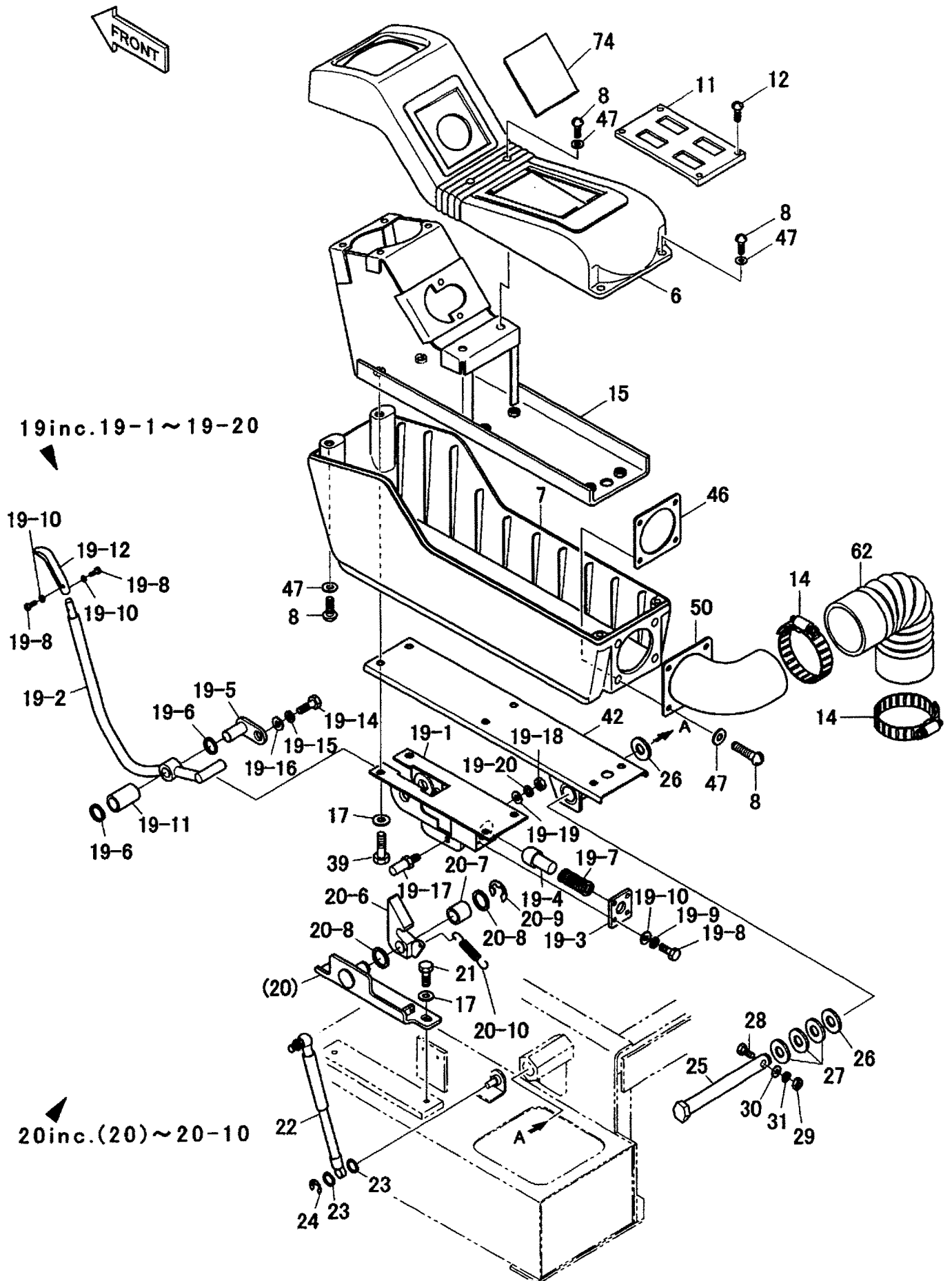
Fig. 31 CONTROL STAND-L. H.
