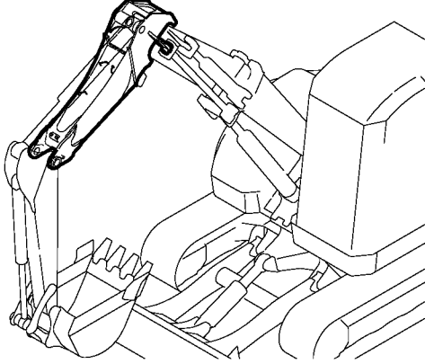
Fig. 73 BOOM-C
