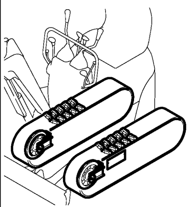
Fig. 16 クローラ、アイドル & アジャスタ CRAWLER, IDLER & ADJUST
