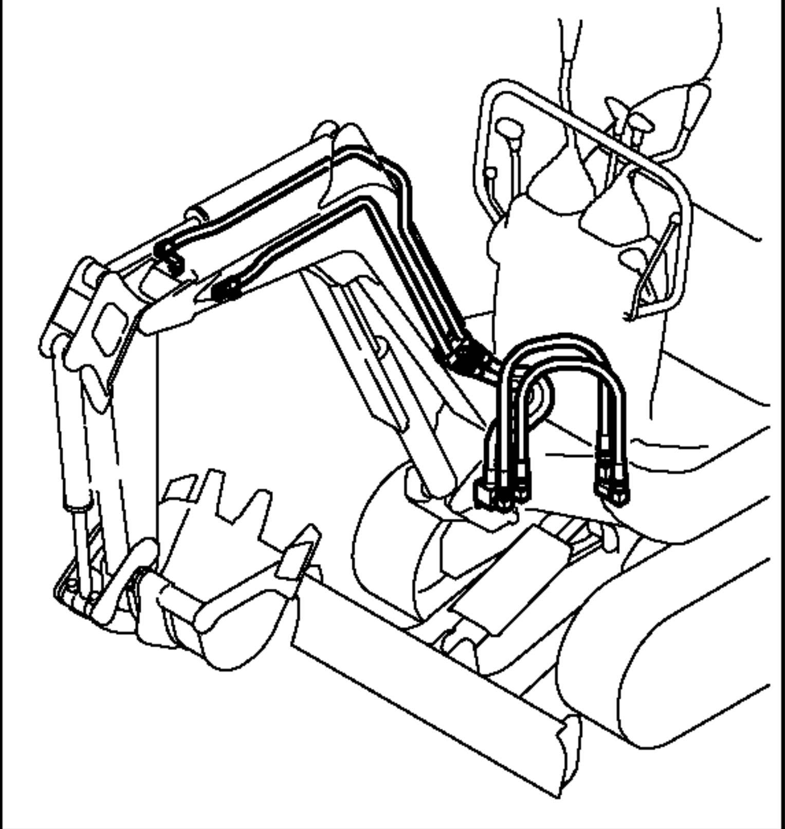
Fig. 62 油圧配管 (PT0ブームエンド) HYD. OIL PIPING (P. T. O. BOOM END)
