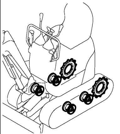
Fig. 16 クローラ、アイドル & アジャスタ CRAWLER, IDLER & ADJUST
