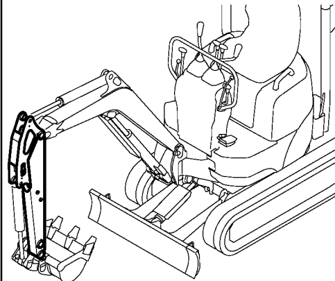
Fig. 59 ARM
