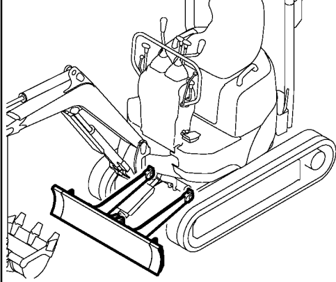
Fig. 62 BLADE
