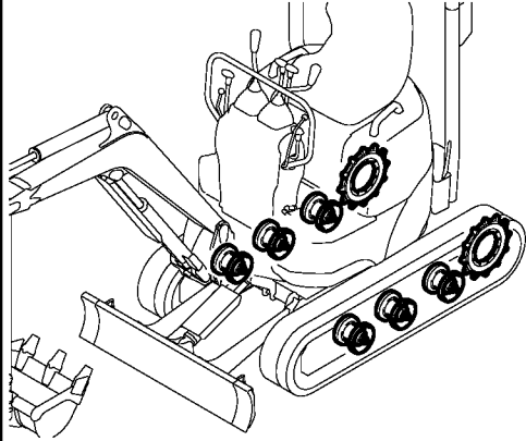
Fig. 13 SPROCKET & TRACK ROLLER
