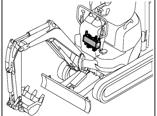
Fig. 36 CONTROL VALVE (P1 PORT & VARIABLE LEG)
