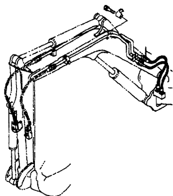
Fig. 62 コントロール配管 (ダイレクト) CONTROL PIPING (DIRECT)
