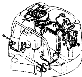
Fig. 16 ワークランプ WORK LAMP
