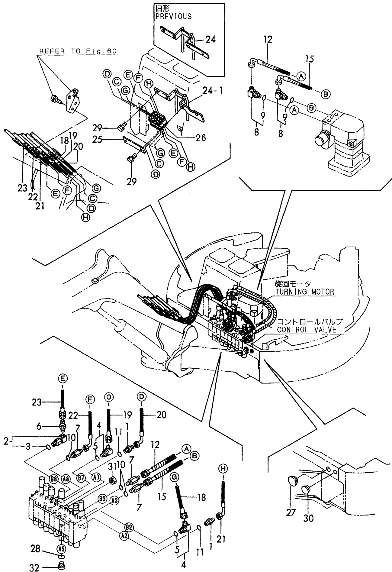
Fig. 53 油圧配管 (バルブ~モータ, ブーム) HYD. OIL PIPING (VALVE~MOTOR, BOOM)
