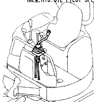
Fig. 22 操縦装置 (走行&ブレード) CONTROL EQUIPMENT (TRAVEL & BLADE)
