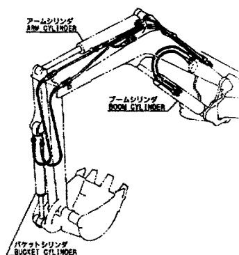
Fig. 60 油圧配管 (ブーム) HYD. OIL PIPING (BOOM)
