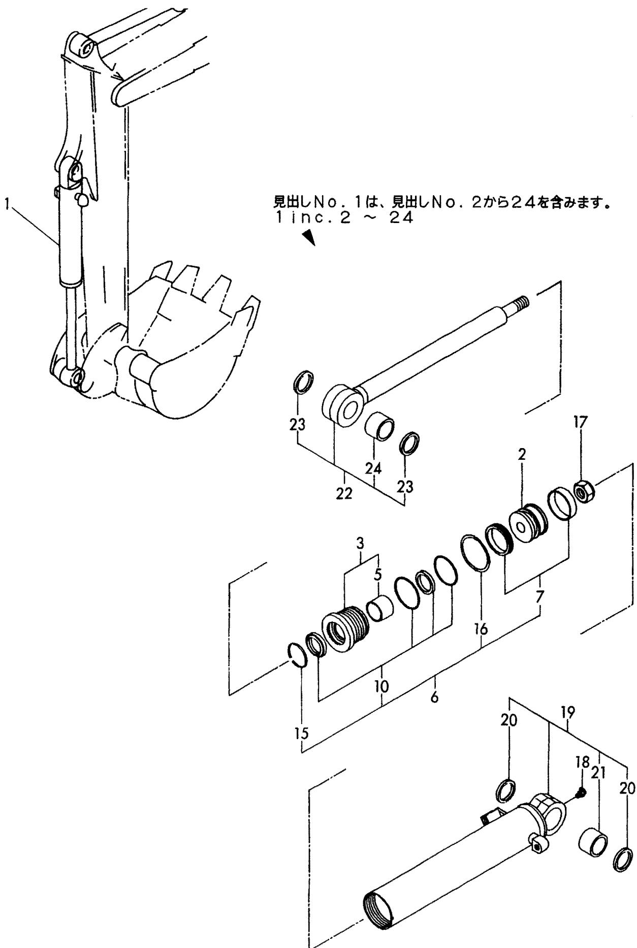
Fig. 37 バケットシリンダ BUCKET CYLINDER
