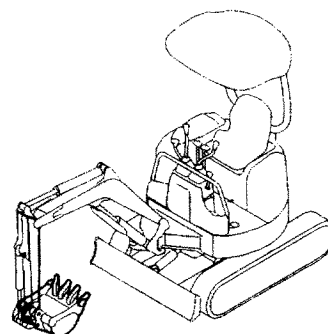
Fig. 70 バケット (400, 350, 300, 250, アタッチメント) BUCKET (400, 350, 300, 250, ATTACHMENT)
