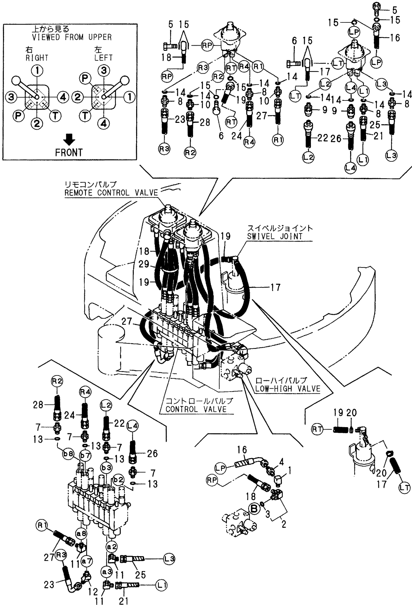
Fig. 62 コントロール配管 (ダイレクト) CONTROL PIPING (DIRECT)
