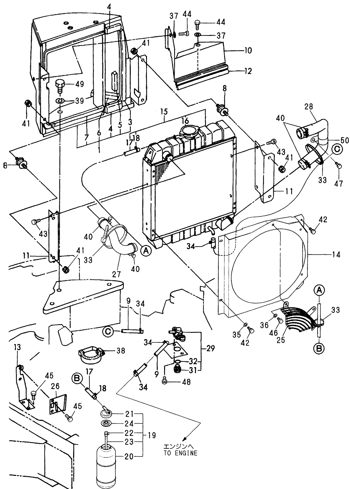
Fig. 10 ラジエータ&マウント (新形, 油圧パイロット仕様) RADIATOR & MOUNT (NEW, HYD. OIL PILOT SPEC.) M/#10501~
