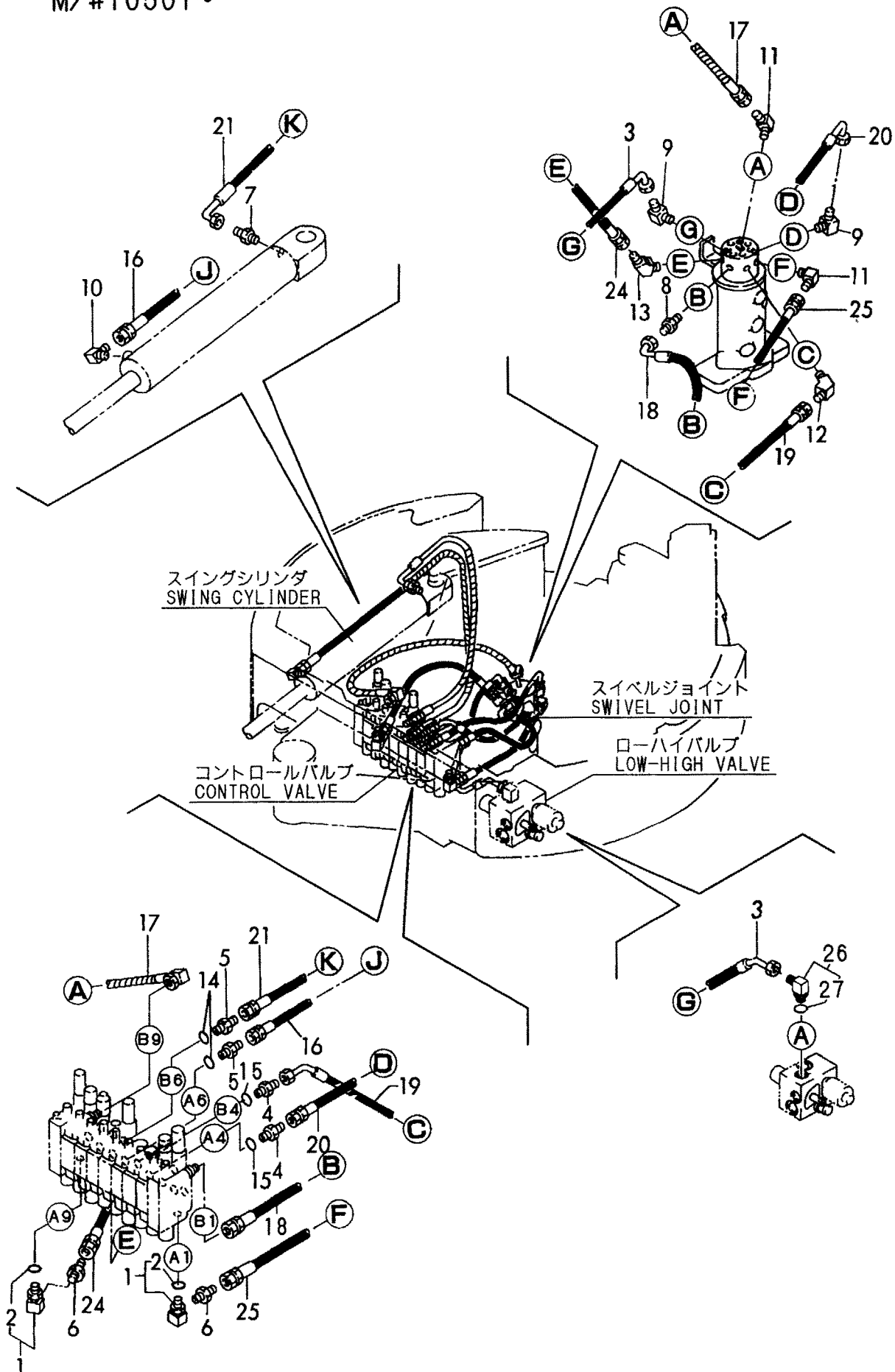
Fig. 55 油圧配管 (バルブ~スィベル, スィング) (新形, 油圧パイロット仕様) HYD. OIL PIPING (VALVE~SWIVEL, SWING) (NEW, HYD. OIL PILOT SPEC.)
