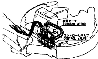
Fig. 54 油圧配管 (バルブ~スィベル スイング) (旧形) HYD. OIL PIPING (VALVE~SWIVEL , SWING) (PREVIOUS)
