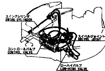
Fig. 55 油圧配管 (バルブ~スィベル, スイング) (新形, 油圧パイロット仕様) HYD. OIL PIPING (VALVE~SWIVEL, SWING) (NEW, HYD. OIL PILOT SPEC.)
