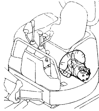
Fig. 34 油圧ポンプ&軸継手 (新形 油圧パイロット仕様) HYD. OIL PUMP & JOINT (NEW, HYD. OIL PILOT SPEC.)
