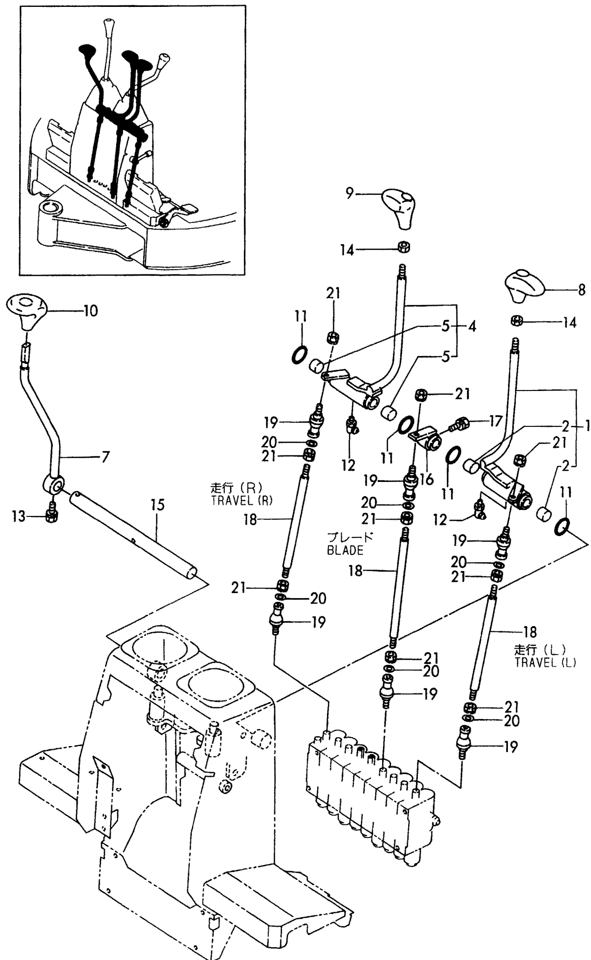
Fig. 22 操縦装置 (走行 & ブレード) CONTROL EQUIPMENT (TRAVEL & BLADE)
