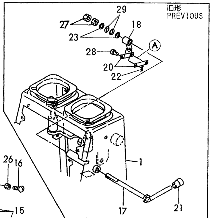
Fig. 18 操縦装置 (リンク台&レバーストッパ) (旧形) CONTROL EQUIPMENT (LINK STAND & LEVER STOPPER) (PREVIOUS) ~M/#10500
