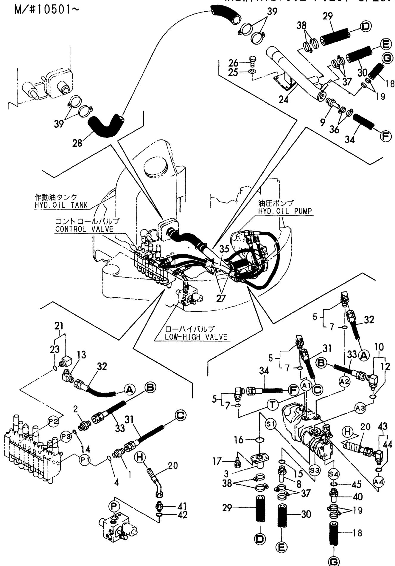
Fig. 52 油圧配管 (タンク~ポンプ~バルブ) (新形, 油圧パイロット仕様) HYD. OIL PIPING (TANK~PUMP~VALVE) (NEW, HYD. OIL PILOT SPEC.)
