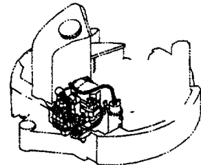
Fig. 58 油圧配管 (PTOバルブ ~ブームブラケット) HYD. OIL PIPING (P.T.O. VALVE ~BOOM BRACKET)
