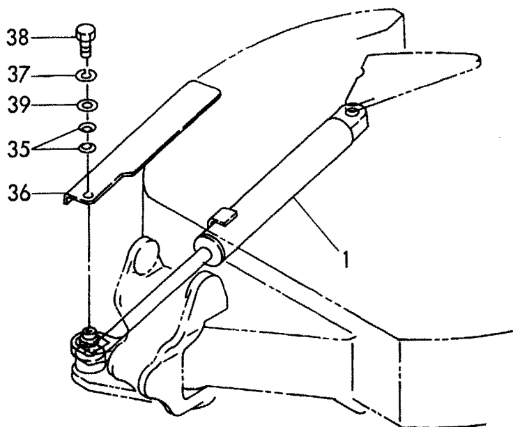
Fig. 38 スイングシリンダ SWING CYLINDER
