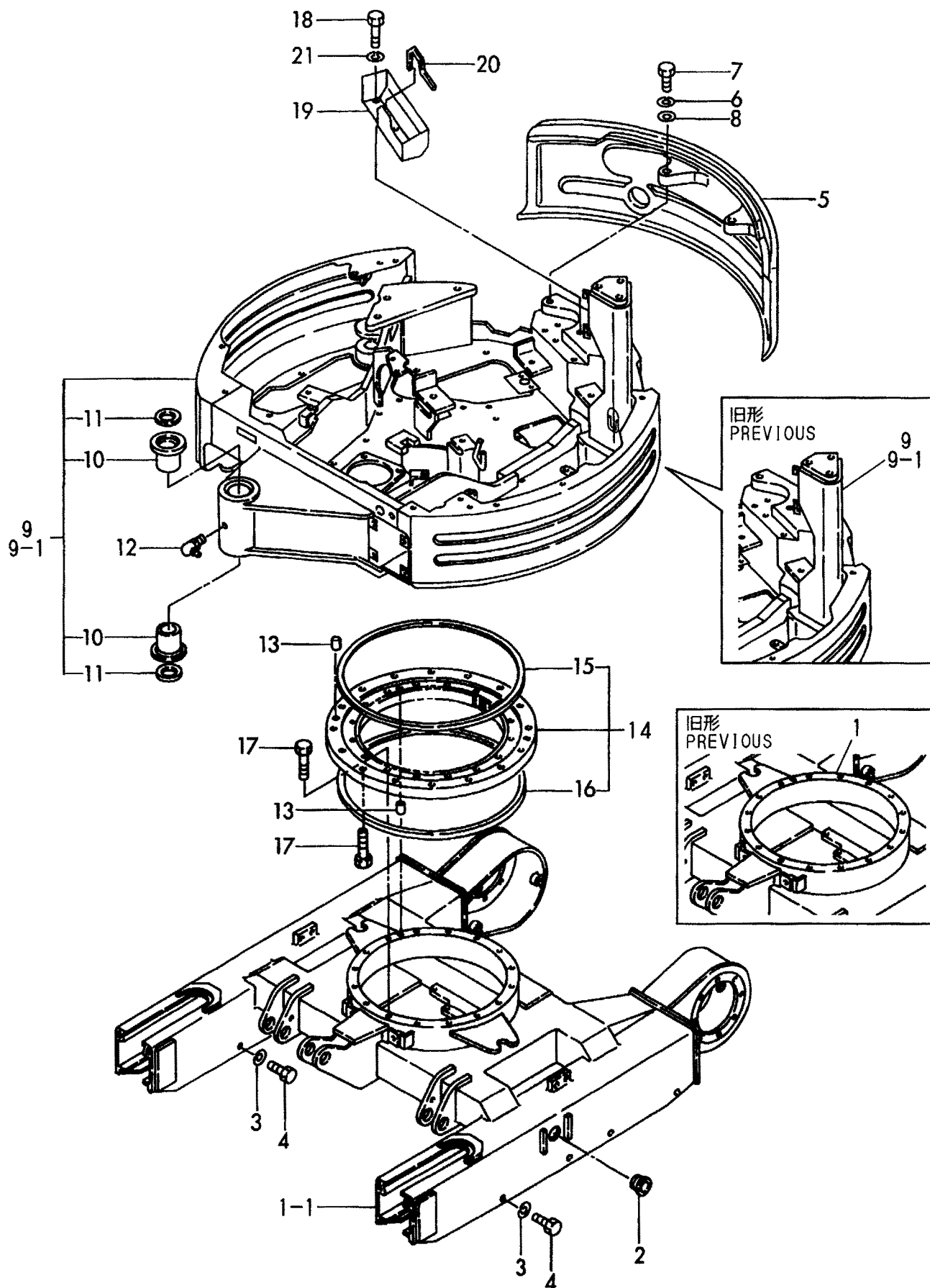
Fig. 27 フレーム&旋回ベアリング FRAME & TURNING BEARING
