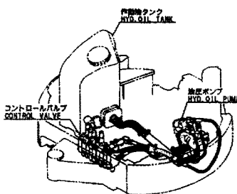
Fig. 51 油圧配管 (タンク~ポンプ ~バルブ) (旧形) HYD. OIL PIPING (TANK~PUMP~VALVE) (PREVIOUS)
