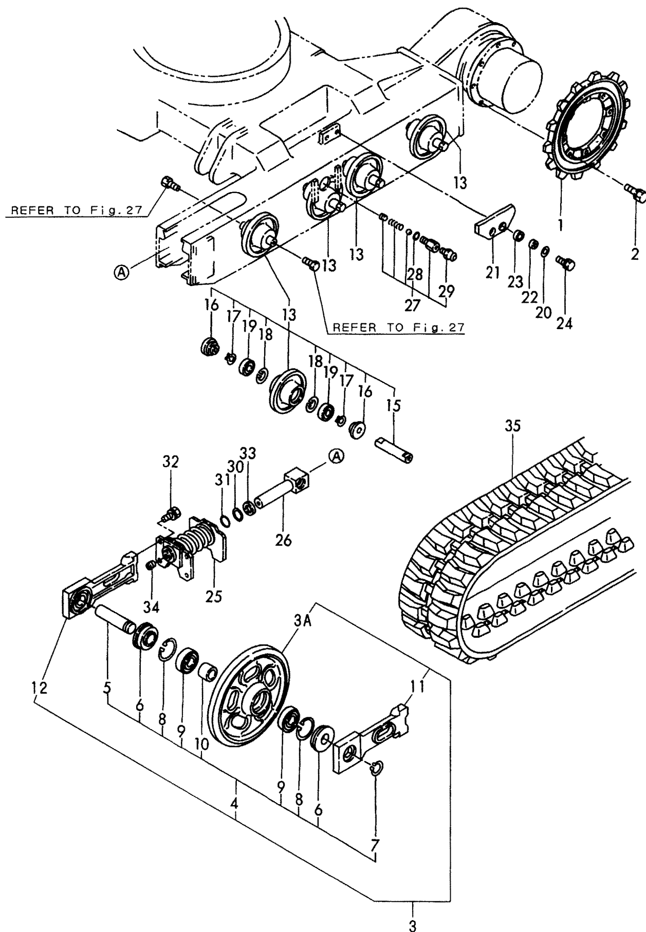
Fig. 17 クローラ、ローラ&アジャスト CRAWLER, ROLLER & ADJUST
