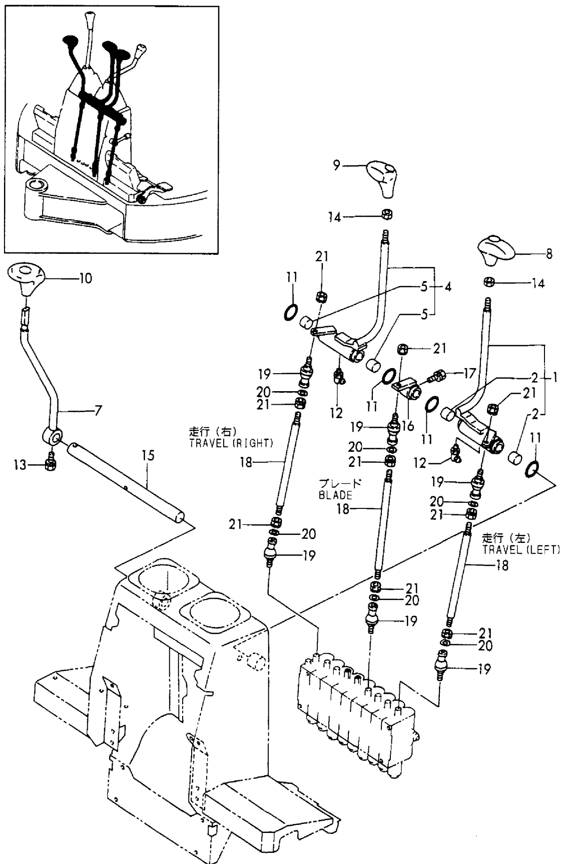
Fig. 18 操縦装置 (走行 & ブレード) CONTROL EQUIPMENT (TRAVEL & BLADE)
