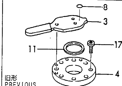
Fig. 40 ロータリバルブ (4ウェイマルチチェンジ) ROTARY VALVE (4WAY MULTI CHANGE)
