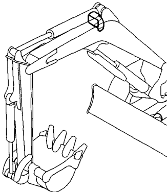
Fig. 14 ワークランプ WORK LAMP
