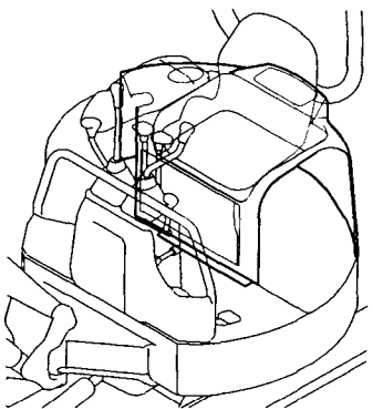
Fig. 27 キャノピ CANOPY
