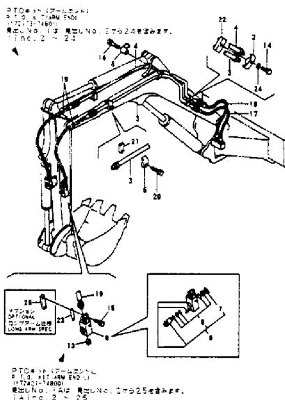
Fig. 50 油圧配管 (PTOアームエンド) HYD. OIL PIPING (P.T.O. ARM END)
