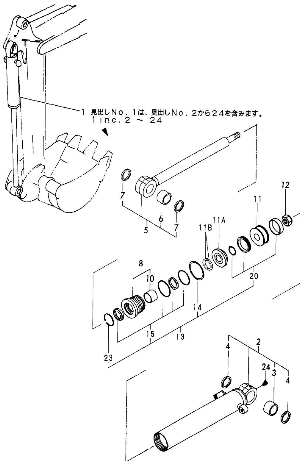
Fig. 31 バケットシリンダ BUCKET CYLINDER
