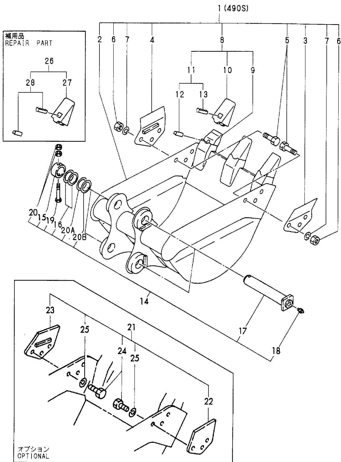
Fig. 60 バケット (490S) BUCKET (490S)
