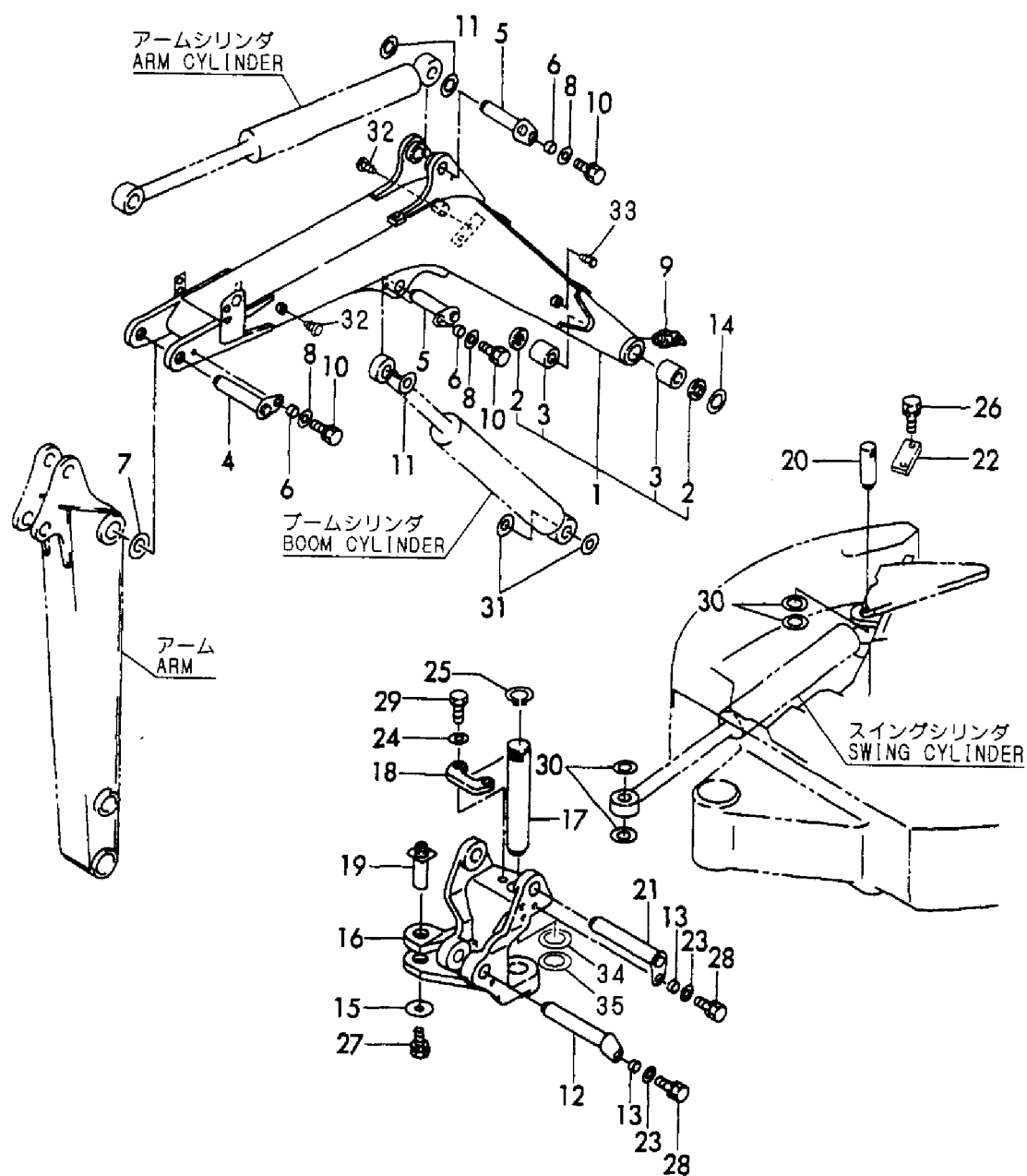
Fig. 58 ブーム&ブームブラケット BOOM & BOOM BRACKET
