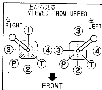
Fig. 52 コントロール配管 (ダイレクト、パターンB) CONTROL PIPING (DIRECT, PATTERN B)
