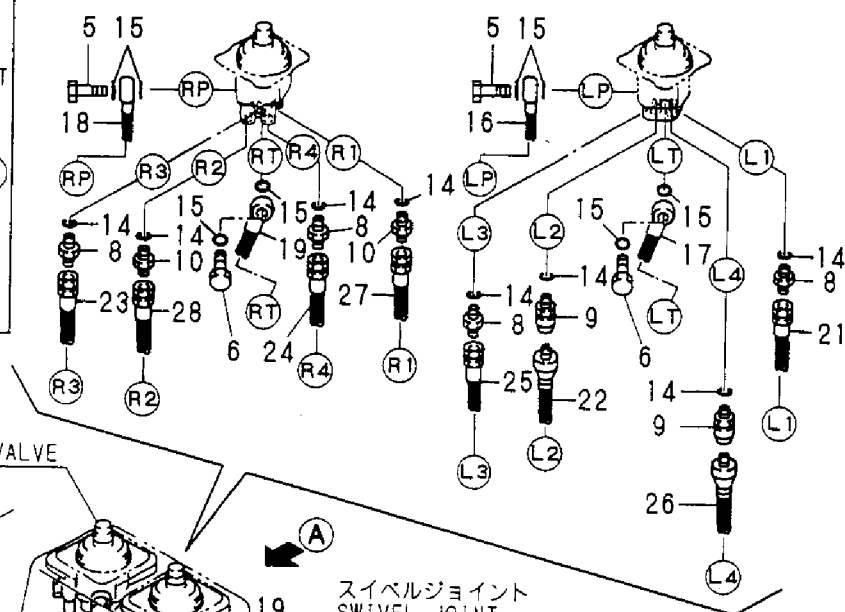
Fig. 52 コントロール配管 (ダイレクト、パターンB) CONTROL PIPING (DIRECT, PATTERN B)
