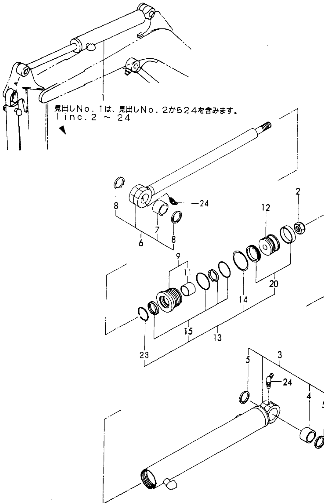
Fig. 30 アームシリンダ ARM CYLINDER
