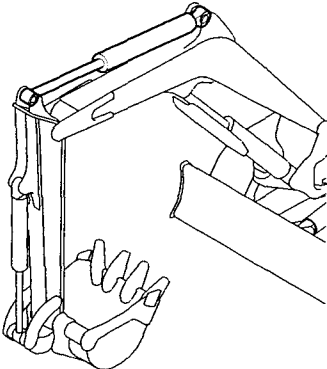
Fig. 31 バケットシリンダ BUCKET CYLINDER
