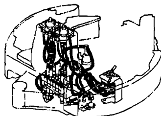
Fig. 55 コントロール配管 (リモコンバルブ ~ロータリバルブ) CONTROL PIPING (REMOT. CONTROL VALVE ~ ROTARY VALVE)
