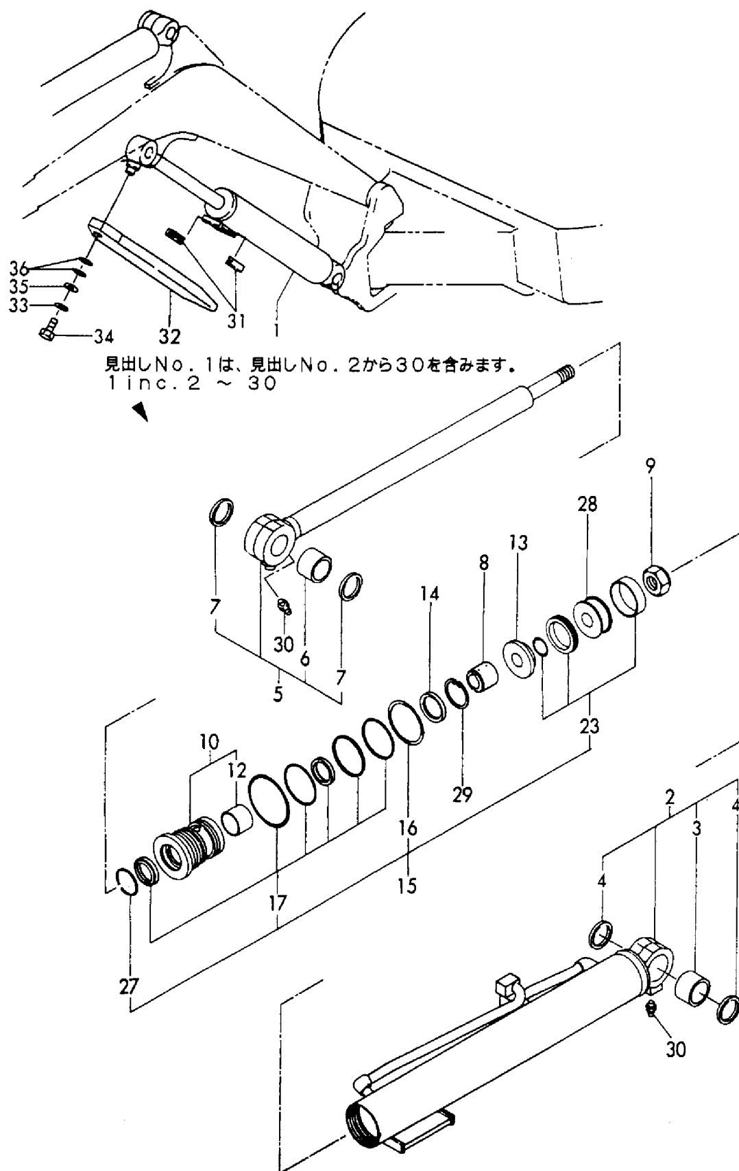
Fig. 29 ブームシリンダ BOOM CYLINDER
