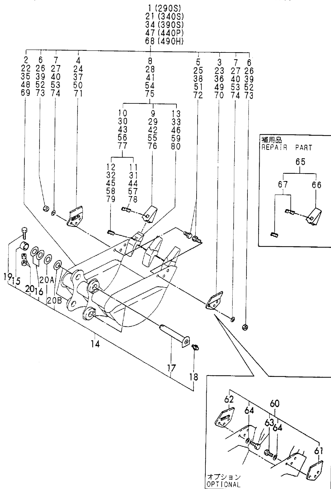
Fig. 61 バケット (Sタイプ、アタッチメント) BUCKET (S TYPE, ATTACHMENT)
