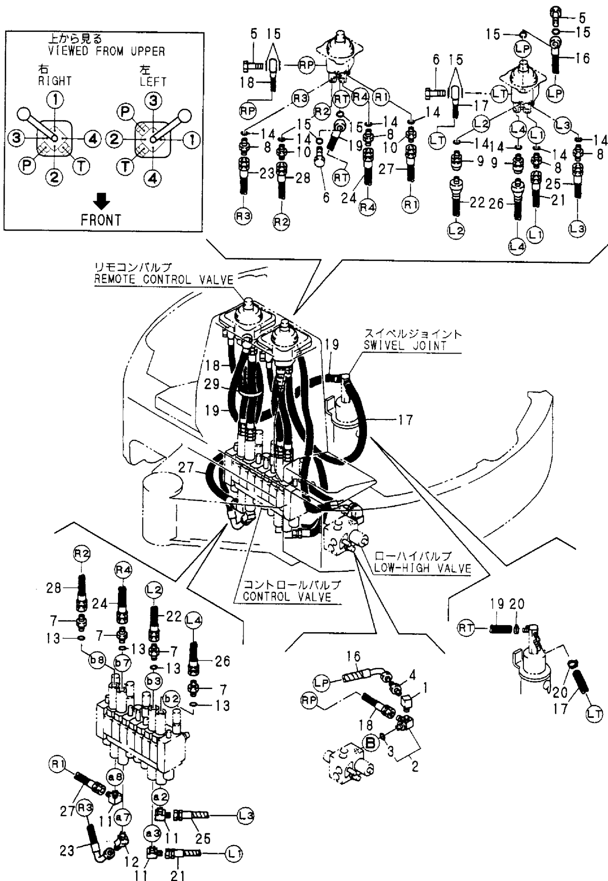
Fig. 51 コントロール配管 (ダイレクト) CONTROL PIPING (DIRECT)
