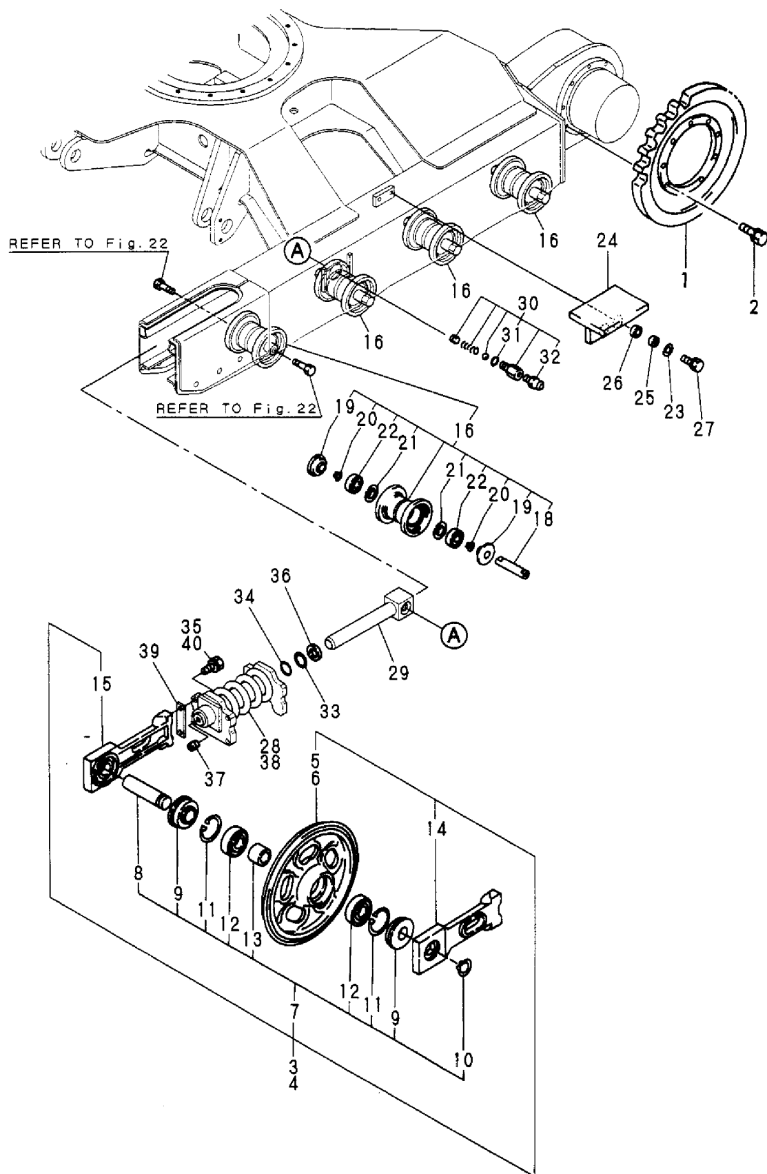
Fig. 15 ローラ&アジャスト ROLLER & ADJUST
