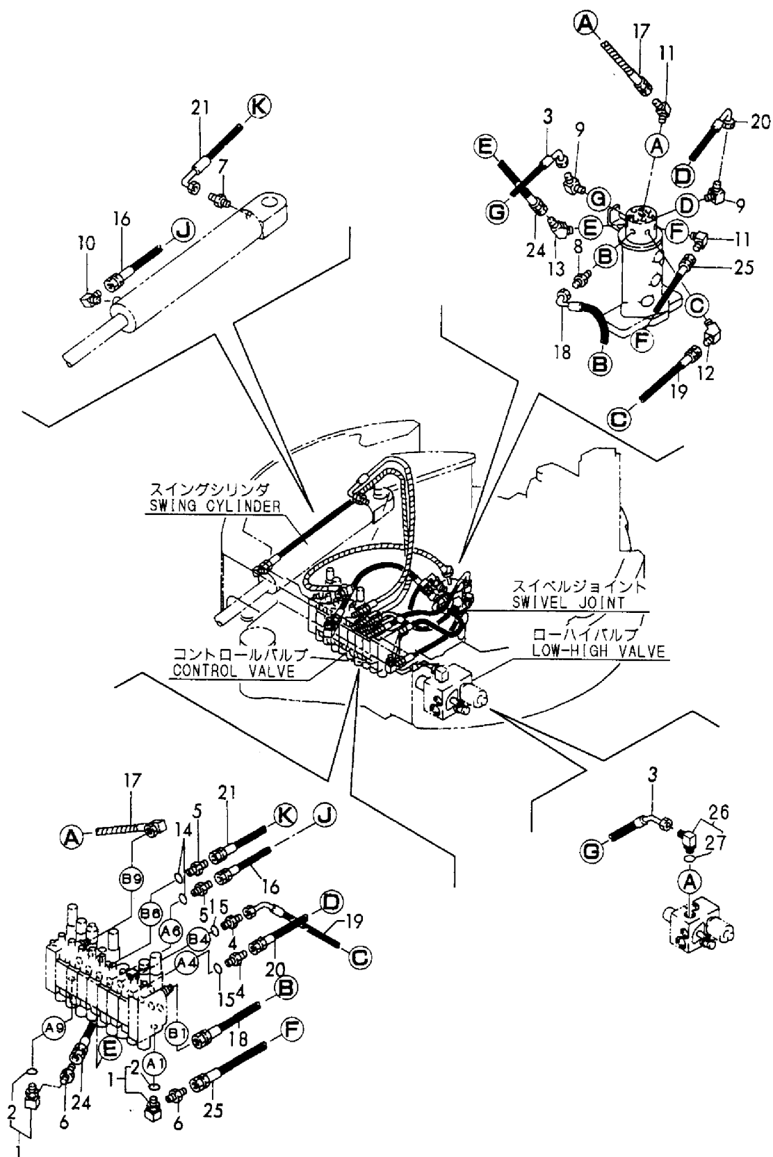
Fig. 45 油圧配管 (バルブ～スイベル、スイング) HYD. OIL PIPING (VALVE ~ SWIVEL, SWING)
