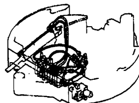
Fig. 46 油圧配管 (リターン) HYD. OIL PIPING (RETURN)
