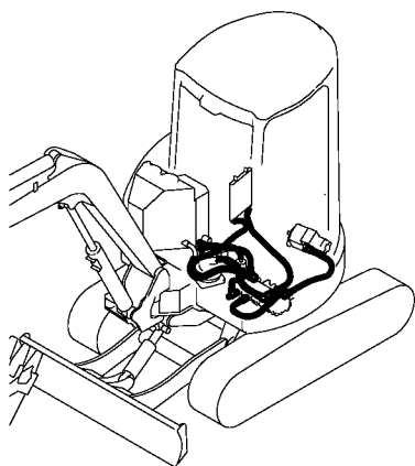
Fig. 74 油圧配管 (PTOフレームエンド) HYD. OIL PIPING (P. T. O. FRAME END)
