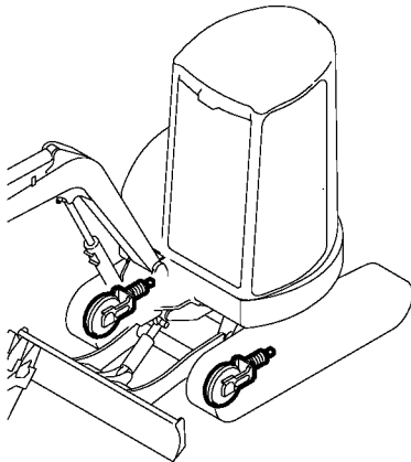
Fig. 31 クローラ CRAWLER
