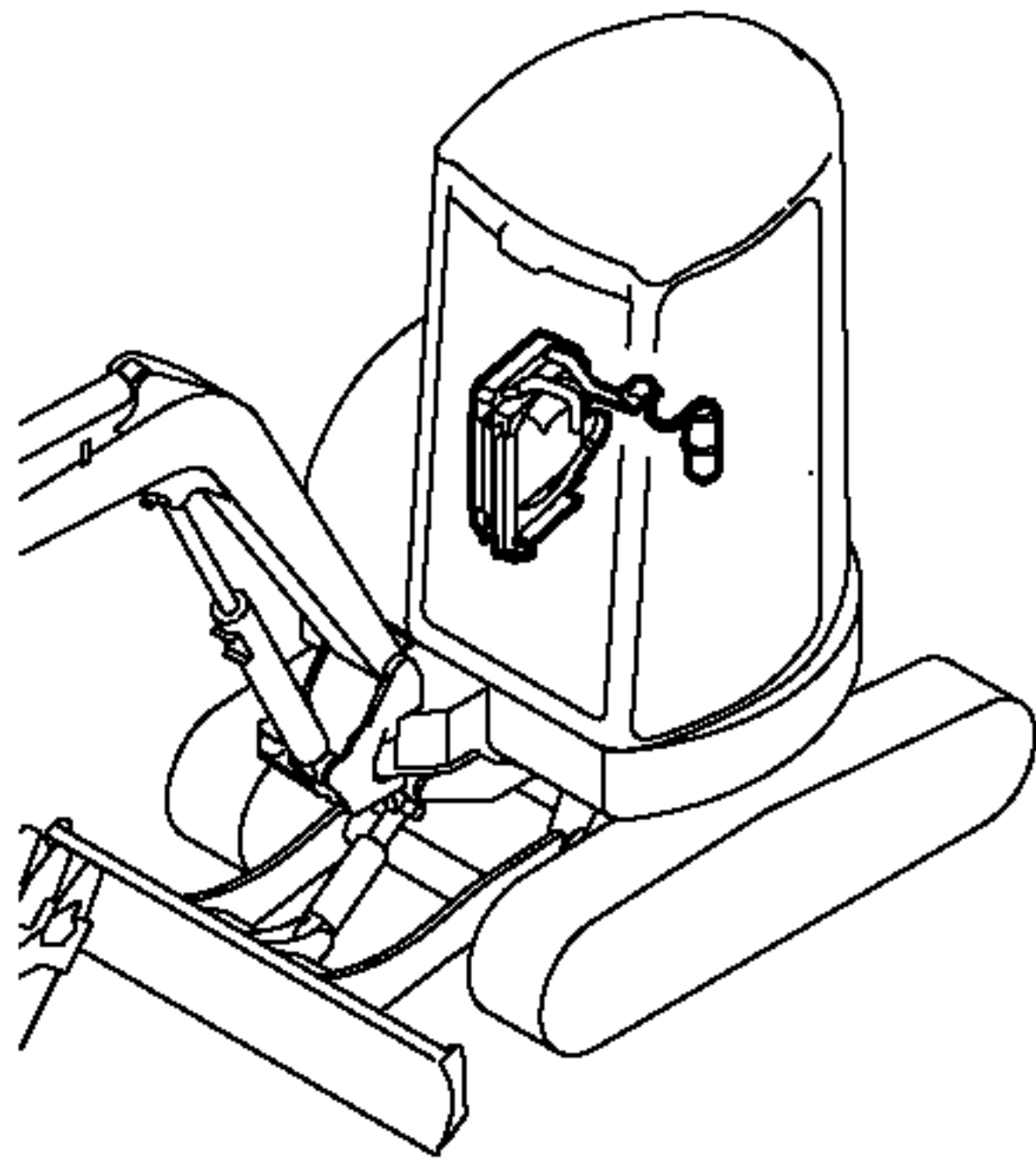
ラジエータ & マウント Fig.14 RADIATOR & MOUNT
