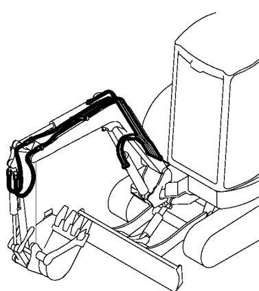
Fig. 76 油圧配管 (ブーム) HYD. OIL PIPING (BOOM)
