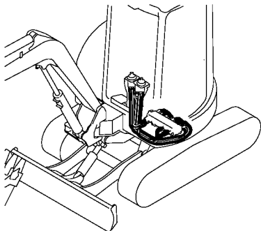
Fig. 80 コントロール配管 (リモコンバルブ～コントロールバルブ :ディレクト仕様) CONTROL PIPING (REMOTE CONTROL V. ~CONTROL V. :DIRECT SPEC.)
