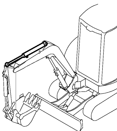
Fig. 54 バケットシリンダ BUCKET CYLINDER
