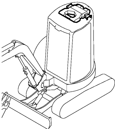
Fig. 28 クーラ (配管) COOLER (PIPING)
