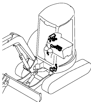
Fig. 19 電装品 (ワンタッチ・セル仕様) ELECTRIC PART (ONE TOUCH DECAL SPEC.)
