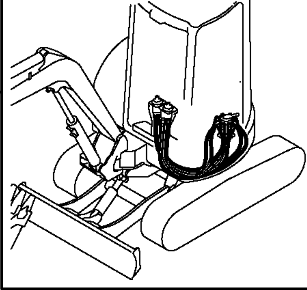
Fig.81 コントロール配管(リモコンバルブ ~ 4ウェイロータリバルブ) CONTROL PIPING (REMOTE CONTROL V. - 4-WAY ROTARY V.)
