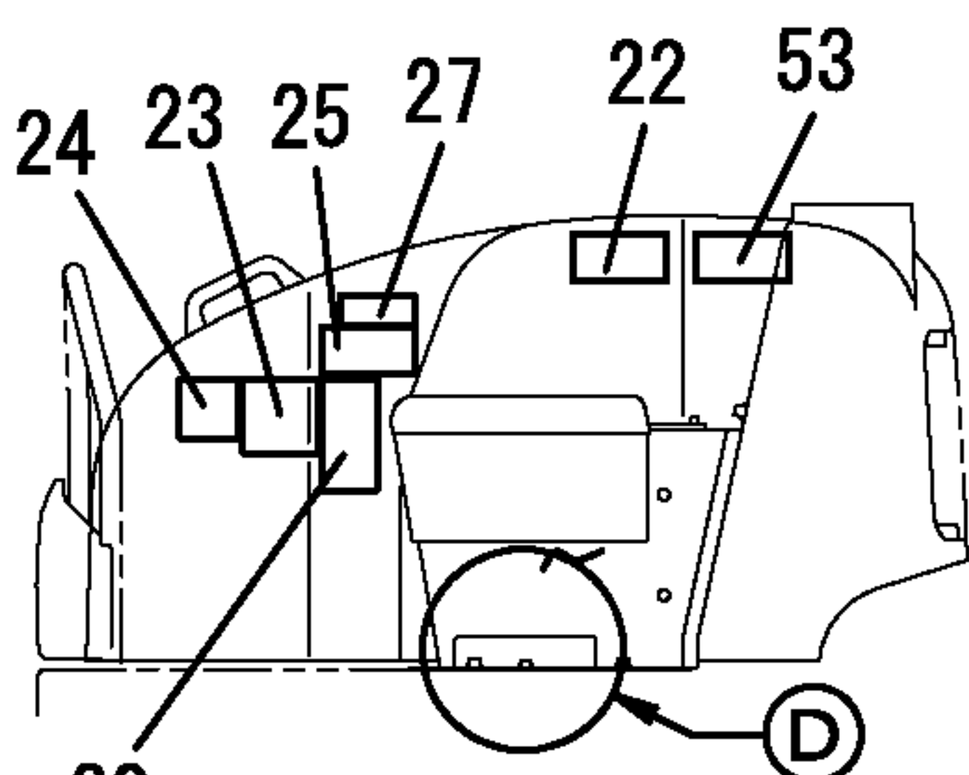
③から見る VIEWED FROM ③
