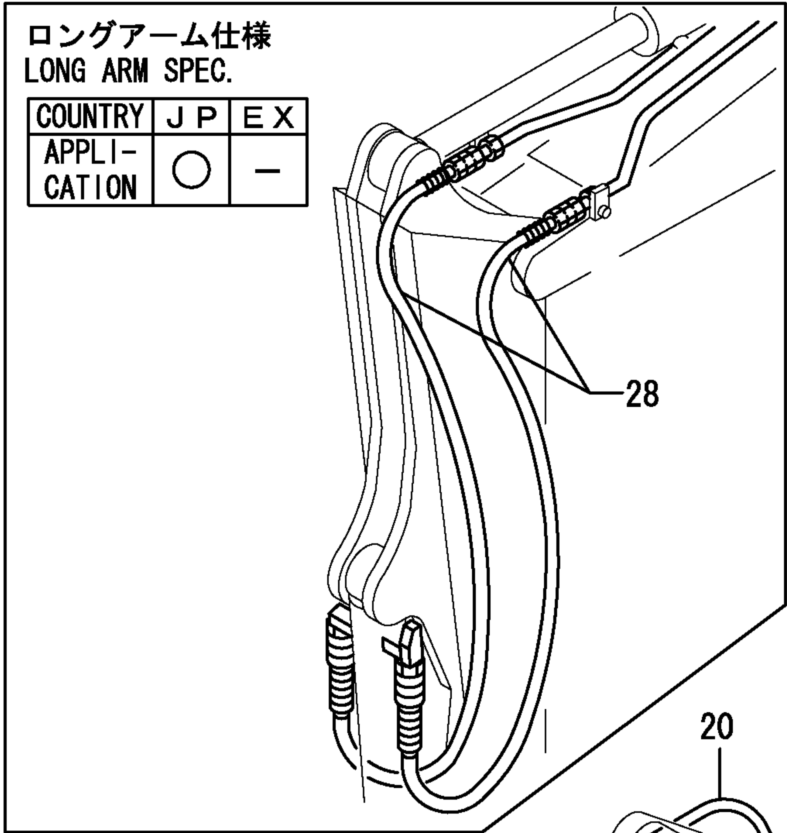
アームシリンダ ARM CYLINDER
