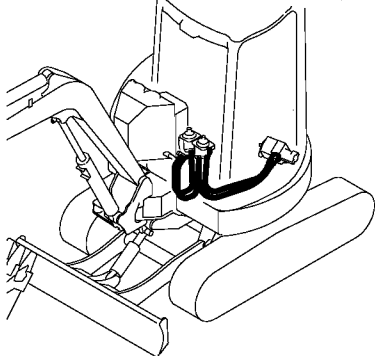
Fig. 80 コントロール配管 (リモコンバルブ～コントロールバルブ :ディレクト仕様) CONTROL PIPING (REMOTE CONTROL V. ~CONTROL V. :DIRECT SPEC.)
