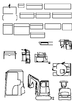
Fig. 8 安全銘板 (キャビン:EX) SAFETY LABEL (CANOPY:EX)
