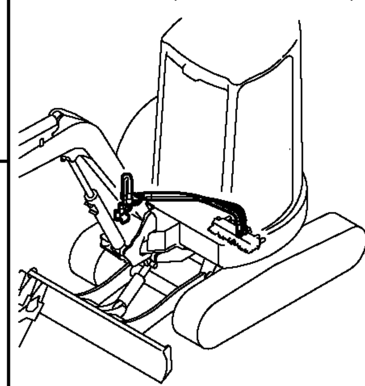
Fig.74 油圧配管 (PTOフレームエンド) HYD. OIL PIPING (P. T. O. FRAME END)
