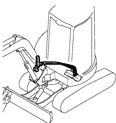
Fig. 75 油圧配管 (トラックフレーム) HYD. OIL PIPING (TRACK FRAME)
