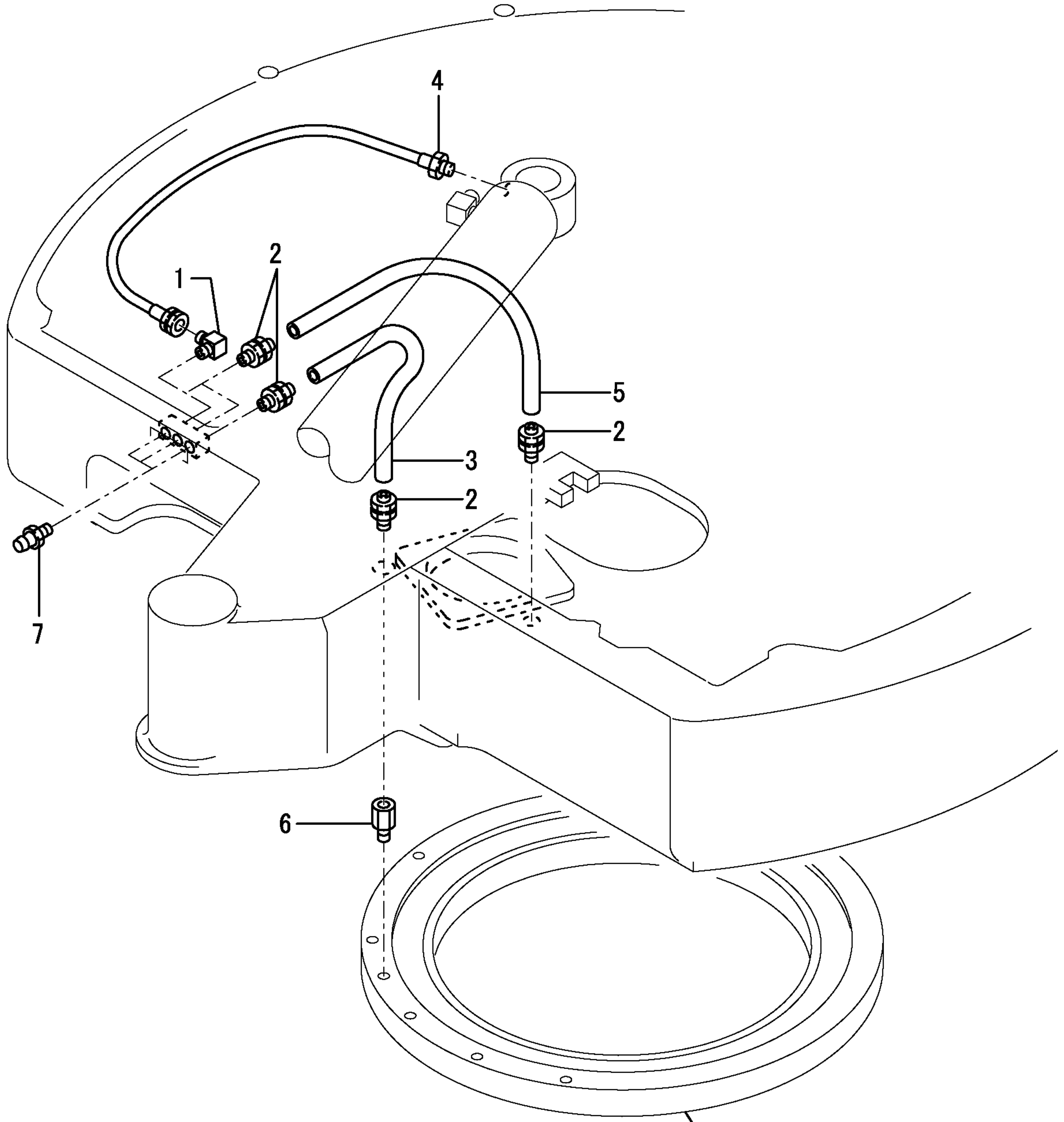
旋回ベアリング TURNIG BEARING
