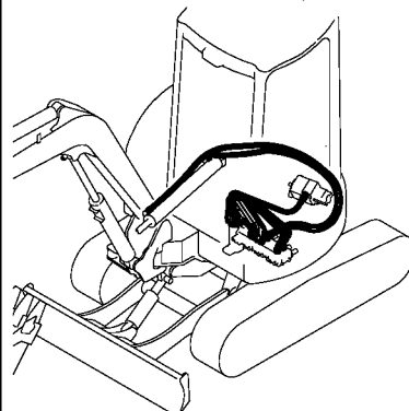
Fig. 72 油圧配管 (コントロールバルブ～ スイベル, スイング) HYD. OIL PIPING (CONTROL V. - SWIVEL, SWING)
