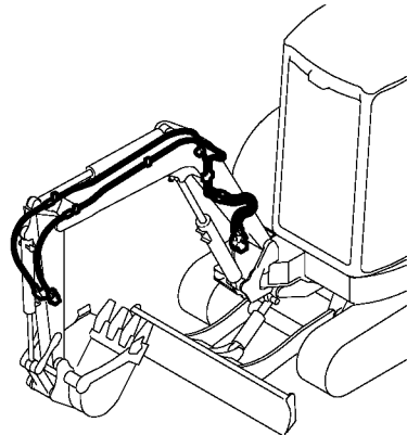
Fig. 78 油圧配管 (テレスコピックアーム) HYD. OIL PIPING (TELESCOPIC ARM)
