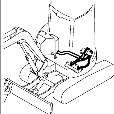
Fig. 71 油圧配管 (ポンプ, コントロールバルブ～モータ, ブーム) HYD. OIL PIPING (PUMP, CONTROL V. - MOTOR, BOOM)
