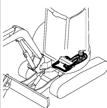
Fig. 83 コントロール配管 (リモコン バルブ～2ウェイロータリバルブ ～コントロールバルブ) CONTROL PIPING (REMOTE CONTROL V. - 2-WAY RORARY V. - CONTROL V.)
