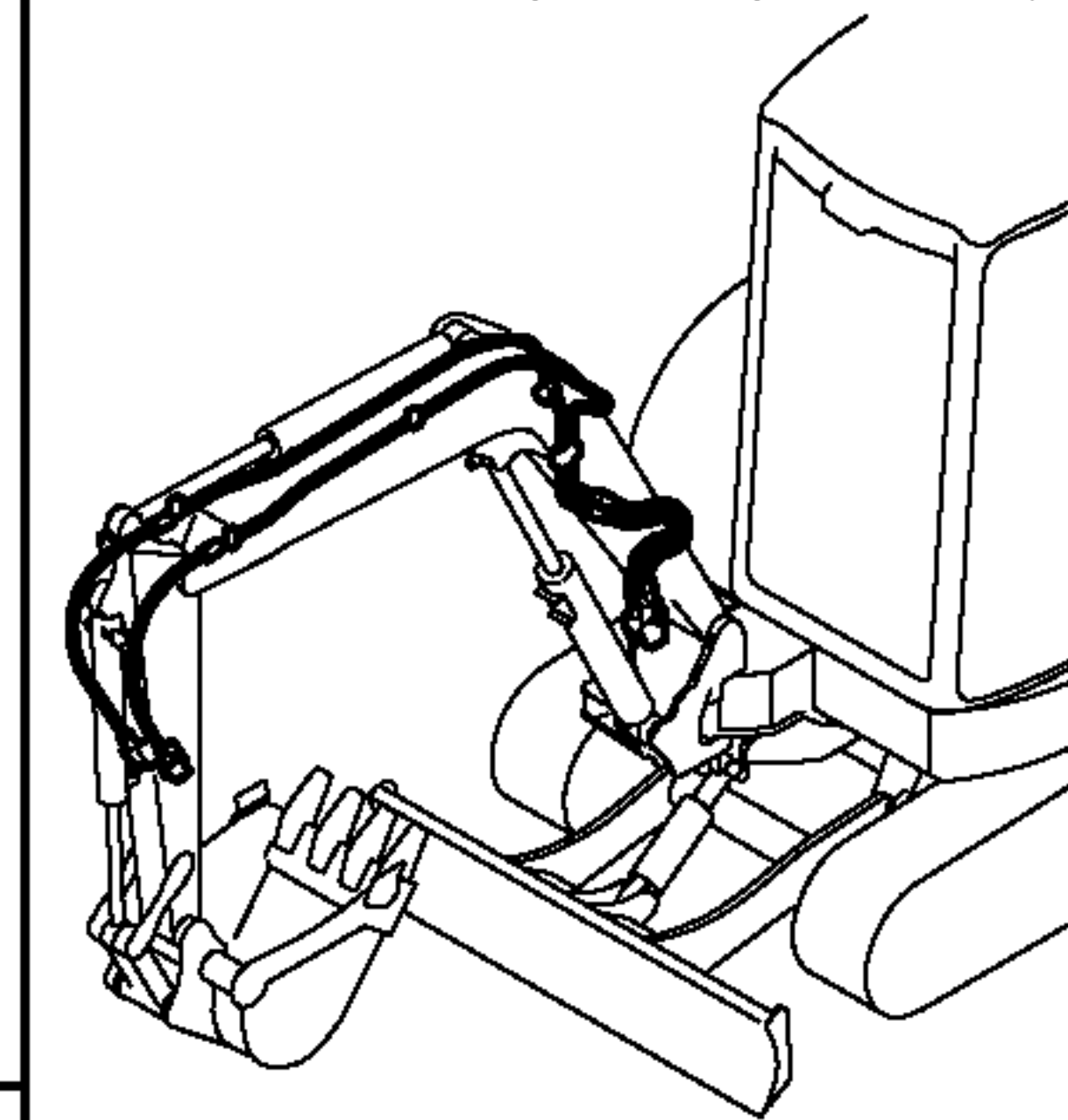
Fig.77 油圧配管 (PTO, アームエンド) HYD. OIL PIPING (P. T. O., ARM END)
