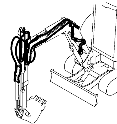
Fig. 79 コントロール配管 (ポンプ ～リモコンバルブ～リターン) CONTROL PIPING (PUMP - REMOTE CONTROL V. - RETURN)
