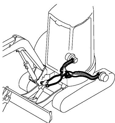
Fig. 76 油圧配管 (ブーム) HYD. OIL PIPING (BOOM)
