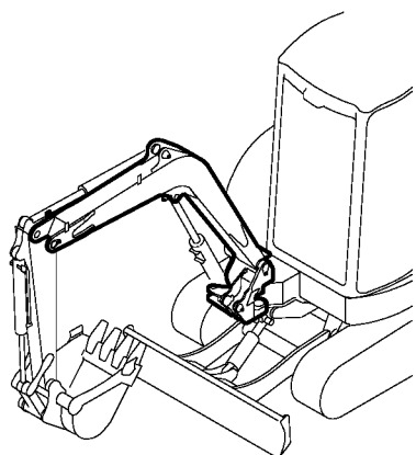
Fig. 86 アーム & バケットリンク ARM & BUCKET LINK
