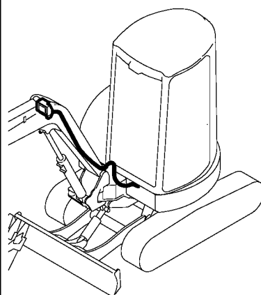
Fig. 23 ヒータ & デフロスタ HEATER & DEFROSTER
