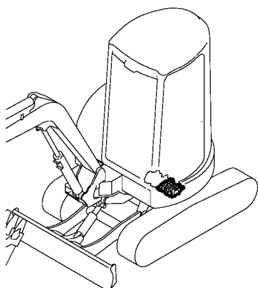
Fig. 64 コントロールバルブ (3/3) CONTROL VALVE (3/3)
