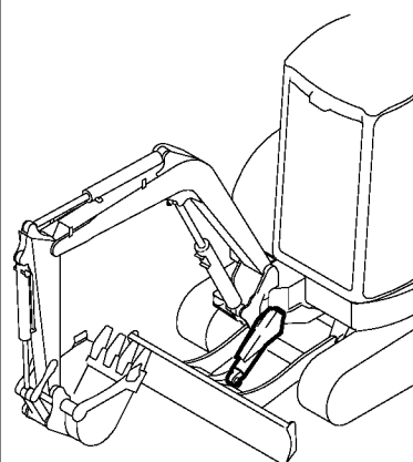
Fig. 58 スライドシリンダ (テレスコピックアーム) SLIDE CYLINDER (TELESCOPIC ARM)
