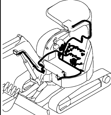
Fig. 31 電装品 (ワイリング) (新形) ELECTRIC PART (WIRING) (NEW)
