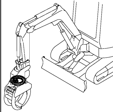
Fig. 68 旋回ピニオン & 旋回 ベアリング (林業仕様) TURNING PINION & TURNING BEARING (FORESTRY SPEC.)
