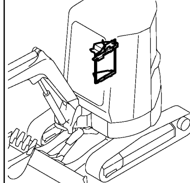
Fig. 24 ラジエータ、オイルクーラ & サブタンク (標準旧形:1 & アイコン仕様) RADIATOR, OIL-COOLER & SUB-TANK (STANDARD PREVIOUS:1 & A/C SPEC.)
