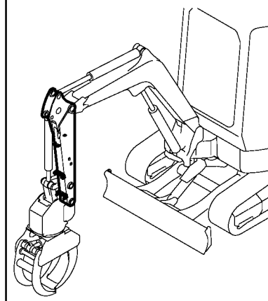
Fig. 156 アーム (林業仕様) ARM (FORESTRY SPEC.)
