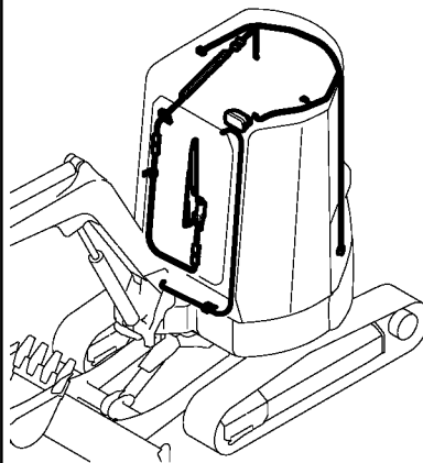
Fig. 91 キャビン(林業仕様) CABIN (FORESTRY SPEC.)
