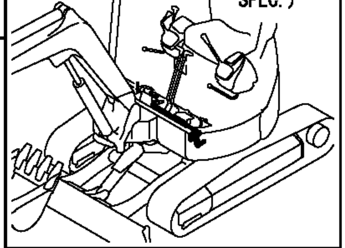
操縦装置 (PTOリンク) Fig.61 (標準 & 林業: 電磁仕様) CONTROL EQUIPMENT (P. T. O. LINK) (STANDARD & FORESTRY: ELECTRICAL SPEC.)
