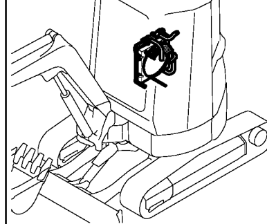
Fig. 24 ラジエータ、オイルクーラ & サブタンク (標準旧形:1 & アイコン仕様) RADIATOR, OIL-COOLER & SUB-TANK (STANDARD PREVIOUS:1 & A/C SPEC.)
