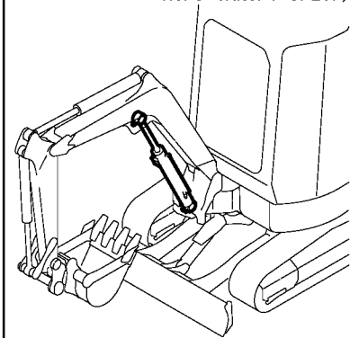
Fig. 100 ブームシリンダ (標準キャノ仕様) BOOM CYLINDER (STANDARD CANOPY SPEC.)
