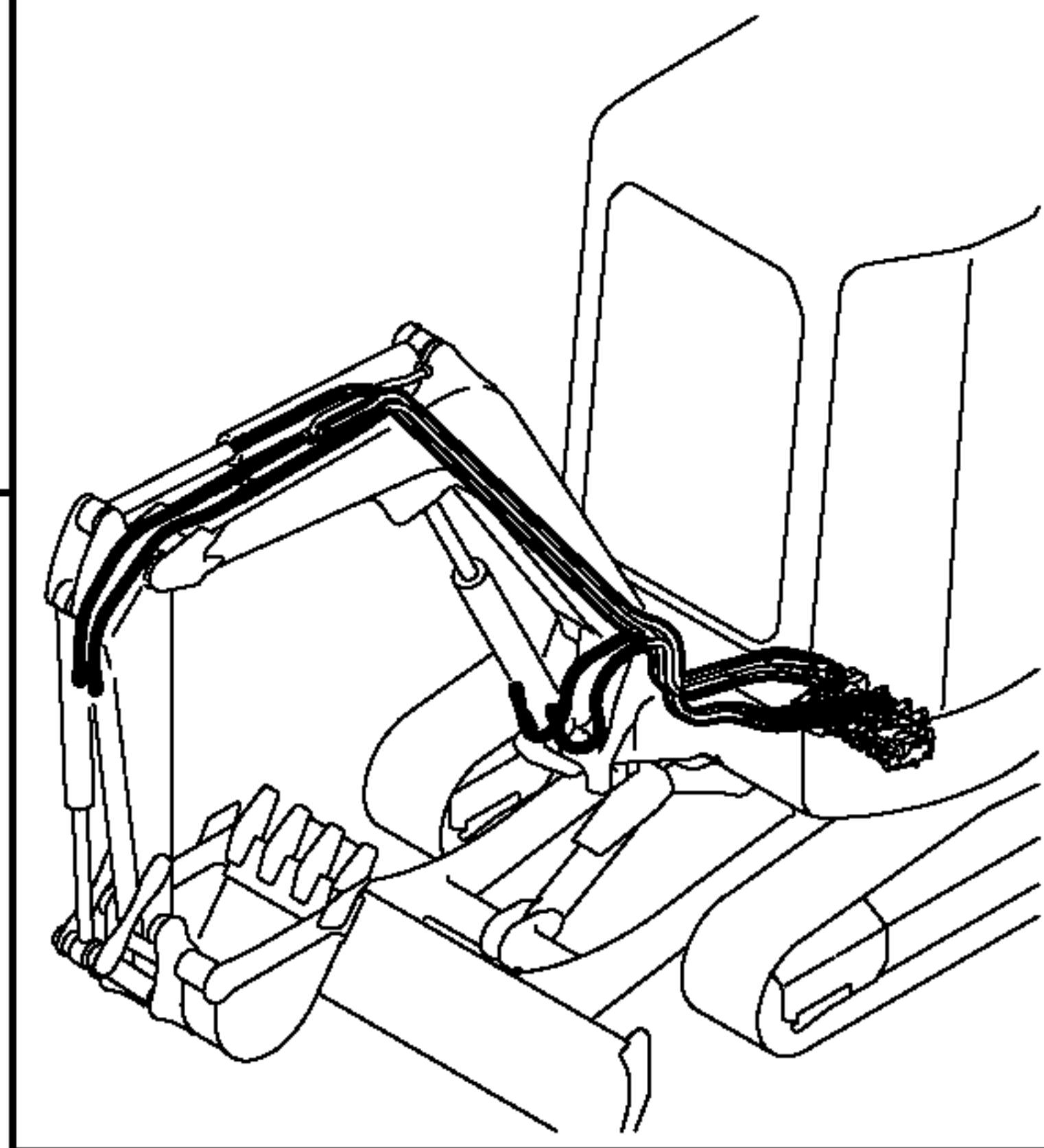
Fig. 135 油圧配管 (ブーム) HYD. OIL PIPING (BOOM)
