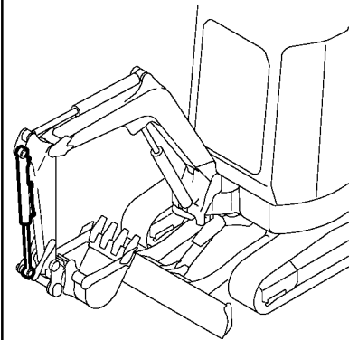
Fig. 104 スイングシリンダ SWING CYLINDER
