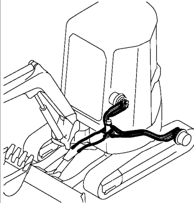
Fig. 135 油圧配管 (ブーム) HYD. OIL PIPING (BOOM)
