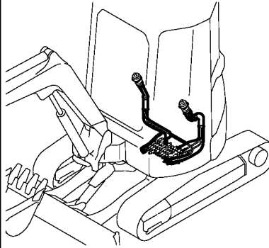
Fig. 147 コントロール配管 (リモコンV～4ウェイマルチ マシチェンジ仕様) CONTROL PIPING (REMOTE CONTROL V.～4-WAY MULTI V.:MULTI CHANGE SPEC.)
