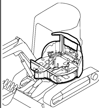
Fig. 66 旋回フレーム (新形) TURNING FRAME (NEW)
