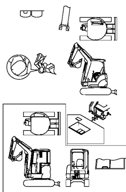
Fig. 4 銘板(クイックヒッチ) (JP) LABEL (QUICK HITCH) (JP)
