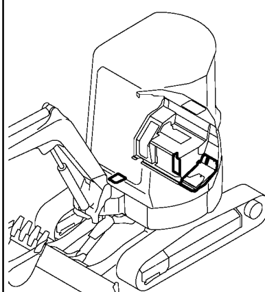
Fig. 72 カバー (キャビン) COVER (CABIN)
