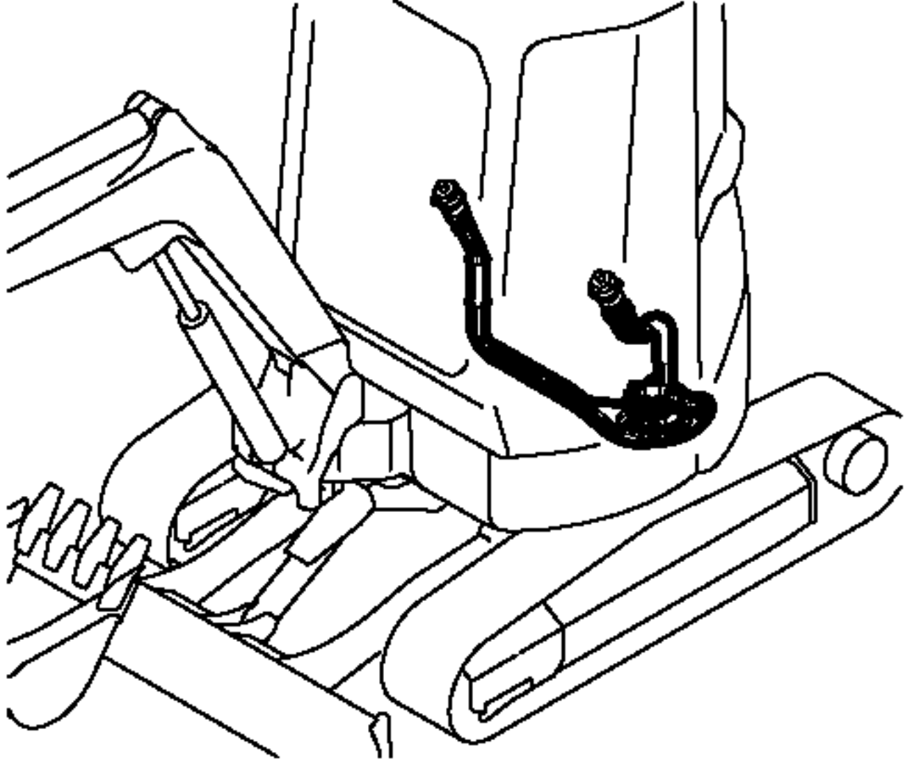
Fig. 147 コントロール配管 (リモコンV～4ウェイマルチV: マルチチェンジ仕様) CONTROL PIPING (REMOTE CONTROL V. ～4-WAY MULTI V. : MULTI CHANGE SPEC.)
