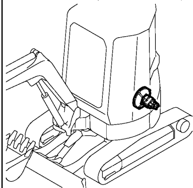
Fig. 98 油圧ポンプ & 軸継手 (クイックヒッチ仕様) HYD. OIL PUMP & JOINT (QUICK HITCH SPEC.)
