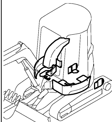
Fig. 70 カバー (フレーム) (林業仕様) COVER (FRAME) (FORESTRY SPEC.)
