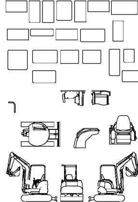
Fig. 11 安全銘板(クイックヒッチ) (JP) SAFETY LABEL (QUICK HITCH) (JP)
