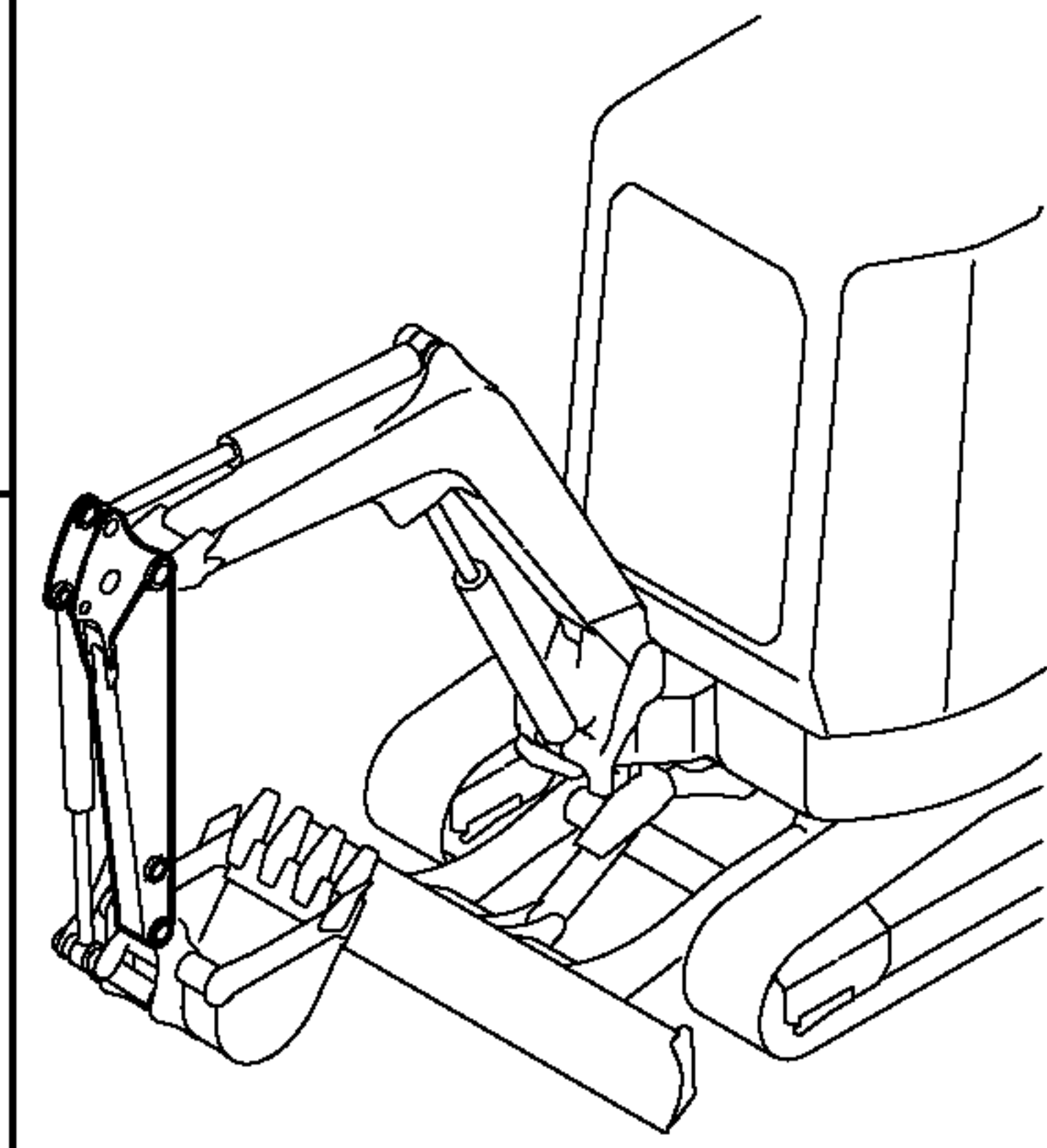
Fig. 155 アーム (ロング仕様) ARM (LONG SPEC.)
