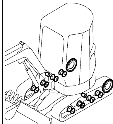
Fig. 48 スプロケット & ローラ SPROCKET & ROLLER
