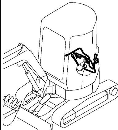
Fig. 19 エンジンマウント (標準旧形 & アイコン仕様 & ロフスカビ仕様) ENGINE MOUNT (STANDARD PREVIOUS, A/C SPEC. & ROPS CANOPY SPEC.)
