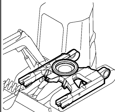
Fig. 68 旋回ピニオン & 旋回 ベアリング (林業仕様) TURNING PINION & TURNING BEARING (FORESTRY SPEC.)
