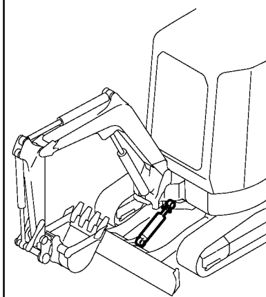
Fig. 106 ヒッチシリンダ HITCH CYLINDER
