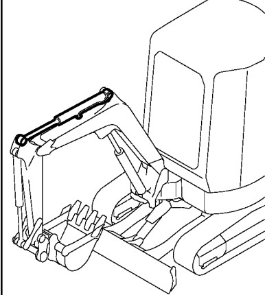
Fig. 102 バケットシリンダ (標準仕様) BUCKET CYLINDER (STANDARD SPEC.)
