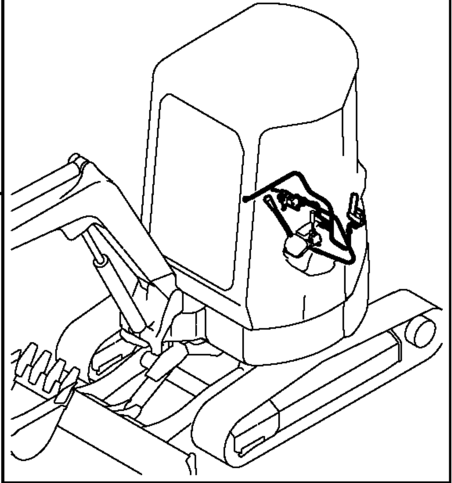
ワンタッチデセル(オプション) Fig. 18 ONE TOUCH DECEL (OPTIONAL)
