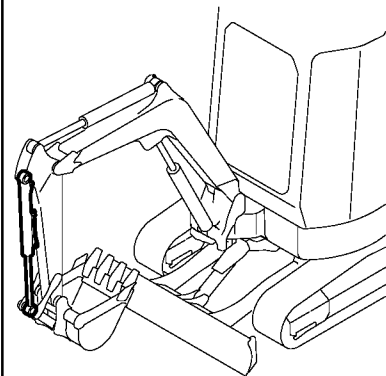
Fig. 103 バケットシリンダ (クイックヒッチ仕様) BUCKET CYLINDER (QUICK HITCH SPEC.)
