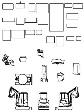
Fig. 14 安全銘板 (キャノピー) (EX) SAFETY LABEL (CANOPY) (EX)
