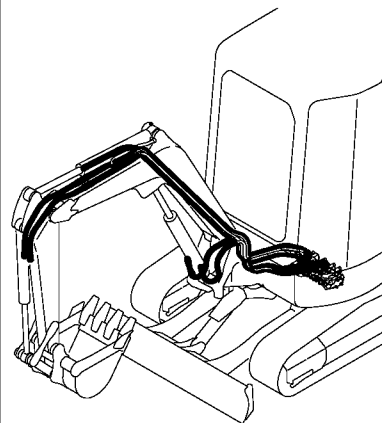
Fig. 136 油圧配管 (PTO, アームエンド) HYD. OIL PIPING (P. T. O., ARM END)
