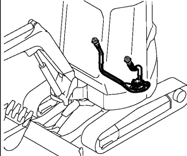
Fig. 148 コントロール配管 (4ウェイマルチ V～コントロールV:マルチチェンジ仕様) CONTROL PIPING (4-WAY MULTI V.～CONTROL V.: MULTI CHANGE SPEC.)
