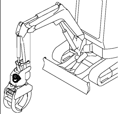
Fig. 111 スイベルジョイント SWIVEL JOINT
