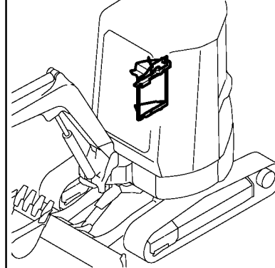
Fig. 23 ラジエータマウント (標準新形) RADIATOR MOUNT (STANDARD NEW)
