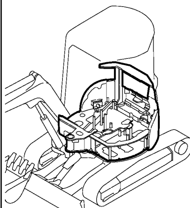
Fig. 67 走行フレーム & 旋回ベアリング TRACK FRAME & TURNING BEARING
