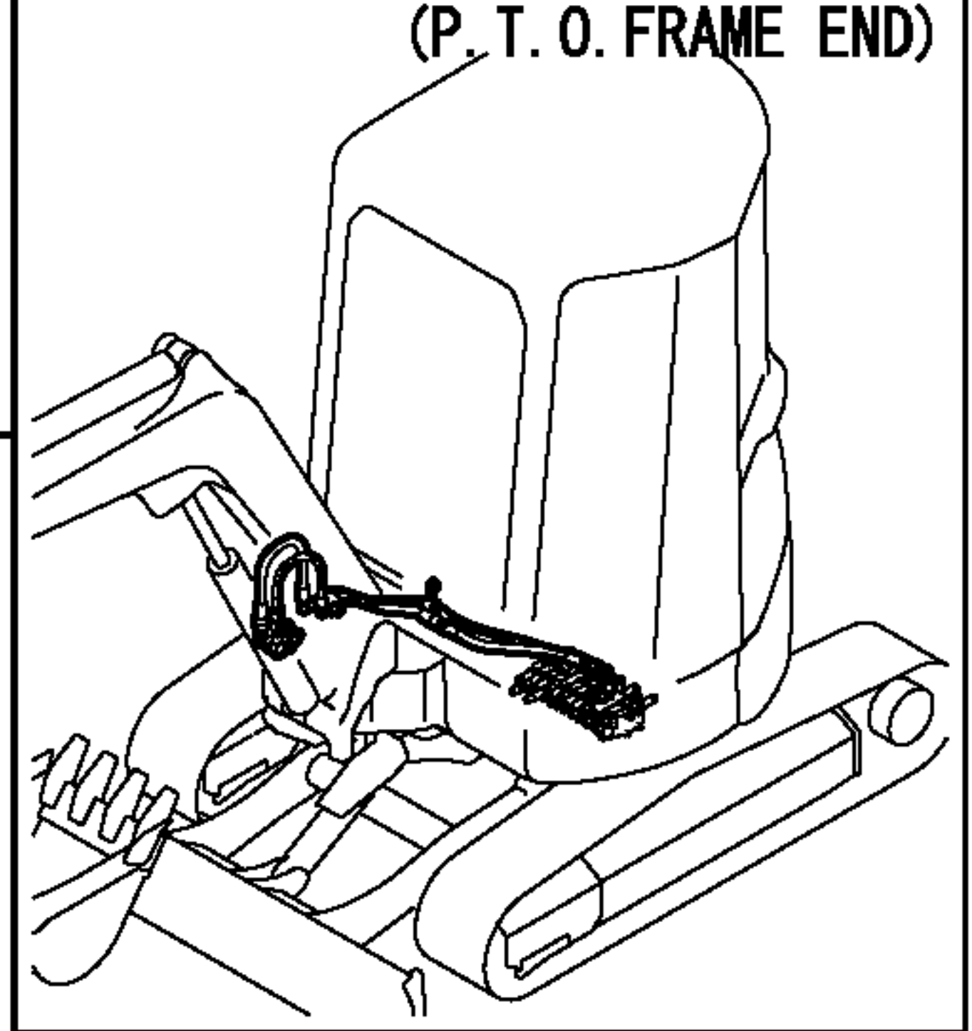
油圧配管 (PTOアームエンド) Fig.136 HYD. OIL PIPING (P. T. O. ARM END)
