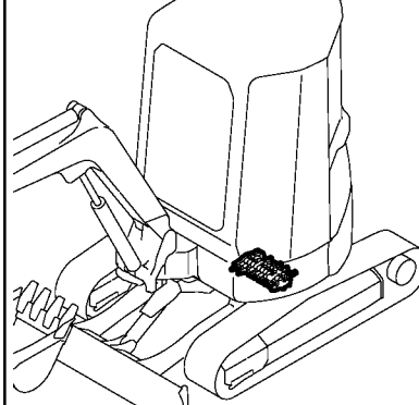
Fig. 115 コントロールバルブ (Pポート & 走行:左) CONTROL VALVE (P-PORT & TRAVEL:LEFT)
