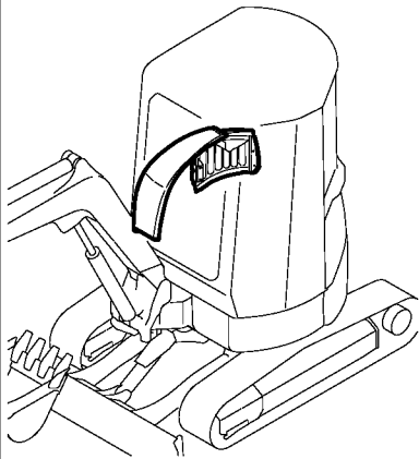
Fig. 86 ボンネット(2) (新形) BONNET (2) (NEW)
