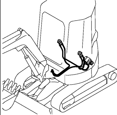
Fig. 146 コントロール配管 (リモコン ～コントロールV:標準仕様) CONTROL PIPING (REMOTE CONTROL V.～CONTROL V. :STANDARD SPEC.)
