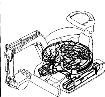
Fig.19 フレーム&旋回ベアリング FRAME & TURNING BEARING
