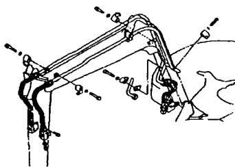
Fig.55 コントロール配管 (ダイレクト) CONTROL PIPING (DIRECT)
