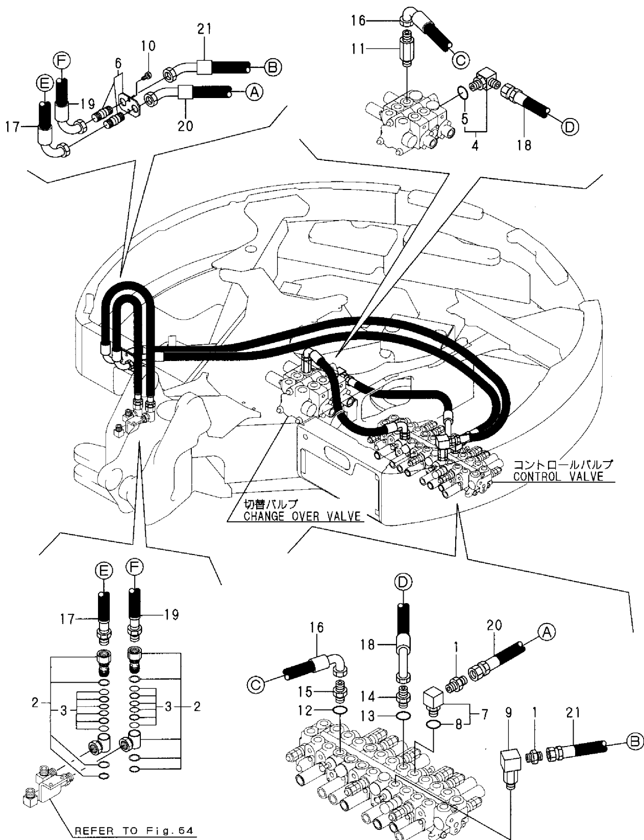
Fig. 51 油圧配管 (バルブ~切替バルブ、フレーム) HYD. OIL PIPING (VALVE~CHANGE OVER VALVE, FRAME)
