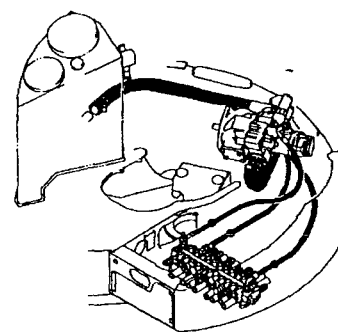
Fig.48 油圧配管 (バルブ〜モータ、ブーム) HYD. OIL PIPING (VALVE~MOTOR, BOOM)
