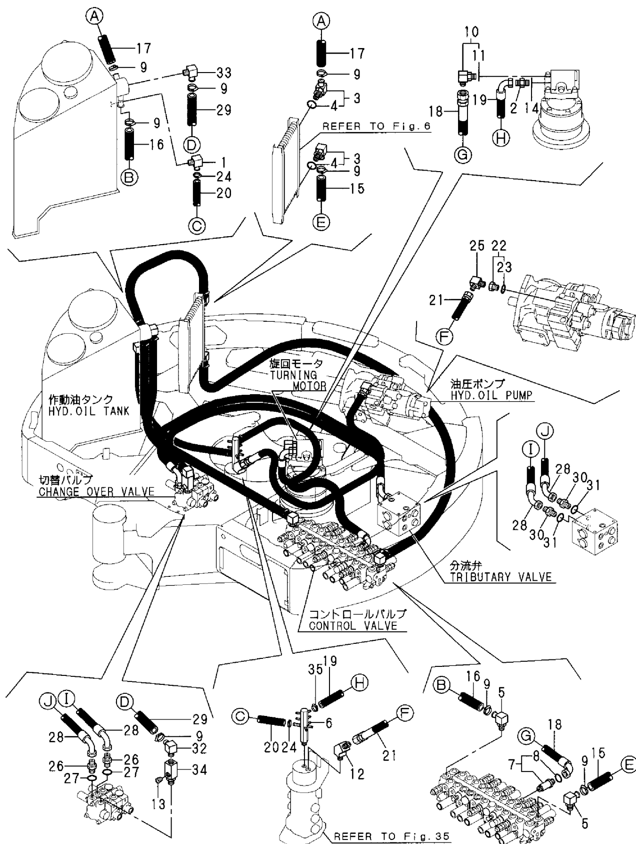
Fig. 50 油圧配管 (リターン) HYD. OIL PIPING (RETURN)
