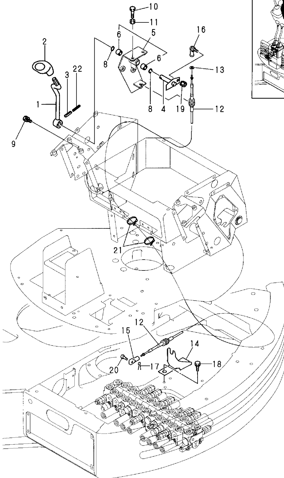
Fig. 16 操縦装置 (ブレード) CONTROL EQUIP. (BLADE)
