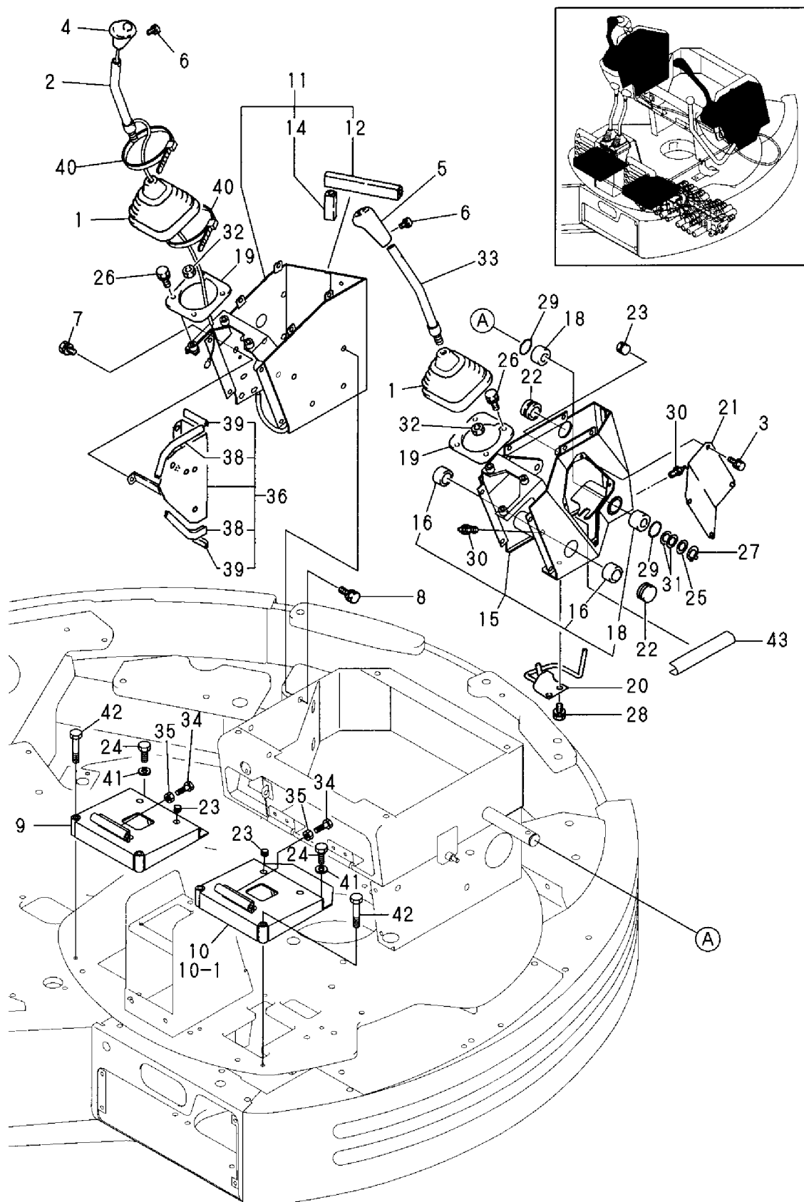
Fig. 13 操縦装置 (作業レバー&スタンド) CONTROL EQUIP. (OPERATION LEVER & STAND)
