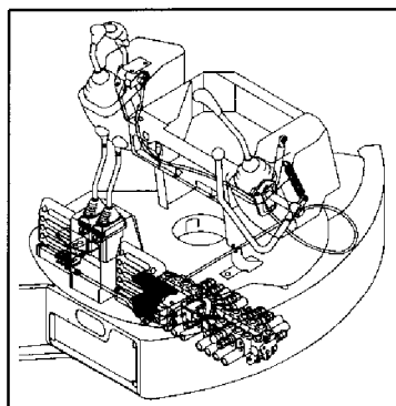
Fig. 18 操縦装置 (P. T. O. コントロール) CONTROL EQUIP. (P. T. O. CONTROL)
