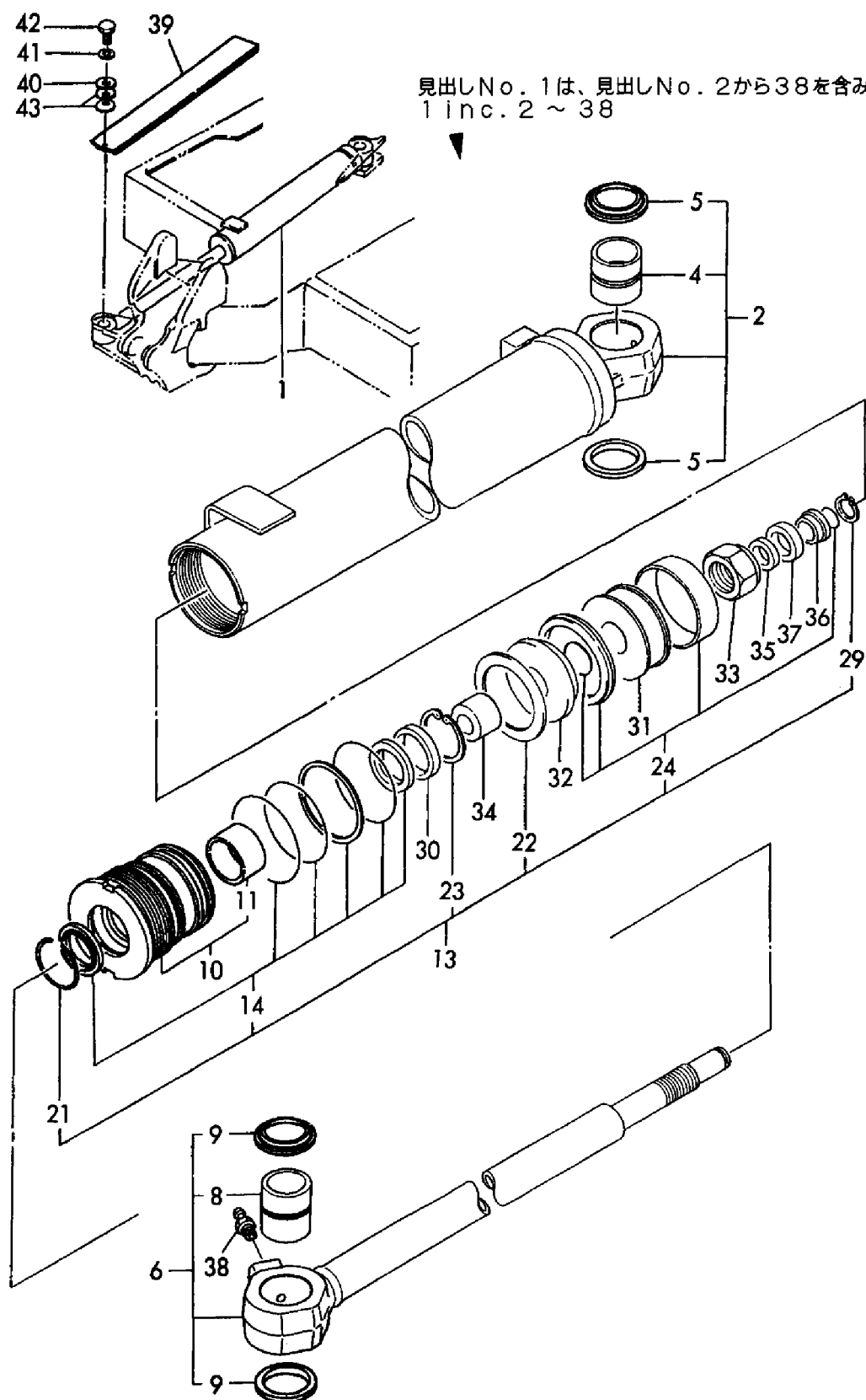
Fig. 31 スイングシリンダ SWING CYLINDER
