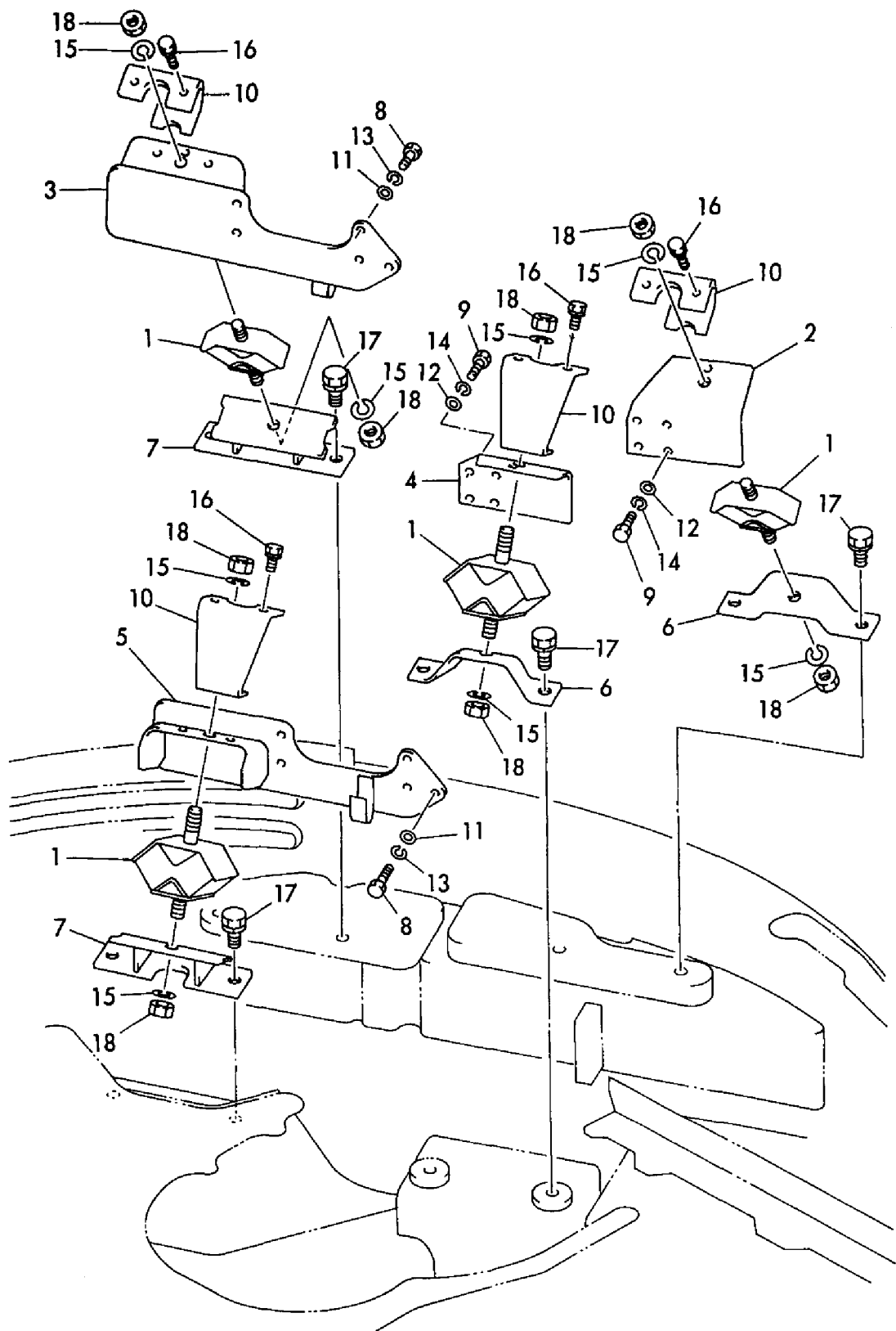
Fig. 5 エンジンマウント ENGINE MOUNT
