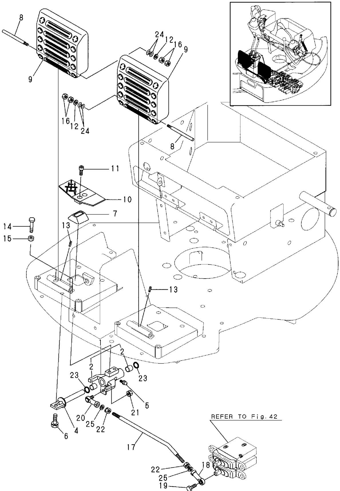
Fig. 15 操縦装置 (スイング) CONTROL EQUIP. (SWING)
