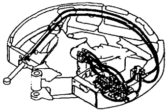
Fig.50 油圧配管 (リターン) HYD.OIL PIPING (RETURN)
