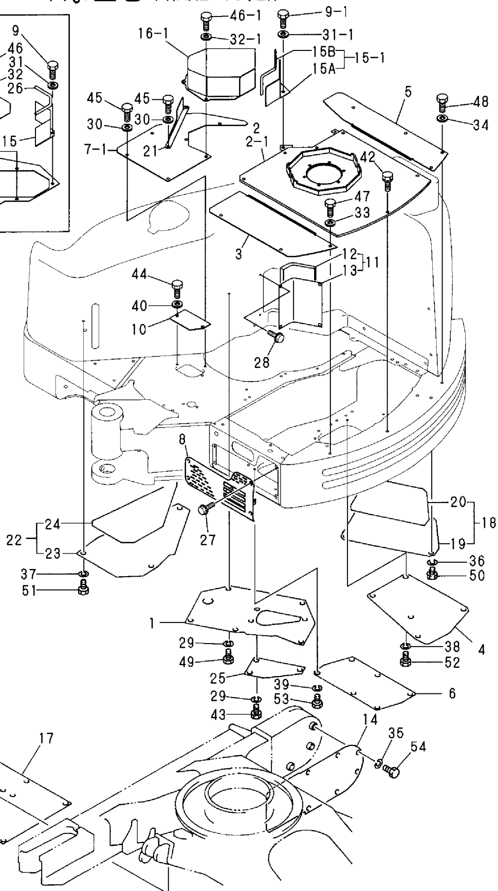
Fig. 20 フレームカバー FRAME COVER
