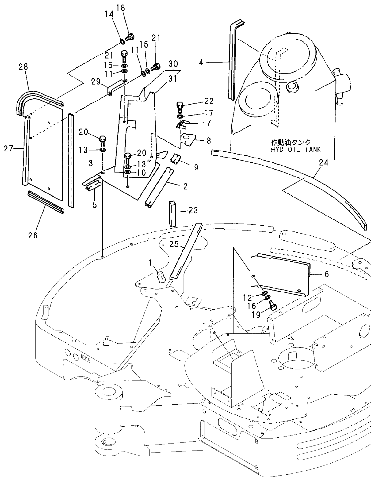
Fig. 25 ダクト DUCT
