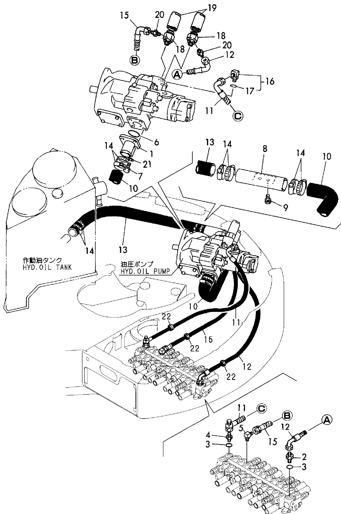
Fig. 47 油圧配管 (タンク~ポンプ~バルブ) HYD. OIL PIPING (TANK~PUMP~VALVE)
