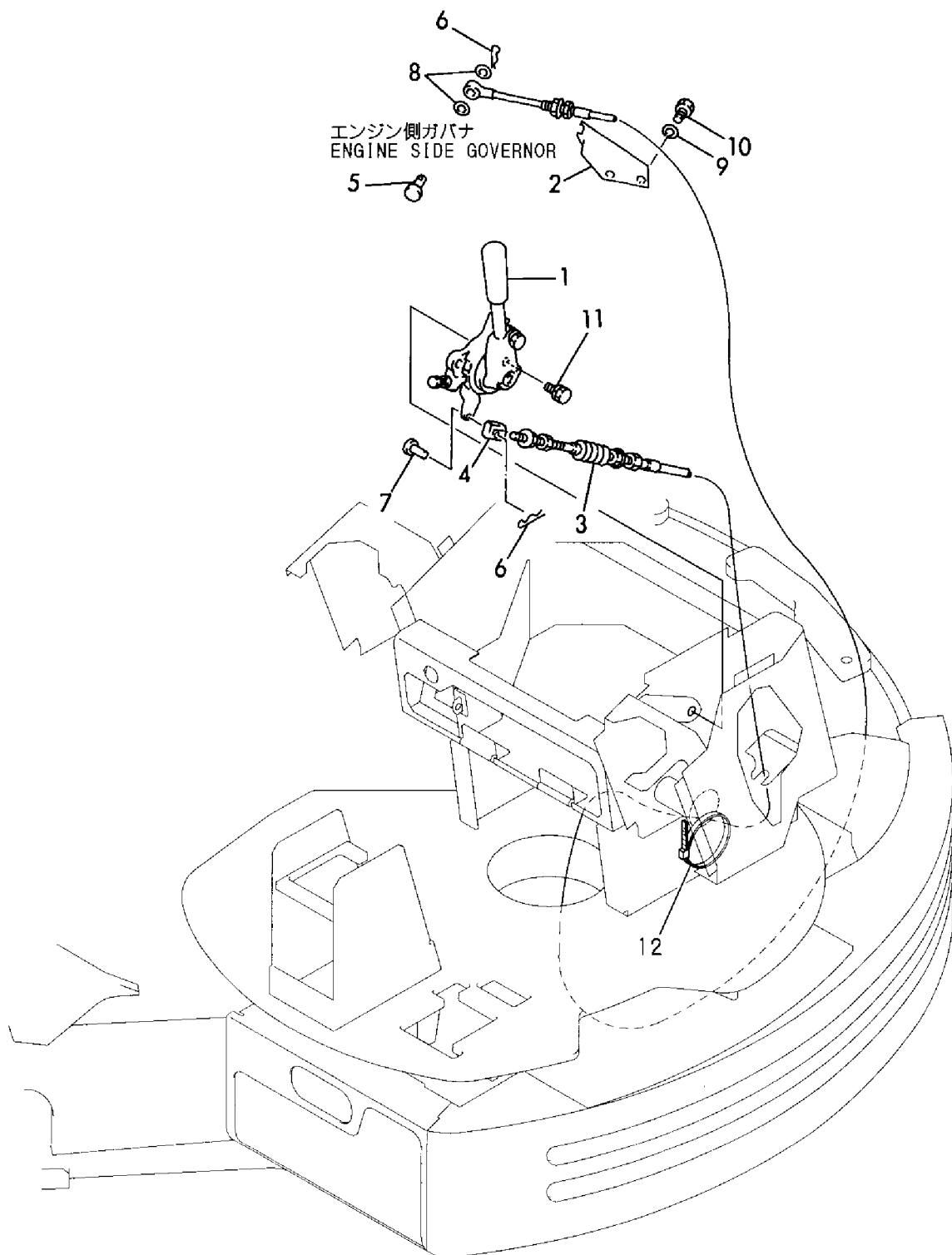
Fig. 4 アクセル ACCELERATOR
