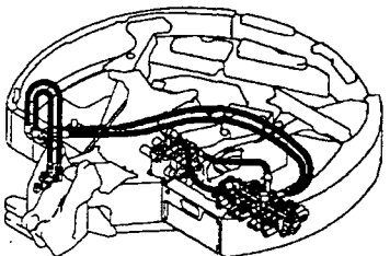
Fig.51 油圧配管 (バルブ〜切換バルブ、フレーム) HYD.OIL PIPING (VALVE~CHANGE OVER VALVE, FRAME)
