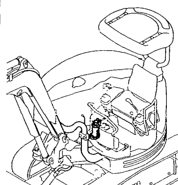
Fig.35 スイベルジョイント SWIVEL JOINT
