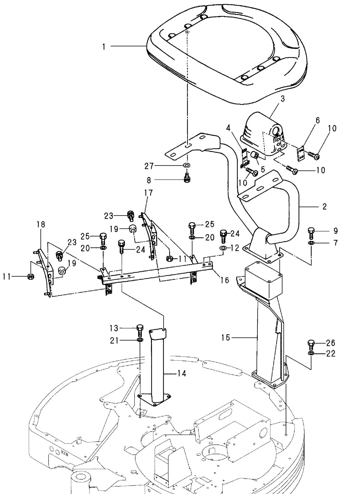
Fig. 26 キヤノピ&キヤノピフレーム CANOPY & CANOPY FRAME
