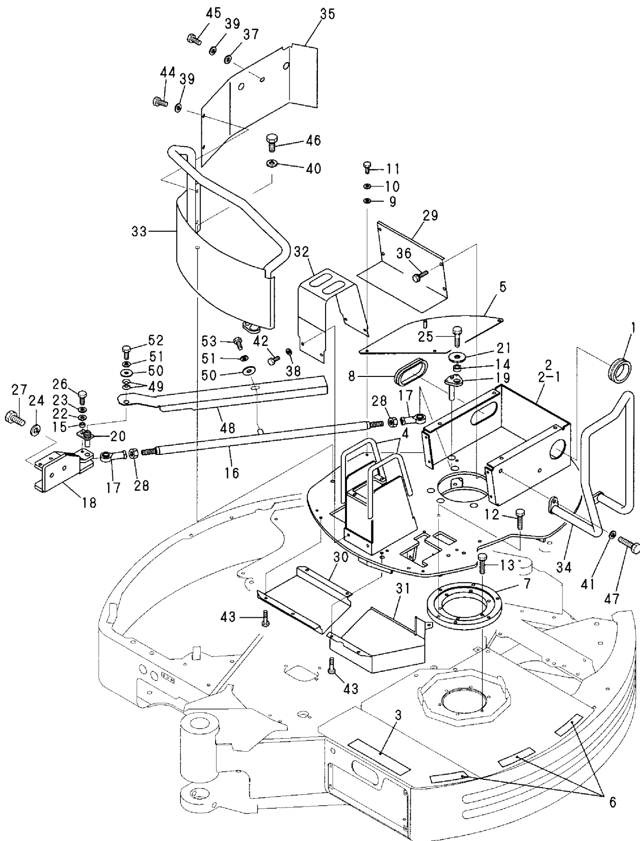
Fig. 21 ターンテーブル TURN TABLE
