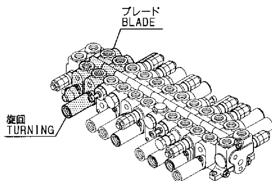
Fig. 40 コントロールバルブ (旋回&ブレード) CONTROL VALVE (TURNING & BLADE)
