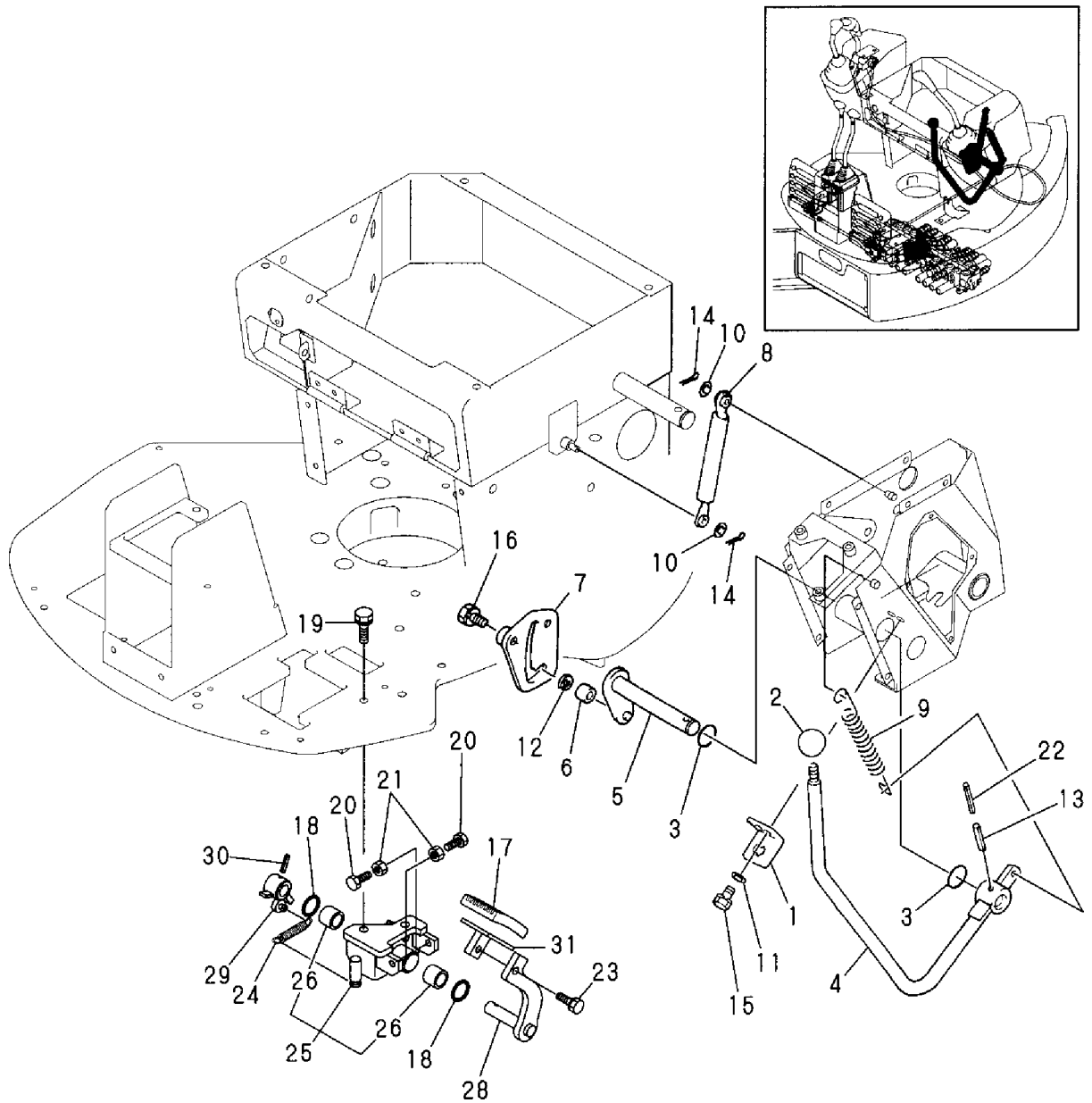
Fig. 17 操縦装置 (カットオフレバーローハイペダル) CONTROL EQUIP. (CUT OFF LEVER & LOW-HIGH PEDAL)
