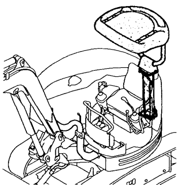
Fig.26 キャノピ&キャノピフレーム CANOPY & CANOPY FRAME
