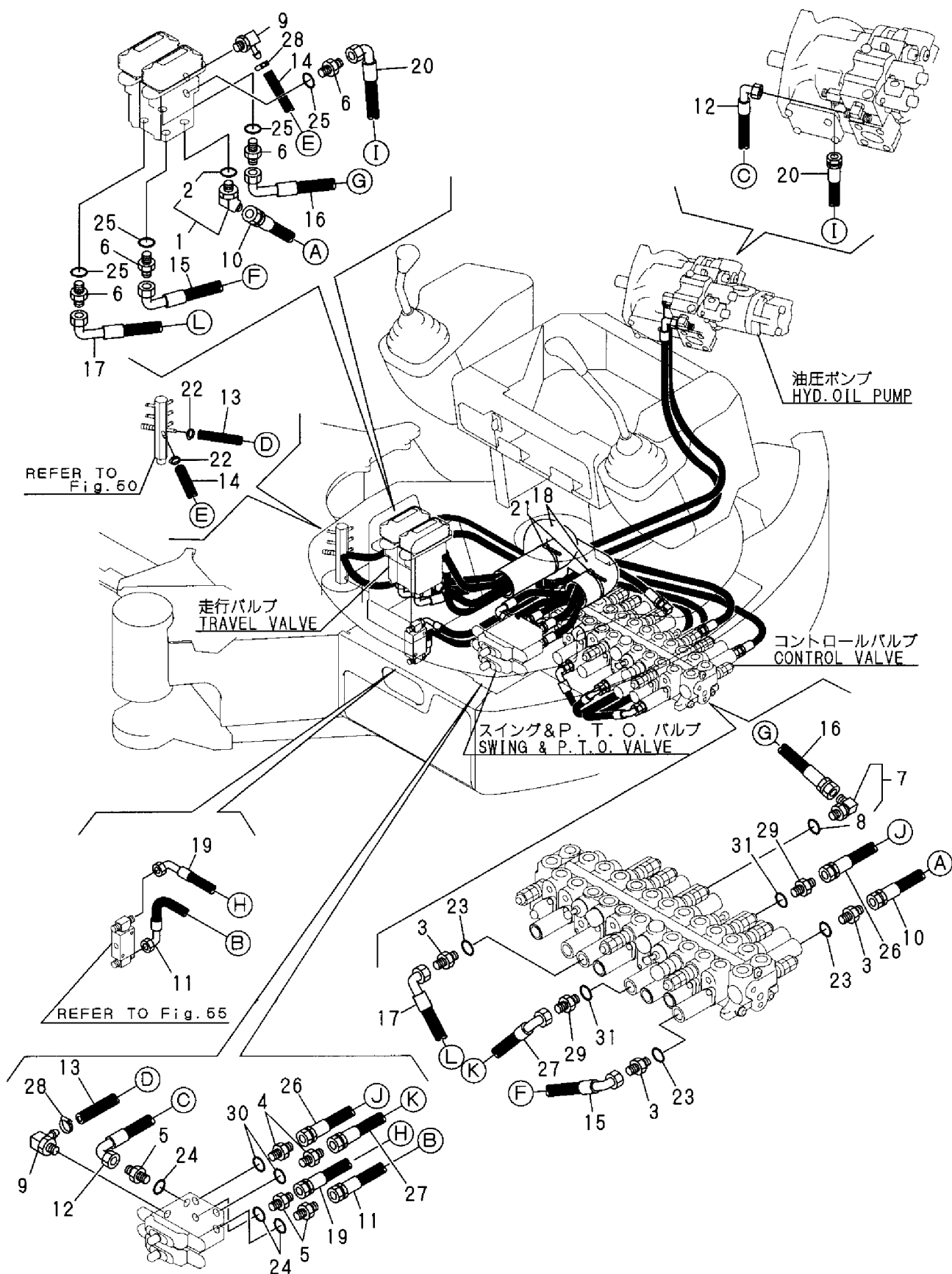
Fig. 56 コントロール配管 (走行&スイング) CONTROL PIPING (TRAVEL & SWING)
