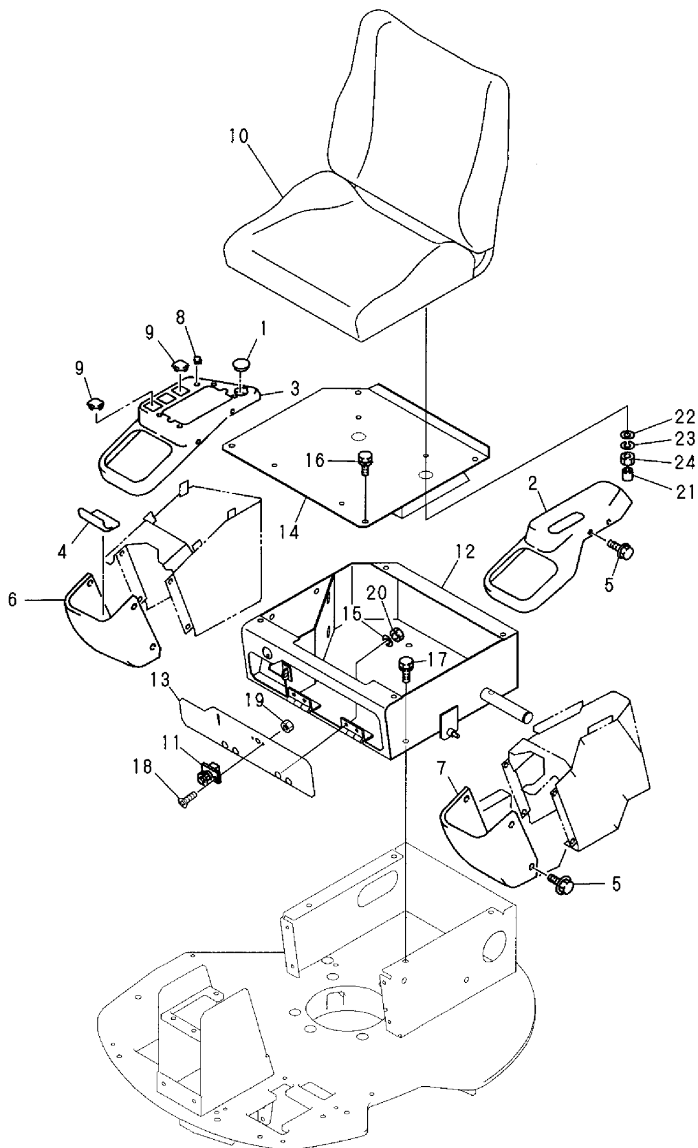
Fig. 22 シート & シートマウント SEAT & SEAT MOUNT
