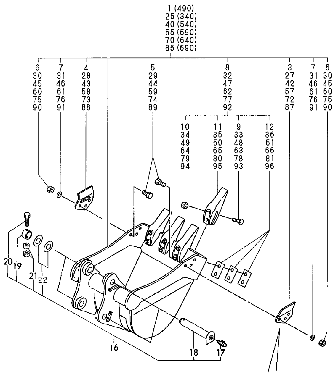
Fig. 62 バケット (アタッチメント) BUCKET (ATTACHMENT)
