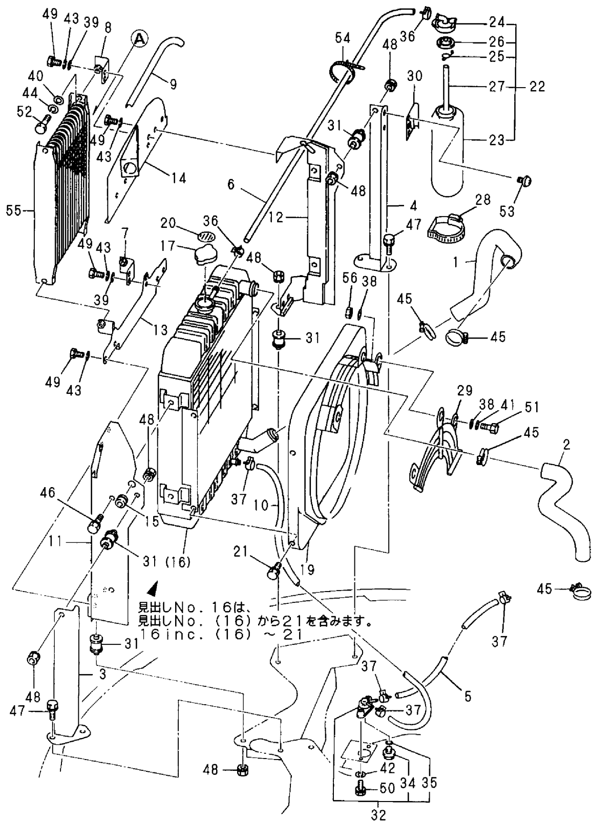
Fig. 6 ラジエーター&オイルクーラ RADIATOR & OIL COOLER
