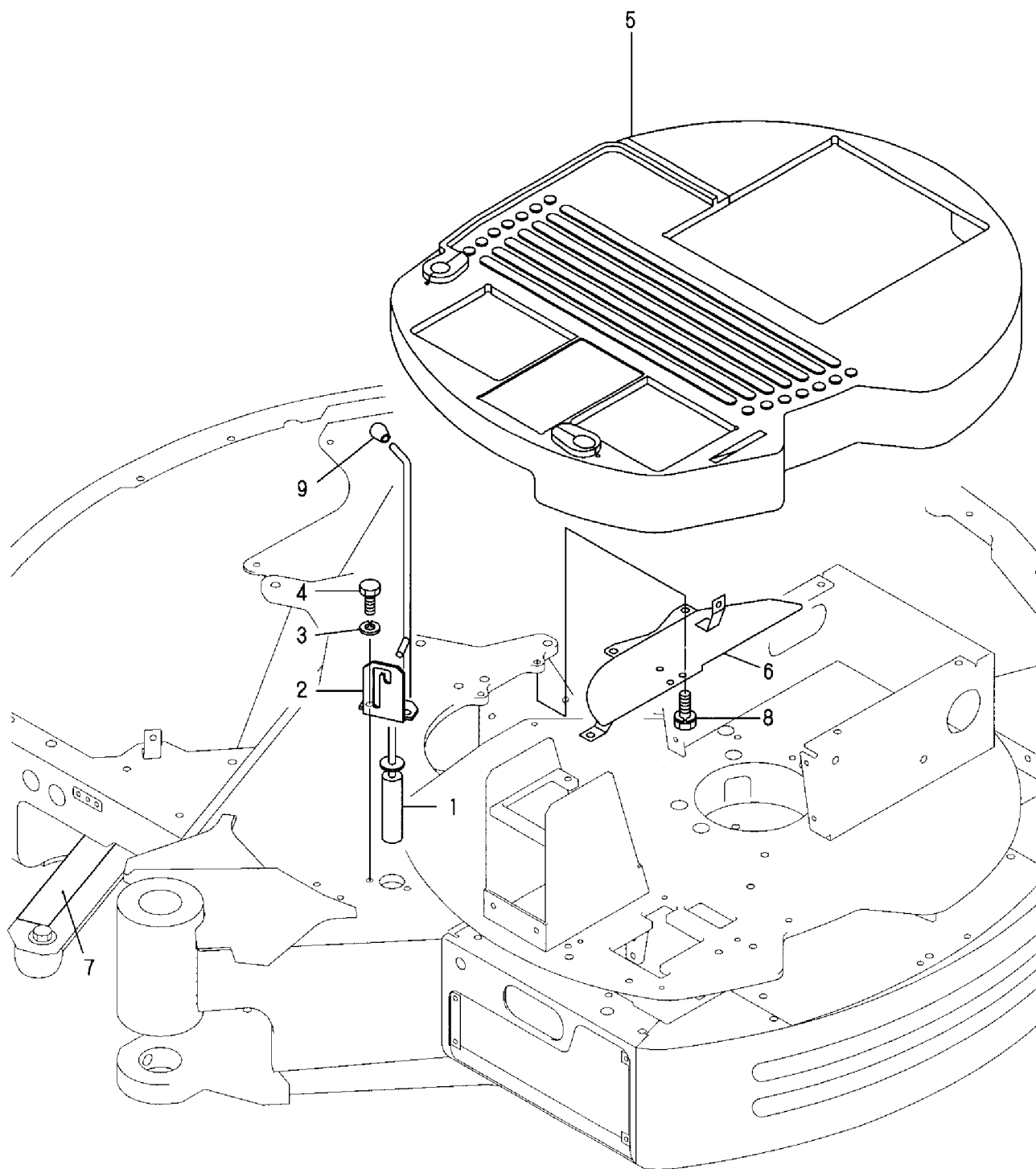
Fig. 23 ステップ STEP
