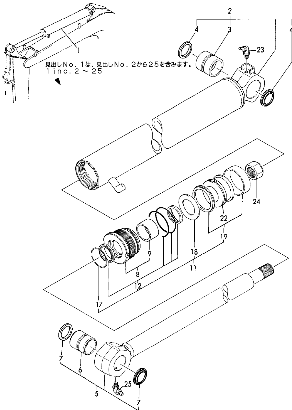
Fig. 29 アームシリンダ ARM CYLINDER
