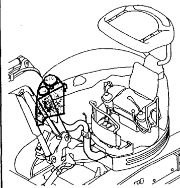
Fig.47 油圧配管 (タンク〜ポンプ〜バルブ) HYD. OIL PIPING (TANK~PUMP~VALVE)
