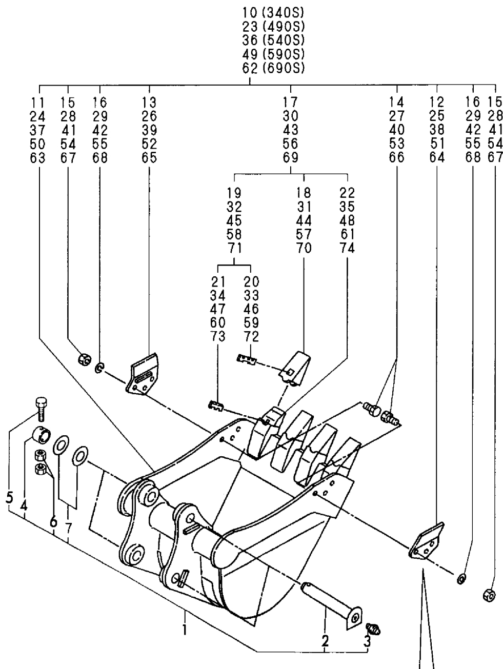
Fig. 61 バケットSタイプ (アタッチメント) BUCKET S TYPE (ATTACHMENT)
