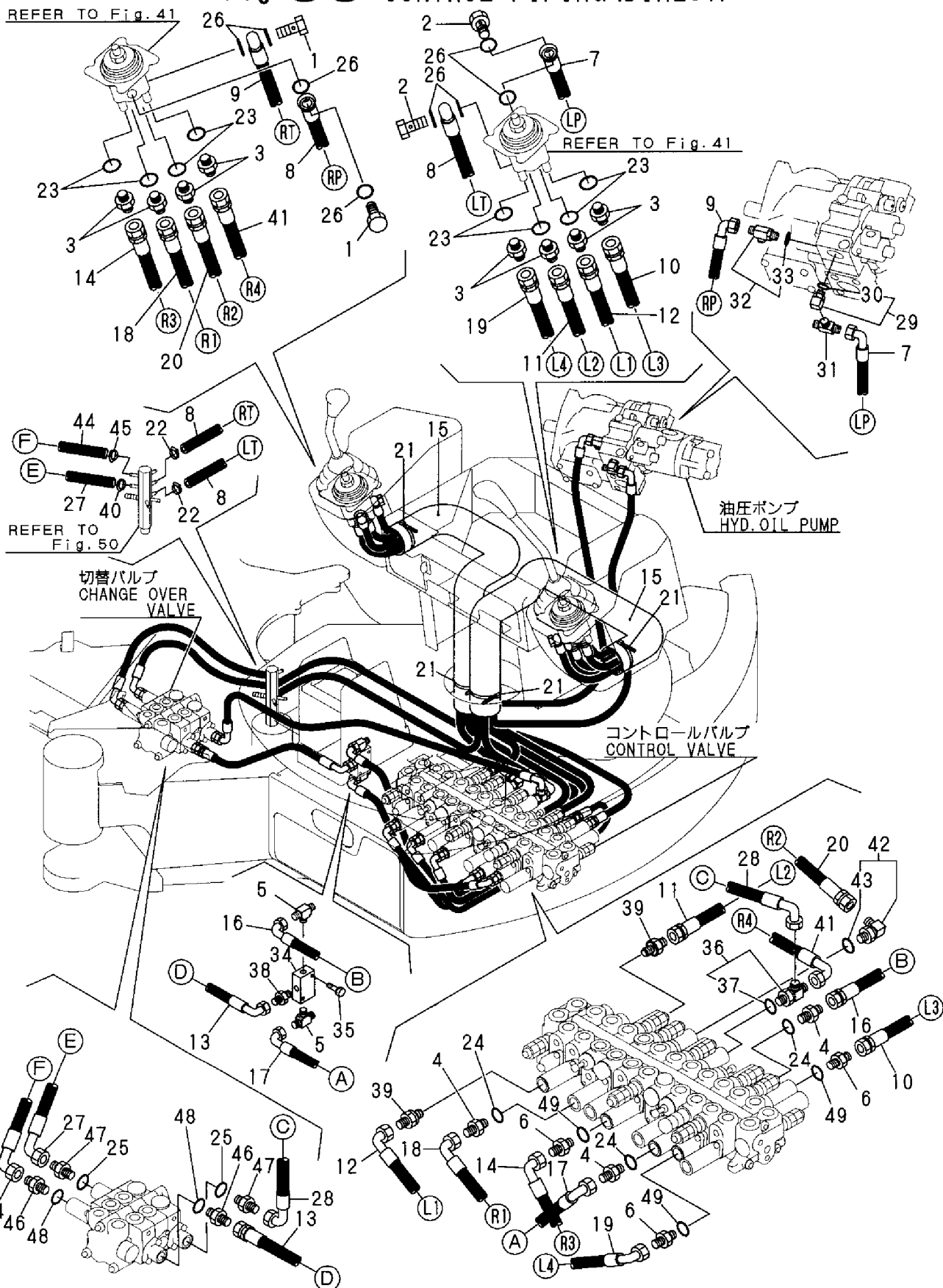
Fig. 55 コントロール配管 (ダイレクト) CONTROL PIPING (DIRECT)
