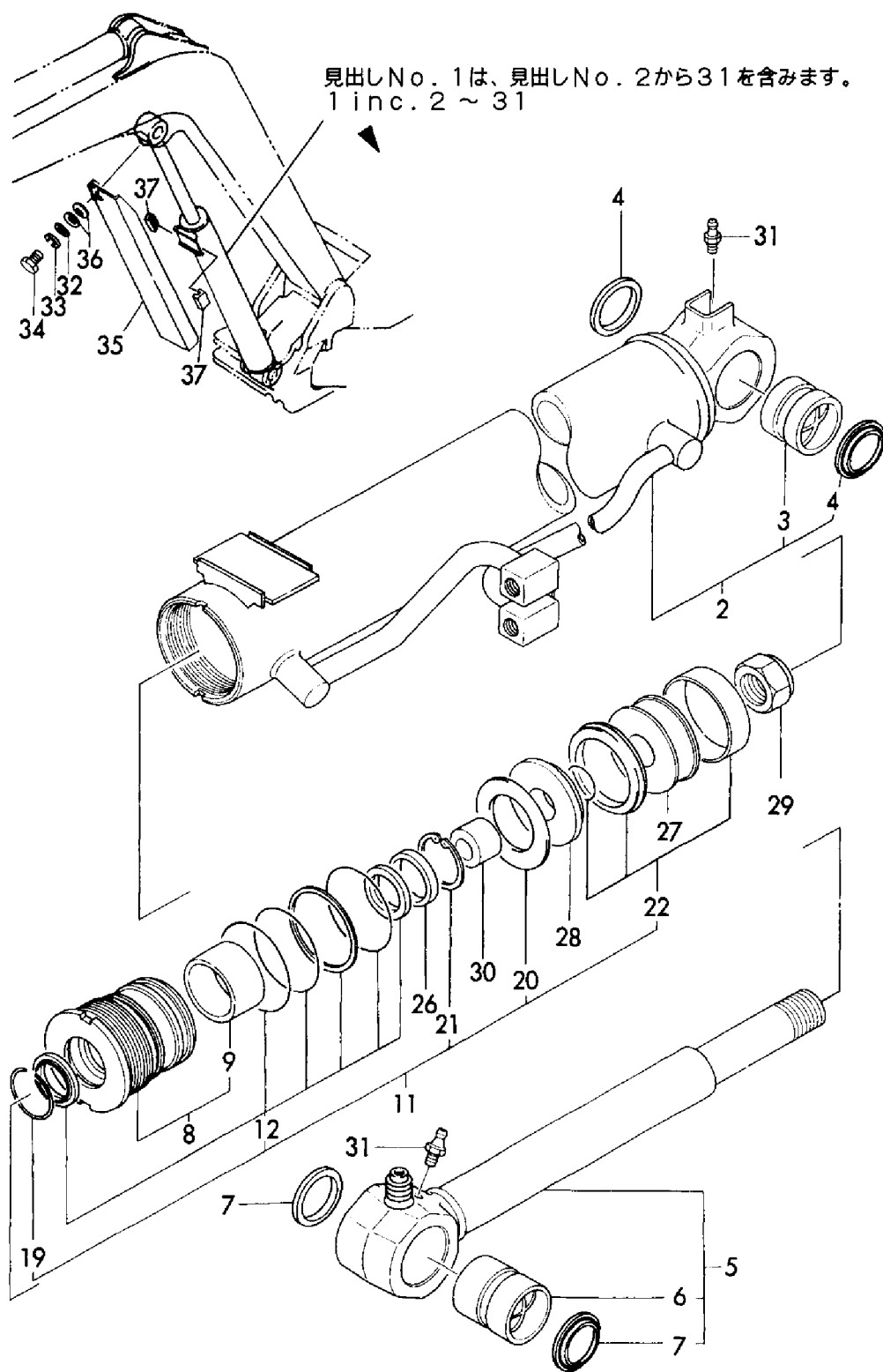
Fig. 28 ブームシリンダ BOOM CYLINDER
