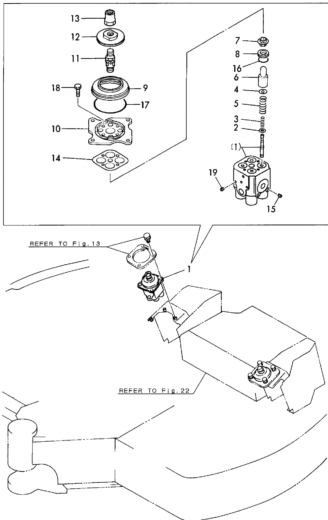
Fig. 41 リモコンバルブ (作業機) REMOTE CONTROL VALVE (WORK EQUIPMENT)
