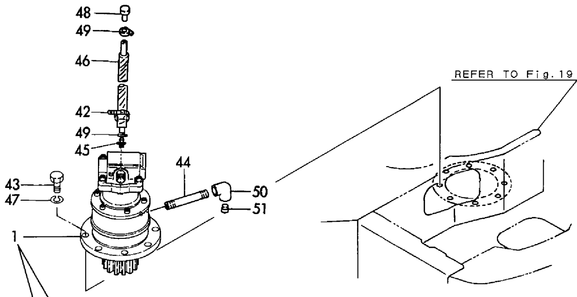
Fig. 34 旋回モータ TURNING MOTOR
