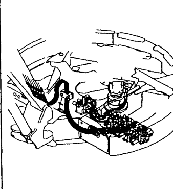
Fig.48 油圧配管 (バルブ〜モータ、ブーム) HYD. OIL PIPING (VALVE~MOTOR, BOOM)
