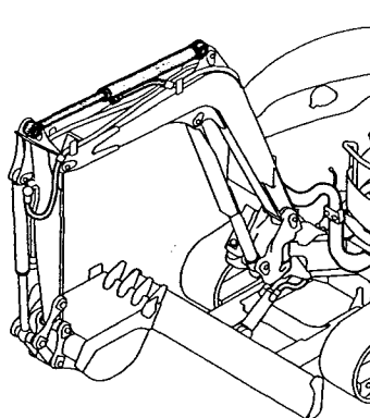
Fig.30 バケットシリンダ BUCKET CYLINDER
