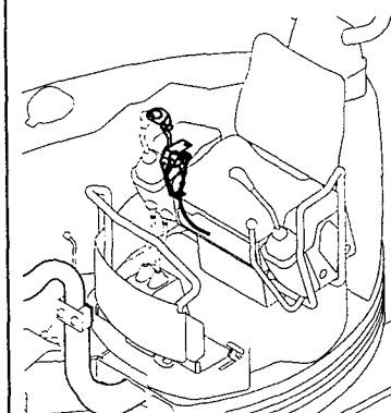
Fig.16 操縦装置 (ブレード) CONTROL EQUIP. (BLADE)
