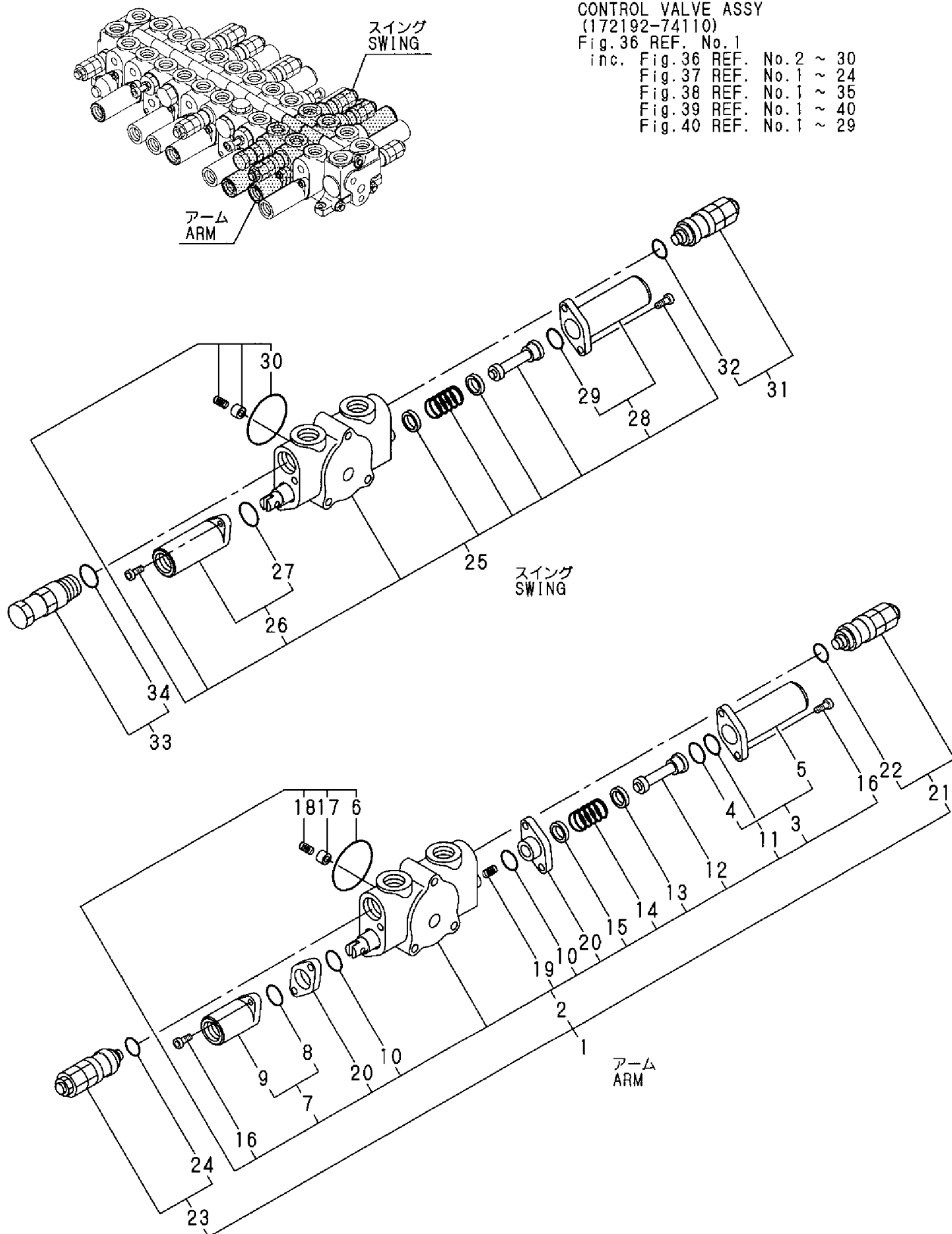
Fig. 38 コントロールバルブ (アーム&スイング) CONTROL VALVE (ARM & SWING)
