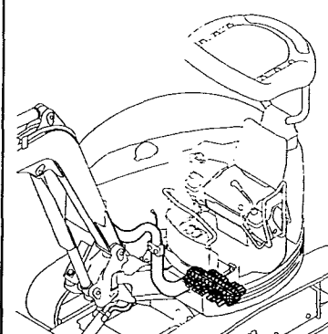
Fig.36 コントロールバルブ (Pポート) CONTROL VALVE (P PORT)
