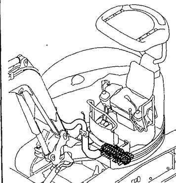
Fig.40 コントロールバルブ (旋回&ブレード) CONTROL VALVE (TURNING & BLADE)
