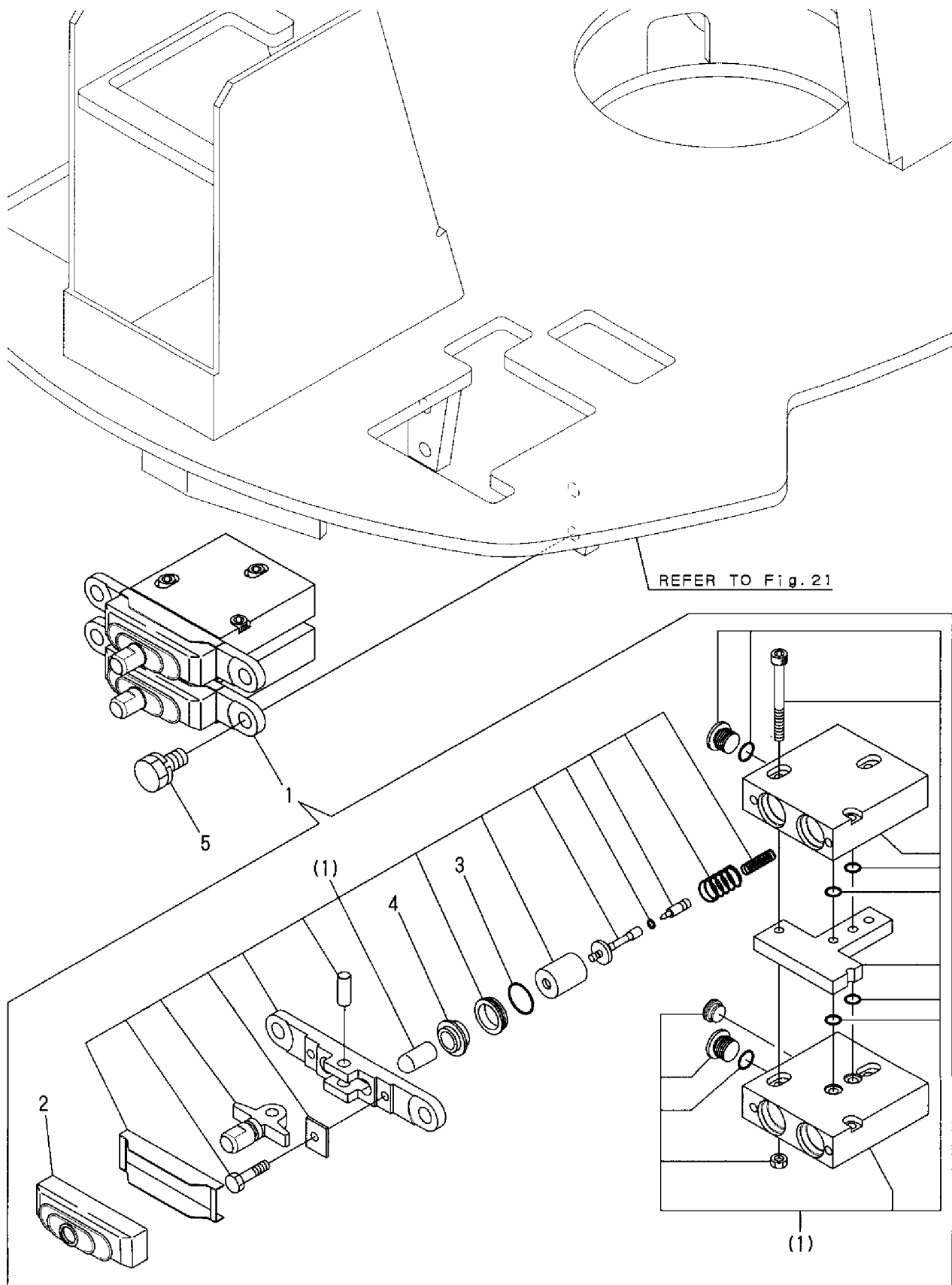
リモコンバルブ (スイング&P.T.O.) REMOTE CONTROL VALVE (SWING & P.T.O.)
