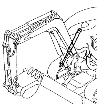
Fig.31 スイングシリンダ SWING CYLINDER
