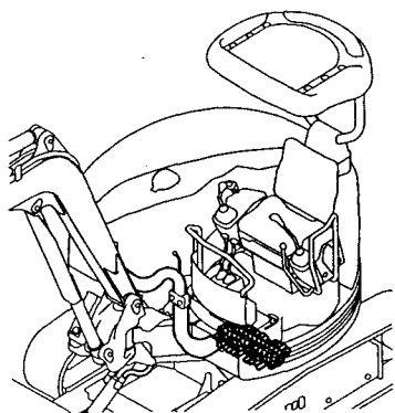
Fig.38 コントロールバルブ (アーム&スイング) CONTROL VALVE (ARM & SWING)
