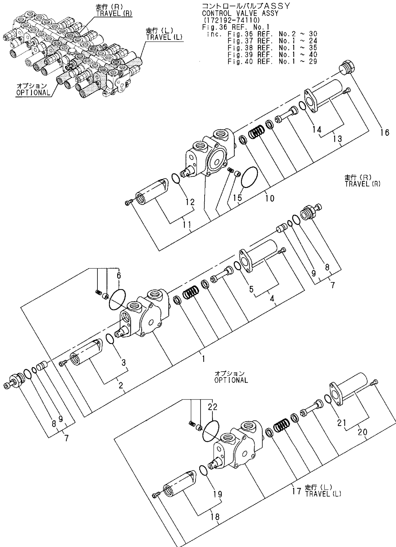
Fig. 37 コントロールバルブ (走行&P.T.O.) CONTROL VALVE (TRAVEL & P.T.O.)
