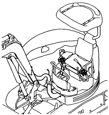
Fig.42 リモコンバルブ (スイング&P. T. O.) REMOTE CONTROL VALVE (SWING & P. T. O.)
