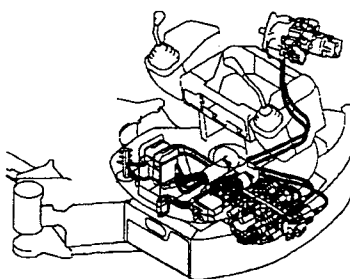
Fig.56 コントロール配管 (走行&スイング) CONTROL PIPING (TRAVEL & SWING)
