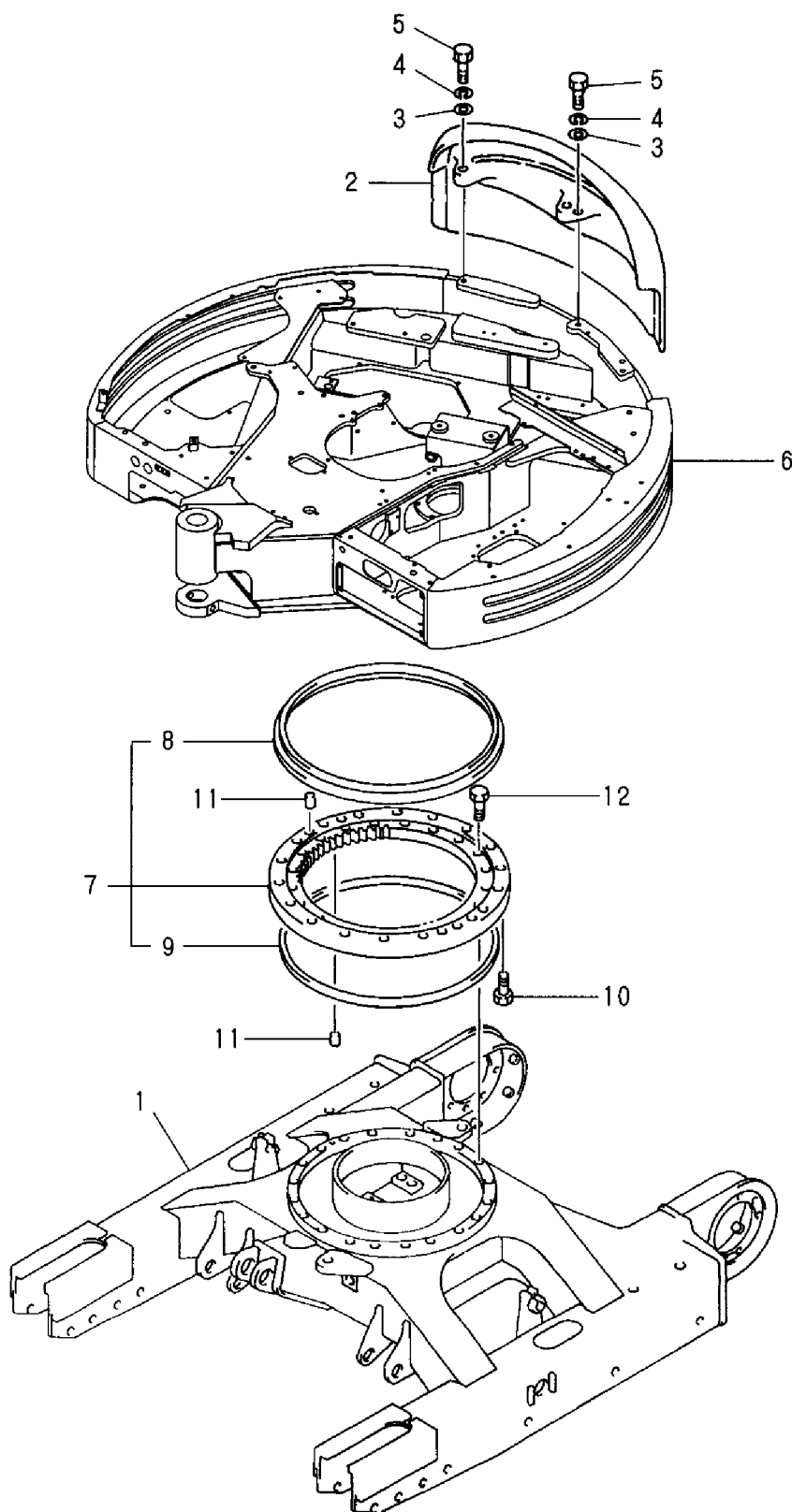
Fig. 19 フレーム & 旋回ベアリング FRAME & TURNING BEARING
