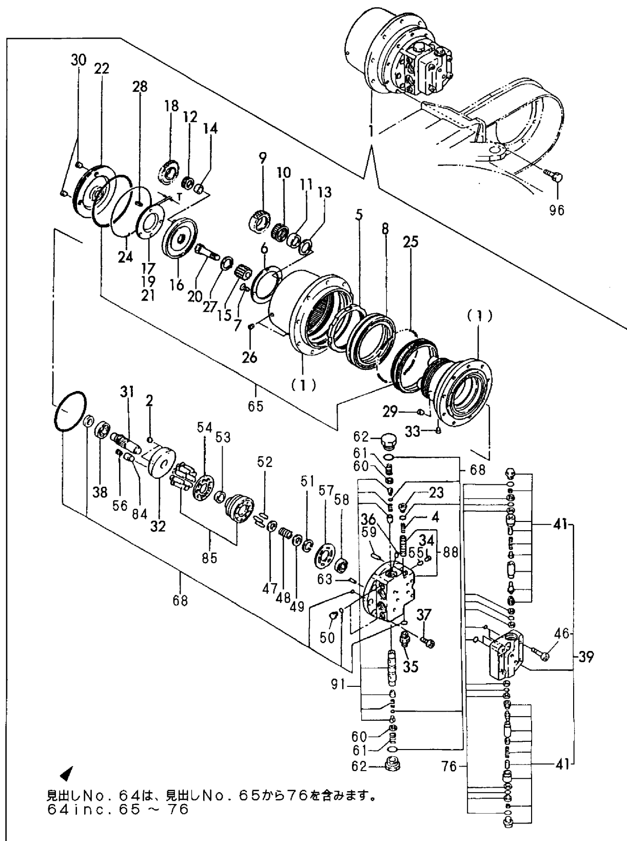
Fig. 33 走行モータ TRAVEL MOTOR
