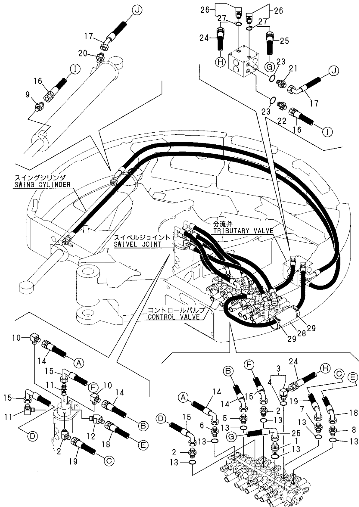
Fig. 49 油圧配管 (バルブ~スイベル、スイング) HYD. OIL PIPING (VALVE~SWIVEL, SWING)
