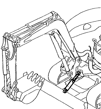
Fig.32 ブレードシリンダ BLADE CYLINDER
