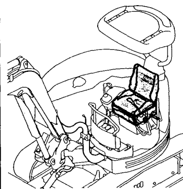
Fig.22 シート&シートマウント SEAT & SEAT MOUNT
