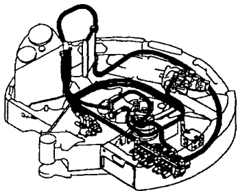
Fig.50 油圧配管 (リターン) HYD.OIL PIPING (RETURN)
