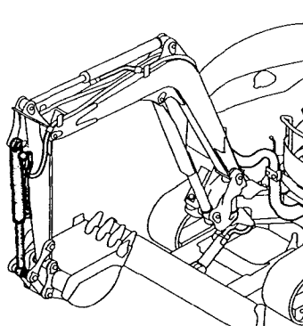
Fig.30 バケットシリンダ BUCKET CYLINDER
