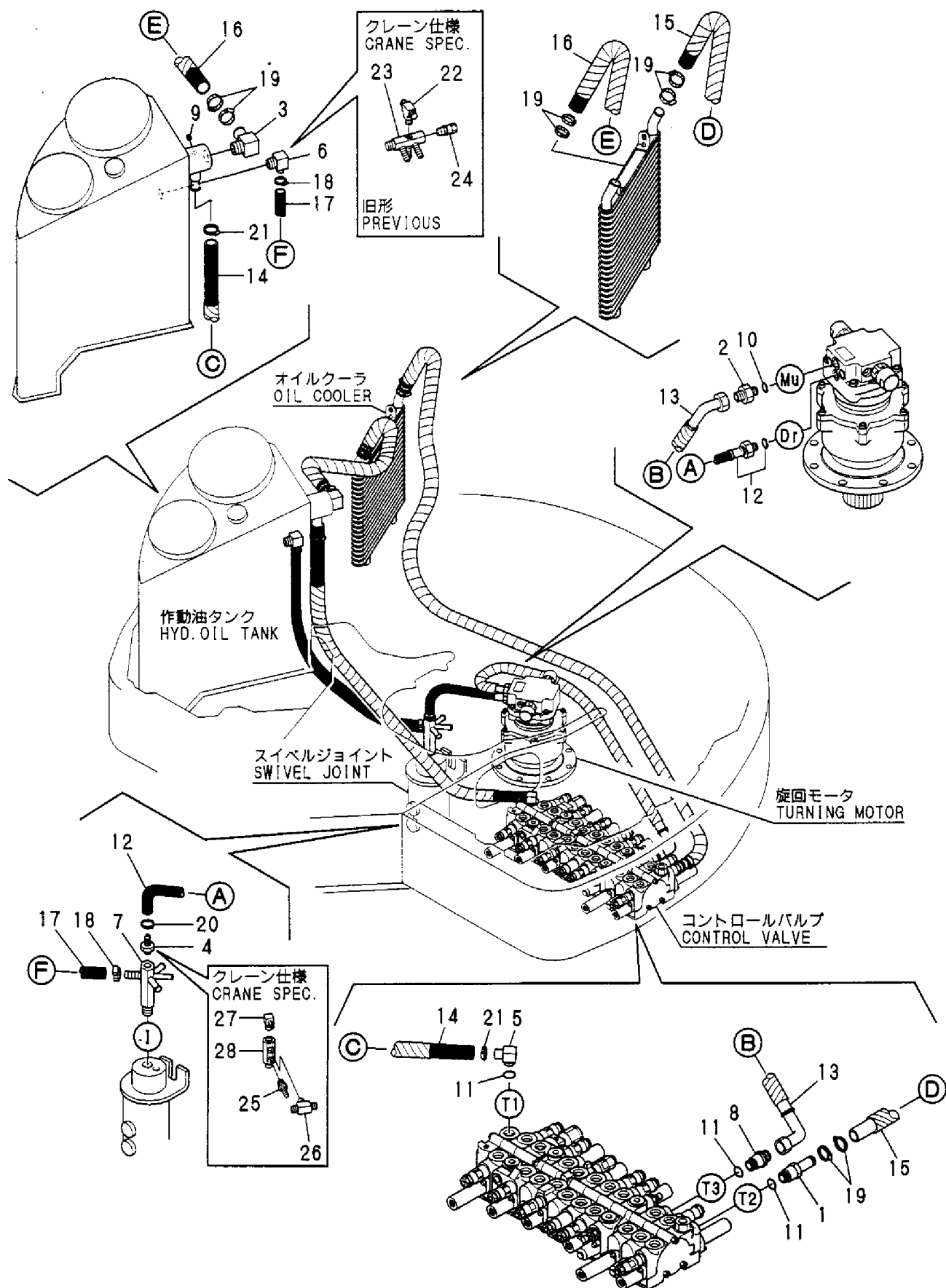
Fig. 72 油圧配管 (リターン: 1) HYD. OIL PIPING (RETURN: 1)
