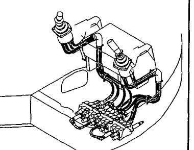
Fig. 84 コントロール配管 (2ウェイマルチチェンジ) CONTROL PIPING (2-WAY MULTI CHANGE)
