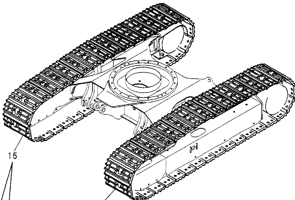
Fig. 26 クローラ CRAWLER
