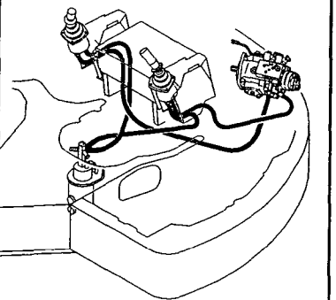
Fig. 83 コントロール配管 (リモコンバルブ ~コントロールバルブ) (AS) CONTROL PIPING (REMO.-CON. V. ~CONTROL. V.) (AS)
