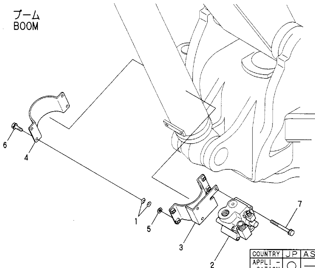
Fig. 67 ホールドバルブ (クレーン仕様) HOLD VALVE (CRANE SPEC.)
