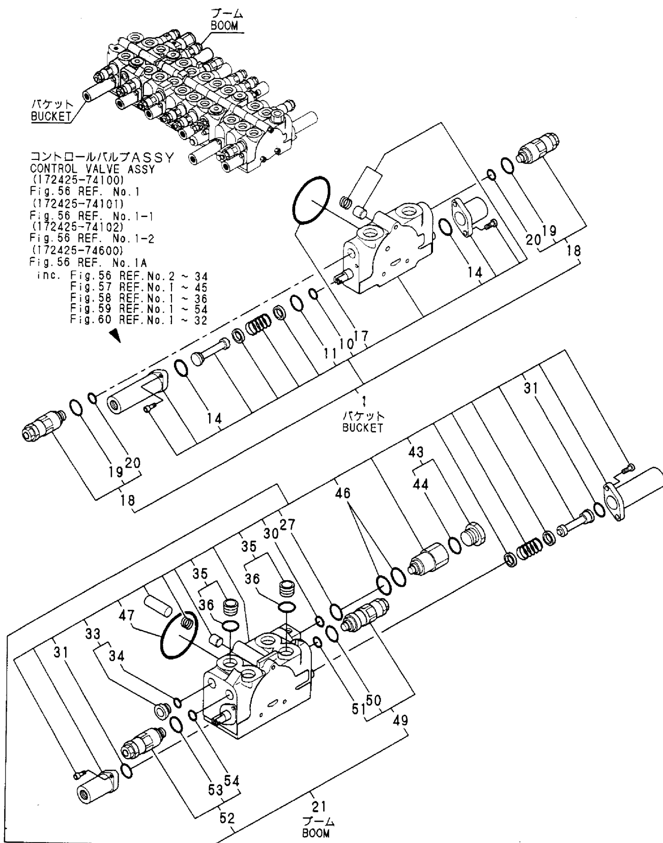
Fig. 59 コントロールバルブ (ブーム&バケット) CONTROL VALVE (BOOM & BUCKET)
