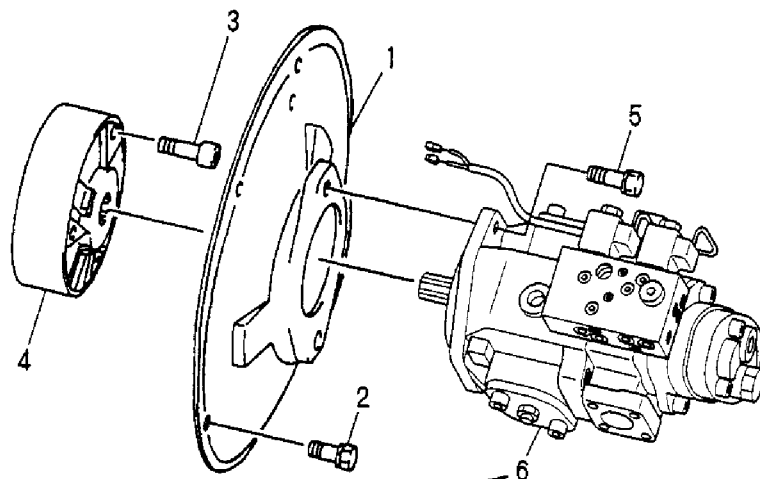
Fig. 46 油圧ポンプ&軸継手 HYD. OIL PUMP & JOINT
