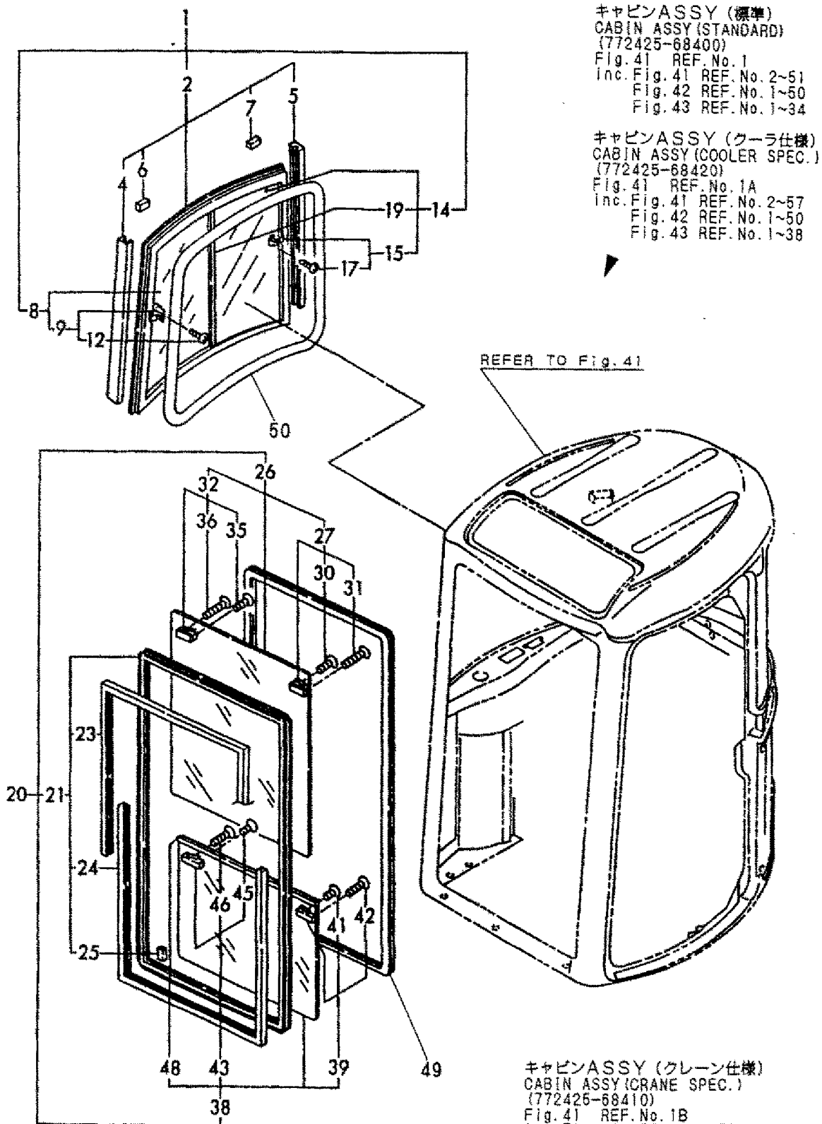
Fig. 42 キャビン (2) (サッシ) CABIN (2) (SASH)
