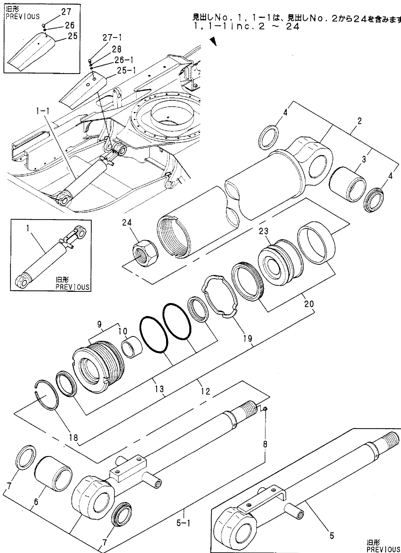
Fig. 52 ブレードシリンダ BLADE CYLINDER
