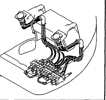
Fig. 80 コントロール配管 (リモコンバルブ ~コントロールバルブ) CONTROL PIPING (REMO.-CON. V. ~CONTROL. V.)
