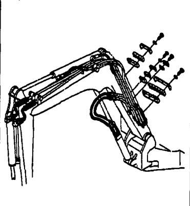
Fig. 76 油圧配管 (ブーム) (クレーン仕様) HYD. OIL PIPING (BOOM) (CRANE SPEC.)
