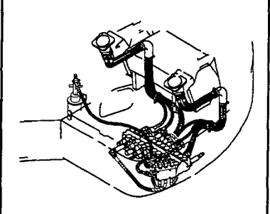
Fig. 82 コントロール配管 (ポンプ~リモコンバルブ ~リターン) (AS) CONTROL PIPING (PUMP~REMO.-CON. V. ~RETURN) (AS)
