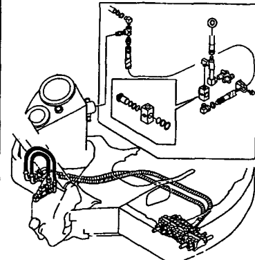
Fig. 78 油圧配管 (PTOアームエンド) HYD. OIL PIPING (P. T. O. ARM END)
