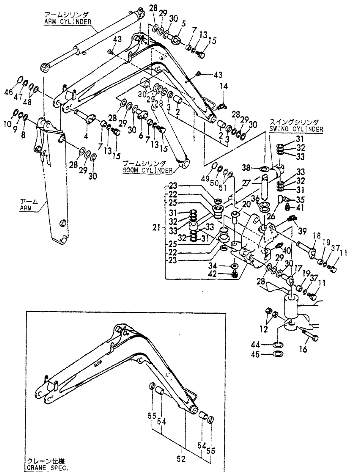
Fig. 91 ブーム&ブームブラケット BOOM & BOOM BRACKET
