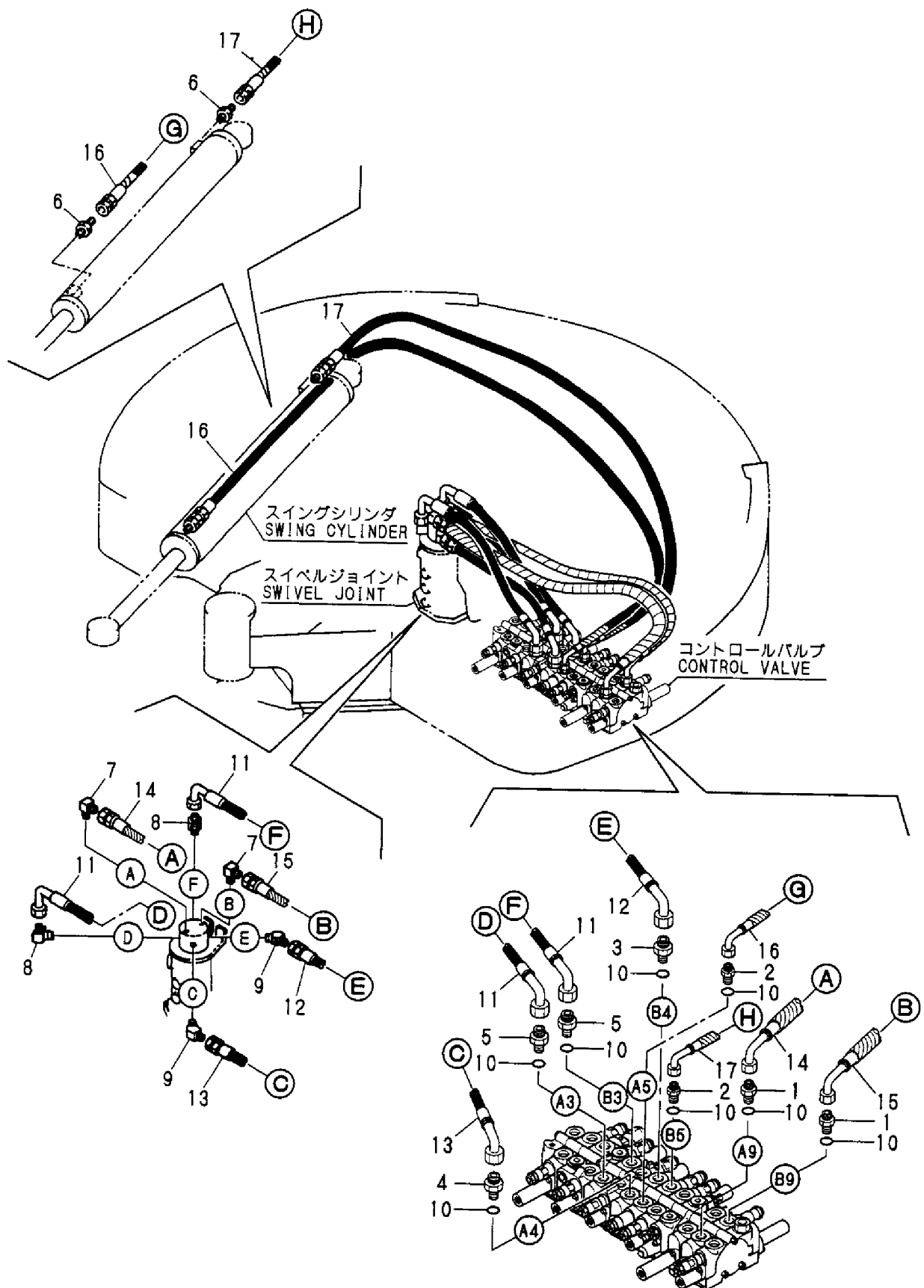
Fig. 71 油圧配管 (バルブ~スィベル、スイング) HYD. OIL PIPING (VALVE~SWIVEL, SWING)
