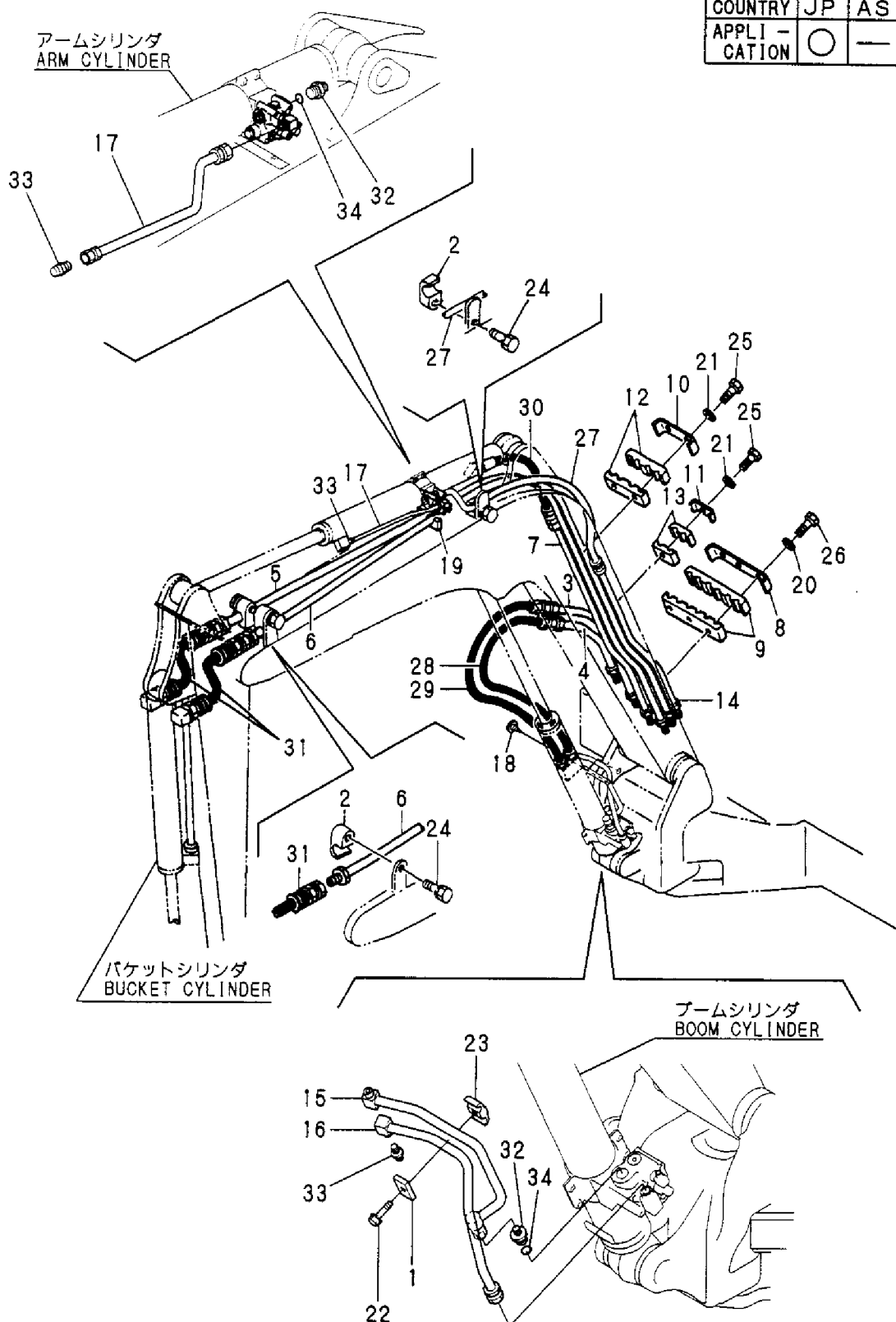
Fig. 76 油圧配管（ブーム）（クレーン仕様） HYD. OIL PIPING (BOOM) (CRANE SPEC.)
