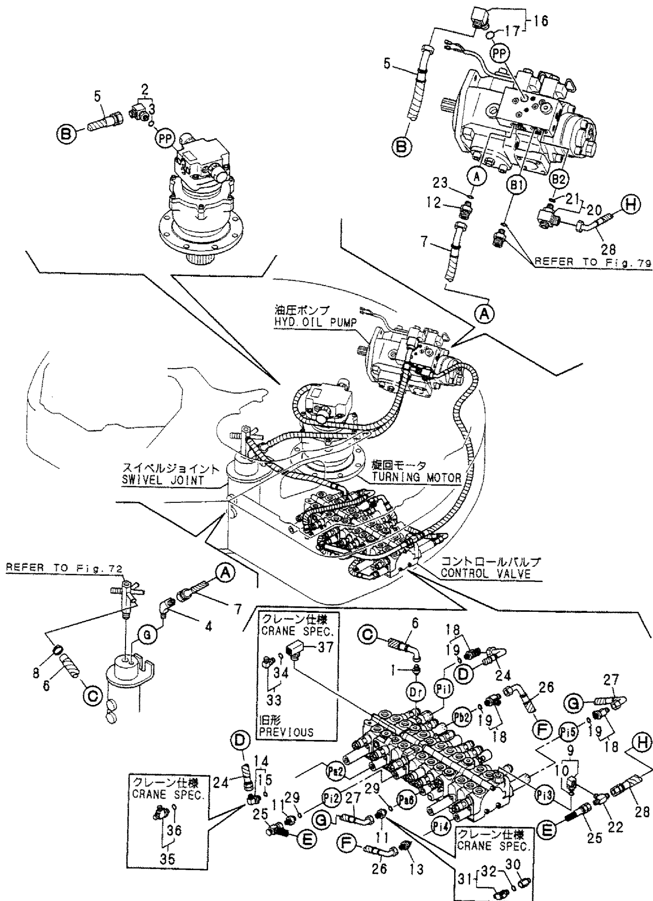
Fig. 73 油圧配管 (リターン: 2) HYD. OIL PIPING (RETURN: 2)
