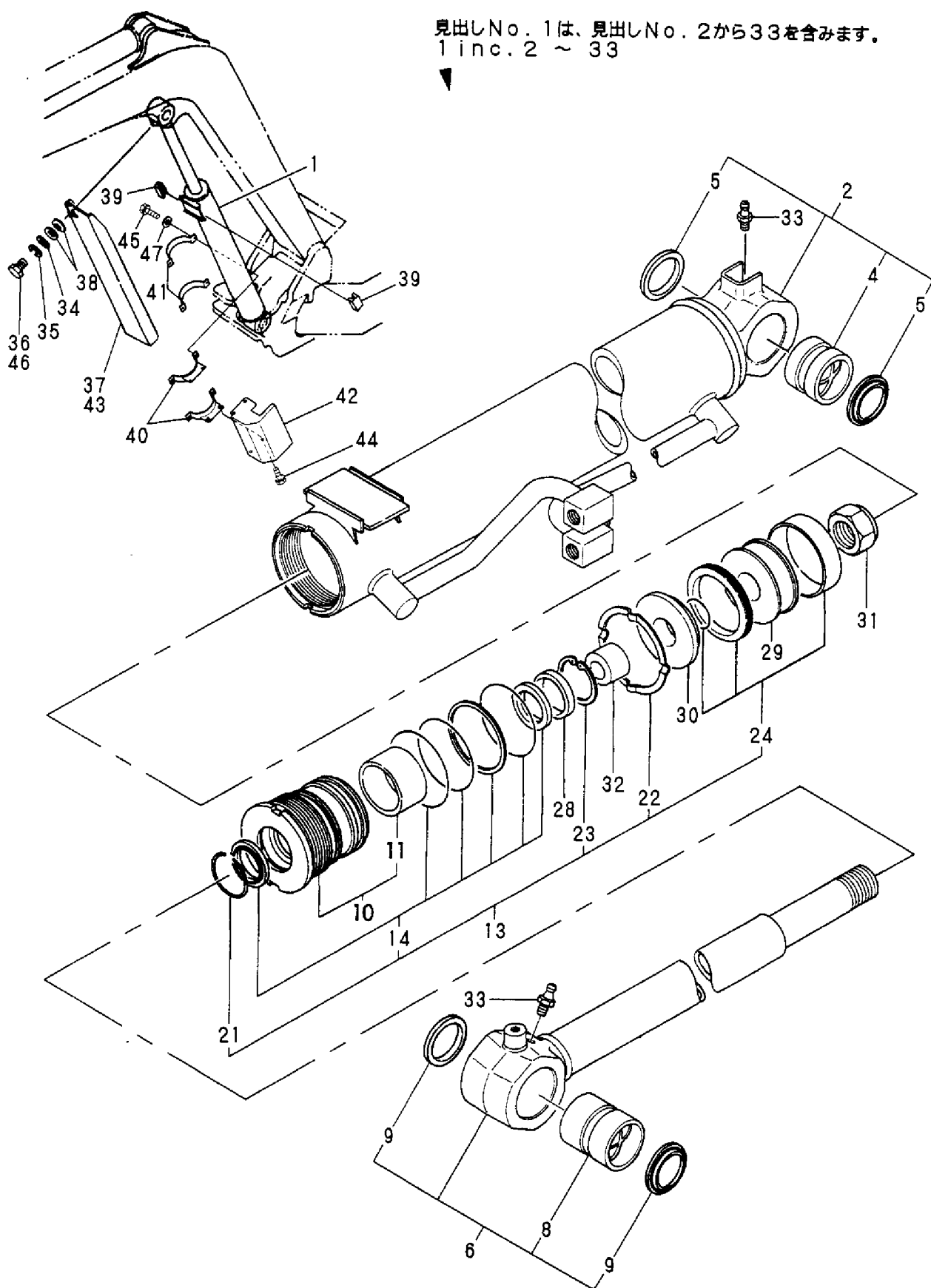
Fig. 48 ブームシリンダ (キャノピ) BOOM CYLINDER (CANOPY)
