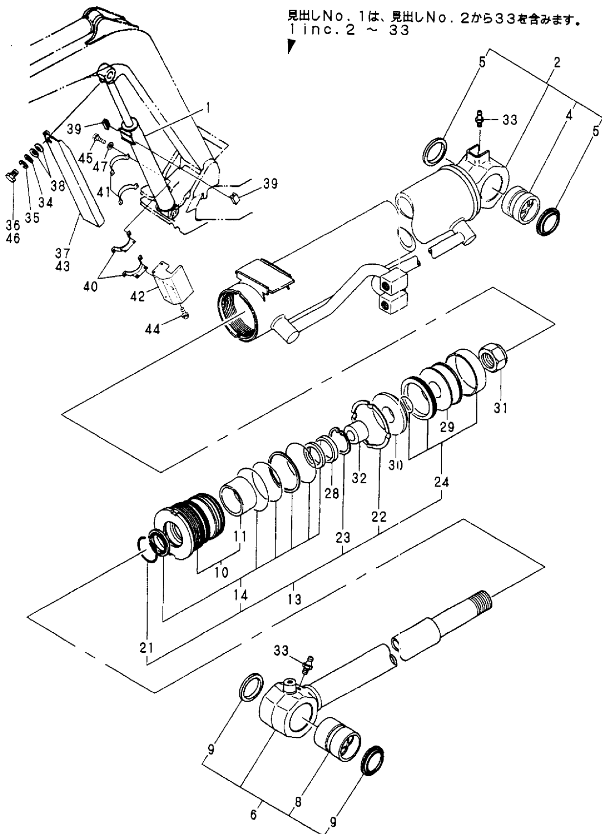
Fig. 47 ブームシリンダ (キャビン) BOOM CYLINDER (CABIN)
