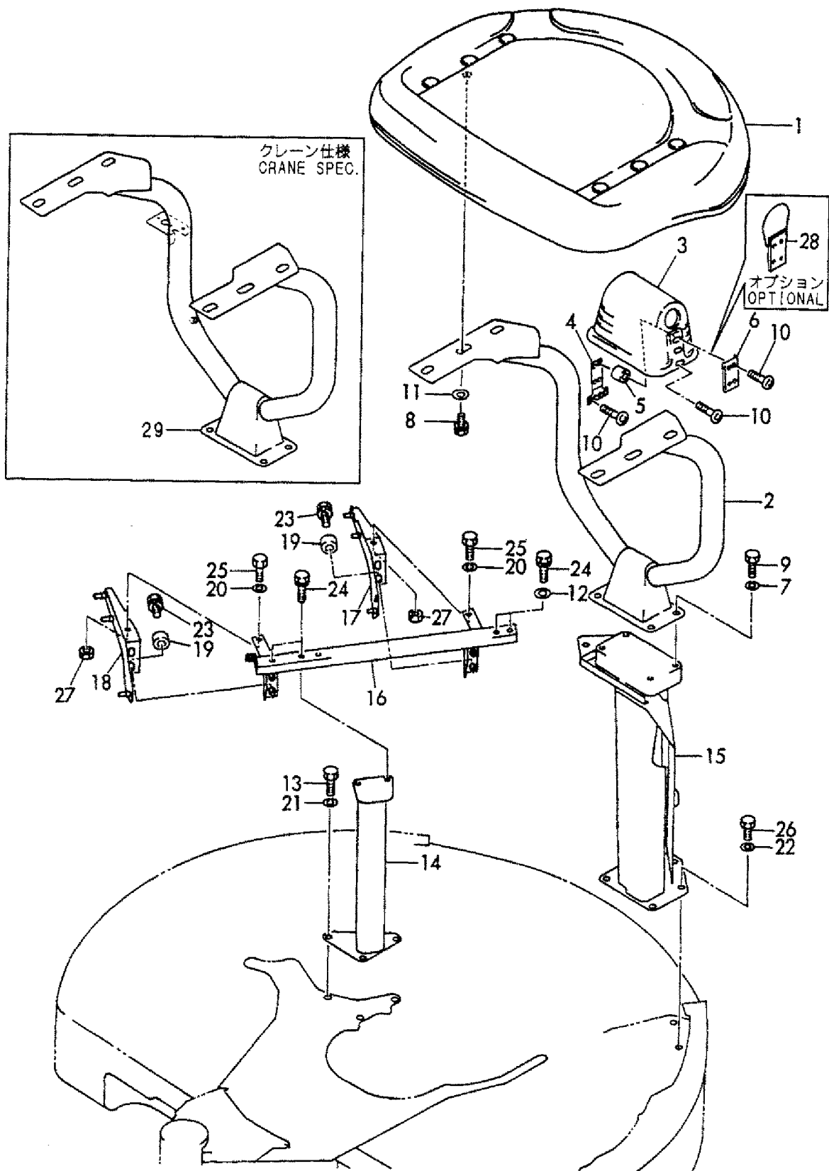
Fig. 45 キャノピ&キャノピフレーム CANOPY & CANOPY FRAME
