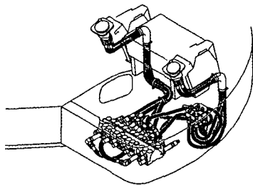
Fig. 86 コントロール配管 (4ウェイマルチチェンジ: 1) CONTROL PIPING (4 WAY MULTI CHANGE: 1)
