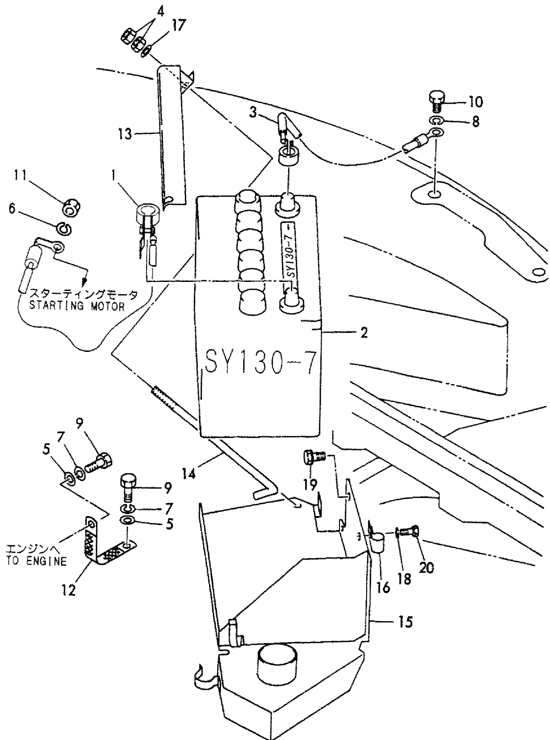
Fig. 13 バッテリ BATTERY
