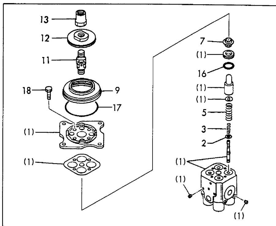
Fig. 61 リモコンバルブ REMOTE CONTROL VALVE
