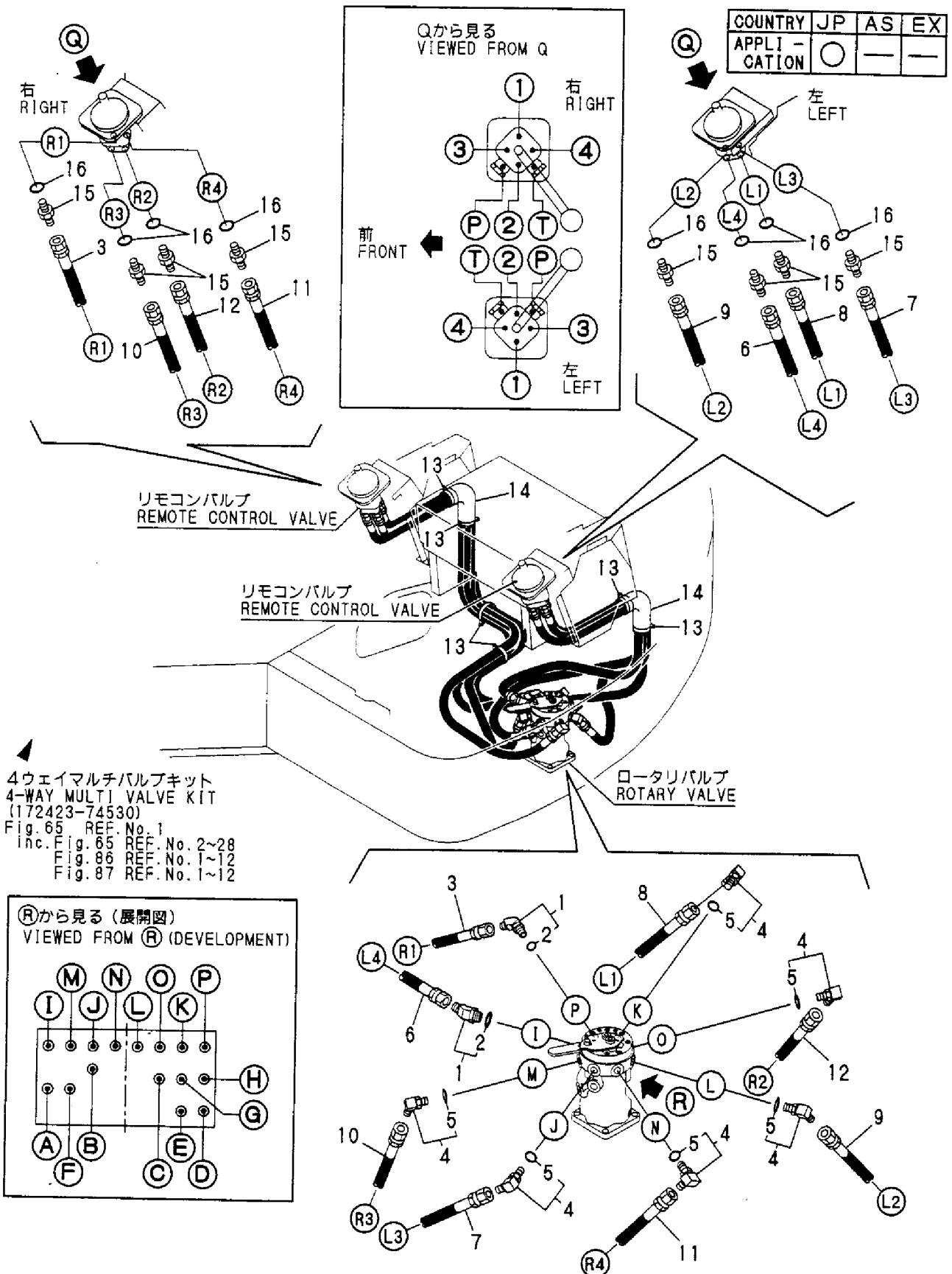
Fig. 86 コントロール配管 (4ウェイマルチチェンジ: 1) CONTROL PIPING (4-WAY MULTI CHANGE: 1)
