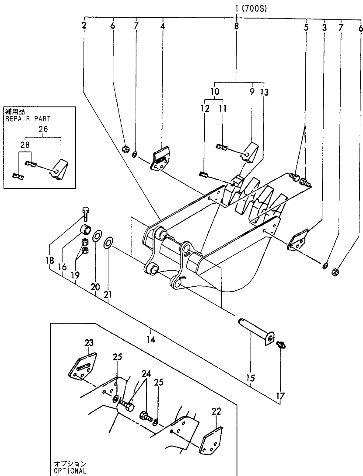
Fig. 93 バケットSタイプ BUCKET S TYPE
