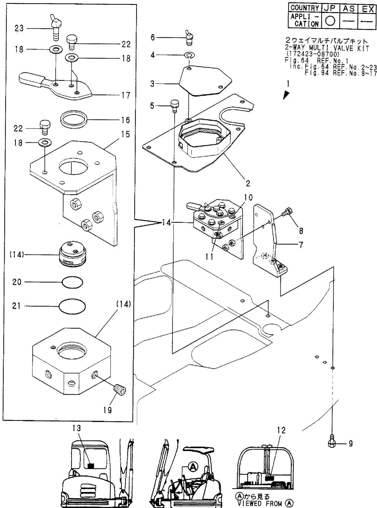
Fig. 64 2ウェイバルブ (2ウェイマルチチェンジ) 2-WAY VALVE (2-WAY MULTI CHANGE)
