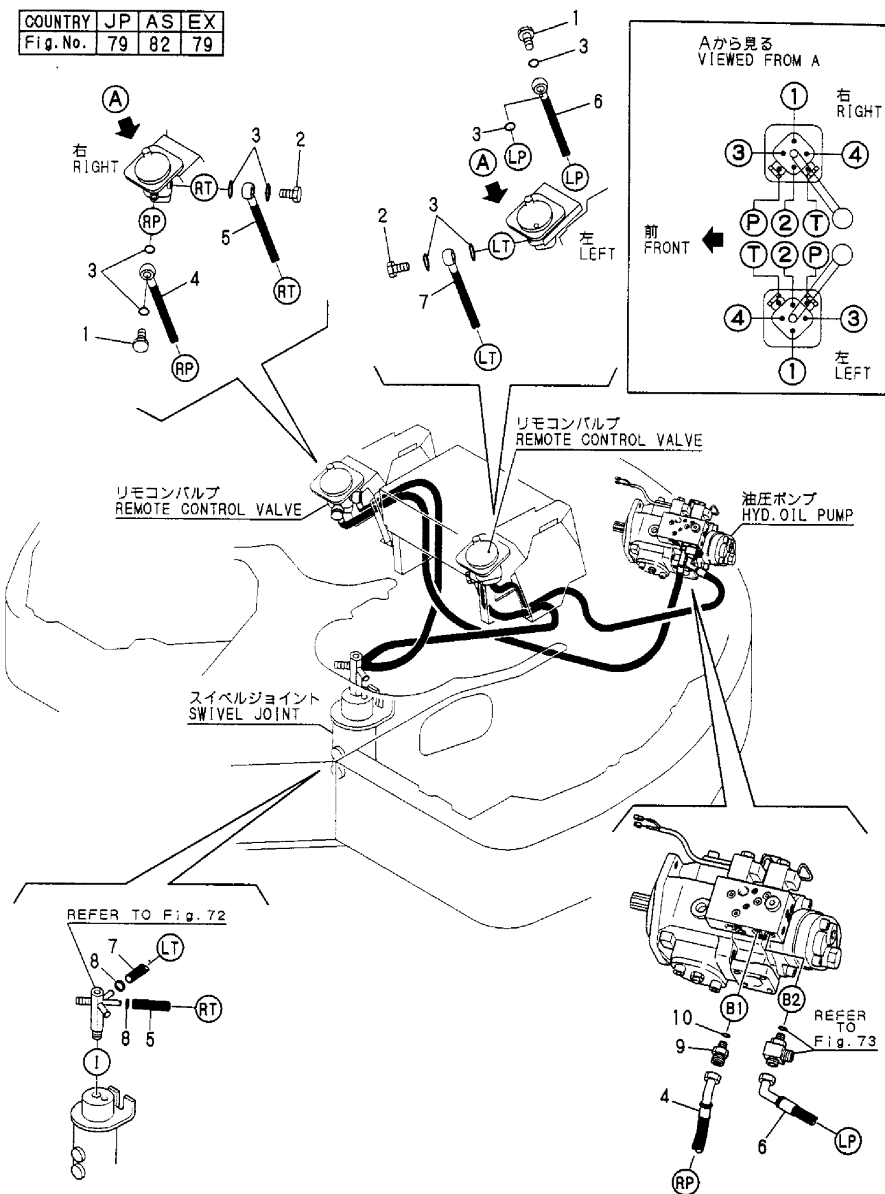
Fig. 79 コントロール配管 (ポンプ~リモコンバルブ~リターン) CONTROL PIPING (PUMP~REMO. -CON. V.~RETURN)
