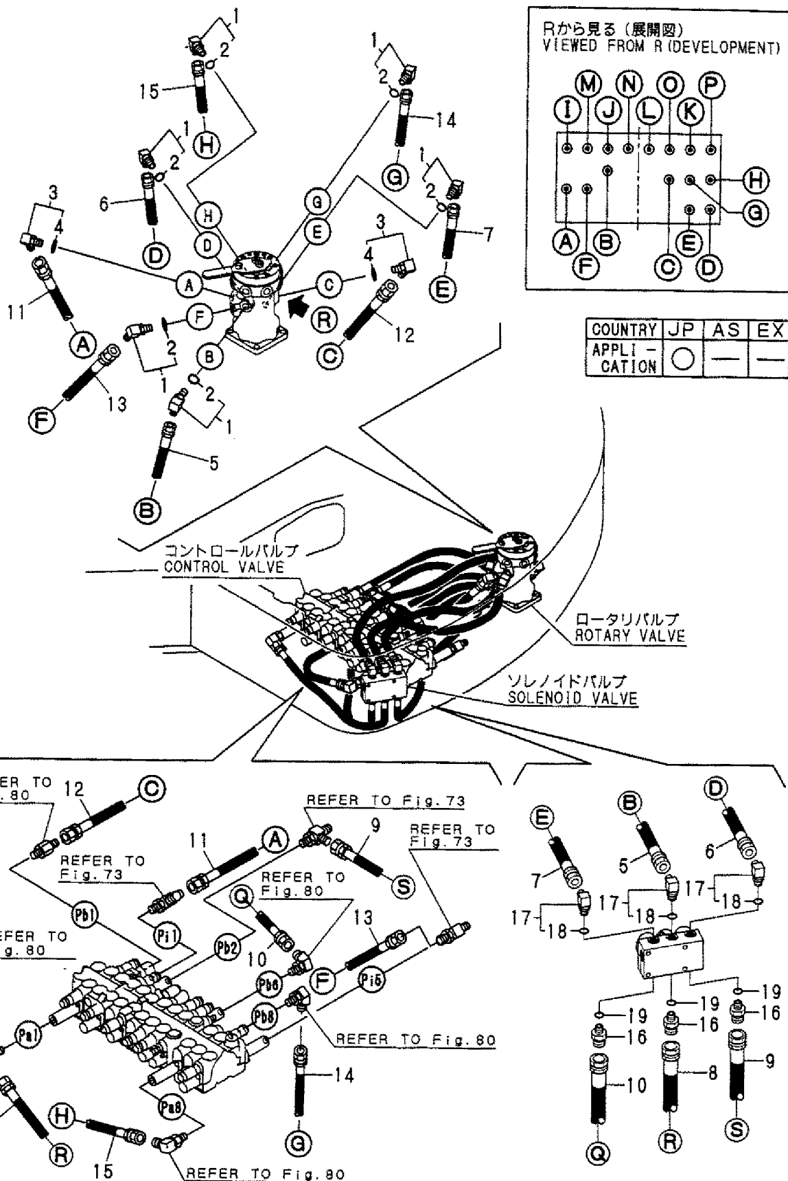
Fig. 88 コントロール配管 (4ウェイマルチチェンジ: 2) (クレーン仕様) CONTROL PIPING (4-WAY MULTI CHANGE: 2) (CRANE SPEC.)
