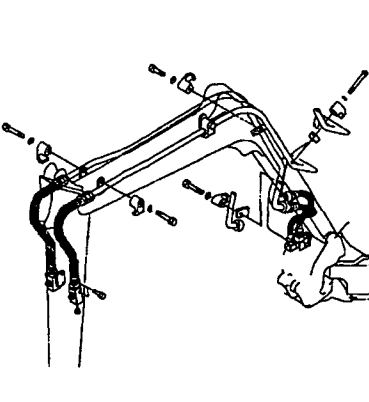
Fig. 79 コントロール配管 (ポンプ ~リモコンバルブ~リターン) CONTROL PIPING (PUMP~REMO.-CON. V. ~RETURN)
