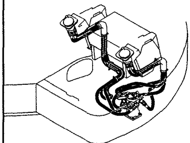
Fig. 87 コントロール配管 (4ウェイマルチチェンジ: 2) CONTROL PIPING (4 WAY MULTI CHANGE: 2)
