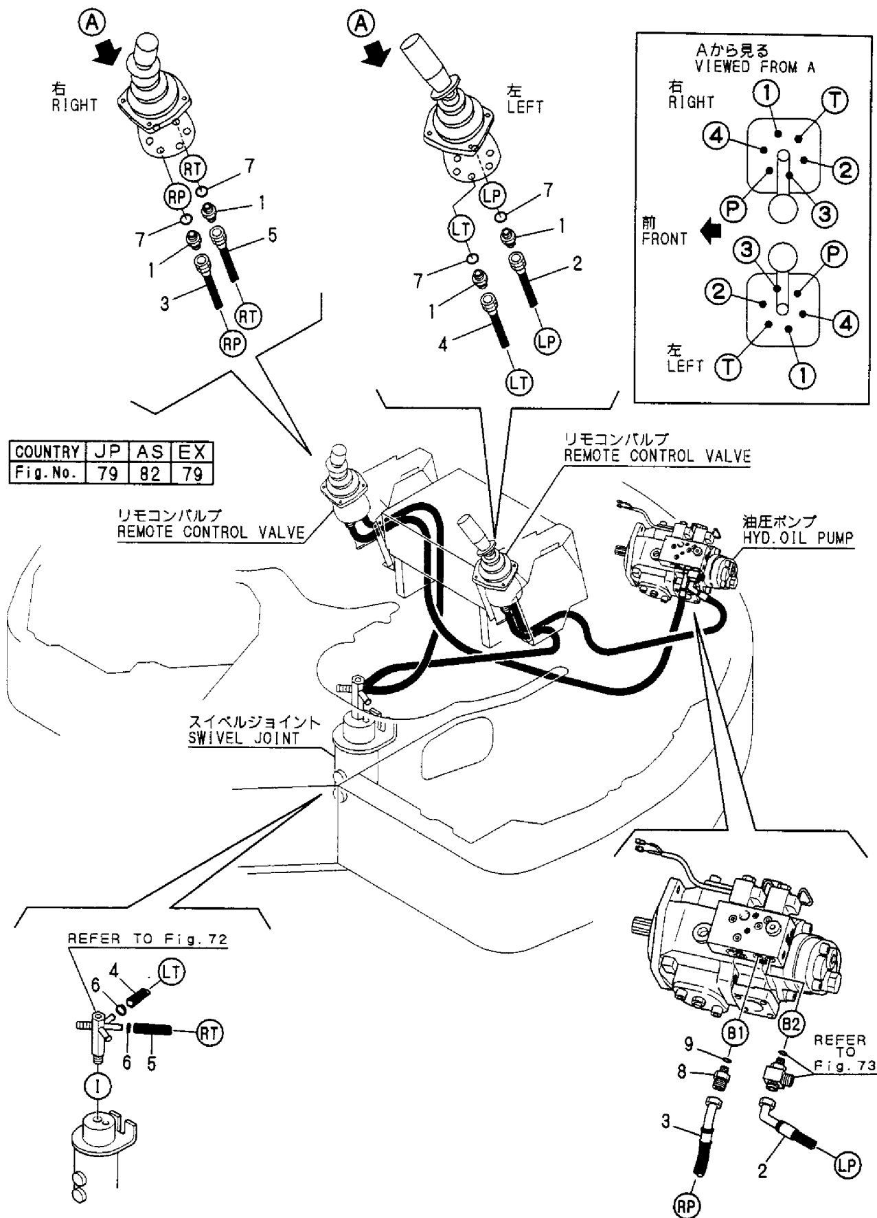
Fig. 82 コントロール配管 (ポンプ~リモコンバルブ~リターン) (AS) CONTROL PIPING (PUMP~REMO. -CON. V. ~RETURN) (AS)
