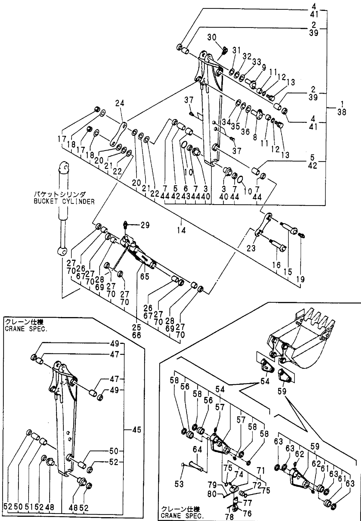
Fig. 92 アーム&バケットリンク ARM & BUCKET LINK
