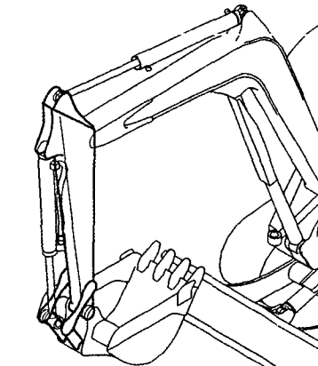
Fig. 92 アーム&バケットリンク ARM & BUCKET LINK
