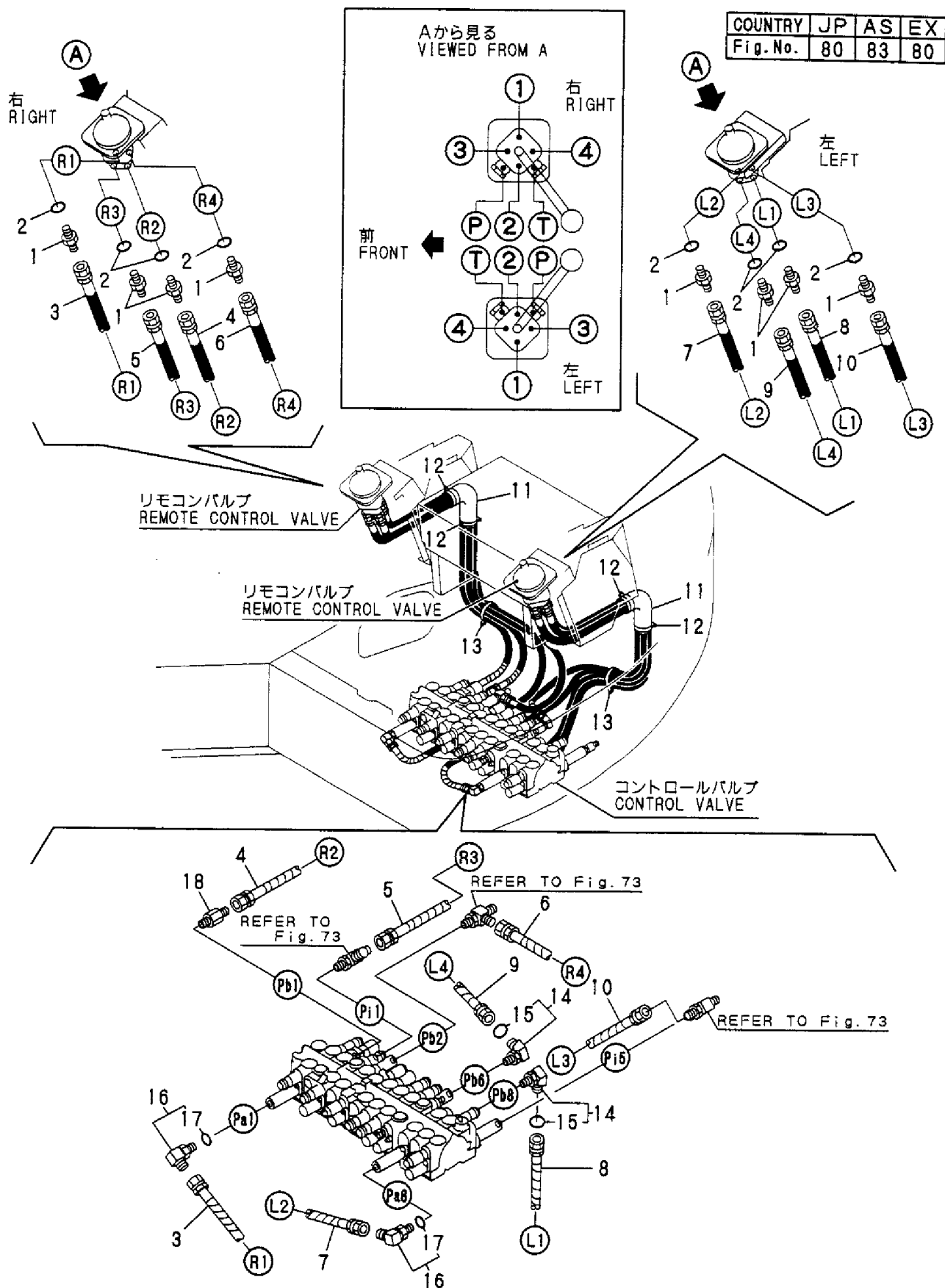
Fig. 80 コントロール配管 (リモコンバルブ~コントロールバルブ) CONTROL PIPING (REMO.-CON. V. ~CONTROL. V.)
