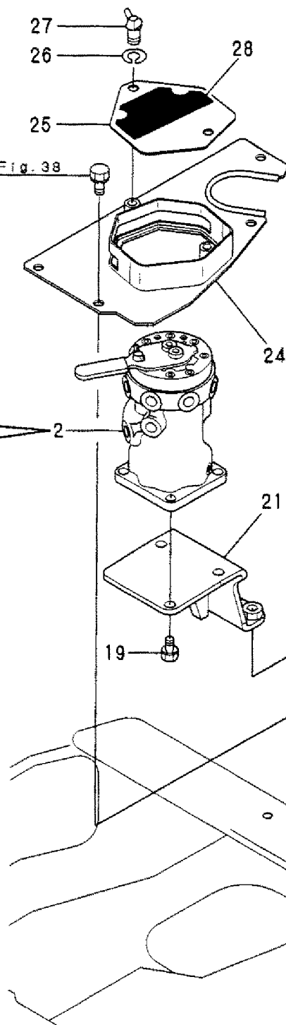
Fig. 65 ロータリバルブ (4ウェイマルチチェンジ) ROTARY VALVE (4-WAY MULTI CHANGE)
