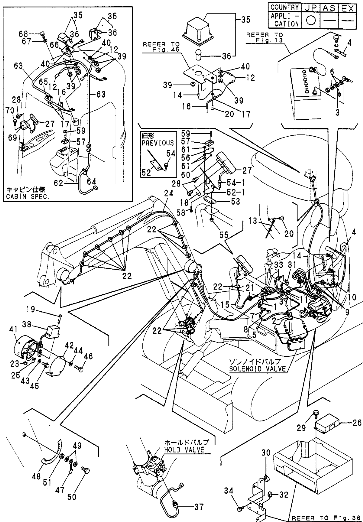
Fig. 17 電装品 (クレーン仕様) ELECTRIC PART (CRANE SPEC.)
