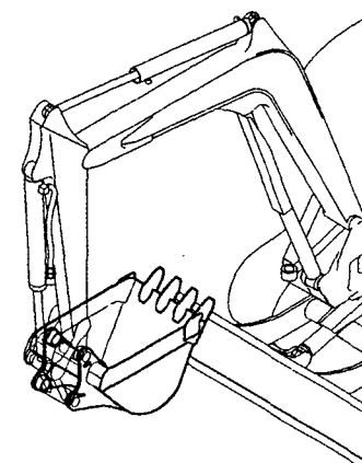
Fig. 94 バケットSタイプ (アタッチメント) BUCKET S TYPE (ATTACHMENT)
