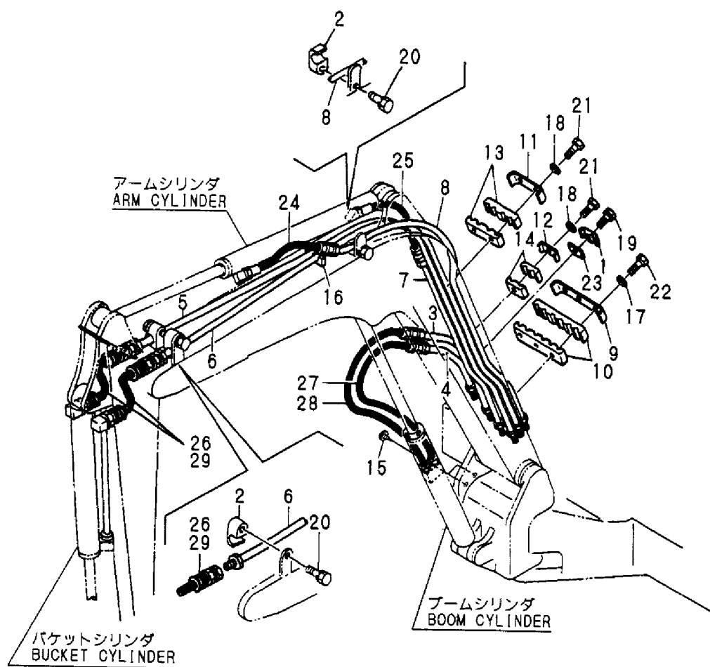
Fig. 75 油圧配管 (ブーム) HYD. OIL PIPING (BOOM)
