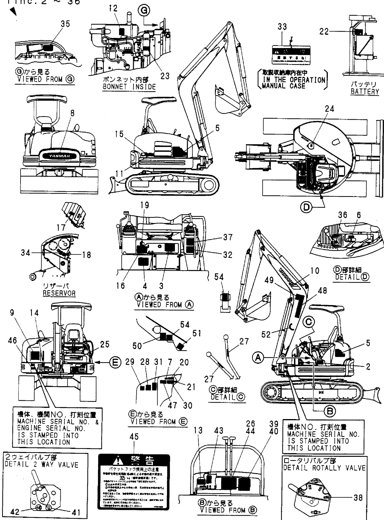
Fig. 3 銘板 (キャノピ) (JP) LABEL (CANOPY) (JP)
