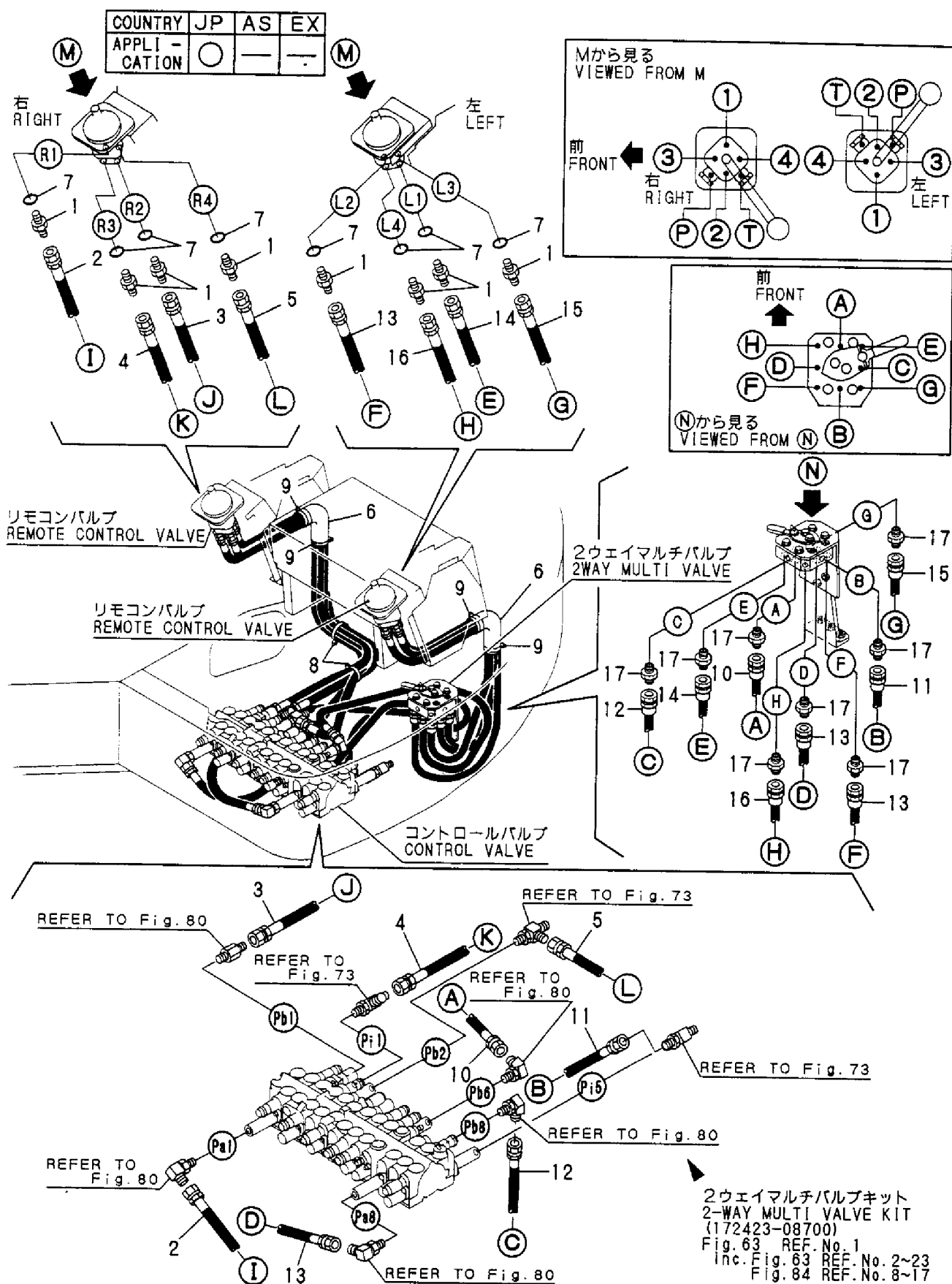
Fig. 84 コントロール配管 (2ウェイマルチチェンジ) CONTROL PIPING (2-WAY MULTI CHANGE)
