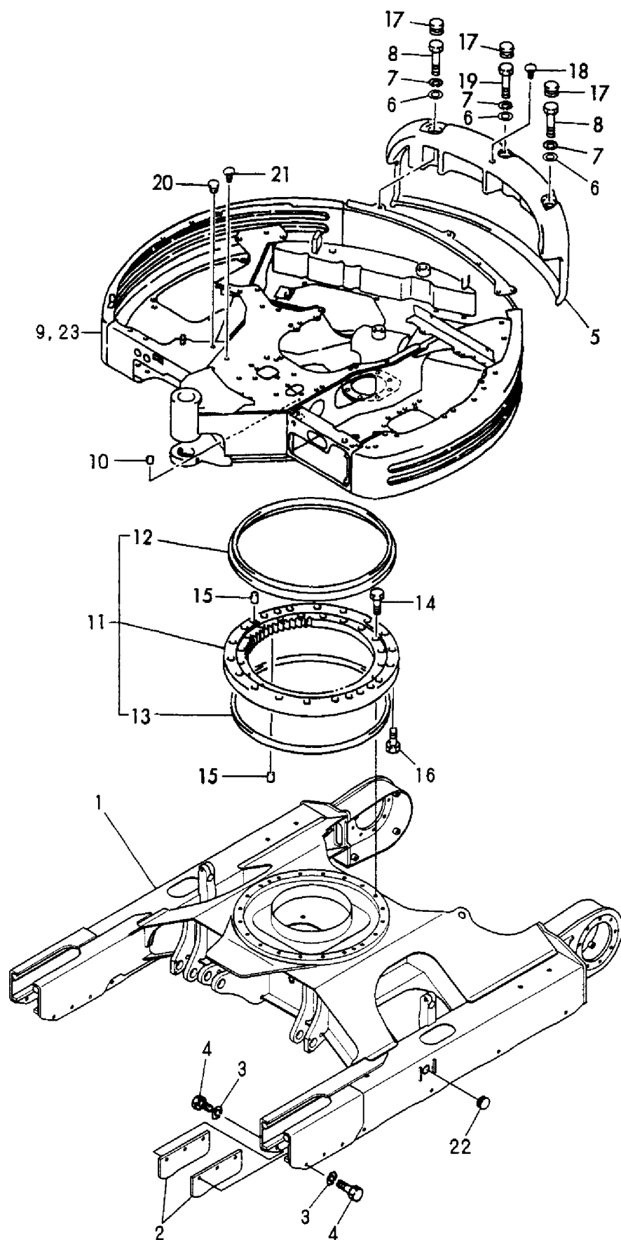
Fig. 34 フレーム&旋回ベアリング FRAME & TURNING BEARING
