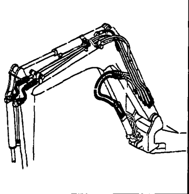
Fig. 76 油圧配管 (ブーム) (クレーン仕様) HYD. OIL PIPING (BOOM) (CRANE SPEC.)
