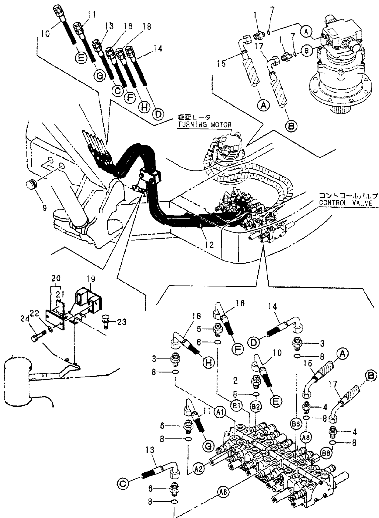
Fig. 70 油圧配管 (バルブ~モータ、ブーム) HYD. OIL PIPING (VALVE~MOTOR, BOOM)
