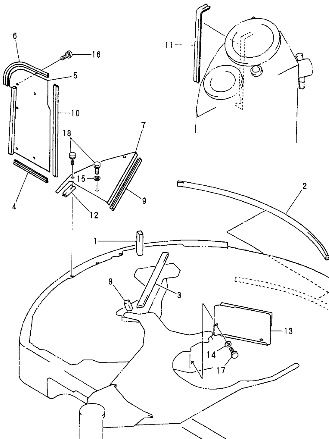
Fig. 40 ダクト DUCT
