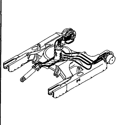
Fig. 75 油圧配管 (ブーム) HYD. OIL PIPING (BOOM)
