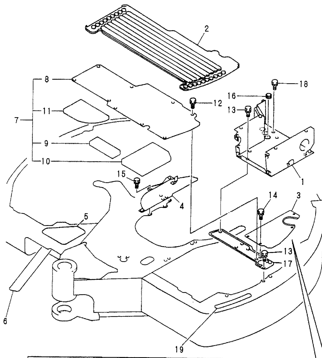
Fig. 38 ステップ STEP
