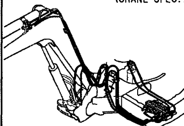
Fig. 89 コントロール配管 (ホールドバルブ) (クレーン仕様) CONTROL PIPING (HOLD VALVE) (CRANE SPEC.)
