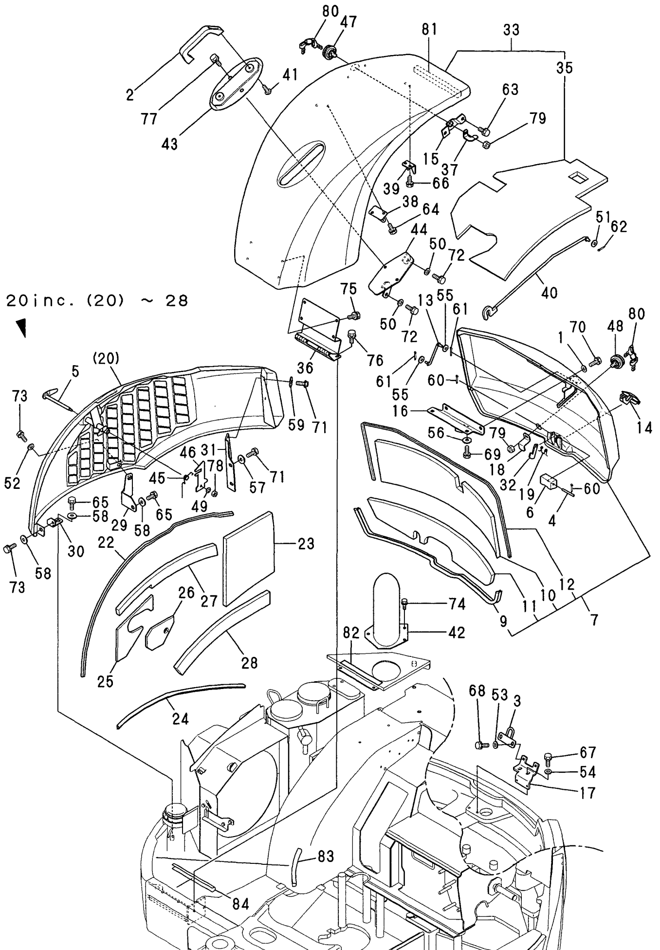
Fig. 26 BONNET
