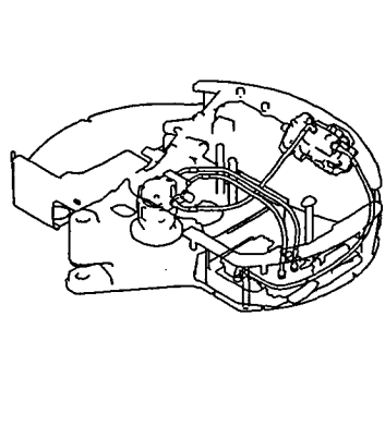
Fig. 46 HYD.OIL PIPING (VALVE~SWIVEL~SWING)
