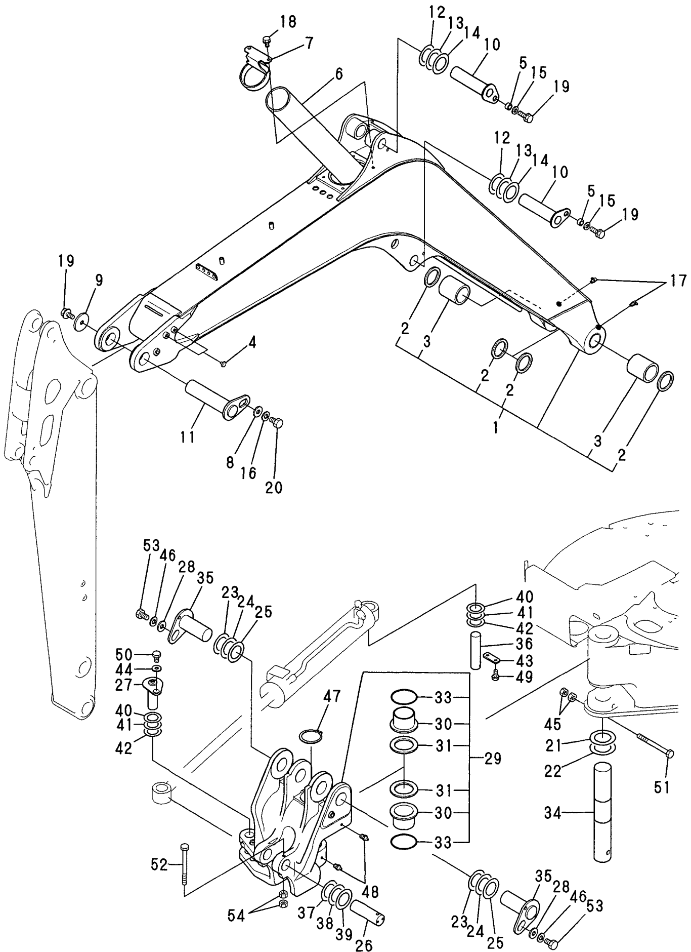
Fig. 54 BOOM & BOOM BRACKET
