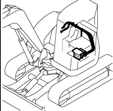
Fig. 32 ヒータ HEATER
