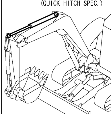
Fig. 72 アームシリンダ (クイックヒッチ仕様) ARM CYLINDER (QUICK HITCH SPEC.)
