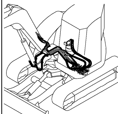
Fig. 96 油圧配管 (バルブ〜旋回モータ, ブーム) HYD. OIL PIPING (VALVE - TURNING MOTOR, BOOM)
