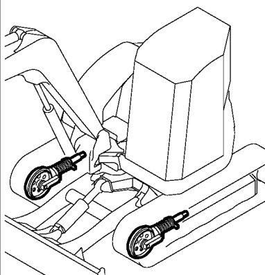
Fig. 40 クローラ CRAWLER
