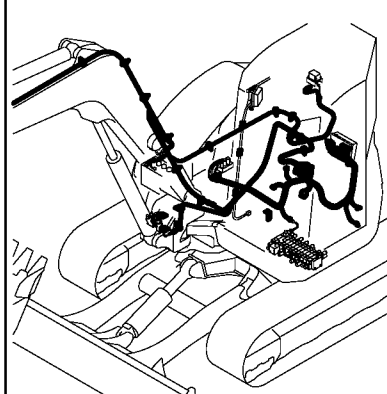
Fig. 24 電装品 (ワイリング : クレーン仕様) ELECTRIC PART (WIRING : CRANE SPEC.)
