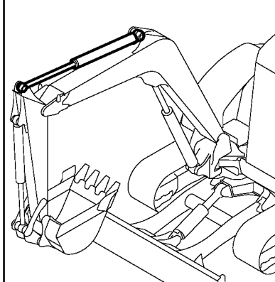
Fig. 72 アームシリンダ (クイックヒッチ仕様) ARM CYLINDER (QUICK HITCH SPEC.)
