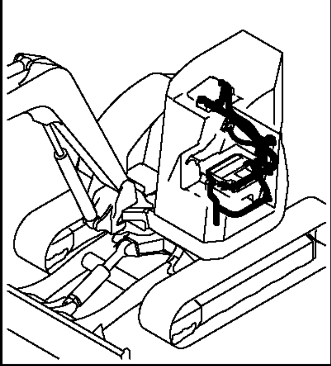
エアコン (配管) Fig. 37 AIR CONDITIONER (PIPING)
