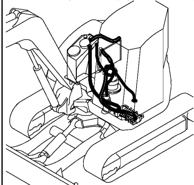
Fig. 100 油圧配管 (リターン:1) (クレーン仕様) HYD. OIL PIPING (RETURN:1) (CRANE SPEC.)
