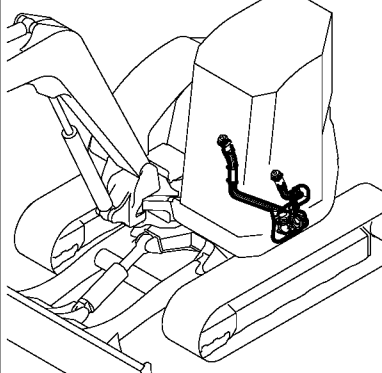
Fig. 112 コントロール配管 (リモコンバルブ〜4ウェイバルブ) CONTROL PIPING (REMOTE CONTROL V. - 4-WAY V.)
