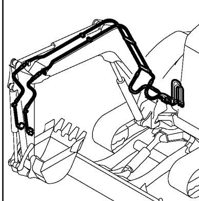
Fig. 108 油圧配管 (クイックヒッチ) HYD. OIL PIPING (QUICK HITCH)
