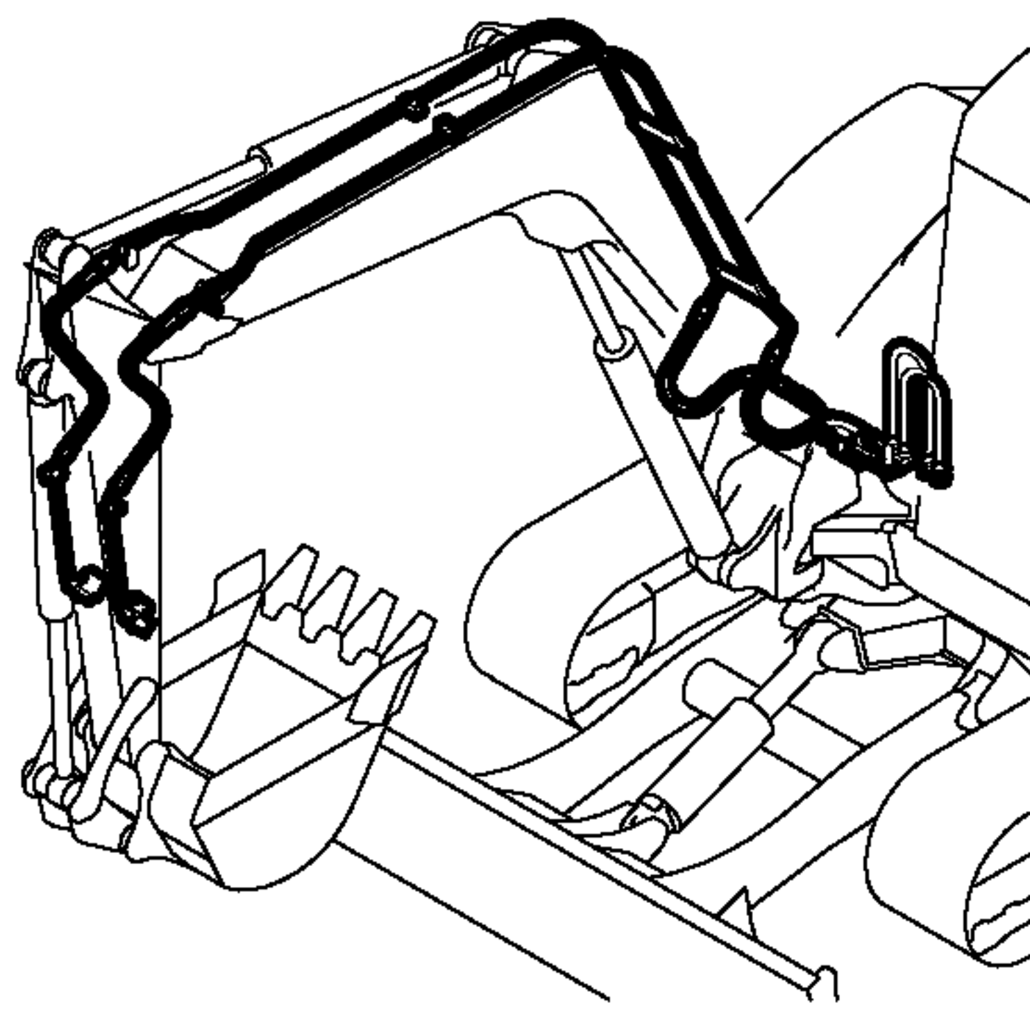
Fig. 107 油圧配管 (PTO; アームエンド) HYD. OIL PIPING (P. T. O. ; ARM END)
