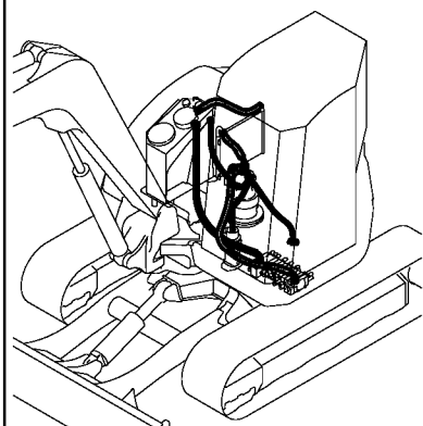
Fig. 100 油圧配管 (リターン:1) (クレーン仕様) HYD. OIL PIPING (RETURN:1) (CRANE SPEC.)
