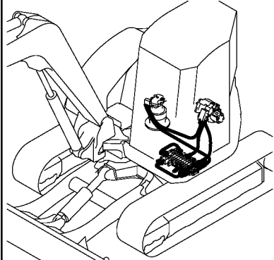
Fig. 103 油圧配管 (PTO:フレームエンド) HYD. OIL PIPING (P. T. O. :FRAME END)
