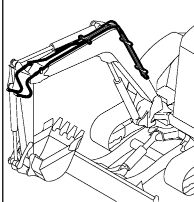
Fig. 106 油圧配管 (ブーム:クレーン仕様) HYD. OIL PIPING (BOOM:CRANE SPEC.)
