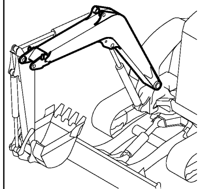
Fig. 119 ブーム(クレーン仕様) BOOM (CRANE SPEC.)
