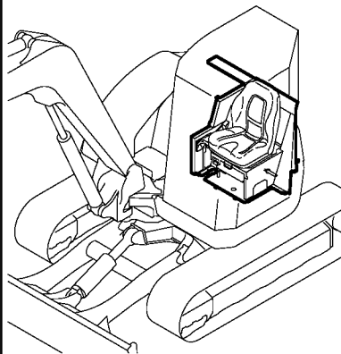
Fig. 55 シート & シートマウント (エアコン仕様) SEAT & SEAT MOUNT (A/C SPEC.)
