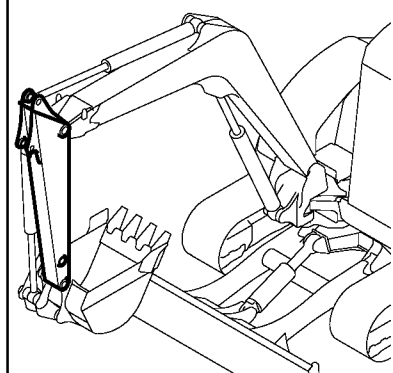
Fig. 120 アーム ARM
