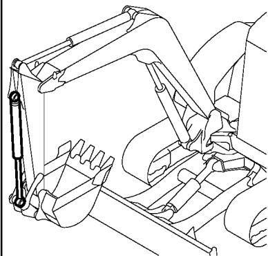
Fig. 74 バケットシリンダ (クイックヒッチ仕様) BUCKET CYLINDER (QUICK HITCH SPEC.)
