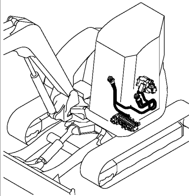
Fig. 110 コントロール配管(リモコン バルブ〜コントロールバルブ) CONTROL PIPING (REMOTE CONTROL V. - CONTROL V.)
