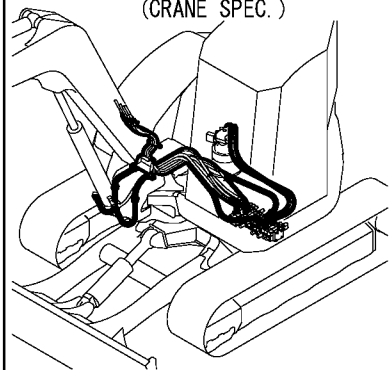
Fig. 98 油圧配管 (ポンプ, バルブ ~ スイベル, スイング) (クレーン仕様) HYD. OIL PIPING (PUMP, VALVE - SWIVEL, SWING) (CRANE SPEC.)
