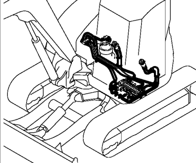
Fig. 112 コントロール配管 (リモコンバルブ〜4ウェイバルブ) CONTROL PIPING (REMOTE CONTROL V. - 4-WAY V.)
