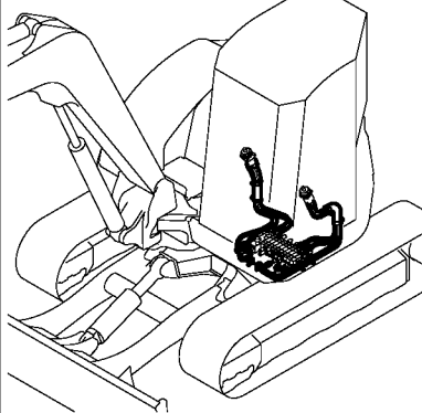
Fig. 111 コントロール配管(リモコン バルブ〜コントロールバルブ) (クレーン仕様) CONTROL PIPING (REMOTE CONTROL V. - CONTROL V.) (CRANE SPEC.)
