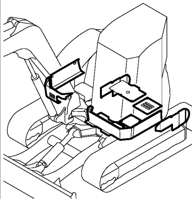
Fig. 51 カバー(操縦廻り:1) COVER (AROUND THE CONTROL:1)
