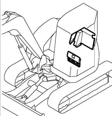
Fig. 52 カバー(操縦廻り:2) COVER (AROUND THE CONTROL:2)
