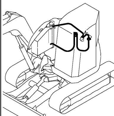
Fig. 20 燃料パイプ FUEL LINE
