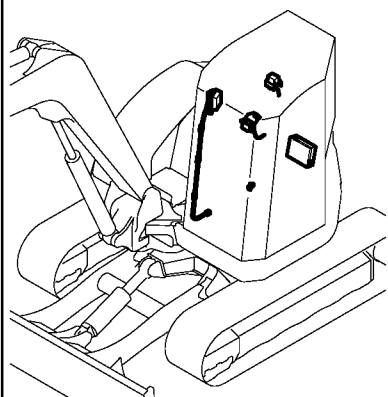
Fig. 28 電装品 (クレーン専用:2) ELECTRIC PART (CRANE:2)
