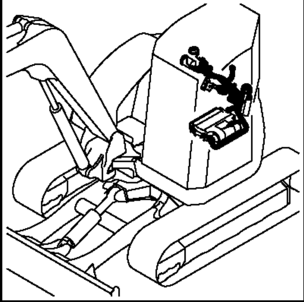
電装品 (ワイリング :エアコン仕様) Fig. 23 ELECTRIC PART (WIRING: A/C SPEC.)
