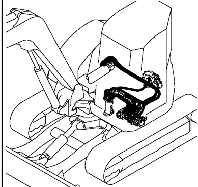
Fig. 99 油圧配管 (リターン:1) HYD. OIL PIPING (RETURN:1)
