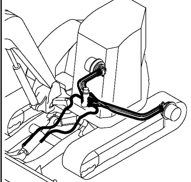
Fig. 104 油圧配管 (トラックフレーム) HYD. OIL PIPING (TRACK FRAME)
