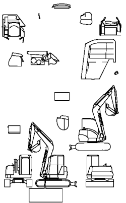
Fig. 3 銘板(キャノピー:JP) LABEL (CANOPY:JP)
