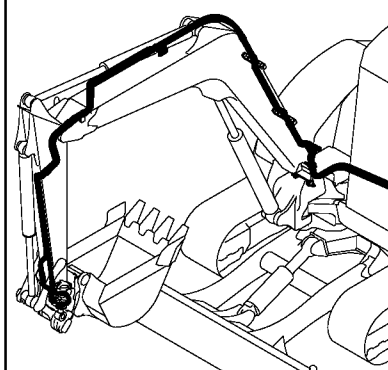
Fig. 108 油圧配管 (クイックヒッチ) HYD. OIL PIPING (QUICK HITCH)
