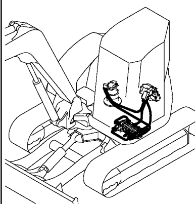
Fig. 102 油圧配管 (リターン:2) (クレーン仕様) HYD. OIL PIPING (RETURN:2) (CRANE SPEC.)
