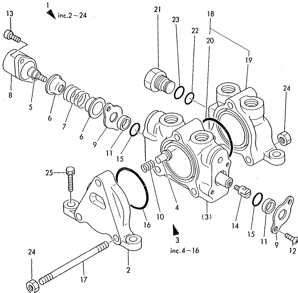
Fig. 76 コントロールバルブ(サード)(オプション) CONTROL VALVE (3RD) (OPTIONAL)
