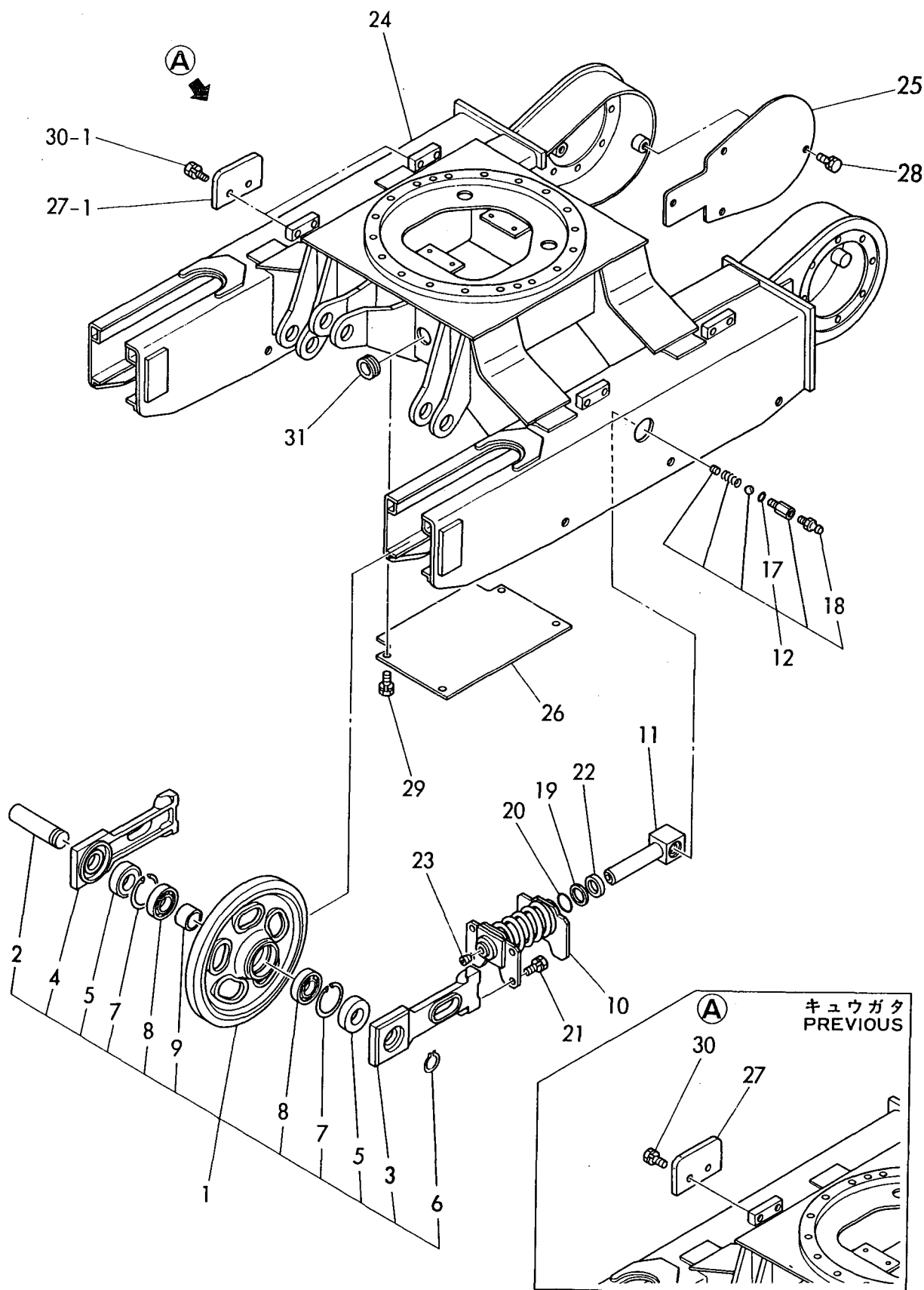
Fig. 16 トラックフレーム&アイドラ https://trackmanualshub.com/ TRACK FRAME & IDLER
