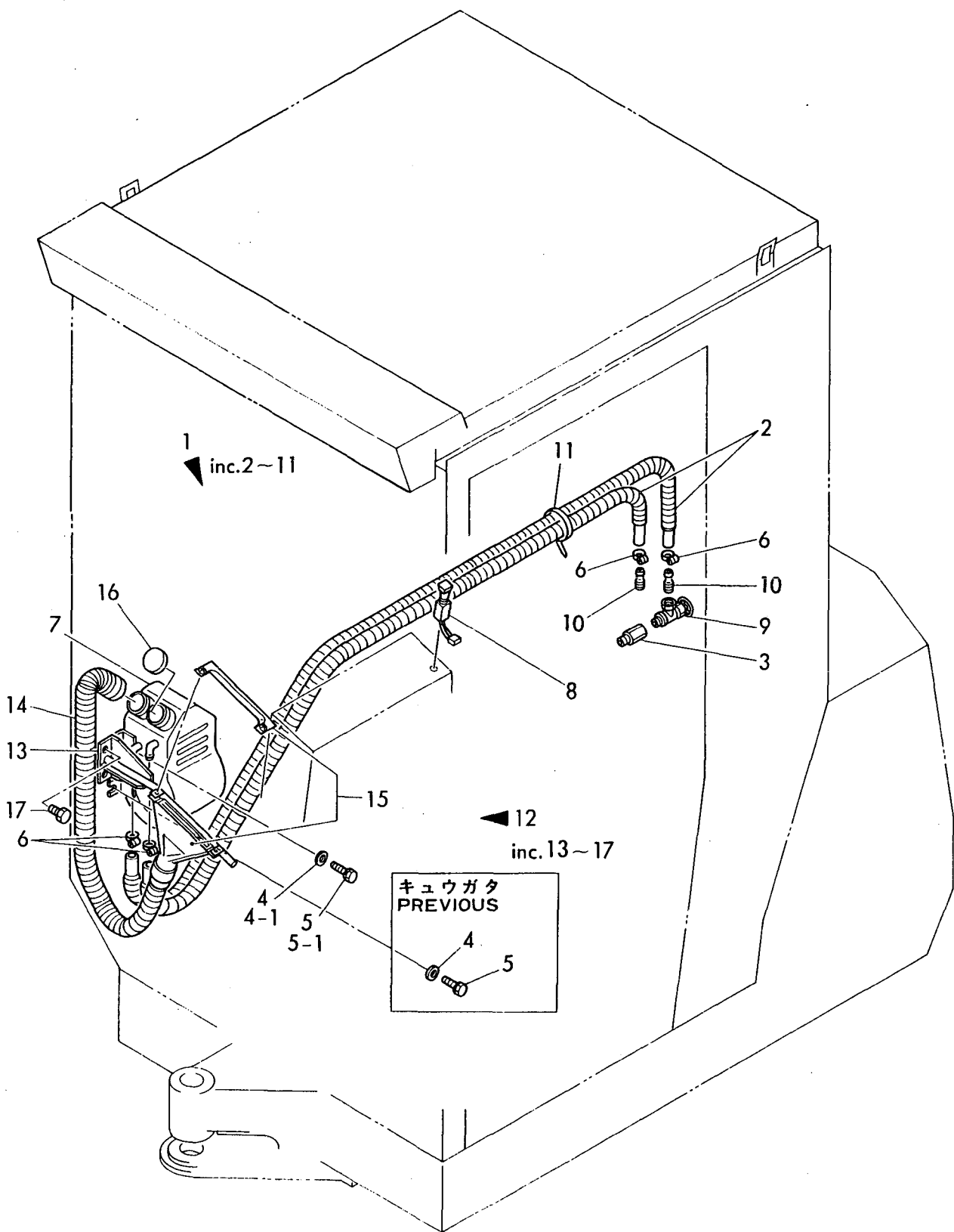
Fig. 70 ヒータ & デフロスタ (オプション) HEATER & DEFROSTER (OPTIONAL)
