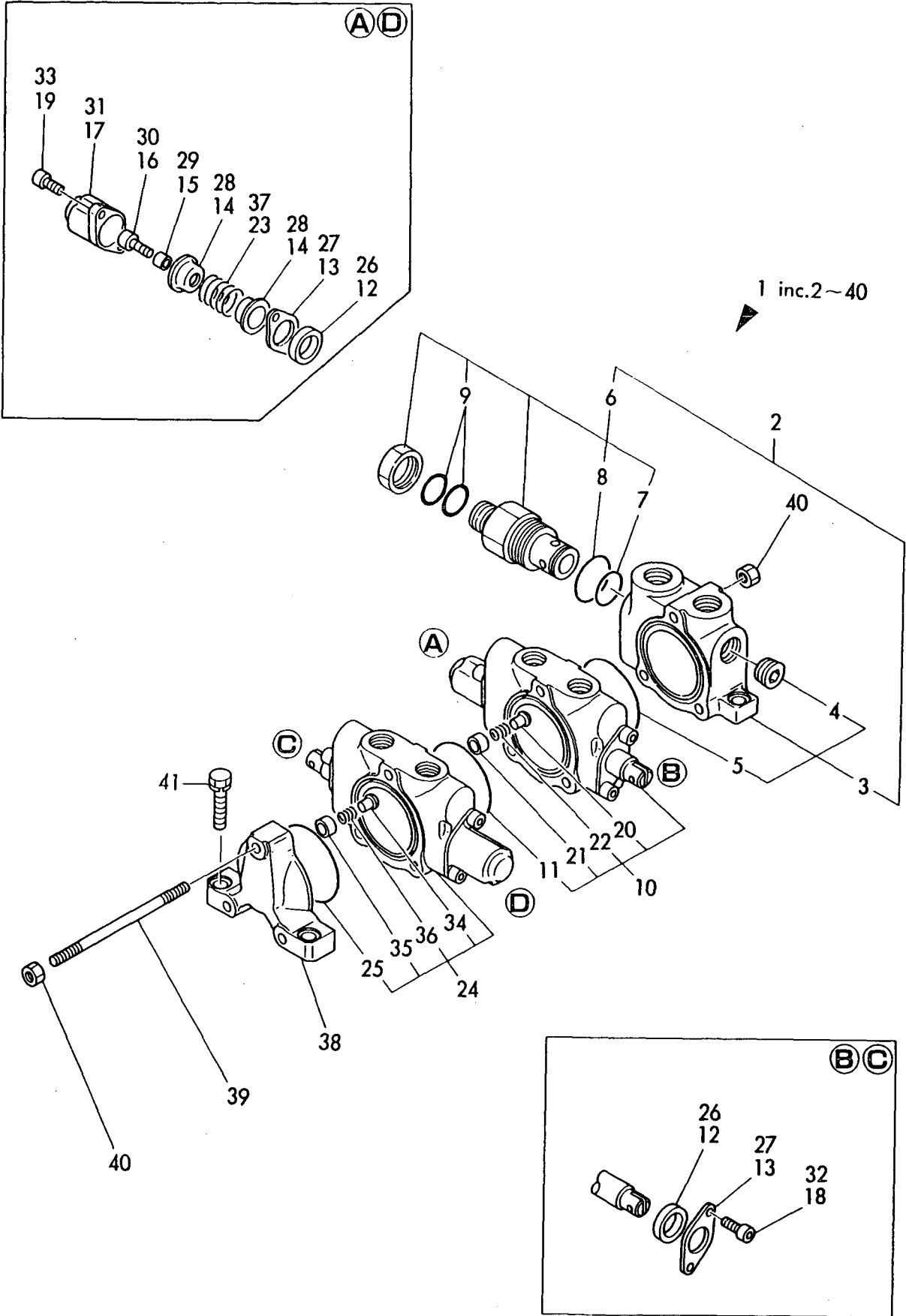
Fig. 45 コントロールバルブ(ブレード) CONTROL VALVE(BLADE)
