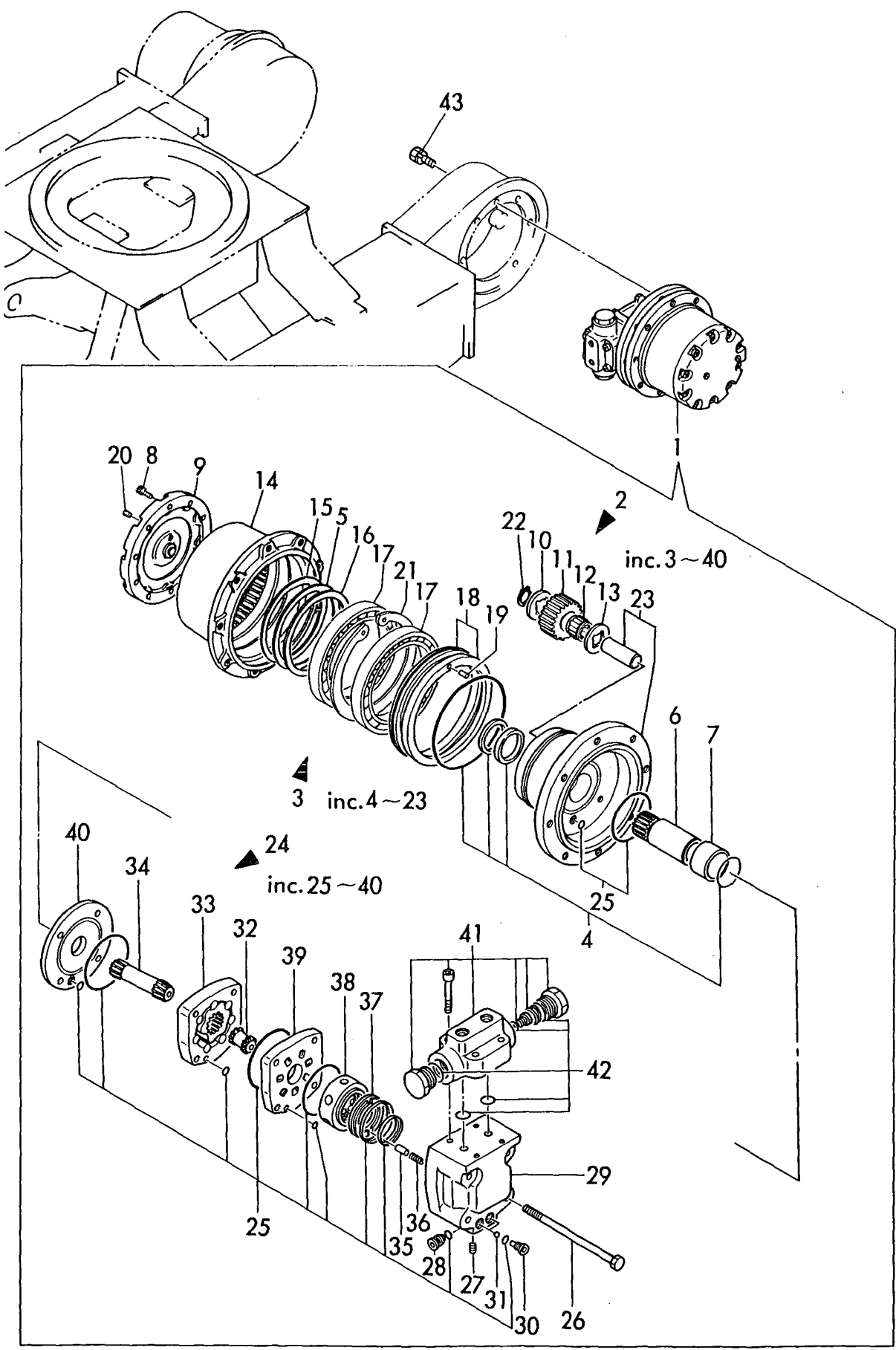
Fig. 60 ソウコウモータ(キュウガタ) TRAVEL MOTOR (PREVIOUS)
