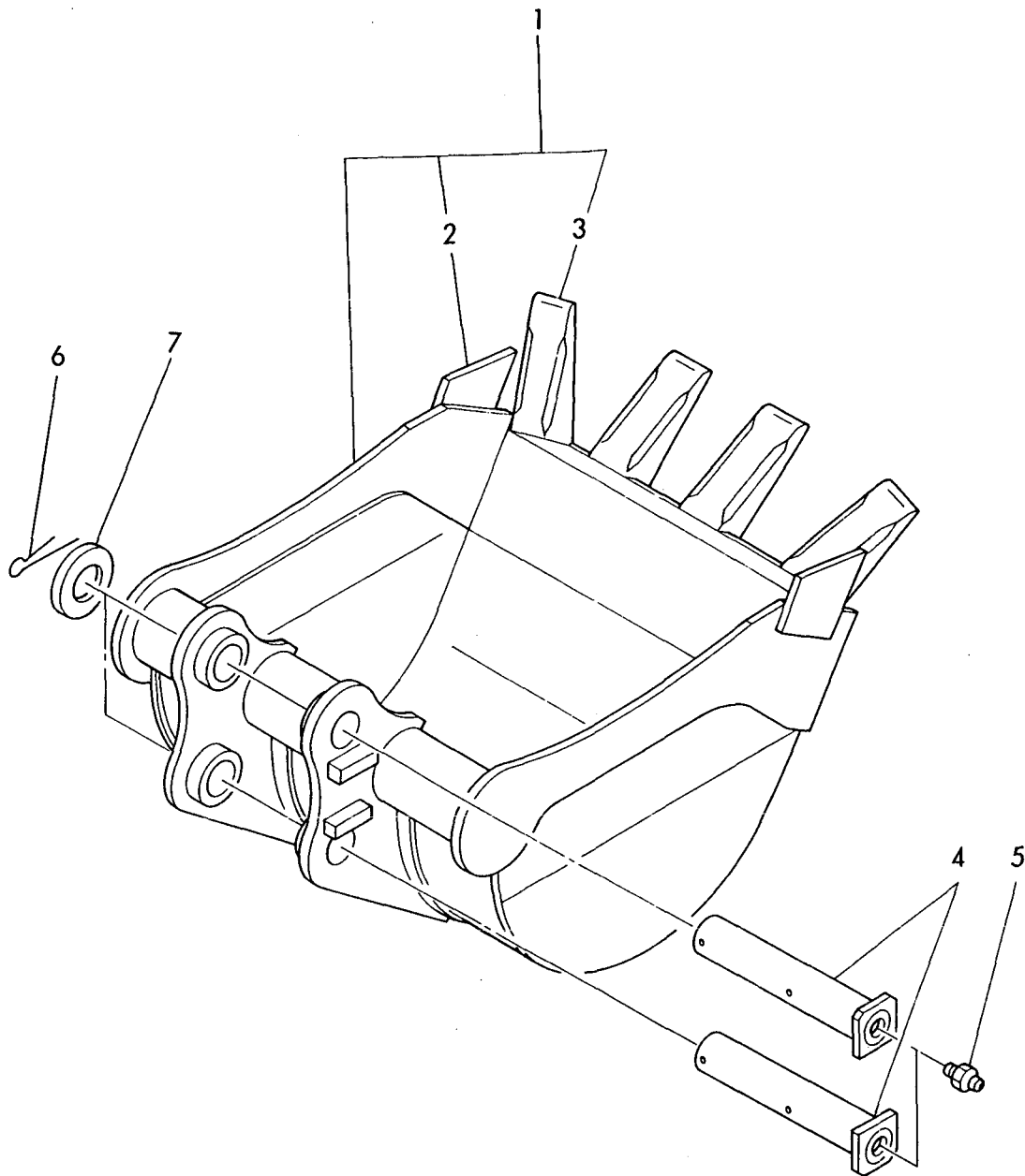
Fig. 69 バケット450W(アタッチメント) BUCKET 450W (ATTACHMENT)
