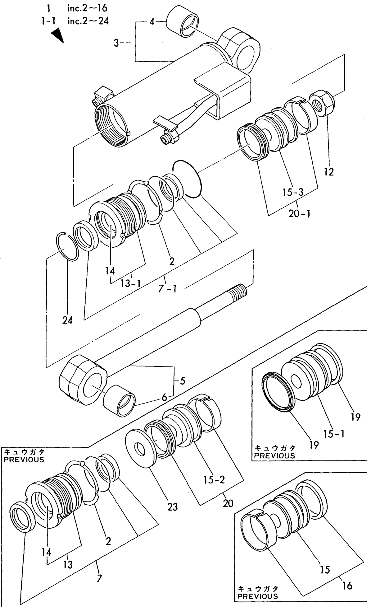
Fig. 56 ブレードシリンダ BLADE CYLINDER https://truckmanualshub.com/
