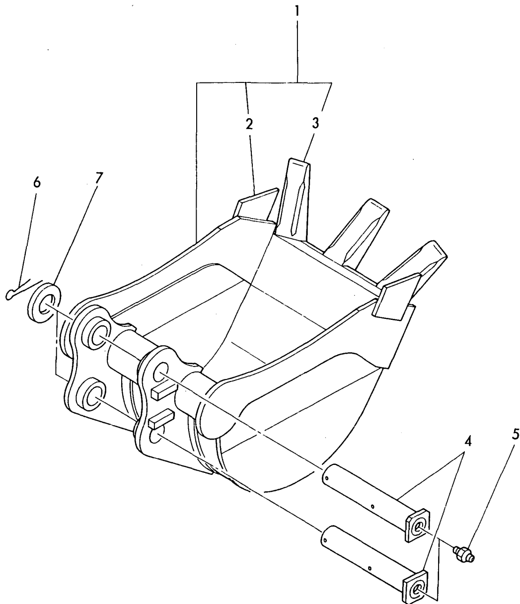
Fig. 67 バケット300W(アタッチメント) BUCKET 300W (ATTACHMENT)
