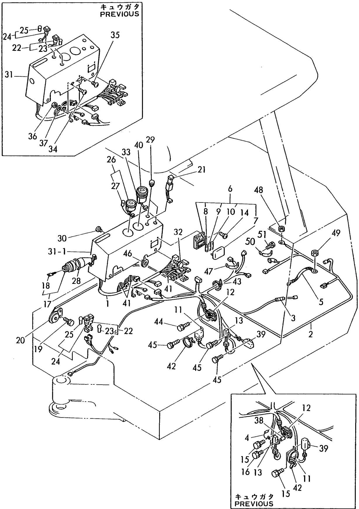
Fig. 12 デンソウヒン(キャノピ) ELECTRIC PART (CANOPY SPEC.)
