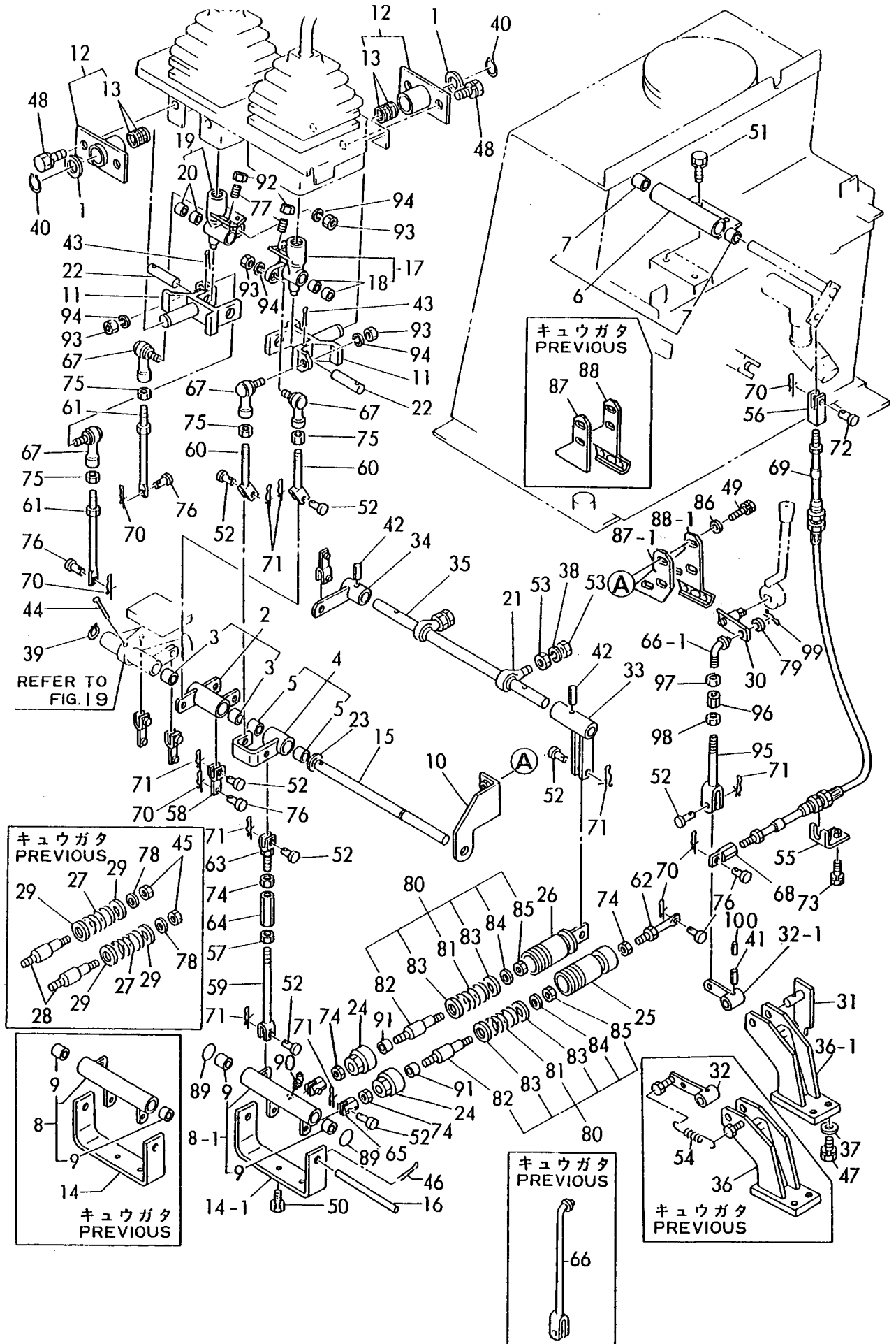
Fig. 21 ソウジュウソウチ(リンク & ロッド)(シンガタ) CONTROL EQUIPMENT (LINK & ROD)(NEW TYPE) (YB121U, YB151U: M/ #10501カラ) (YB121U, YB151U: FROM M/ #10501)
