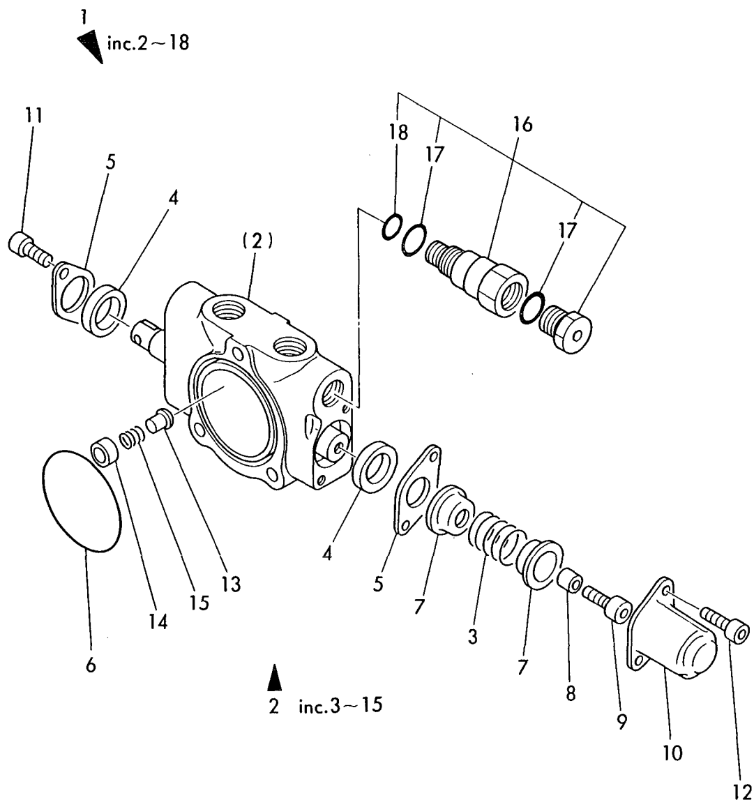
Fig. 47 コントロールバルブ(スイング) CONTROL VALVE (SWING)
