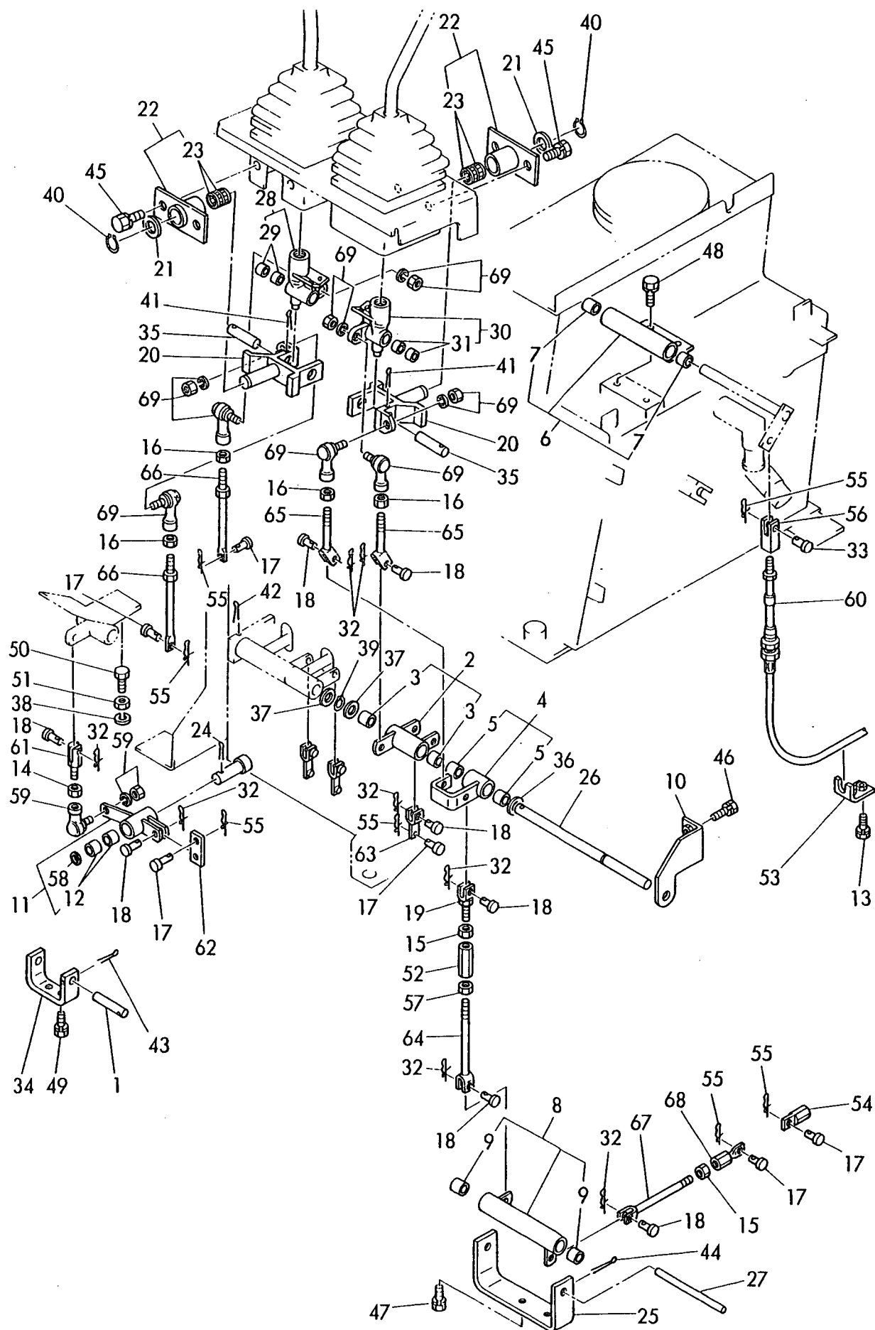
Fig. 20 ソウジュウソウチ(リンク & ロッド)(キュウガタ) CONTROL EQUIPMENT (LINK & ROD)(PREVIOUS) (YB121U: M/ #00698マデ) (YB151U: M/ #00608マデ) (YB121U: TO M/ #00698) (YB151U: TO M/ #00608)
