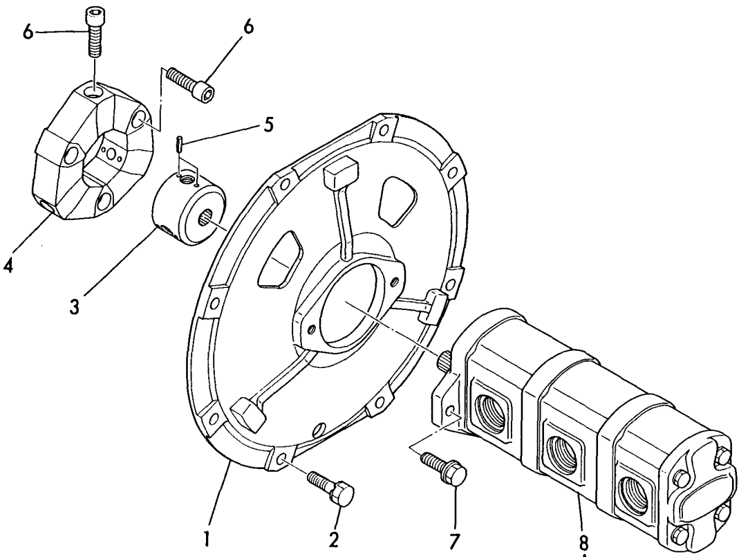
Fig. 32 ポンプ&ジョイント HYD. OIL PUMP & JOINT
