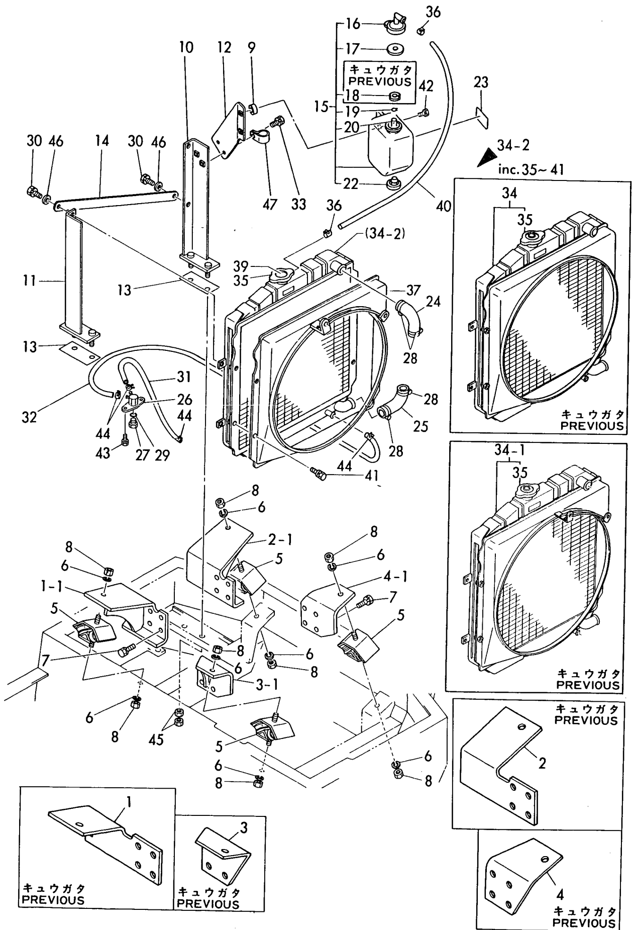
Fig. 7 エンジンマウント & ラジエータ ENGINE MOUNT & RADIATOR
