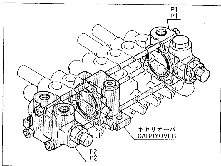
Fig. 46 コントロールバルブ(P1、P2) CONTROL VALVE (P1、P2)
