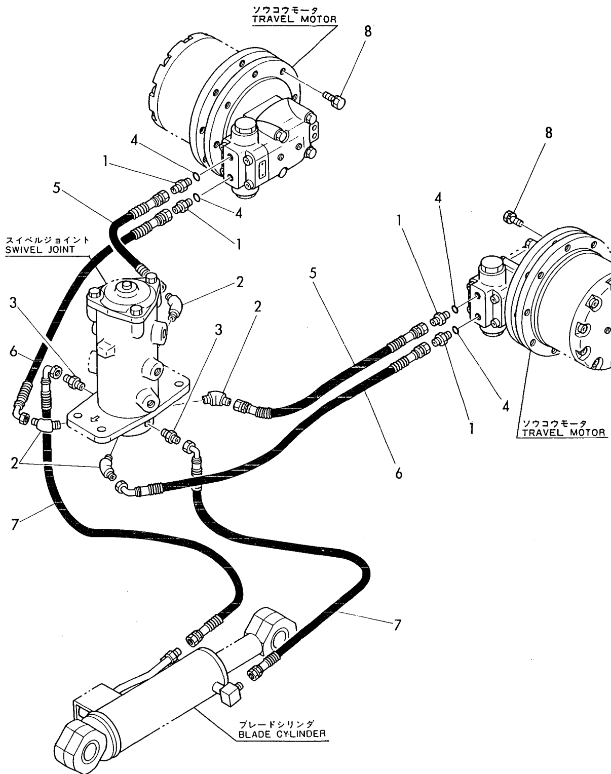
Fig. 38 ユアツハイカン(ソウコウ) HYD. OIL PIPING (TRAVEL)
