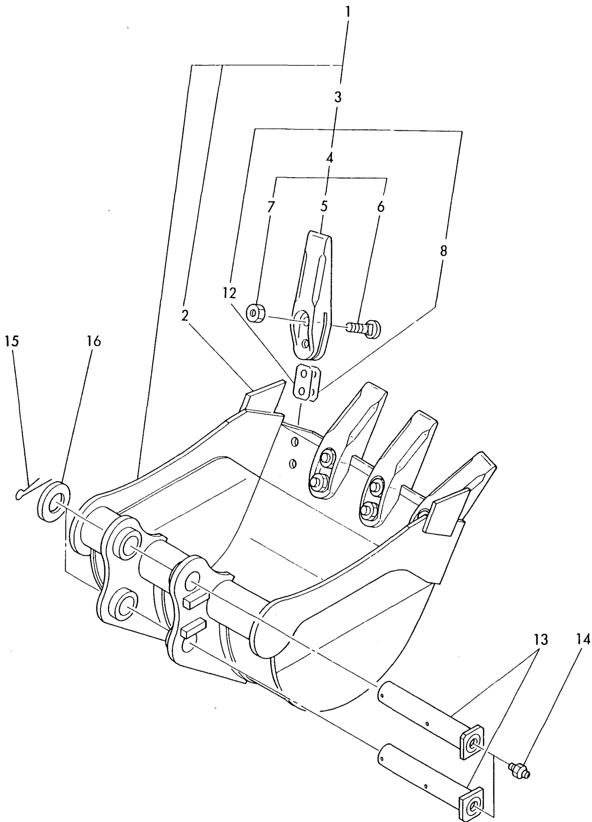
Fig. 65 バケット450(アタッチメント) BUCKET 450 (ATTACHMENT)
