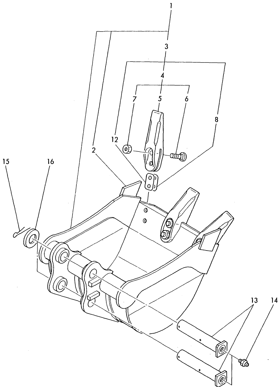
Fig. 64 バケット350(アタッチメント) BUCKET 350 (ATTACHMENT)
