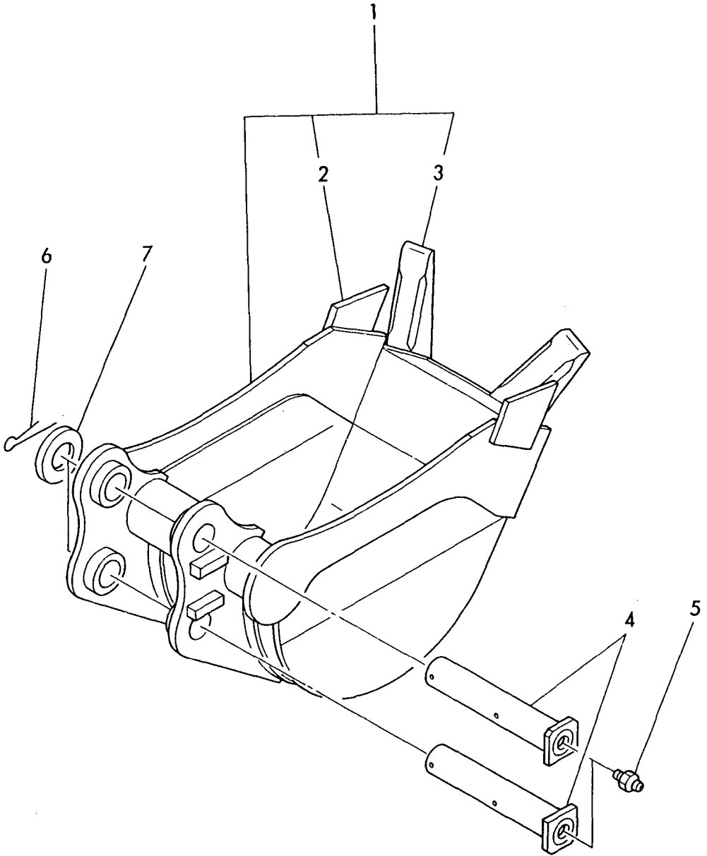
Fig. 66 バケット 250W (アタッチメント) BUCKET 250W (ATTACHMENT)
