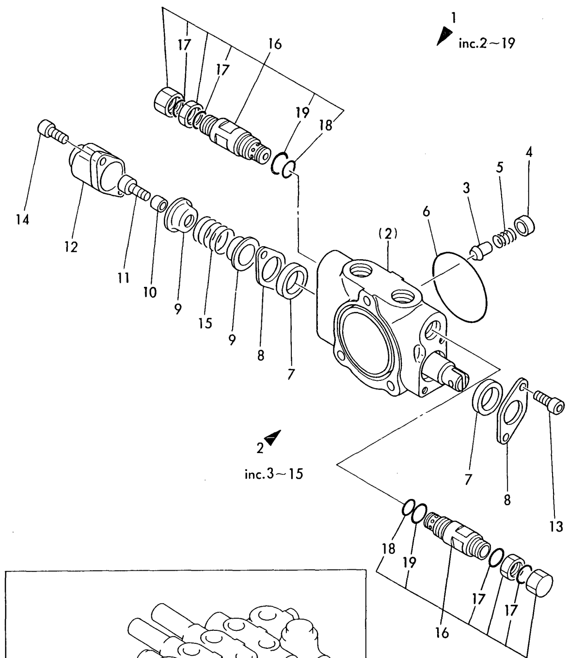
Fig. 51 コントロールバルブ(アーム) CONTROL VALVE (ARM)
