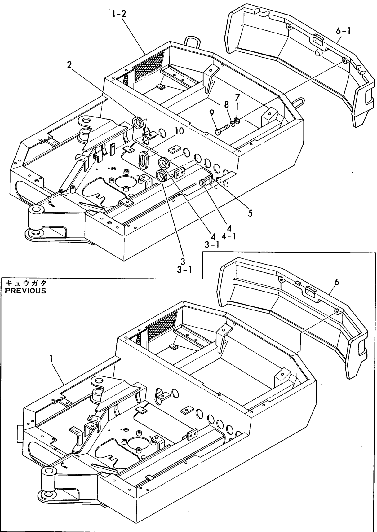
Fig. 23 センカイフレーム(YB151U) TURNING FRAME (YB151U)
