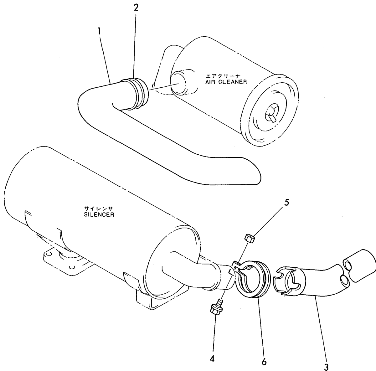
Fig. 6 キュウキカン & フンシュツコウ INLET HOUSE & EXHAUST PIPE
