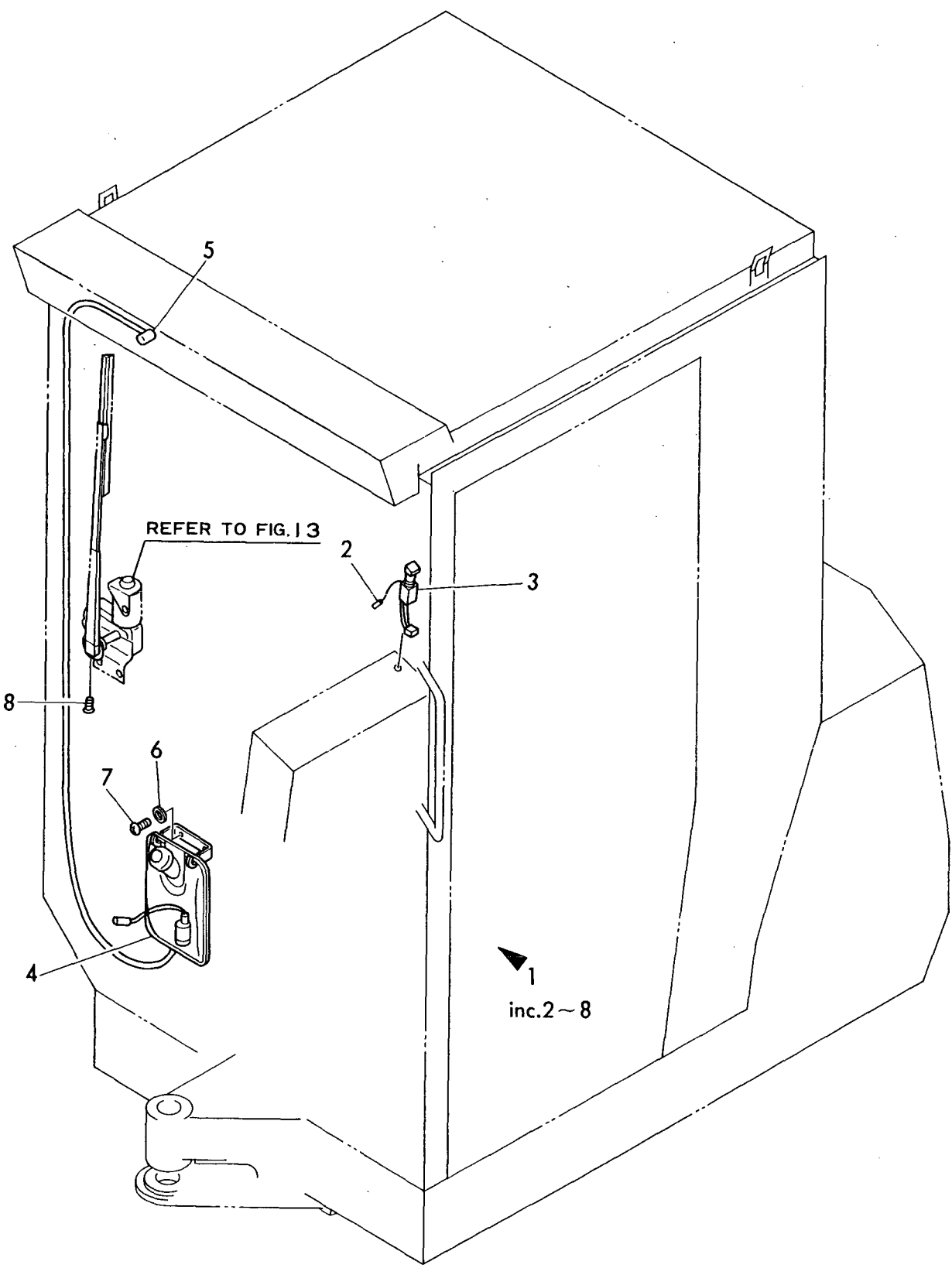
Fig. 71 ウィンドウワッシャ(オプション) WIND WASHER (OPTIONAL)
