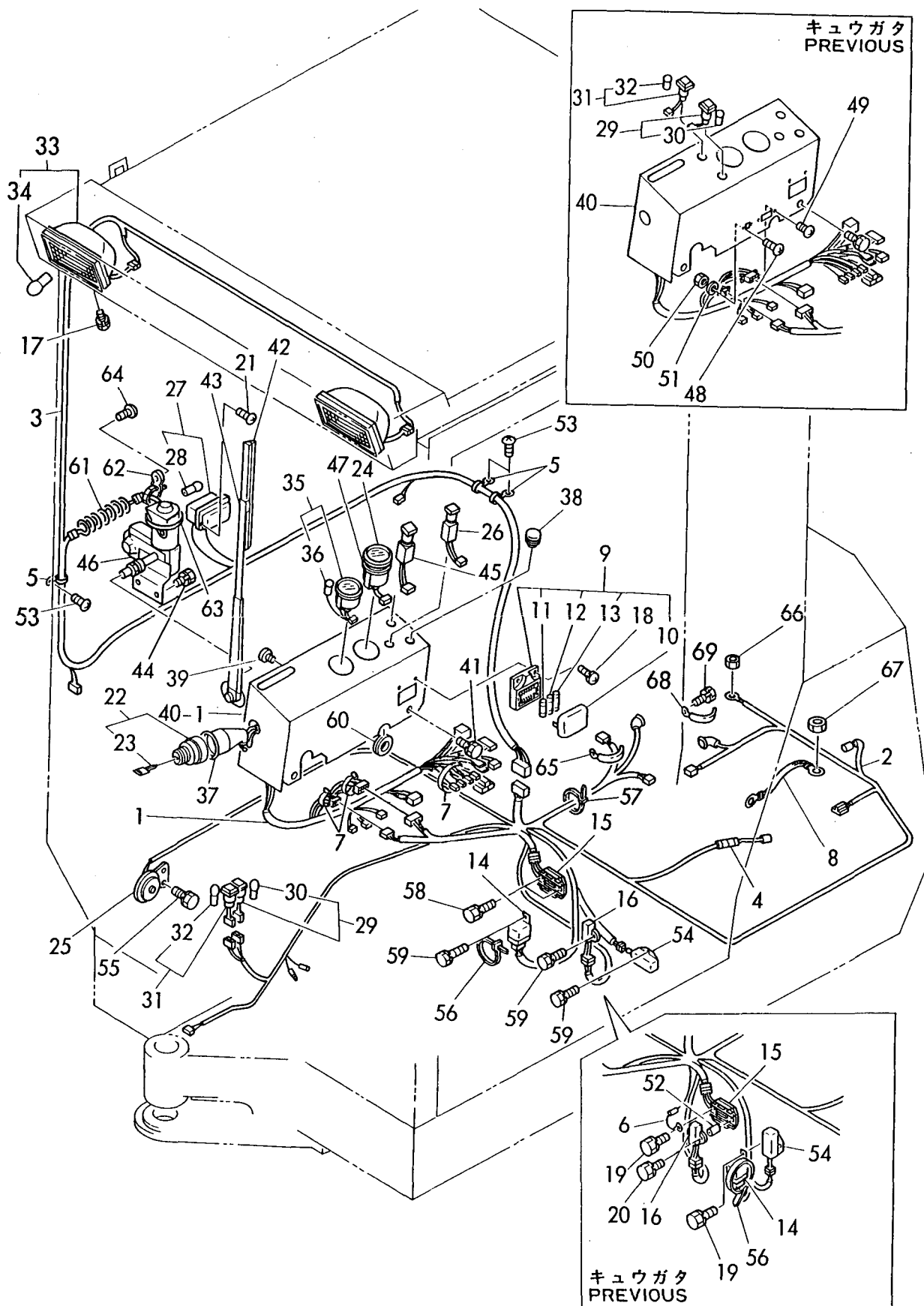
Fig. 13 デンソウヒン(キャビン) ELECTRIC PART (CABIN SPEC.)
