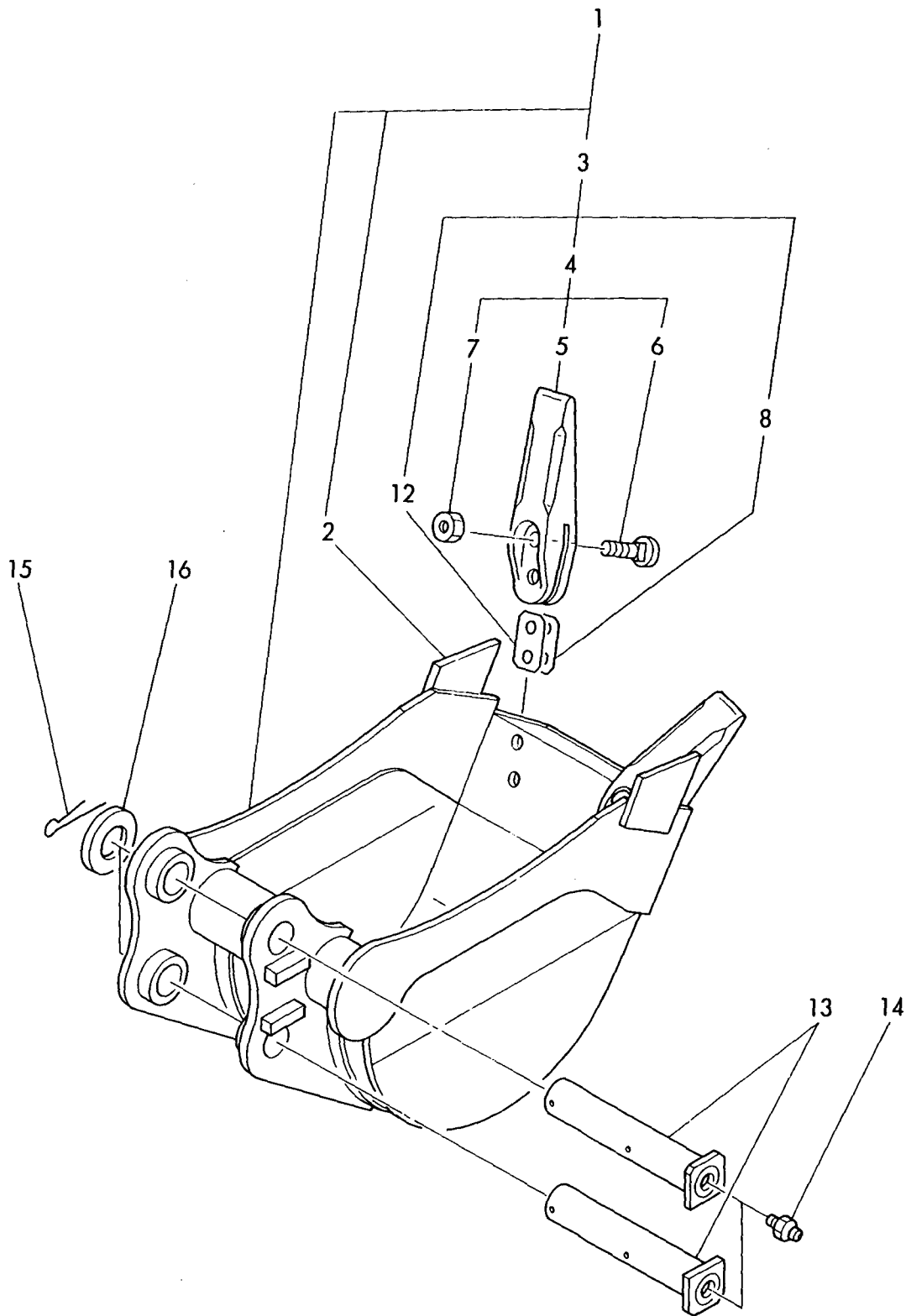
Fig. 62 バケット250(アタッチメント) BUCKET 250 (ATTACHMENT)
