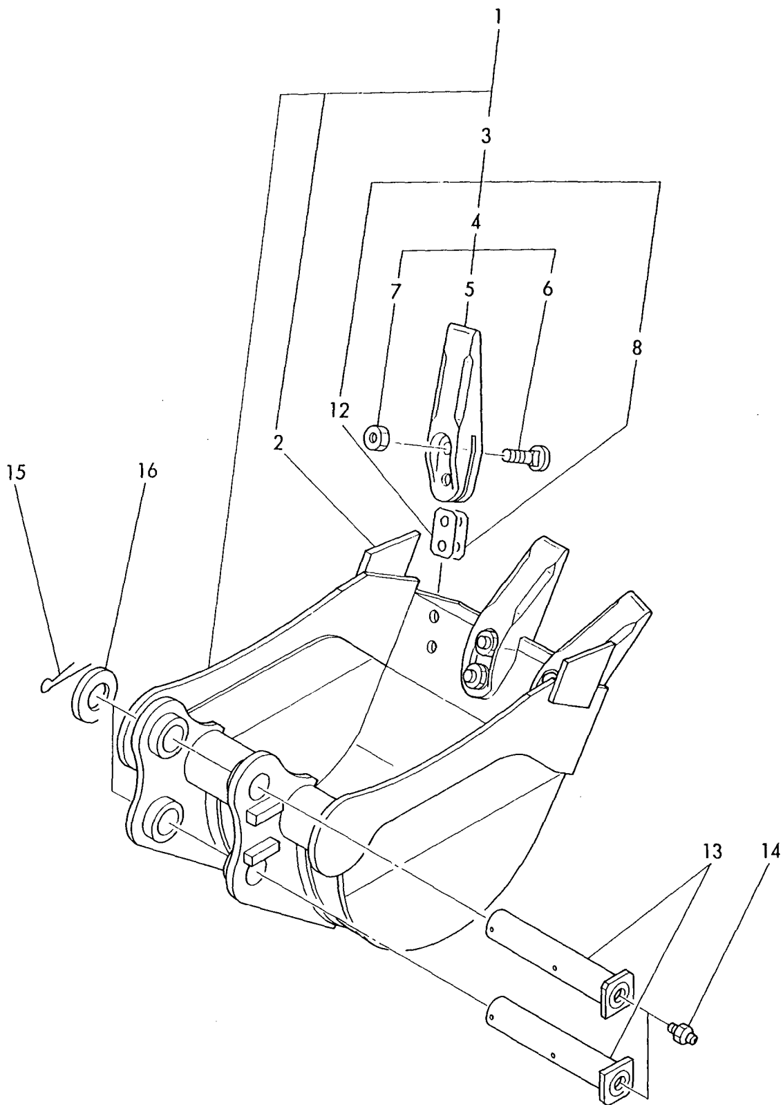
Fig. 63 バケット300(アタッチメント) BUCKET 300 (ATTACHMENT)
