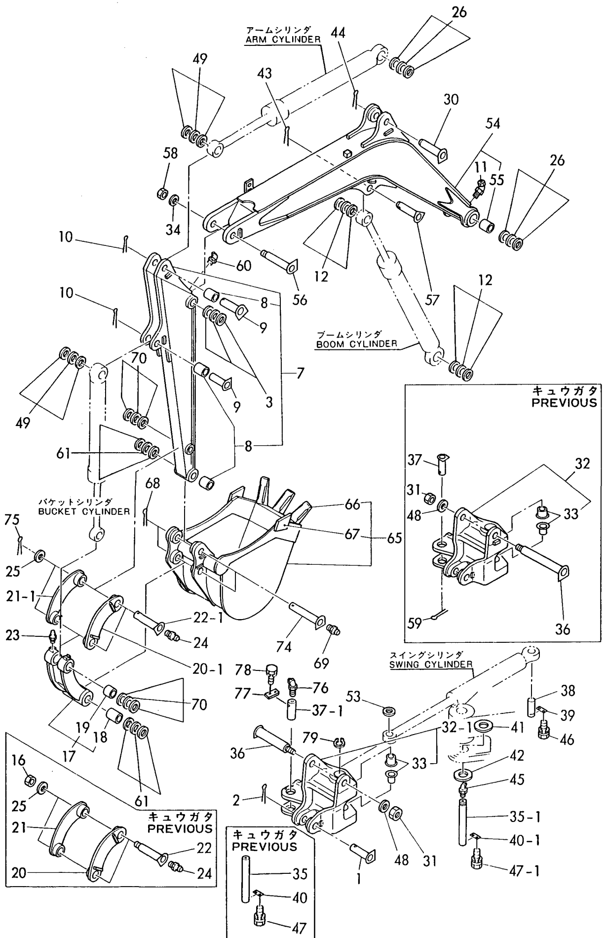
Fig. 42 ブーム&バケット (YB121U) BOOM & BUCKET (YB121U)
