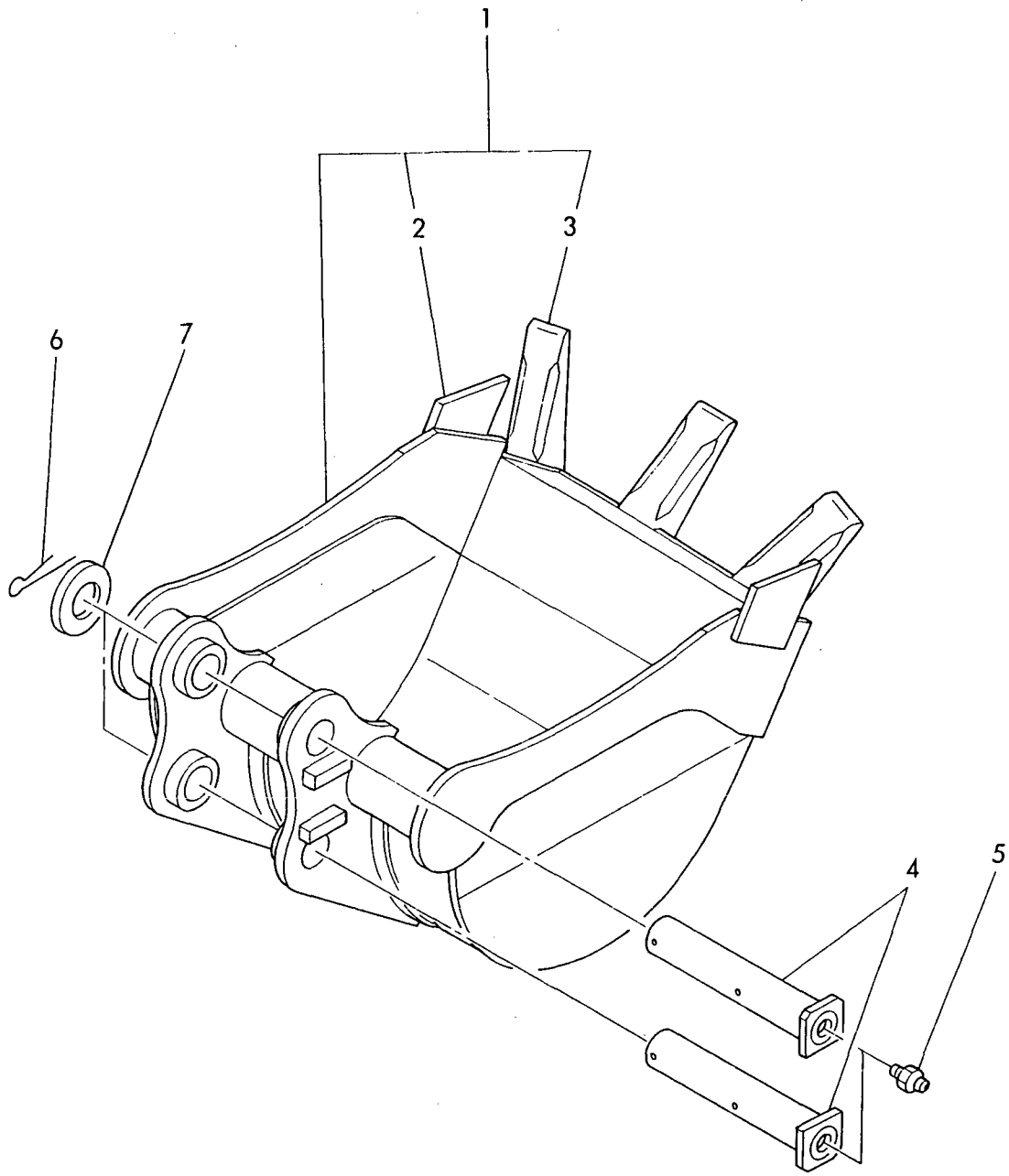
Fig. 68 バケット350W(アタッチメント) BUCKET 350W (ATTACHMENT)
