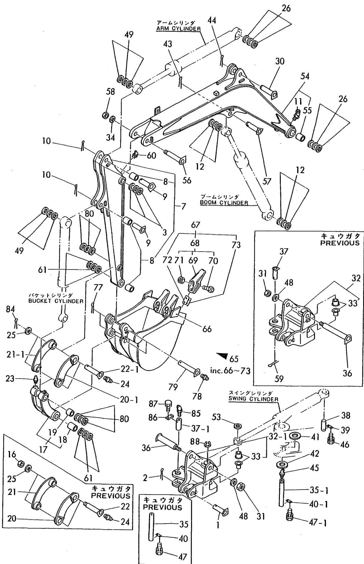
Fig. 43 ブーム&バケット (YB151U) BOOM & BUCKET (YB151U)
