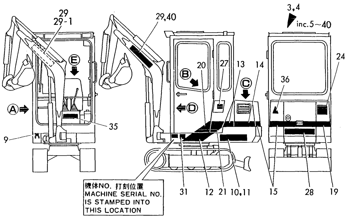
Fig. 2 2 メイバン(キャビン) LABEL (CABIN SPEC.) https://truckmanualshub.com/
