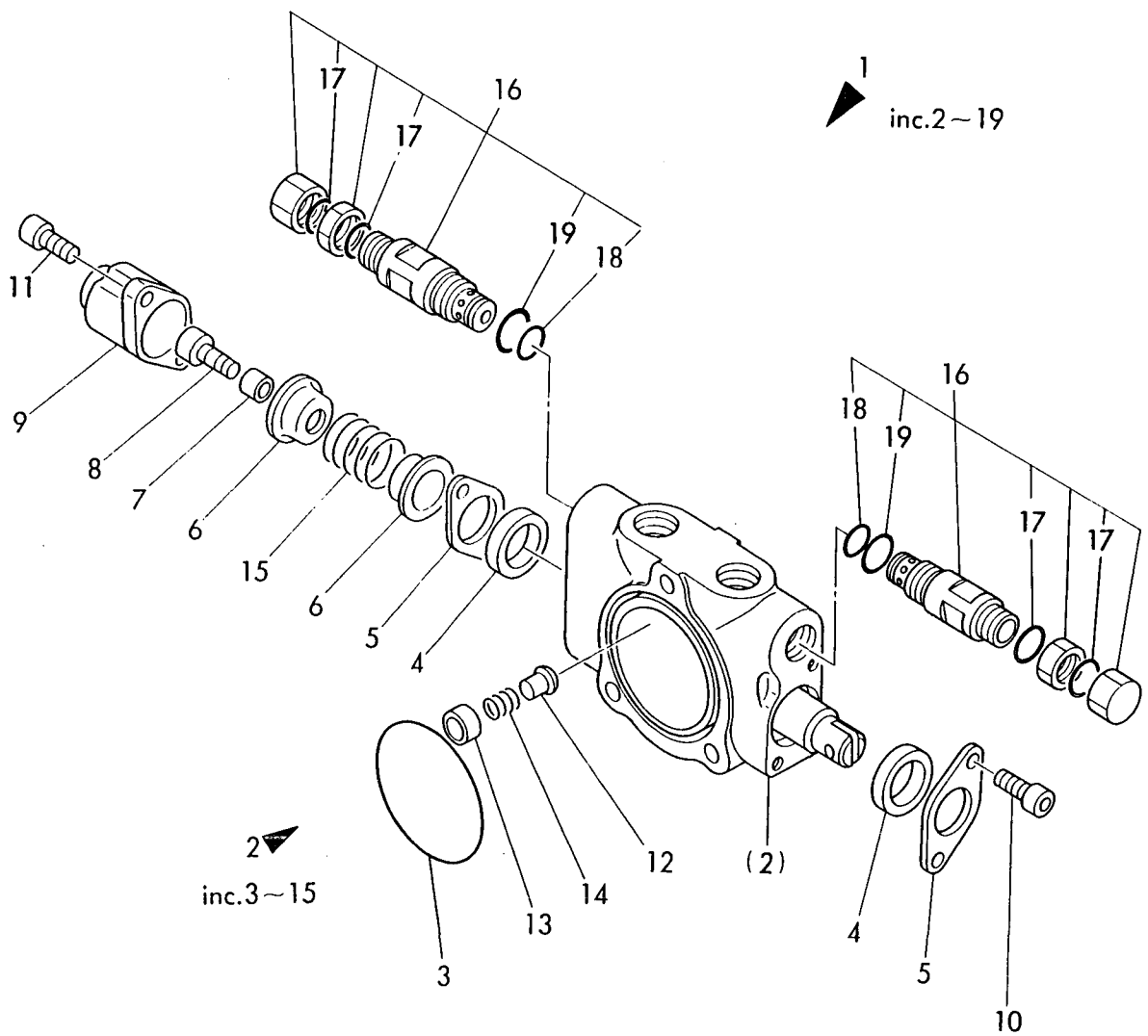
Fig. 48 コントロールバルブ(ブーム) CONTROL VALVE (BOOM) https://truckmanualshub.com/
