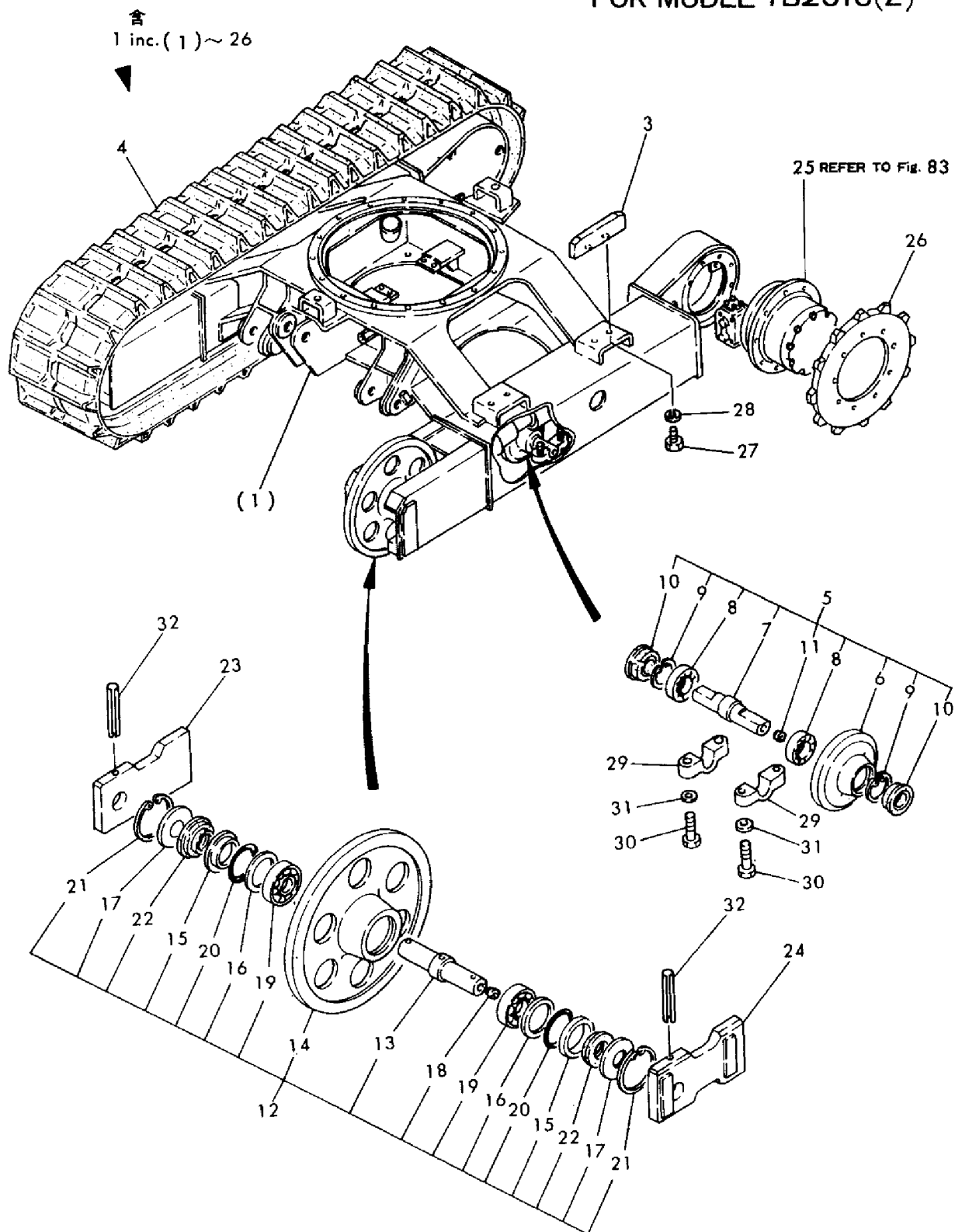
Fig. 82 ローアーマシン (ゴムクローラ), オプション, YB201U (Z) ヨウ LOWER MACHINE (RUBBER CRAWLER), OPTIONAL FOR MODEL YB201U(Z)
