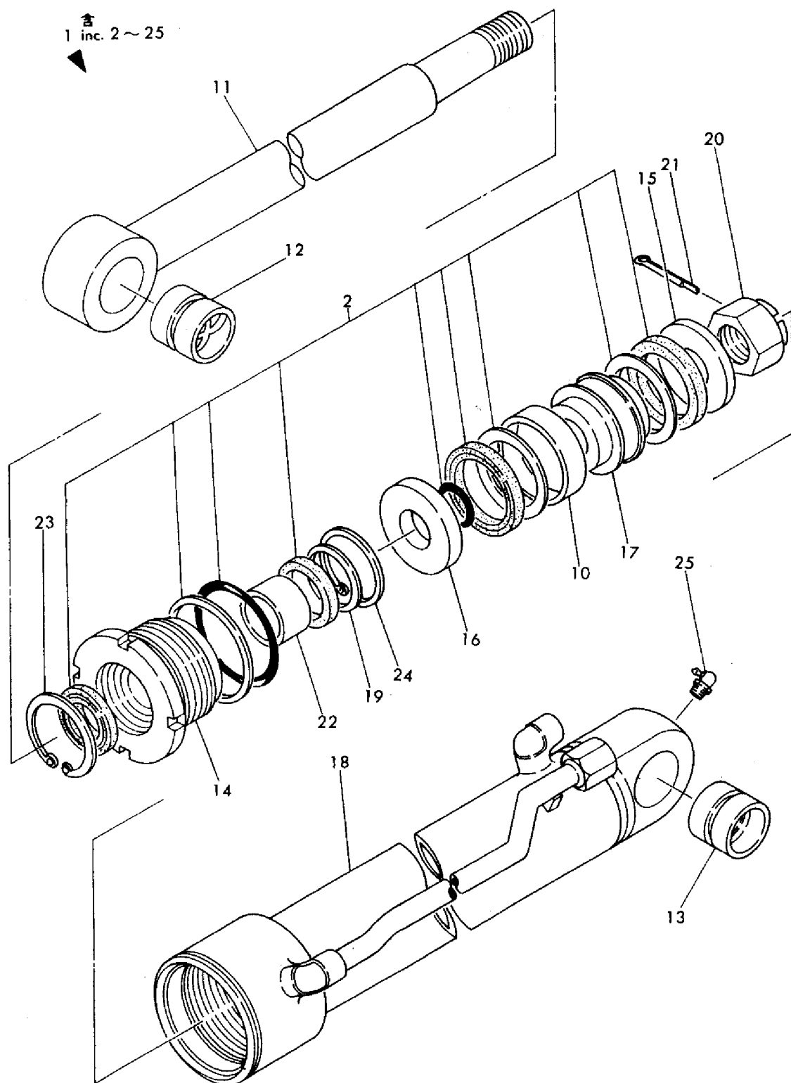
Fig. 72 アームシリンダー, YB201U (Z) ヨウ ARM CYLLINDER, FOR MODEL YB201U (Z)
