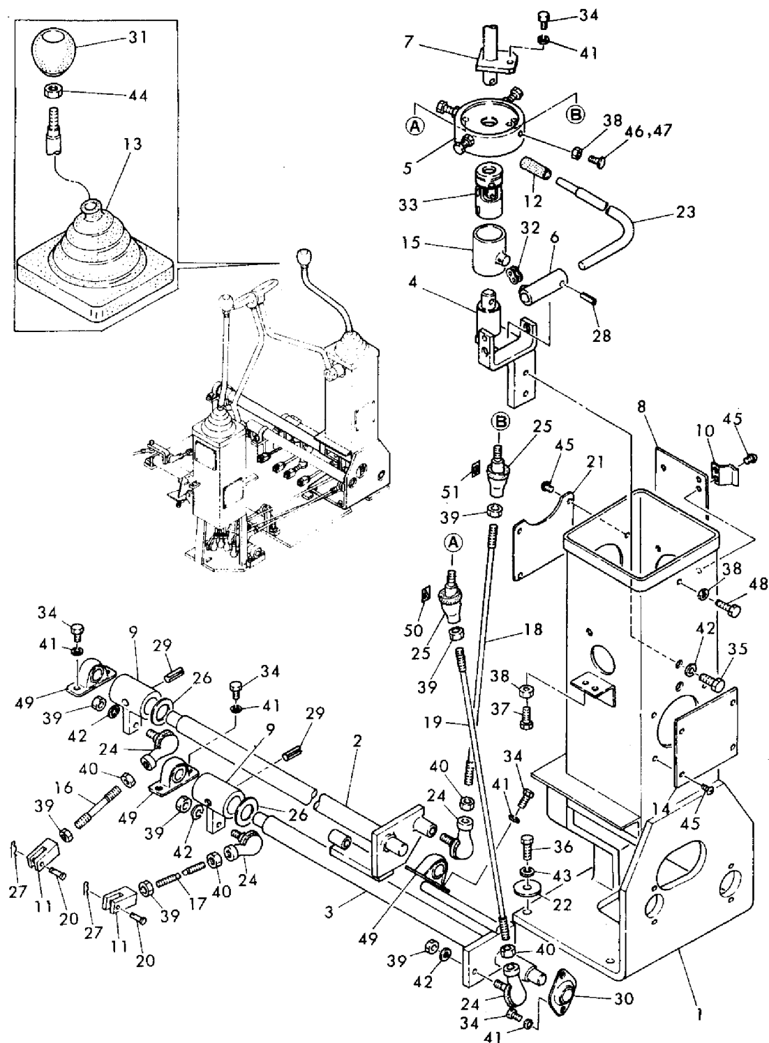
Fig. 18 コントロールレバー (操作用) 左, YB201U(Z) ヨウ CONTROL LEVER (OPERATION) LEFT, FOR MODEL YB201U (Z)
