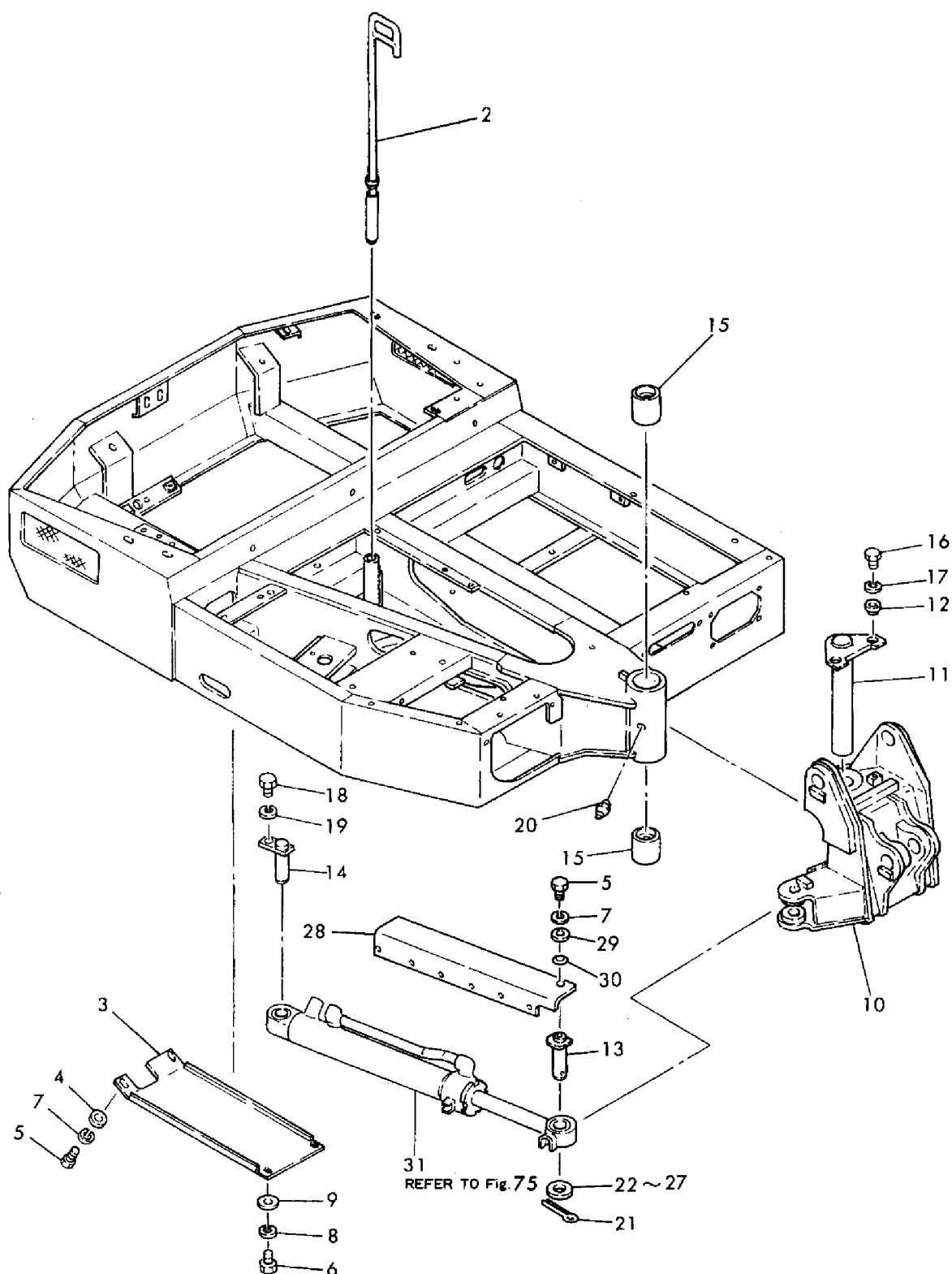
Fig. 10 本体 (YB20IZ ヨウ) MAIN FRAME (FOR MODEL YB20IZ)
