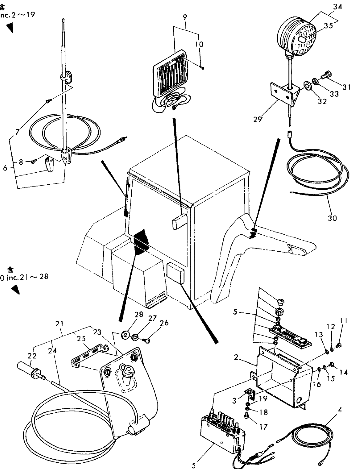
Fig. 88 電装品 (オプション), YB201U ヨウ ELECTRIC PART (OPTIONAL), FOR MODEL YB201U
