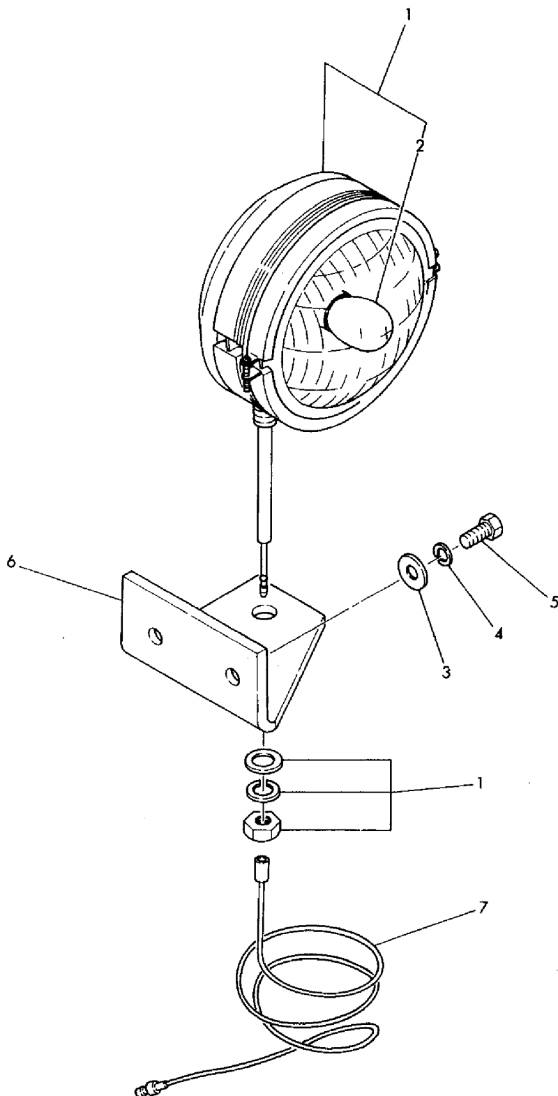
Fig. 90 ブームライト (オプション), YB201UZ ヨウ BOOM LAMP (OPTIONAL), FOR MODEL YB201UZ
