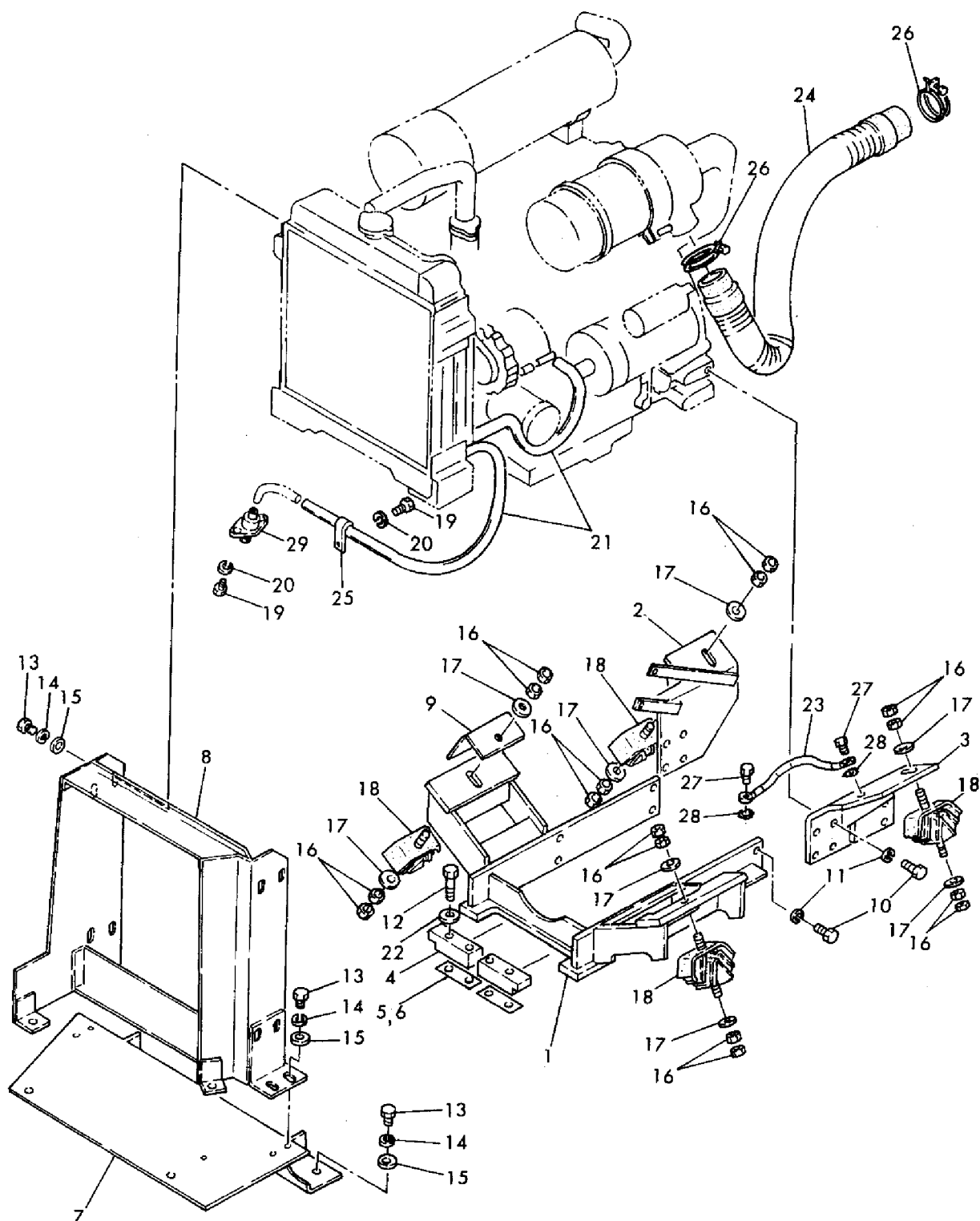
Fig. 23 エンジン関連装置 (エンジンマウント), YB201 (Z) ヨウ ENGINE RELATED DEVICE (ENG. MOUNT), FOR MODEL YB201 (Z)
