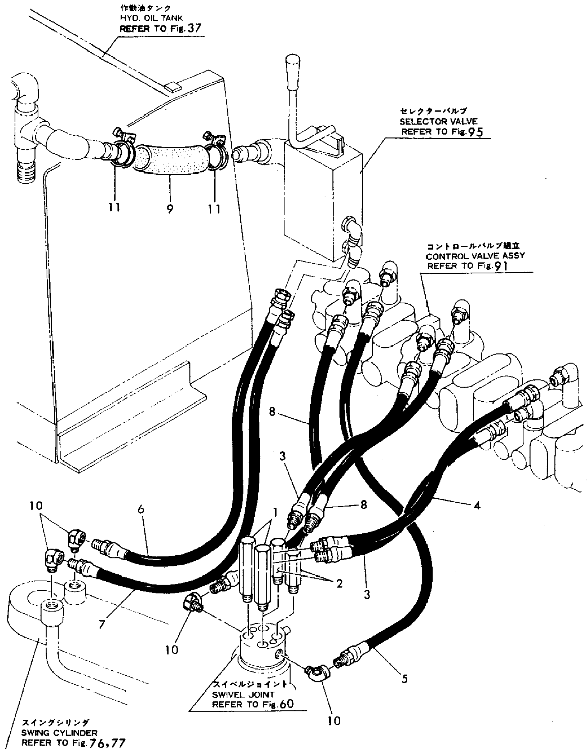
Fig. 92 上部油圧配管 (1), オプション, YB201U (Z) ヨウ UPPER HYDRAULIC OIL PIPING (1), (OPTIONAL), FOR MODEL YB201U (Z)
