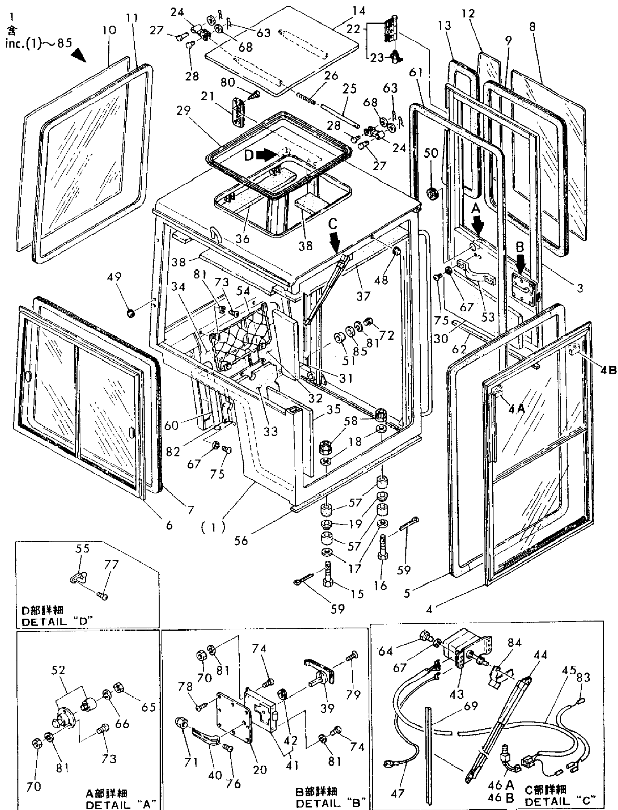
Fig. 46 スチールキャビン (オプション), YB201 ヨウ STEEL CABIN (OPTIONAL), FOR MODEL YB201
