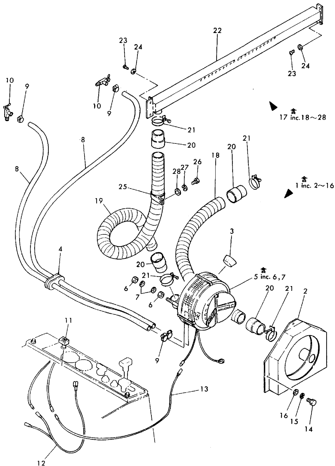
Fig. 98 ヒーター & デフロスター (オプション) YB201 ヨウ HEATER & DEFROSTER.....OPTIONAL (FOR MODEL YB201)
