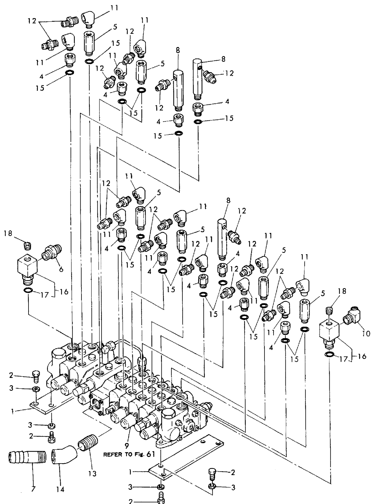
Fig. 30 コントロールバルブクミタテ, YB201 (Z) ヨウ CONTROL VALVE ASSY, FOR MODEL YB201 (Z)
