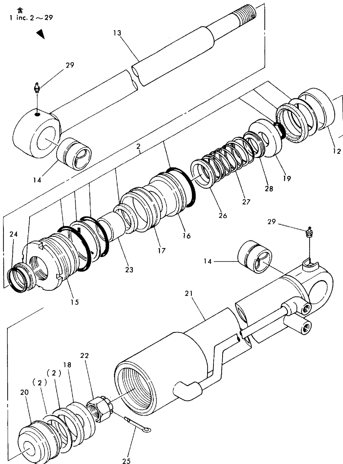
Fig. 65 メインブームシリンダー (YB201Zヨウ) MAIN BOOM CYLINDER (FOR MODEL YB201Z)
