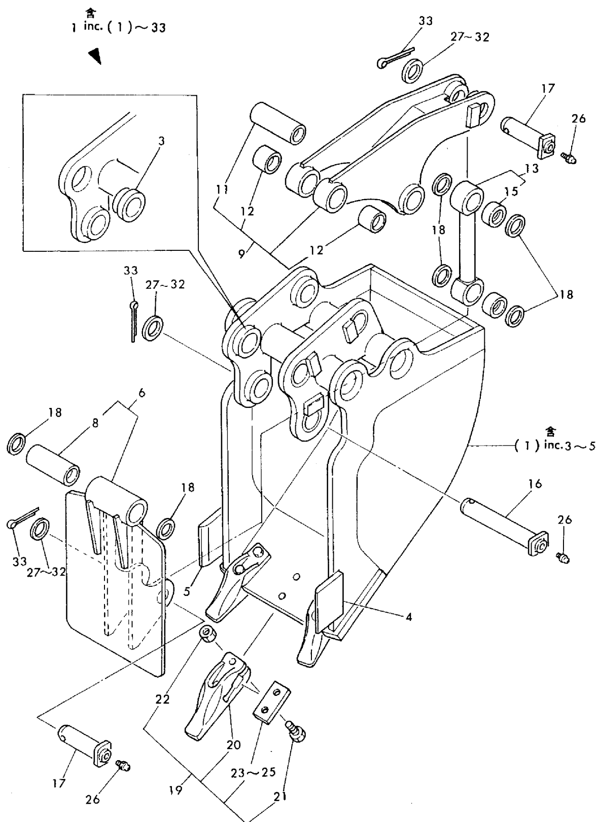
Fig. 100 エゼクター付バケット (オプション), YB201 (Z) ヨウ EJECTOR BUCKET (OPTIONAL), FOR MODEL YB201 (Z)
