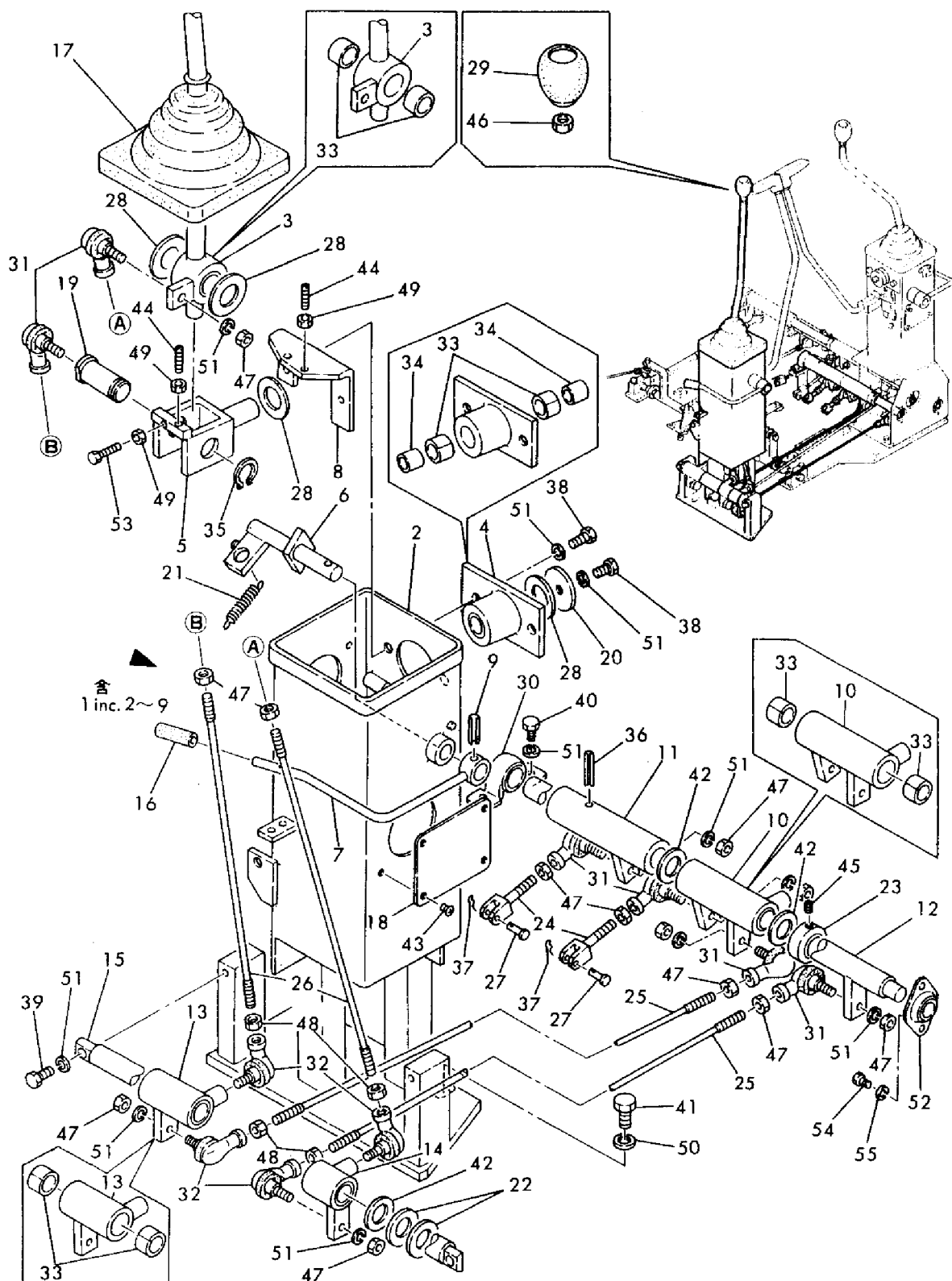
Fig. 85 クイックチェンジレバー (操作・右) オプション, YB201 (Z) ヨウ QUICK CHANGE LEVER (OPERATION, RIGHT) OPTIONAL, FOR MODEL YB201 (Z)
