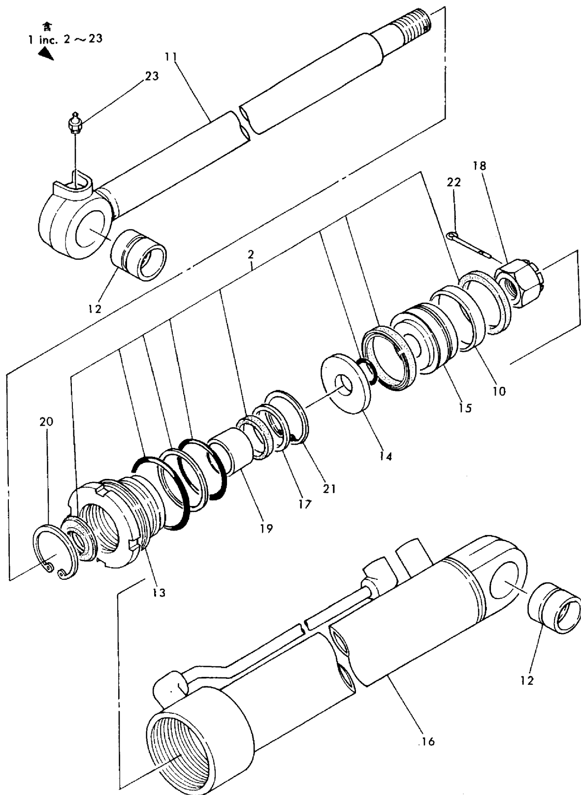
Fig. 75 スイングシリンダー, YB201 (Z) ヨウ SWING CYLINDER, FOR MODEL YB201 (Z)
