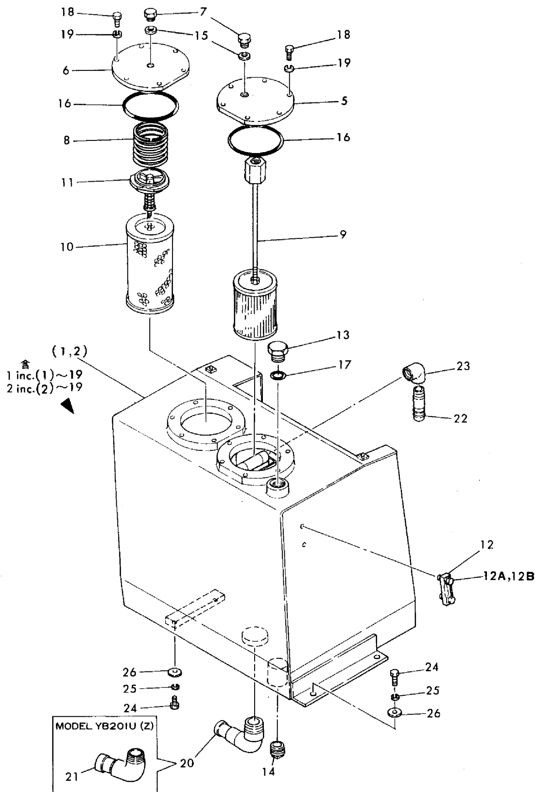
Fig. 37 作動油タンク HYDRAULIC OIL TANK
