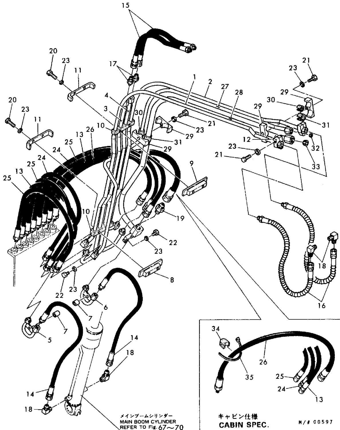
Fig. 94 油圧配管 (ブーム & アーム) オプション, YB201U (Z) ヨウ HYD. OIL PIPING (BOOM & ARM), OPTIONAL, FOR MODEL YB201U (Z)
