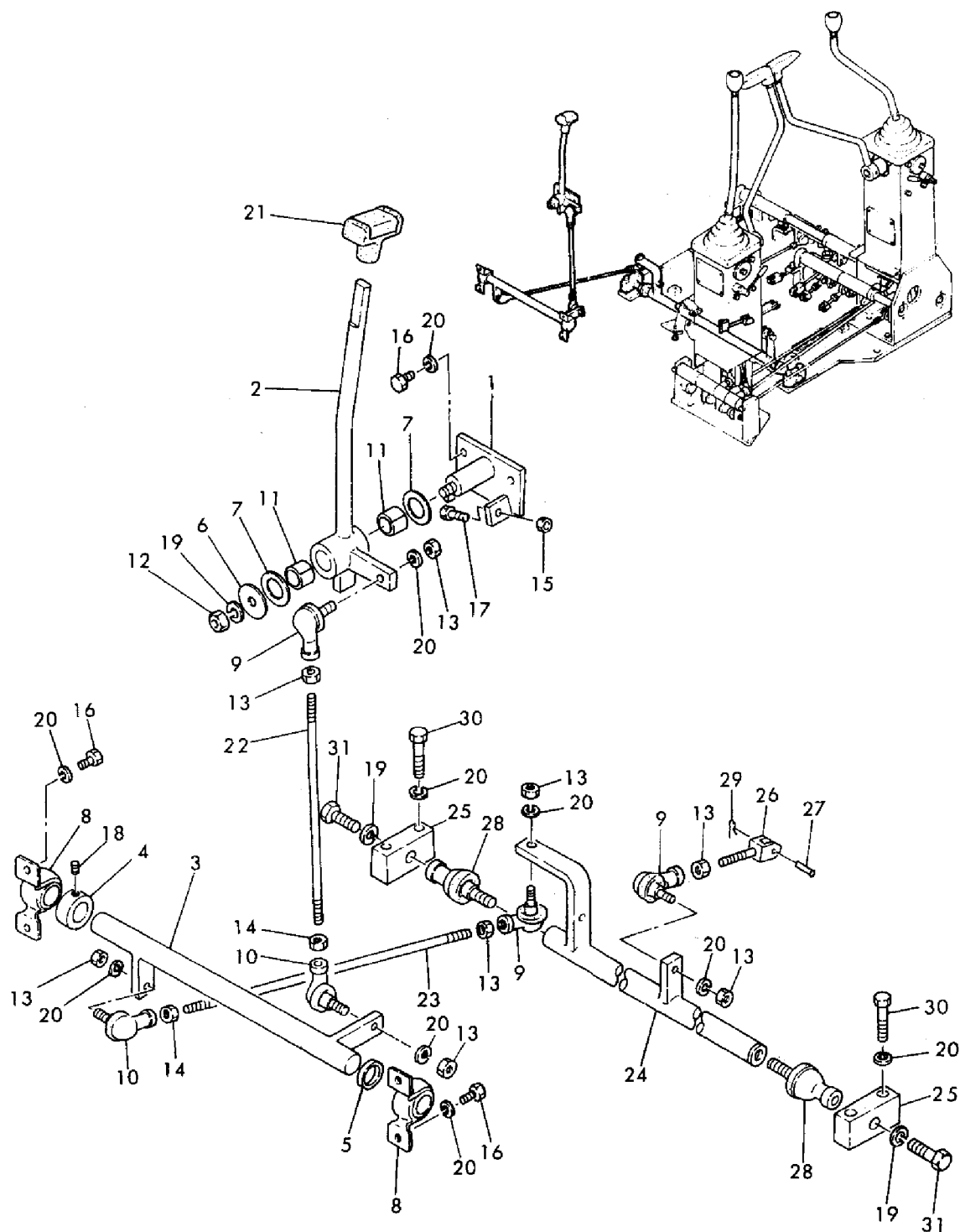
Fig. 21 コントロールレバー (排土板), YB201 (Z) ヨウ CONTROL LEVER (BLADE), FOR MODEL YB201 (Z)
