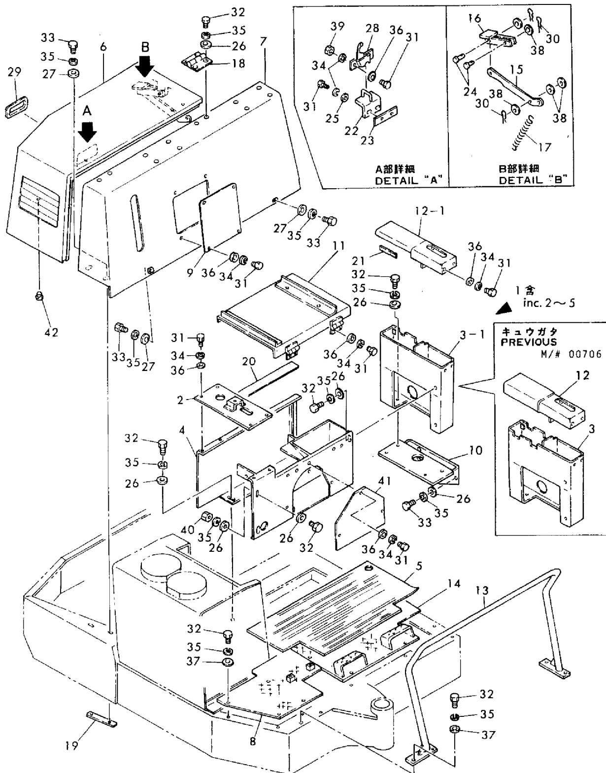
Fig. 40 ボンネット関係 (キャビン仕様), YB201ヨウ, オプション BONNET RELATION (CABIN SPEC.), FOR MODEL YB201...OPTIONAL
