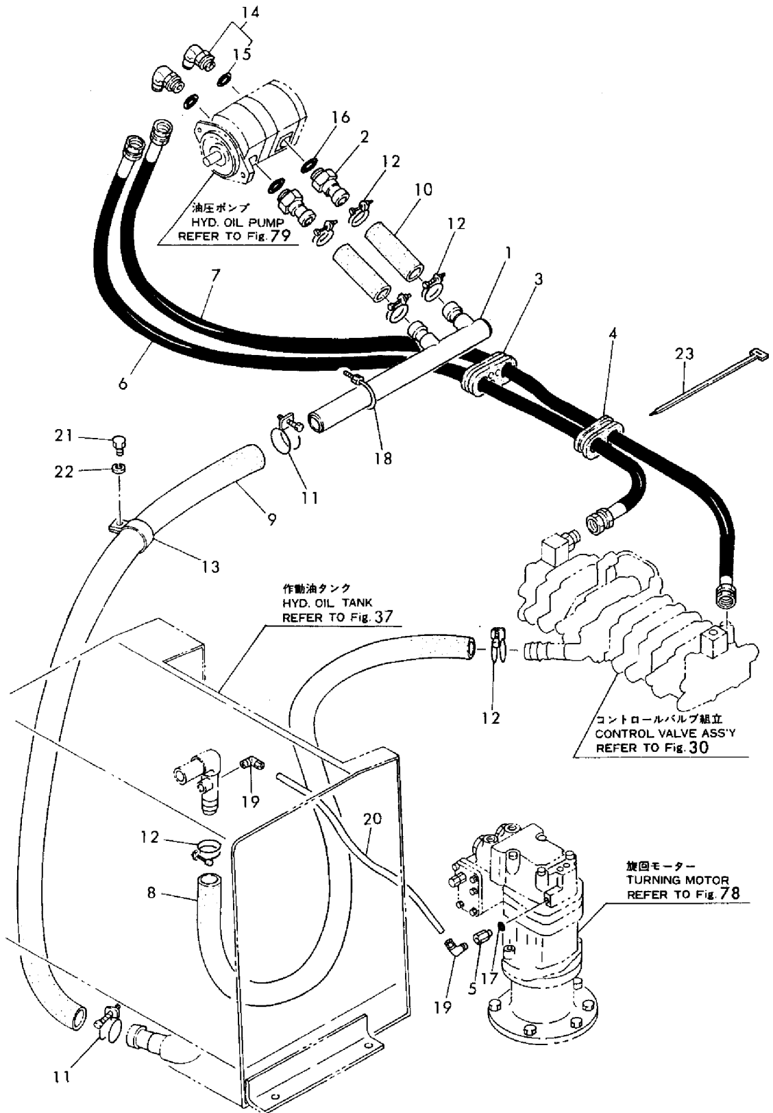
Fig. 32 上部油圧配管 (1), YB201 (Z) ヨウ UPPER HYDRAULIC OIL PIPING (1), FOR MODEL YB201 (Z)
