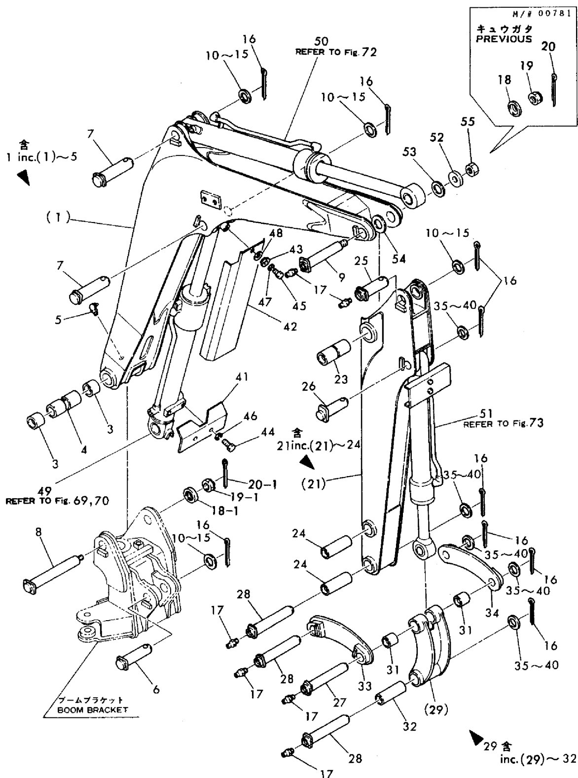
Fig. 51 ブーム & アーム (YB201UZ ヨウ) BOOM & ARM (FOR MODEL YB201UZ)
