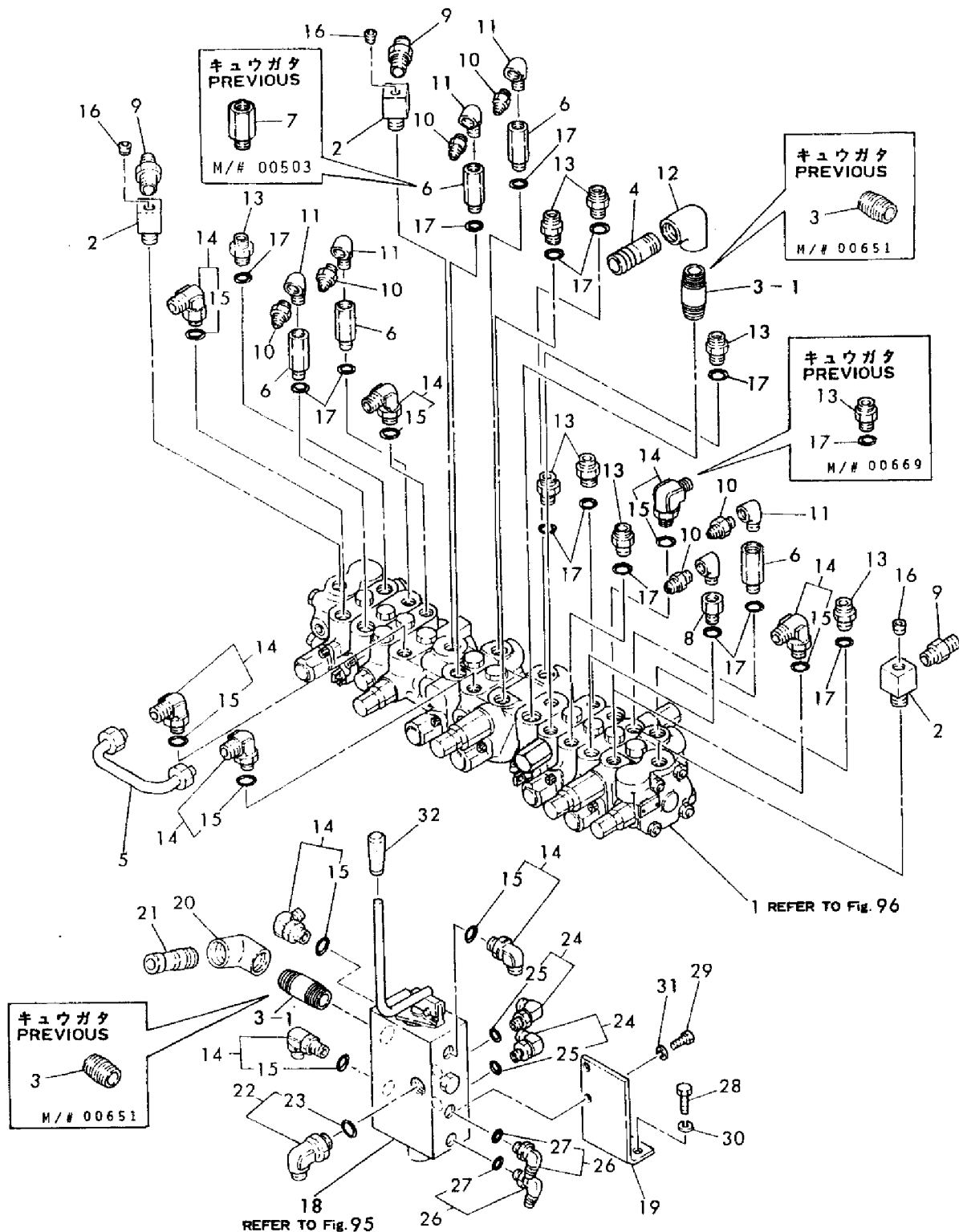
Fig. 91 コントロールバルブクミタテ (オプション), YB201U (Z) ヨウ CONTROL VALVE ASSY (OPTIONAL), FOR MODEL YB201U (Z)
