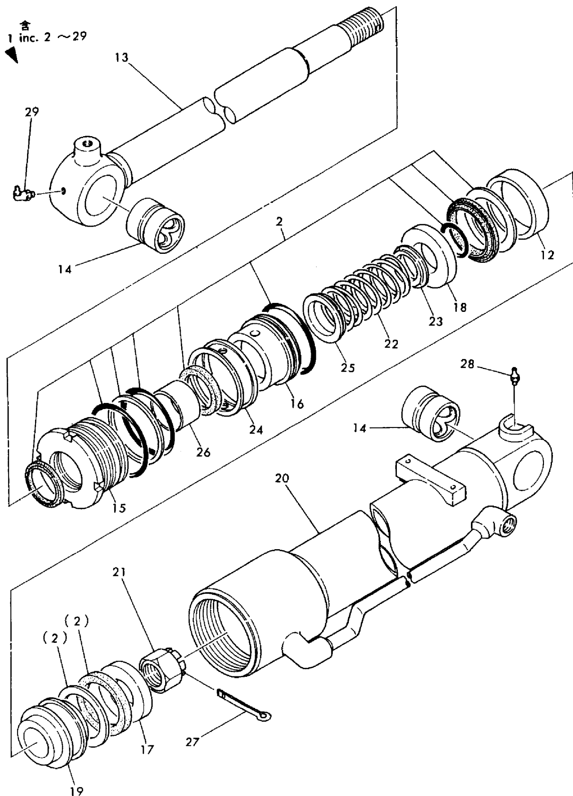
Fig. 69 メインブームシリンダ, YB201UZ ヨウ MAIN BOOM CYLINDER, FOR MODEL YB201UZ
