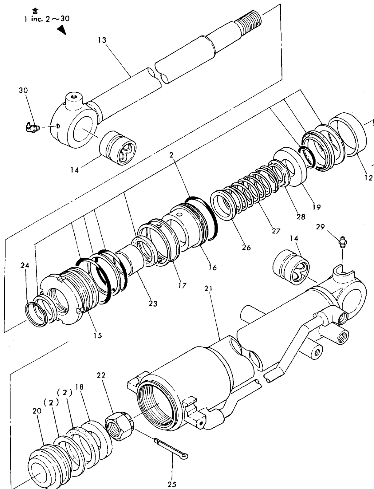
Fig. 66 メインブームシリンダー (YB20IZヨウ), M/#00573 MAIN BOOM CYLINDER (FOR MODEL YB20IZ)
