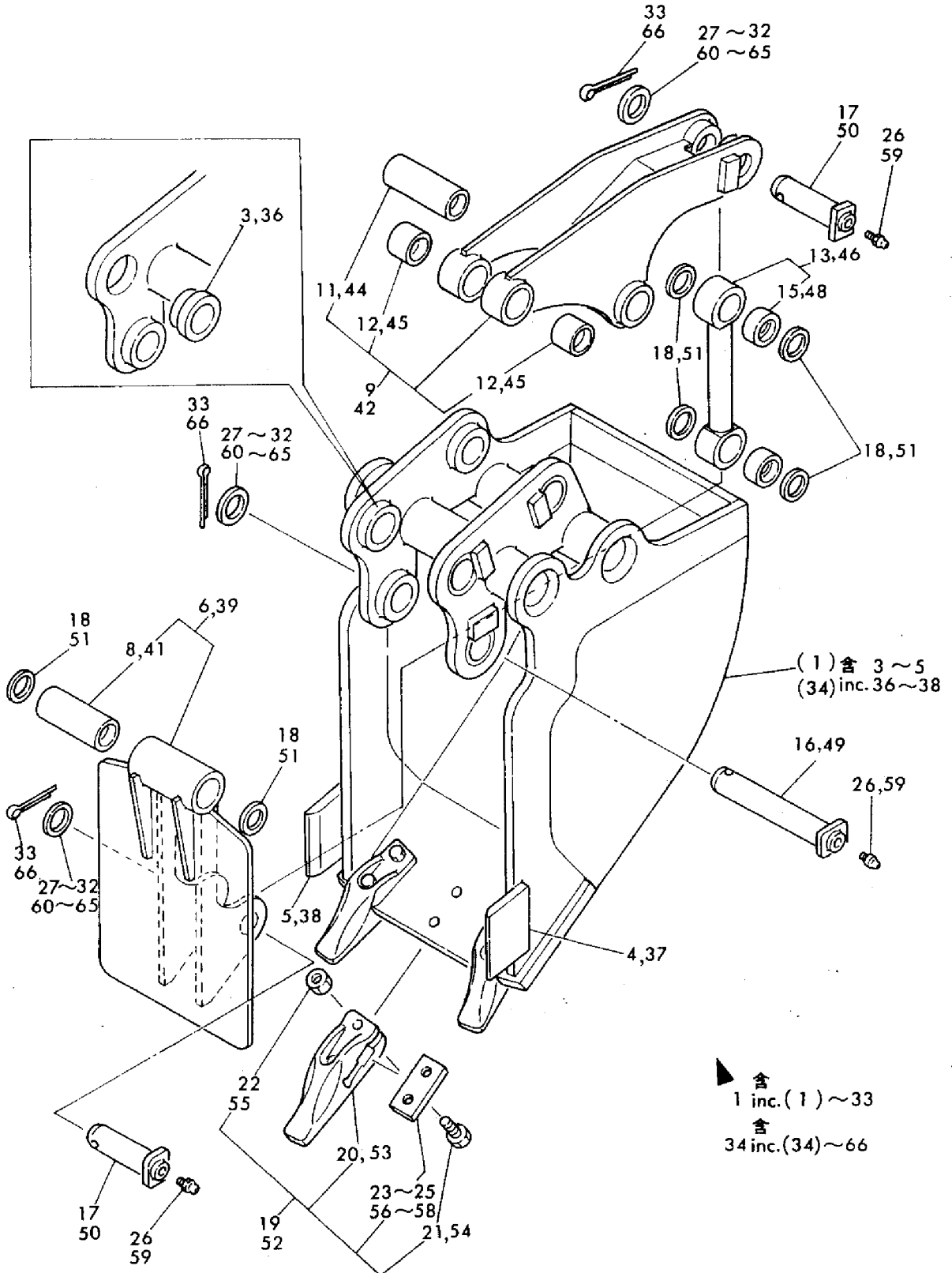
Fig. 101 エゼクター付バケット (オプション), YB201U (Z) ヨウ EJECTOR BUCKET (OPTIONAL), FOR MODEL YB201U(Z)
