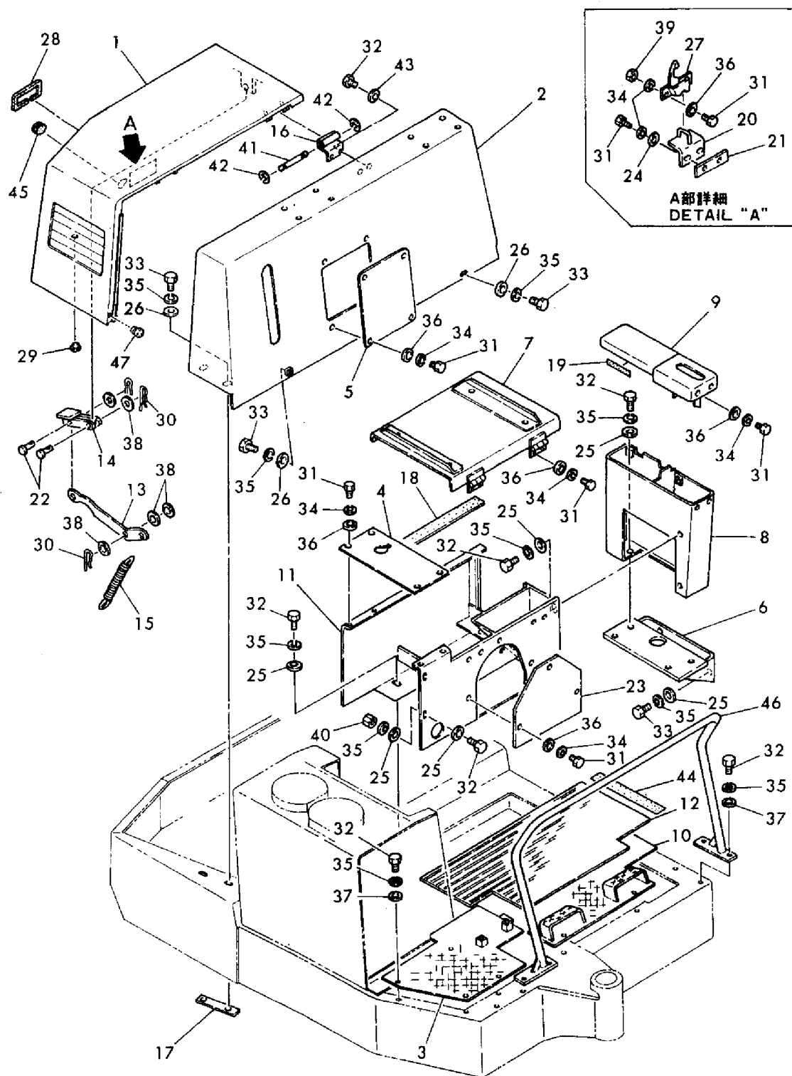
Fig. 41 ボンネット関係 (キャノピー仕様), YB201U ヨウ BONNET RELATION (CANOPY SPEC.), FOR MODEL YB201U
