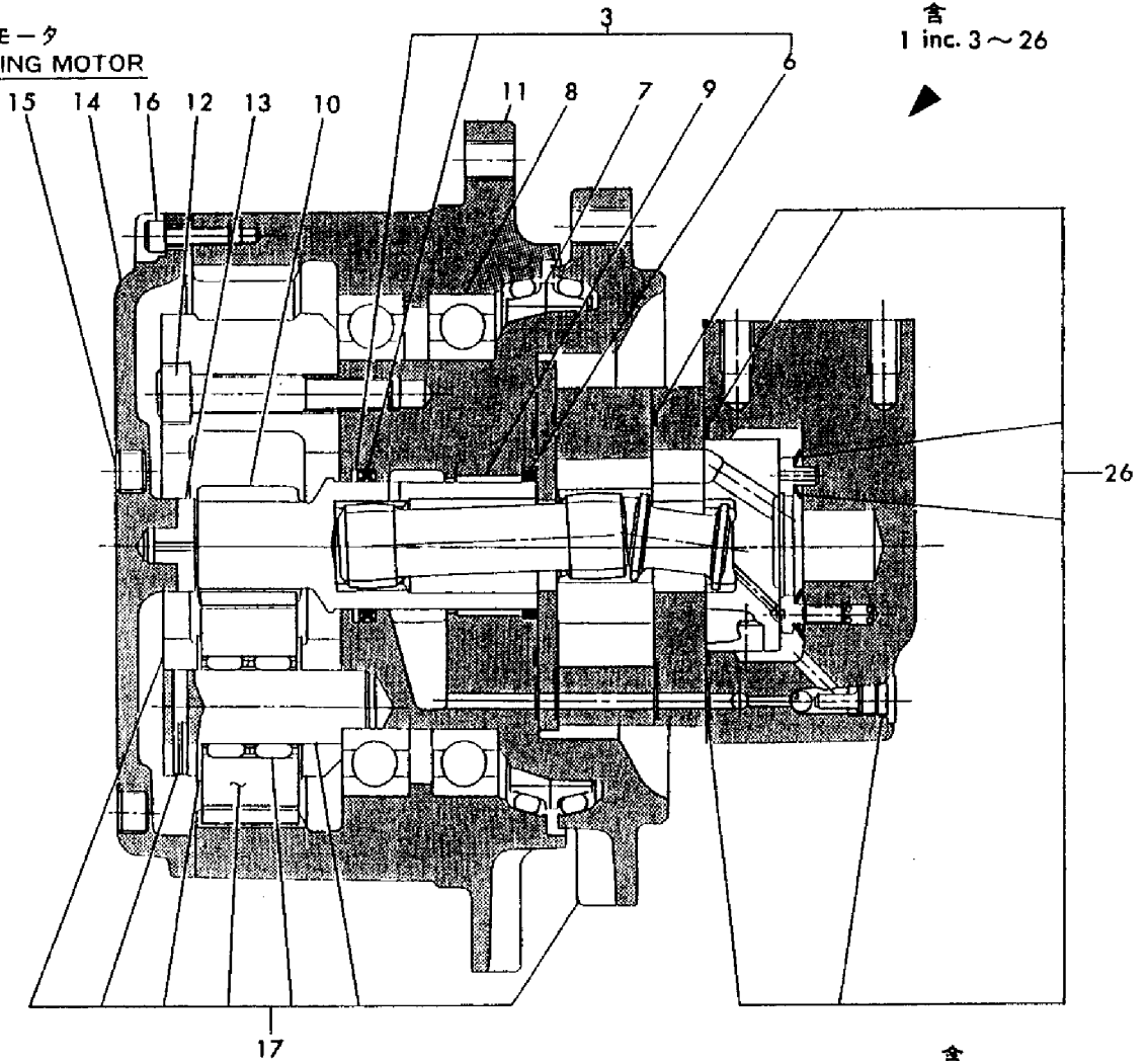
Fig. 78 油圧モータ (走行 & 旋回) HYDRAULIC MOTOR (DRIV. & TURN)
