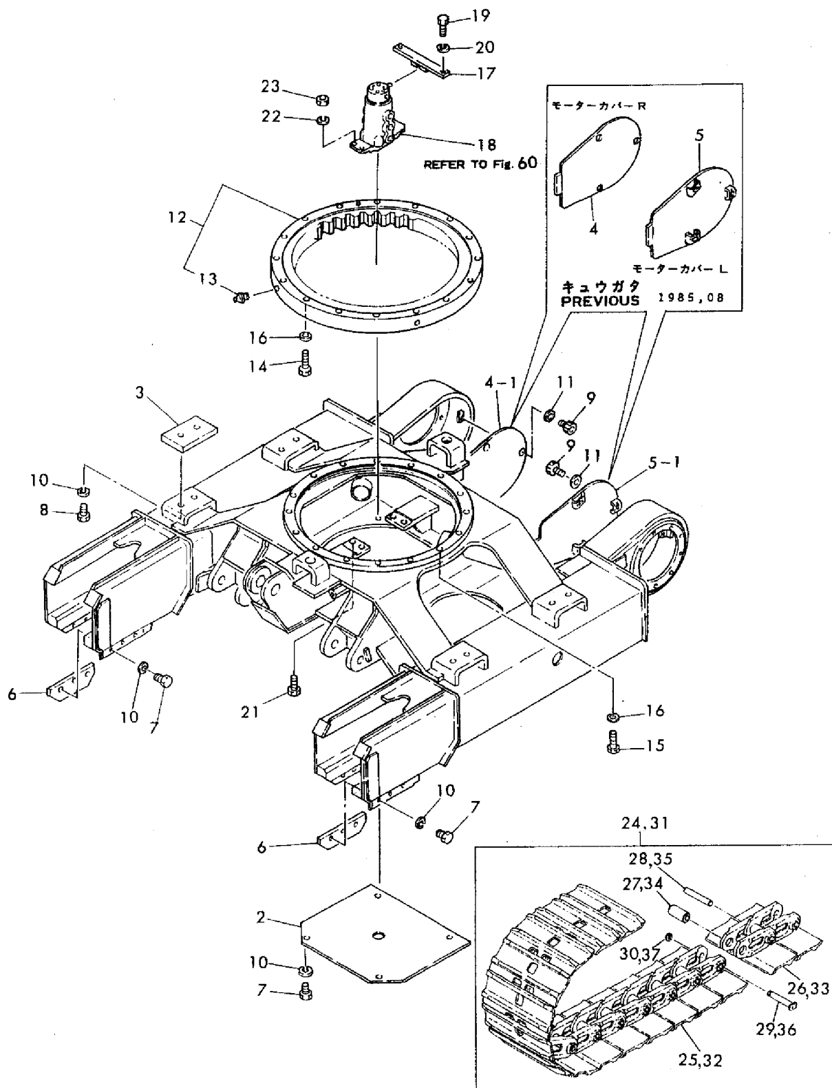
Fig. 1 ロアフレーム & トラックシュー LOWER FRAME & TRUCK SHOE
