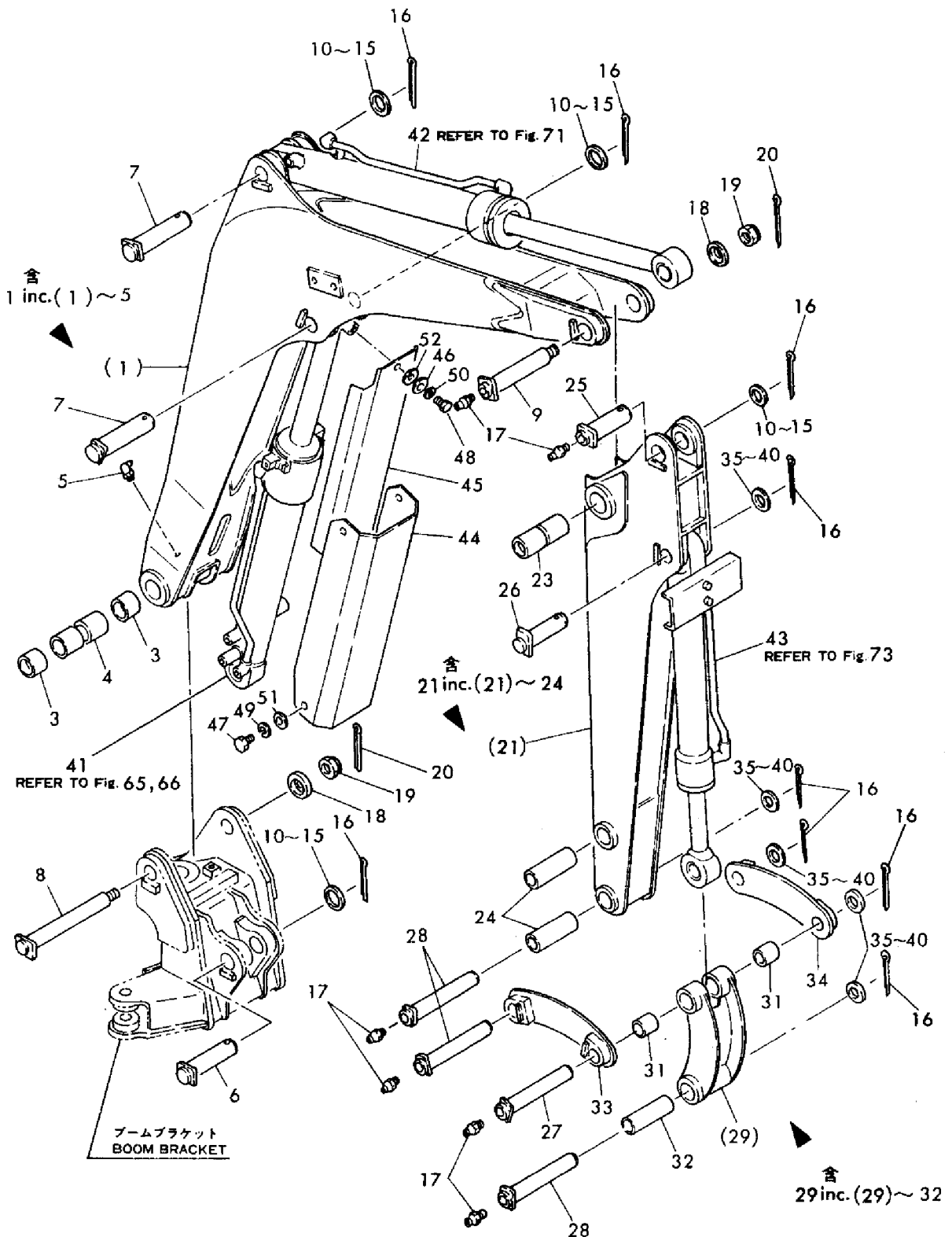
Fig. 49 ブーム & アーム (YB201Z ヨウ) BOOM & ARM (FOR MODEL YB201Z)
