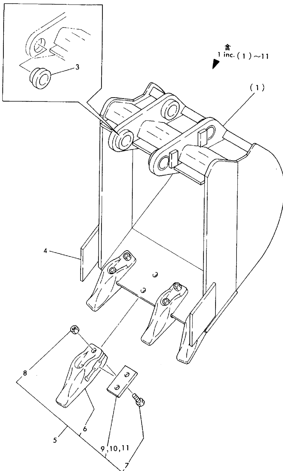
Fig. 52 バケットアッセンブリ BUCKET ASSY
