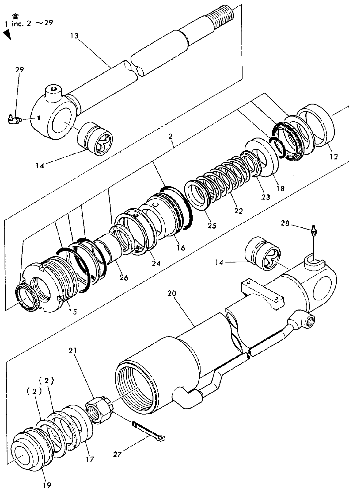
Fig. 70 メインブームシリンダ (YB201UZ ヨウ), M/# 00935 MAIN BOOM CYLINDER, FOR MODEL YB201UZ
