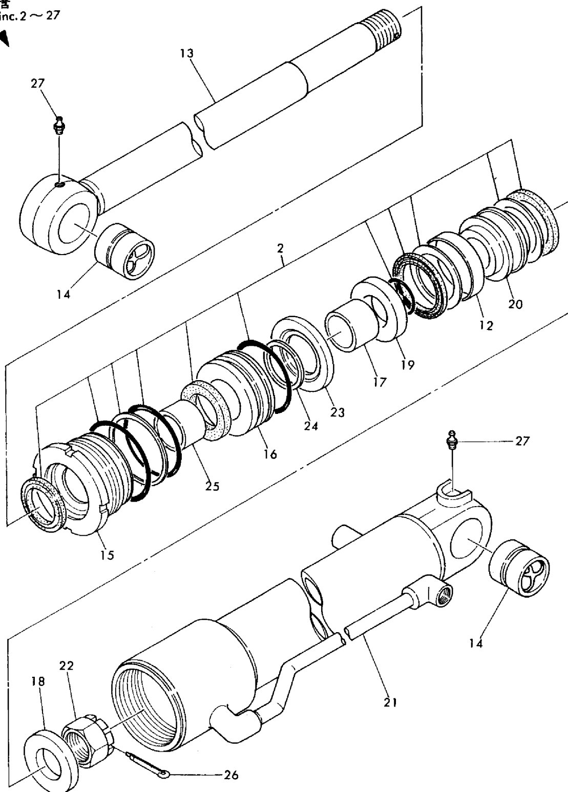
Fig. 67 メインブームシリンダ, YB201U ヨウ MAIN BOOM CYLINDER, FOR MODEL YB201U
