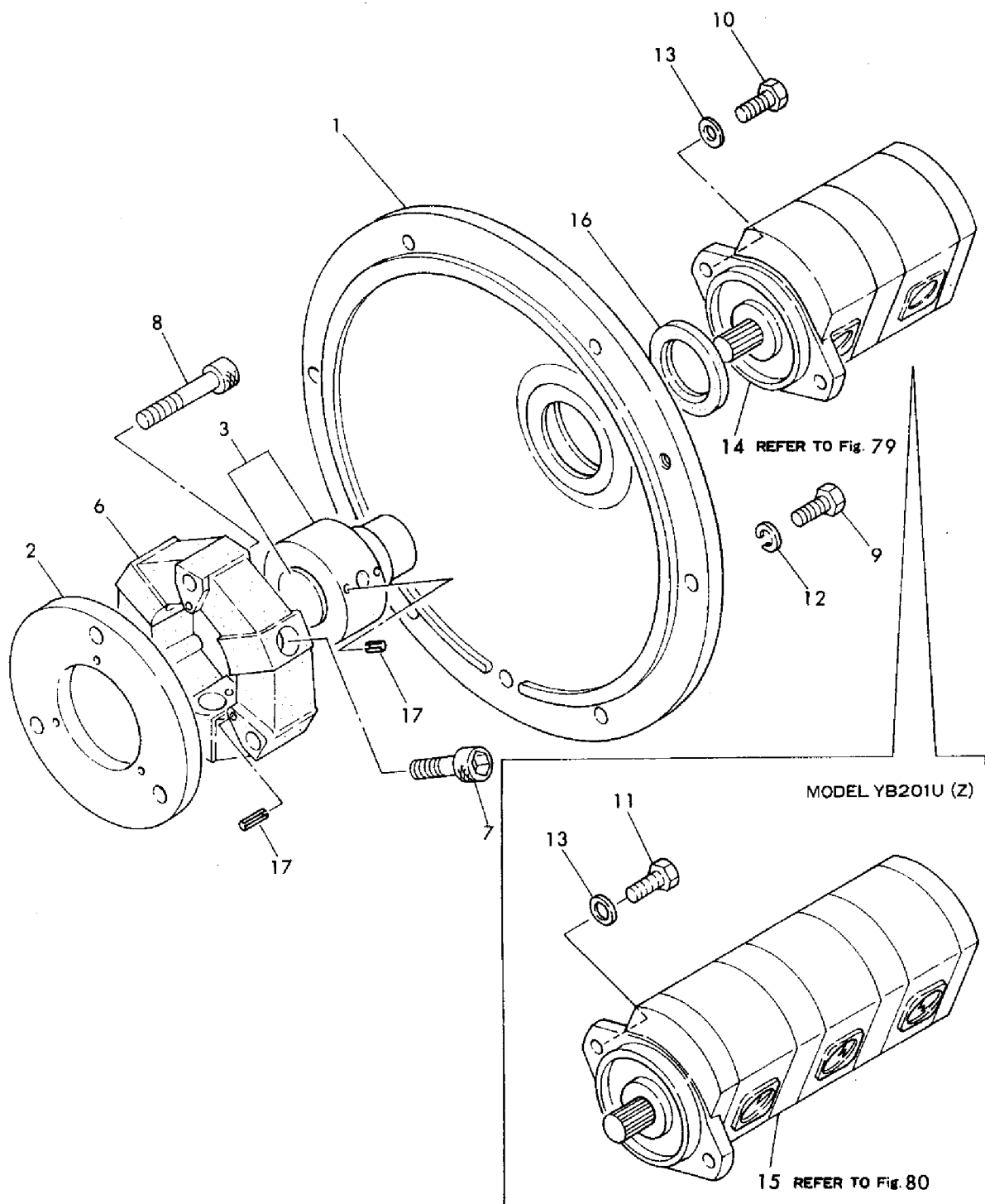
Fig. 36 ポンプ駆動 PUMP DRIVING
