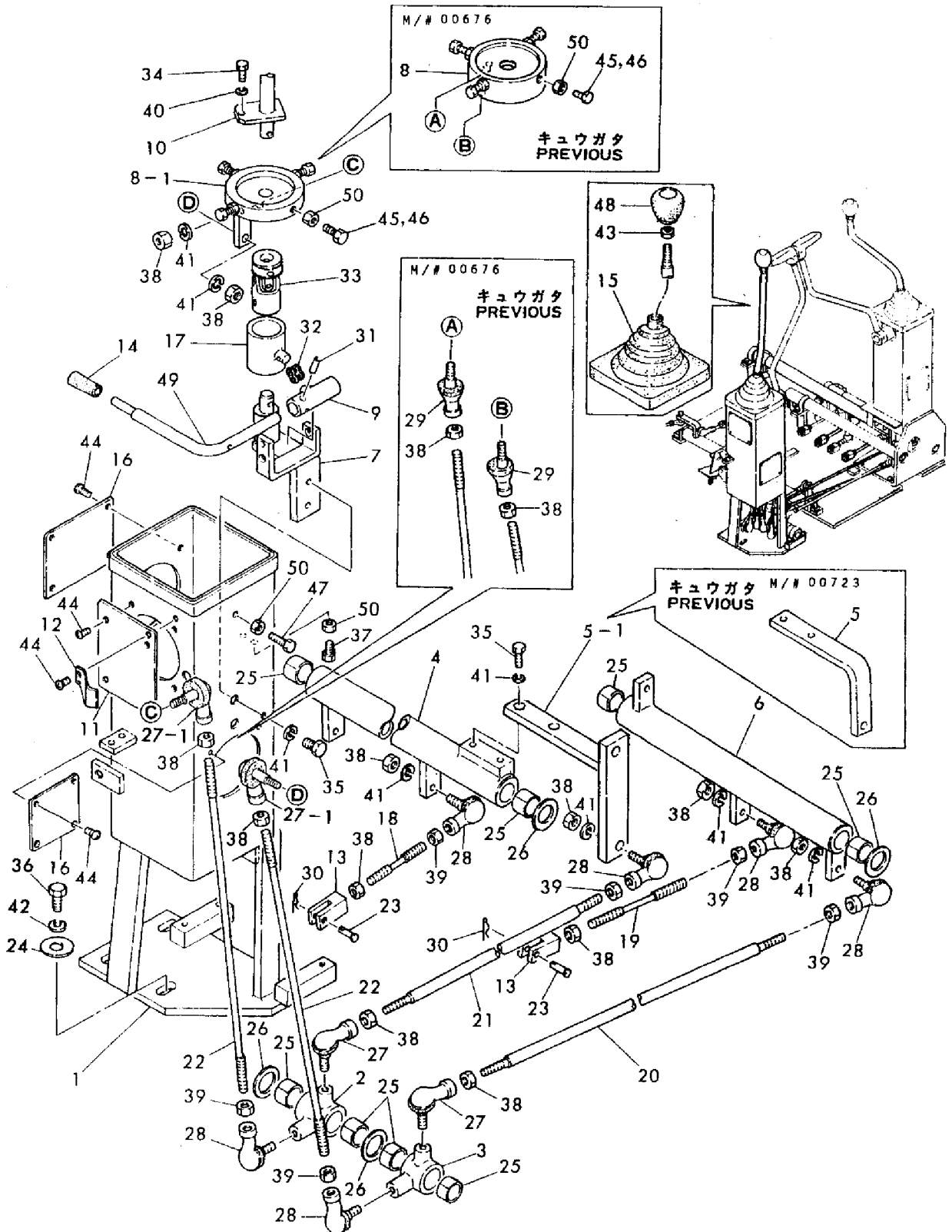
Fig. 16 コントロールレバー (操作用) 右, YB201U(Z) ヨウ CONTROL LEVER (OPERATION) RIGHT, FOR MODEL YB201U (Z)
