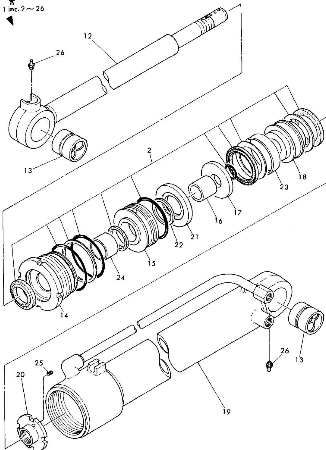
Fig. 76 スイングシリンダー, YB201U (Z) ヨウ SWING CYLINDER, FOR MODEL YB201U (Z)
