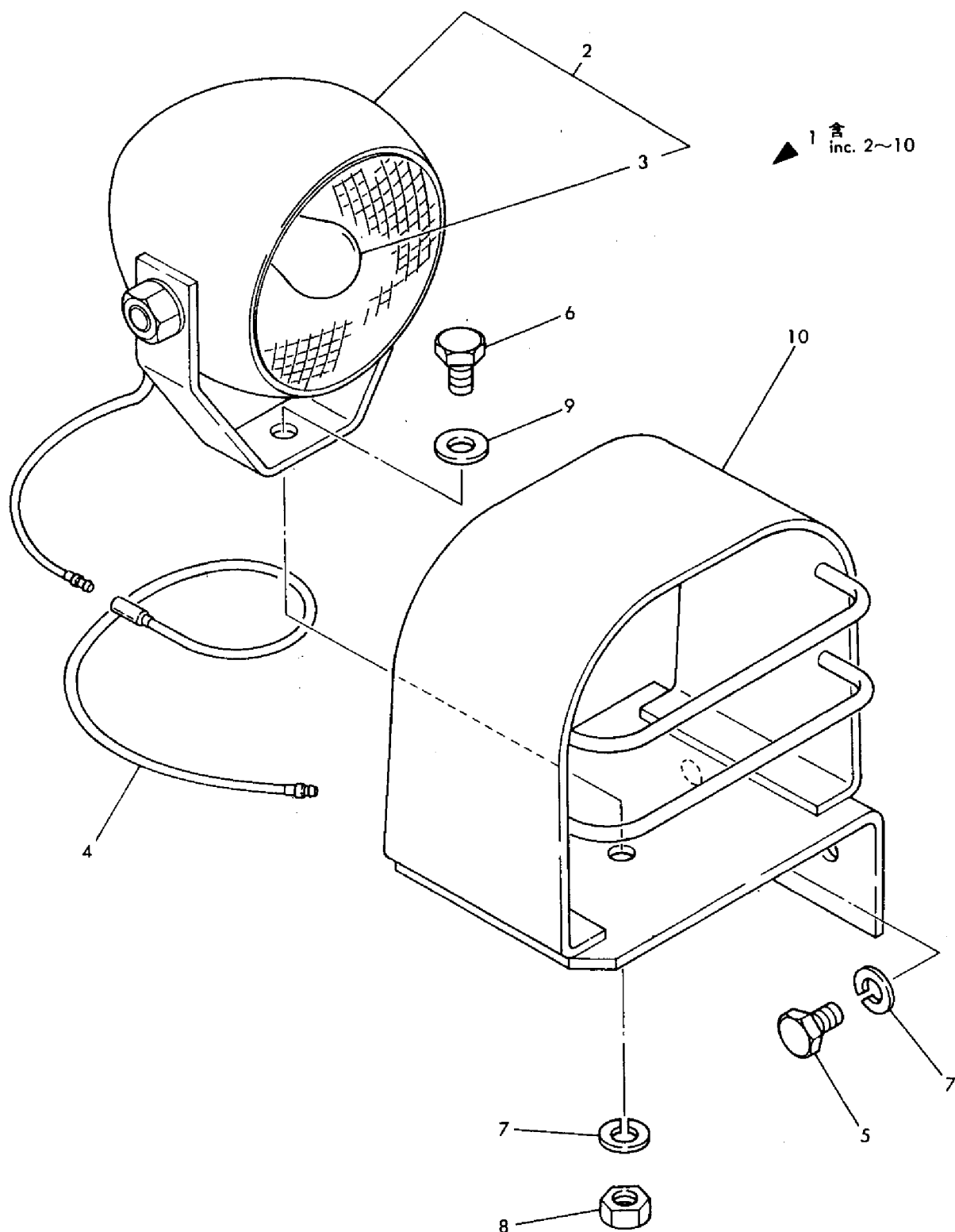
Fig. 89 ブームライト (オプション), YB201 (Z) ヨウ BOOM LAMP (OPTIONAL), FOR MODEL YB201 (Z)
