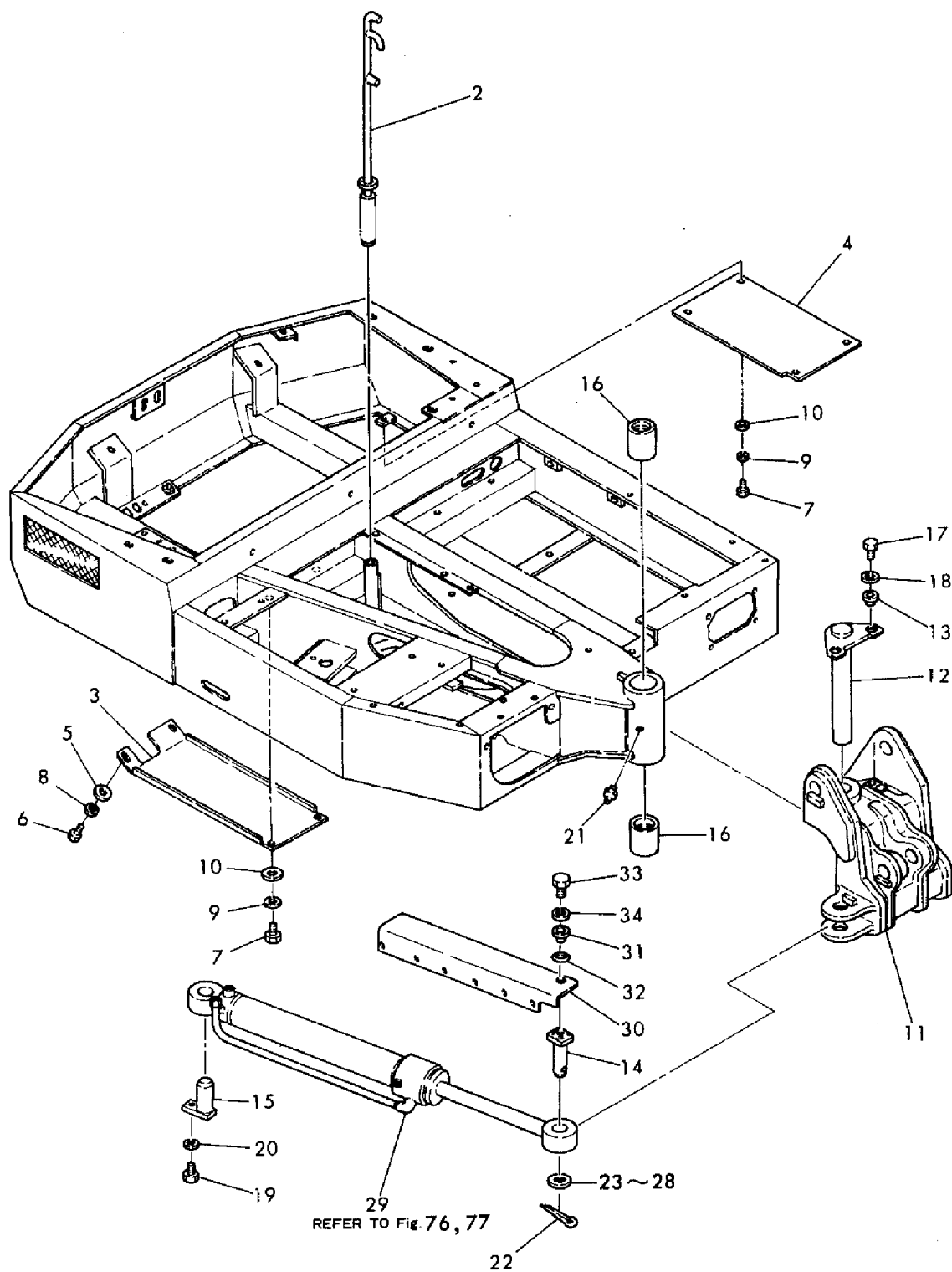
Fig. 12 本体 (YB201UZ ヨウ) MAIN FRAME (FOR MODEL YB201UZ).
