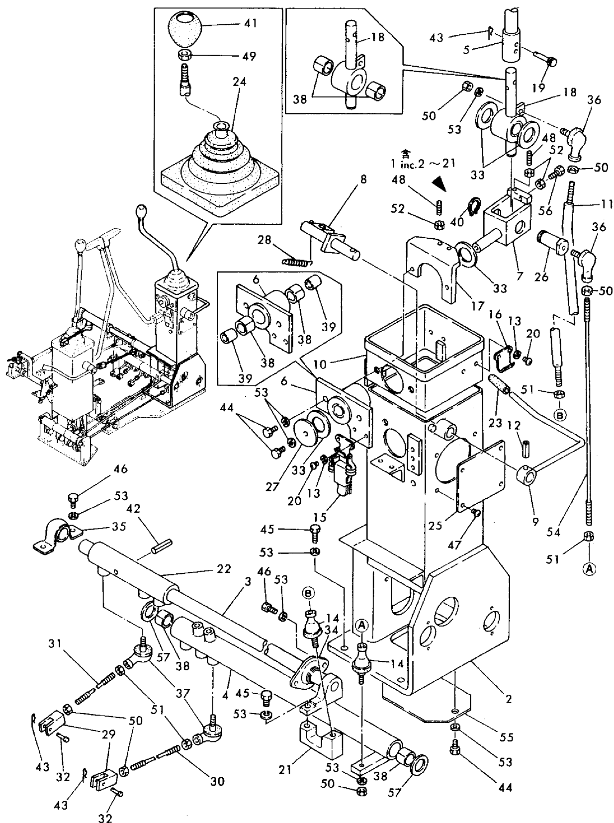
Fig. 86 クイックチェンジレバー (操作・左) オプション, YB201 (Z) ヨウ QUICK CHANGE LEVER (OPERATION, LEFT) OPTIONAL, FOR MODEL YB201 (Z)
