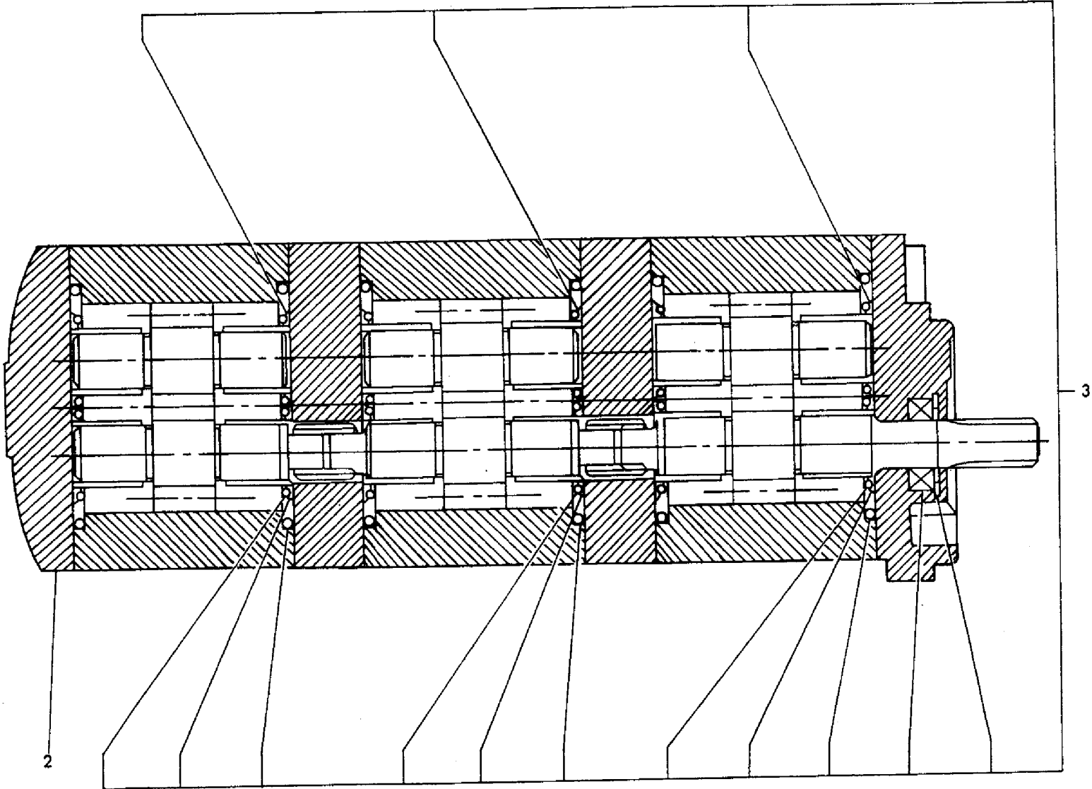
Fig. 80 油圧ポンプ (メイン), YB201U (Z) ヨウ HYDRAULIC PUMP (MAIN), FOR MODEL YB201U (Z)
