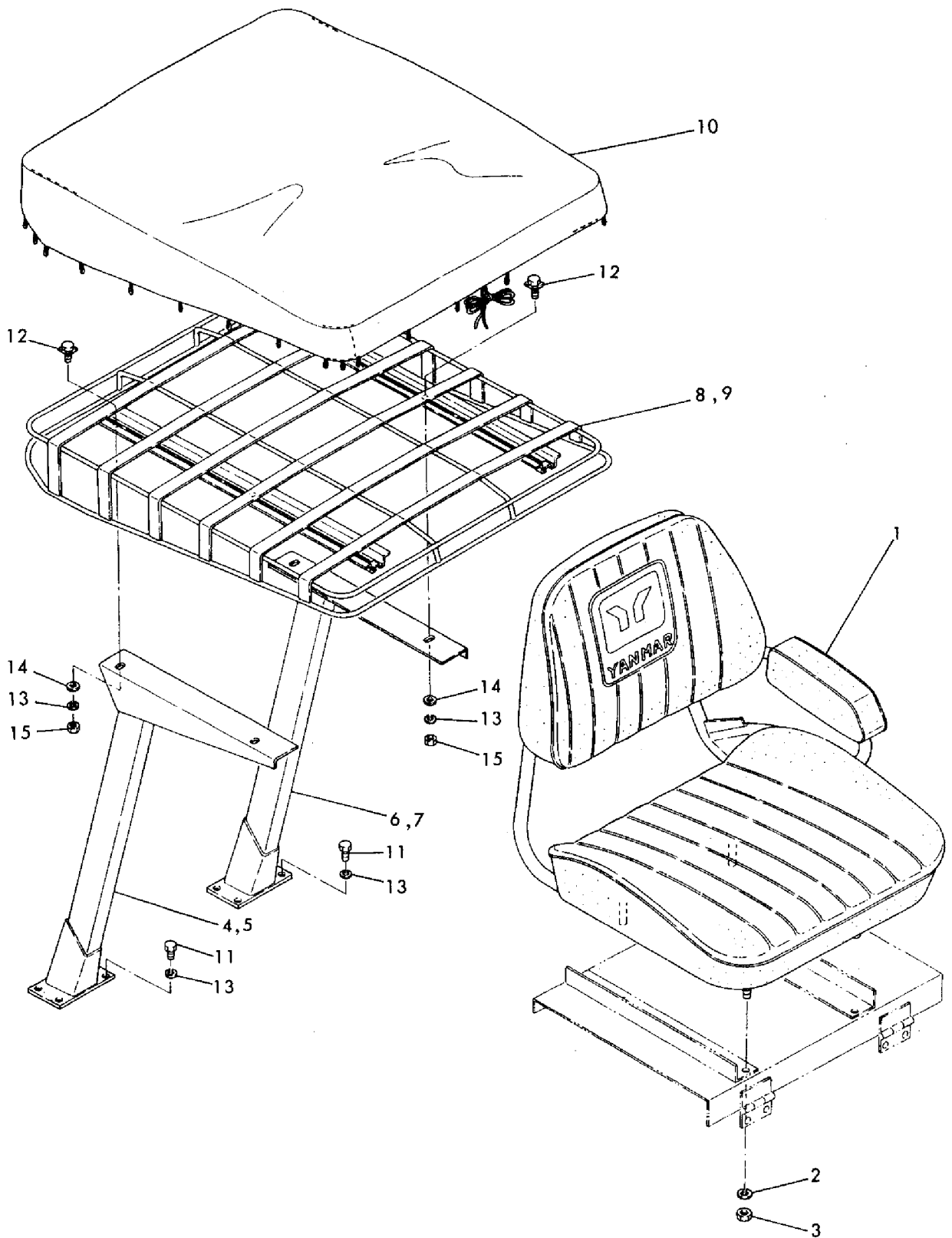
Fig. 45 キヤノピー & シート CANOPY & SHEAT
