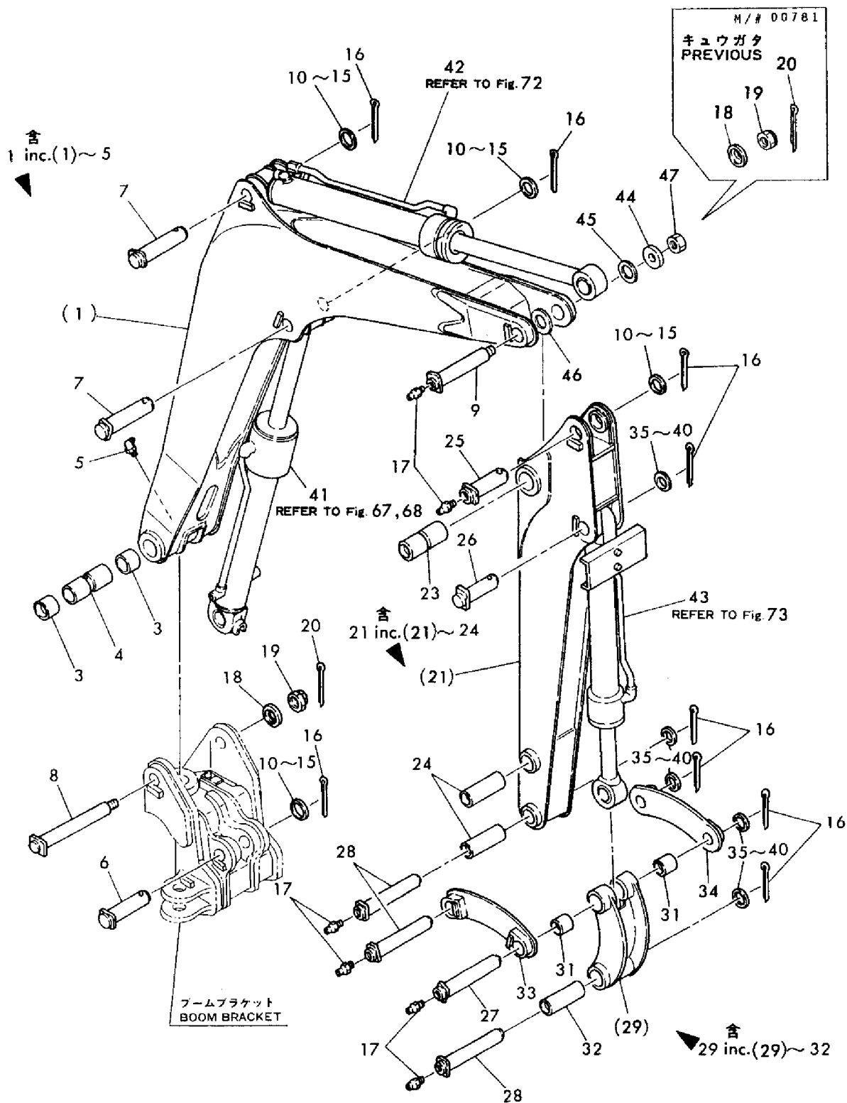
Fig. 50 ブーム & アーム (YB201U ヨウ) BOOM & ARM (FOR MODEL YB201U)
