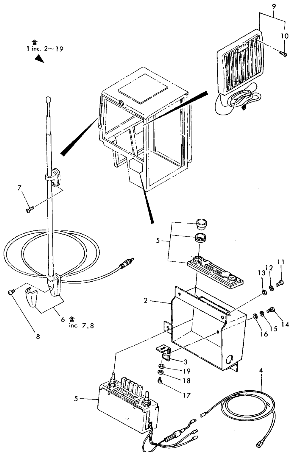
Fig. 87 ラジオ (オプション) YB201 ヨウ RADIO.....OPTIONAL (FOR MODEL YB201)
