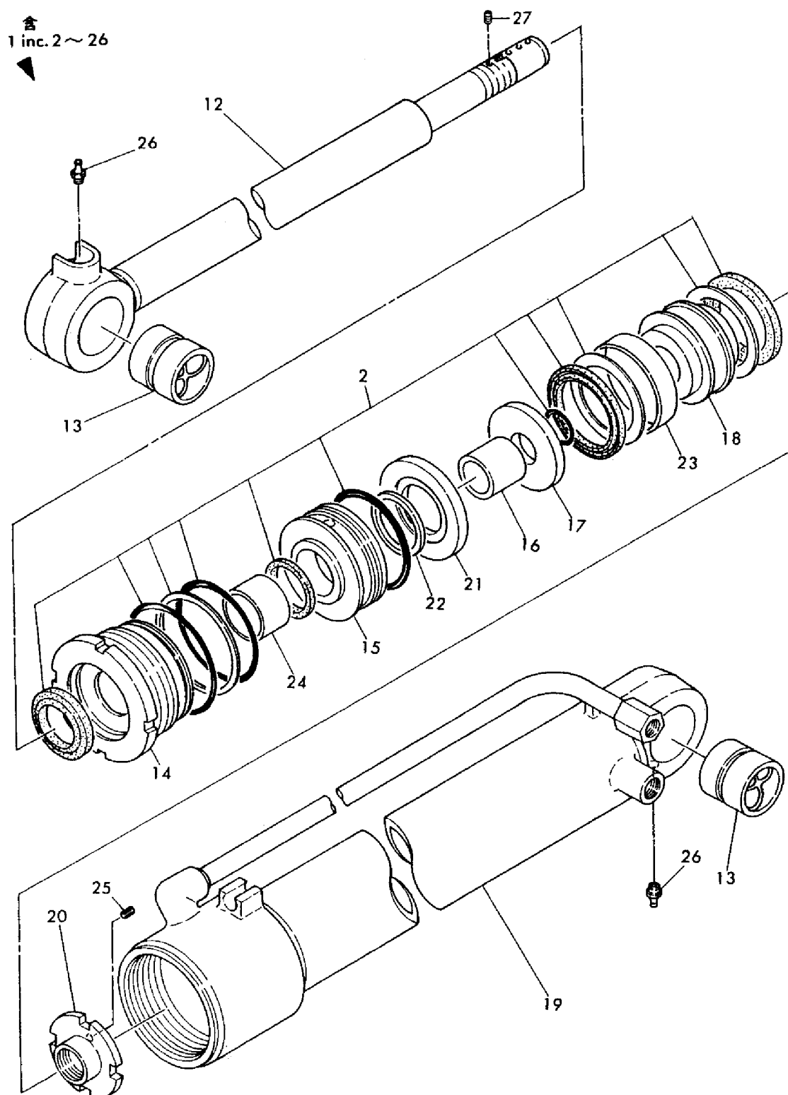
Fig. 77 スイングシリンダー(YB201UZヨウ), M/# 00956 SWING CYLINDER, FOR MODEL YB201U (Z)
