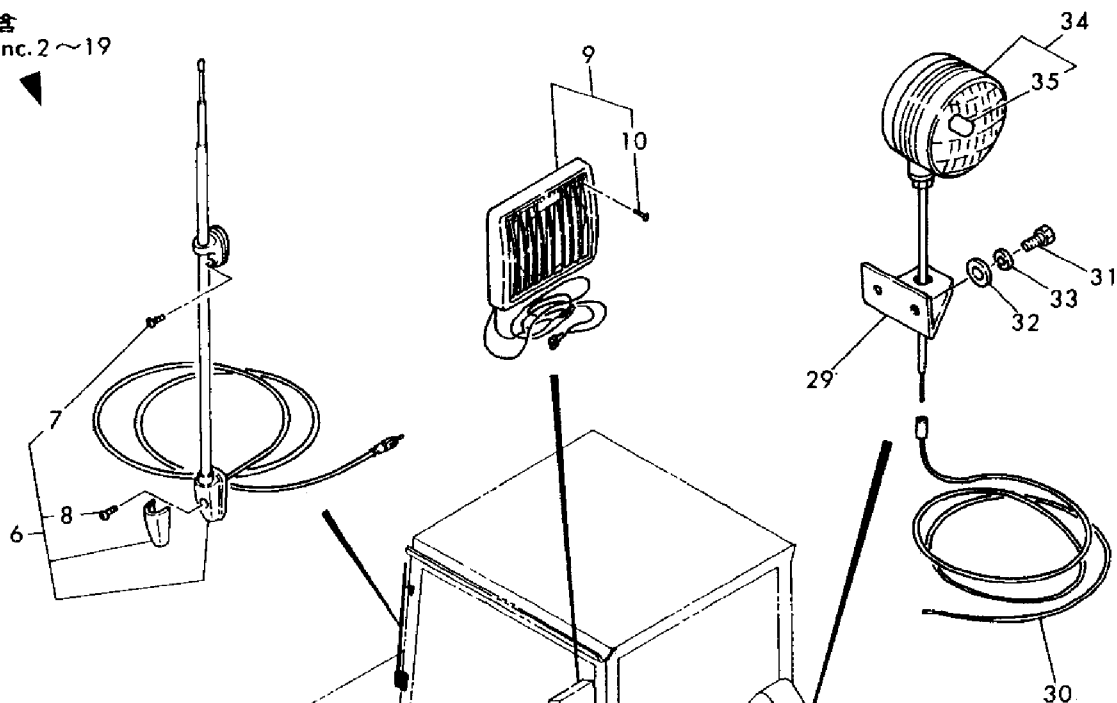
Fig. 88 電装品 (オプション), YB201U ヨウ ELECTRIC PART (OPTIONAL), FOR MODEL YB201U
