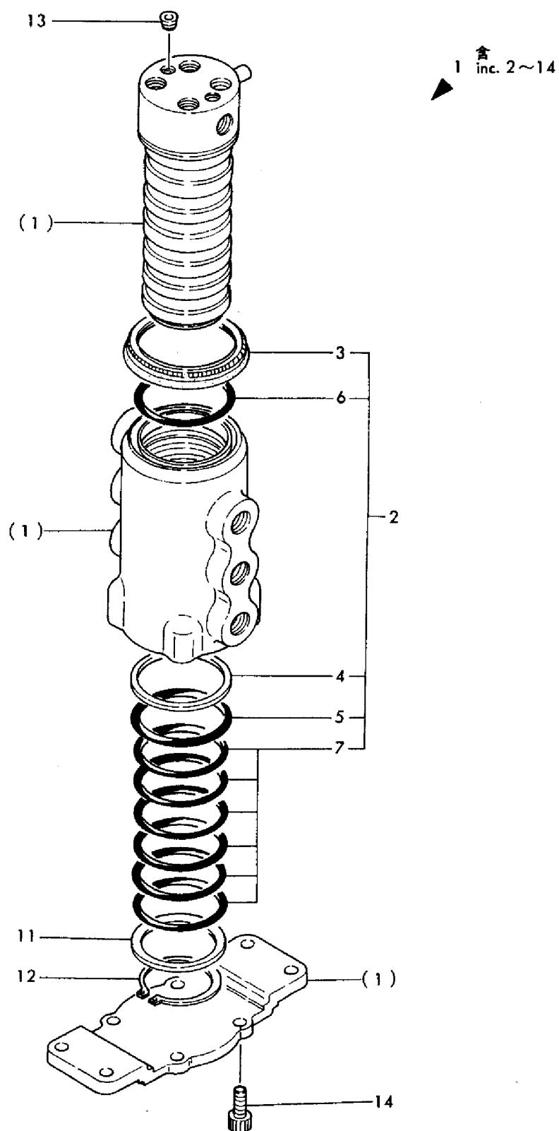
Fig. 60 スイベルジョイント SWIVEL JOINT
