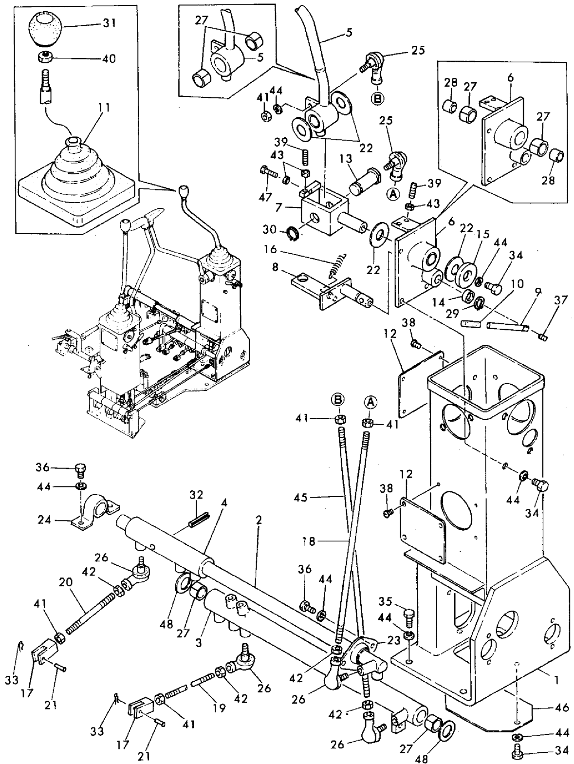
Fig. 17 コントロールレバー (操作用) 左, YB201 (Z) ヨウ CONTROL LEVER (OPERATION) LEFT, FOR MODEL YB201 (Z)
