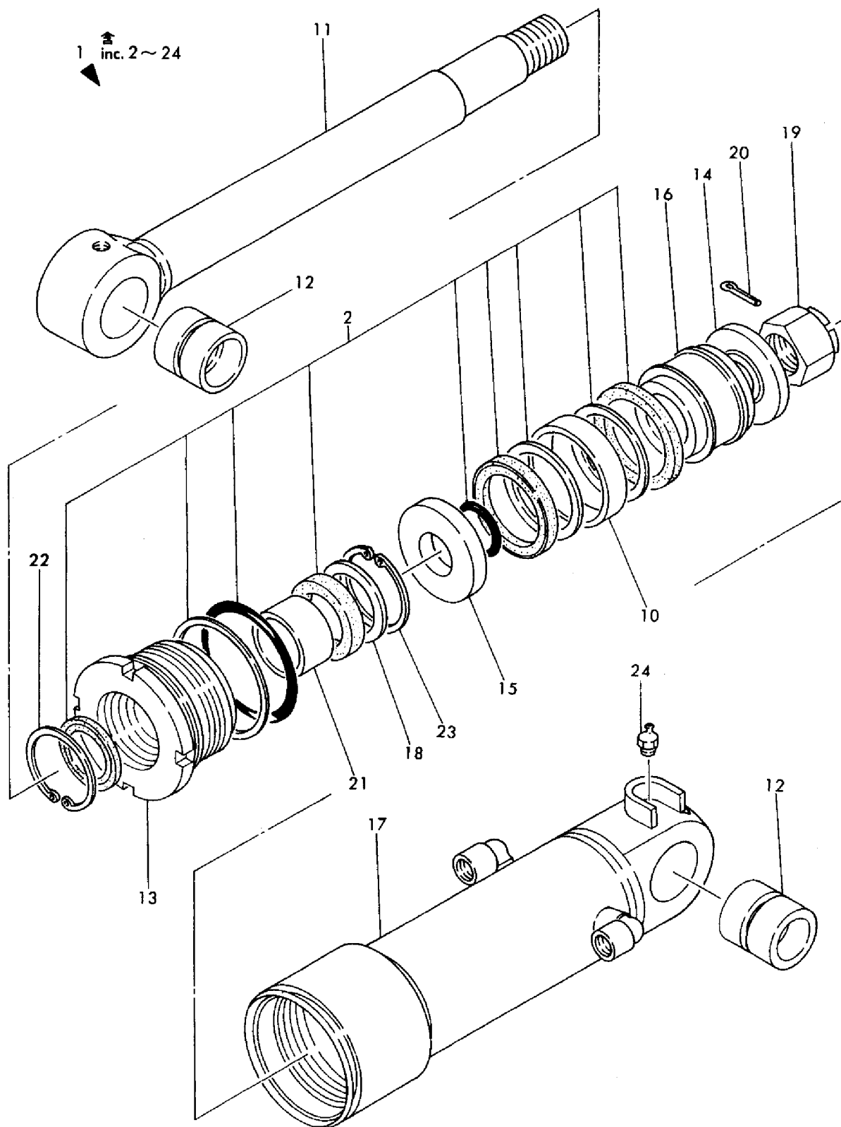
Fig. 74 ハイドバンシリンダー BLADE CYLINDER
