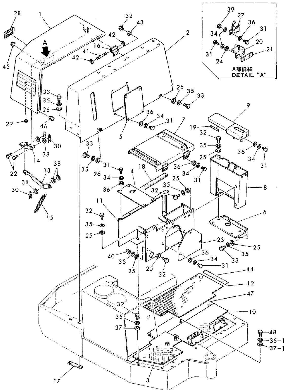
Fig. 42 ボンネット関係 (キャビン仕様), YB201U ヨウ, オプション BONNET RELATION (CABIN SPEC.), FOR MODEL YB201U .....OPTIONAL
