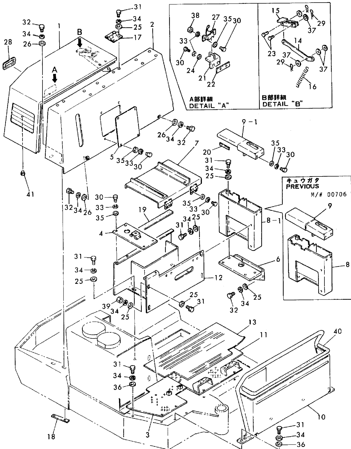
Fig. 43 ボンネット関係, YB201Z ヨウ BONNET RELATION, FOR MODEL YB201Z
