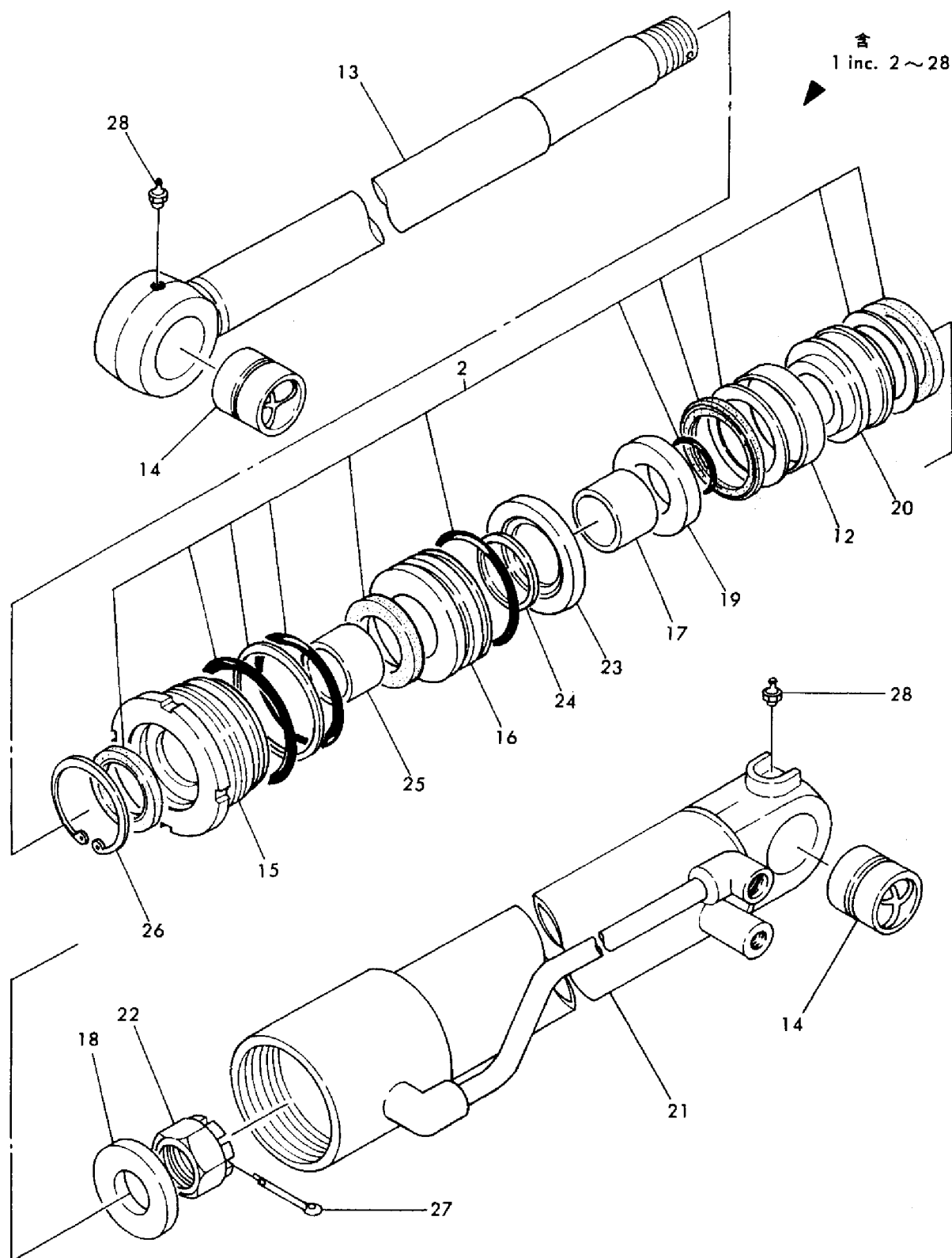
Fig. 64 メインブームシリンダー (YB20I ヨウ) MAIN BOOM CYLINDER (FOR MODEL YB20I)
