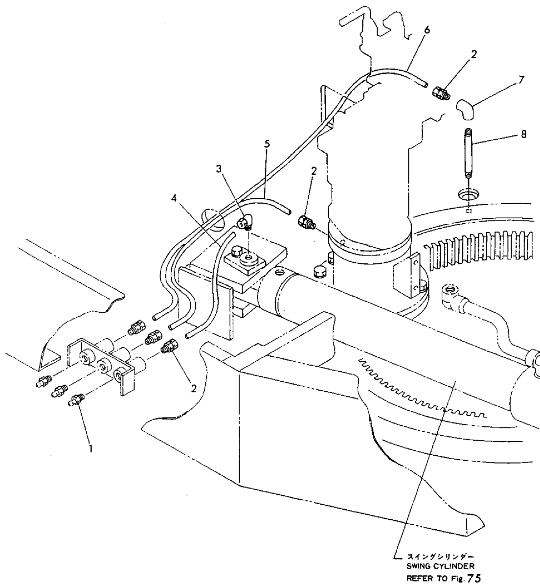
Fig. 28 グリース配管, YB201 (Z) ヨウ GREASE PIPING, FOR MODEL YB201 (Z)
