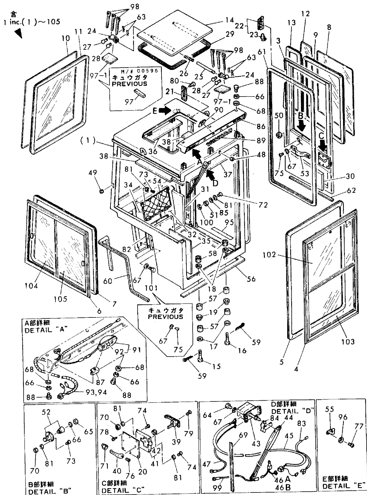
Fig. 47 スチールキャビン (オプション), YB201U ヨウ STEEL CABIN (OPTIONAL), FOR MODEL YB201U
