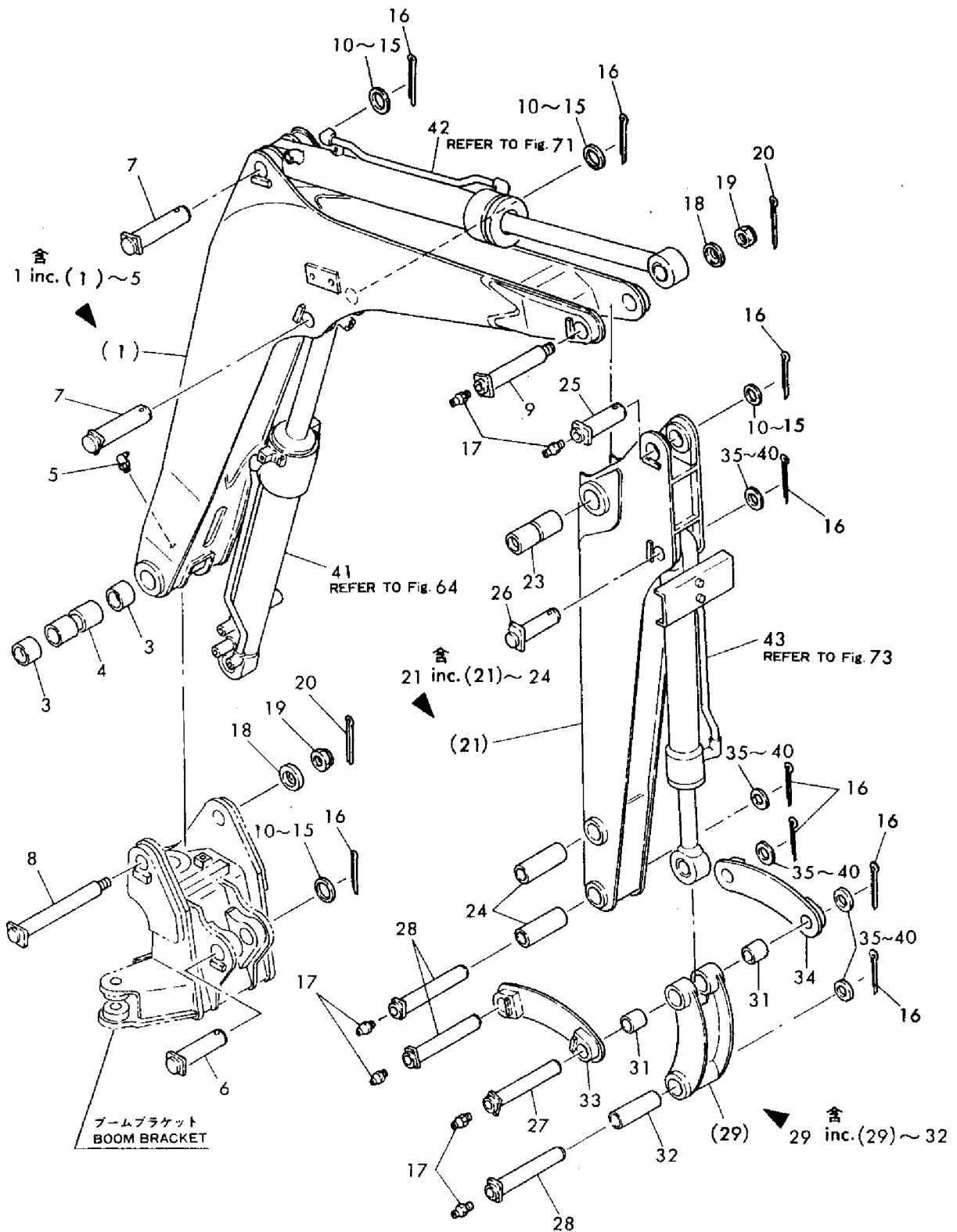
Fig. 48 ブーム & アーム (YB20I ヨウ) BOOM & ARM (FOR MODEL YB20I)
