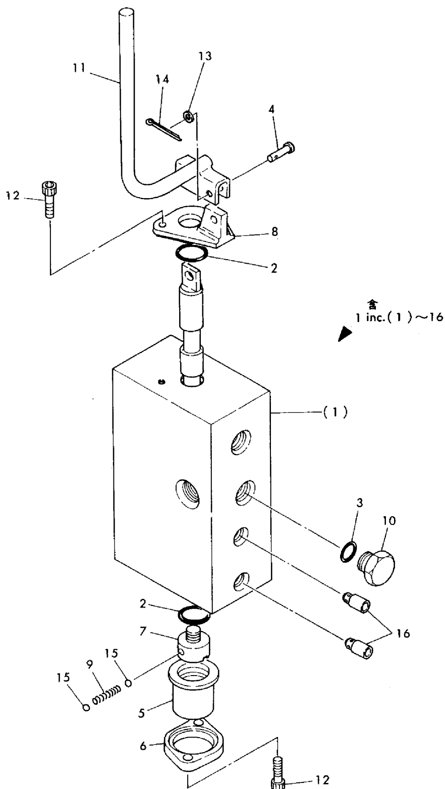
Fig. 95 セレクターバルブ (オプション), YB201U (Z) ヨウ SELECTOR VALVE (OPTIONAL), FOR MODEL YB201U (Z)
