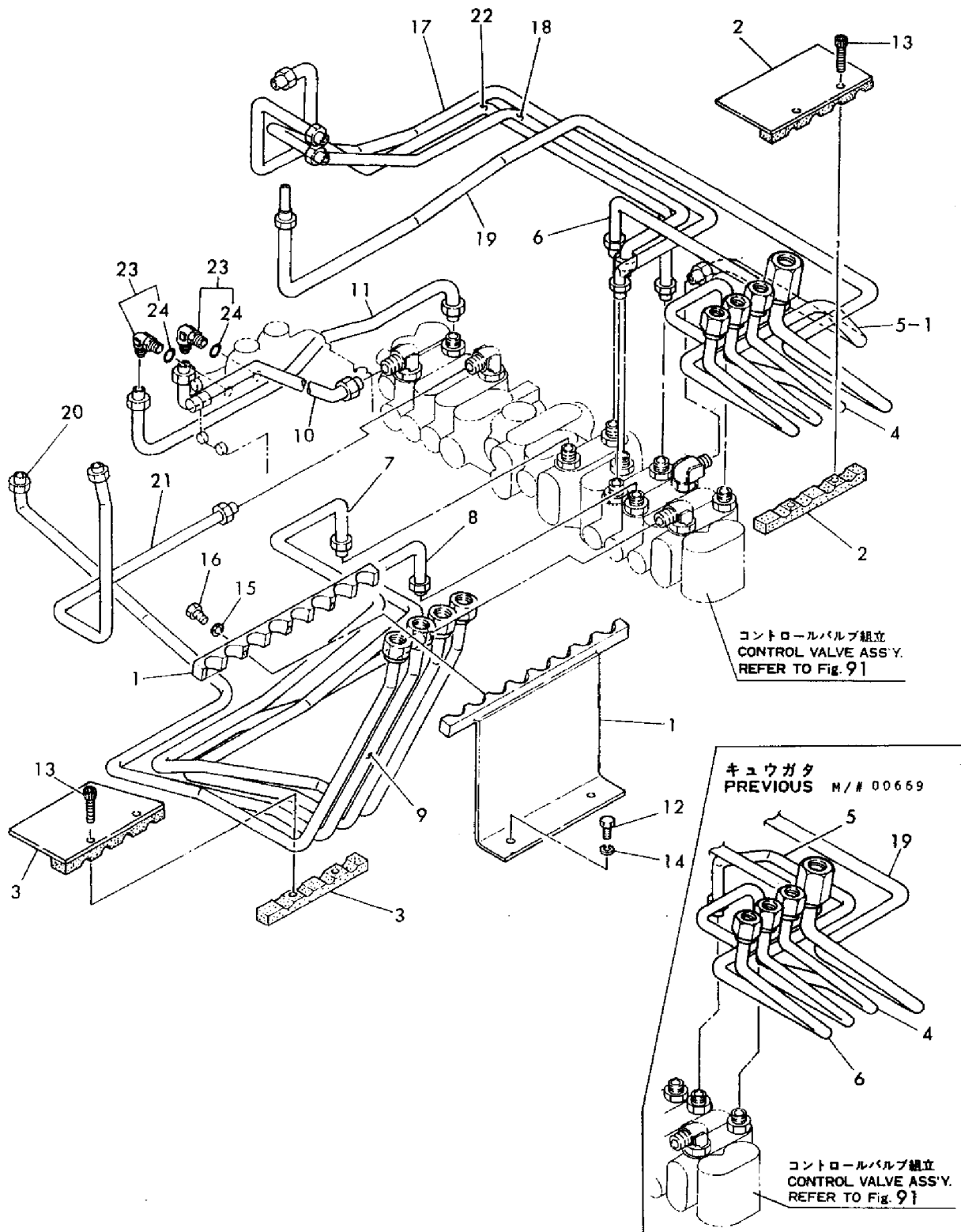
Fig. 93 上部油圧配管 (2), オプション, YB201U (Z) ヨウ UPPER HYDRAULIC OIL PIPING (2), (OPTIONAL), FOR MODEL YB201U (Z)
