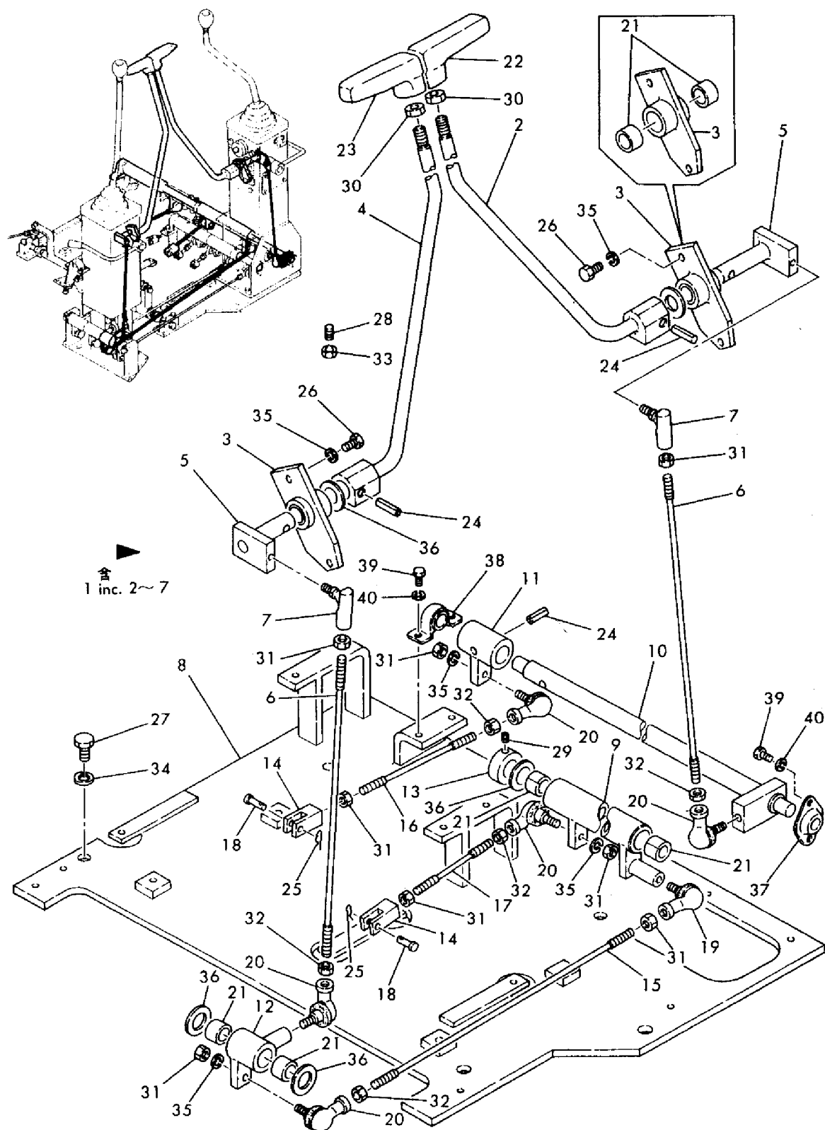
84 クイックチェンジレバー (走行) オプション, YB201 (Z) ヨウ Fig. 84 QUICK CHANGE LEVER (DRIV.) OPTIONAL, FOR MODEL YB201 (Z)
