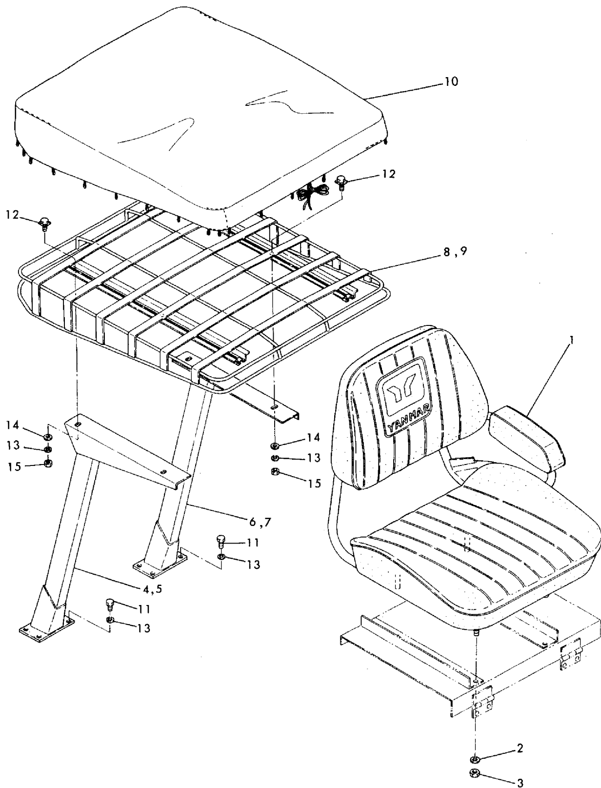
Fig. 45 キャンピー & シート CANOPY & SHEAT
