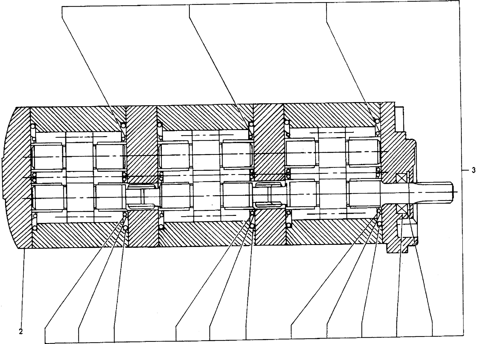
Fig. 80 油圧ポンプ (メイン), YB201U (Z) ヨウ HYDRAULIC PUMP (MAIN), FOR MODEL YB201U (Z)
