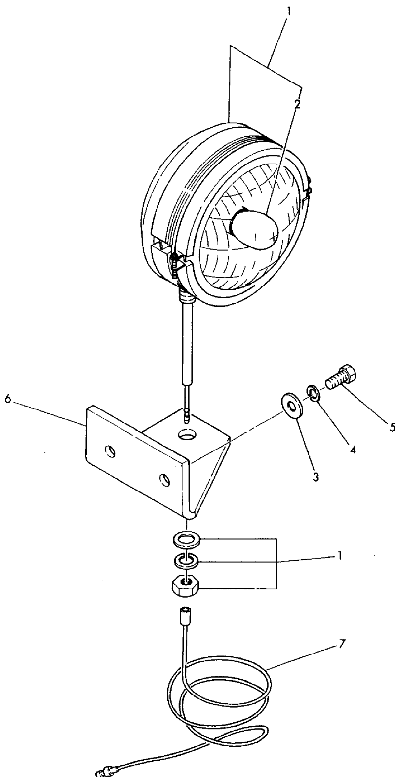
Fig. 90 ブームライト (オプション), YB201UZ ヨウ BOOM LAMP (OPTIONAL), FOR MODEL YB201UZ
