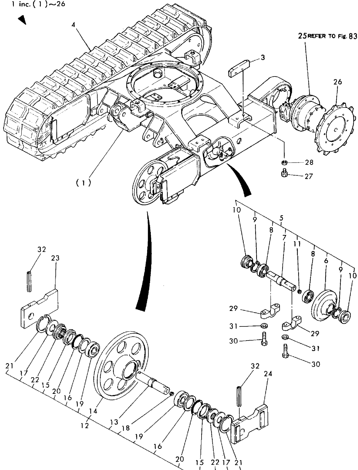
Fig. 81 ロアーマシーン (ゴムクローラ), オプション, YB201 (Z) ヨウ LOWER MACHINE (RUBBER CRAWLER), OPTIONAL FOR MODEL YB201 (Z)
