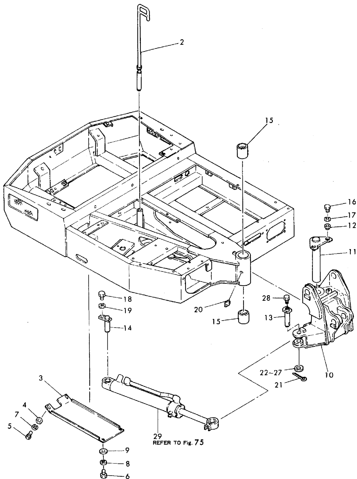
ホンタイ (YB201 ヨウ) Fig. 9 MAIN FRAME (FOR MODEL YB201)
