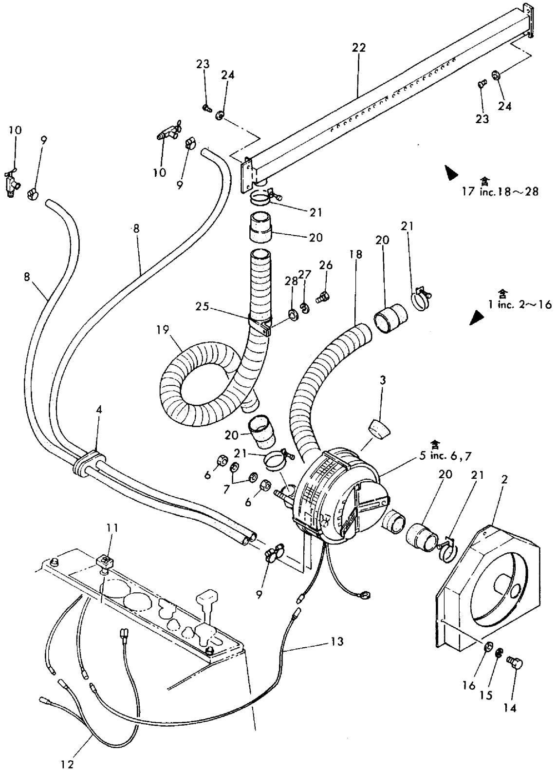
Fig. 98 ヒーター & デフロスター (オプション) YB201 ヨウ HEATER & DEFROSTER.....OPTIONAL (FOR MODEL YB201)
