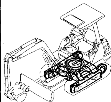
Fig.15 トラックフレーム & アイドラ (旧形) TRACK FRAME & IDLER (PREVIOUS)
