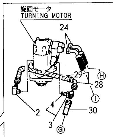
Fig. 49 油圧配管 (バルブ～スイベル～モータ) HYD. OIL PIPING (VALVE ~ SWIVEL ~ MOTOR)
