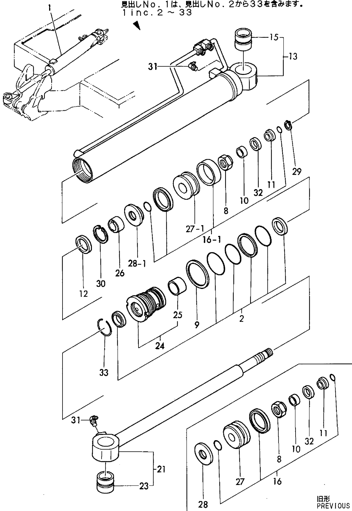
Fig. 35 スイグシリンダ (キャビン) SWING CYLINDER (CABIN)
