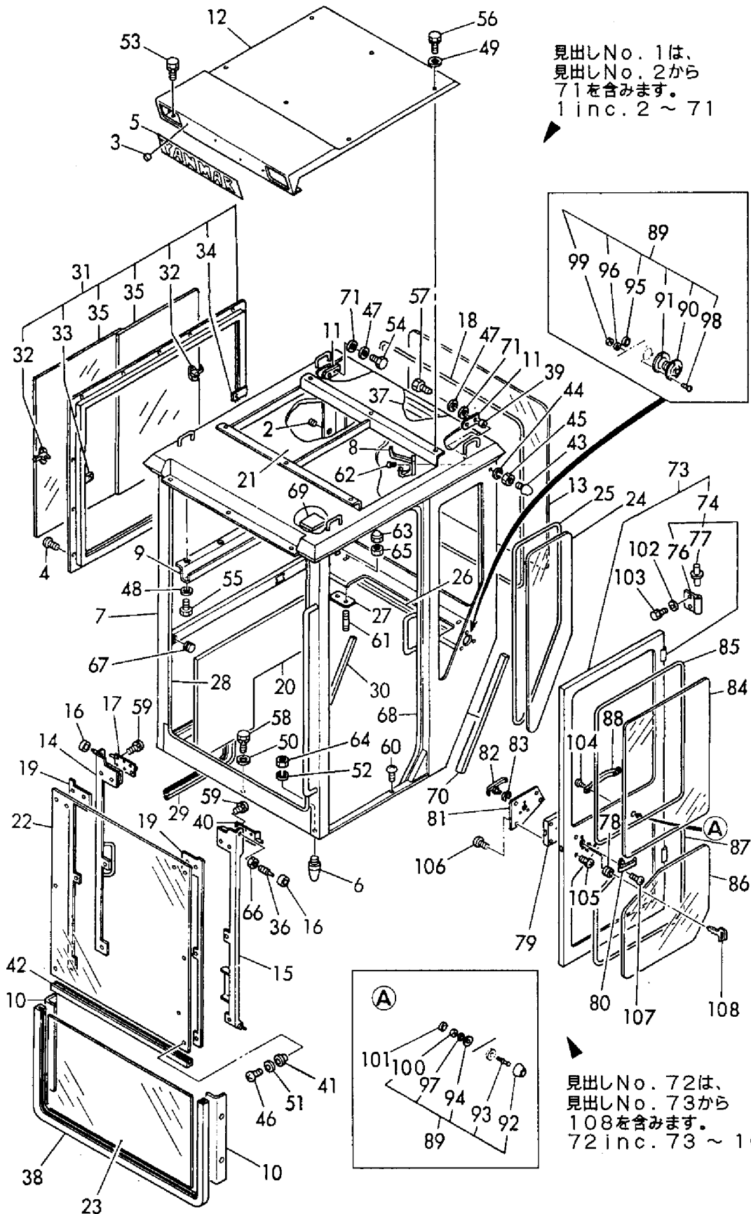
Fig. 30 キャビン CABIN
