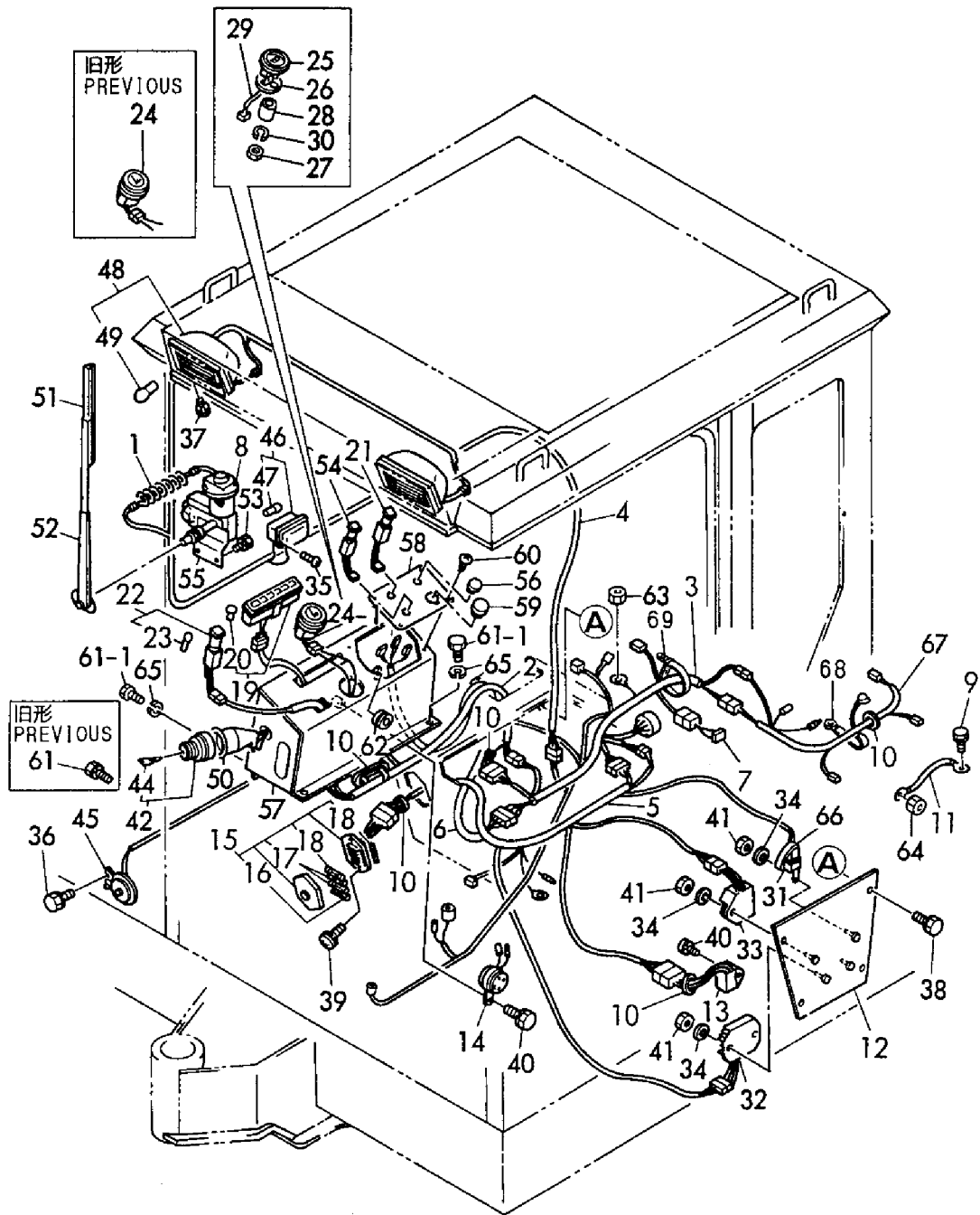
Fig. 10 電装品 (キャビン) ELECTRIC PART (CABIN)
