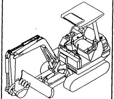
Fig.34 バケットシリンダ BUCKET CYLINDER
