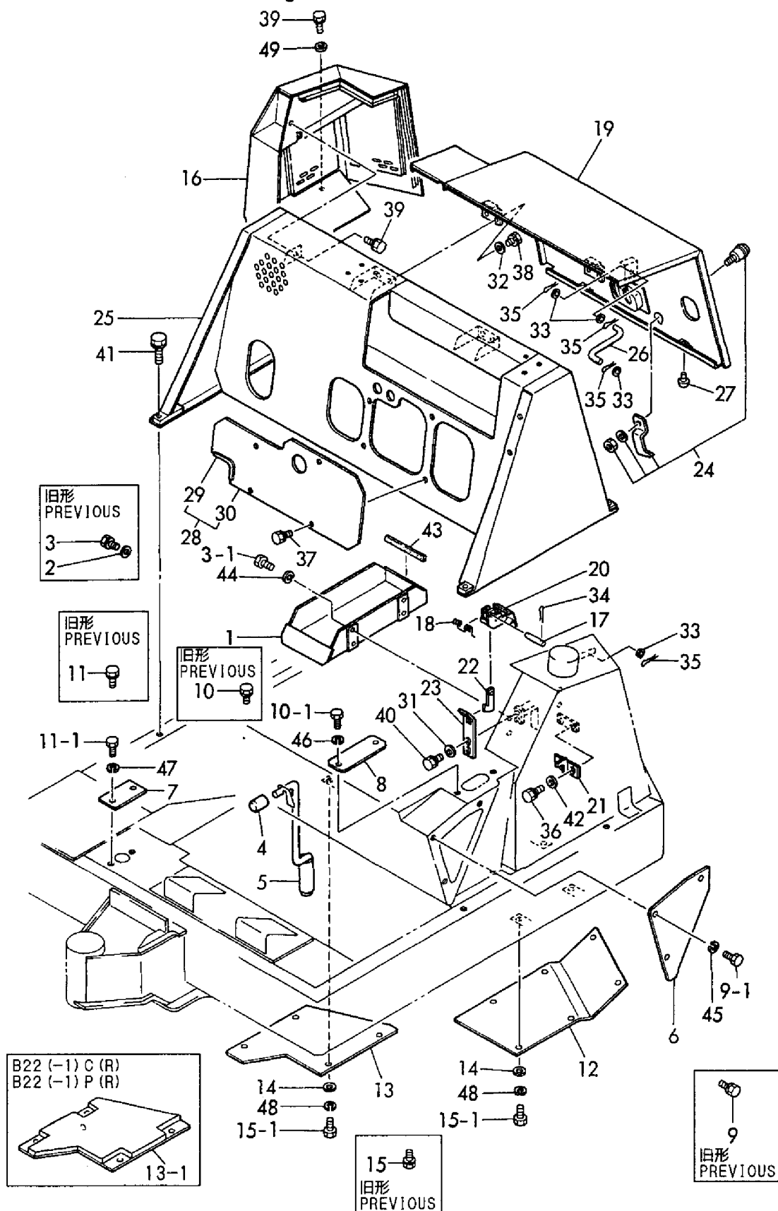
Fig. 27 ポンネット BONNET
