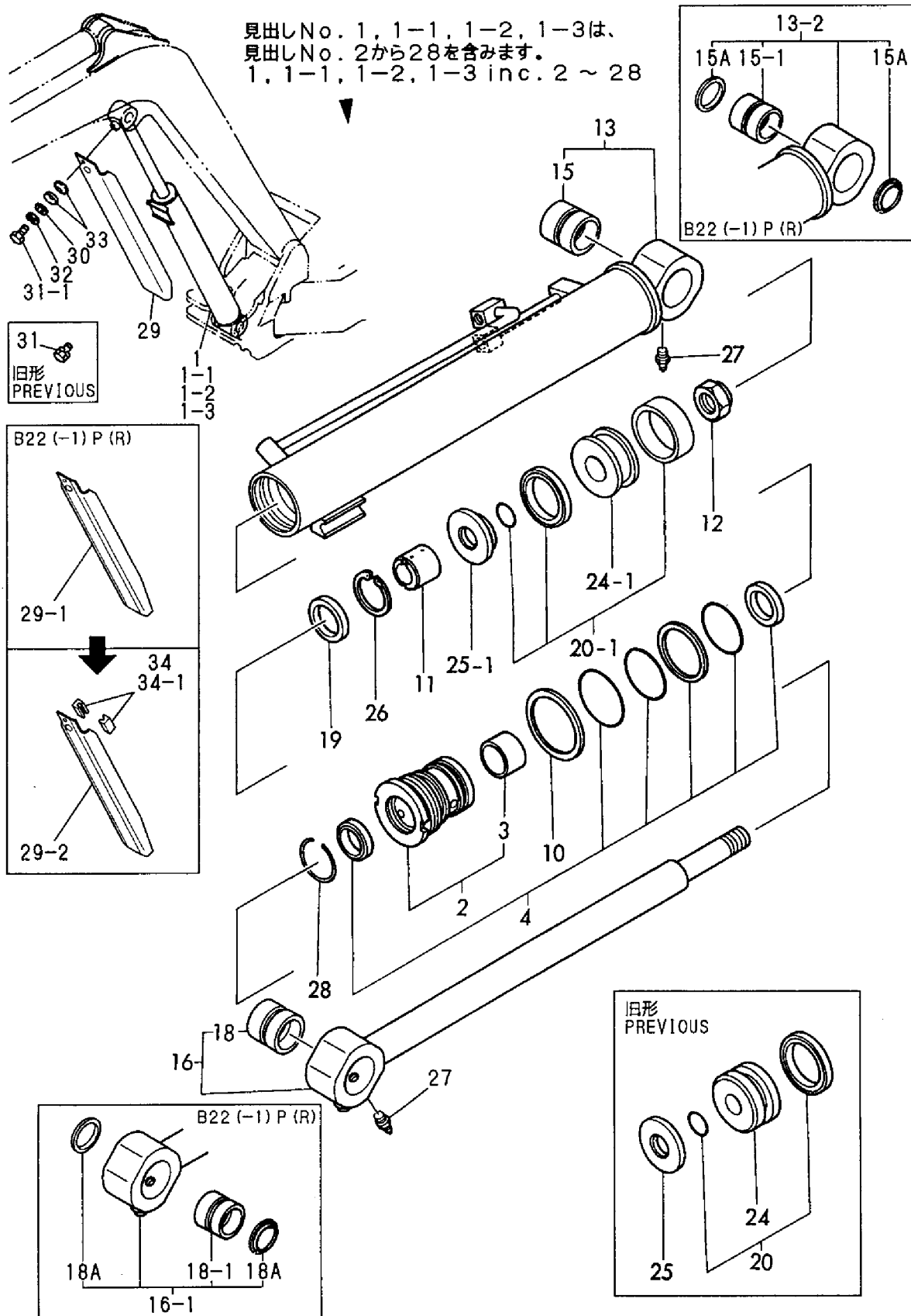
Fig. 32 ブームシリンダ (キャノピ) BOOM CYLINDER (CANOPY)
