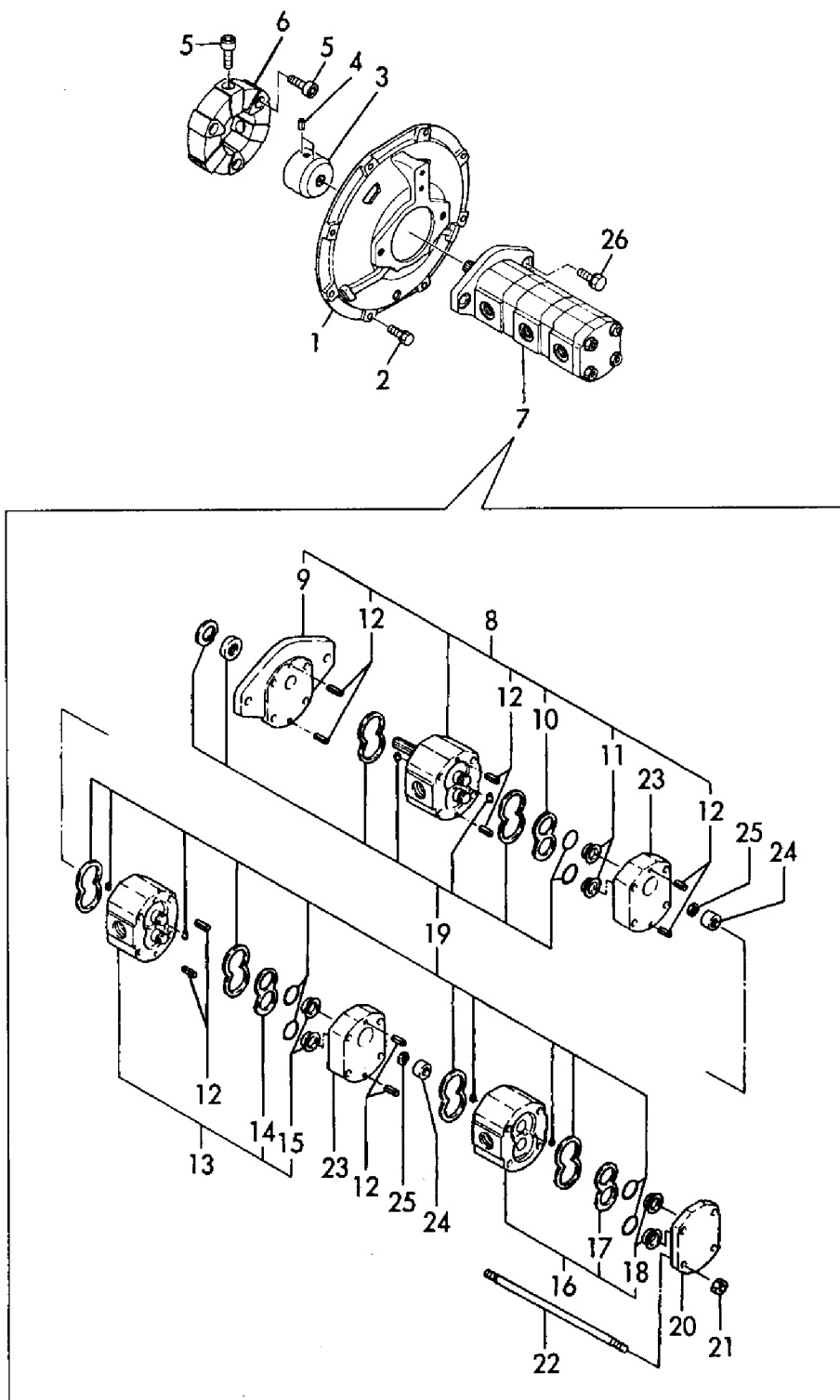
Fig. 38 油圧ポンプ&軸継手 HYD. OIL PUMP & JOINT
