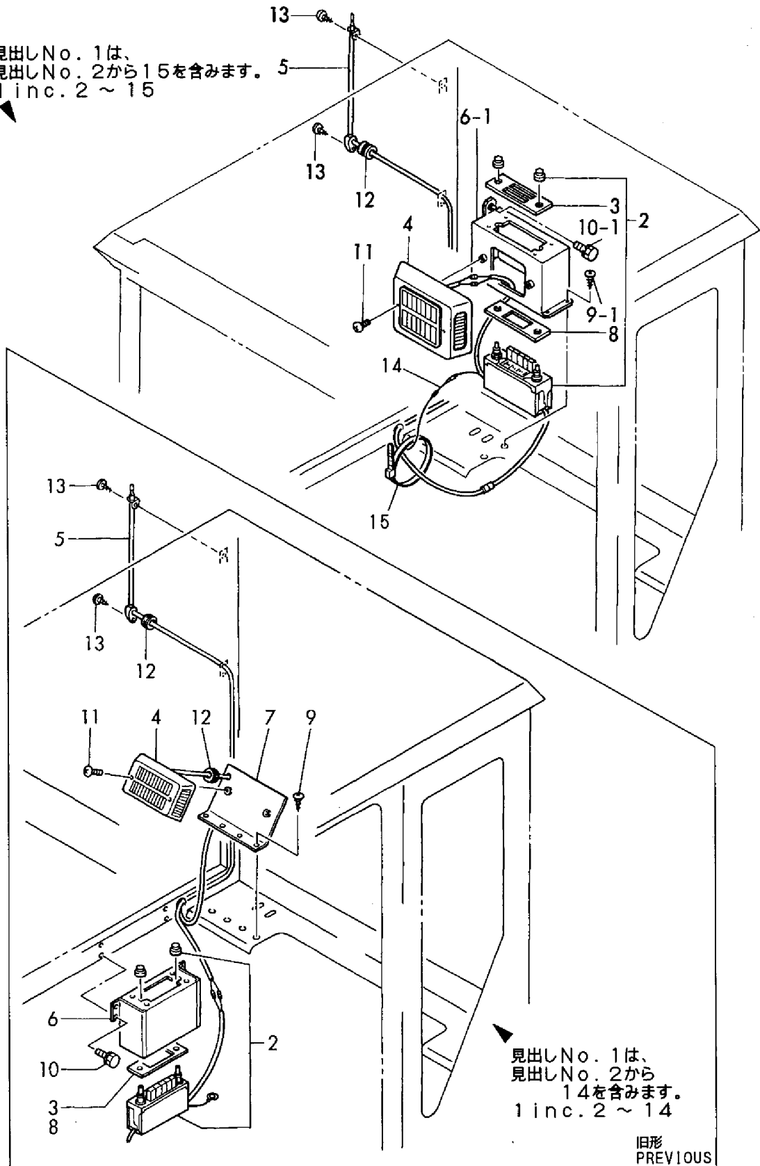
Fig. 59 ラジオ (オプション) RADIO (OPTIONAL)
