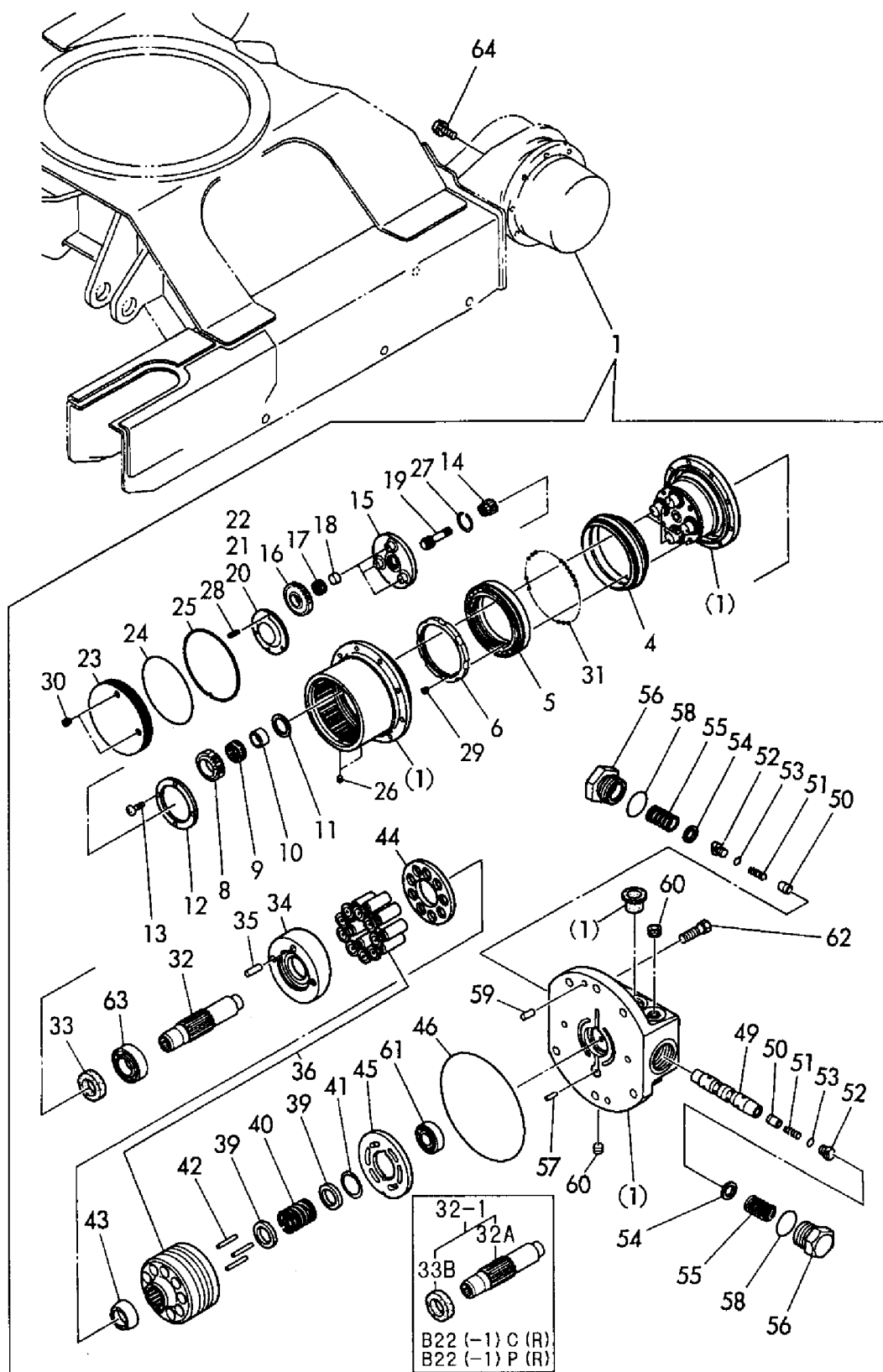
Fig. 40 走行モータ TRAVEL MOTOR
