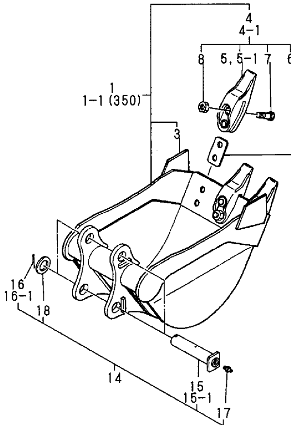
Fig. 68 バケット (アタッチメント) BUCKET (ATTACHMENT)
