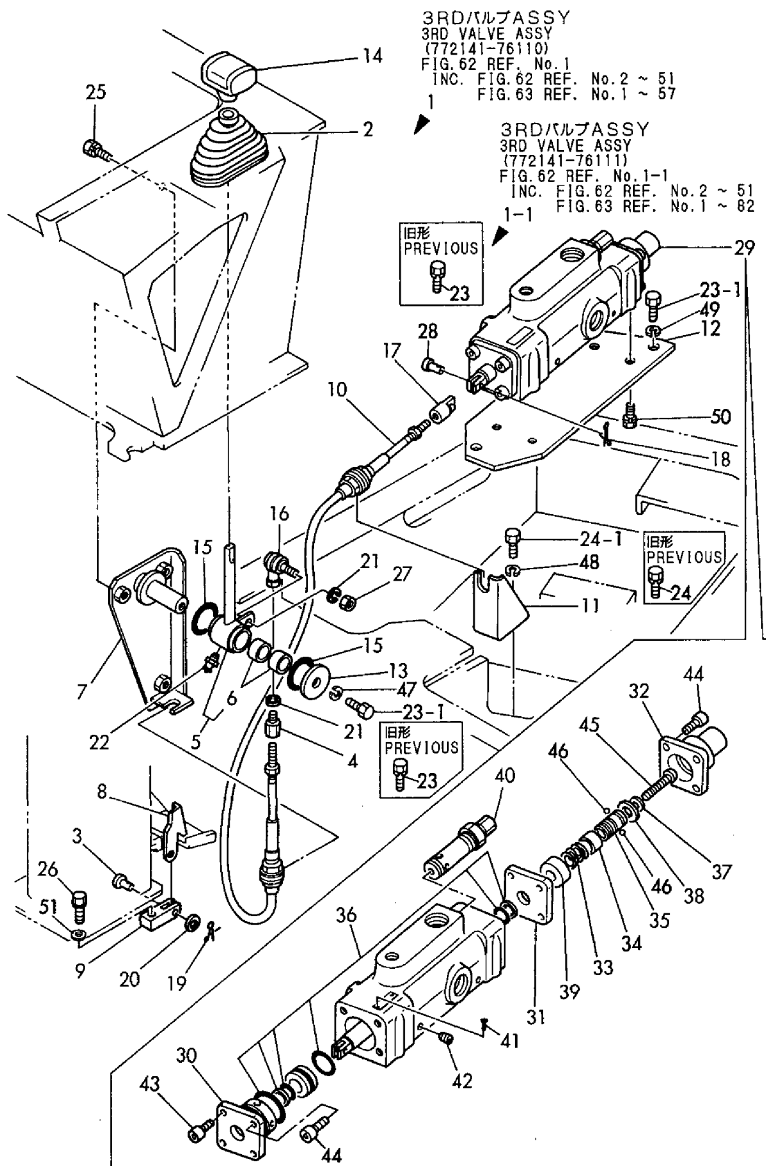
Fig. 62 3RDバルブコントロール (オプション) 3RD VALVE CONTROL (OPTIONAL)
