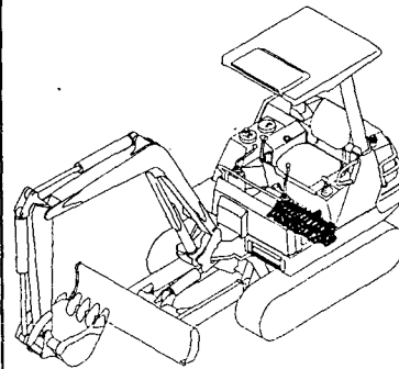
Fig.43 コントロールバルブ (アーム&バケット) CONTROL VALVE (ARM & BUCKET)
