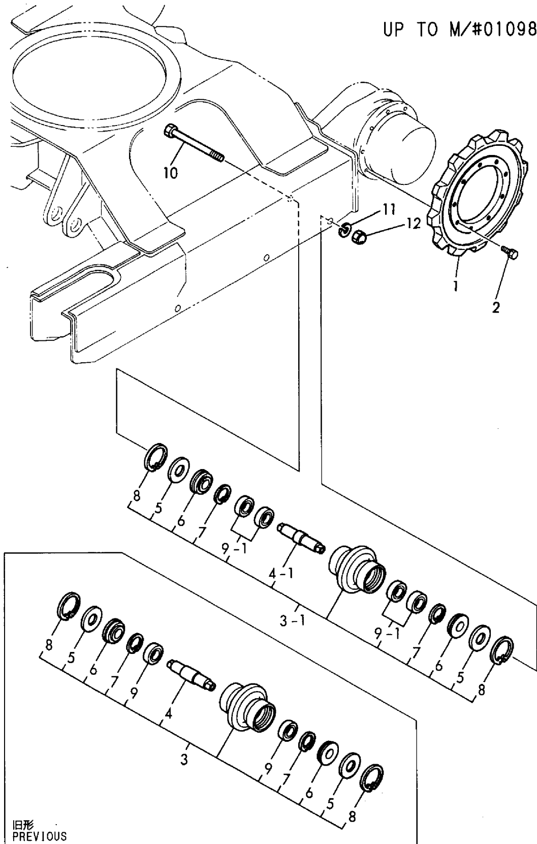
Fig. 13 トラックローラ (R) (旧形) TRACK ROLLER (R) (PREVIOUS)
