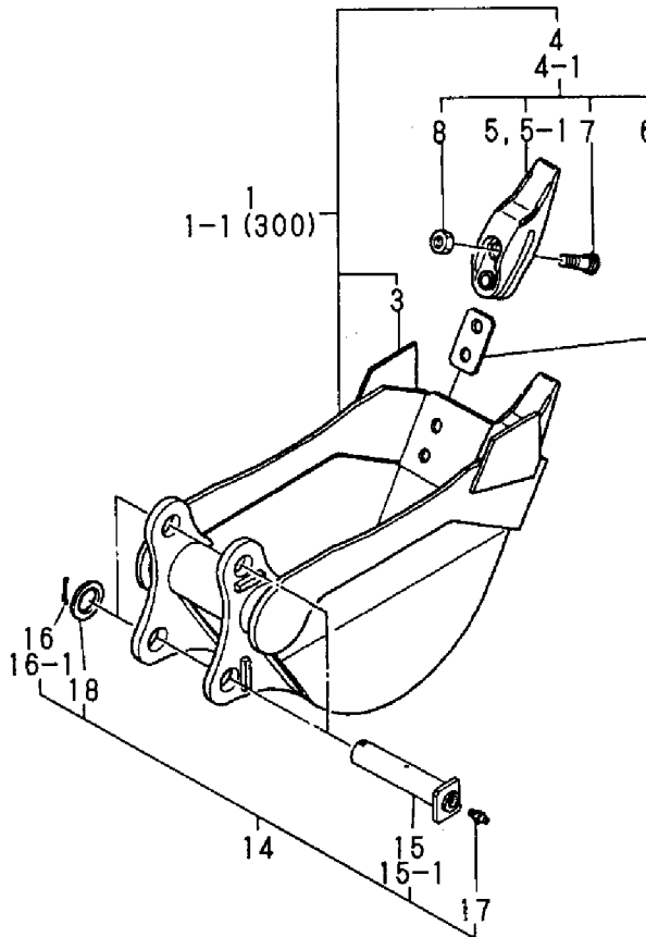
Fig. 67 バケット (アタッチメント) BUCKET (ATTACHMENT)
