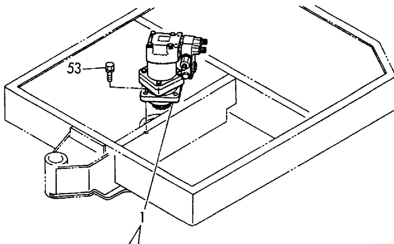
Fig. 39 旋回モータ TURNING MOTOR
