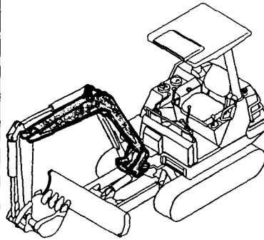
Fig.54 アーム&バケットリンク ARM & BUCKET LINK
