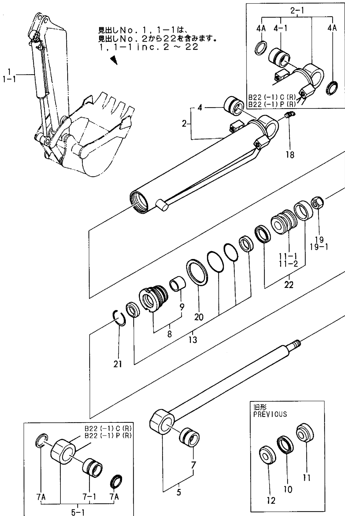
Fig. 34 バケットシリンダ BUCKET CYLINDER
