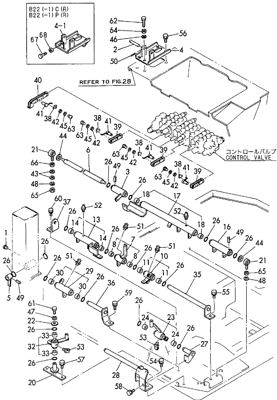
Fig. 22 操縦装置 (リンク) (マルチリンク仕様) CONTROL EQUIPMENT (LINK) (MULTI LINK SPEC.)
