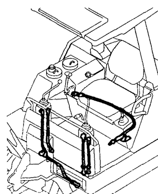
Fig.24 操縦装置 (ロッド) (マルチリンク仕様) CONTROL EQUIPMENT (ROD) (MULTI LINK SPEC.)
