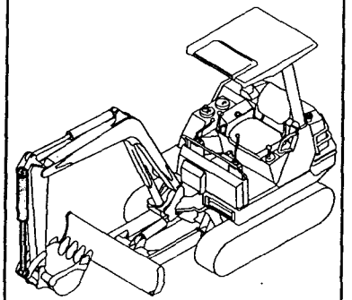
Fig.35 スイングシリンダ (キャビン) SWING CYLINDER (CABIN)
