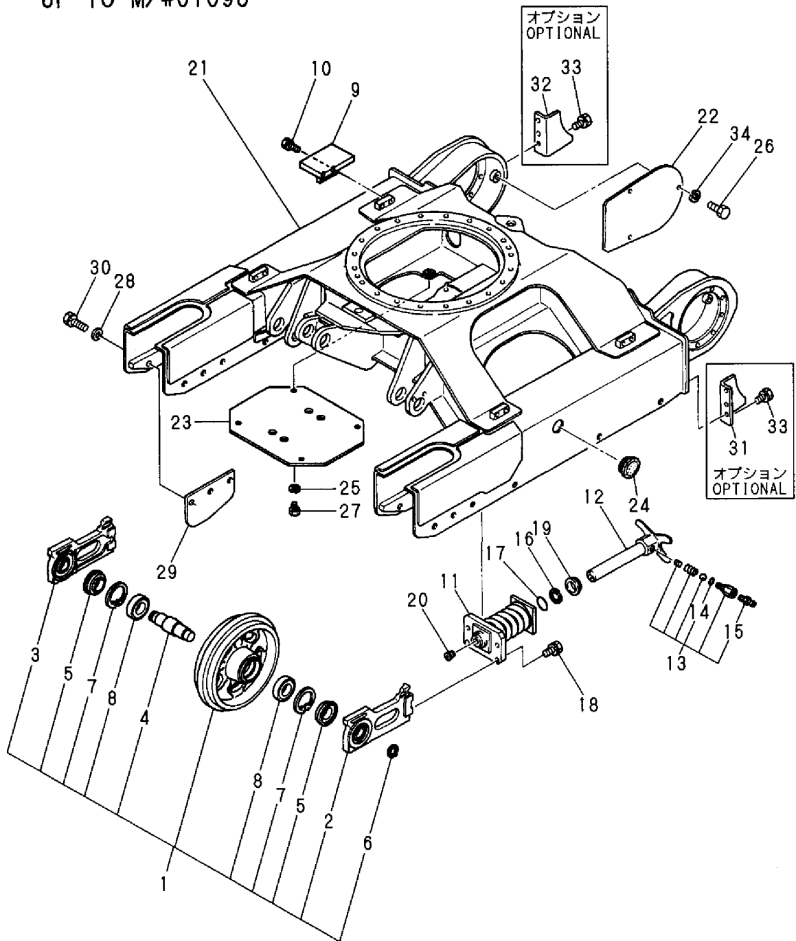
Fig. 15 トラックフレーム&アイドラ (旧形) TRACK FRAME & IDLER (PREVIOUS)
