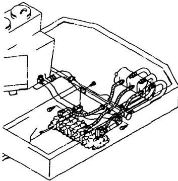
Fig.50 油圧配管 (タンク〜バルブ) HYD.OIL PIPING (TANK ~ VALVE)
