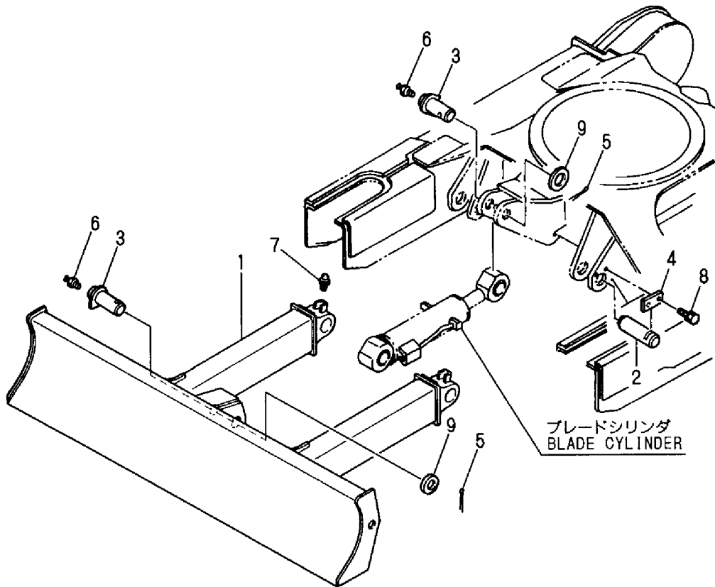
Fig. 56 ブレード (850) BLADE (850)
