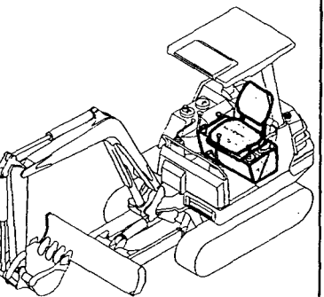
Fig.28 シート&ステップ SEAT & STEP
