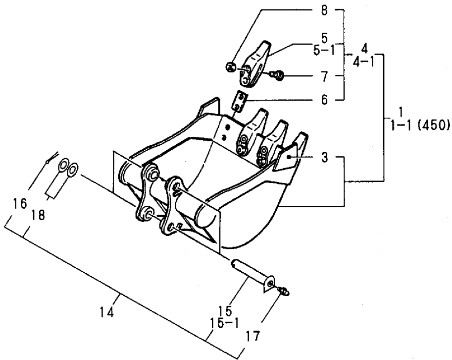
Fig. 55 バケット BUCKET
