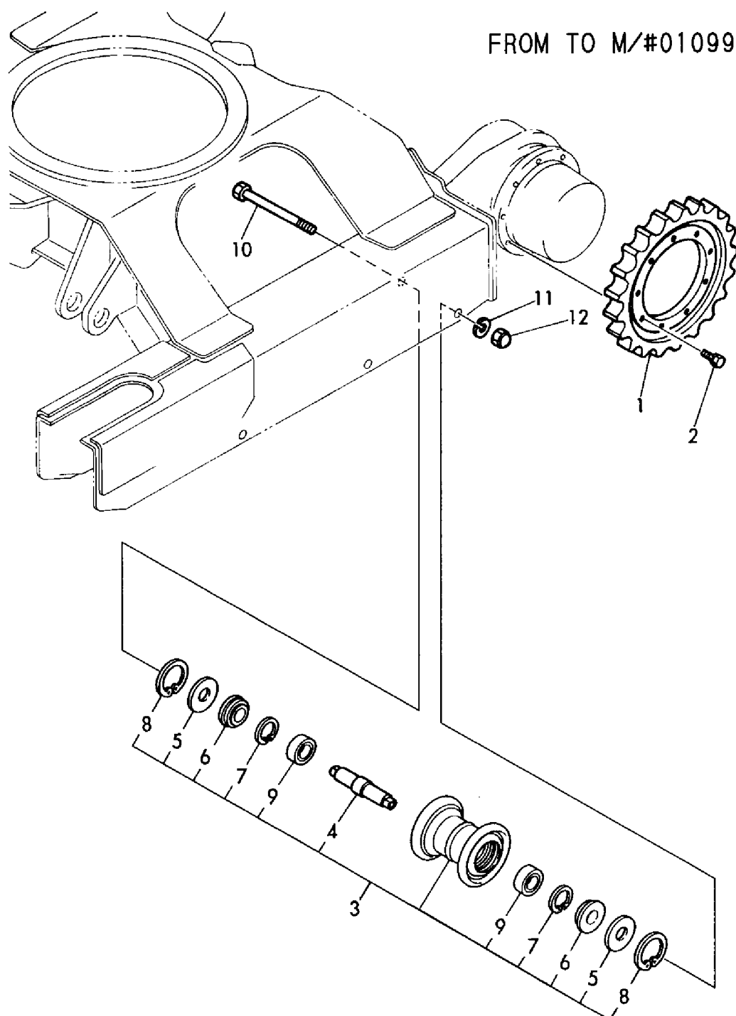
Fig. 14 トラックローラ (新形) TRACK ROLLER (NEW)
