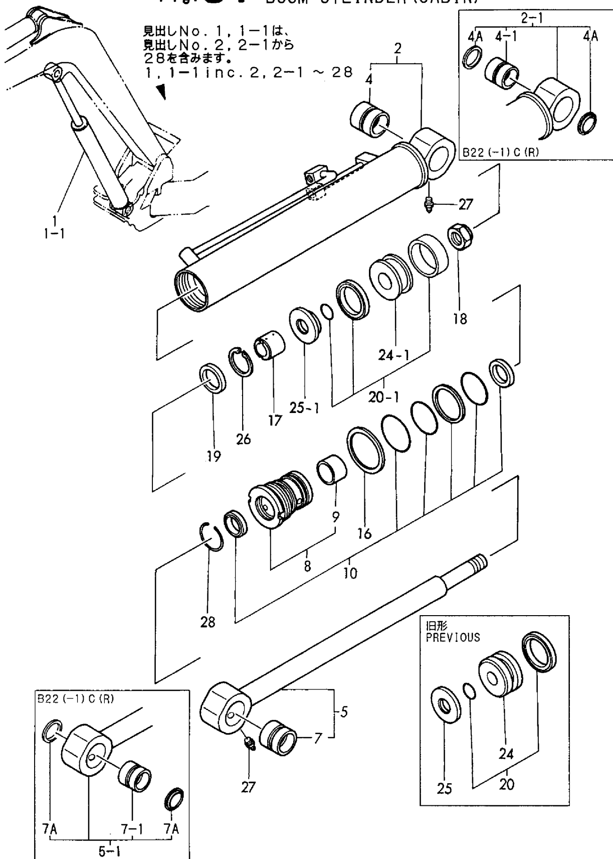
Fig. 31 ブームシリンダ (キャビン) BOOM CYLINDER (CABIN)
