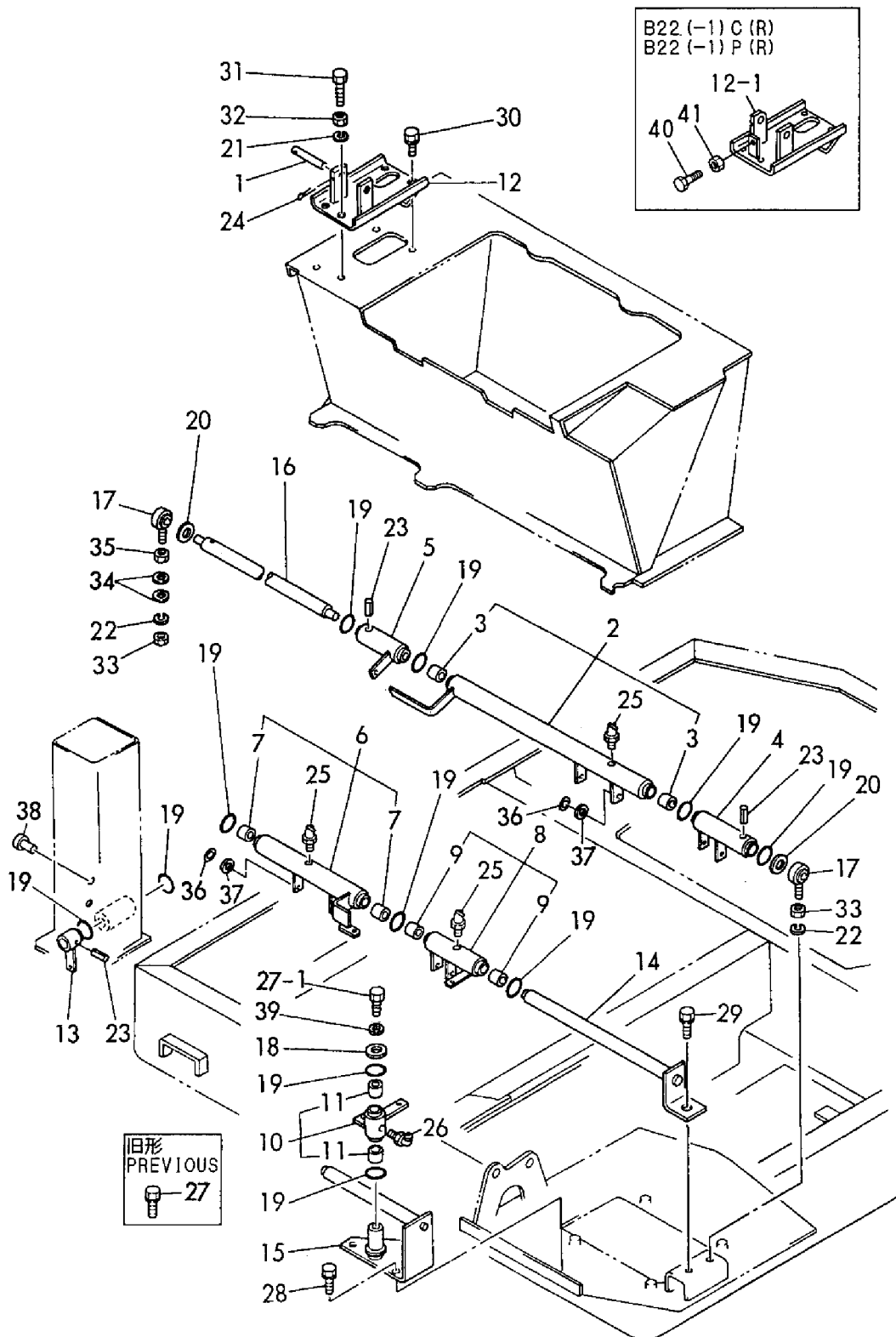
Fig. 21 操縦装置 (リンク) CONTROL EQUIPMENT (LINK)
