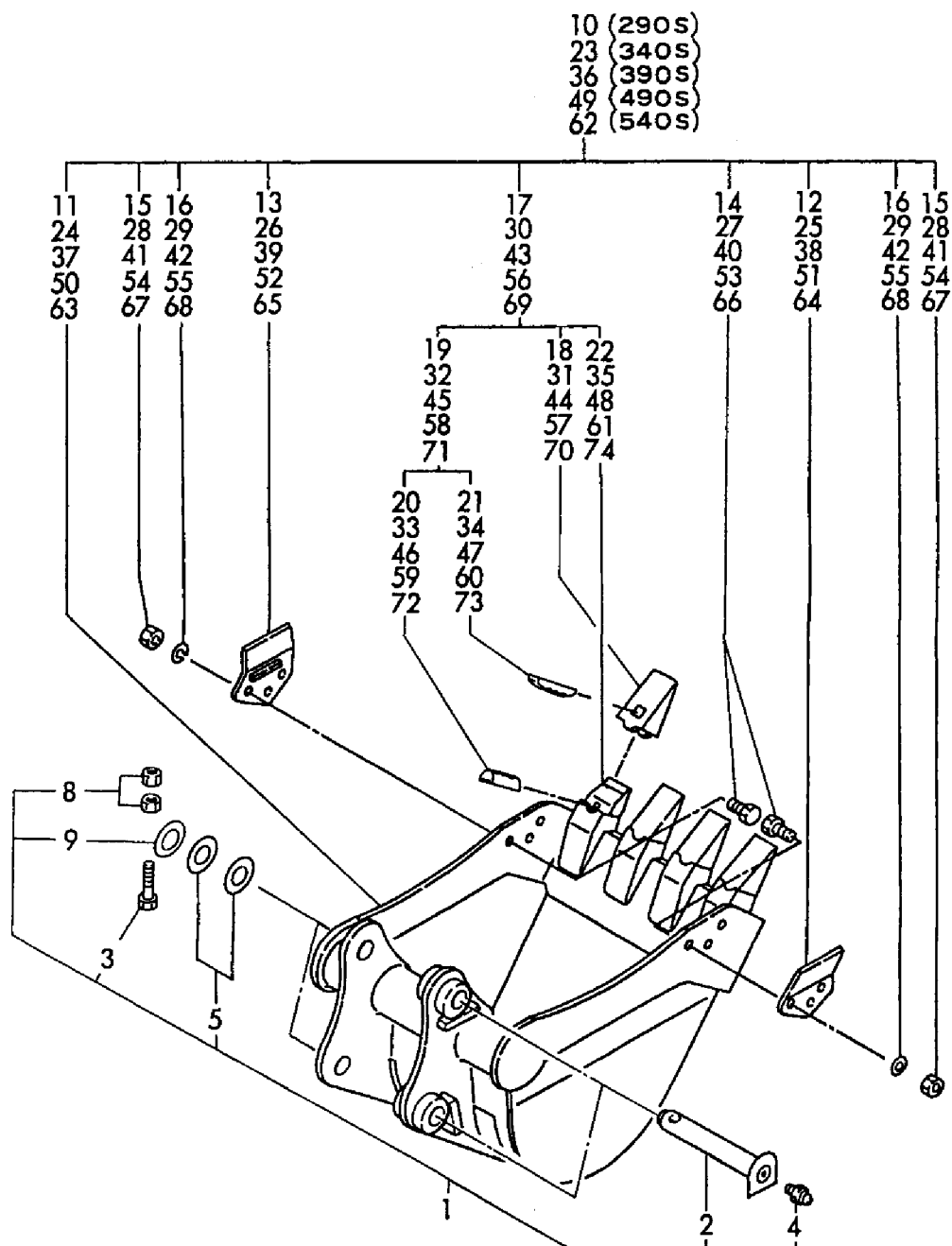
Fig. 70 バケットSタイプ (アタッチメント) BUCKET S - TYPE (ATTACHMENT)
