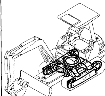
Fig.16 トラックフレーム & アイドラ (R) (旧形) TRACK FRAME & IDLER (R) (PREVIOUS)
