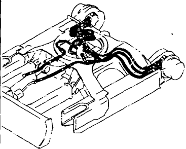
Fig.52 油圧配管 (ブーム) HYD.OIL PIPING (BOOM)
