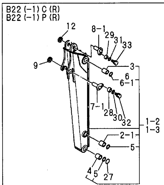
Fig. 54 アーム&バケットリンク ARM & BUCKET LINK
