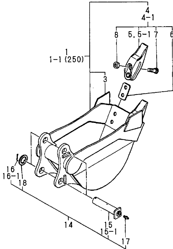
Fig. 66 バケット (アタッチメント) BUCKET (ATTACHMENT)
