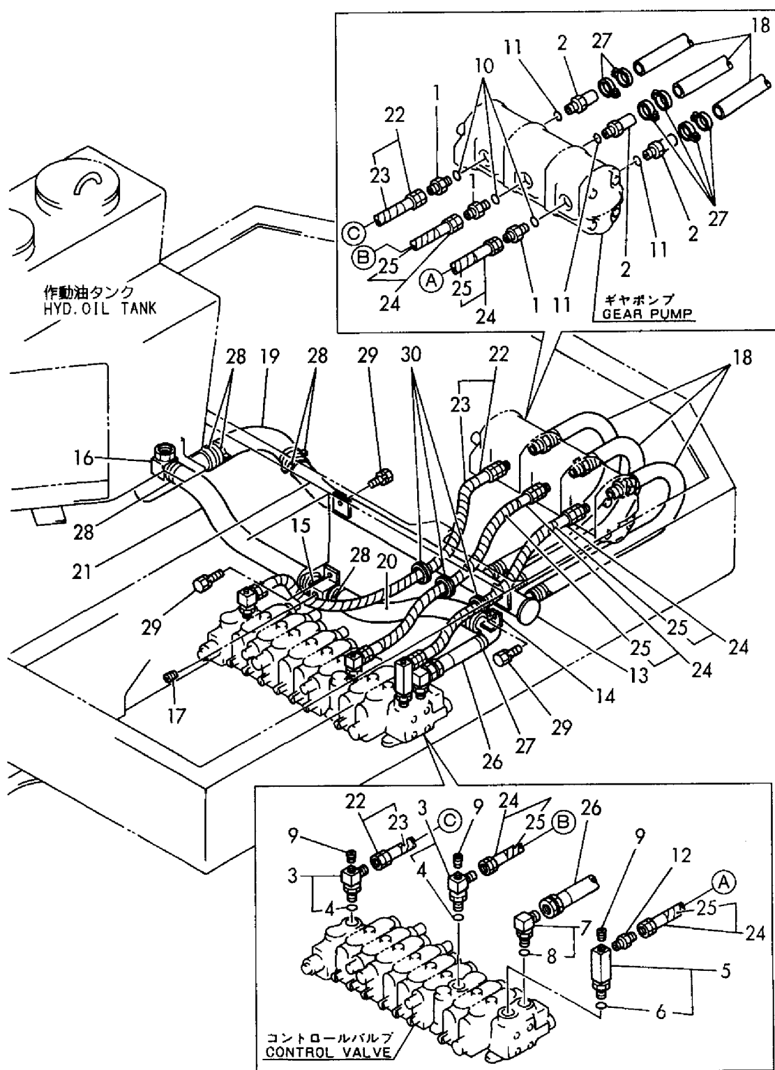
Fig. 50 油圧配管 (タンク~バルブ) HYD. OIL PIPING (TANK~VALVE)
