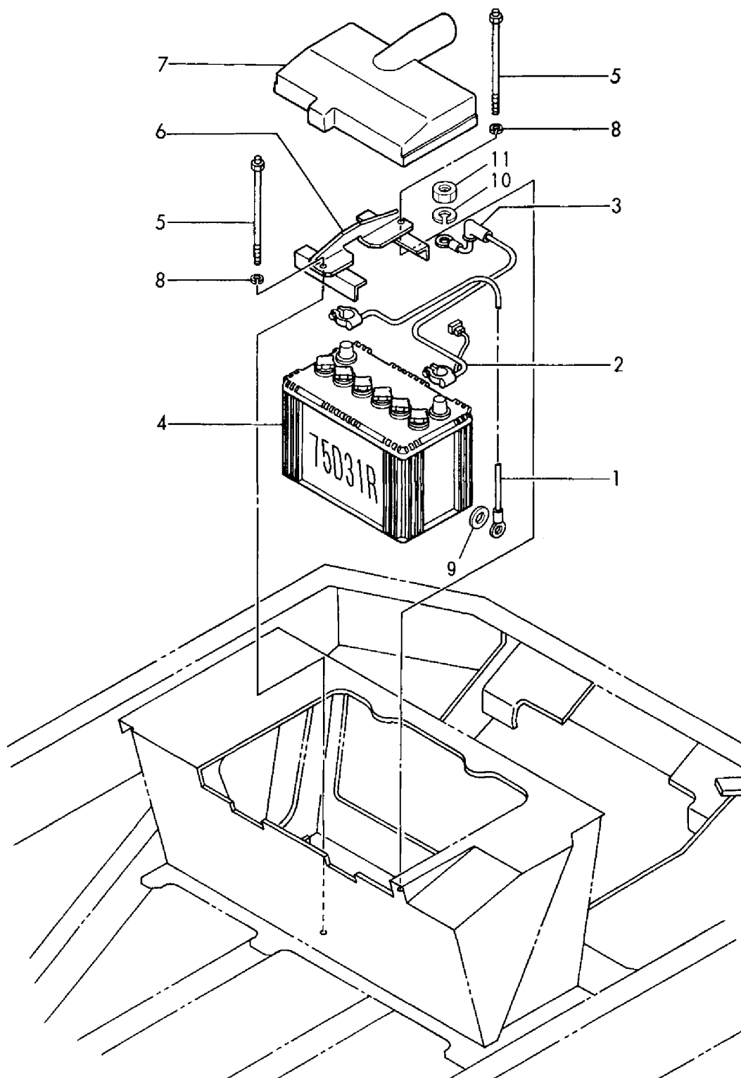
Fig. 8 バッテリー BATTERY
