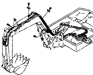
Fig.52 油圧配管 (ブーム) HYD.OIL PIPING (BOOM)
