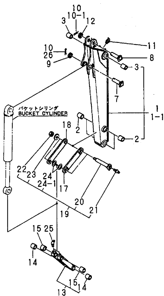
Fig. 54 アーム&バケットリンク ARM & BUCKET LINK
