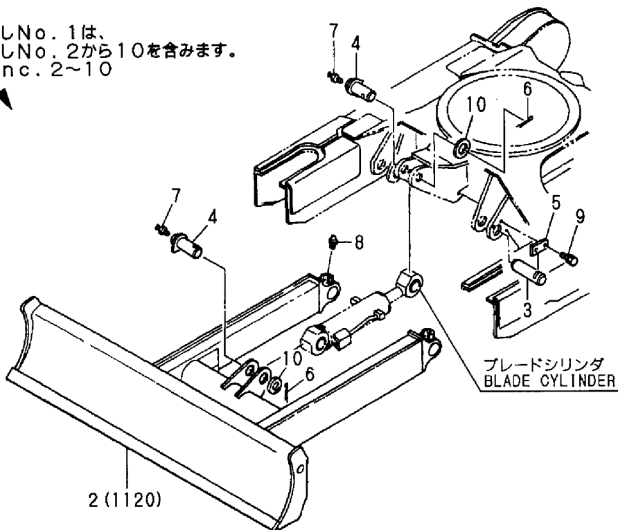
Fig. 65 ブレード (850) (アタッチメント) BLADE (850) (ATTACHMENT)
