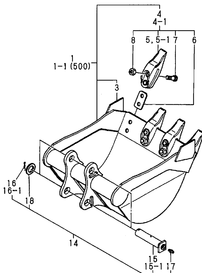
Fig. 69 バケット (アタッチメント) BUCKET (ATTACHMENT)
