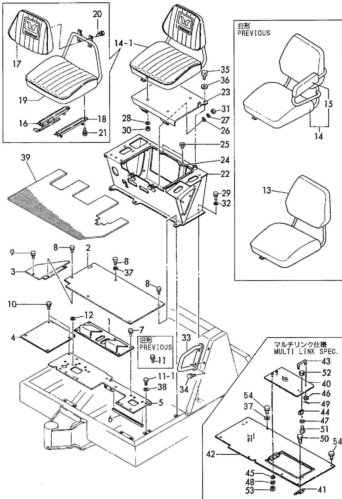
Fig. 28 シート&ステップ SEAT & STEP
