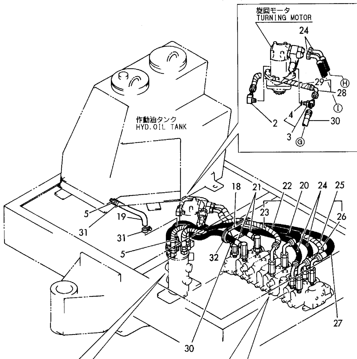
Fig. 49 油圧配管 (バルブ～スイベル～モータ) HYD. OIL PIPING (VALVE ~ SWIVEL ~ MOTOR)
