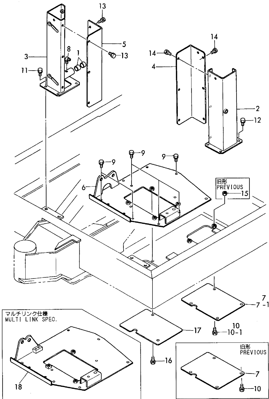
Fig. 19 リンク台 LINK STAND
