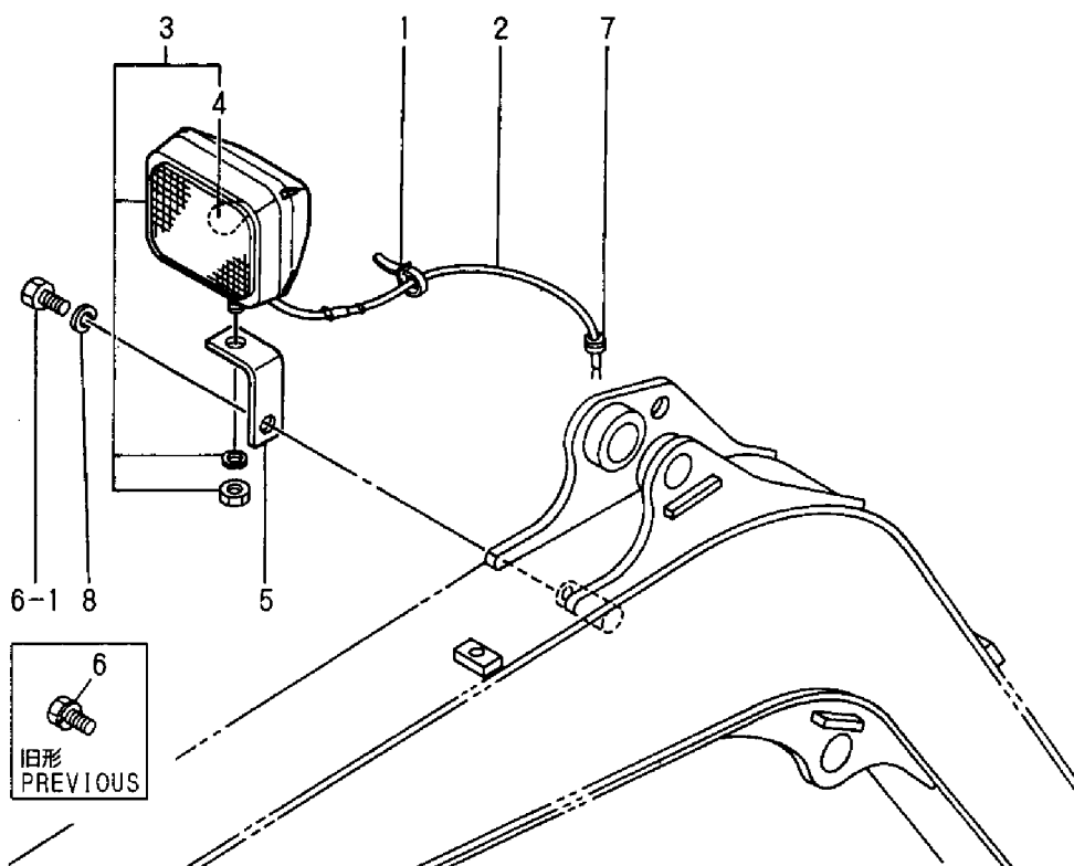
Fig. 11 ワークランプ WORK LAMP
