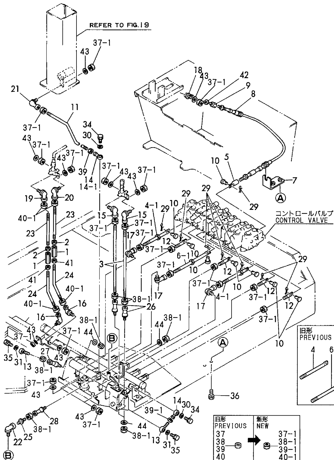
Fig. 24 操縦装置 (ロッド) (マルチリンク仕様) CONTROL EQUIPMENT (ROD) (MULTI LINK SPEC.)
