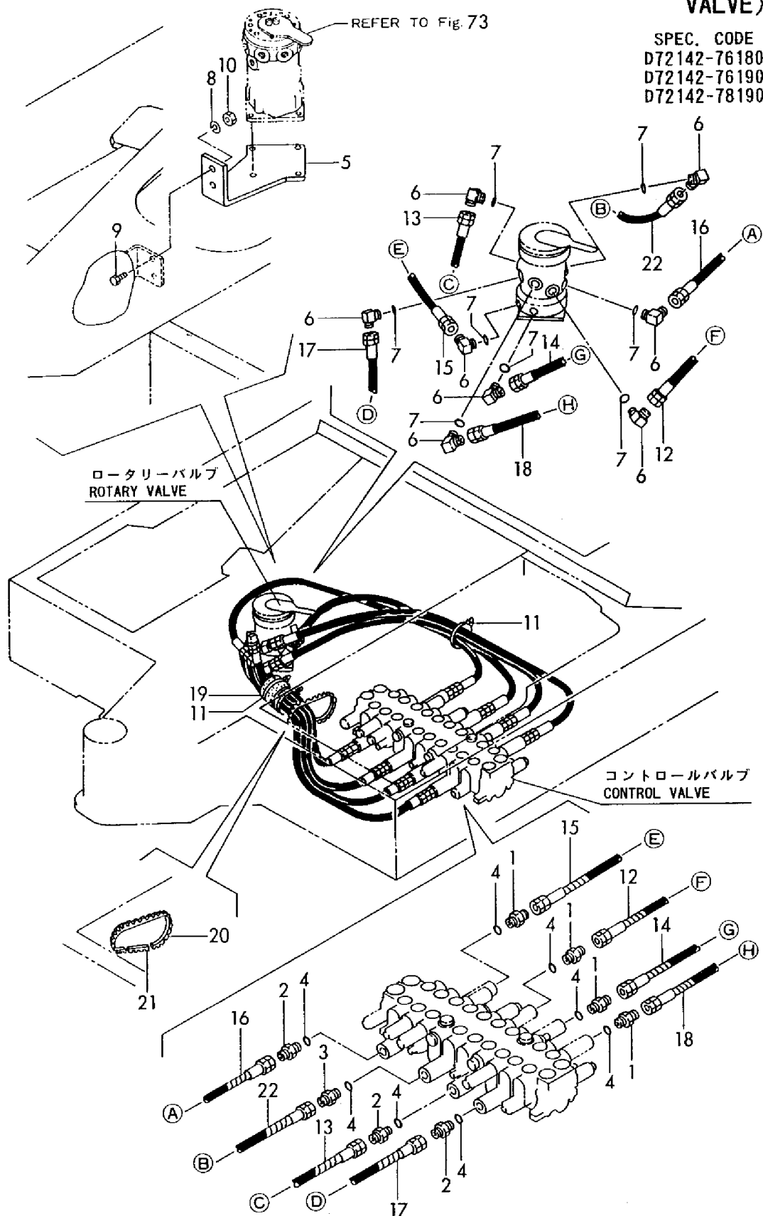
Fig. 97 コントロールハイカン (マルチチェンジバルブ-コントロールバルブ) CONTROL PIPING (MULTI CHANGE VALVE-CONTROL VALVE)
