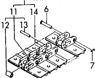
クローラ (320G) CRAWLER(320G)
