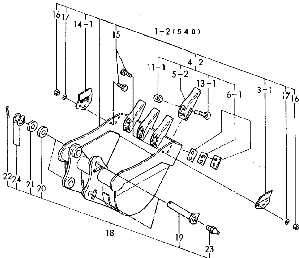
Fig. 103 バケット (500, 540) (7タッチメント) BUCKET (500, 540) (ATTACHMENT)
