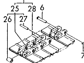
クローラ (370) CRAWLER(370)
