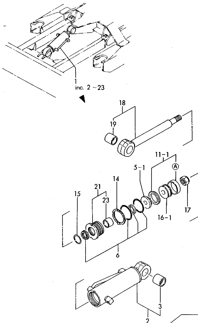
Fig. 57 ブレードシリンダ BLADE CYLINDER
