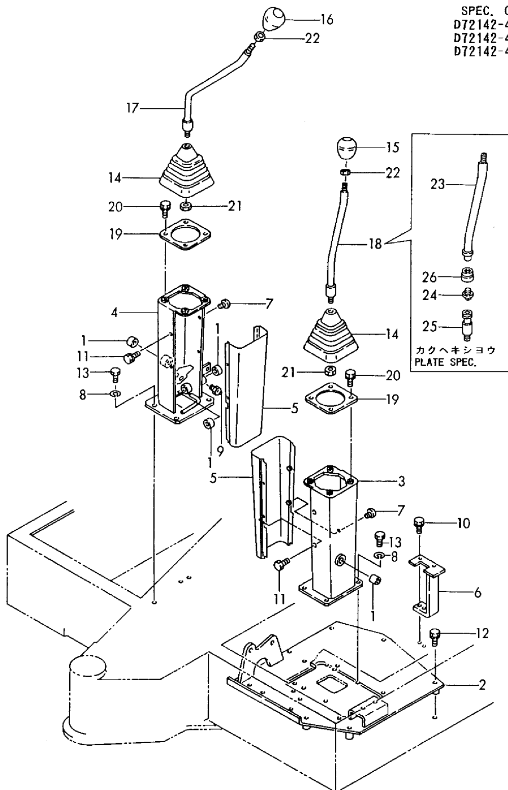
Fig. 27 ソウジュウソウチ (レバー、スタンド & リンクダイ) ユアツパイロット CONTROL EQUIP. (LEVER, STAND & LINK STAND) HYD. OIL PILOT
