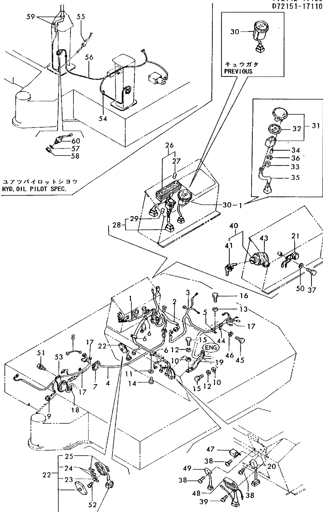
Fig. 17 デンソウヒン(キャビン, キャノピョウツウ) ELECTRIC PART(CABIN, CANOPY)
