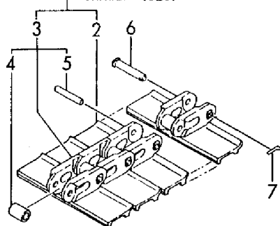
クローラ (320) CRAWLER(320)
