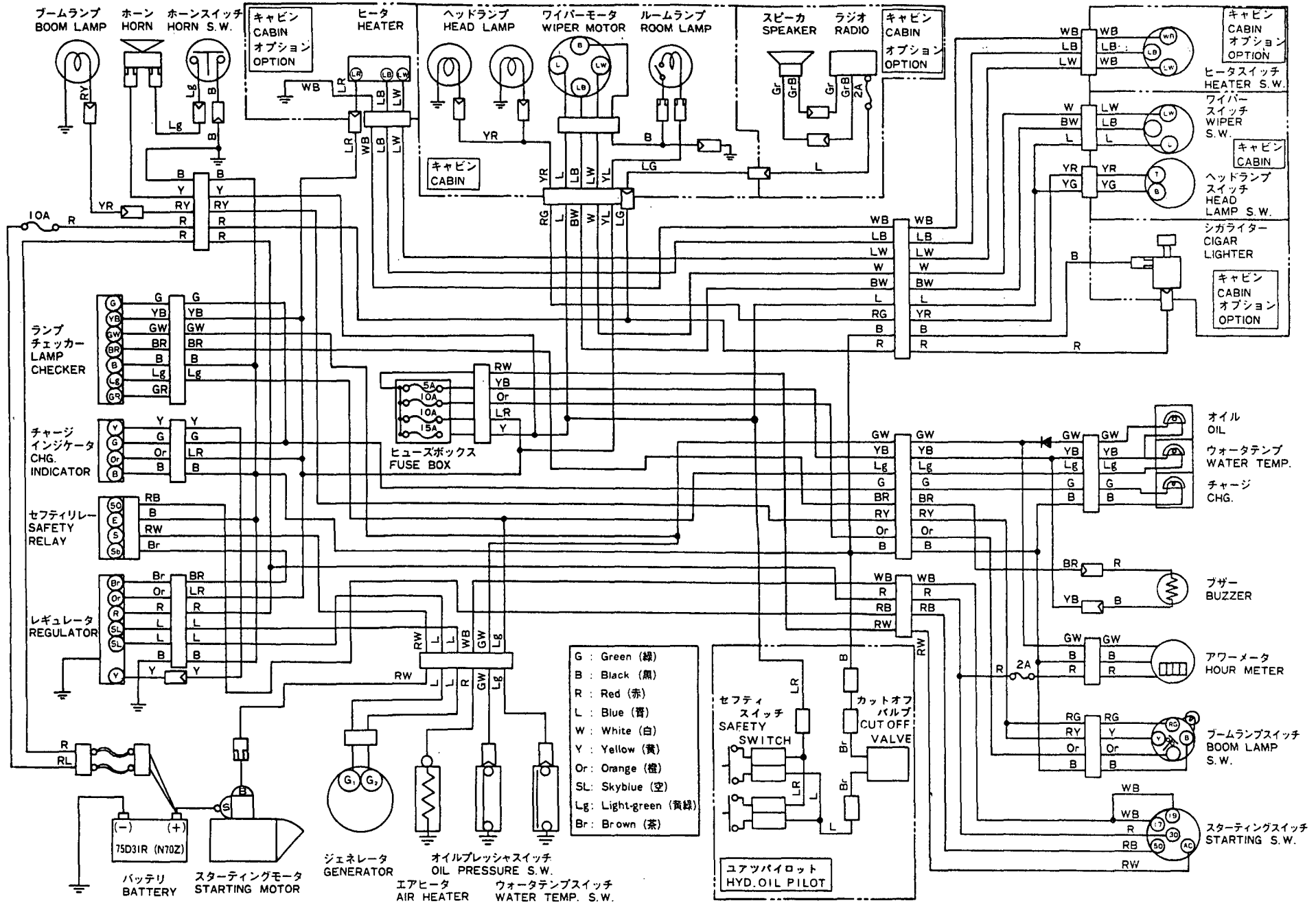
配線図 WIRING DIAGRAM
