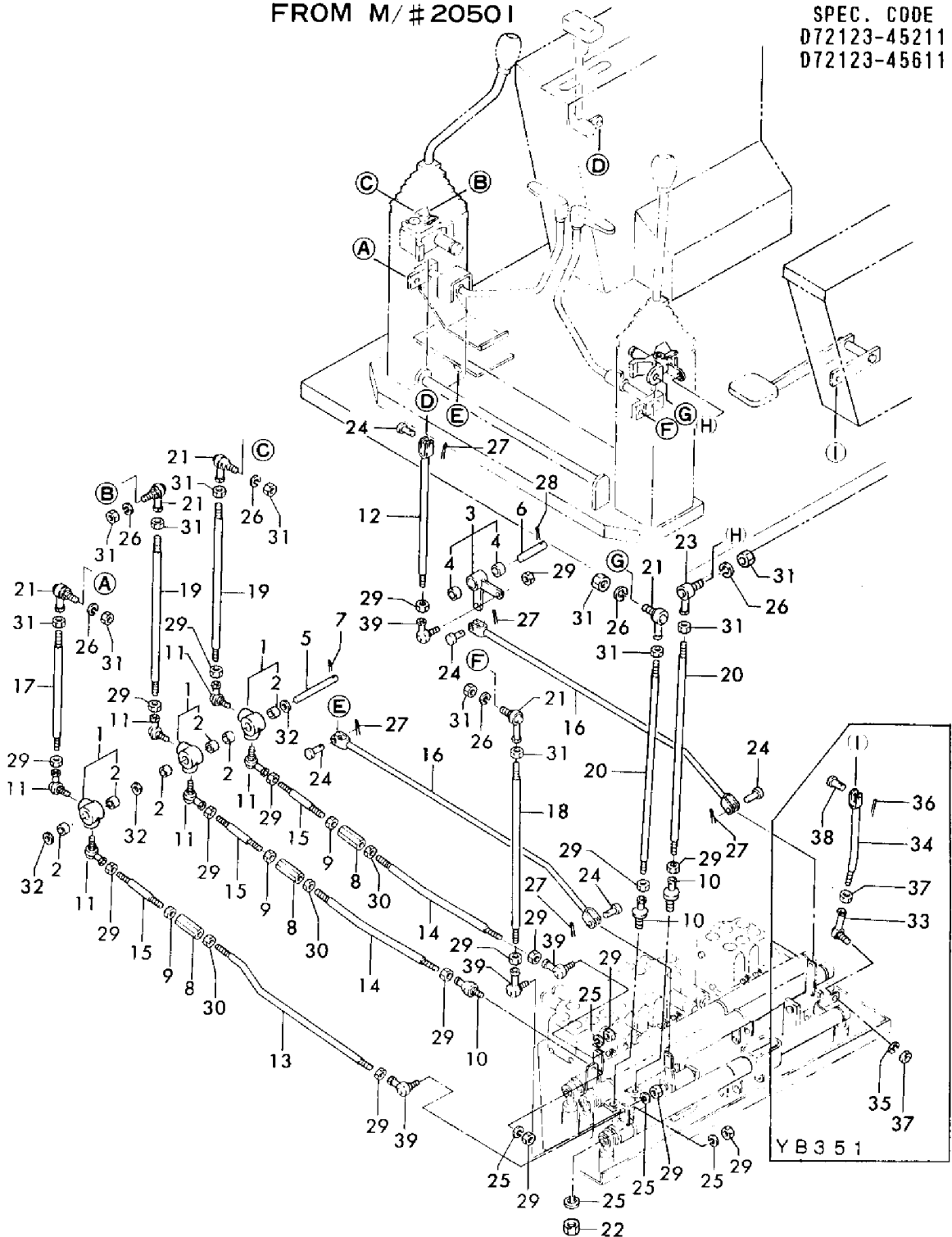
Fig. 34 ソウジュウソウチ(ロッド) (シンガタ) CONTROL EQUIPMENT (ROD) (NEW TYPE)
