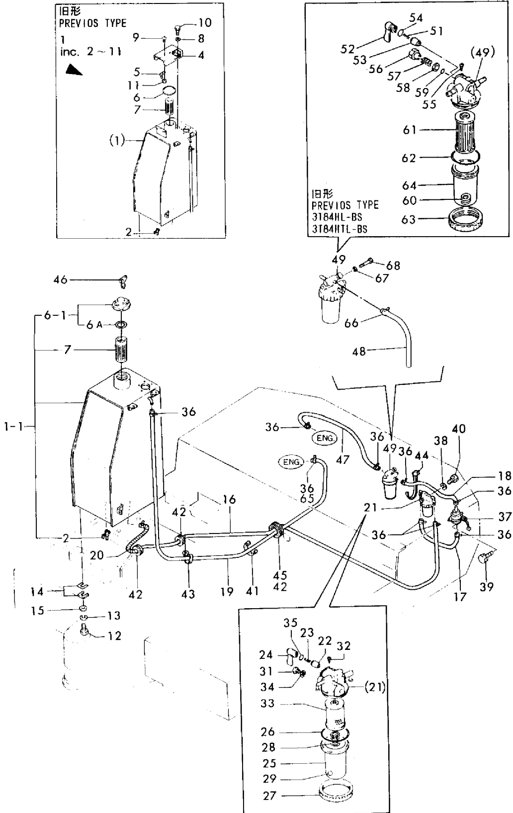
Fig. 12 F.O. タンク & F.O. パイプ FUEL TANK & FUEL LINE
