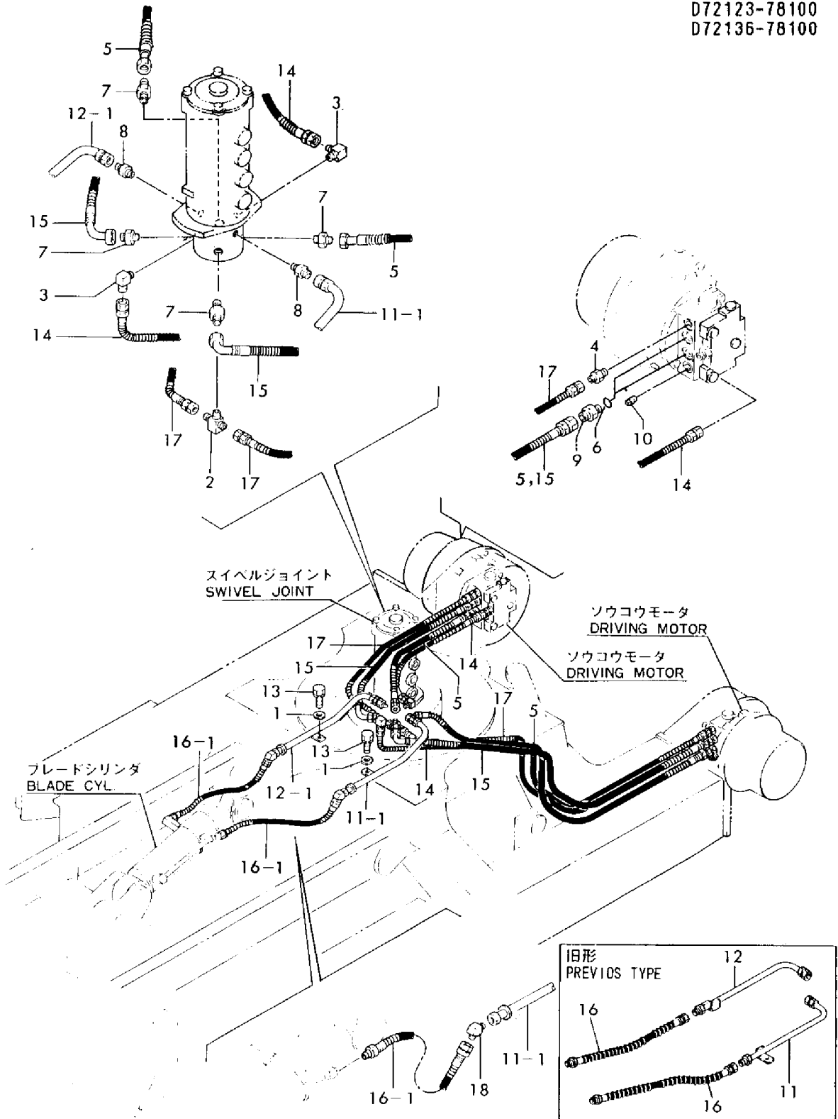
Fig. 80 ユアツハイガン(トラックフレーム) (YB35I) HYD. OIL PIPING (TRACK FRAME) (YB35I)
