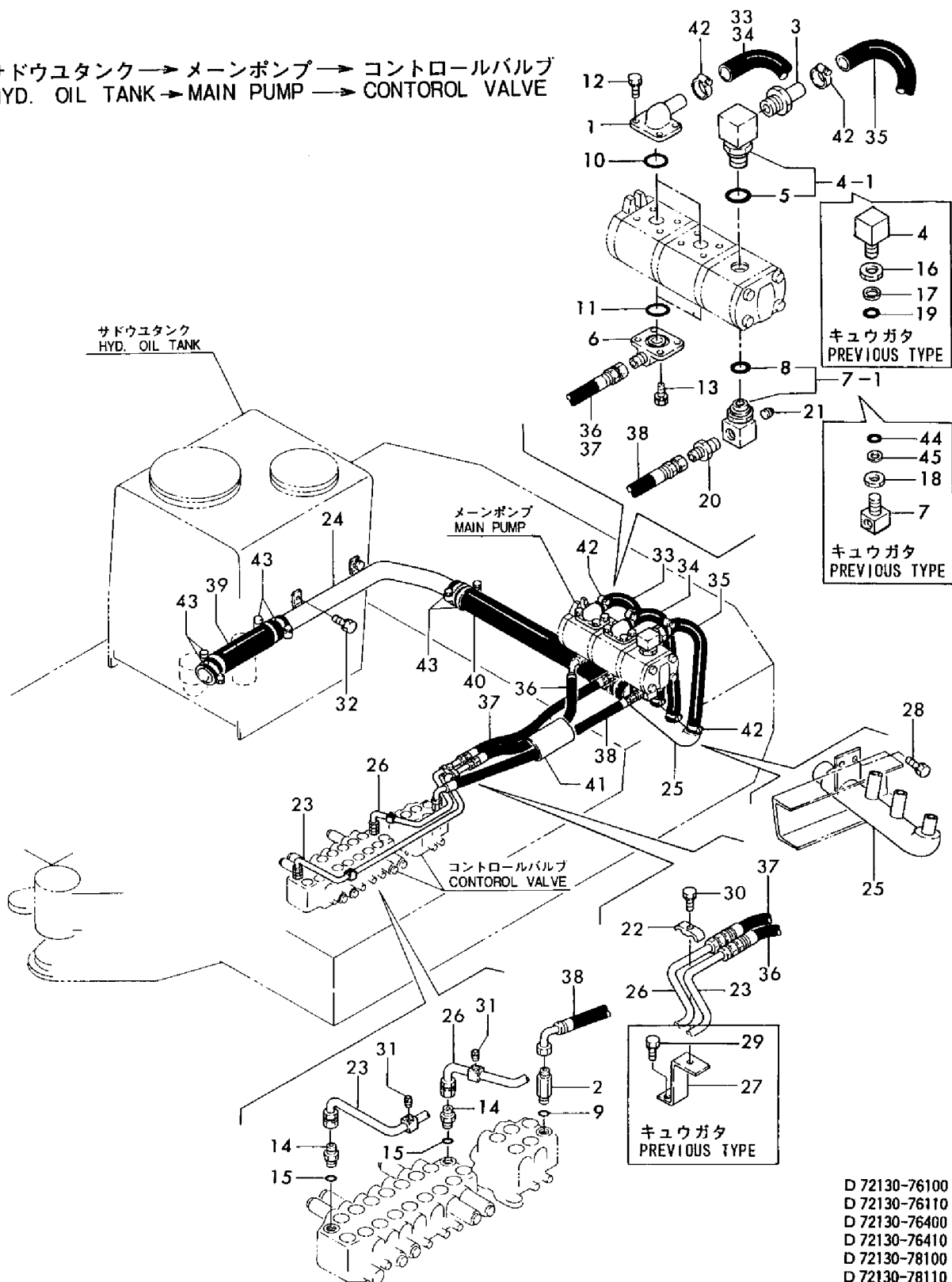
Fig. 61 ユアツハイカン(タンク→ポンプ→バルブ) HYD. OIL PIPING (TANK-PUMP-VALVE)
