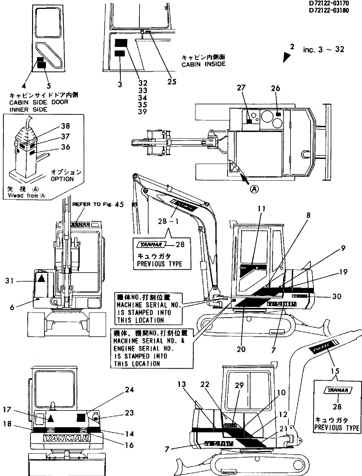
Fig. 2 メイバン(キャビン) (シンガタ) LABEL (CABIN) (NEW TYPE)
