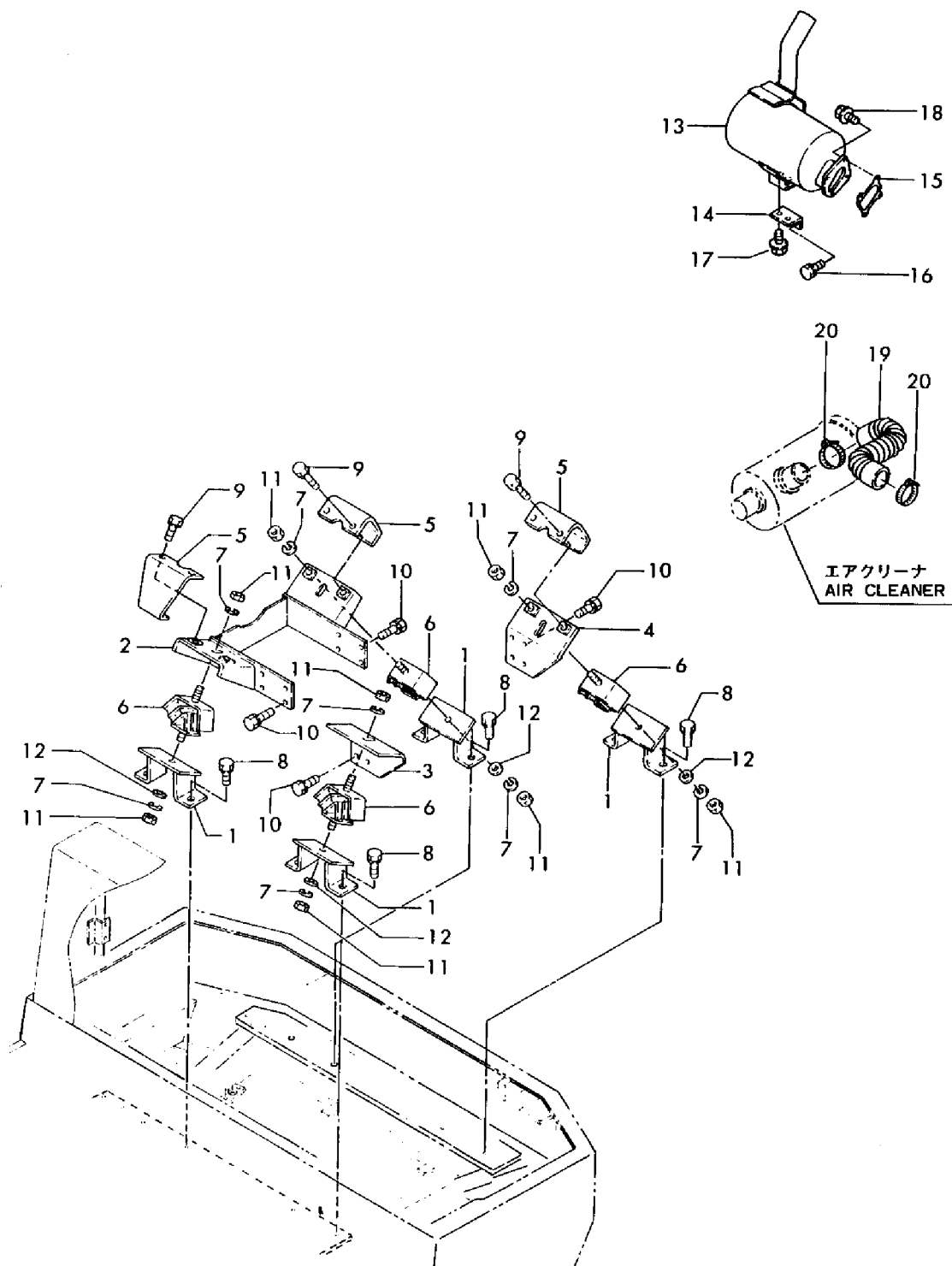
Fig. 8 エンジンマウント ENG. MOUNT
