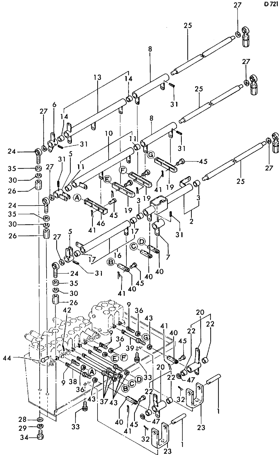
Fig. 29 ソウジュウソウチ(リンク) (キュウガタ) CONTROL EQUIPMENT (LINK) (PREVIOUS TYPE)
