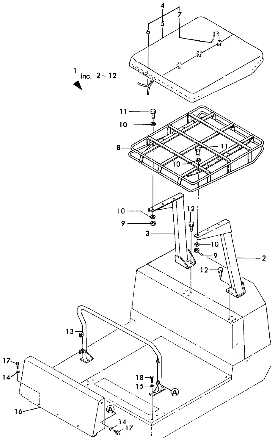
Fig. 41 キャンピ(UZ)(キュウガタ) CANOPY (UZ)(PREVIOS TYPE)
