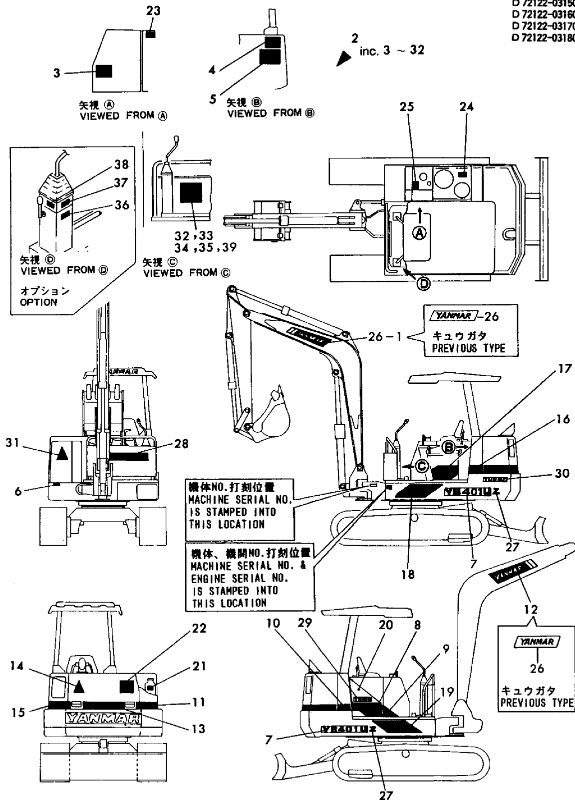
Fig. 4 メイバン (キャノピー) (シンガタ) LABEL (CANOPY) (NEW TYPE)
