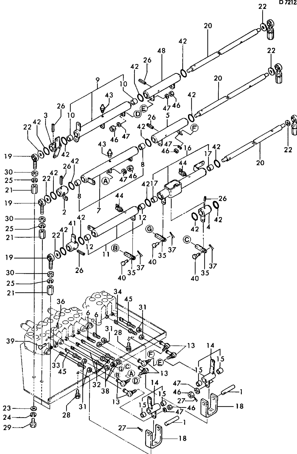
Fig. 30 ソウジュウソウチ(リンク) (シンガタ) CONTROL EQUIPMENT (LINK) (NEW TYPE)
