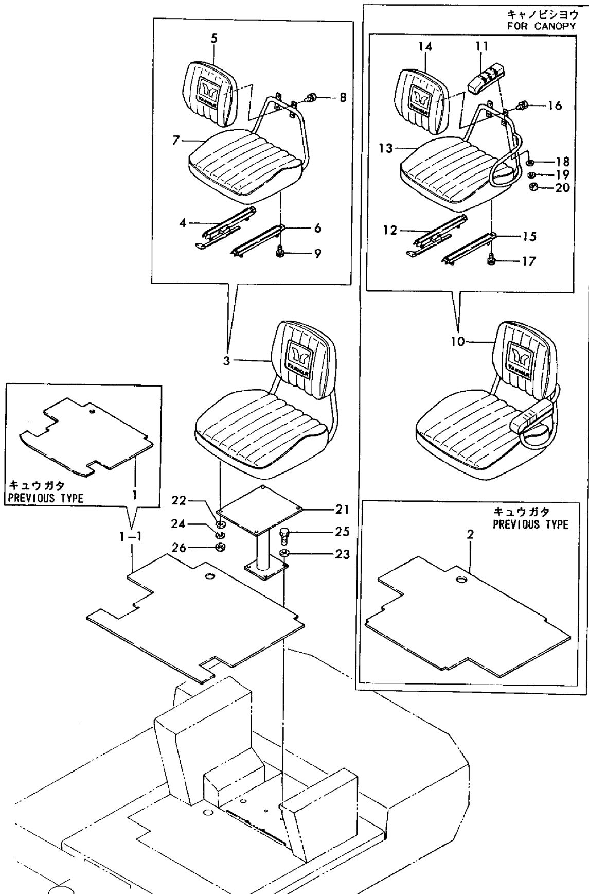
Fig. 37 シート SEAT
