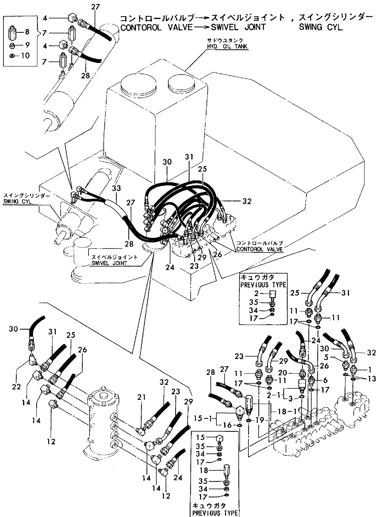
Fig. 63 ユアツハイカン(バルブスイベル, スイング) D 72130-76100 HYD. OIL PIPING (VALVE-SWIVEL, SWING) D 72130-76110 D 72130-78100 D 72130-78110
