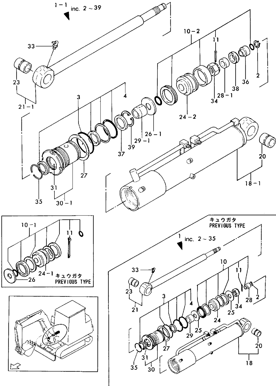
Fig. 51 スイングシリンダ (UZ) SWING CYLINDER (UZ)
