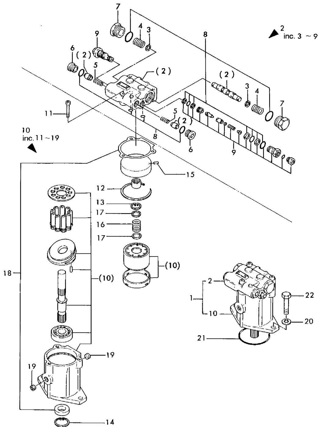
Fig. 56 センカイモータ TURNING MOTOR
