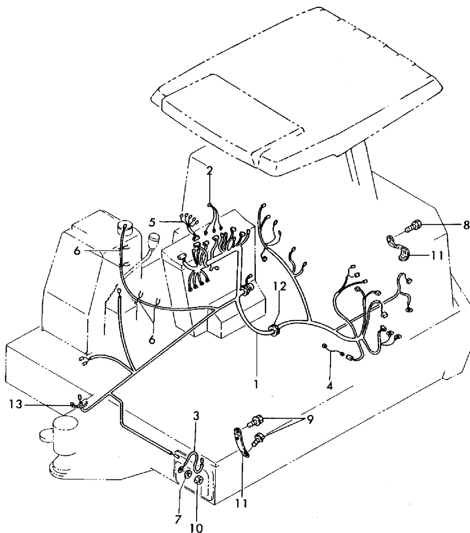
Fig. 14 ワイヤリング (キャノピー) WIRING (CANOPY)
