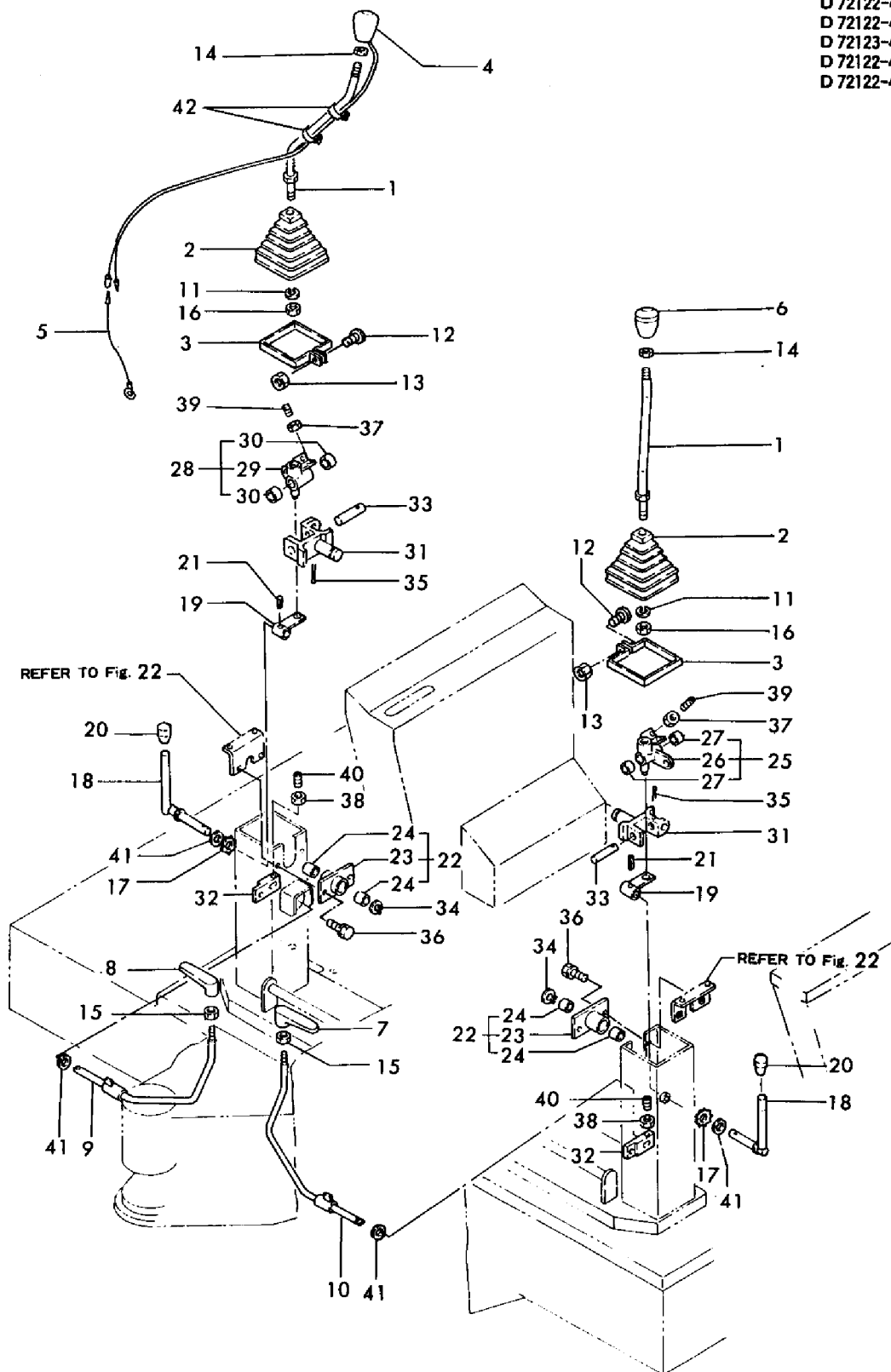
Fig. 23 ソウジウソウチ(レバー) (キュウガタ) CONTROL EQUIPMENT (LEVER) (PREVIOUS TYPE)
