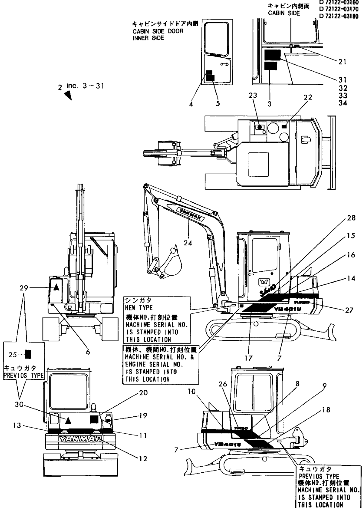
Fig. 1 1 メイバン(キャビン)(キュウガタ) LABEL (CABIN) (PREVIOS TYPE)
