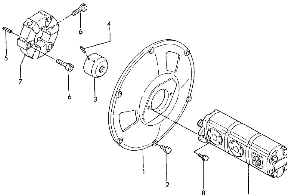
Fig. 54 ユアツポンプ & ジクツギテ HYD. OIL PUMP & COUPLING
