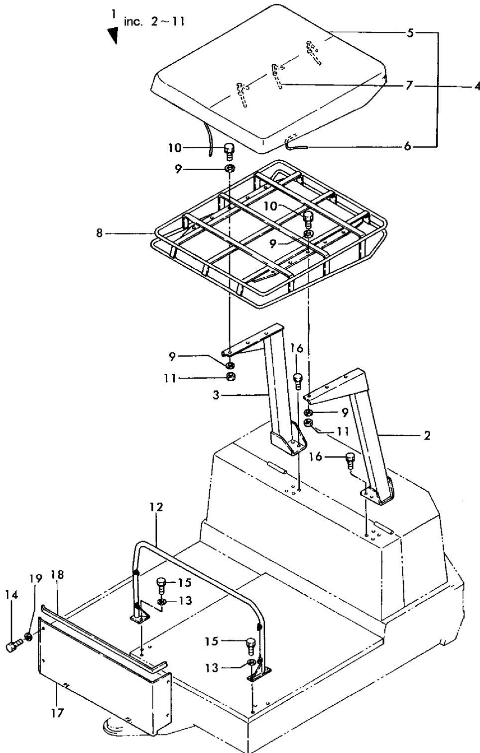
Fig. 40 キャノピ (U) (キューガタ) CANOPY (U) (PREVIOUS TYPE)
