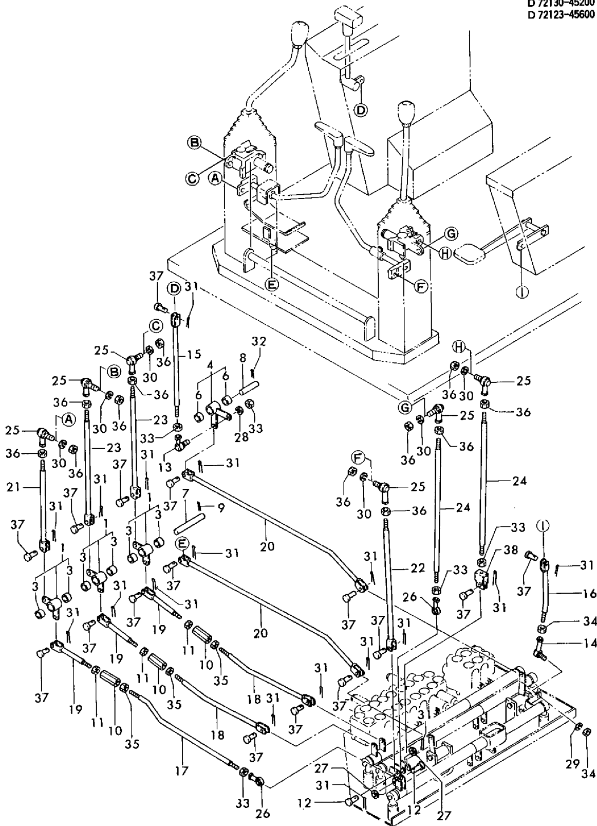
Fig. 27 ソウジュウソウチ(ロッド) (キューガタ) CONTROL EQUIPMENT (ROD) (OLD) (PREVIOUS TYPE)
