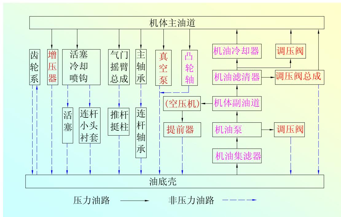
YC4F 柴油机润滑系统示意图
