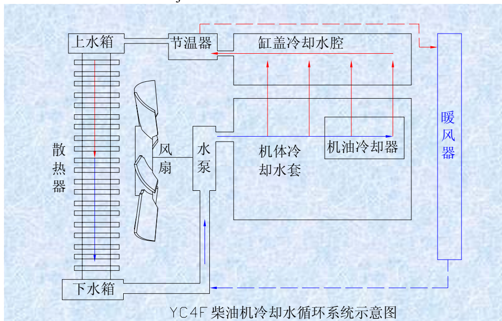
YC4F 柴油机冷却水循环系统示意图 Diagrama de ciclo de agua refrigerador del motor de disel de YC4F
