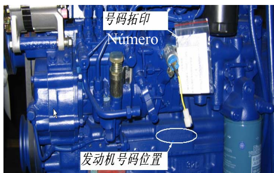
发动机号码位置: Posición de número del motor
