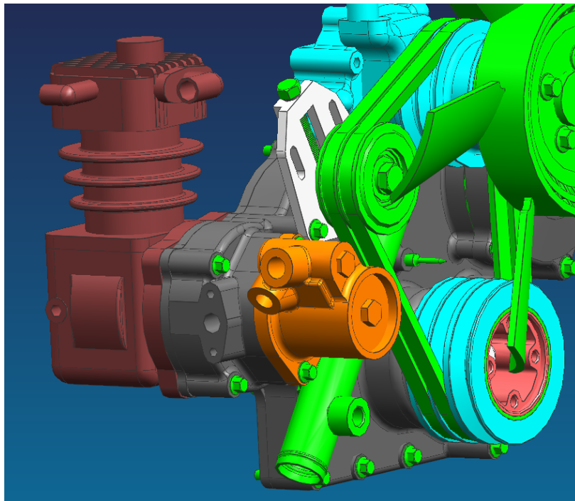
空气压缩机和转向泵在齿轮室上的安装位置示意图 Diagrama de colocación del compresor del aire y la bomba
