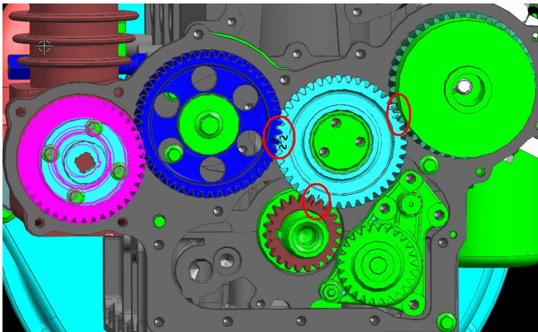
齿轮系配对记号装配示意图
