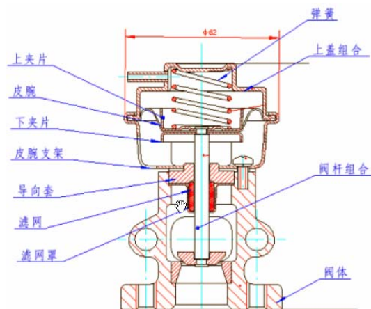
EGR 阀结构示意图
