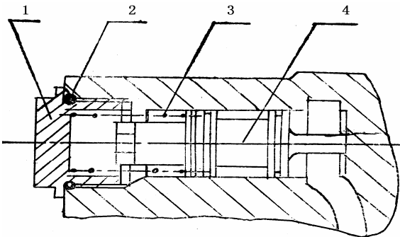
- 64 1、螺帽 2、“O”型圈 3、弹簧 4、伐
