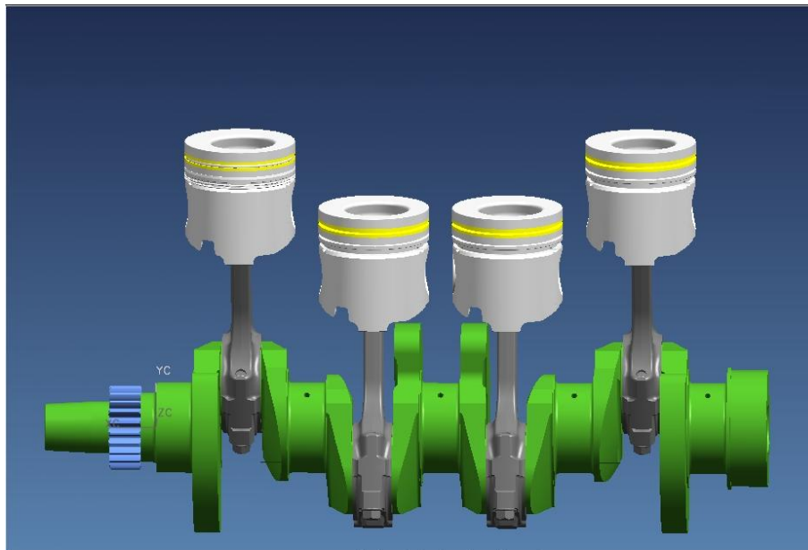
YC4F曲柄连杆机构示
